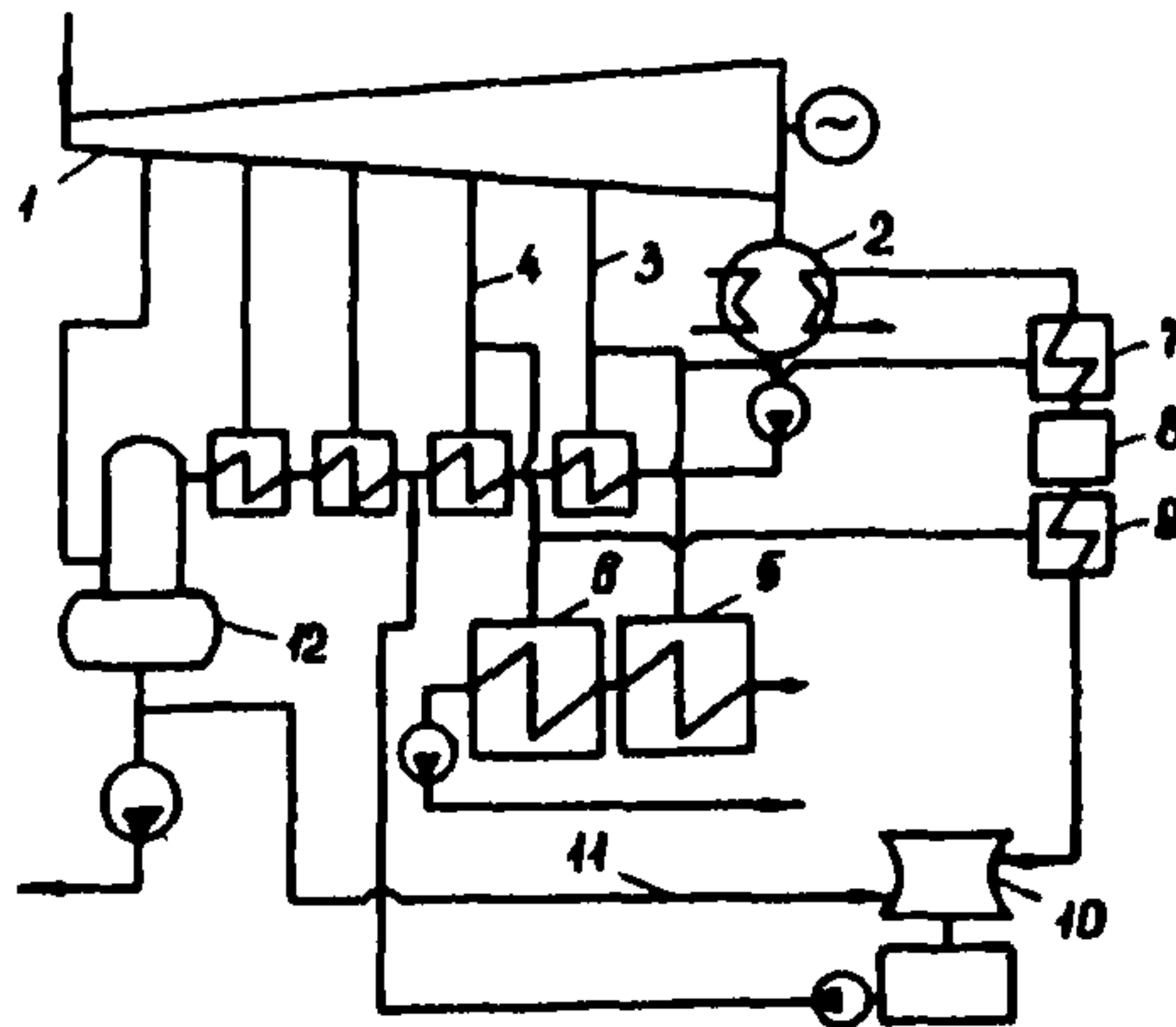
Рис. 5. Схема подогрева исходной воды и греющего агента перед вакуумными деаэраторами в теплофикационной установке с небольшим расходом добавочной питательной воды котлов:
