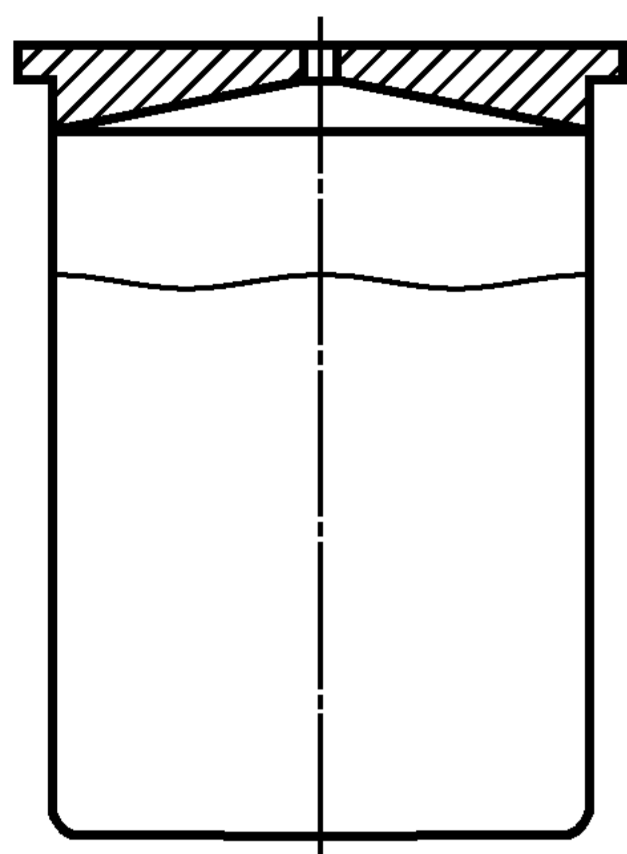
Рисунок 1 — Металлический пикнометр
