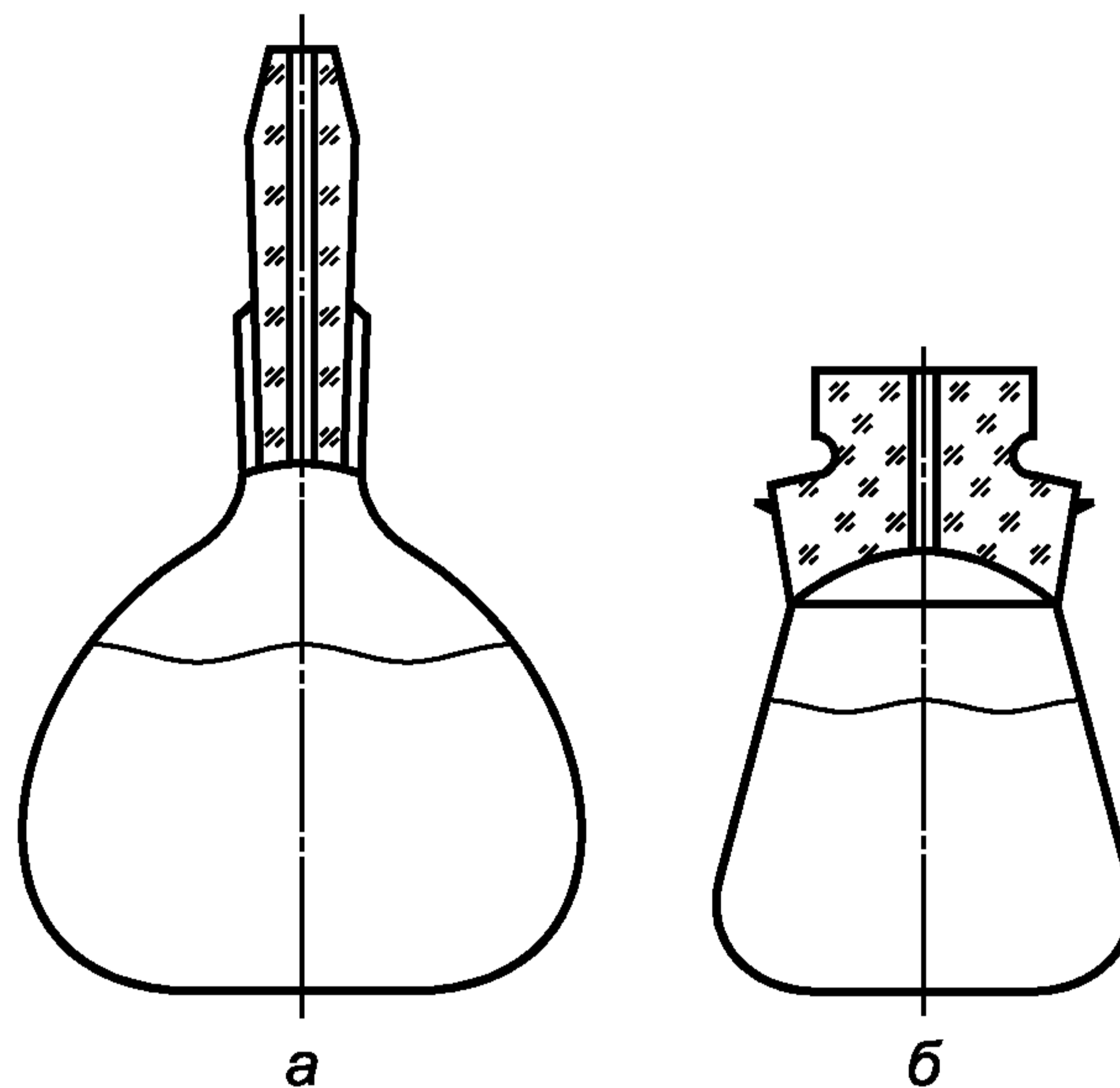
Рисунок 2 — Стекланный пикнометр
