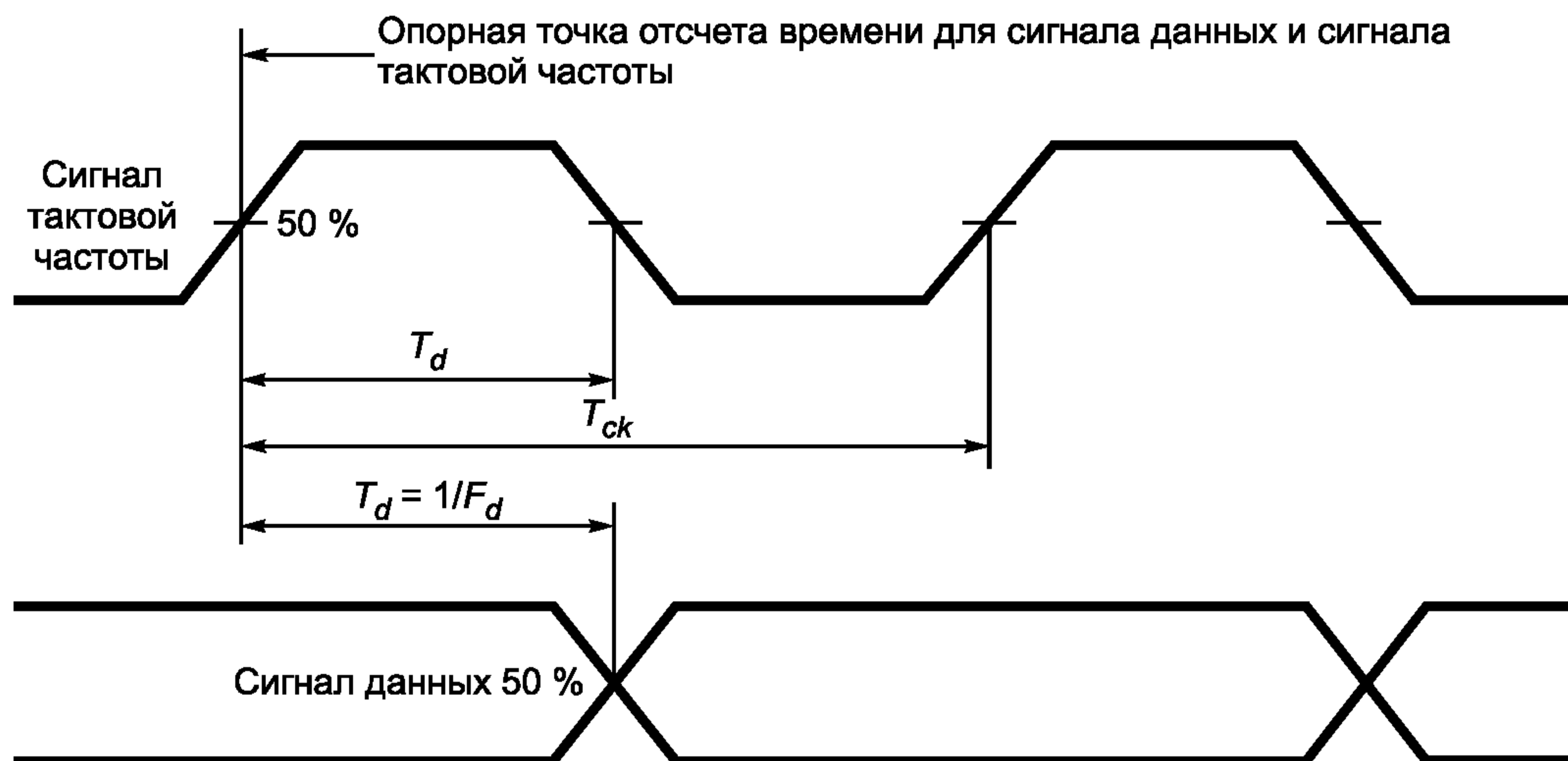
Рисунок 9 — Соотношения параметров синхронизации сигнала и данных
