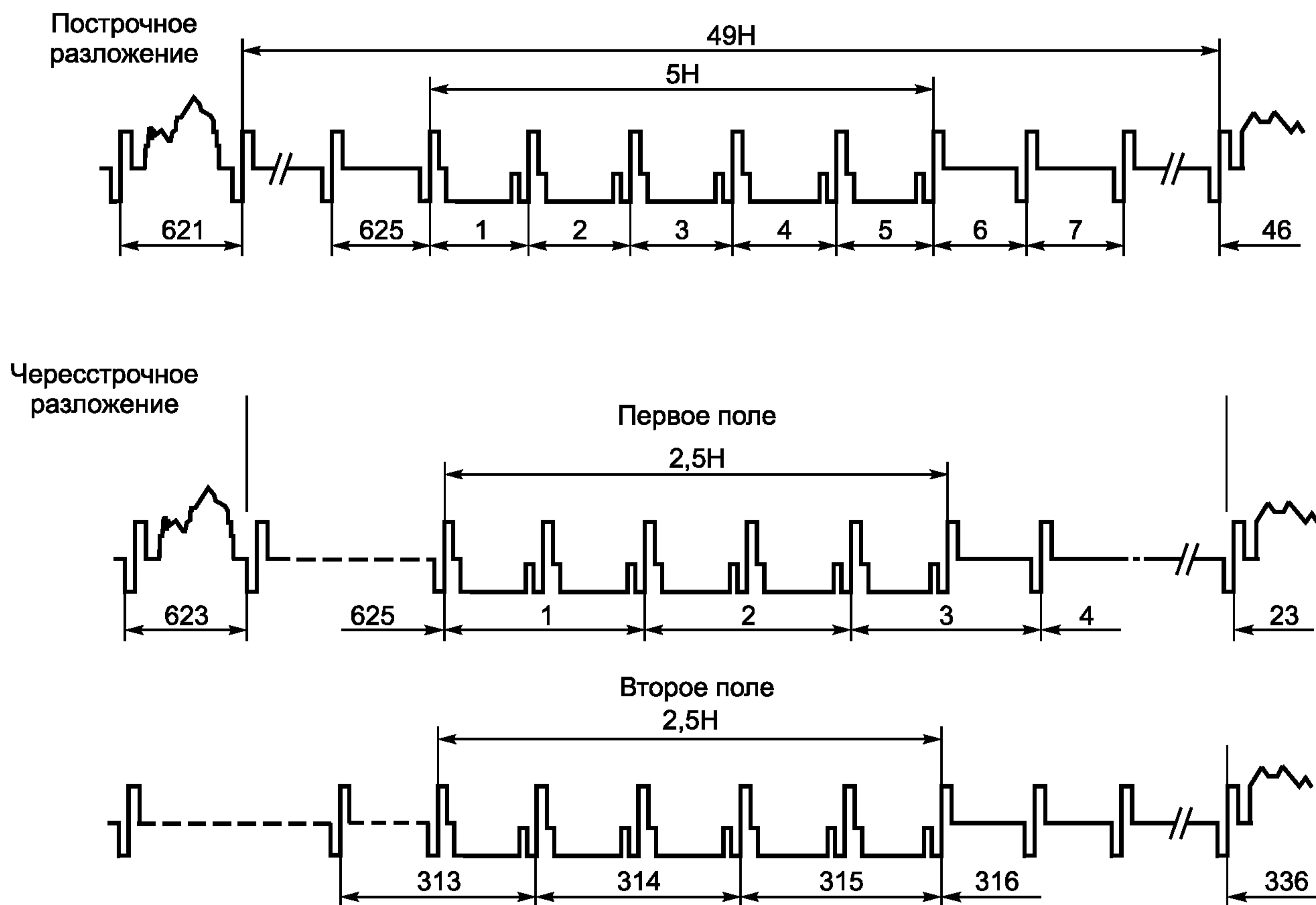
Рисунок 3 — Структура синхросигнала на интервале гашения поля
