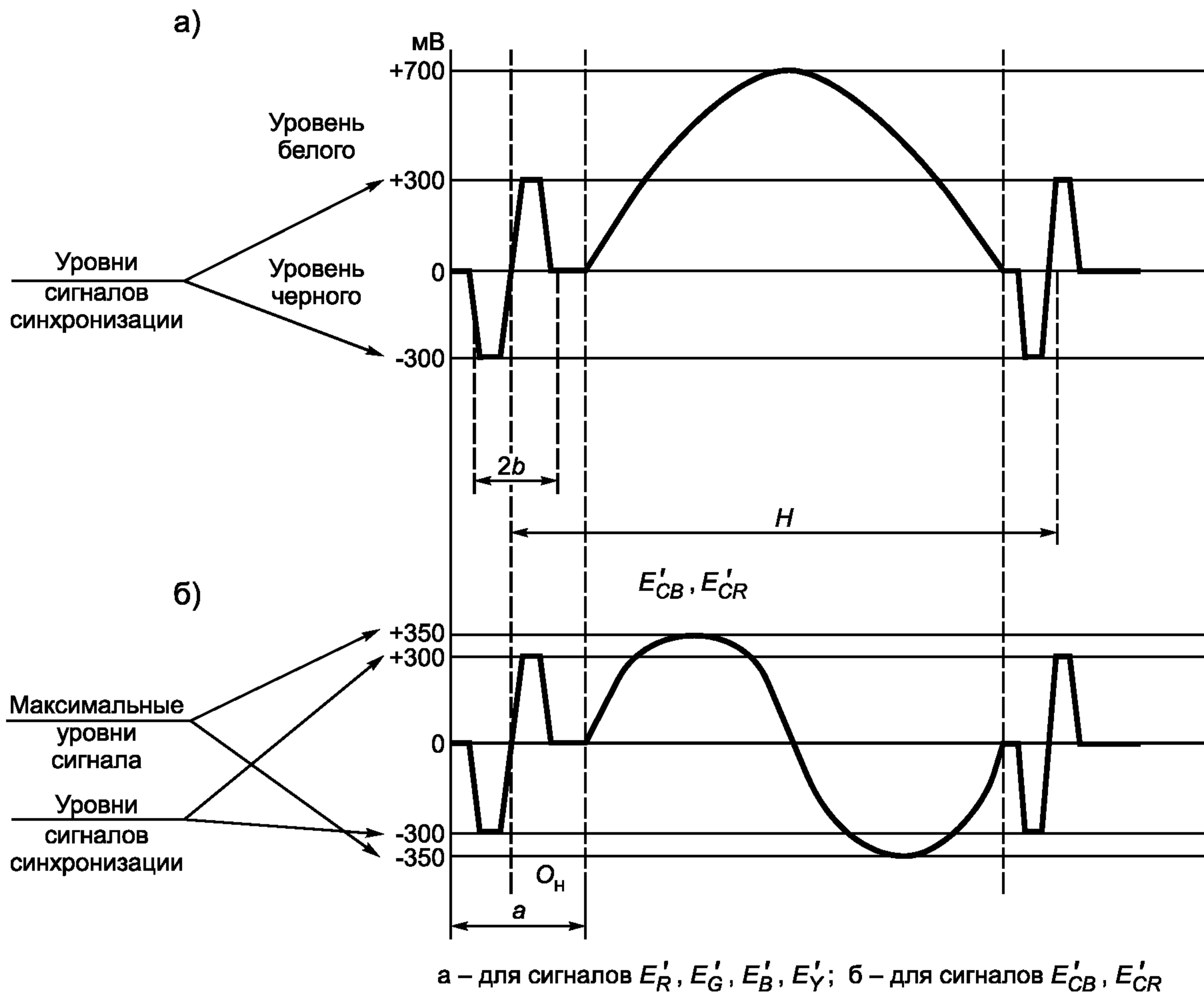
Рисунок 1 — Структура компонентных сигналов на интервале строки
