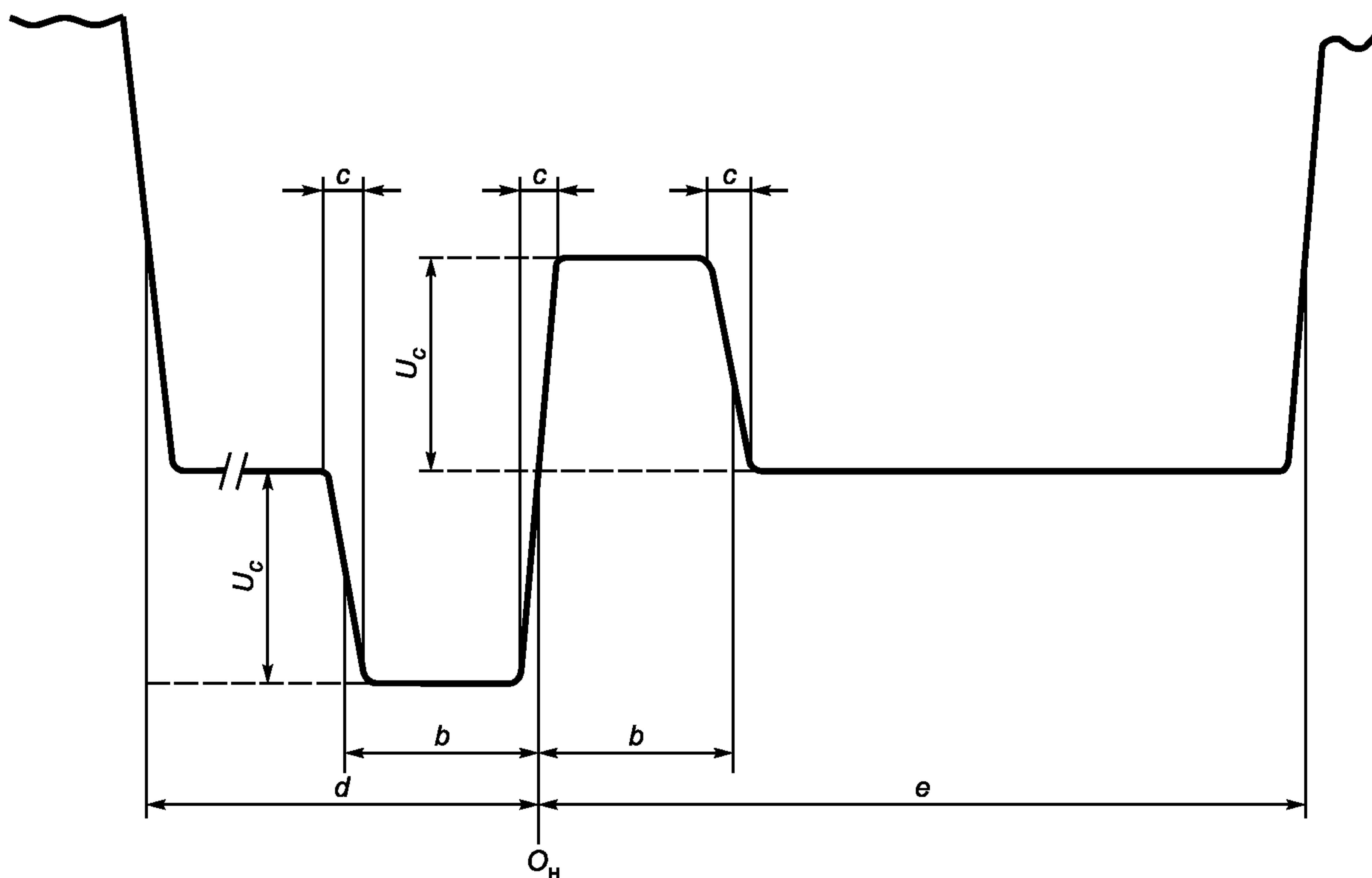
Рисунок 2 — Структура сигнала синхронизации на интервале гашения строки
