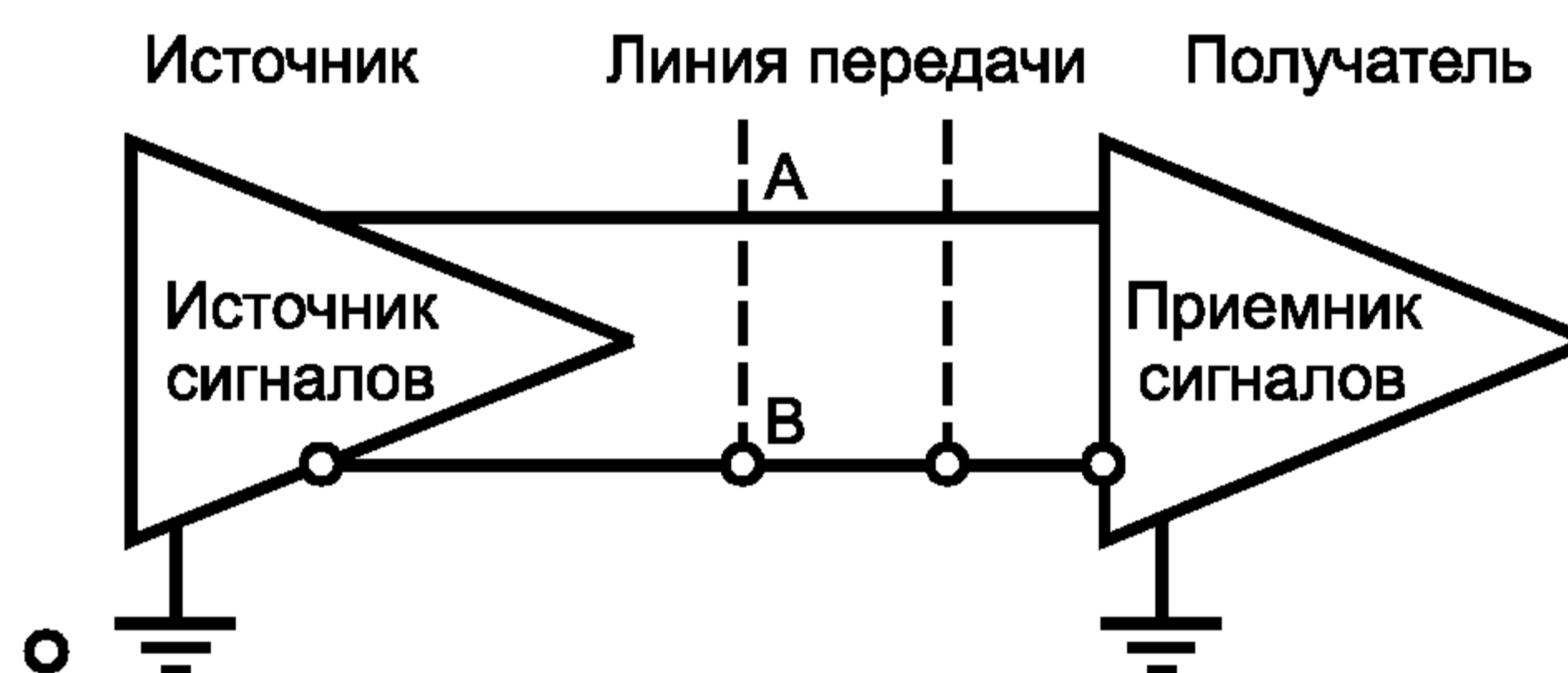
Рисунок 10 — Соединение источника сигналов и приемника сигналов
