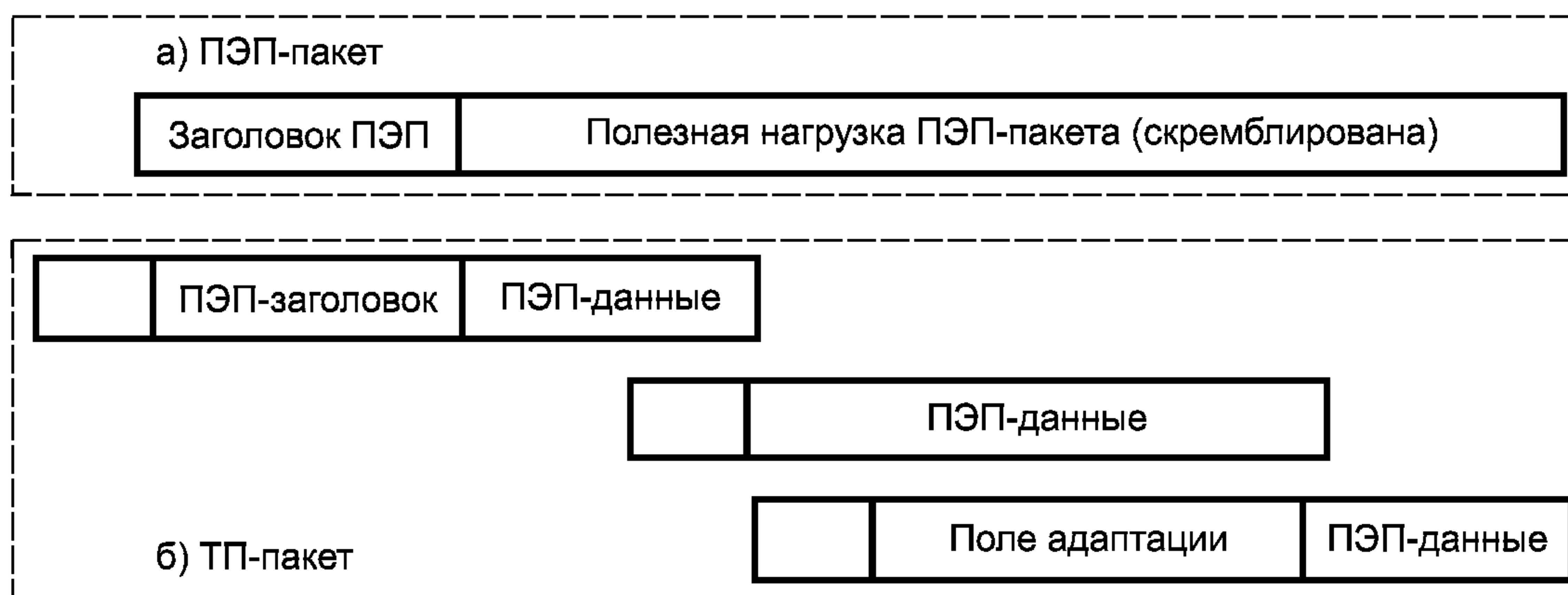
Рисунок Б.1 — Диаграммы скремблирования на уровнях: а) ПЭП-пакета; б) ТП-пакета
