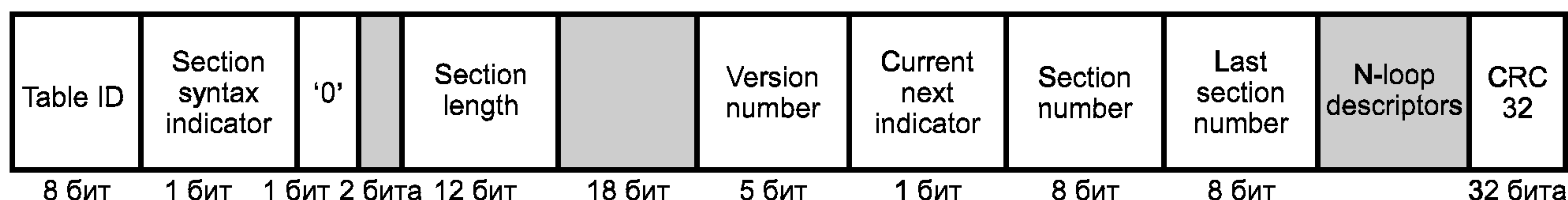
Рисунок А.5 — Диаграмма полей секции таблицы CAT
