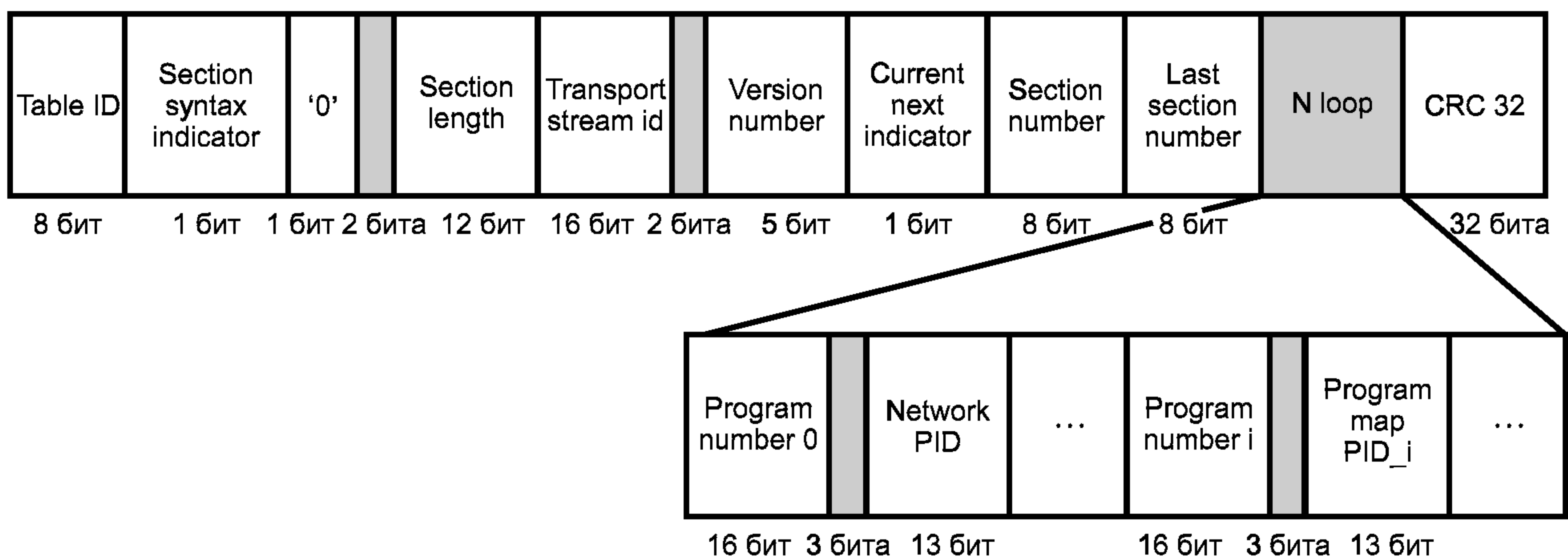
Рисунок А.4 — Диаграмма полей секций таблицы PAT
