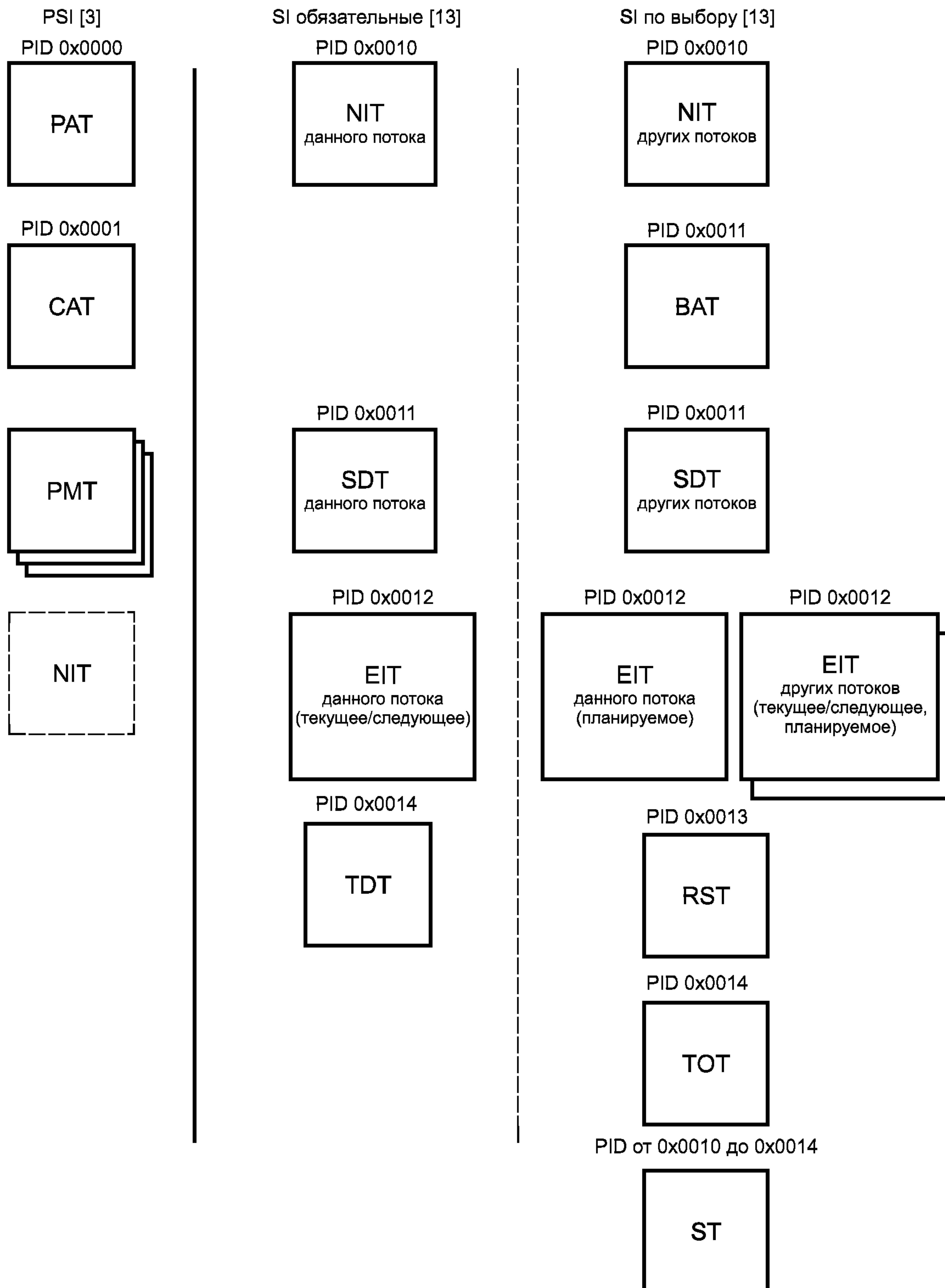
Рисунок А.3 — Полная совокупность таблиц PSI, SI
