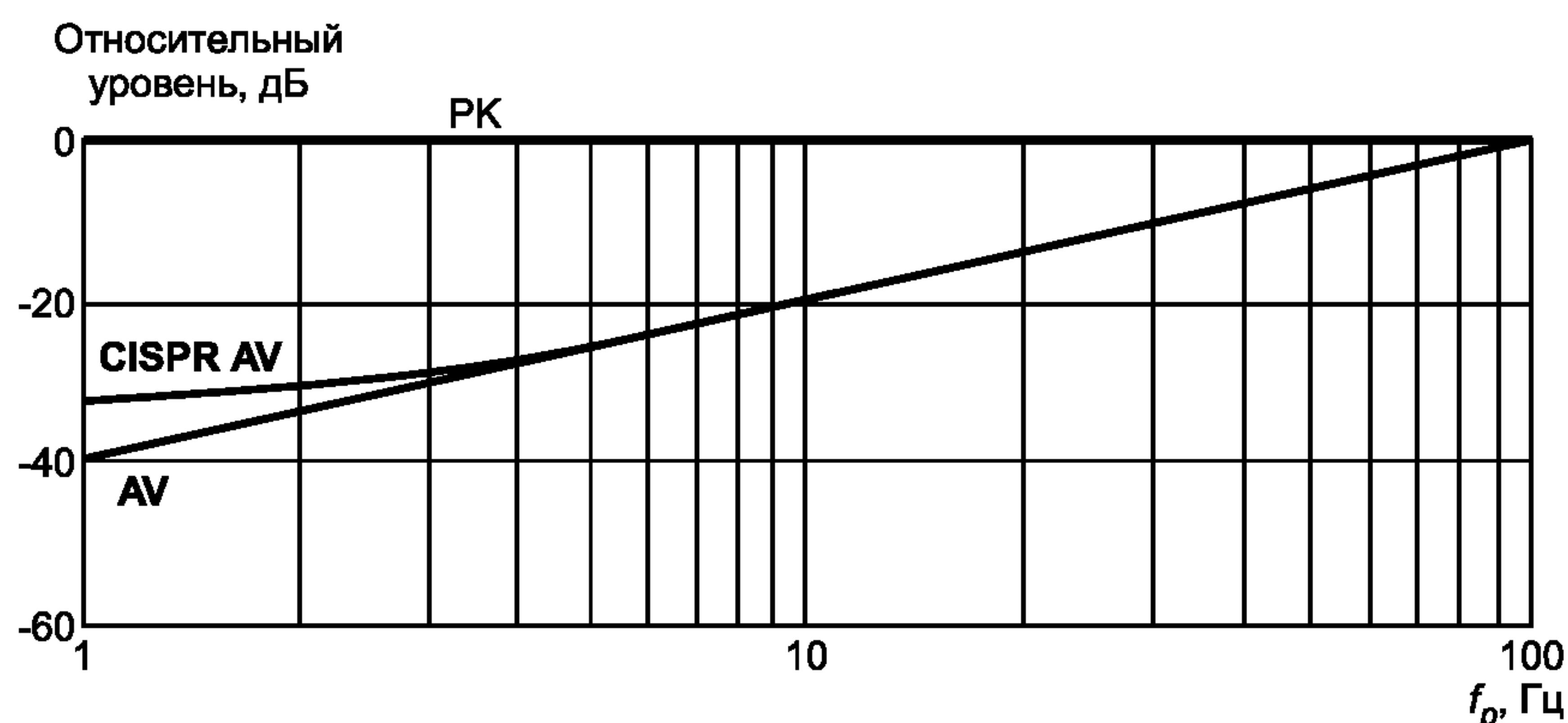
Рисунок С.1 — Весовая функция импульса 10 мс при детектировании пиковым детектором «РК», детектором средних значений при учете пиковых значений «CISPR AV» и детектором средних значений без учета пиковых значений «AV» для постоянной времени прибора 160 мс
