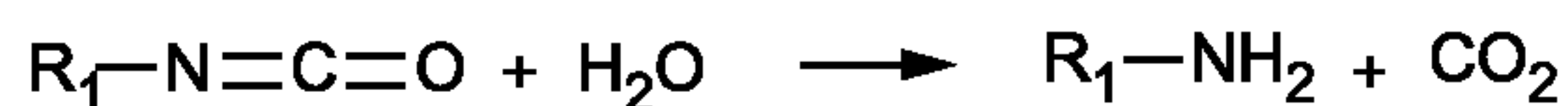
Рисунок 1 — Реакции изоцианатов
