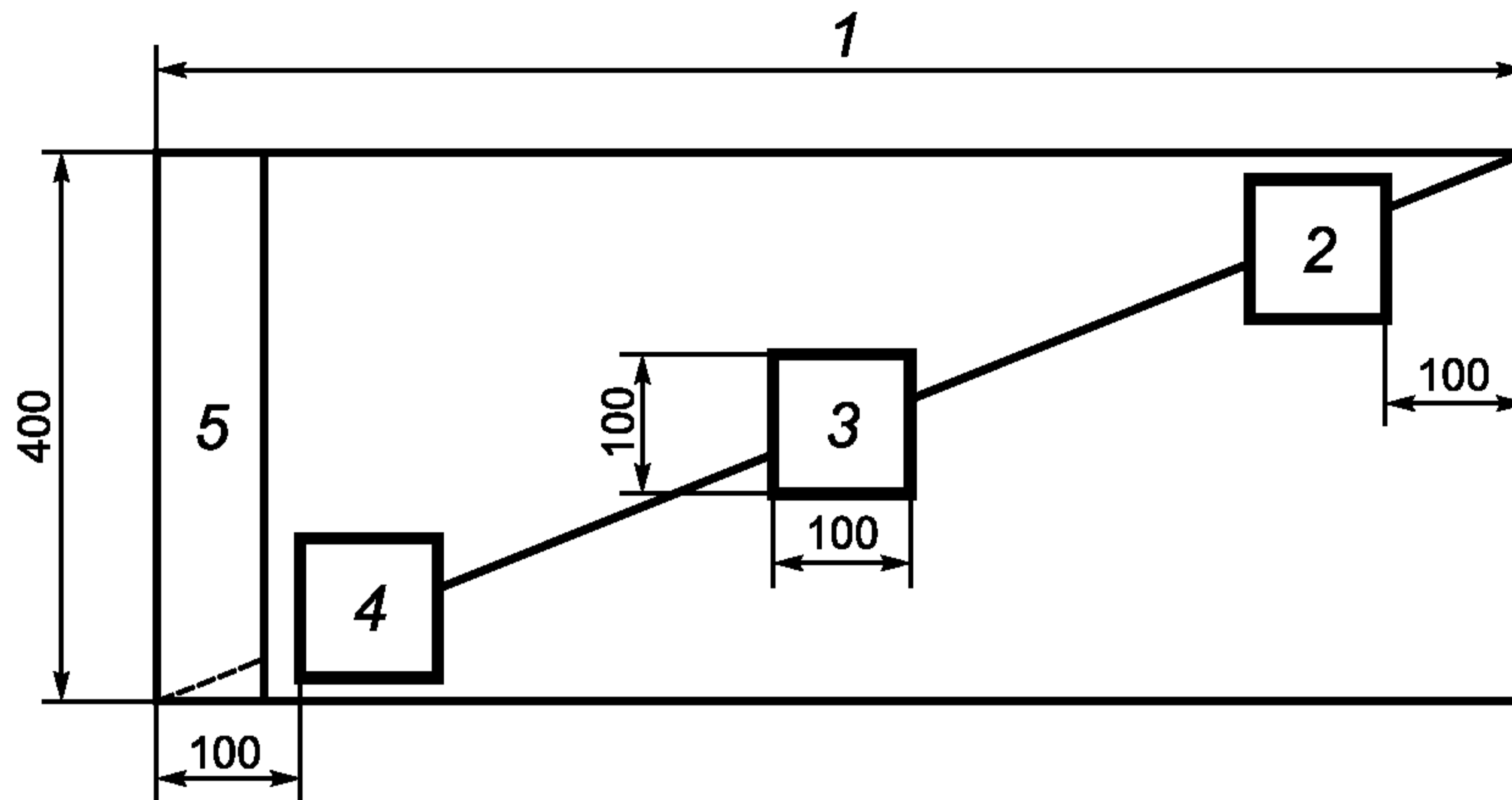
1 — ширина полотна материала; 2, 3, 4 — образцы; 5 — кромка
