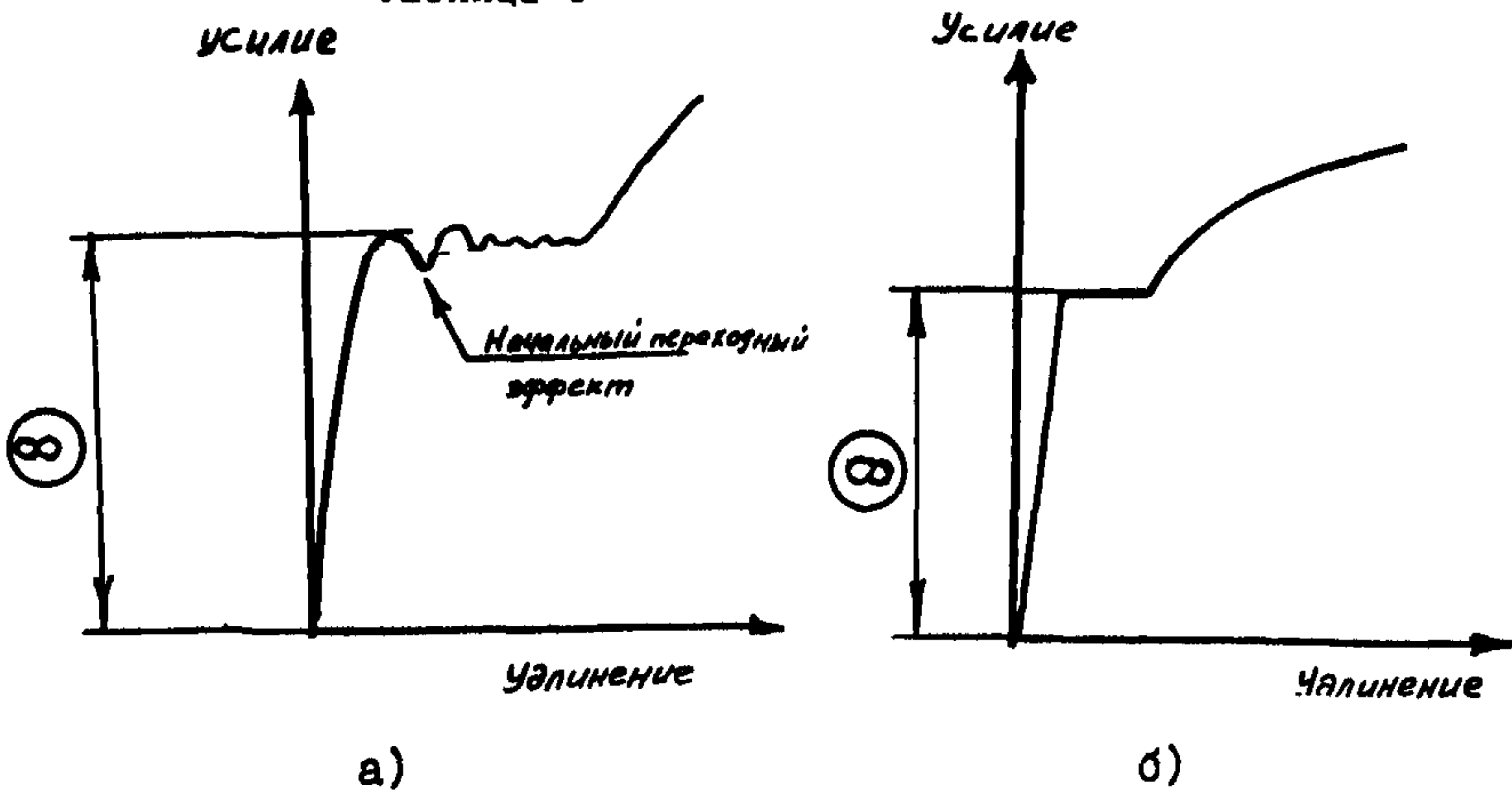
Рисунок 1 - Схема определения относительного удлинения \delta_p, \delta_b Примечание - Пояснения к номерам, заключенным в круг, см. в таблице 1
