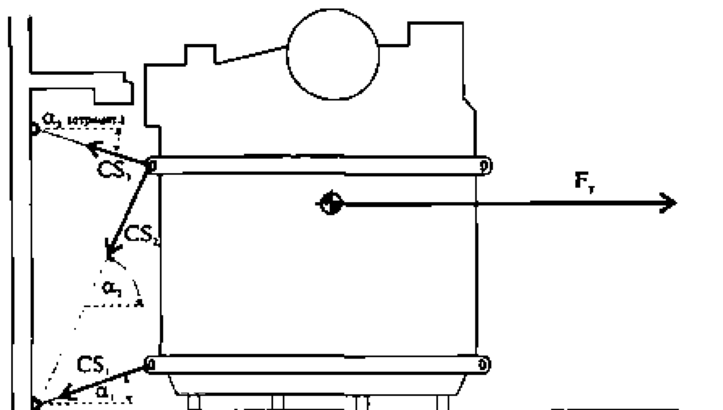
Рис. 1 Равенство поперечных сил
