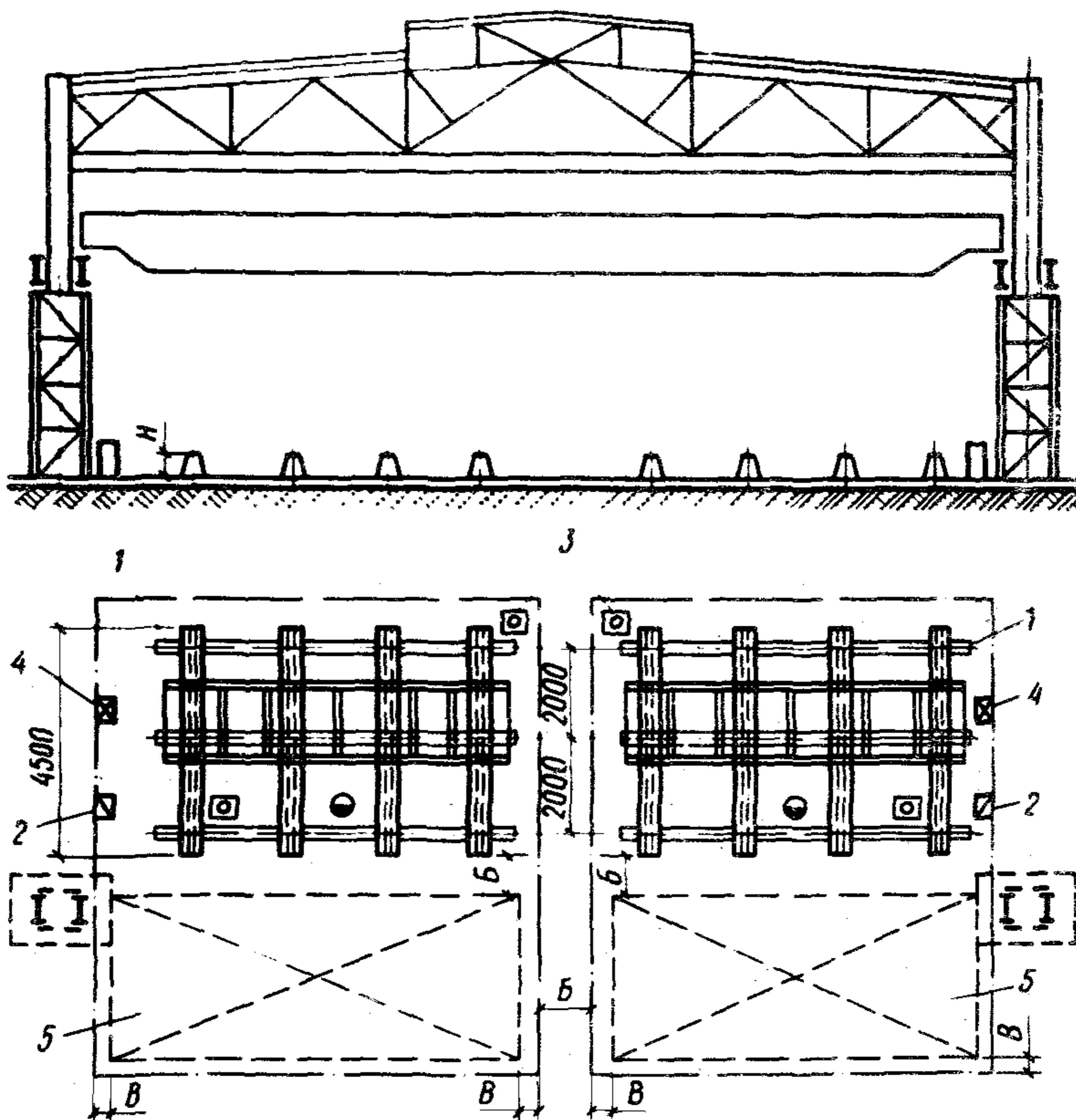
Рис. 38. Размещение стенда для сварки из козелков в поперечном пролете 1 – козелок; 2 – ящик для инструмента; 3 – полуавтомат сварочный; 4 – источник питания; 5 – место складирования; B = 800 \text{ мм} , B = 500 \text{ мм}
