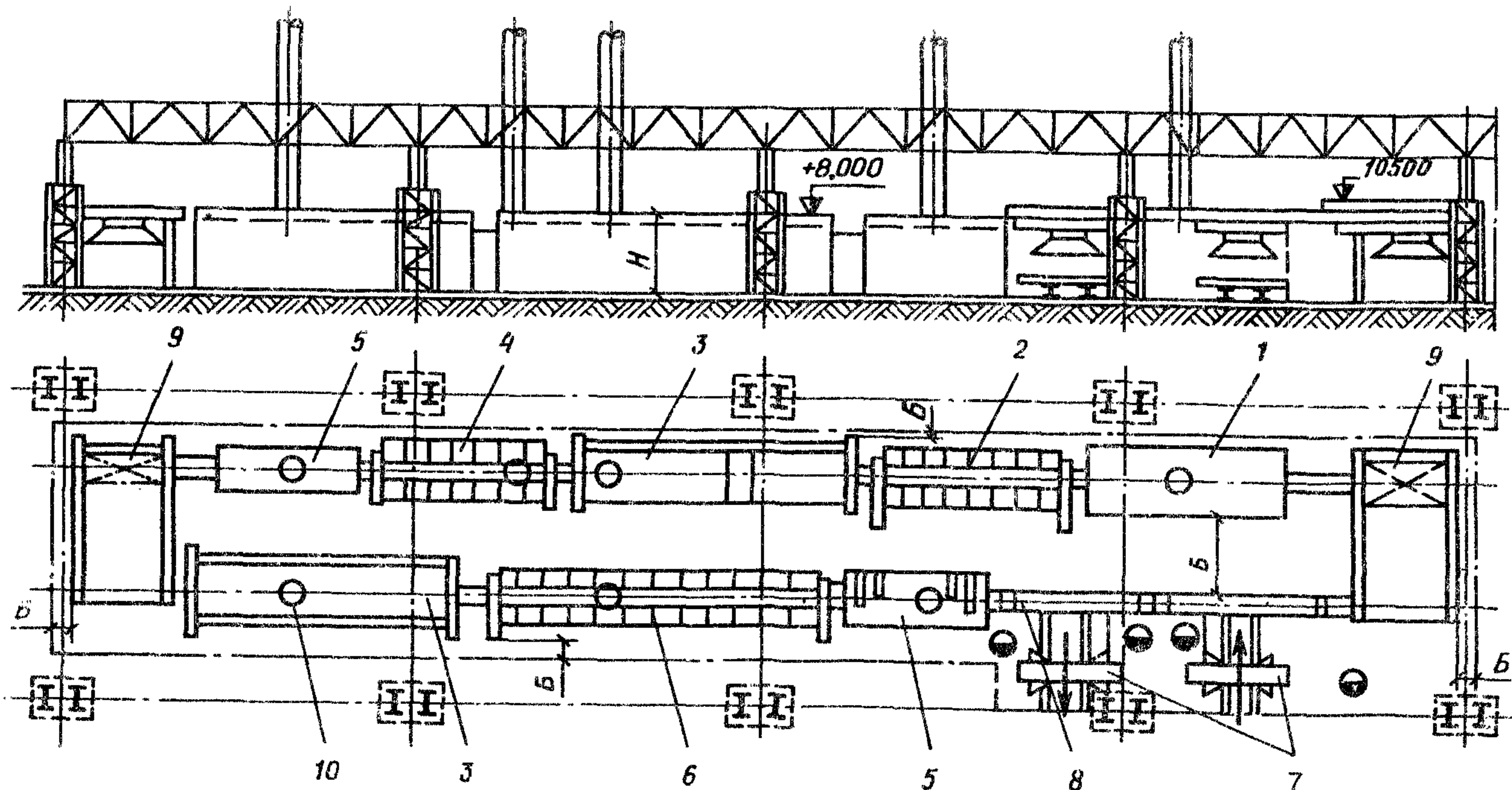
Рис. 40. Размещение поточной линии окраски конструкций методом облива длиной до 12 м
