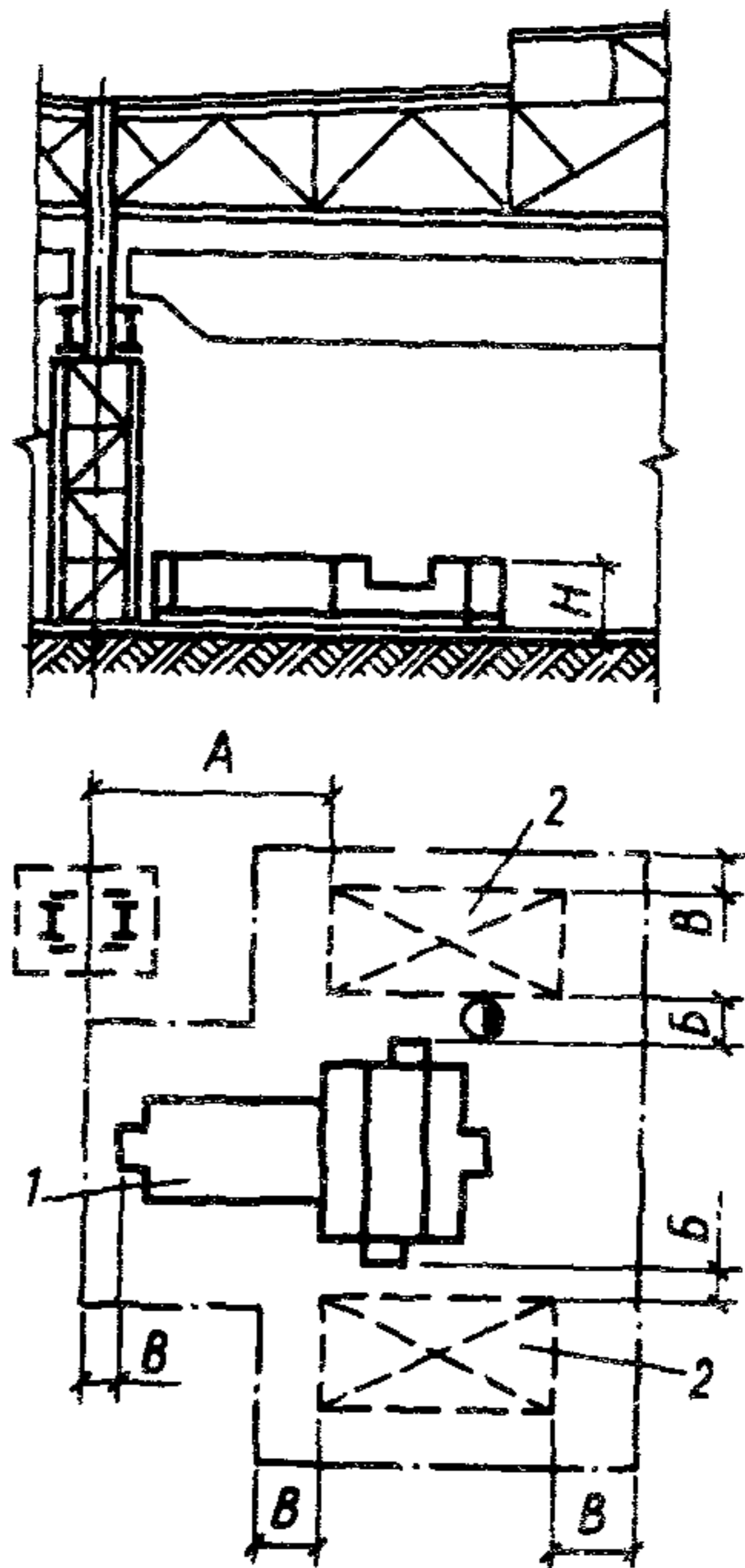
Рис.17. Размещение поперечно-строгального станка в поперечном пролете 1 – станок поперечно-строгальный; 2 – место складирования; А – принимается в зависимости от грузоподъемности мостового крана; Б=800 мм, В=500 мм
