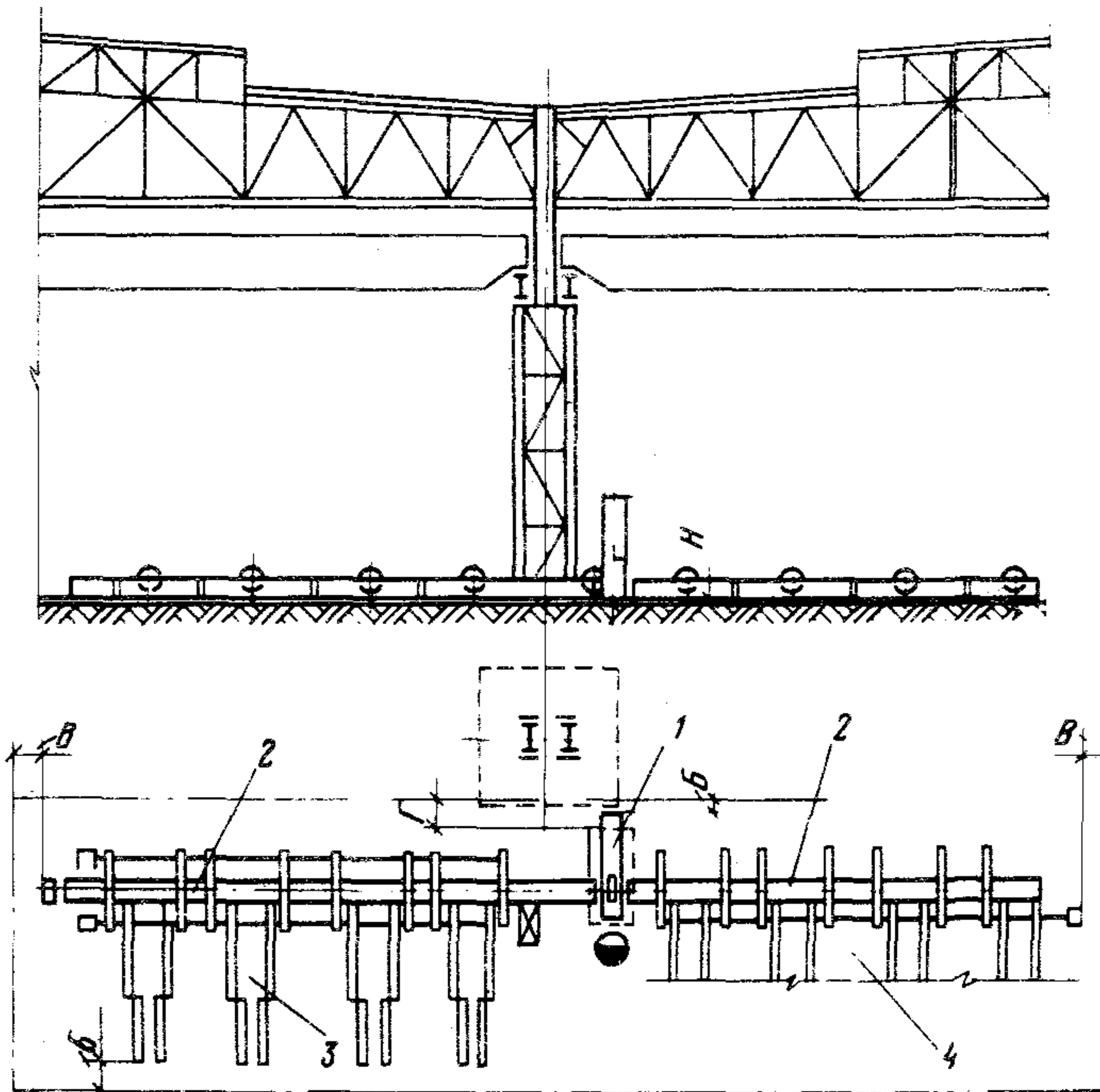
Рис.13. Размещение ножниц для резки профильного проката в поточной линии 1 – ножницы; 2 – рольганг; 3 – стеллаж для проката; 4 – накопитель; B=800 мм, V=500 мм, \Gamma=200 мм
