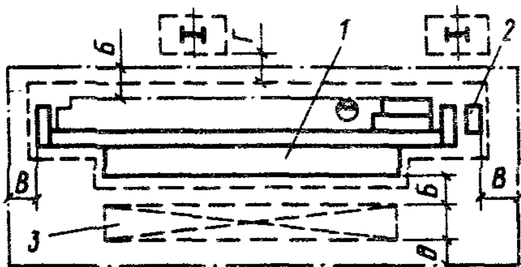
Рис.15. Размещение кромкострогального станка в продольном пролете
