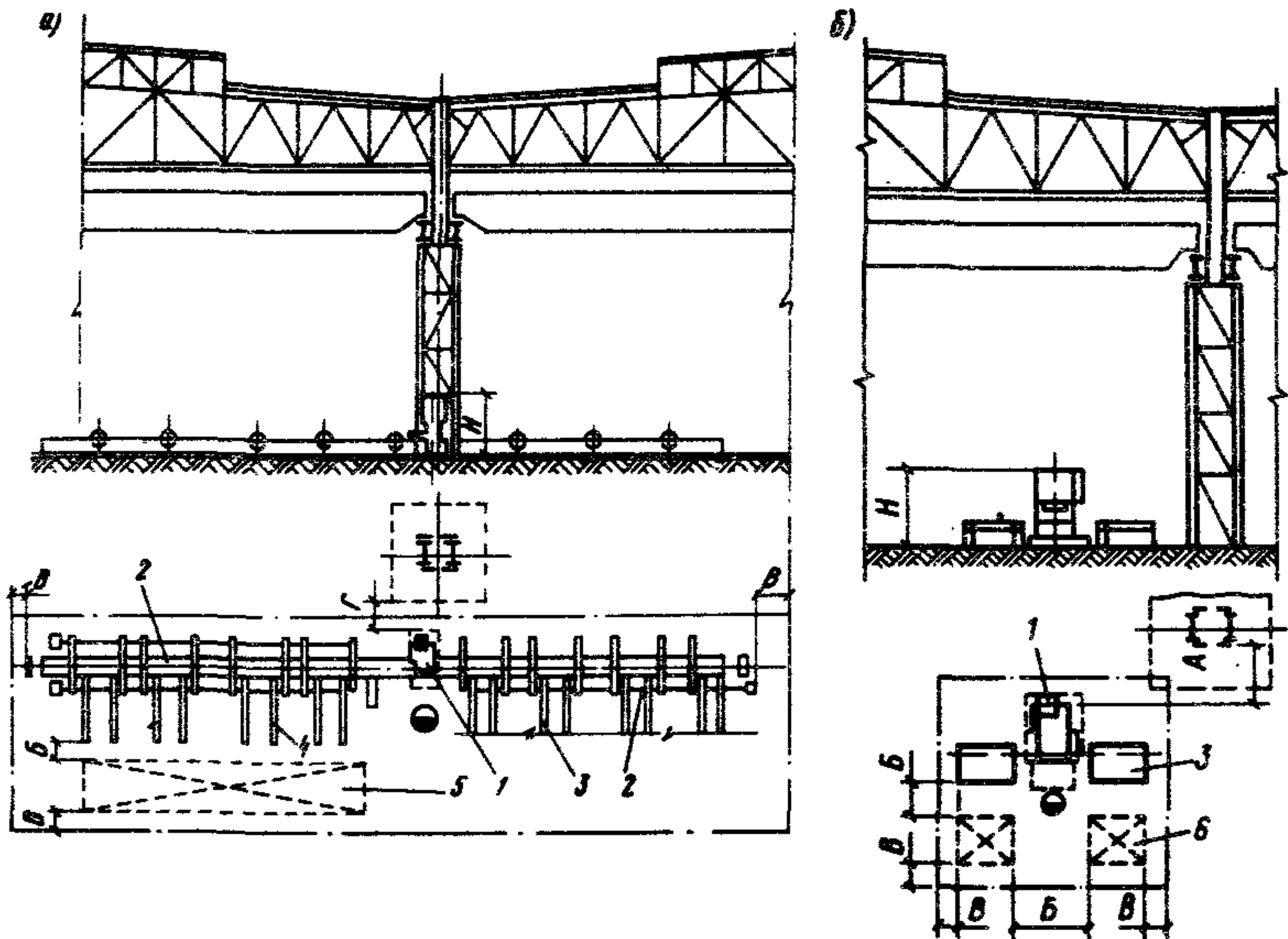
Рис.11. Размещение дыропробивного пресса в поточной линии (а), вне поточной линии (б) 1 – пресс; 2 – рольганг; 3 – стол; 4 – транспортер поперечный; 5 – сбрасыватель; 6 – место складирования; A=400 мм, B=800 мм, B=500 мм, \Gamma=200 мм
