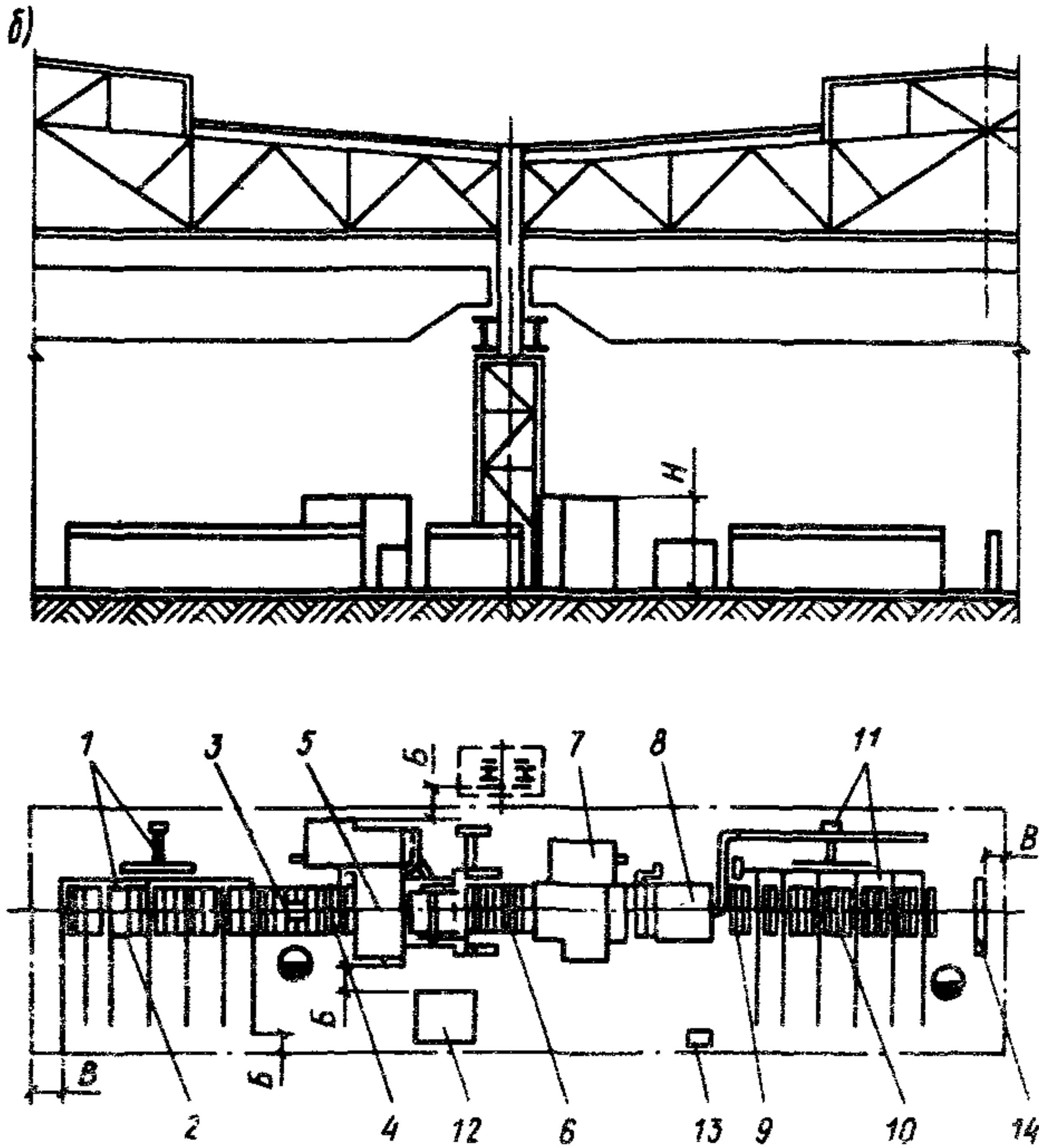
Рис. 23. Размещение поточной линии дробеметной очистки сортового и листового проката без окрасочной и сушильной камер (а), с окрасочной и сушильной камерами (б)
