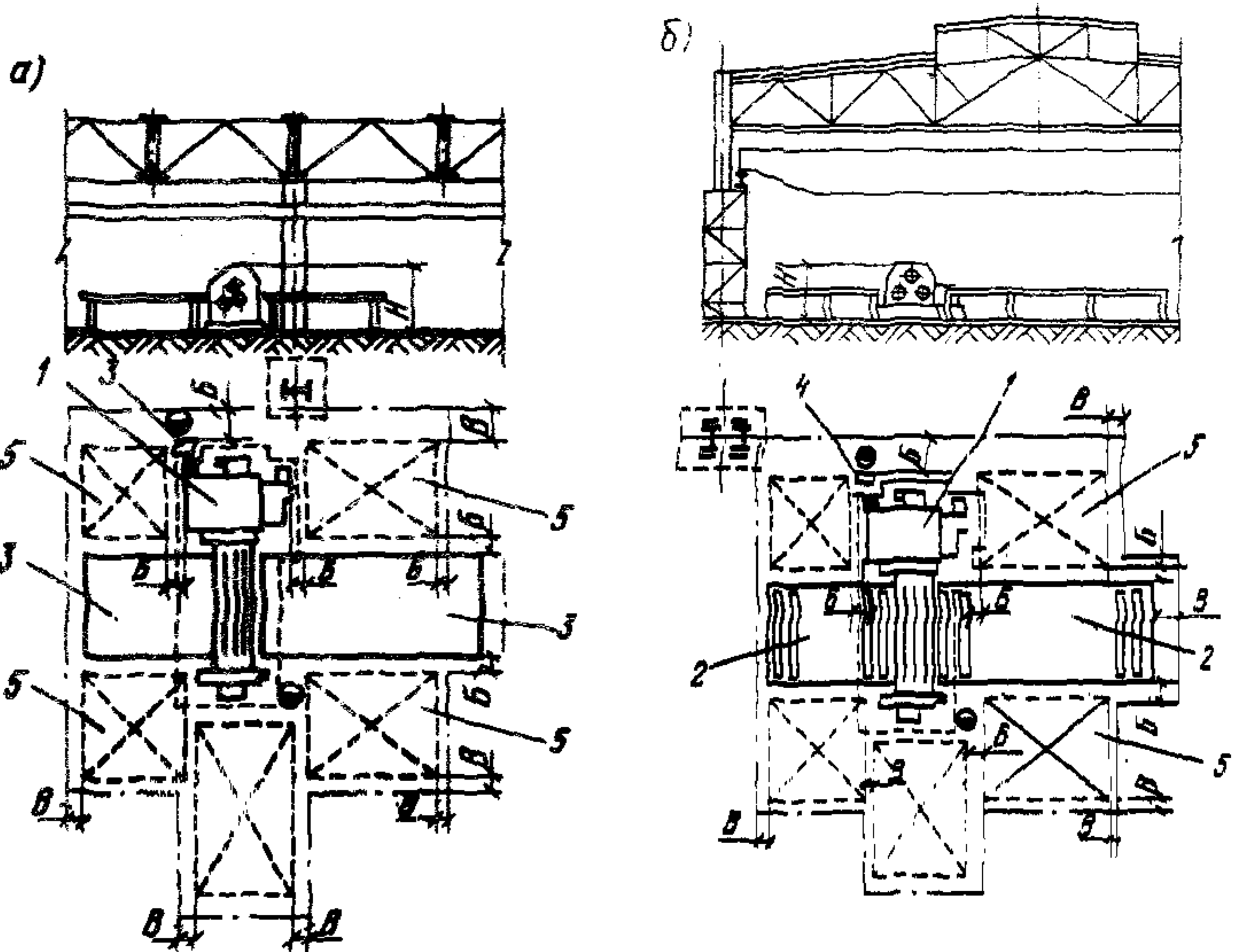
Рис.4. Размещение листогибочной машины в продольном пролете (а), в поперечном пролете (б) 1 - машина; 2 - рольганг; 3 - стол; 4 - пульт управления; 5 - место складирования; A=400 мм, B=800 мм, V=500 мм
