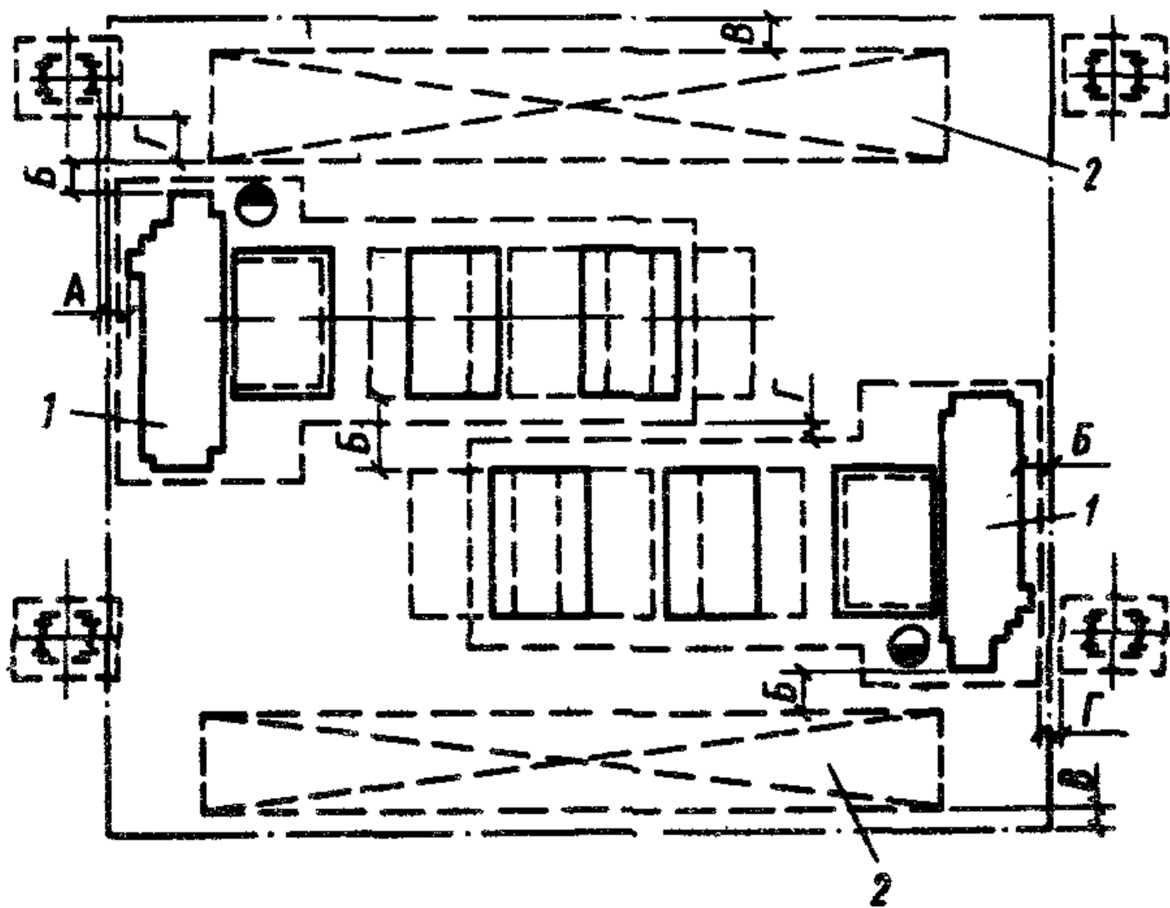
Рис. 28. Размещение двух торцефрезерных станков модели ИР-198 на одной площадке 1 – станок; 2 – место складирования; А – принимается в зависимости от грузоподъемности мостового крана, Б=800 мм, В=500 мм, Г=200 мм
