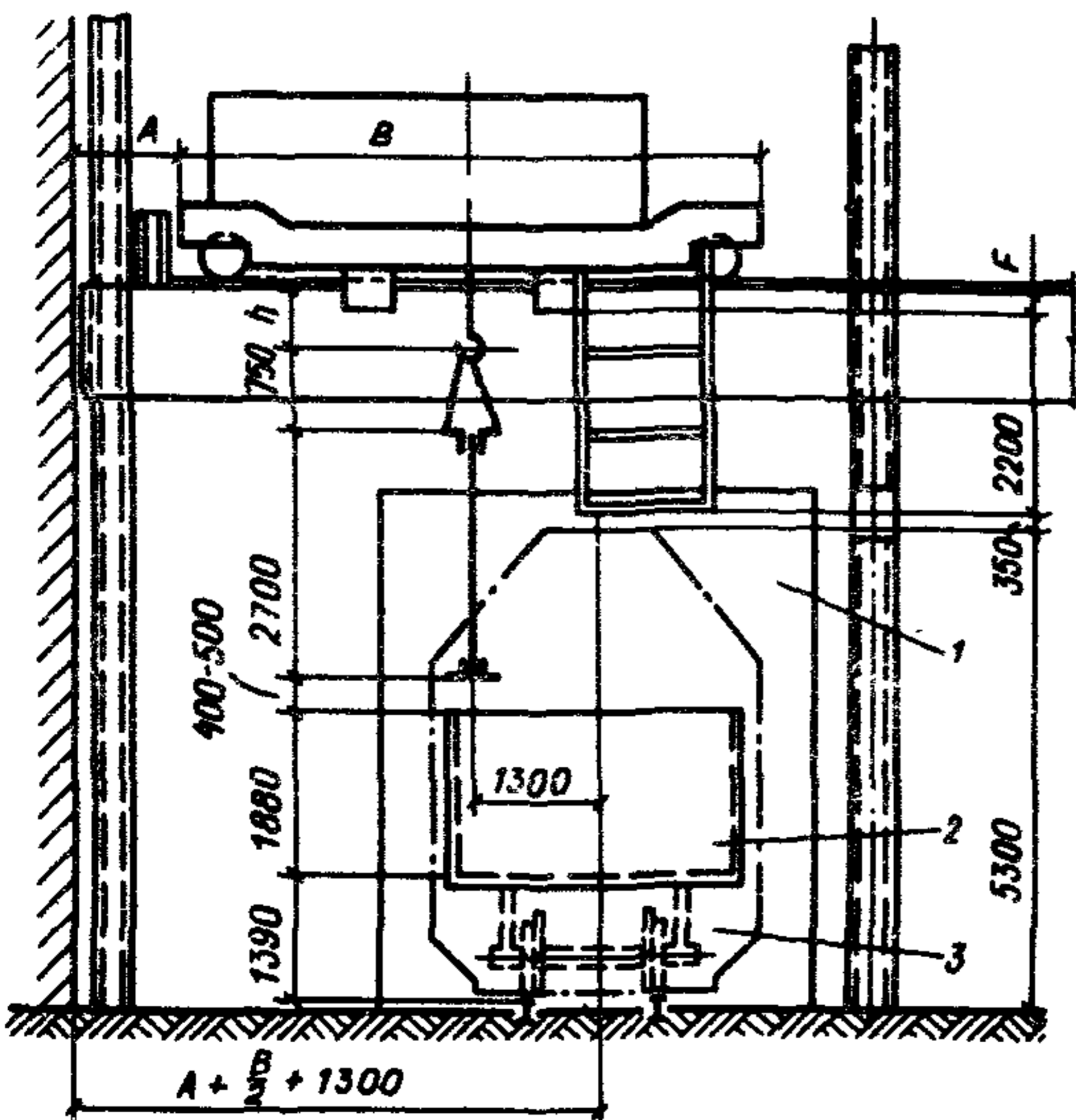
Рис. 44. Схема размещения мостового крана и габариты железнодорожного транспорта 1 – ворота (4700 x 5600 мм); 2 – платформа; 3 – габарит подвижного железнодорожного состава
