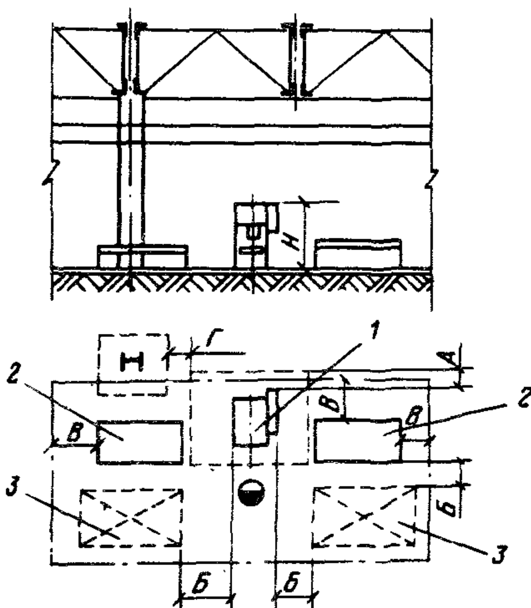
Рис. 9. Размещение прессы однокривошипного простого действия в продольном пролете 1 – пресс; 2 – стол к прессу; 3 – место складирования, A = 400 мм, B = 800 мм, B = 500 мм, \Gamma = 200 мм
