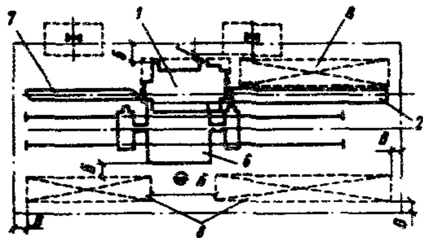
Рис.14. Размещение гильотинных ножниц при поперечной резке листа (а), при продольной резке листа (б)
