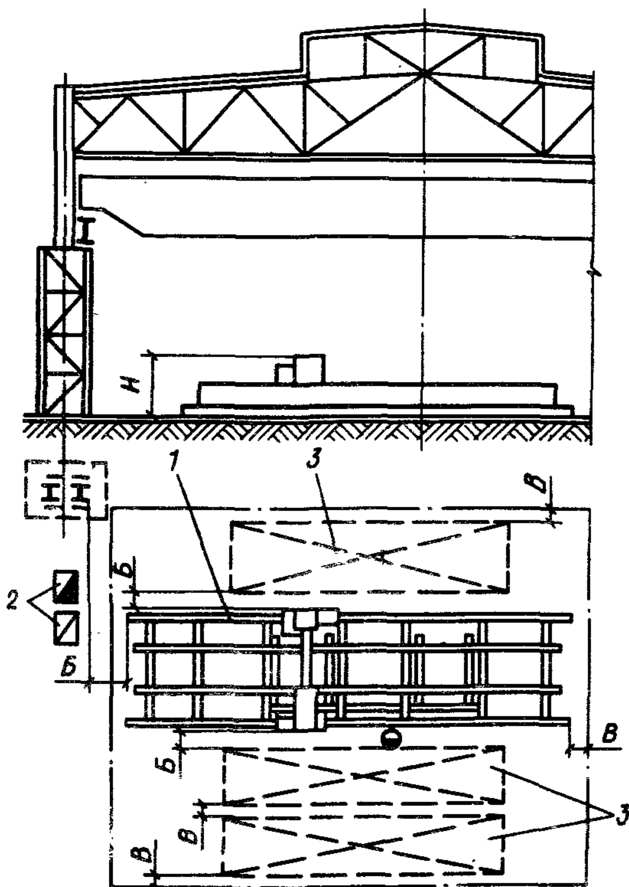
Рис. 37. Размещение установки с пневматическими прижимами для сборки двутавровых стержней высотой до 2500 м в поперечном пролете 1 – установка для сборки стержней; 2 – оборудование сварочное; 3 – место складирования; B=800 мм, V=500 мм
