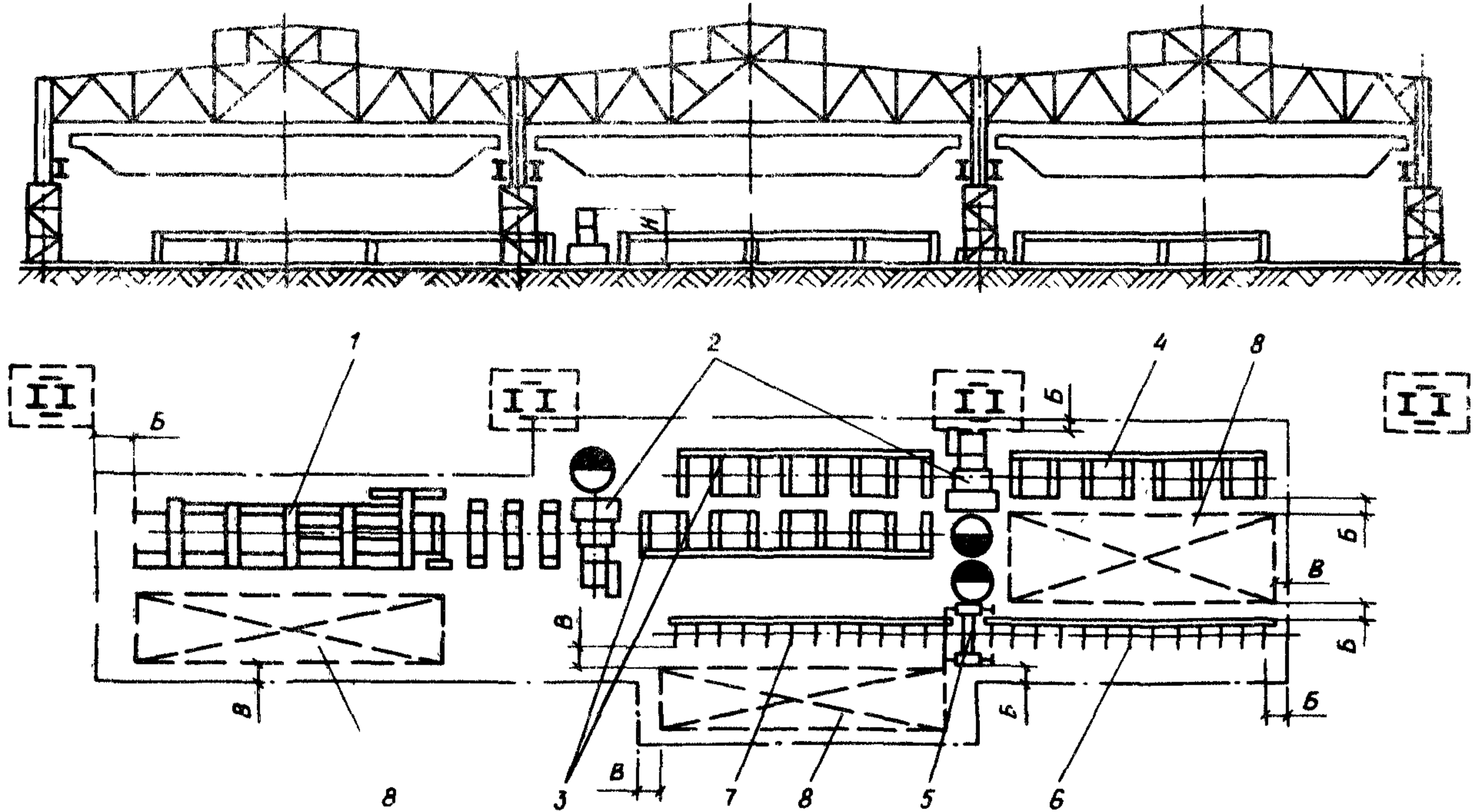
Рис. 32. Размещение поточной линии сборки, сварки и резки стержней двутаврового сечения. 1 – стол для сборки стержней; 2 – агрегат сварочный; 3 – рольганг и кантователь; 4 – рольганг конечный; 5 – машина для кислородной резки трехрезаковая; 6 – рольганг подающий; 7 – рольганг приемный; 8 – место складирования; B=800 мм, B=500 мм
