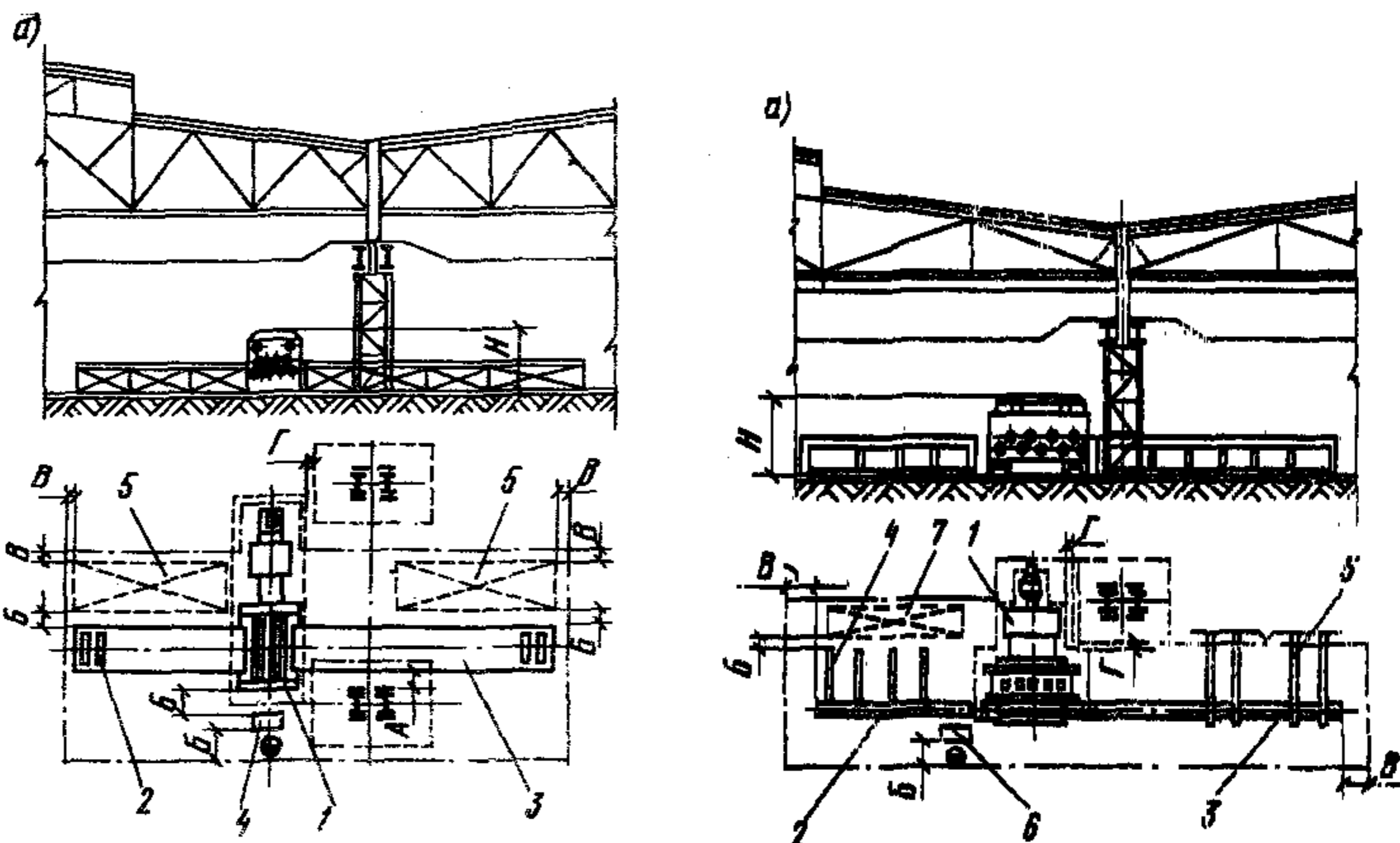
Рис. 1. Размещение листопрямильной машины вне поточной линии (а), в поточной линии (б) 1 - вальцы; 2 - рольганг подающий; 3 - рольганг приемный; 4 - пульт управления; 5 - место складирования; 6 - укладчик магнитный; А = 400 мм, Б = 800 мм, В = 500 мм, Г = 200 мм
