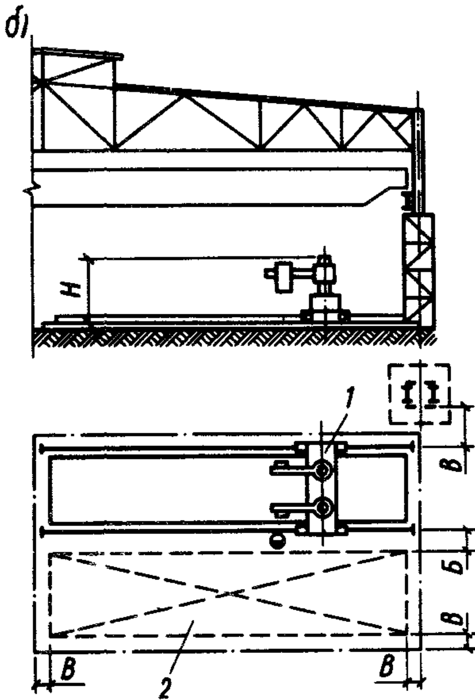
Рис. 29. Размещение в поперечном пролете радиально-сверлильного станка модели 2Р-53 (а), модели ИР-111 (б) 1 – станок; 2 – стеллаж; 3 – место складирования; B=800 мм, B=500 мм
