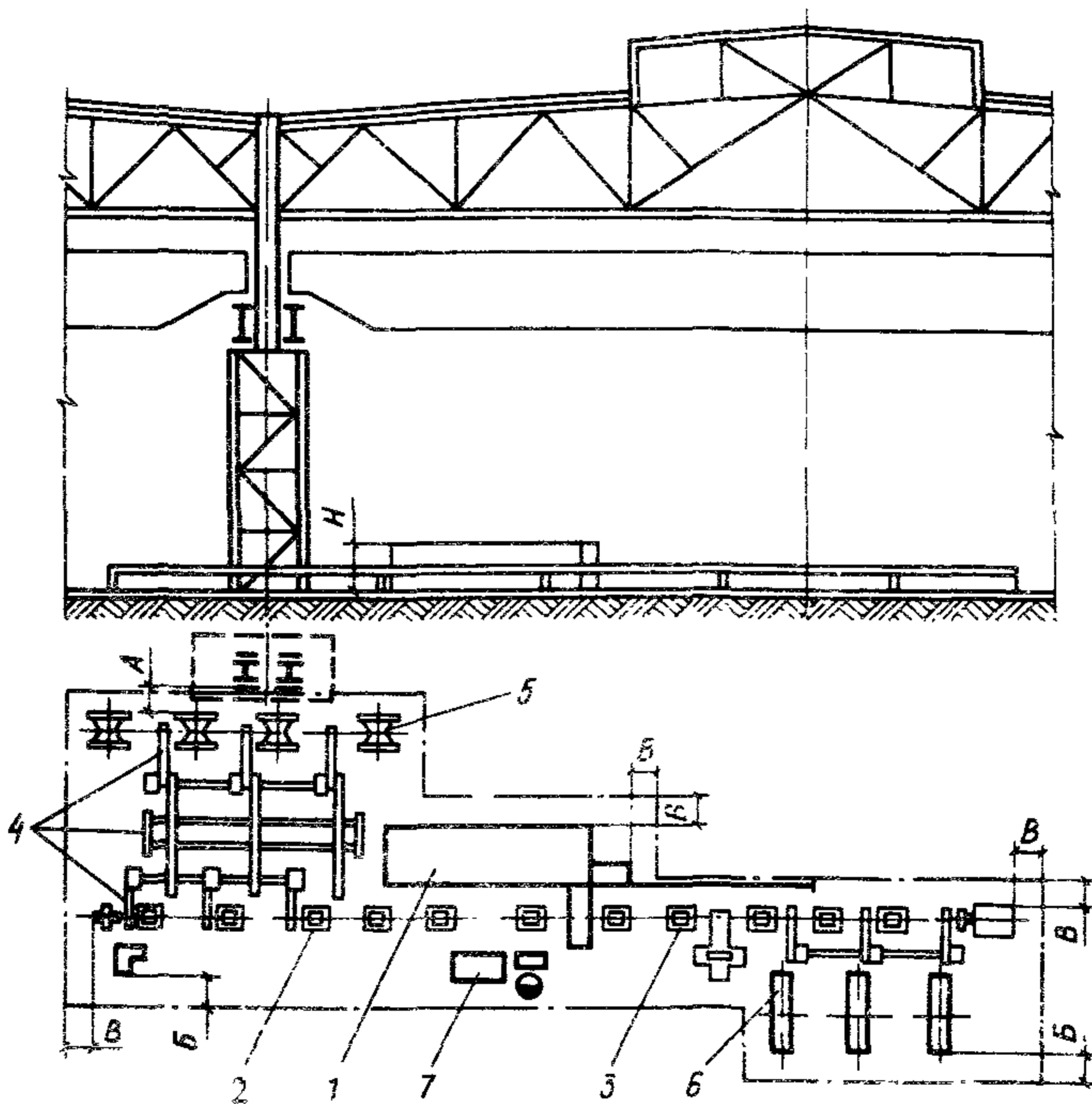
Рис.22. Размещение автомата фирмы "Пайком" для газовой фасонной резки труб в поточной линии 1 – машина; 2 – рольганг подающий; 3 – рольганг приемный; 4 – устройство для укладки труб; 5 – рольганг промежуточный; 6 – стеллаж; 7 – электрошкафы управления; A = 400 мм, B = 800 мм, V = 500 мм
