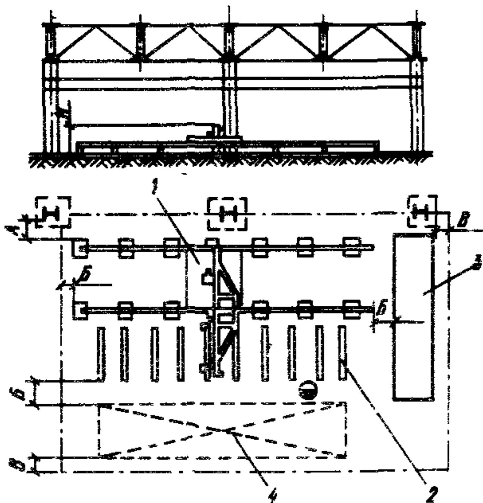
Рис.21. Размещение машин портально-консольного типа для кислородной резки стали в продольном пролете 1 – машина; 2 – стол к машине; 3 – стеллаж для шаблонов; 4 – место складирования; A = 400 мм, B = 800 мм, V = 500 мм
