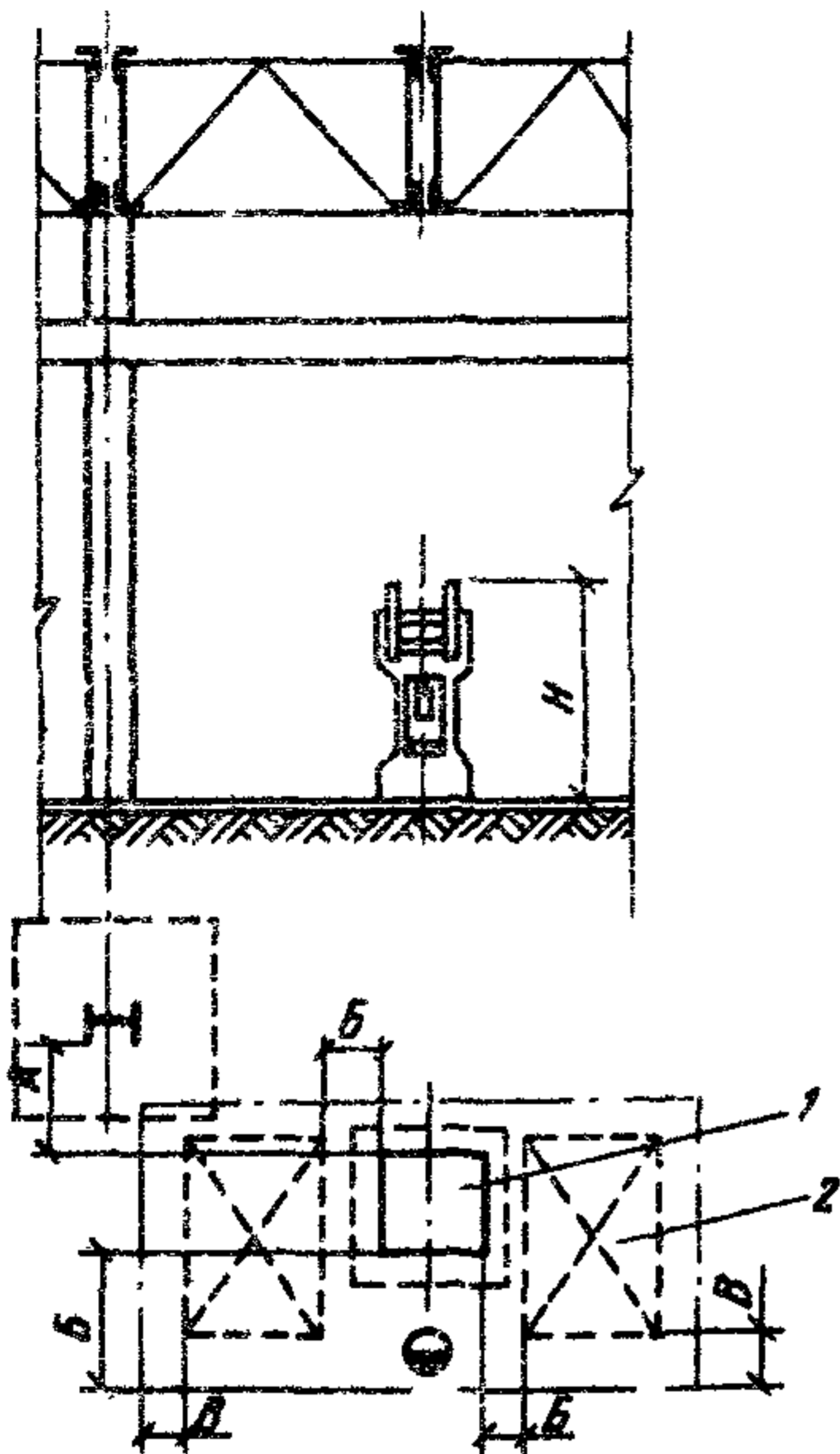
Рис.10. Размещение винтового пресса в продольном пролете 1 – пресс; 2 – место складирования, А – принимается в зависимости от грузоподъемности крана; Б = 800 мм, В = 500 мм
