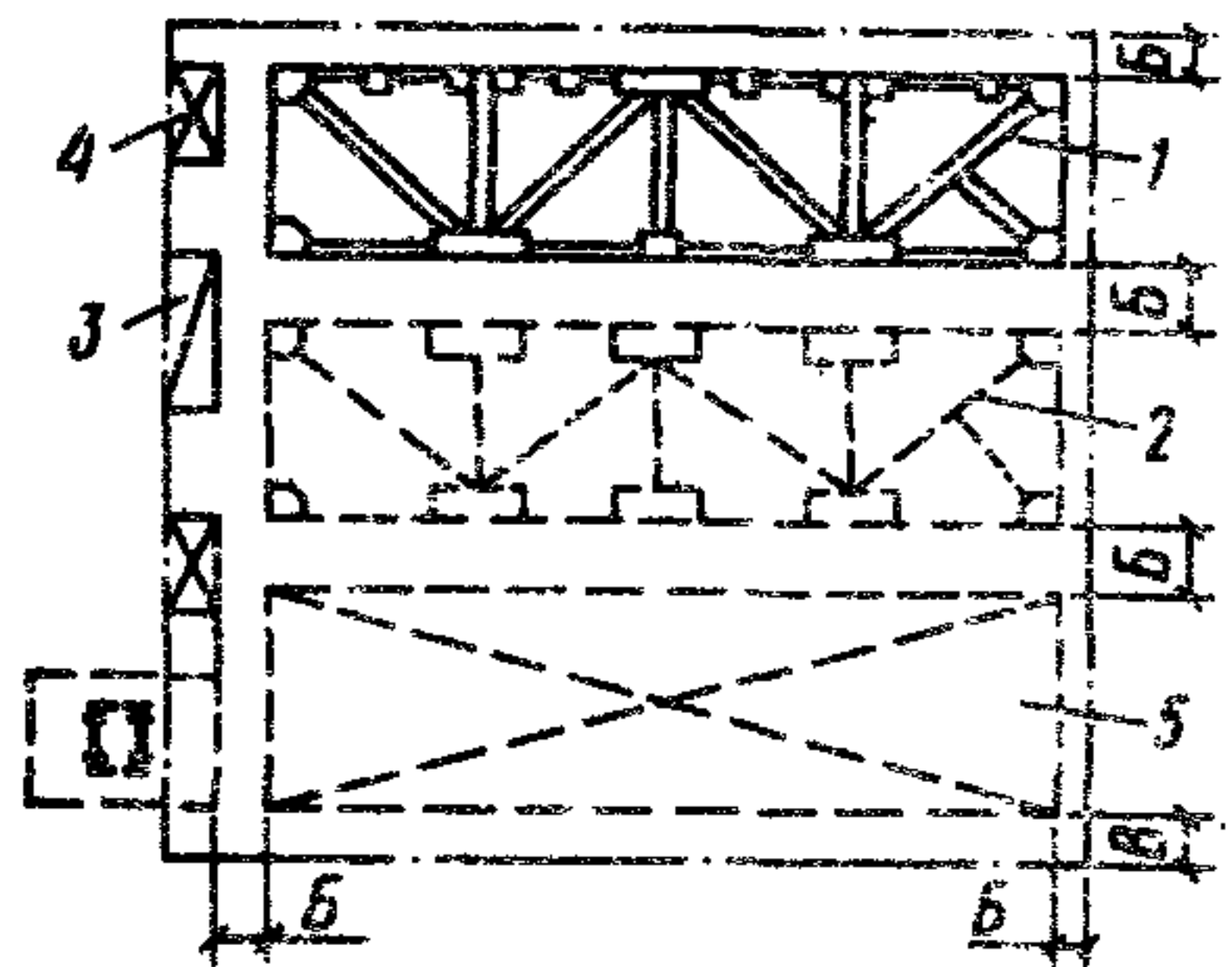
Рис.36. Размещение участка для сборки конструкций в поперечном пролете 1 — сборка окончательная; 2 — кондуктор для сборки; 3 — ящик для инструмента; 4 — трансформатор сварочный; 5 — место складирования; B=800 мм, B=500 мм
