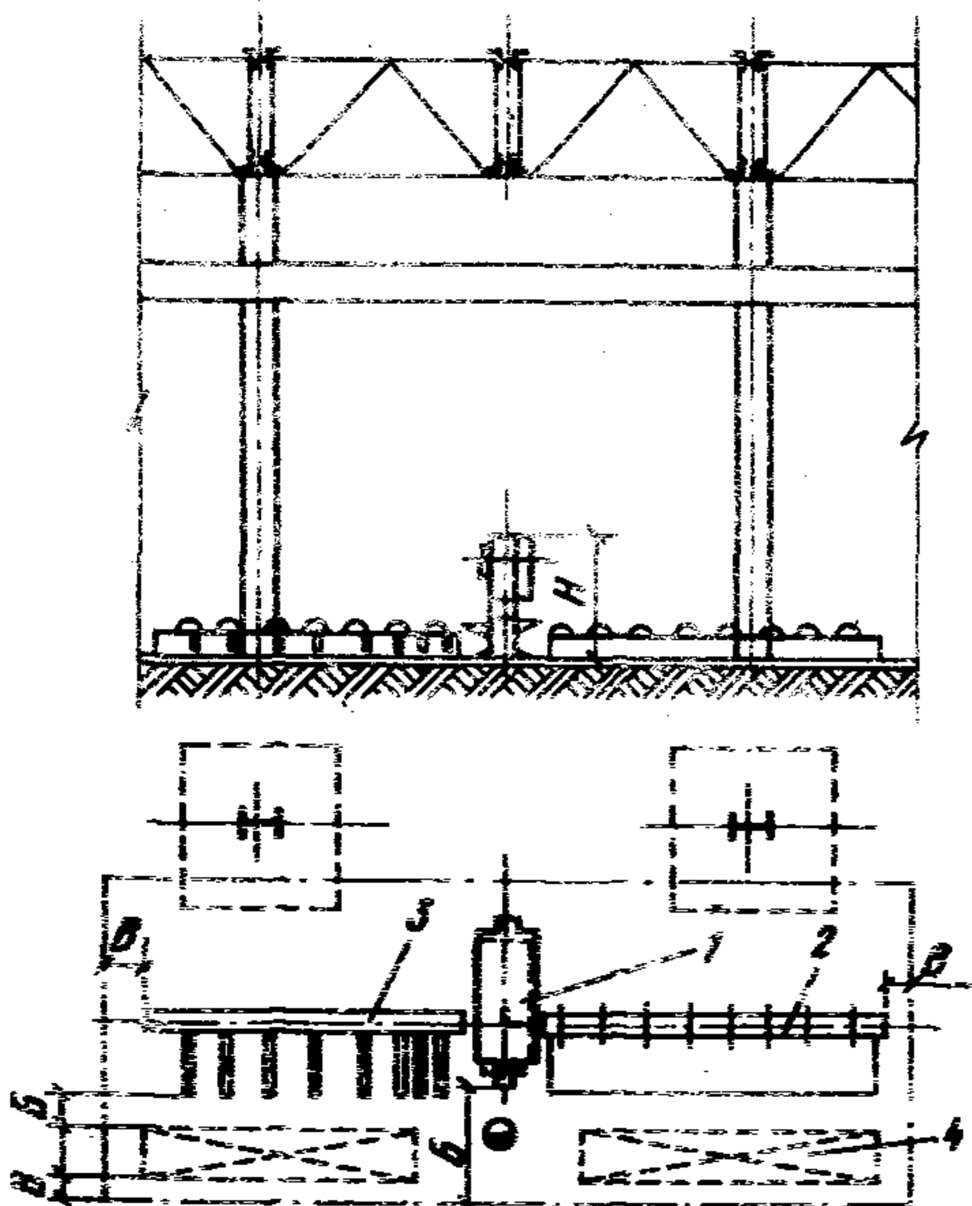
Рис.12. Размещение комбинированных пресс-ножниц в продольном пролете 1 – пресс-ножницы; 2 – ролик подающий; 3 – ролик приемный; 4 – место складирования; B = 800 мм, B_1 = 500 мм
