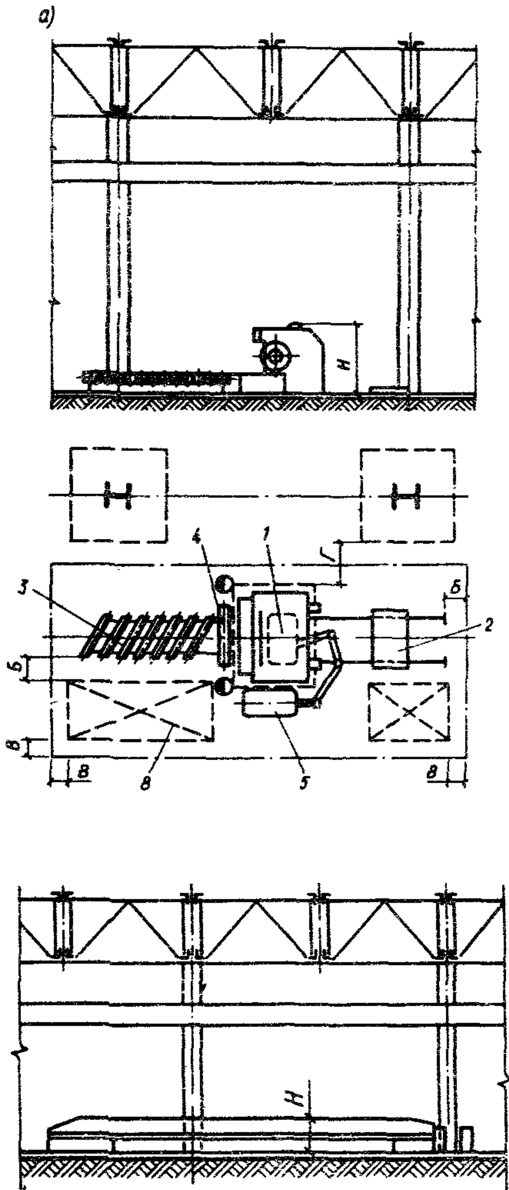
Рис.14. Размещение гильотинных ножниц при поперечной резке листа (а), при продольной резке листа (б)
