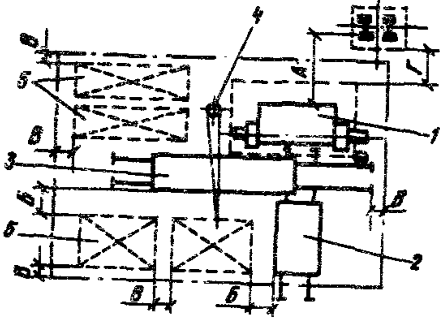
Рис.6. Размещение сортогибочной машины в продольном пролете 1 – машина; 2 – козелок переставной; 3 – место складирования; А = 400 мм, Б = 800 мм, В = 500 мм
