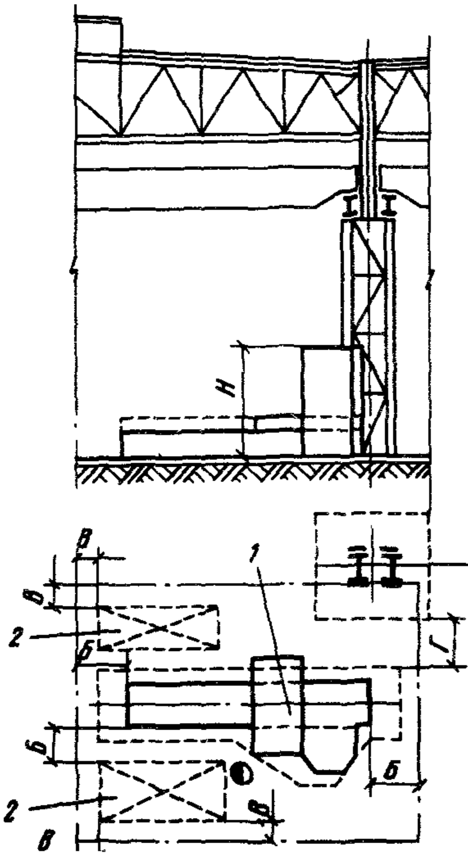
Рис.16. Размещение продольно-строгального или продольно-фрезерного станка в поперечном пролете 1 – станок продольно-строгальный; 2 – место складирования; Б=800 мм, В=500 мм, Г=200 мм
