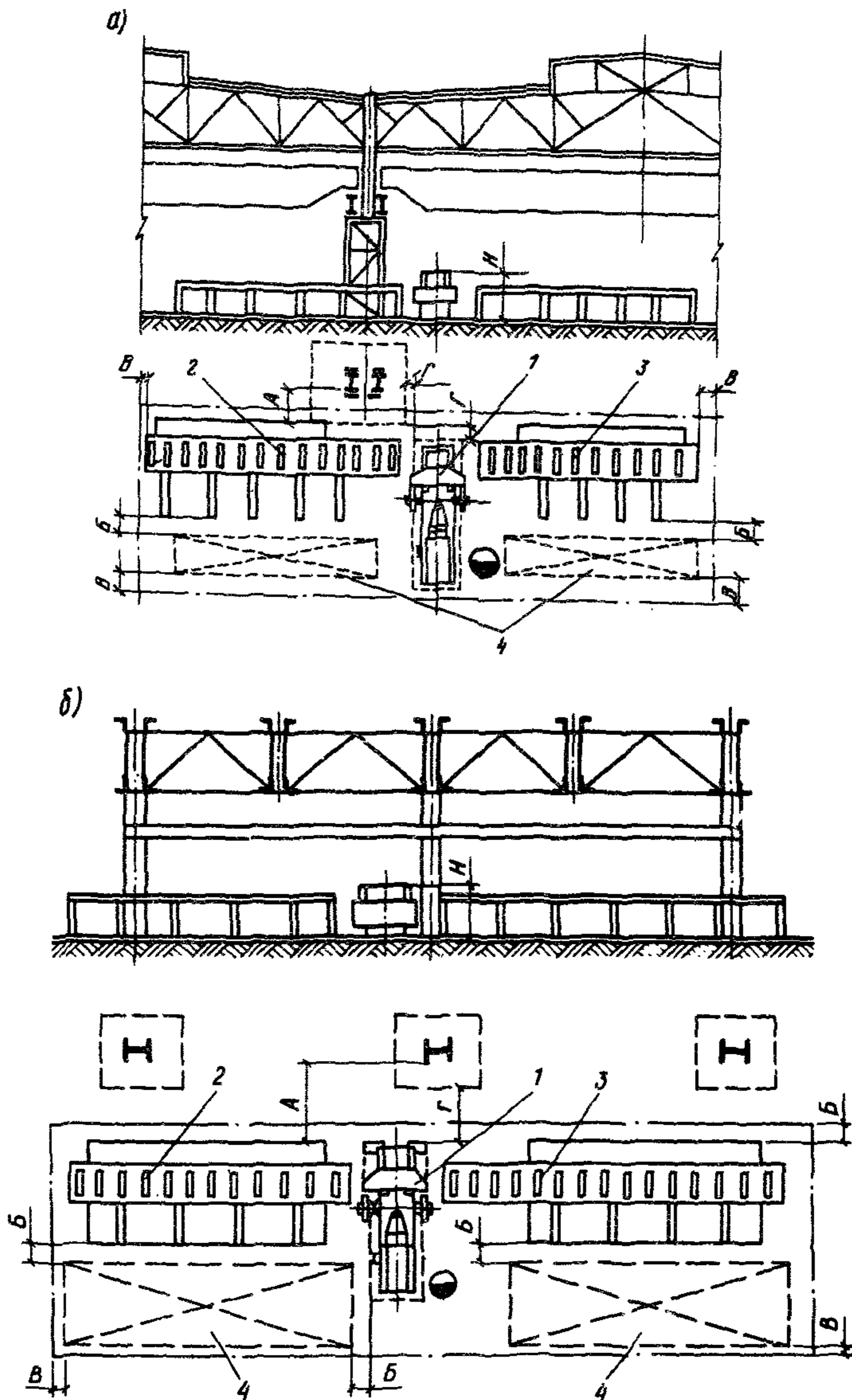
Рис. 8. Размещение горизонтального правильно-гибочного прессы в поперечном пролете (а), в продольном пролете (б) 1 — пресс; 2 — ролик загрузочный; 3 — ролик приемный; 4 — место складирования; A = 400 мм, B = 800 мм, B = 500 мм, \Gamma = 200 мм
