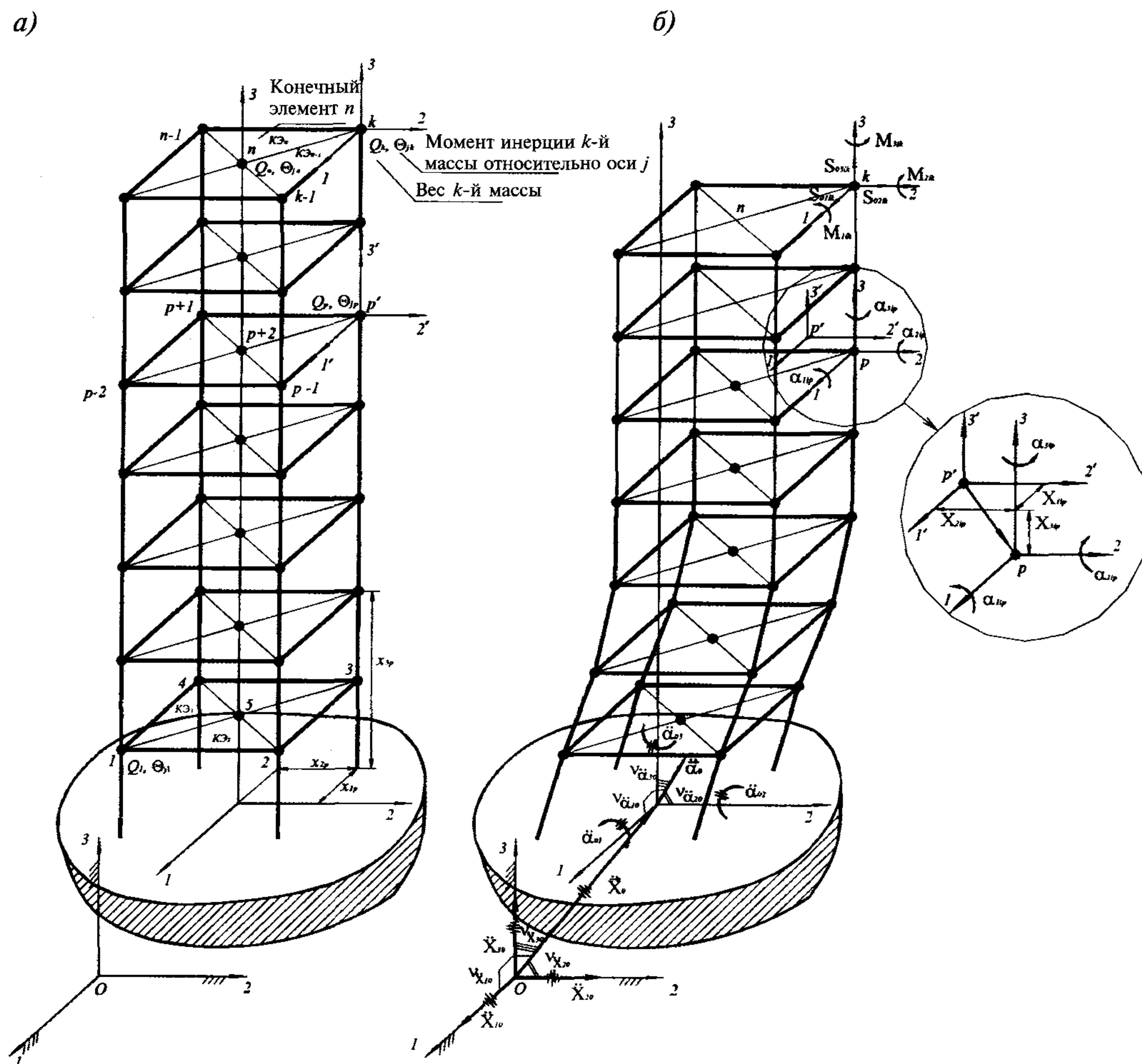
Рис. В.1. Пространственная расчетная динамическая модель сооружения а — состояние покоя; б — i -я форма колебаний
