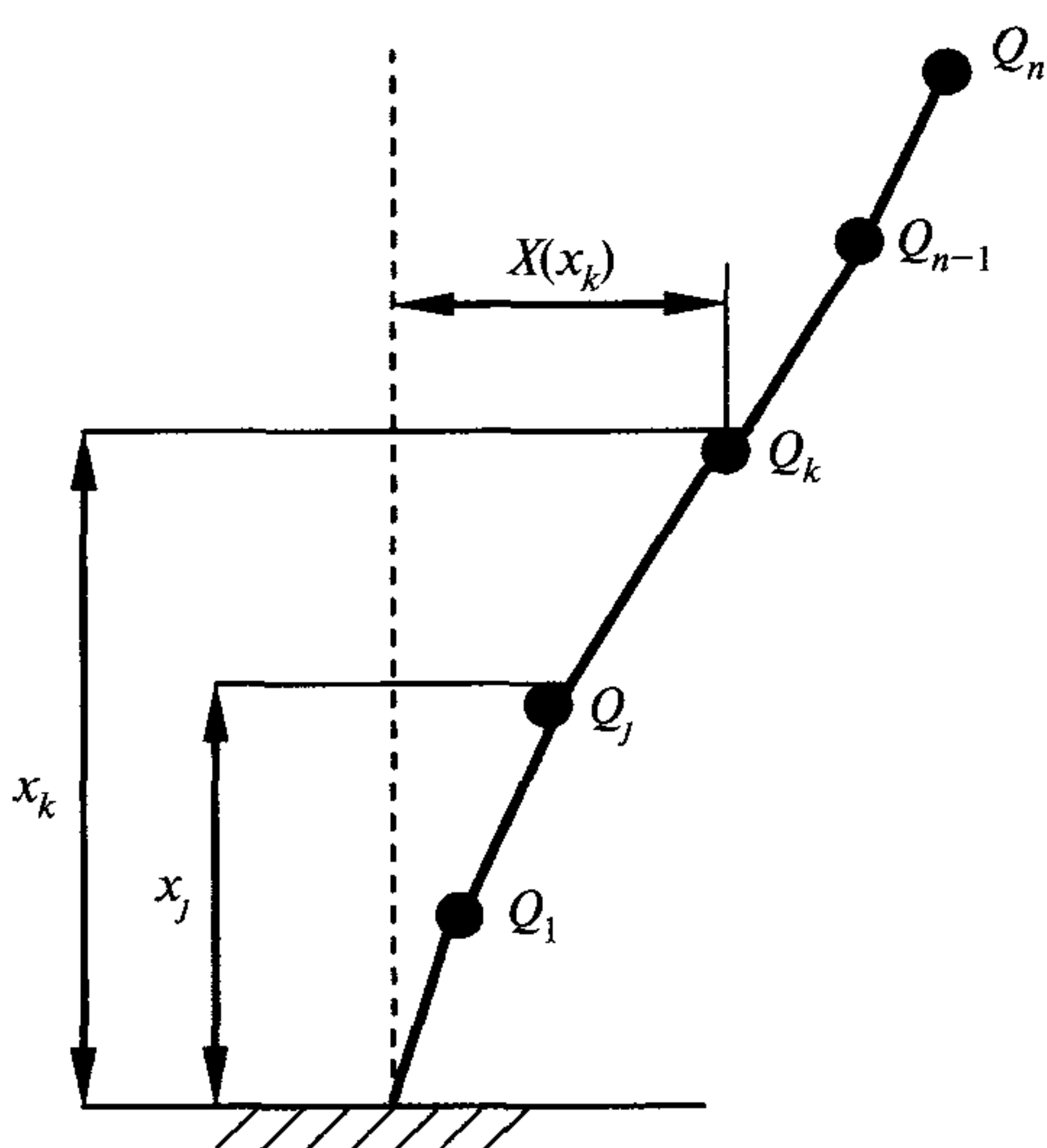
Рис. 1. Упрощенная модель сооружения
