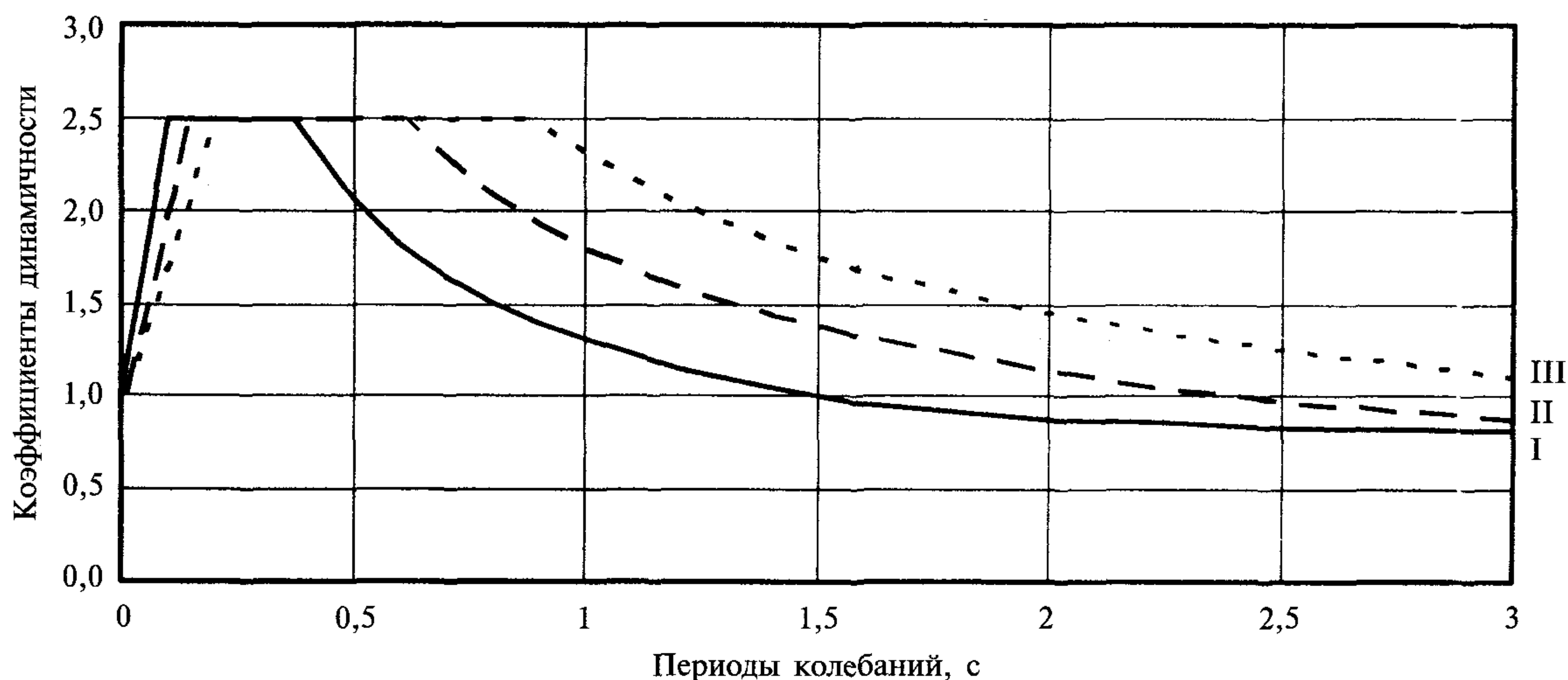
Рис. 2. Значение коэффициента динамичности \beta
