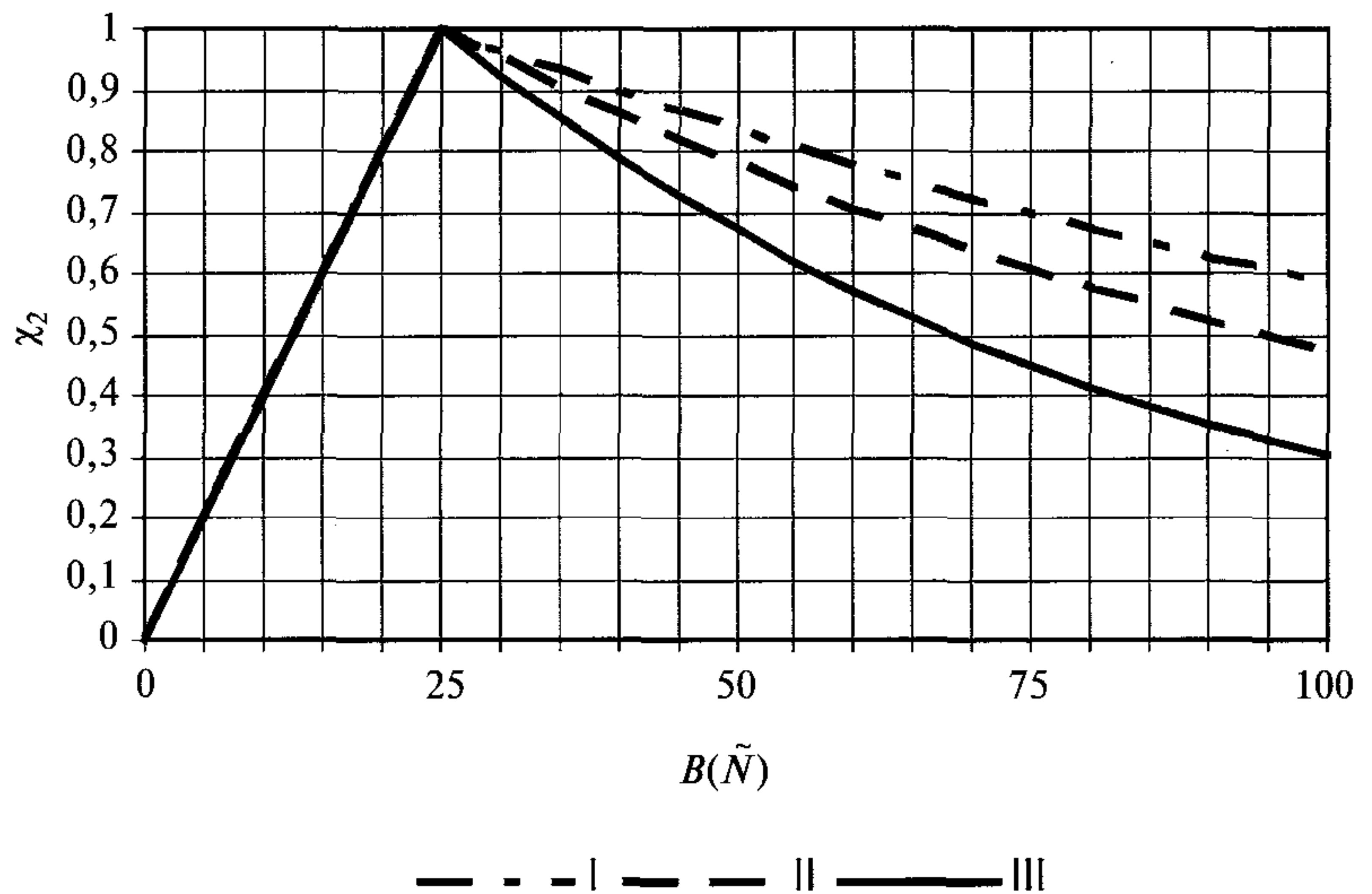
Рис. В.3. Графики нормированных функций \chi_2(B) , B , м — наименьший размер сооружения в плане
