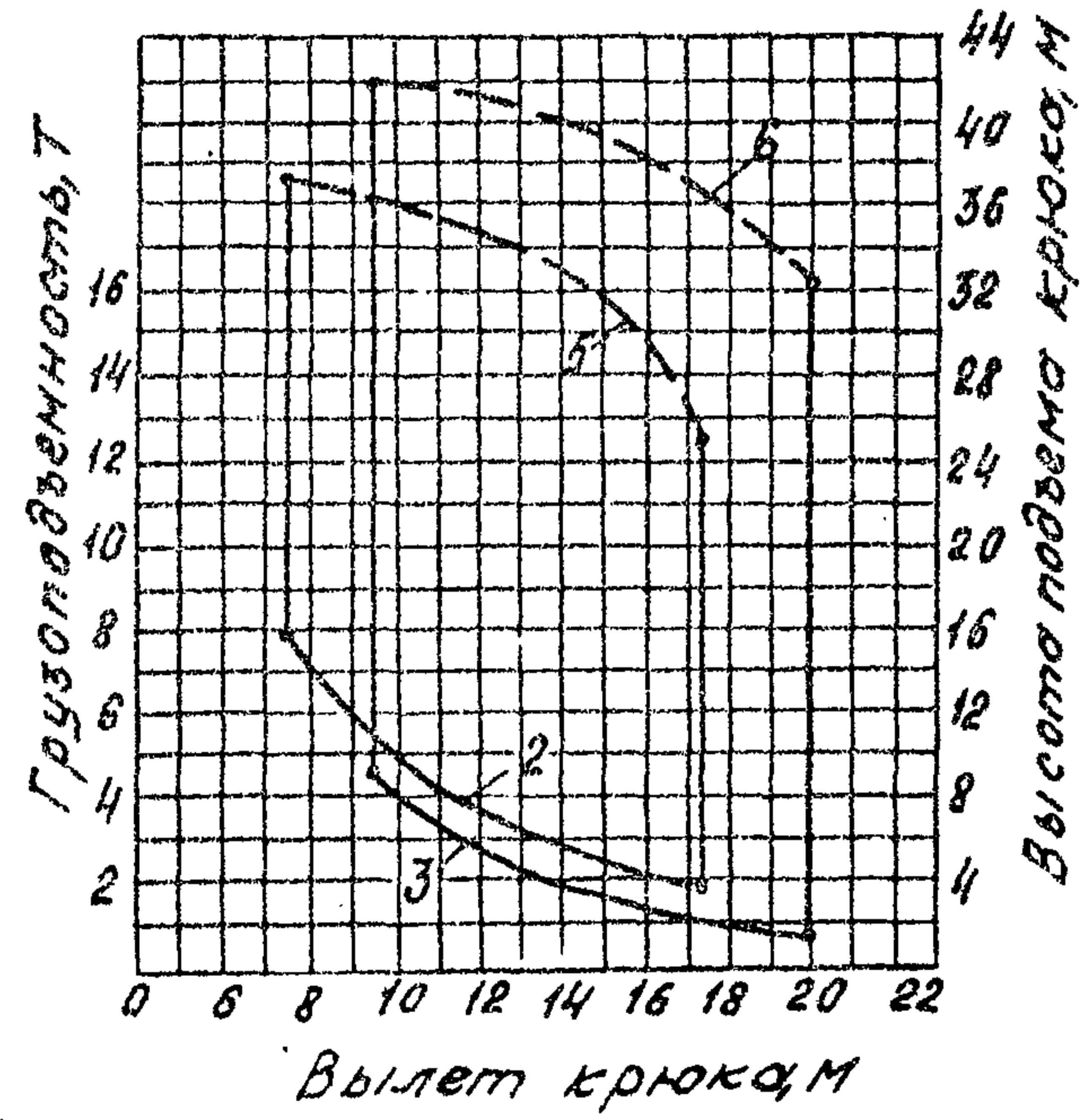
Башня 25м, гуськи 15 и 20м
