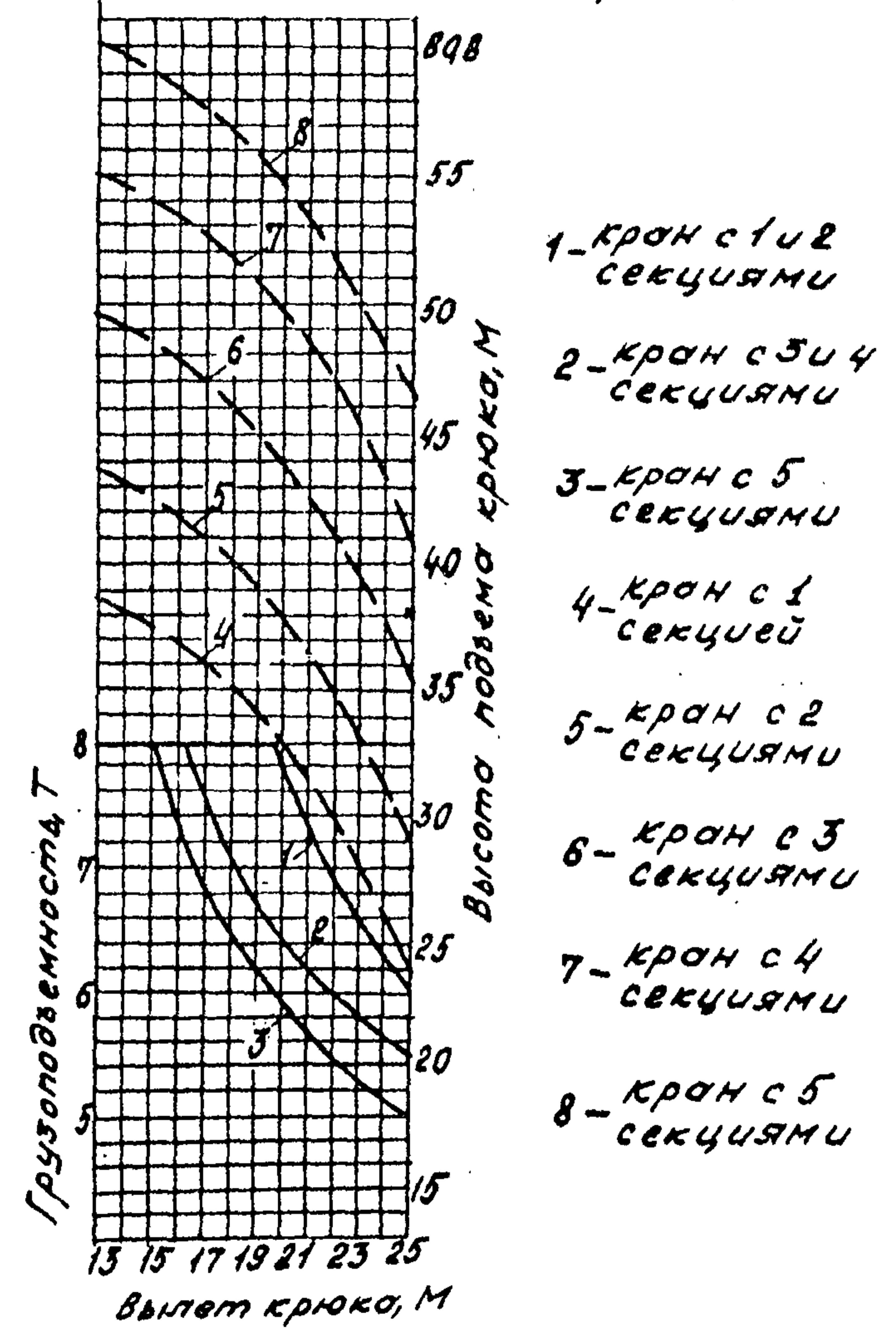
Графики грузоподъемности и высоты подъема крюка в I ветровом районе
