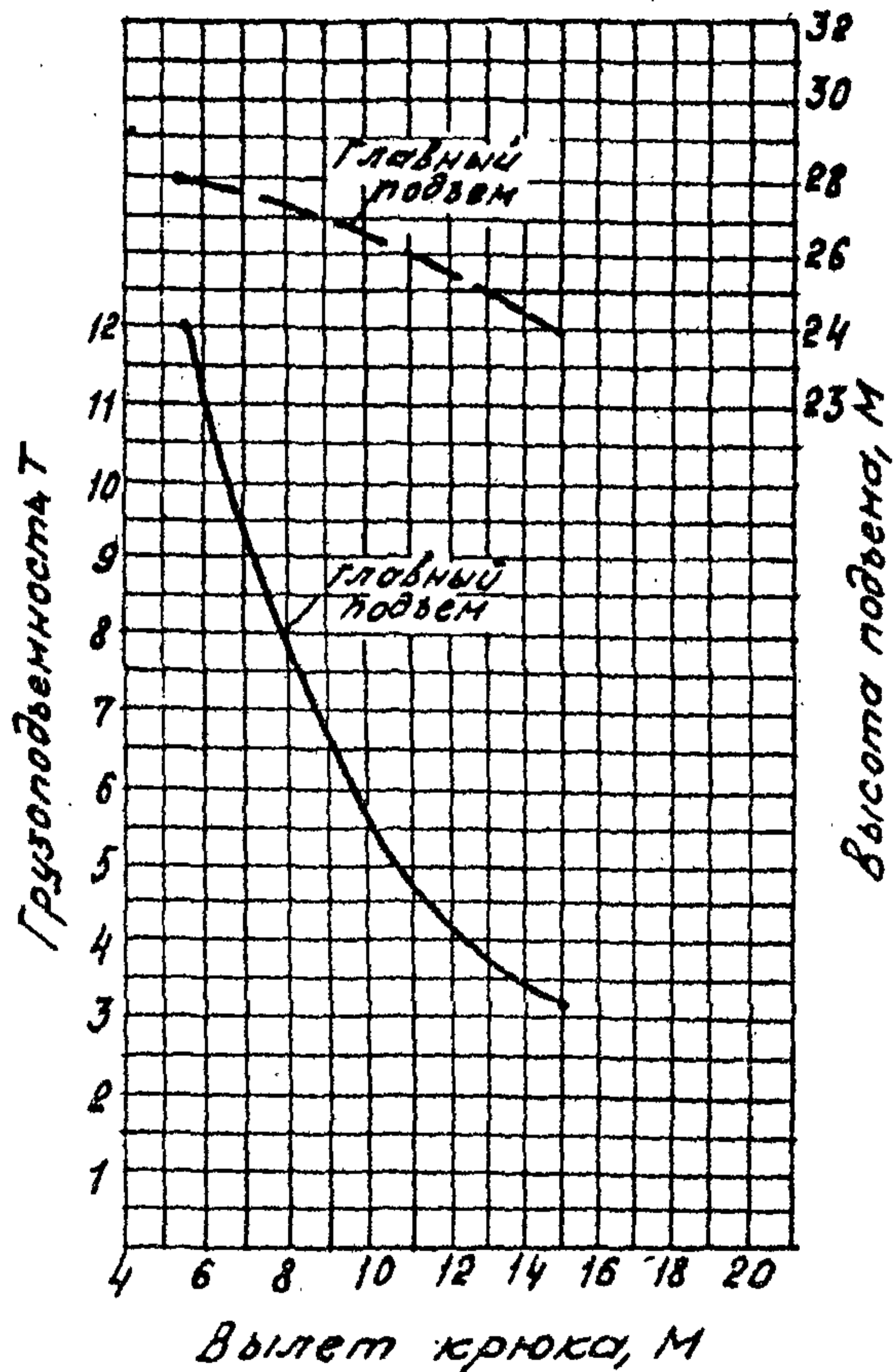
Стрела 28,5 м
