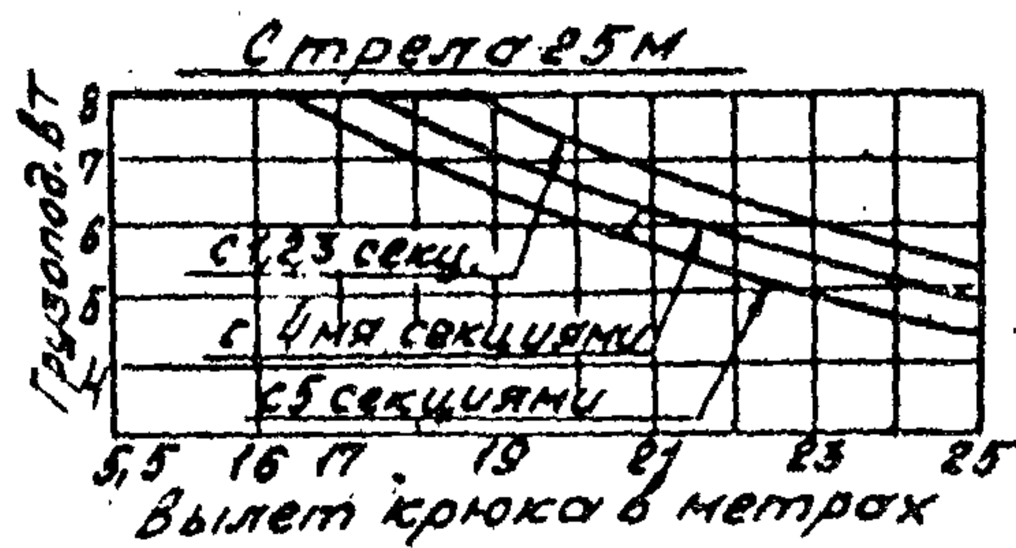
Кривые грузоподъемности для стрел с движущейся кареткой.
