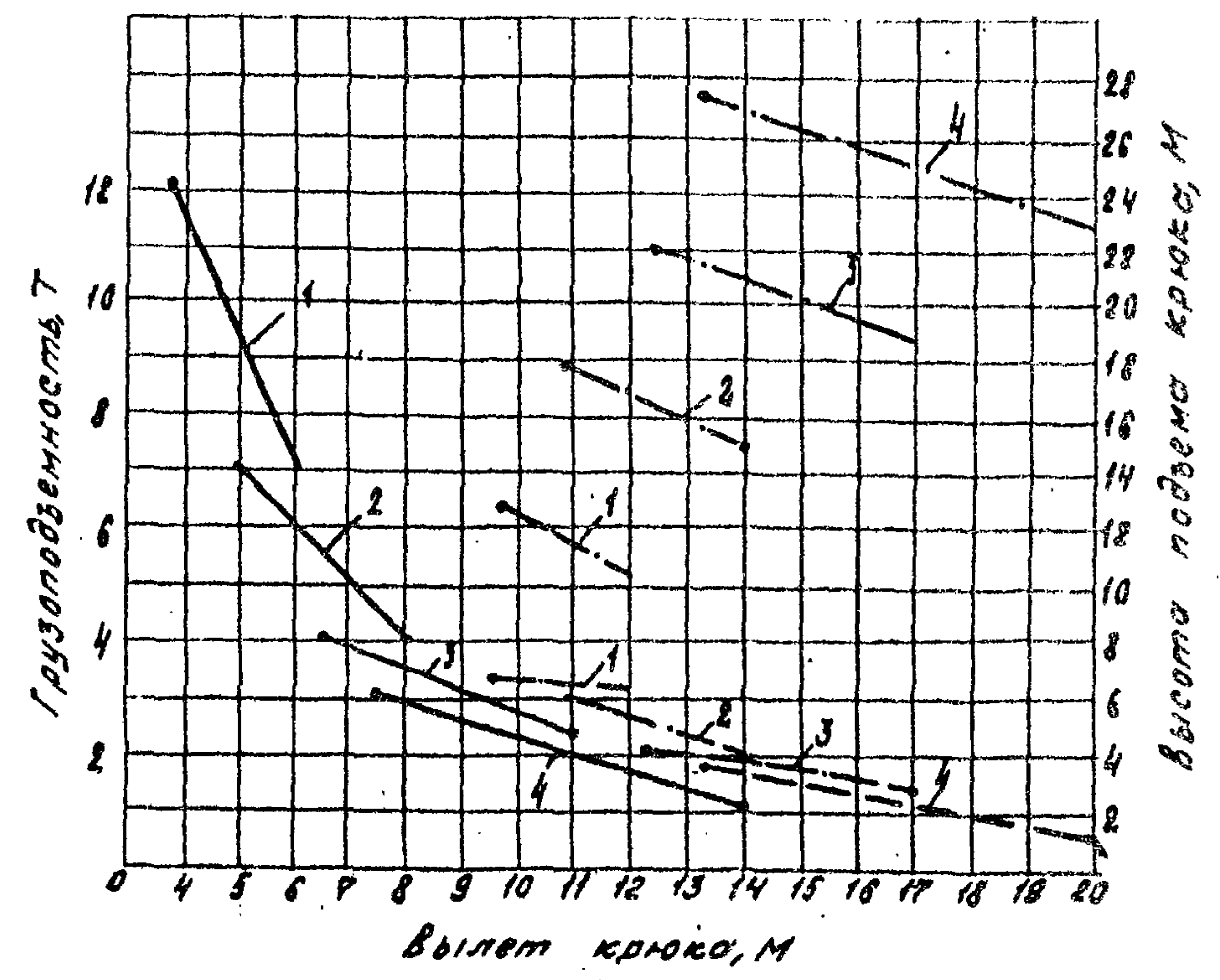
Графики грузоподъемности и высоты подъема крюка крана на опорах, стрела с гуськом (надставкой) в м
