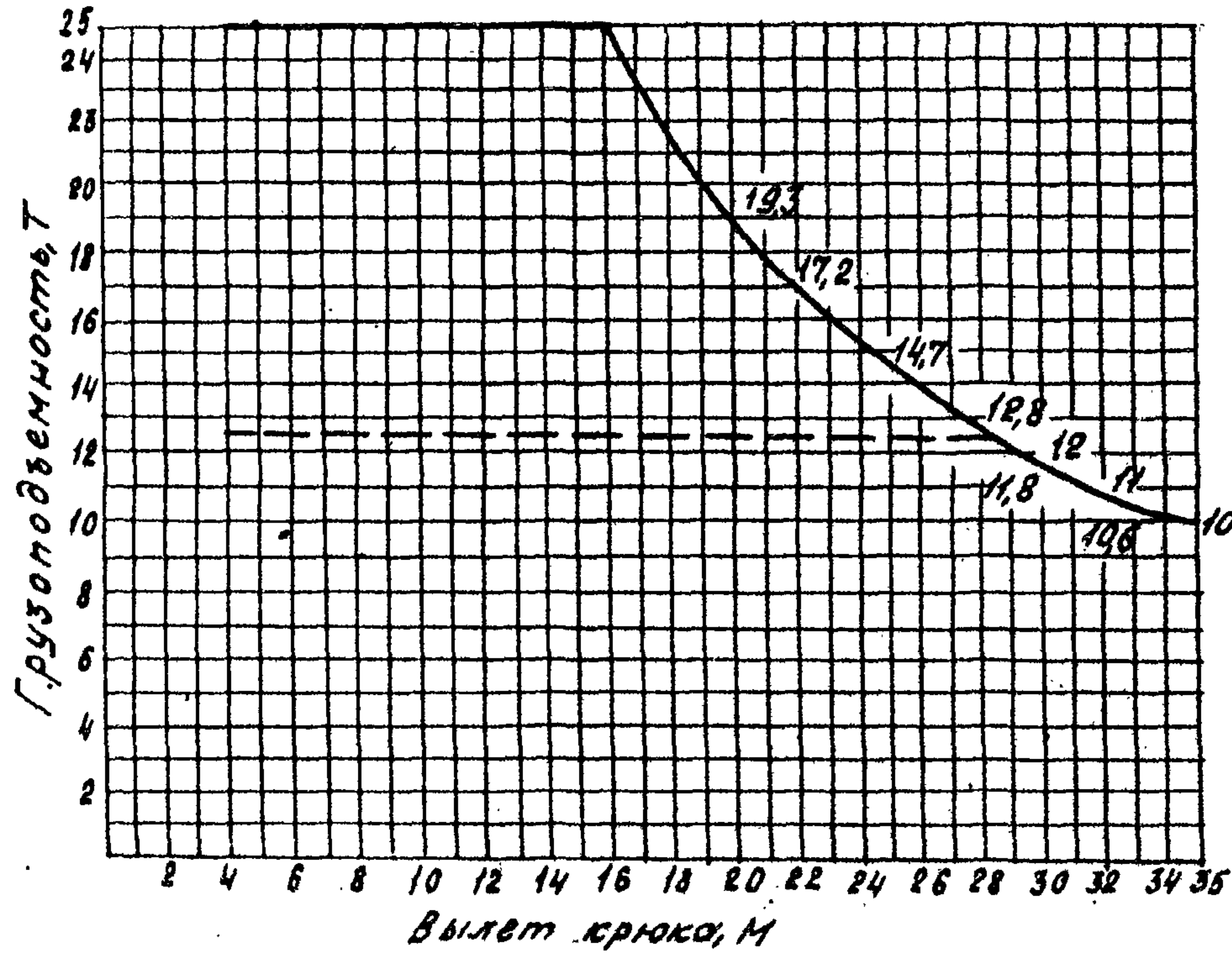
КБ-676-1
