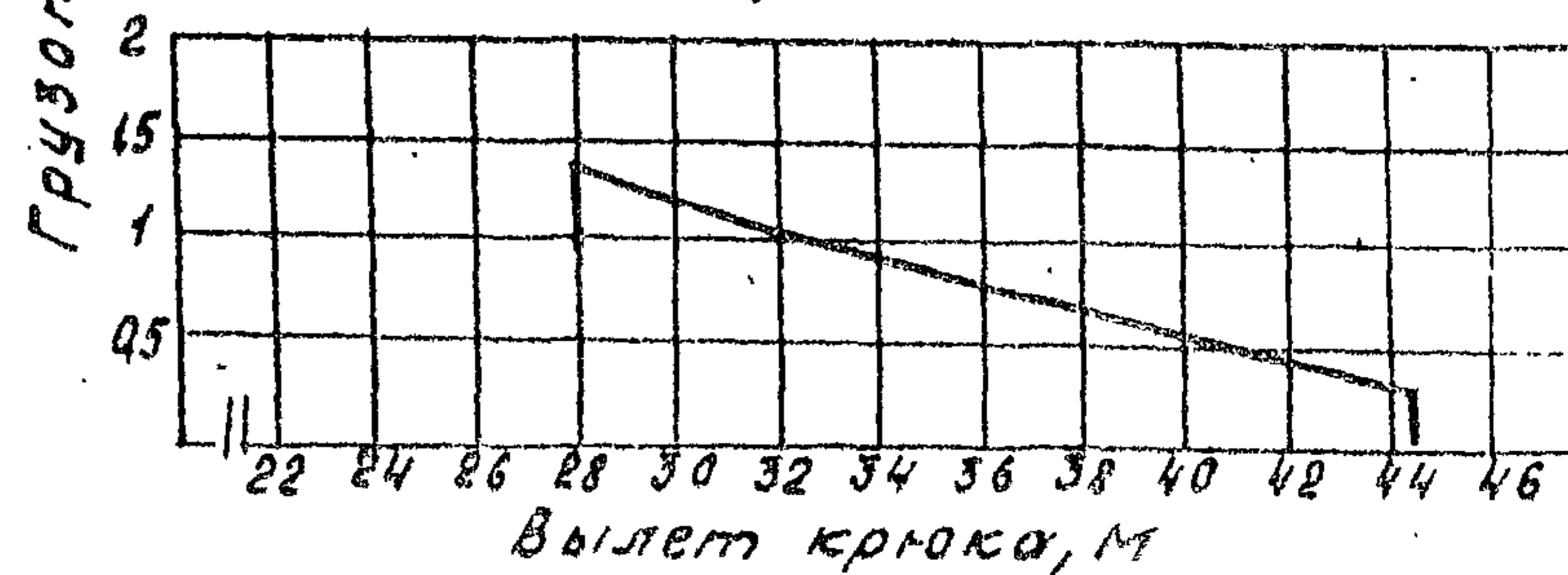
Стрела 80,8 м
