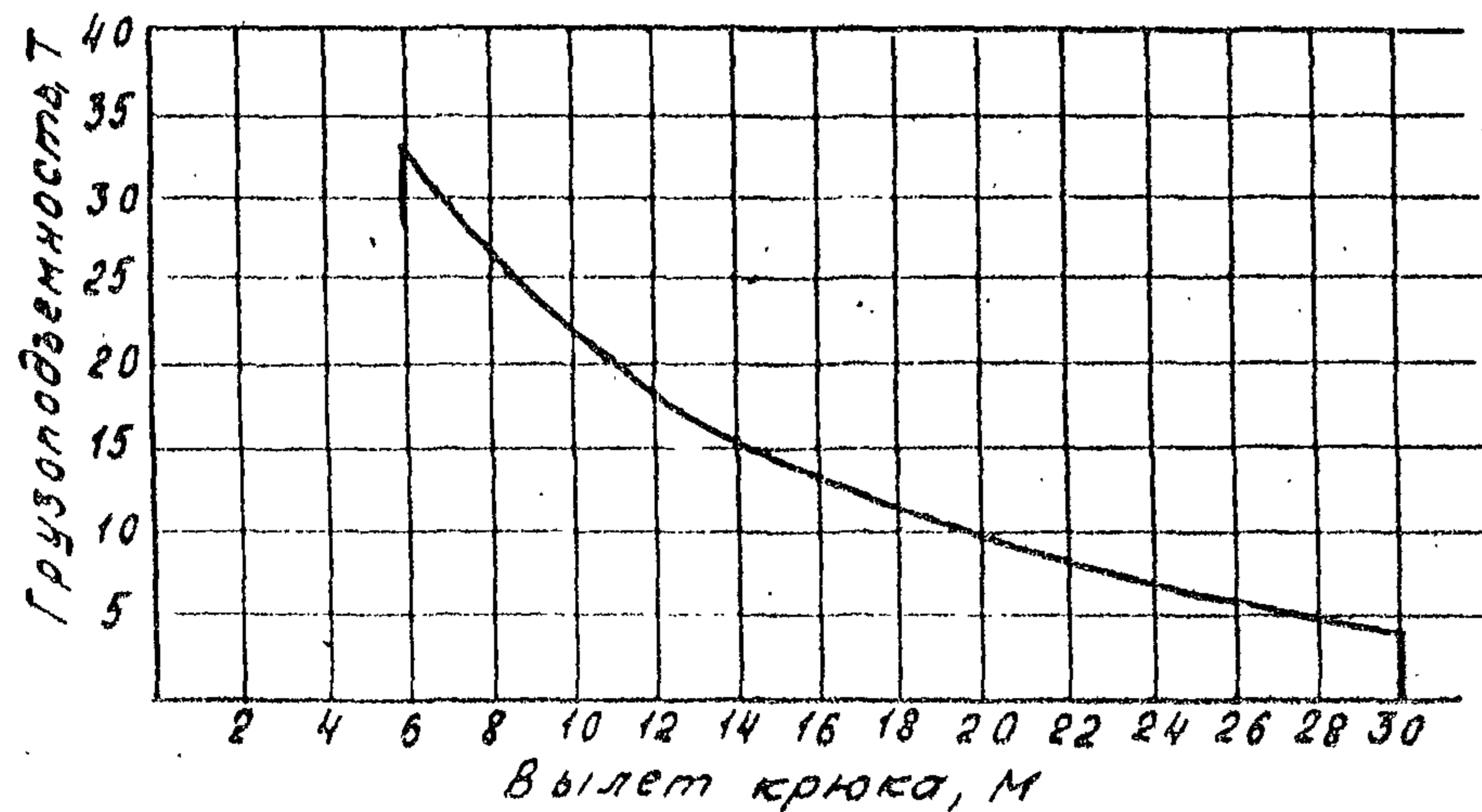
Стрела 33,2 м
