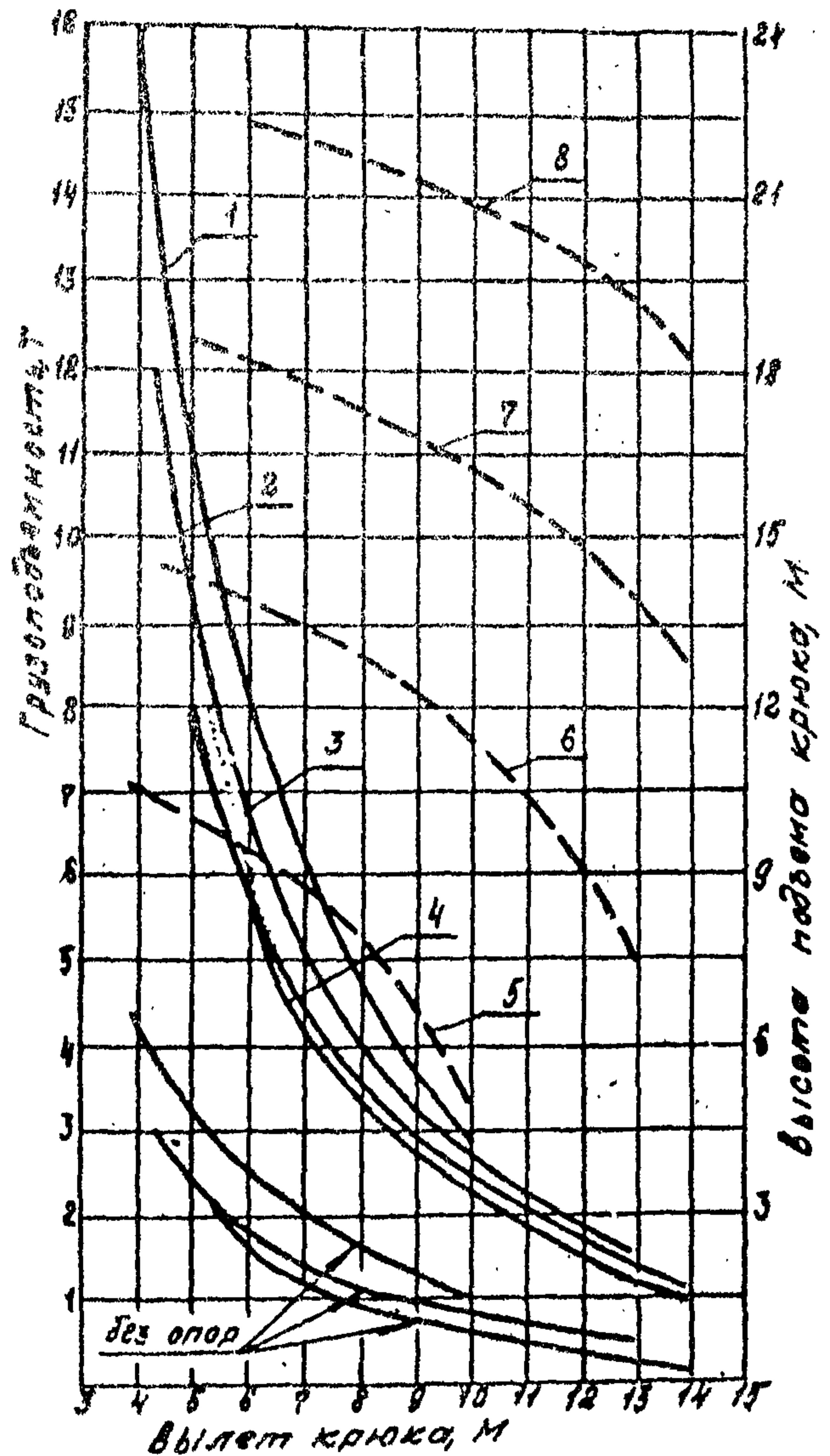
Графики грузоподъемности (без гуська) и высоты подъема крюка
