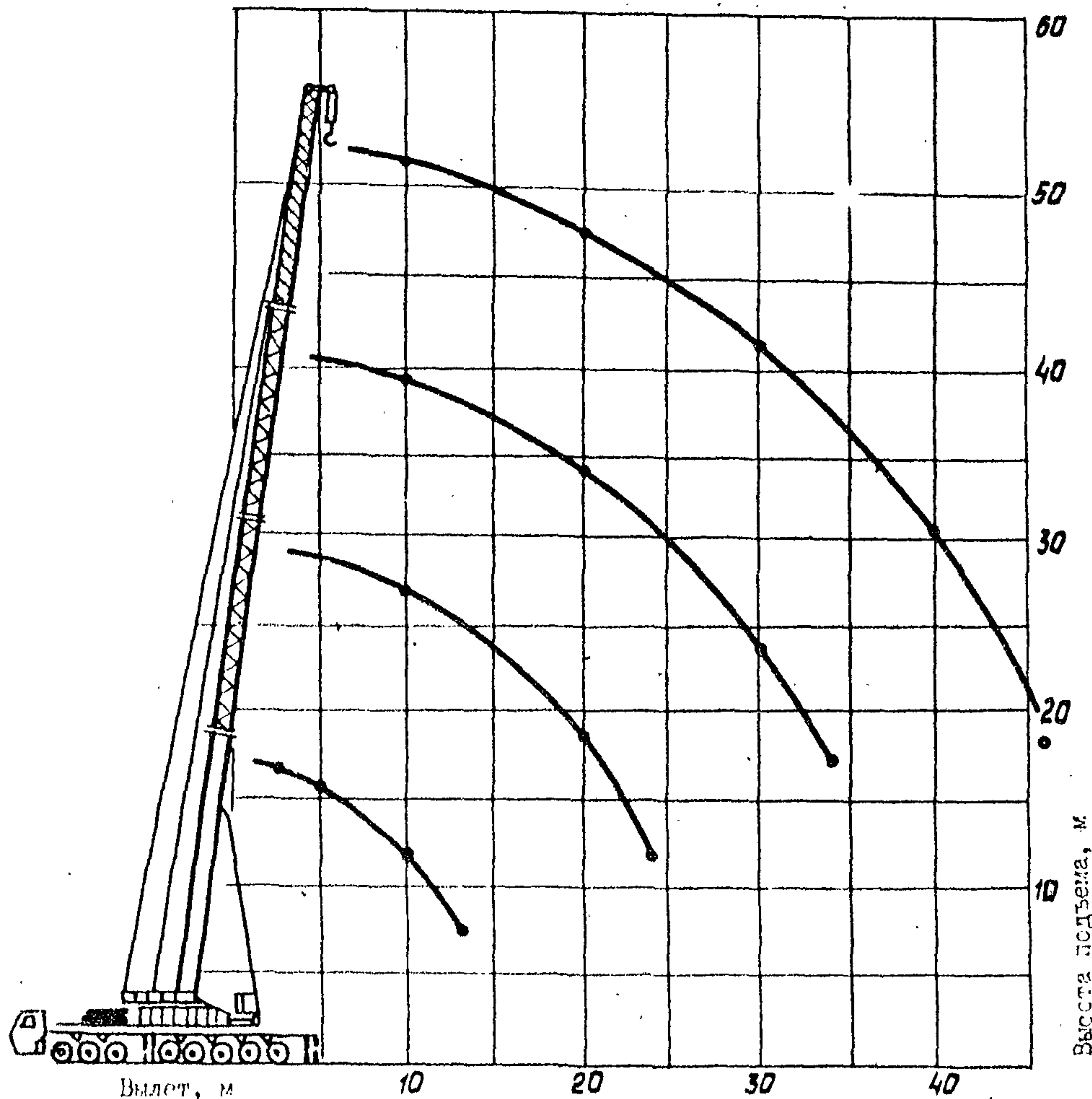
График высоты подъема
