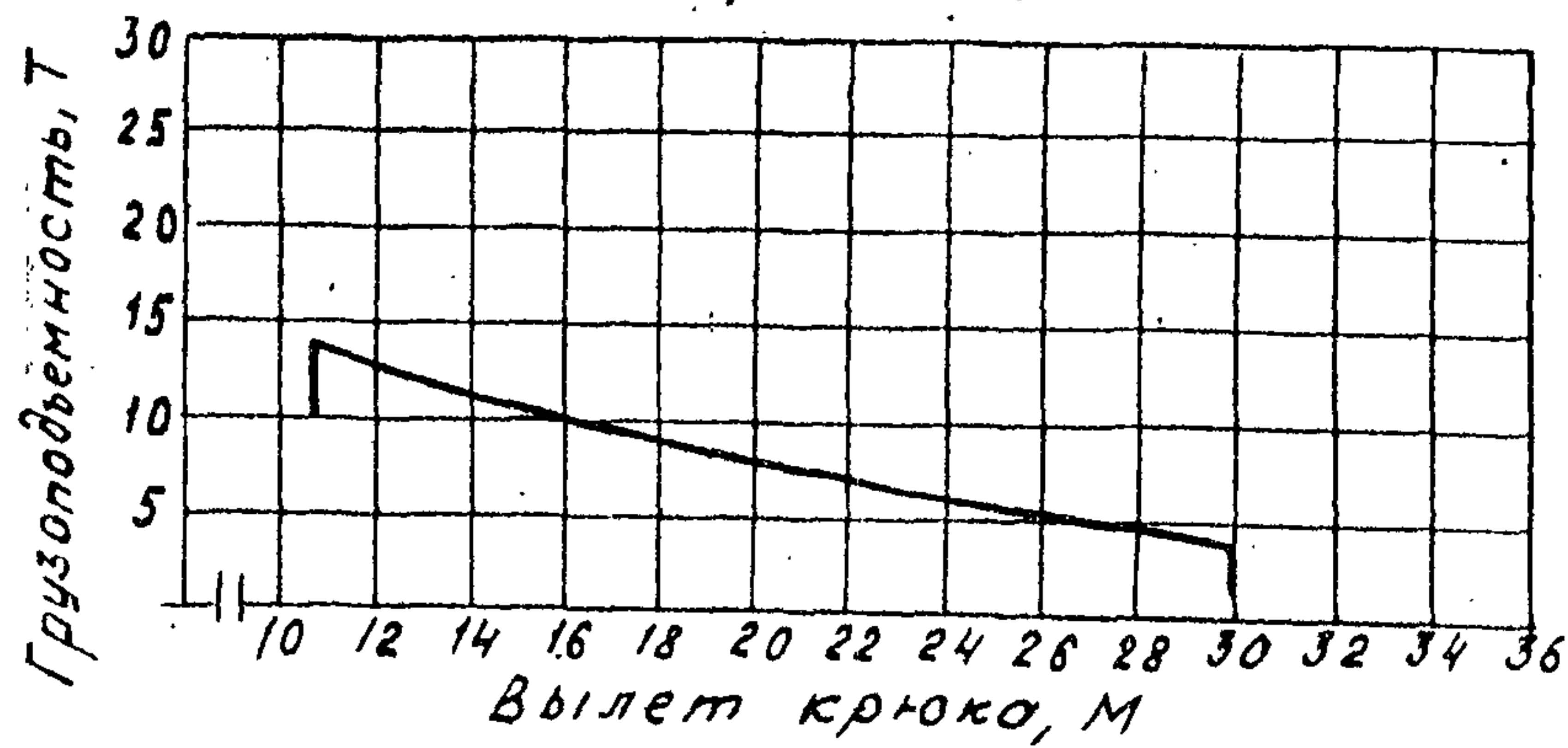
Стрела 45,2
