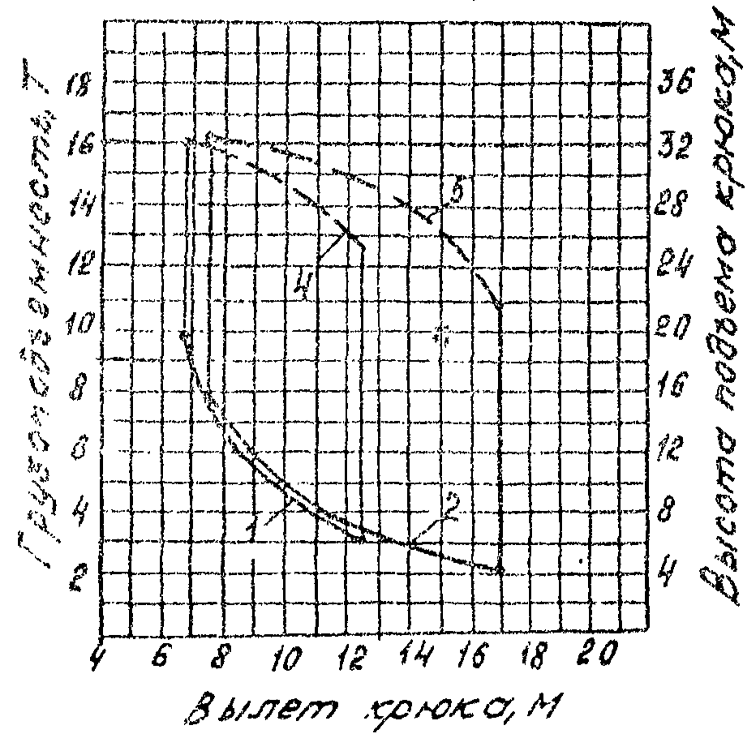
Башня 20м, гусек 10 и 20м
