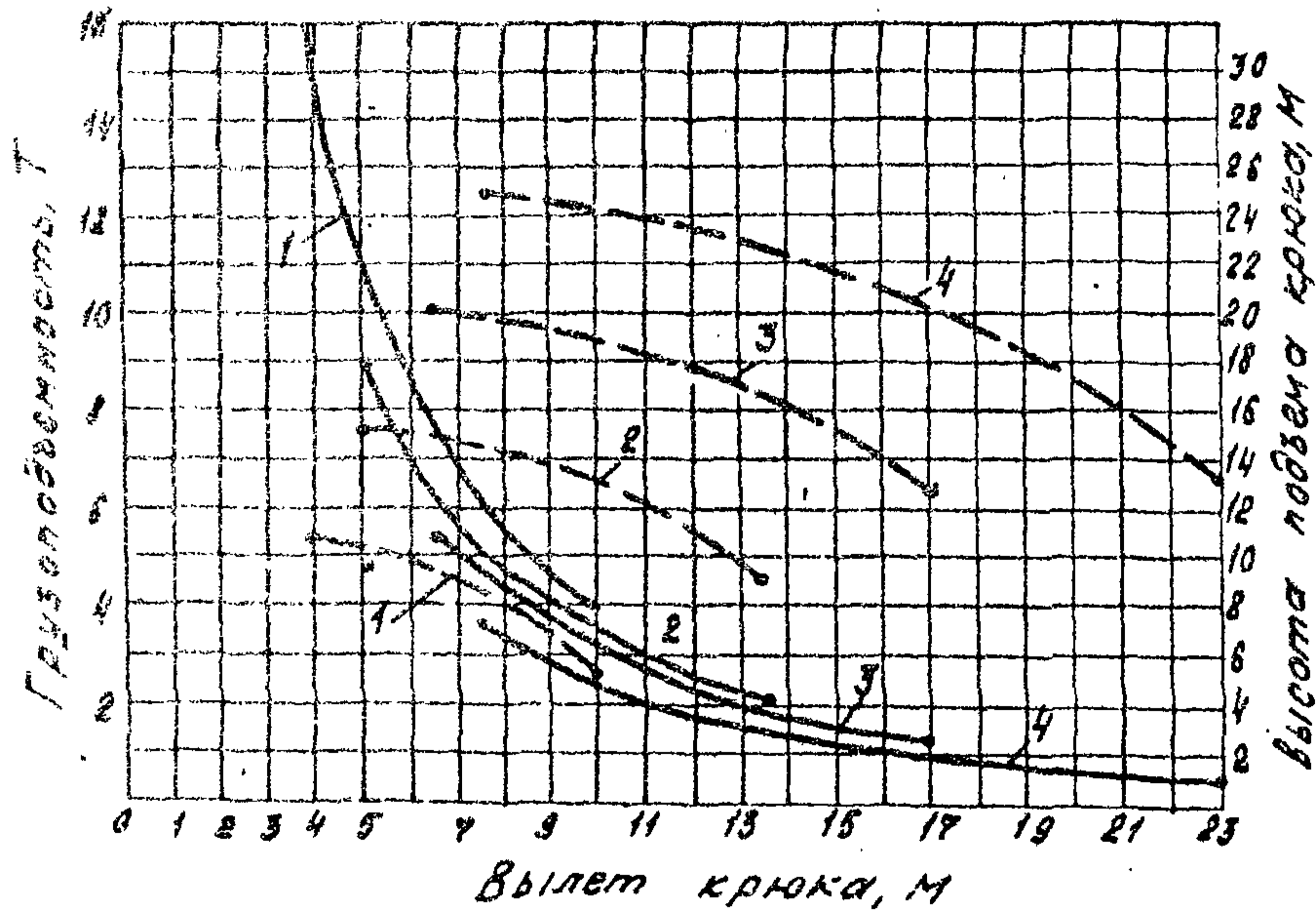
Кран на выносных опорах
