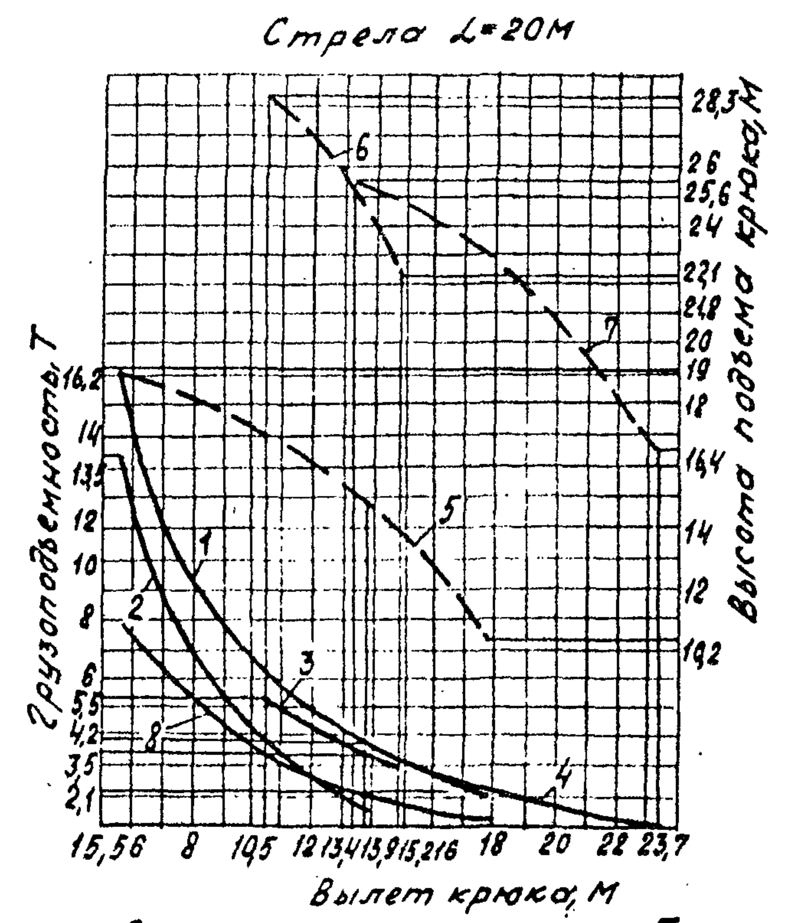
Графики грузоподъемности
