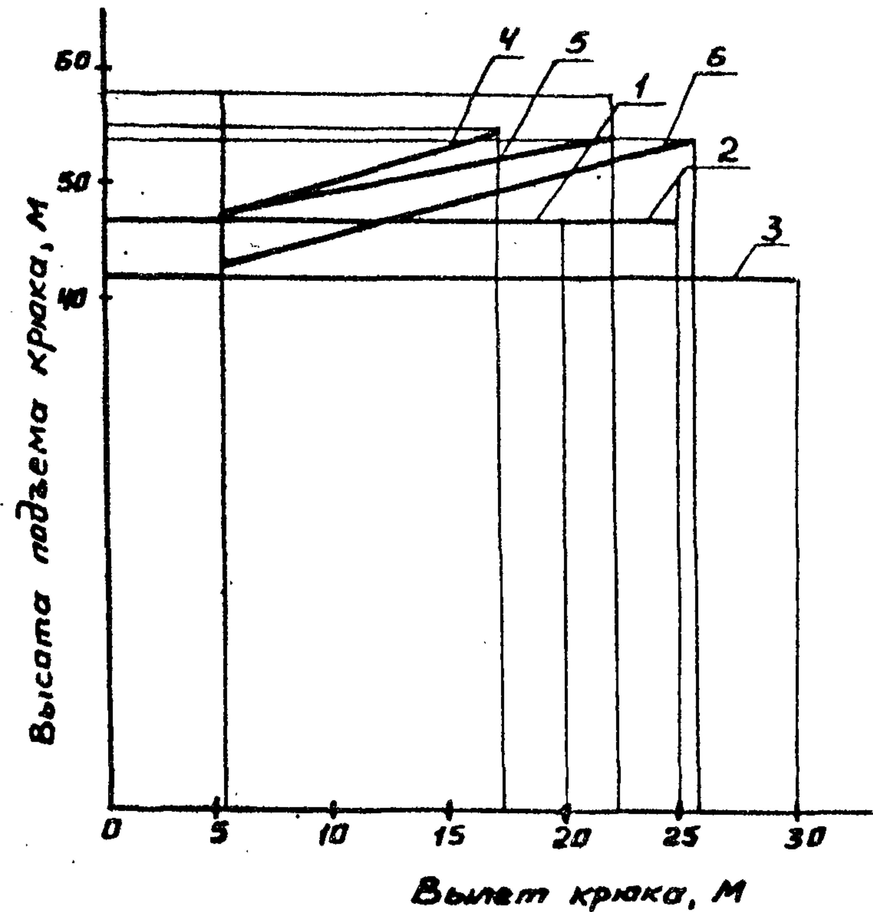
Графики высоты подъема крюка
