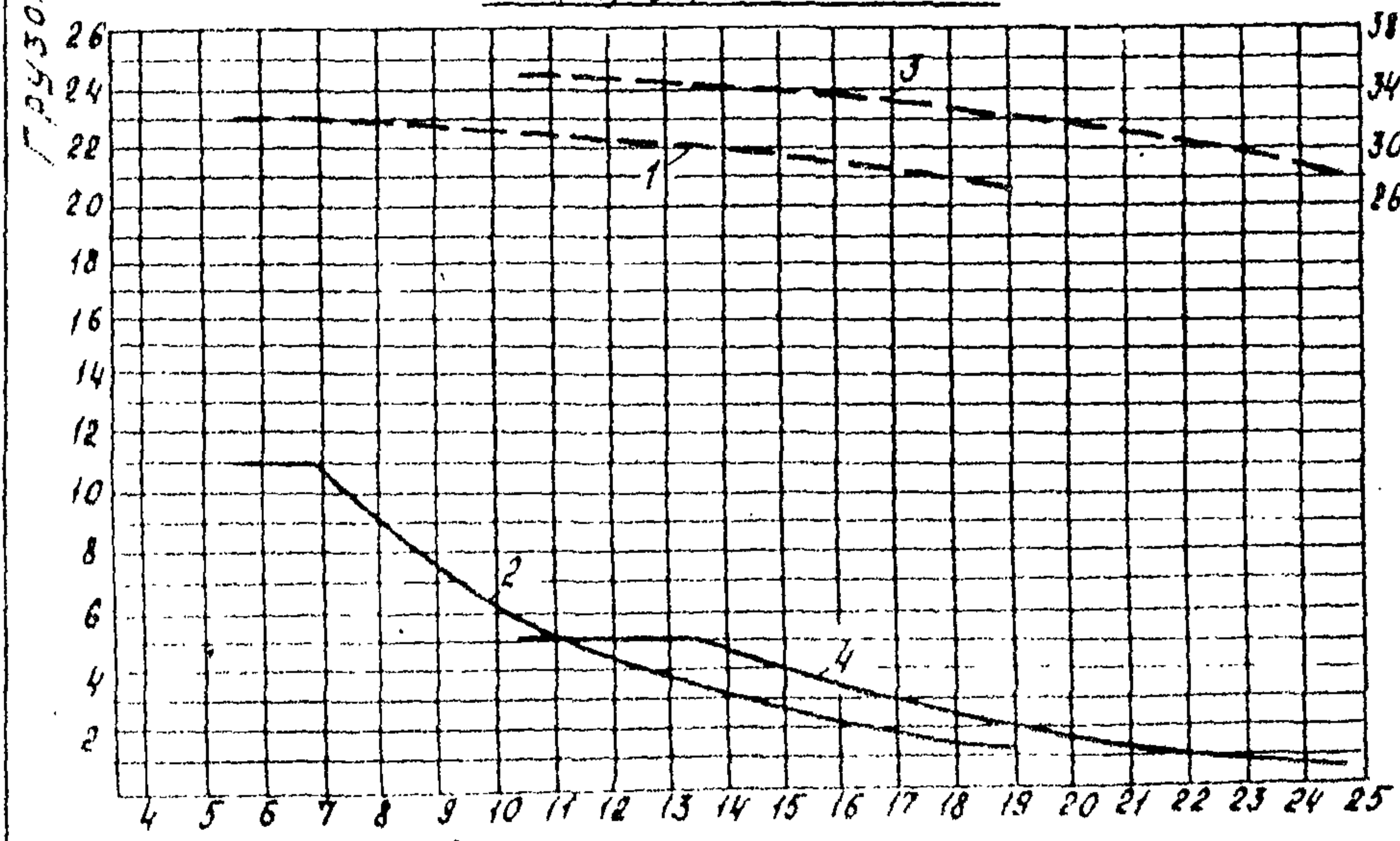
Стрела 32,5м
