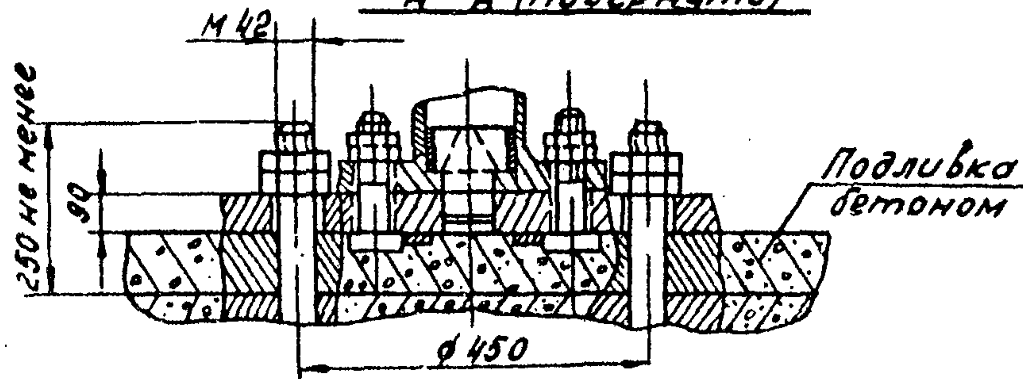
А-А (повернуто)
