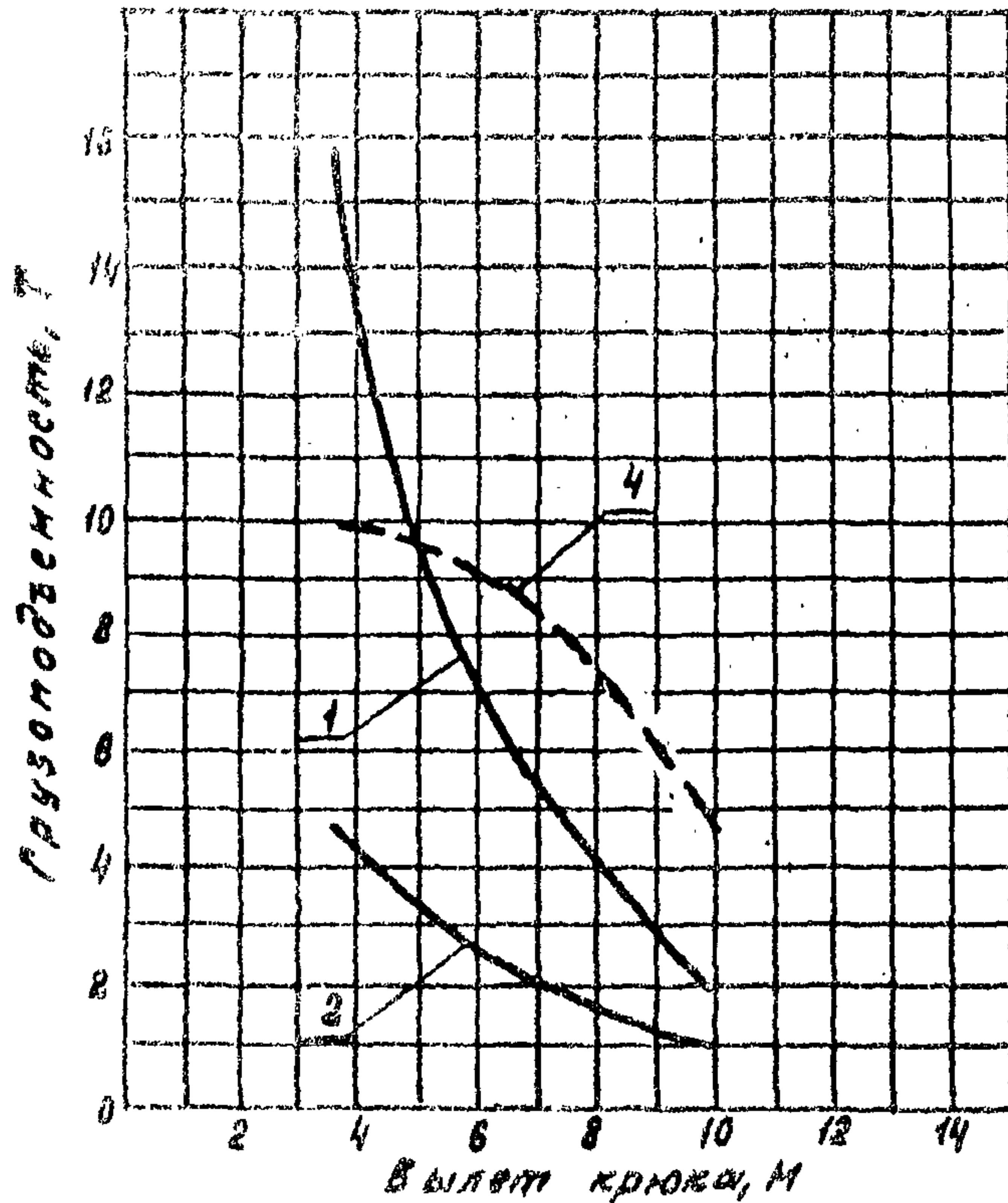
Стрела 10 м
