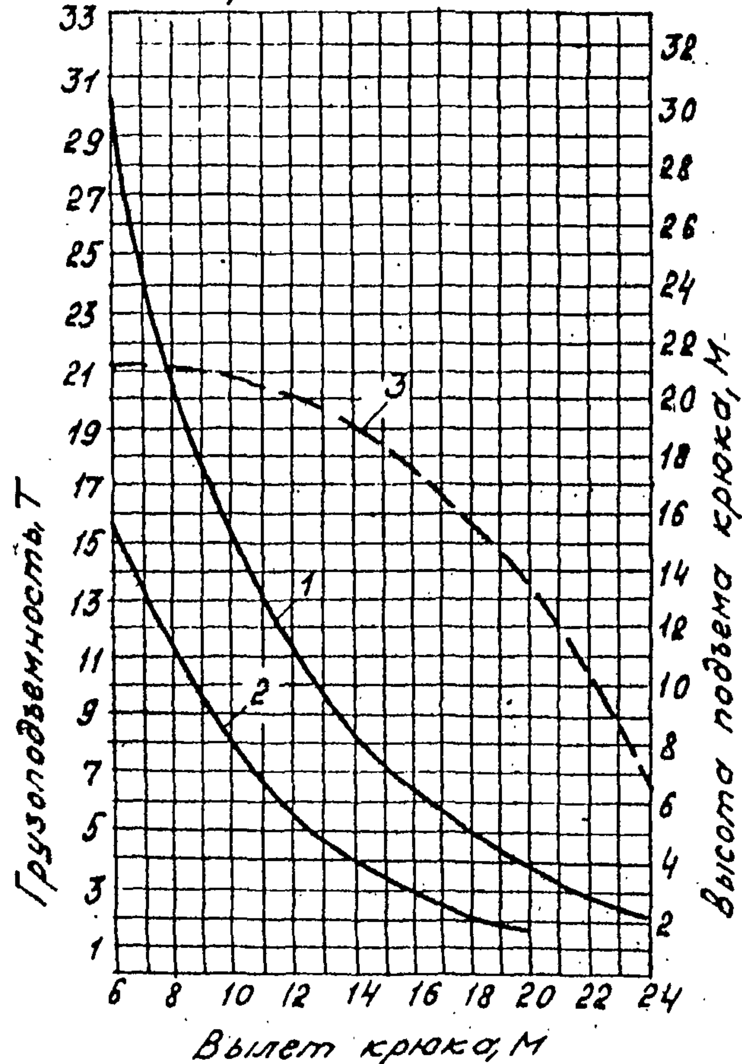
Стрела 24 м
