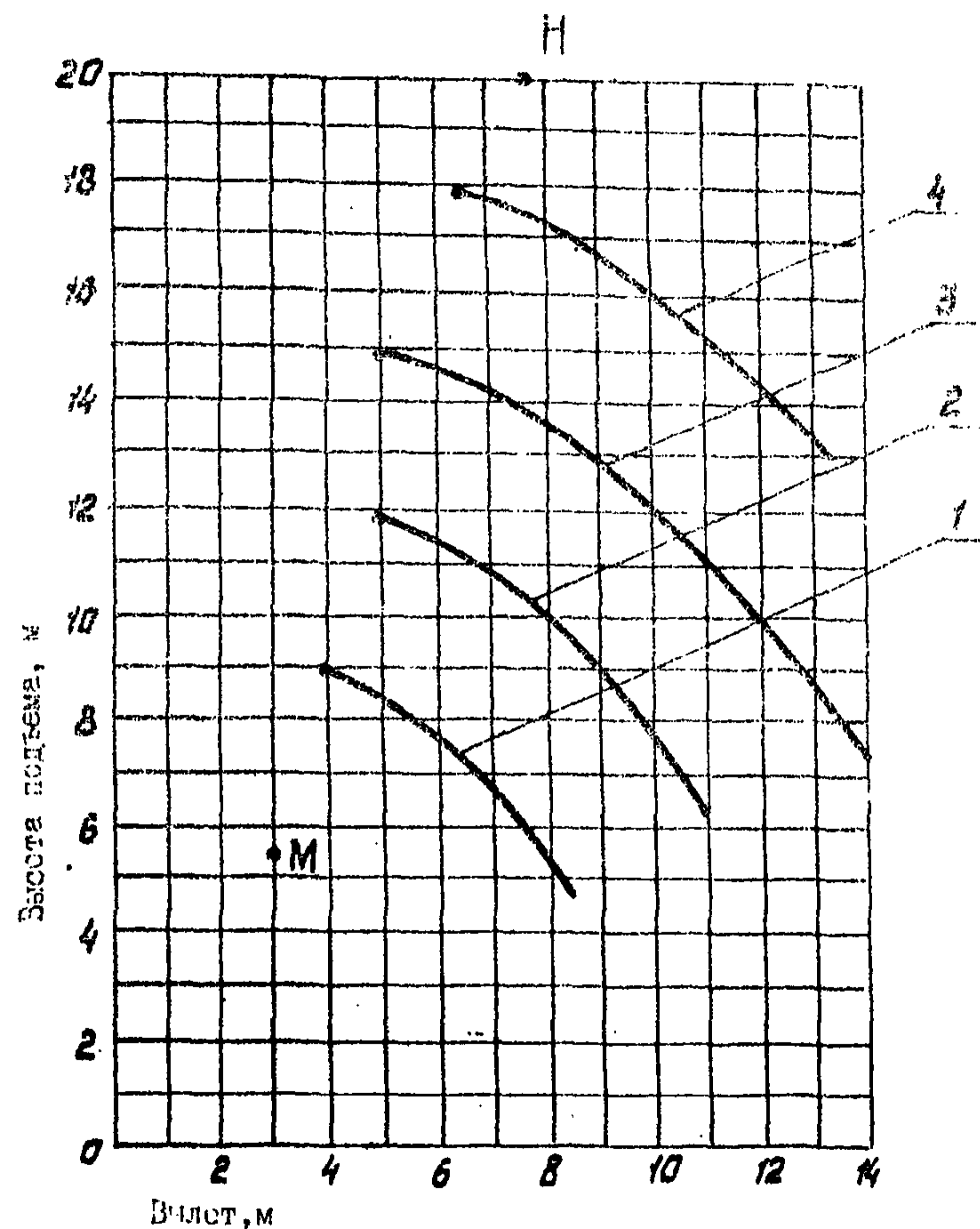
График высоты подъема
