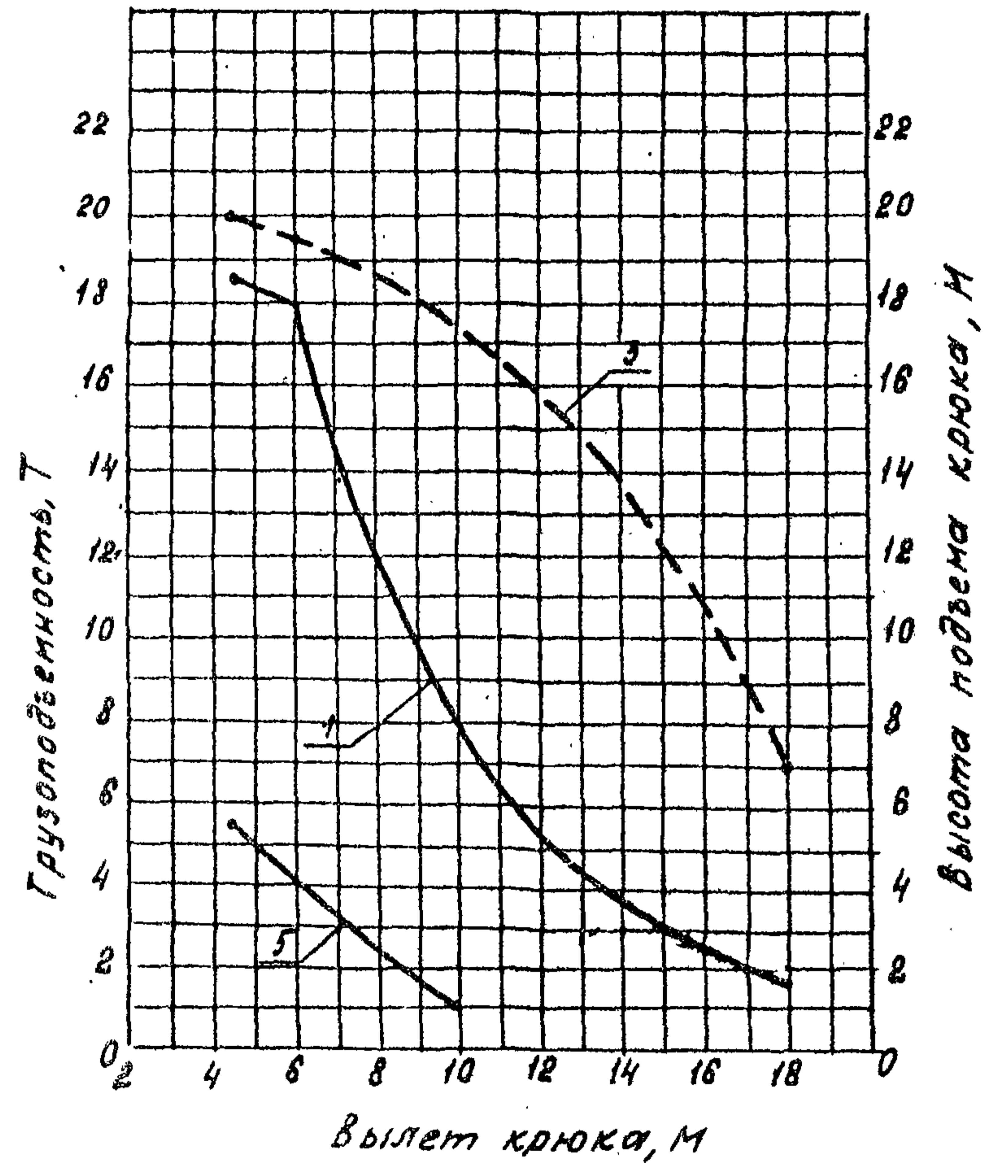
Стрела 20 м
