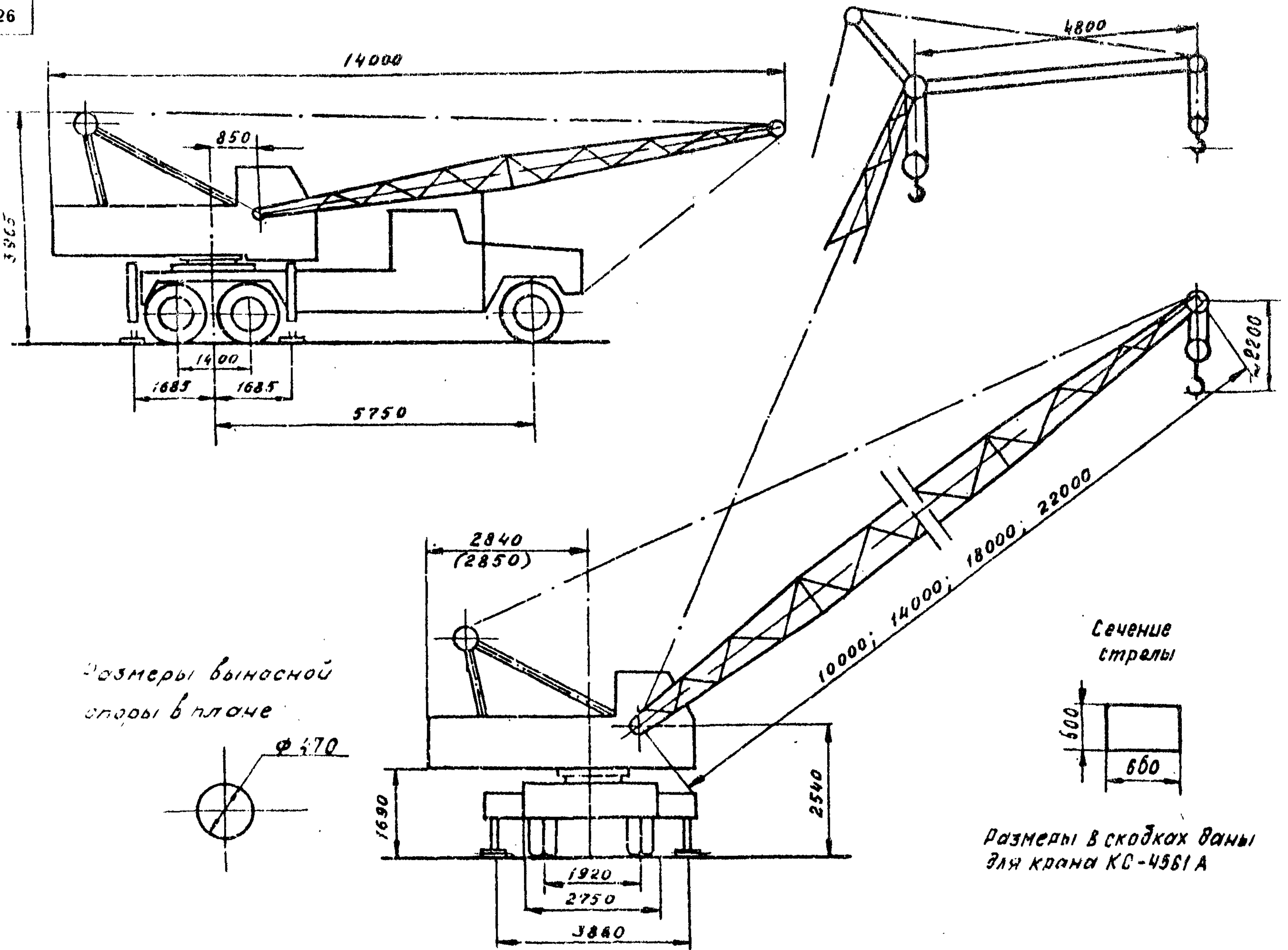
К-162 КС-4561А
