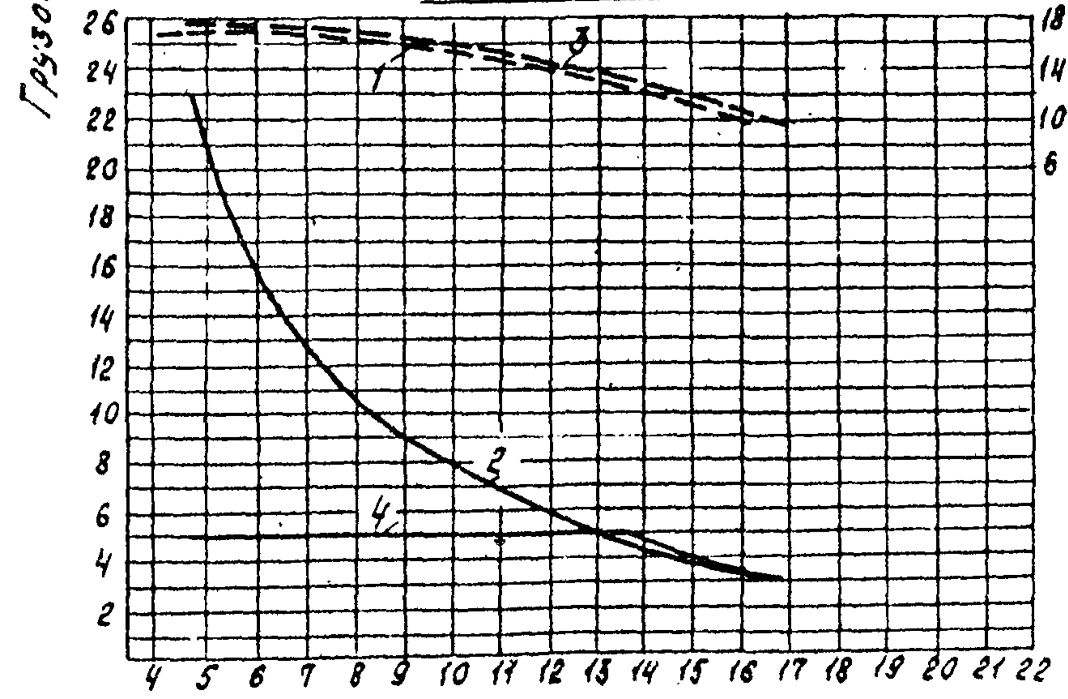
Стрела 17,5 м
