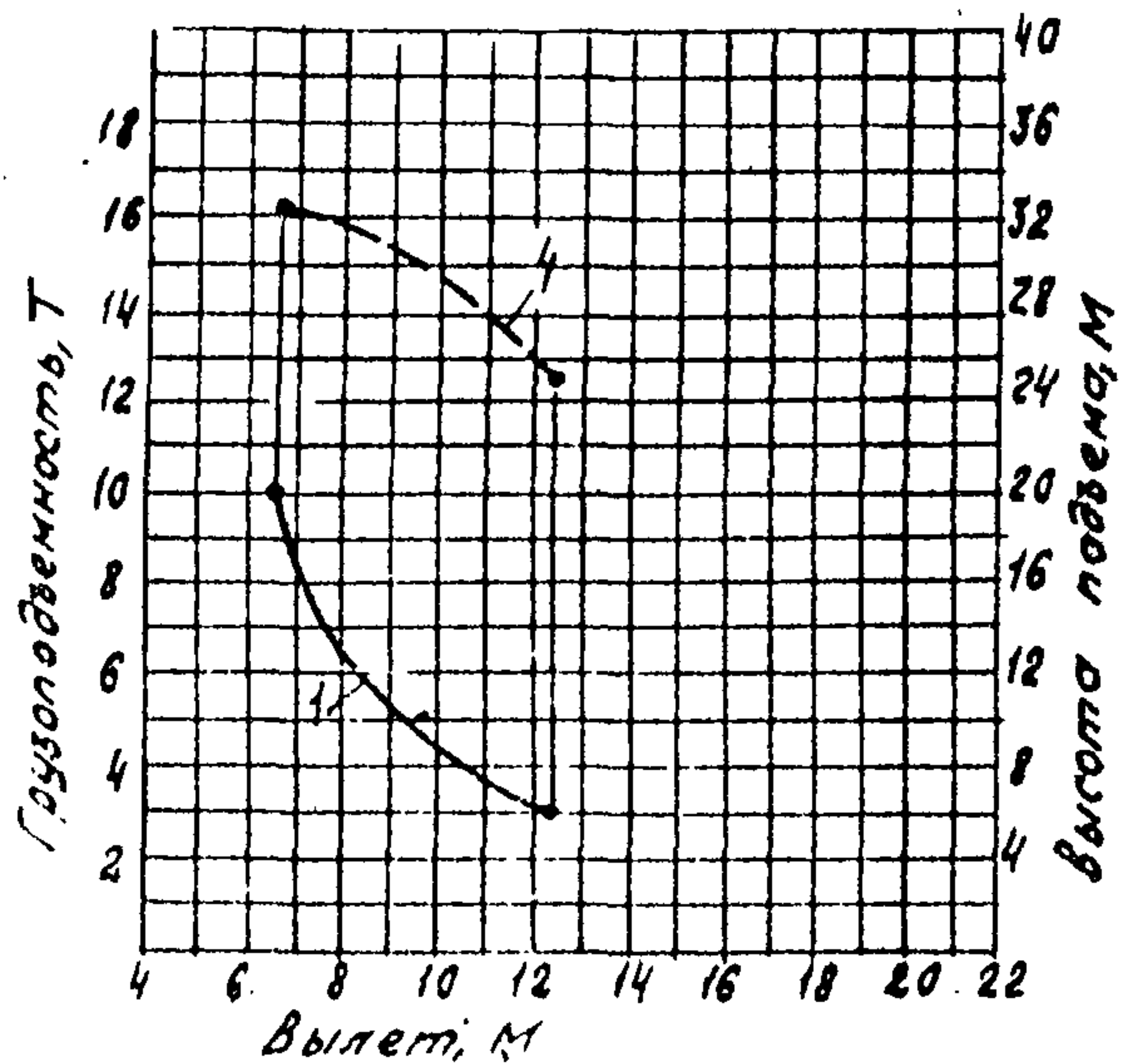
Башня 25 м, гусек 10 м
