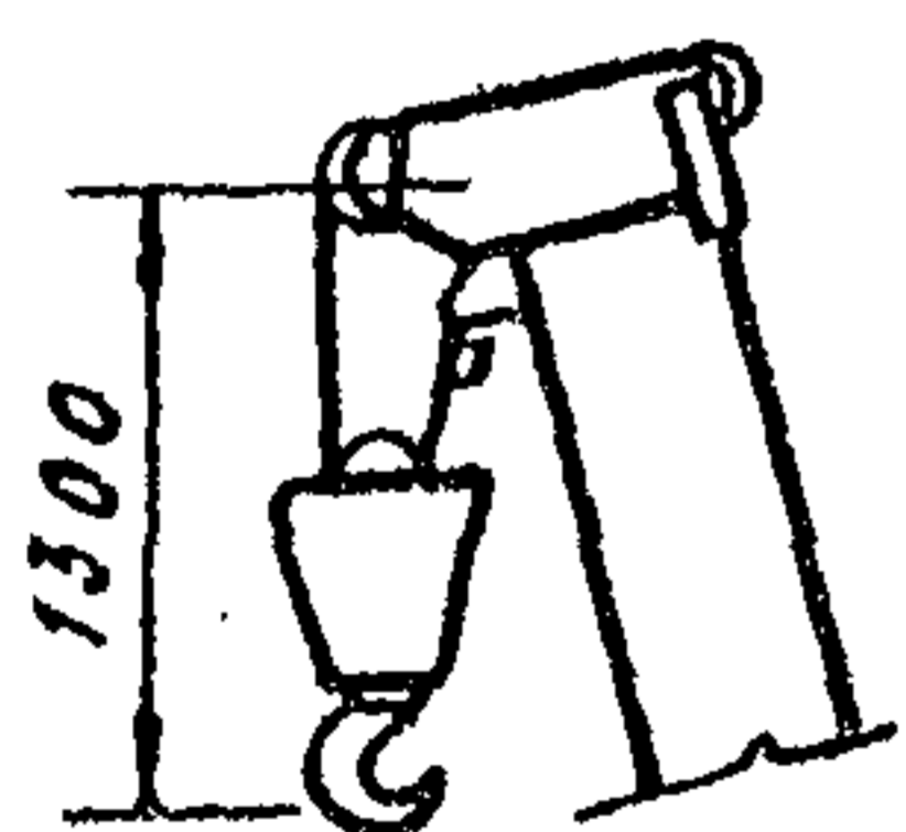
Главный крюк
