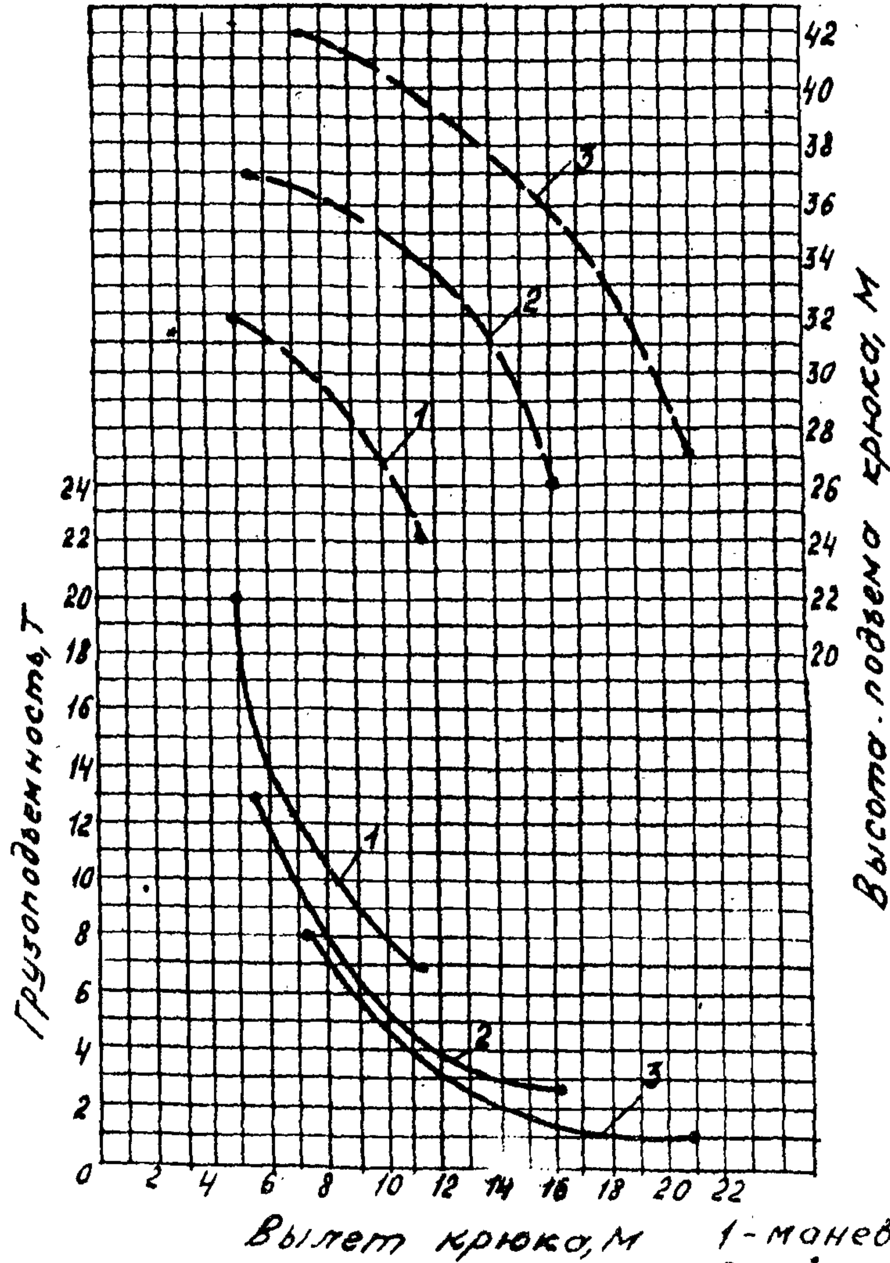
Башня 23,5 м
