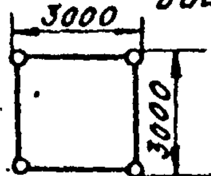
Наружный габарит башни
