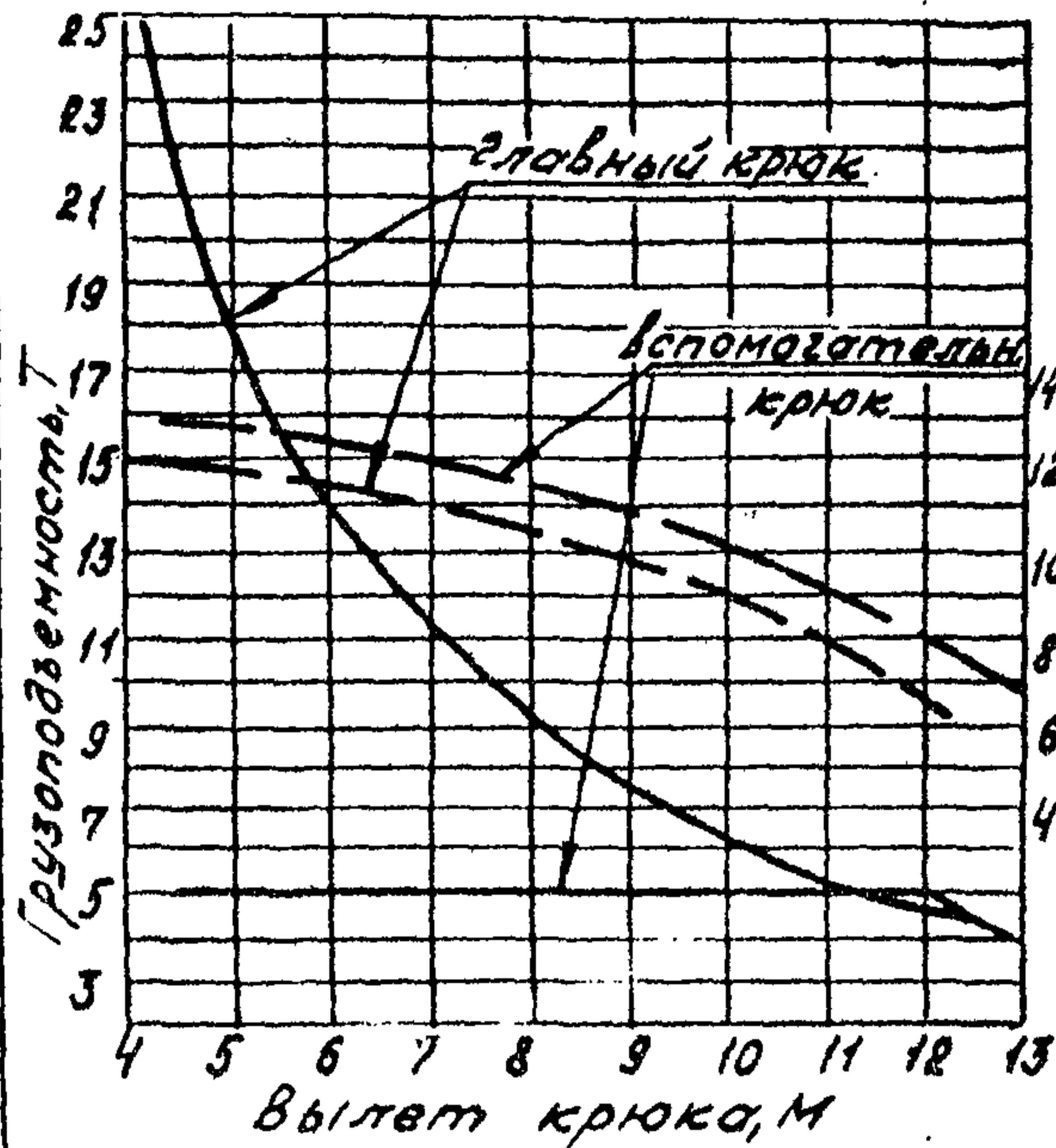
Стрела 12,5 м с гуськом 5 м
