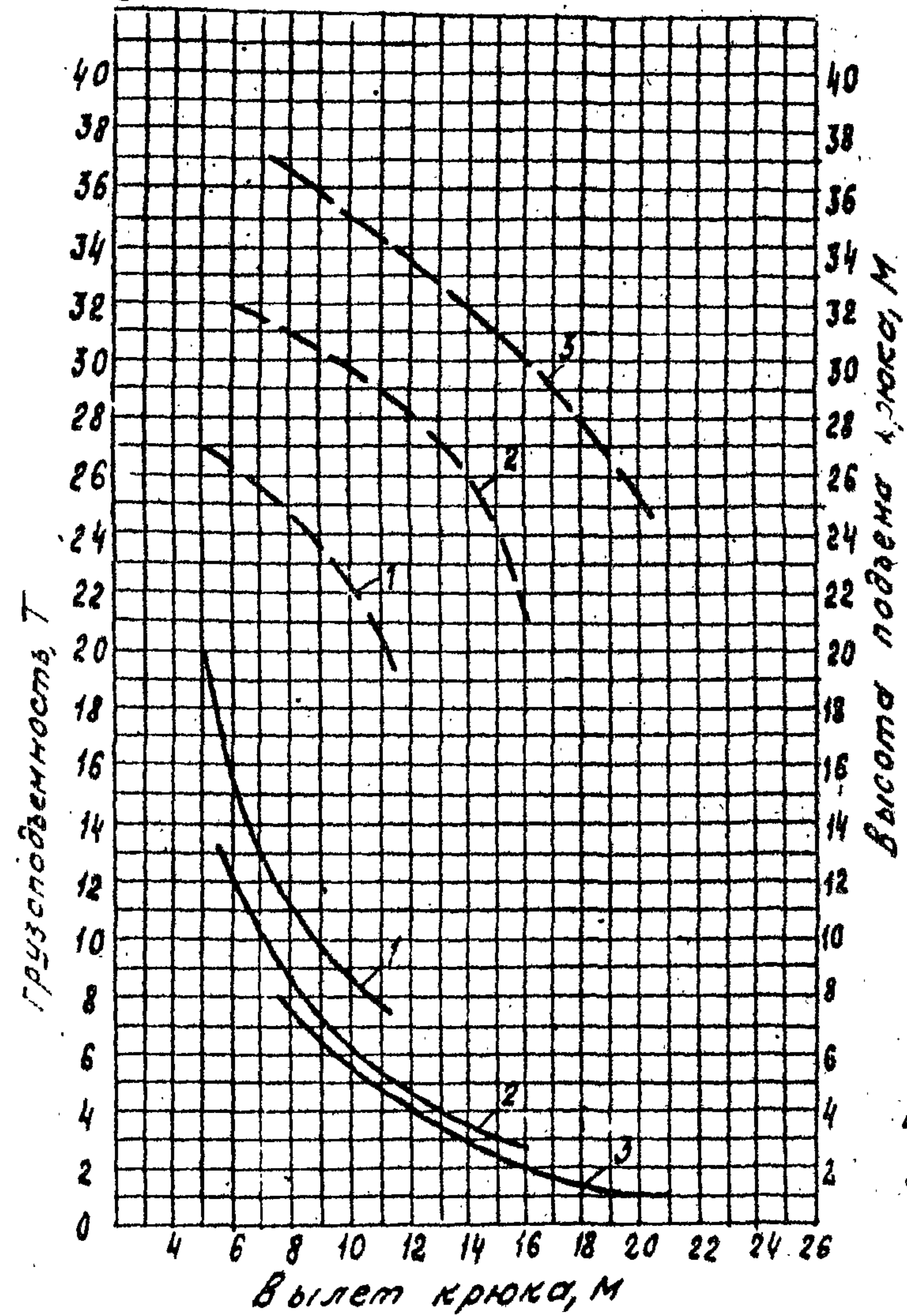
Башня 18,5 м
