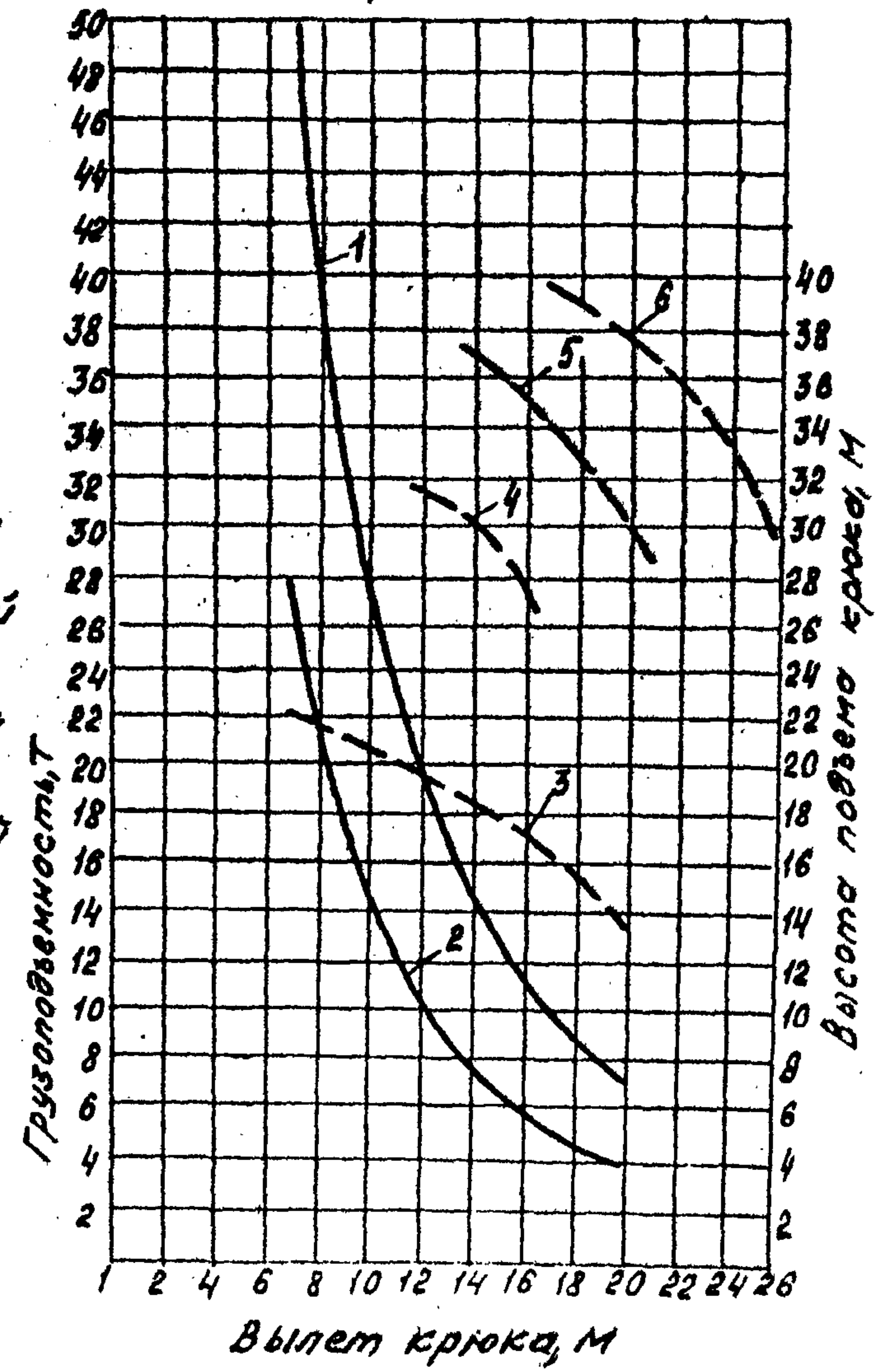
Стрела l=25\text{ м}
