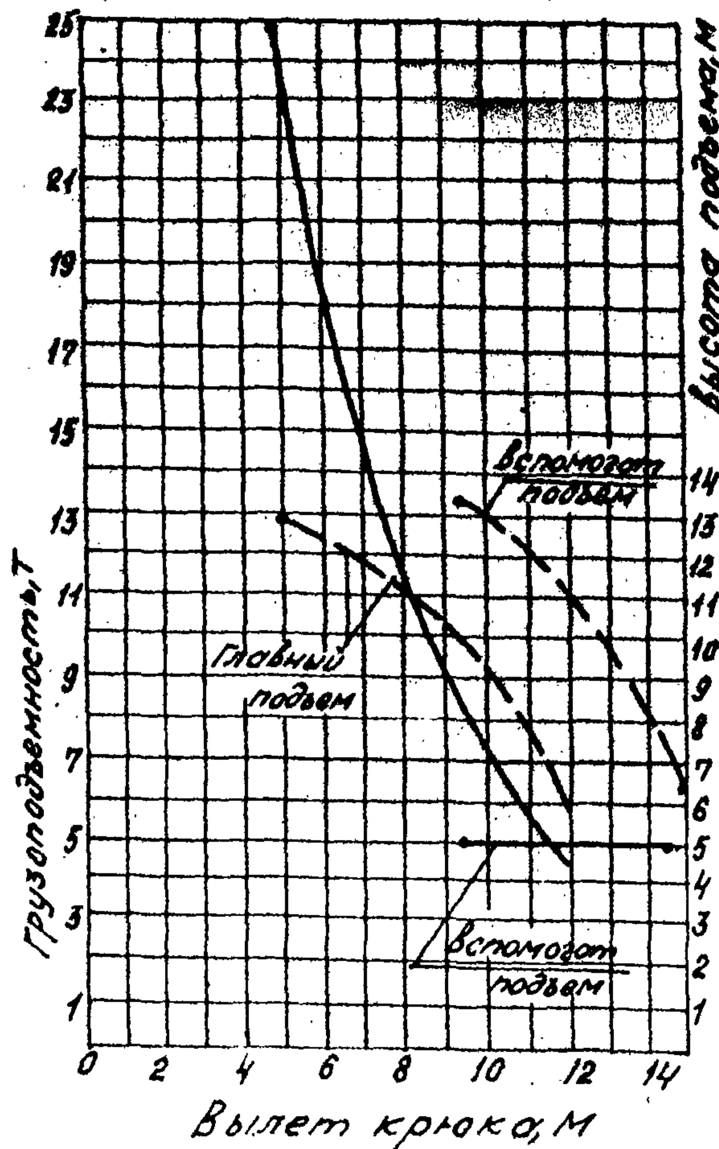
Стрела 13,5 м с жестким гуськом 5 м
