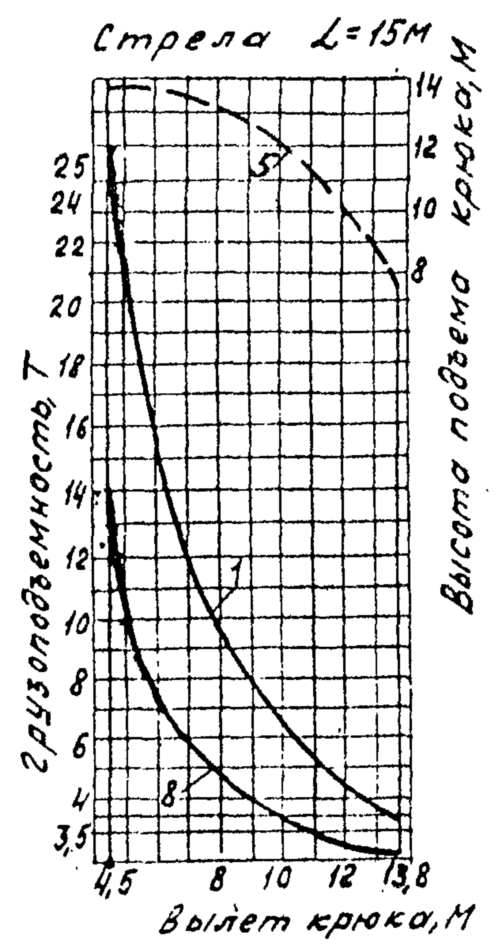
Графики грузоподъемности
