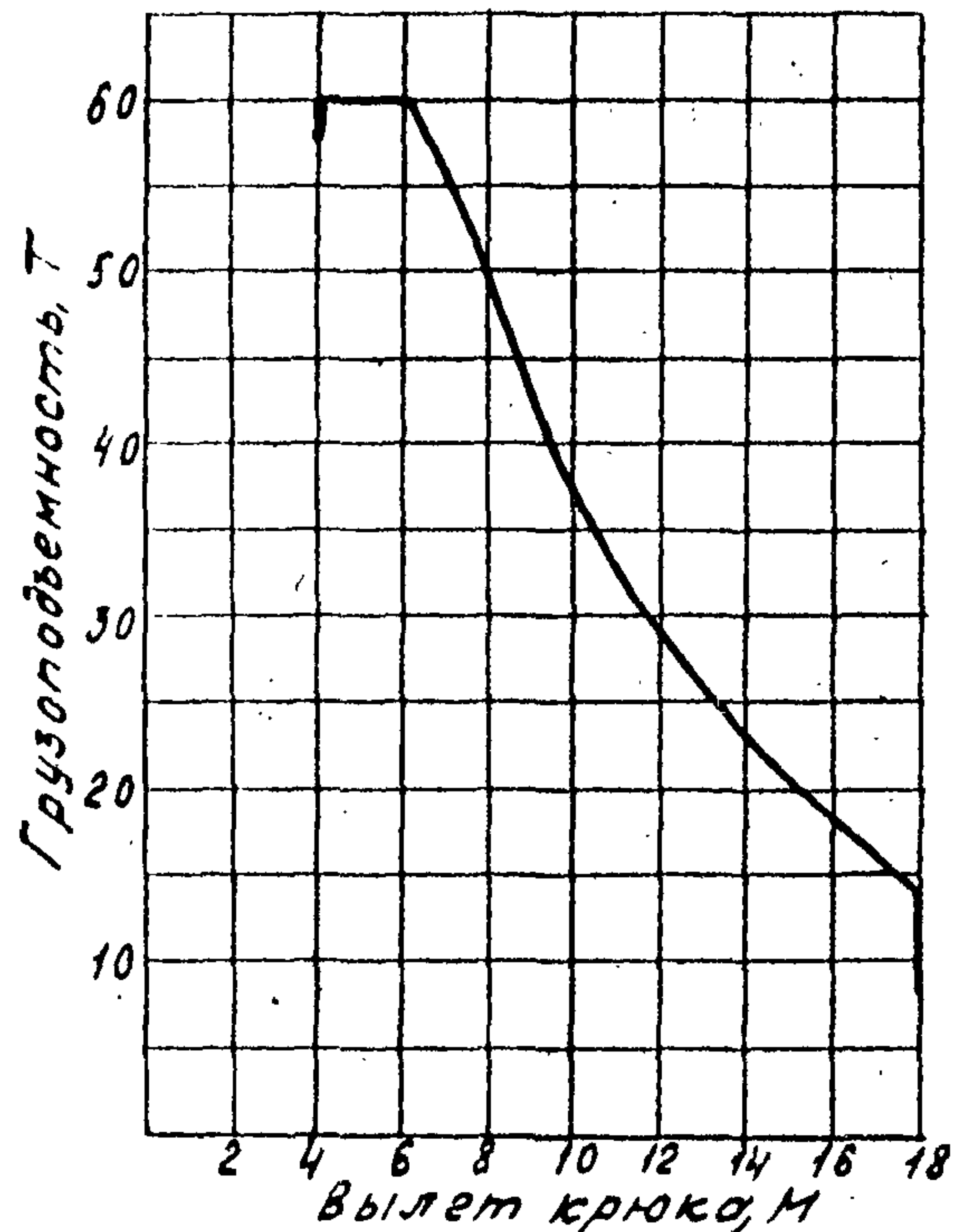
Стрела 20 м
