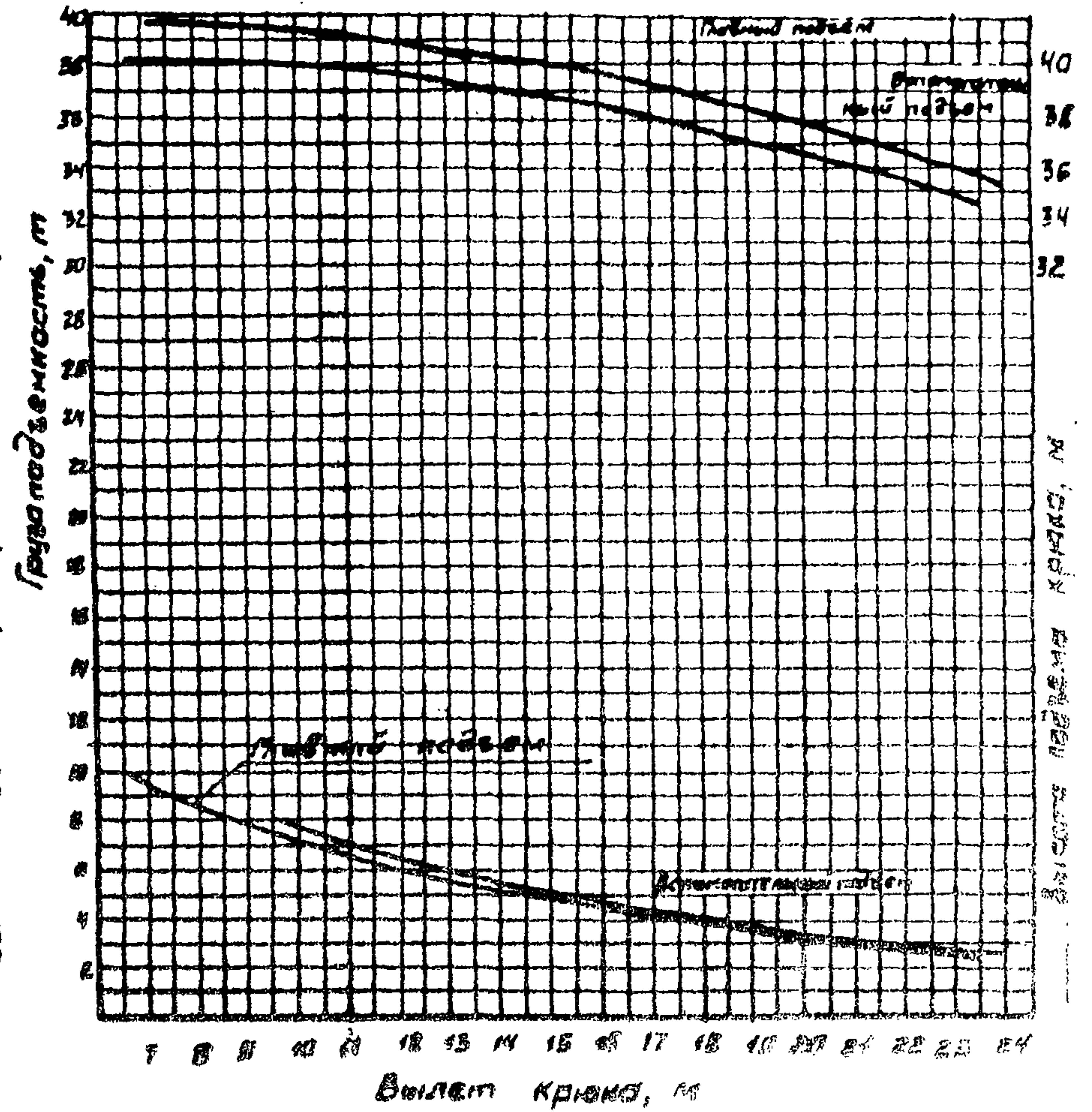
Стрела 41 м без гуська
