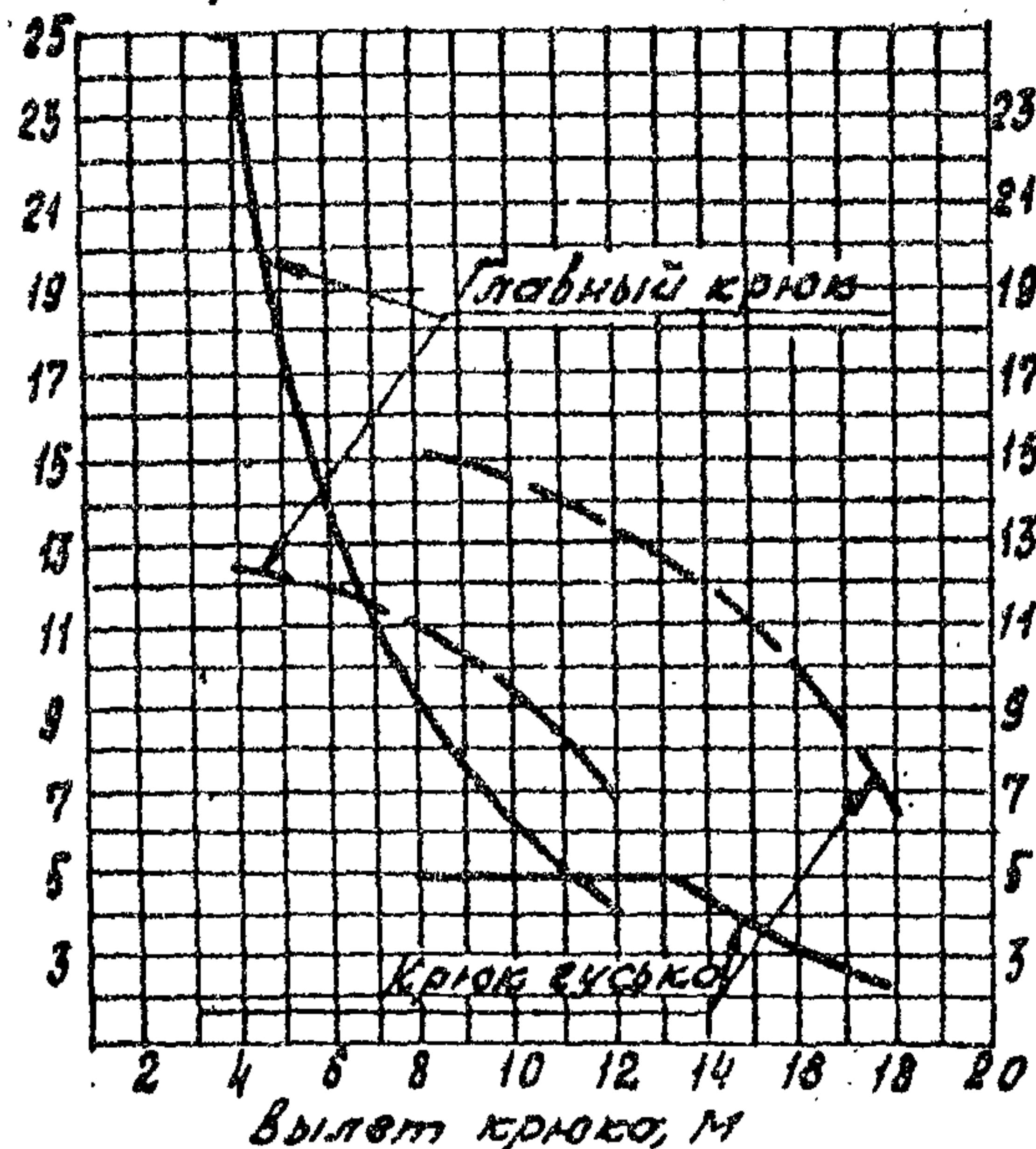
Стрела, 27,5 м
