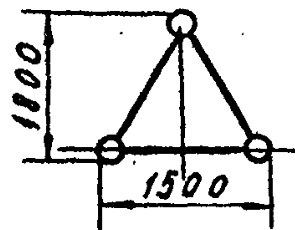
Наружные габариты башни
