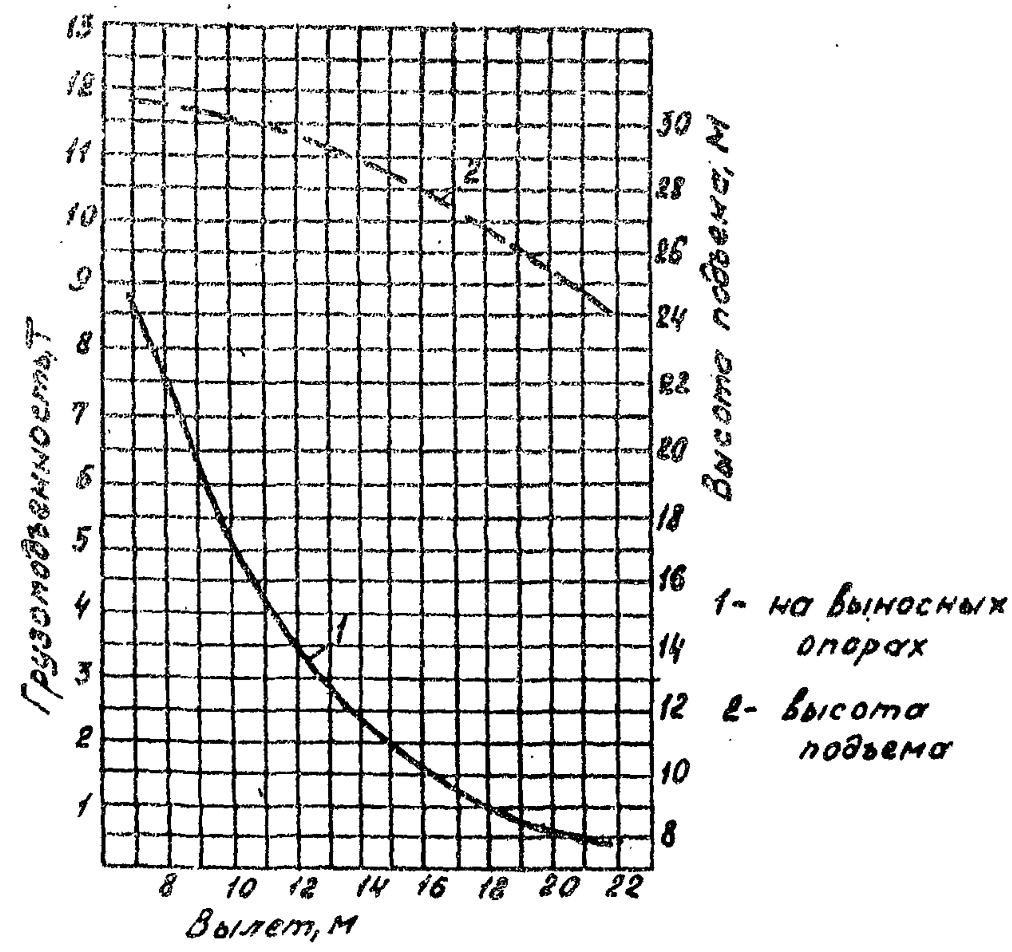
Графики грузоподъемности "высоты подъема" в зависимости от вылетов для стрелы 32,5м
