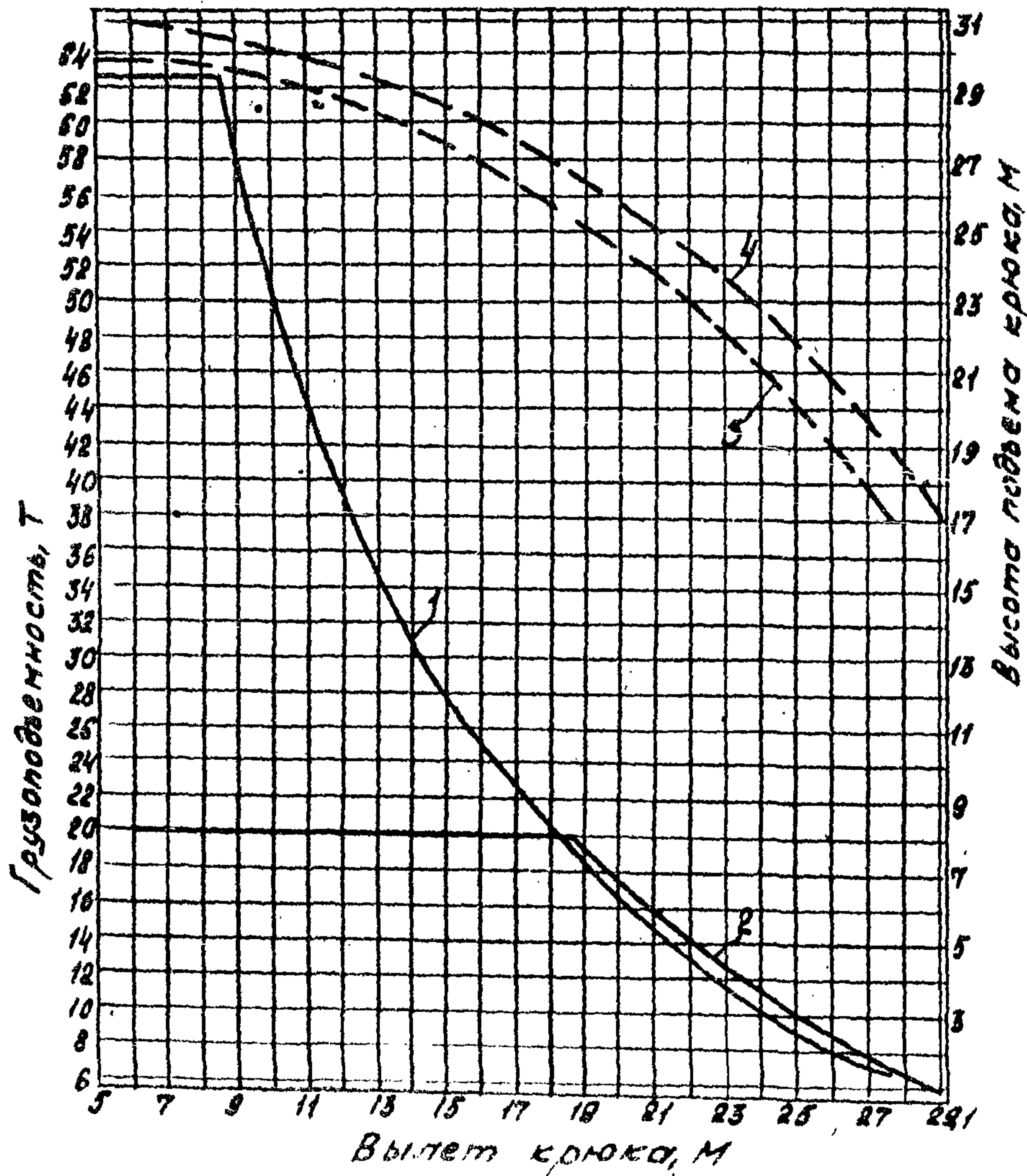
Стрела 31м
