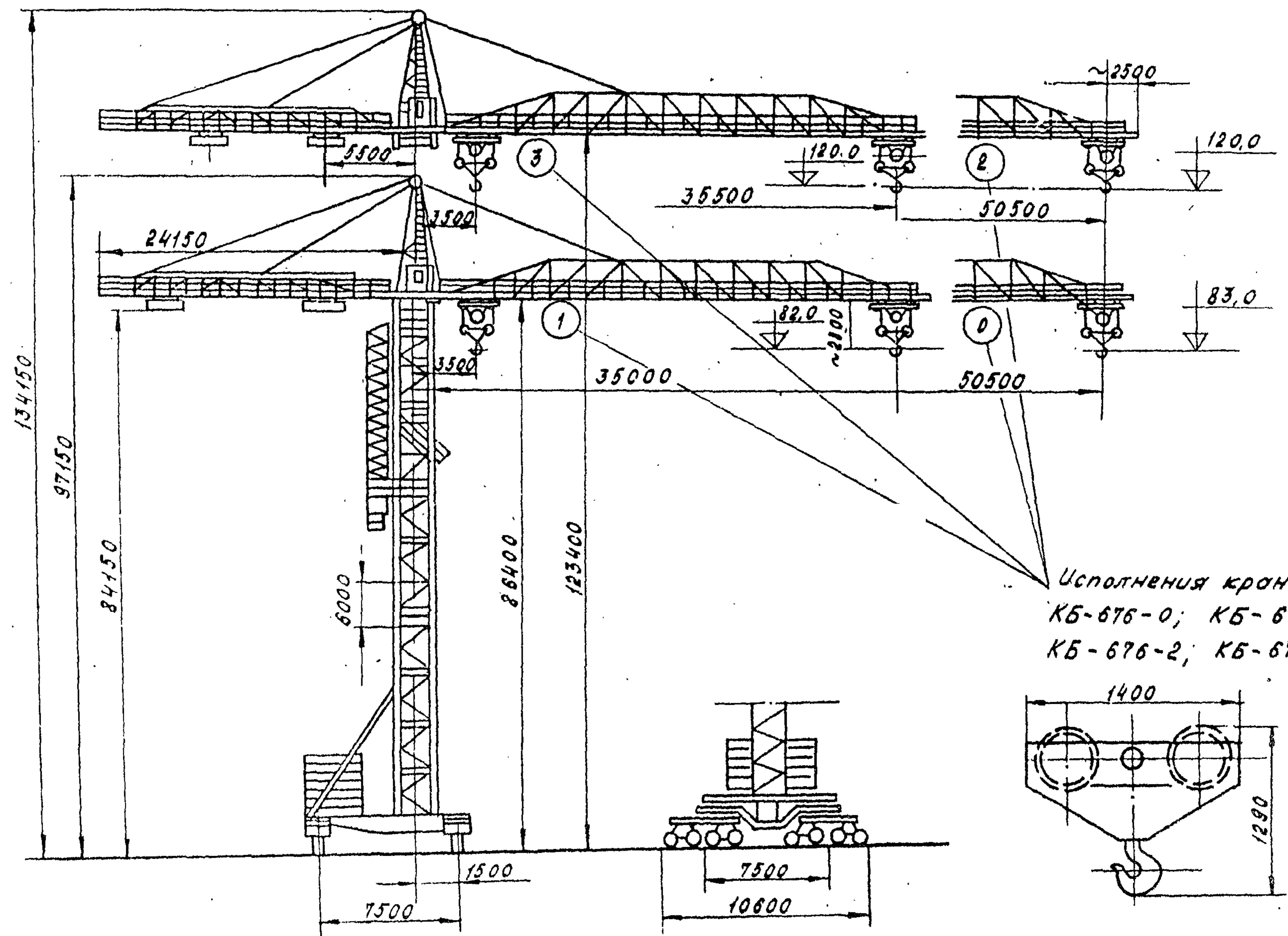
КБ-676
