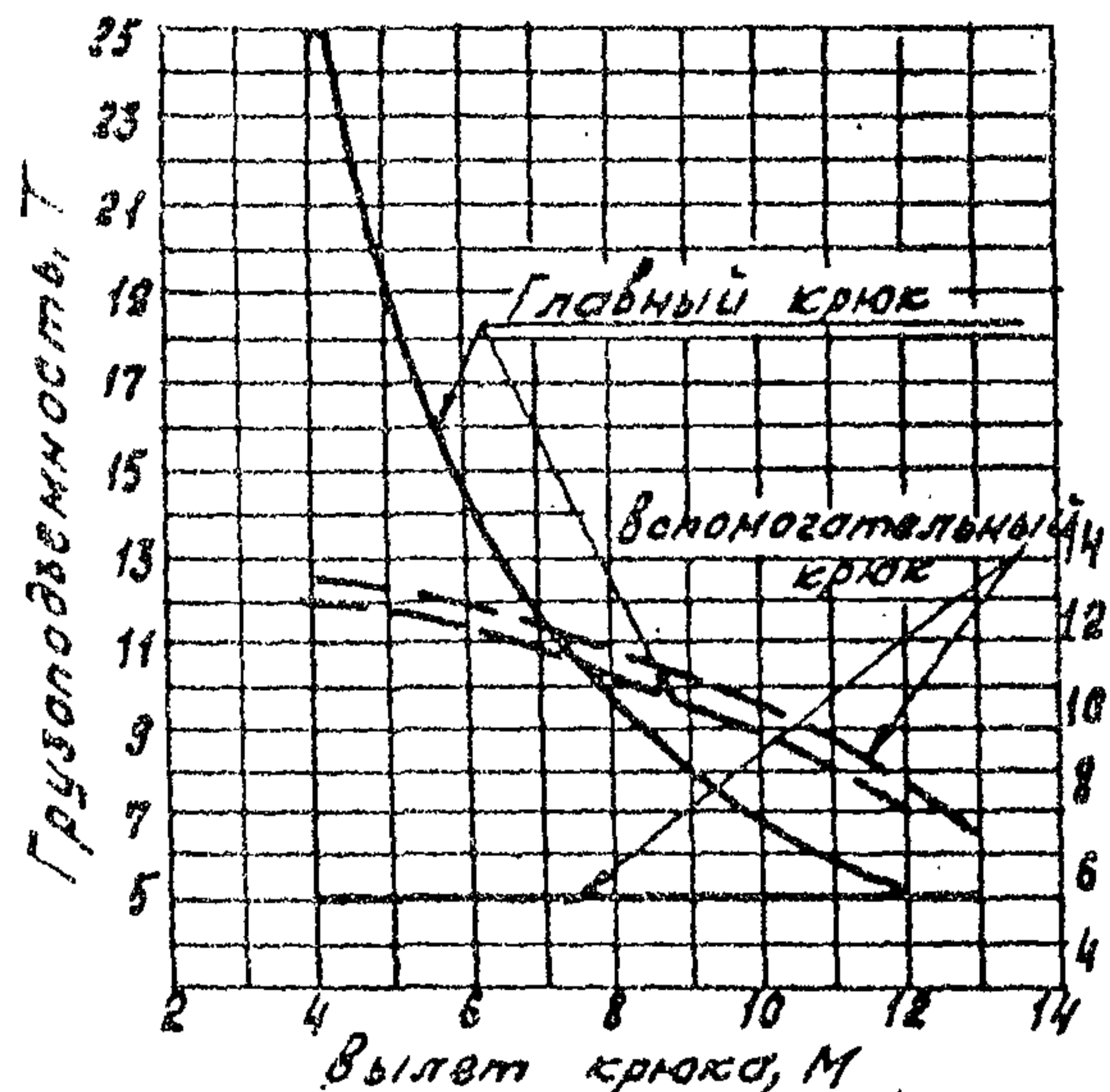
Стрела 22,5 м
