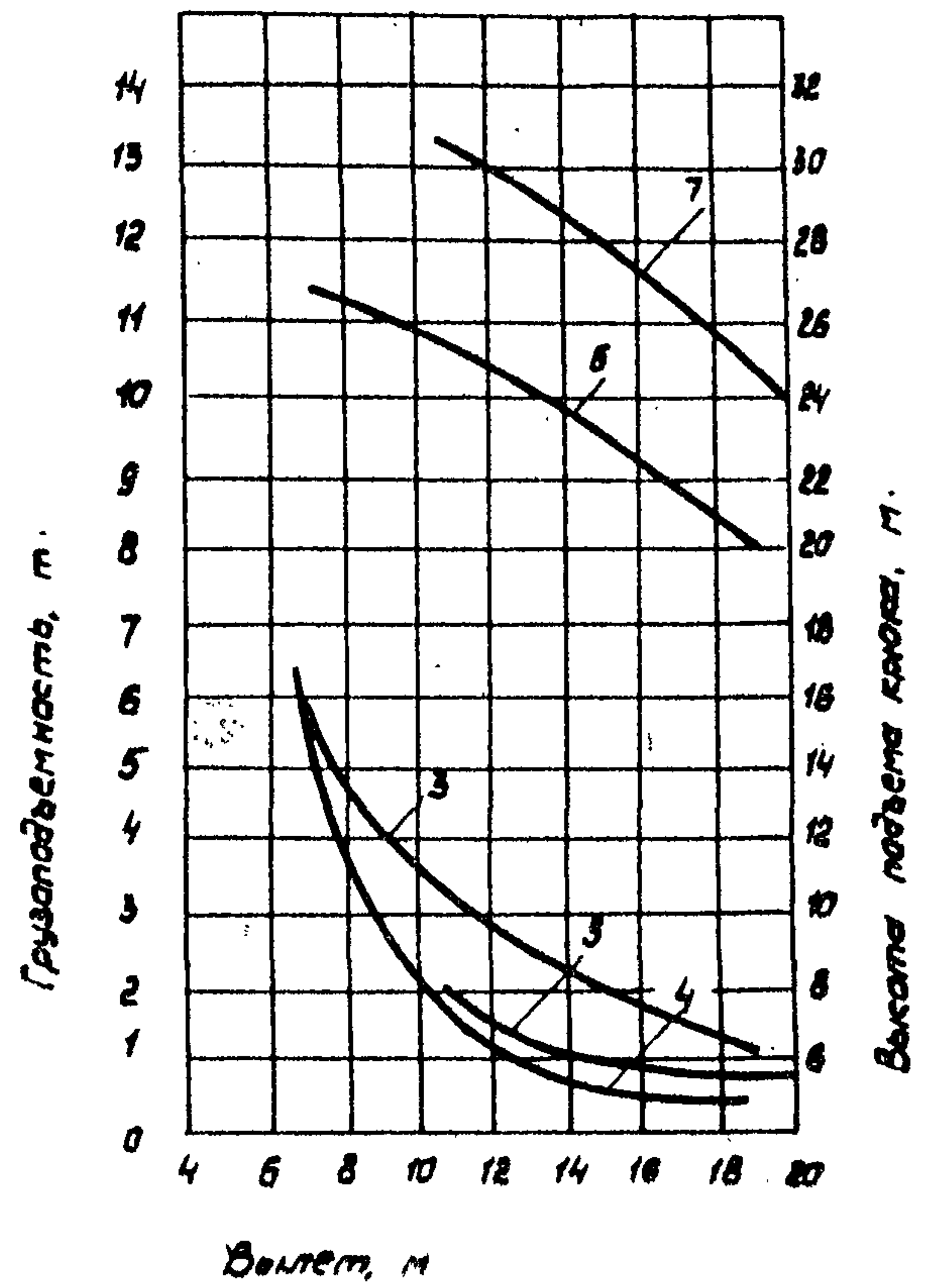
Стрела 26м с гуськом
