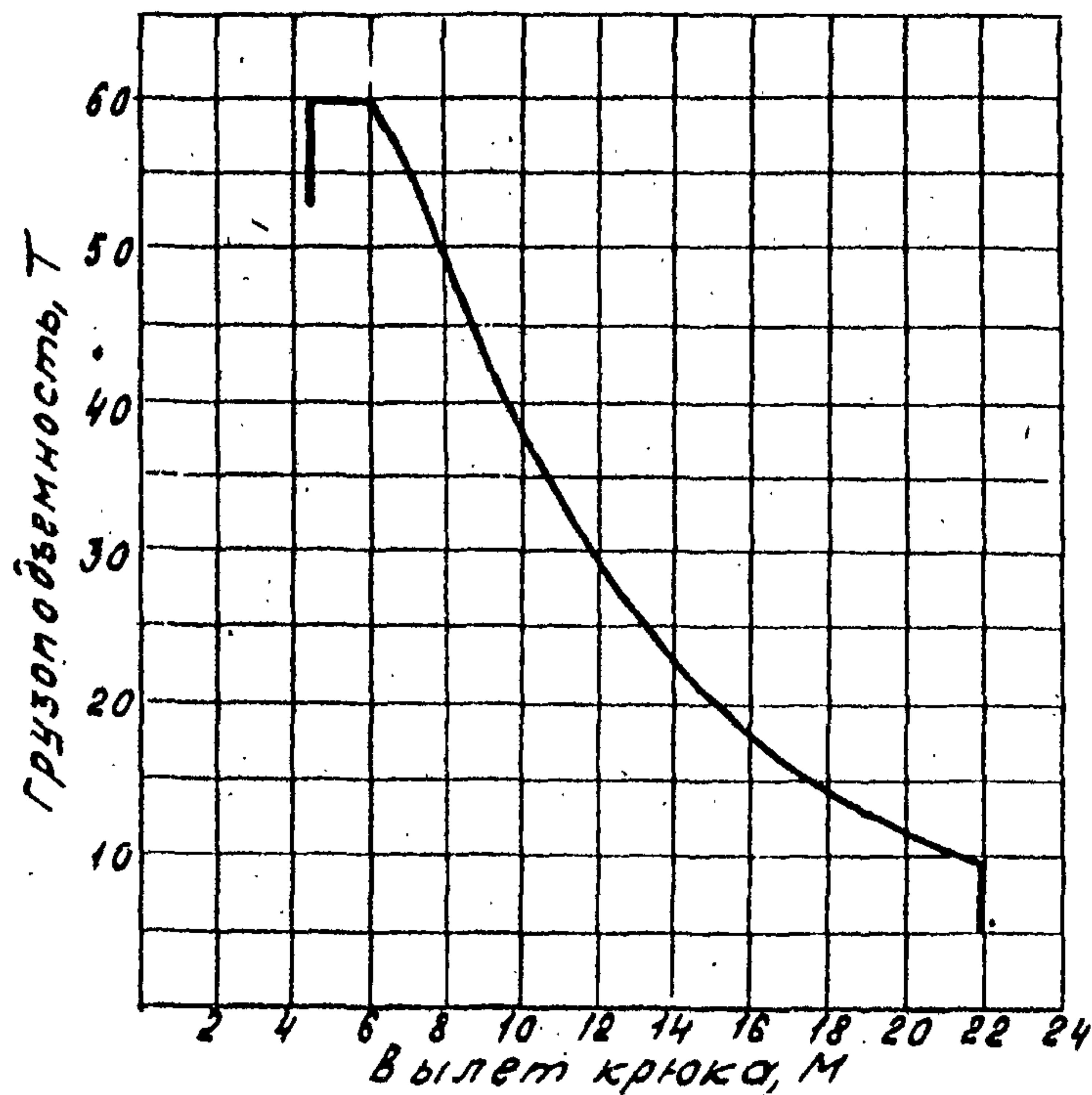
Стрела 45,2
