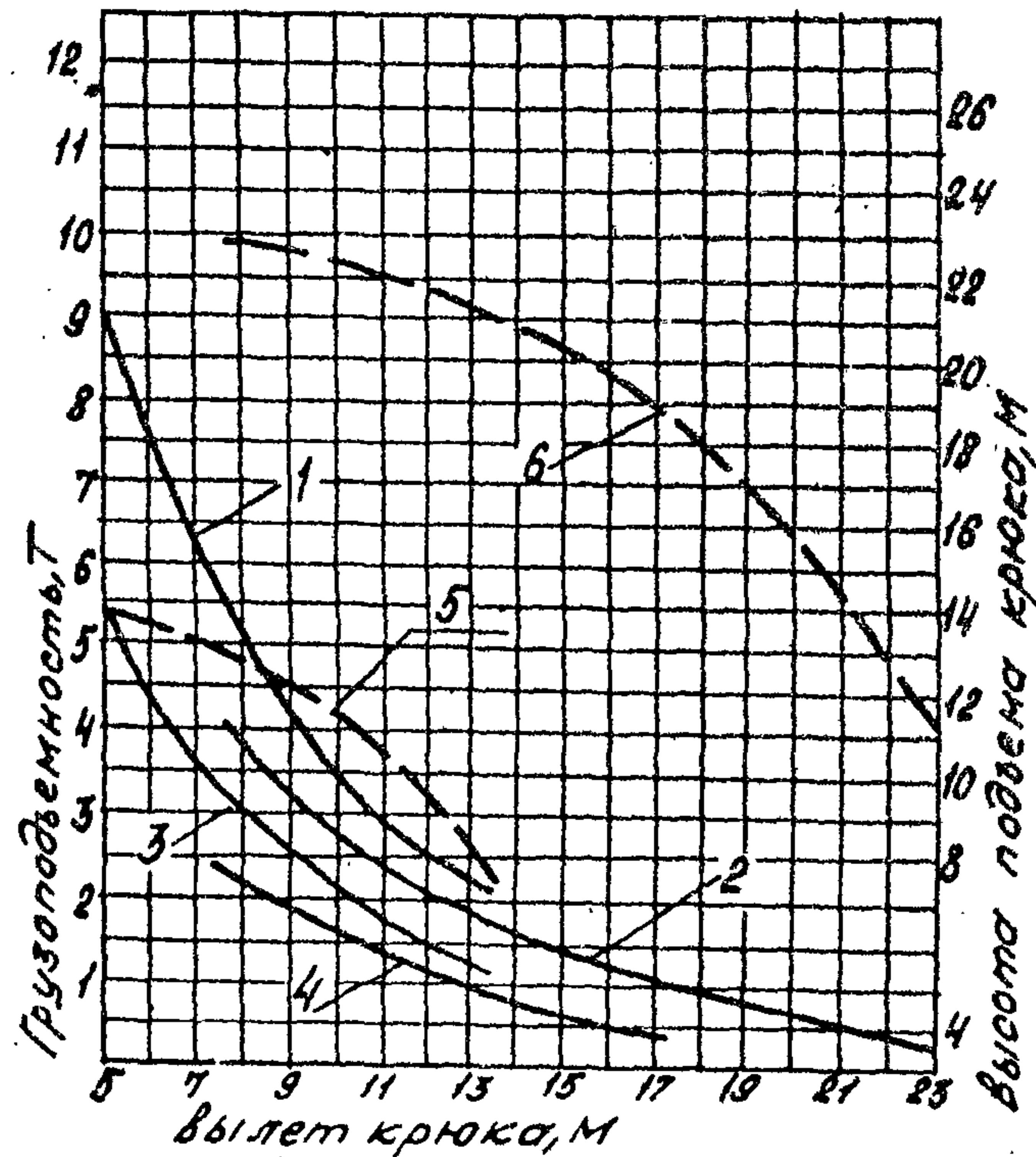
Графики грузоподъемности
