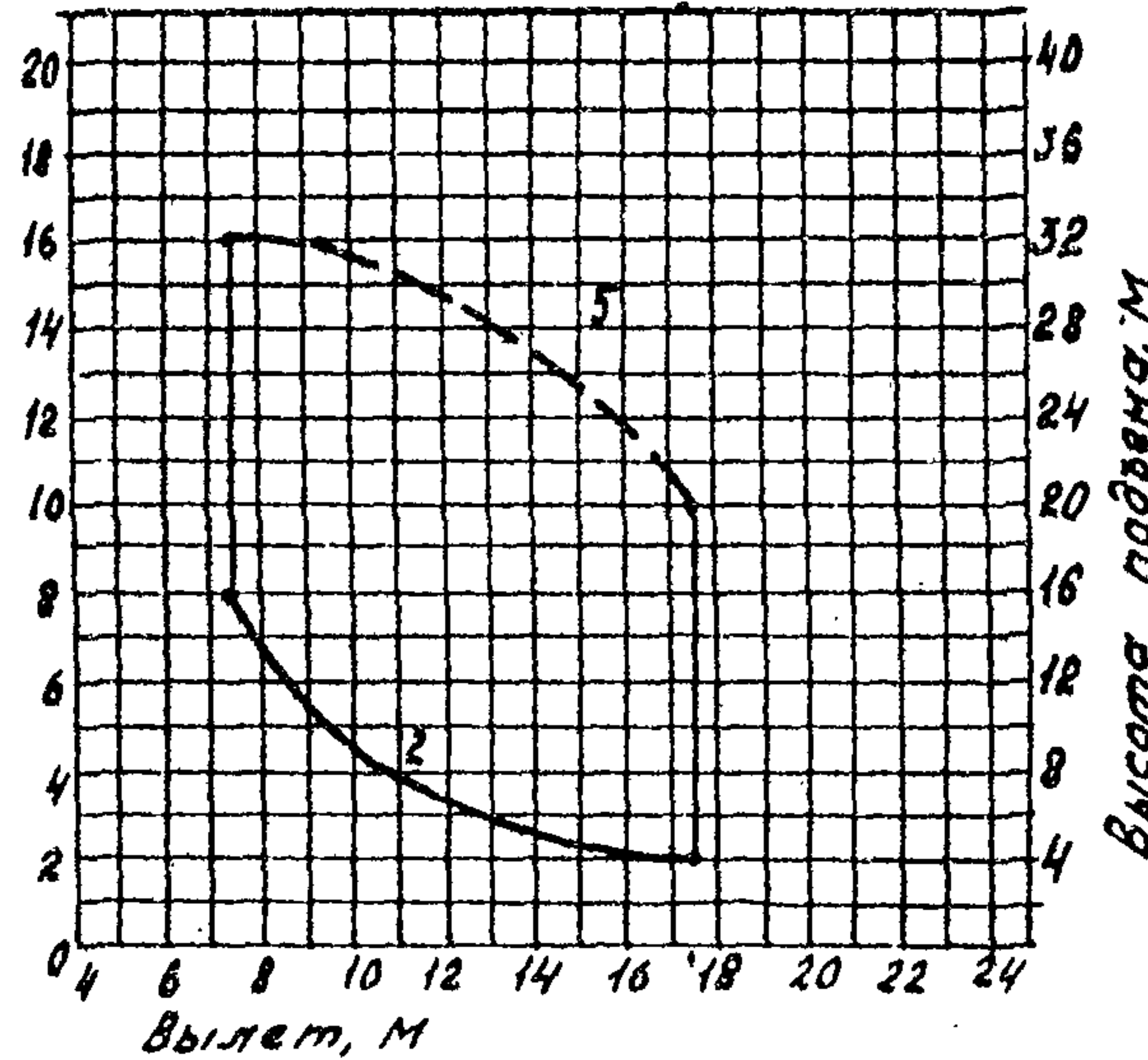
Башня 20м гусек 15м
