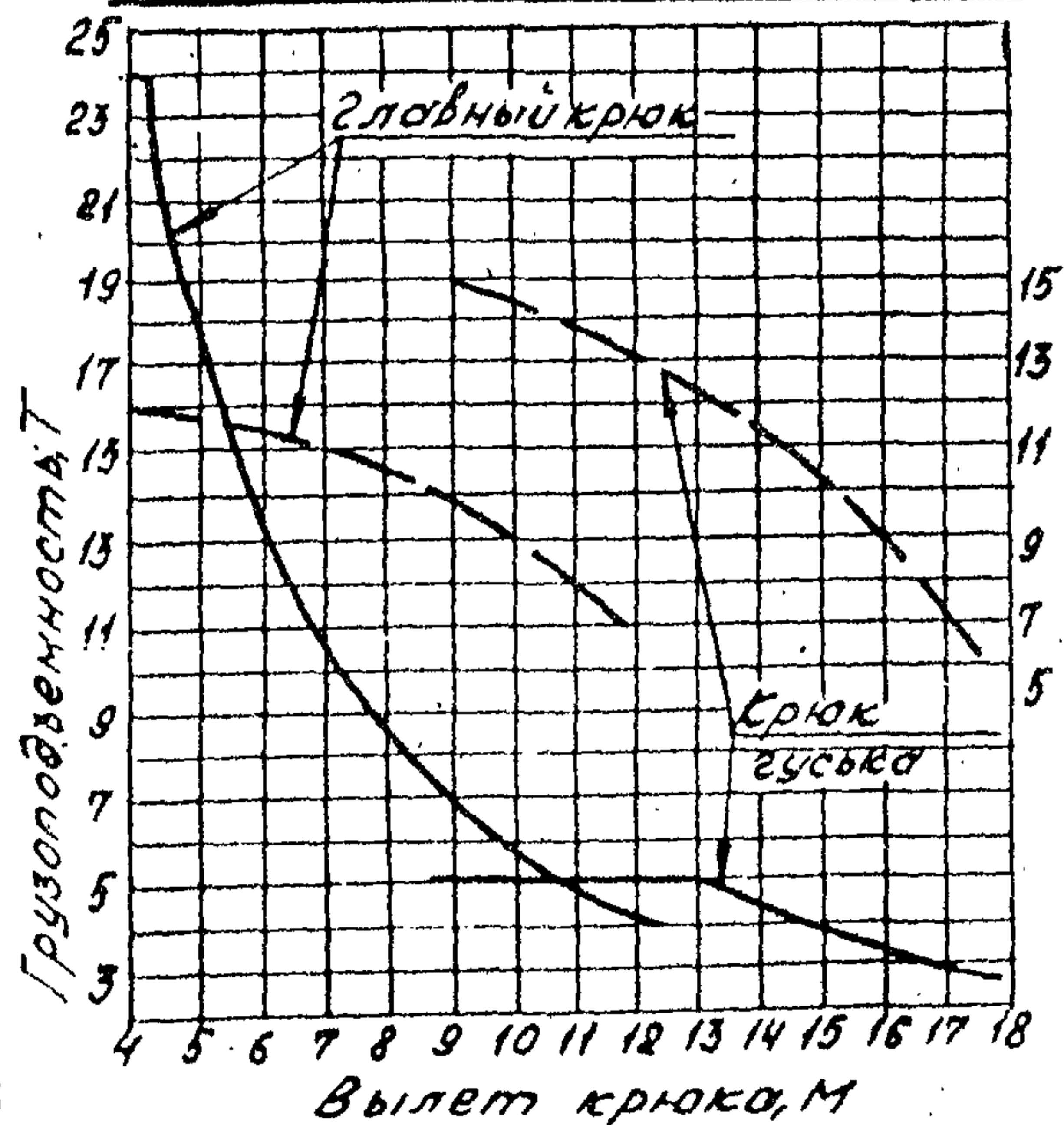
Стрела 12,5 м с гуськом 5 м
