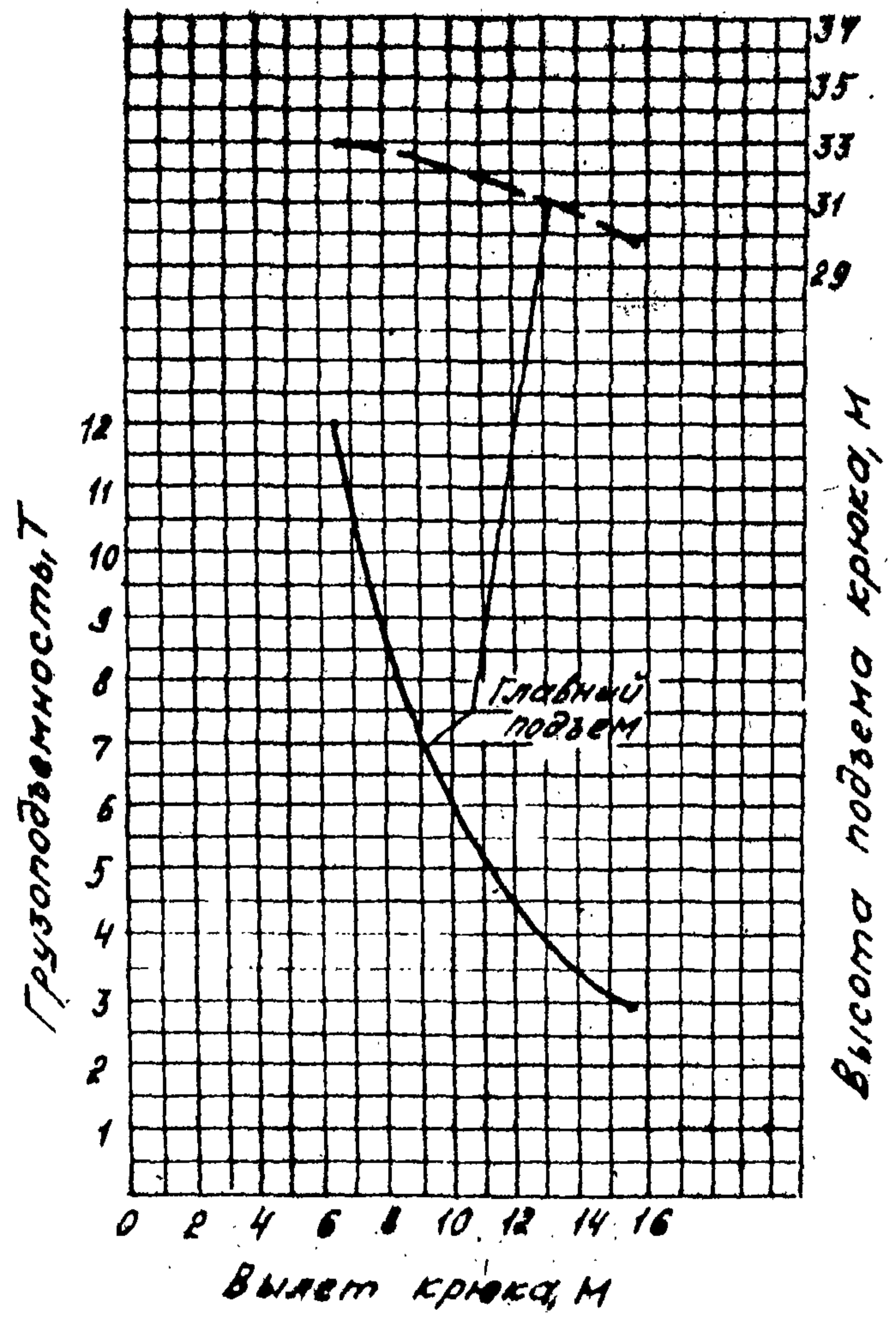
Стрела 33,5 м
