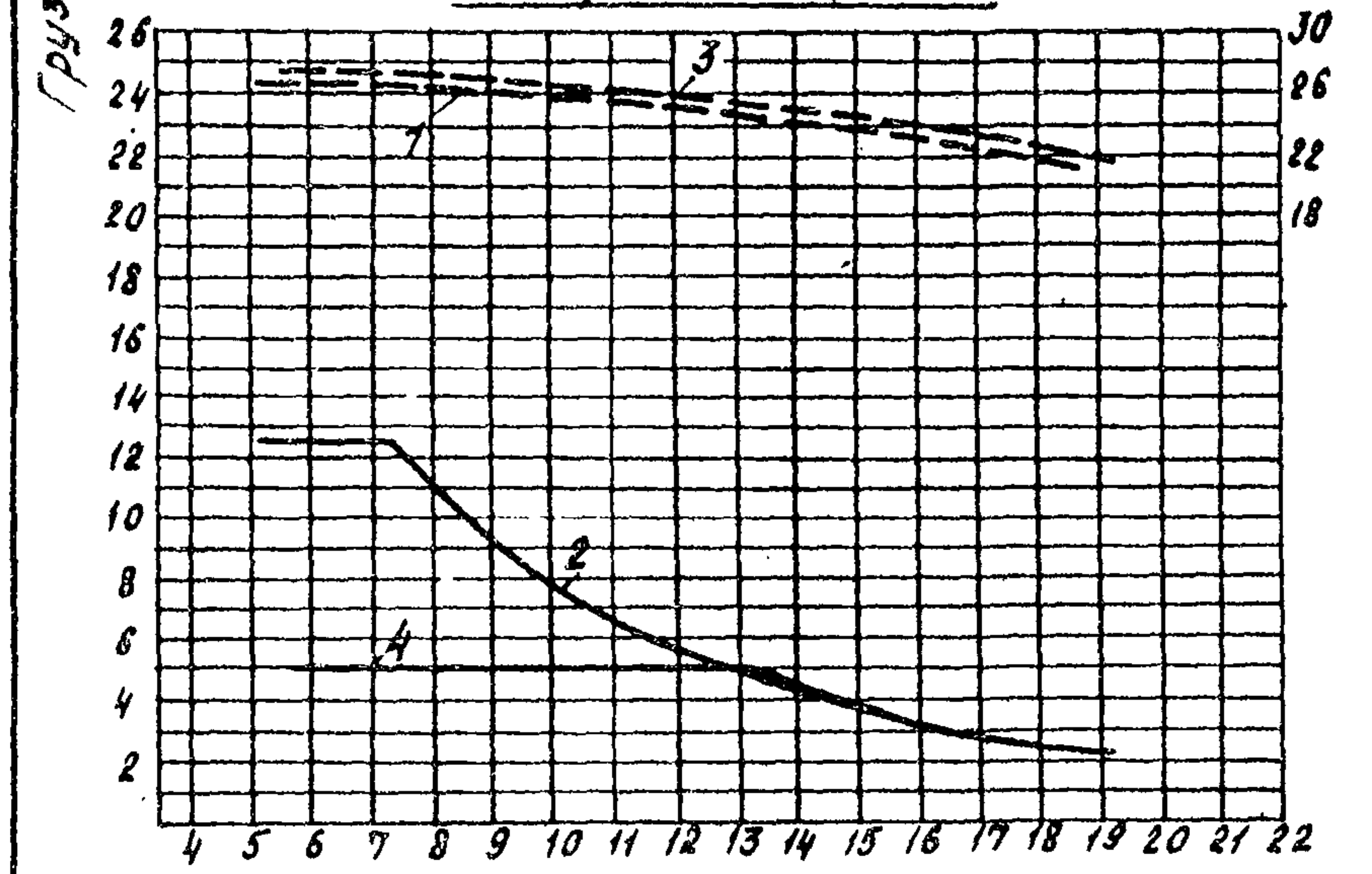
Стрела 27,5м
