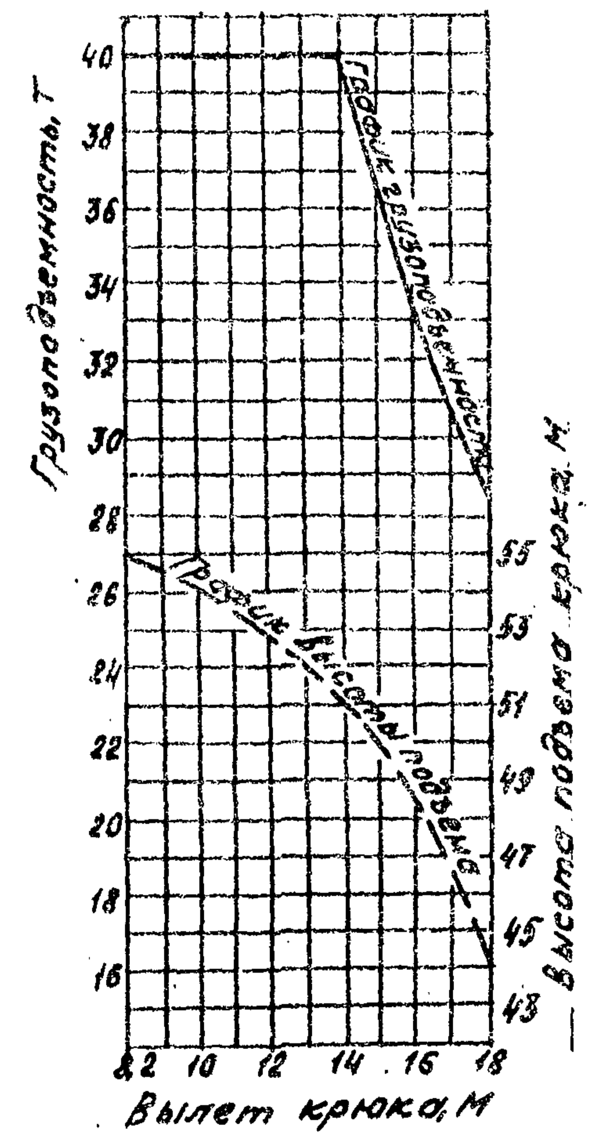
Стрела 41м с гуськом 16м
