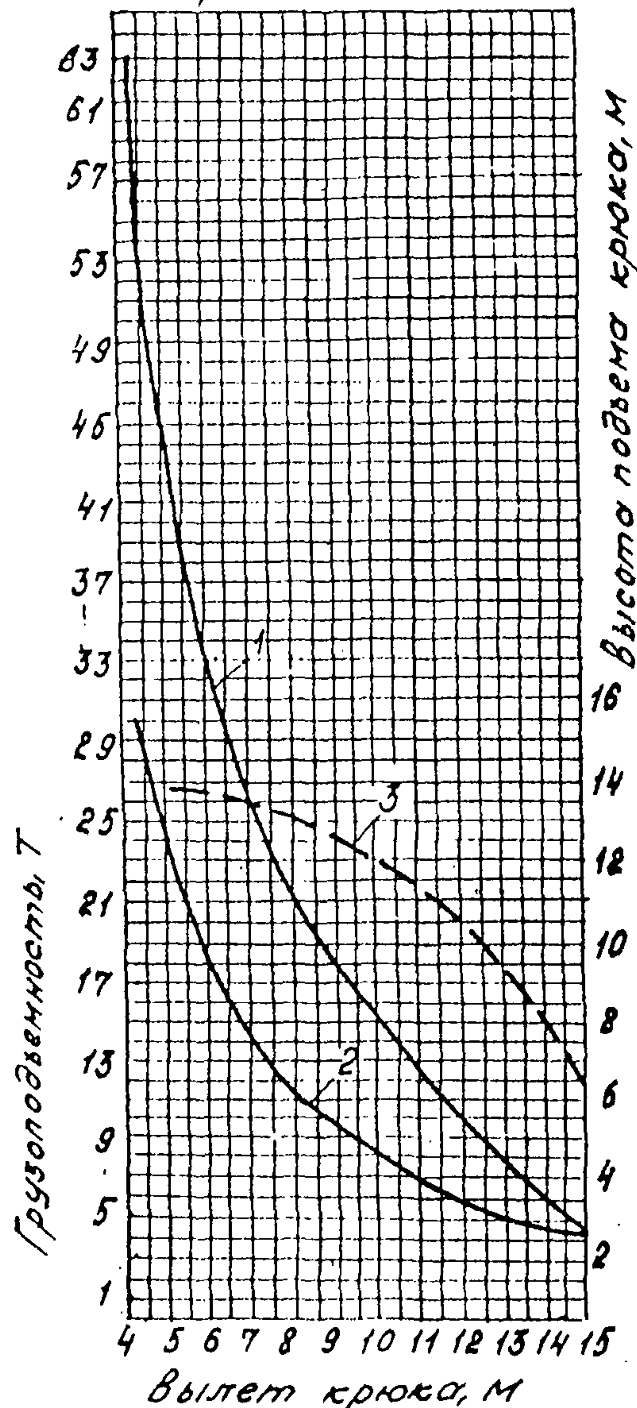
Стрела 15 м
