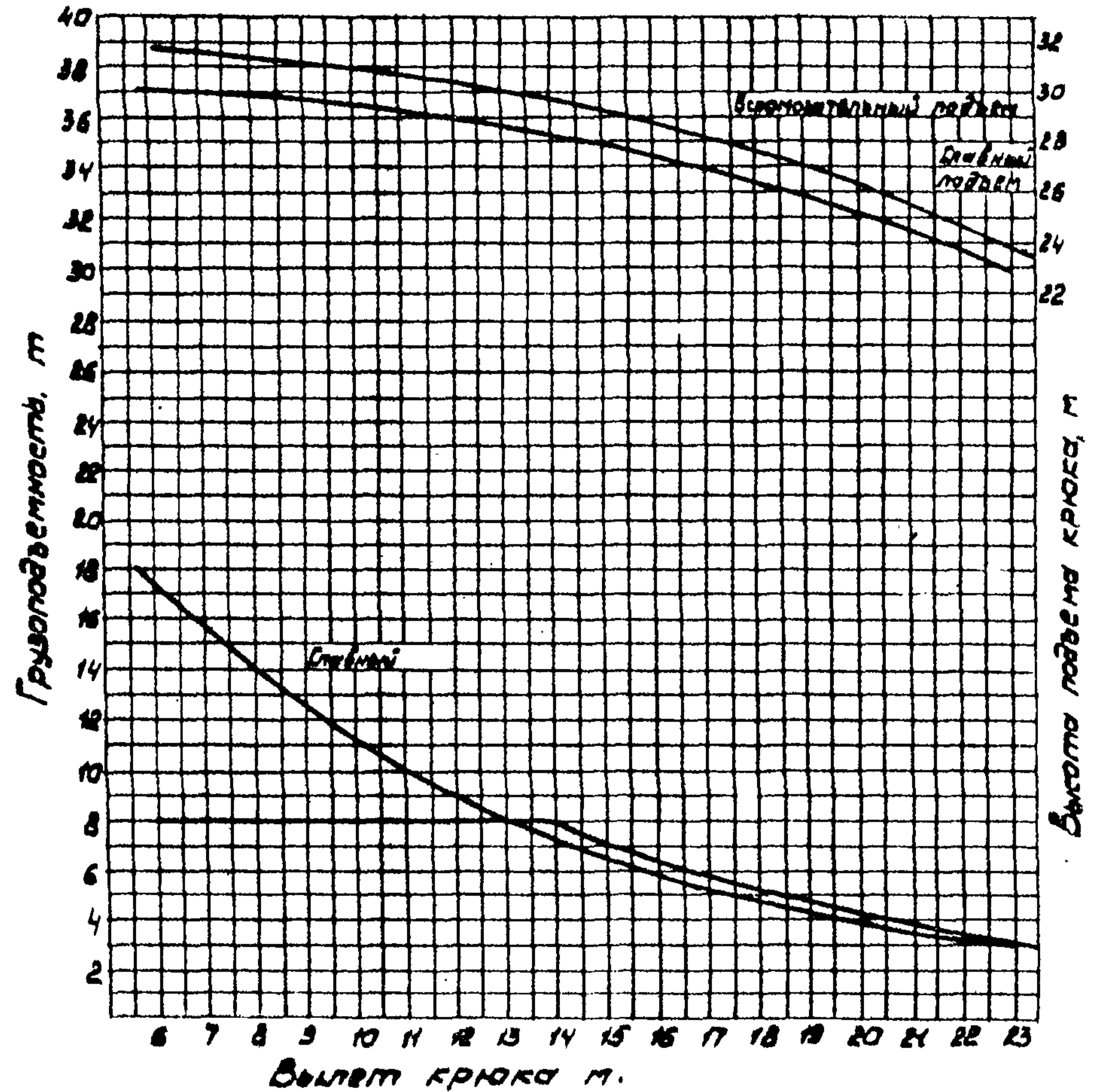
Стрела 31 м без вышка
