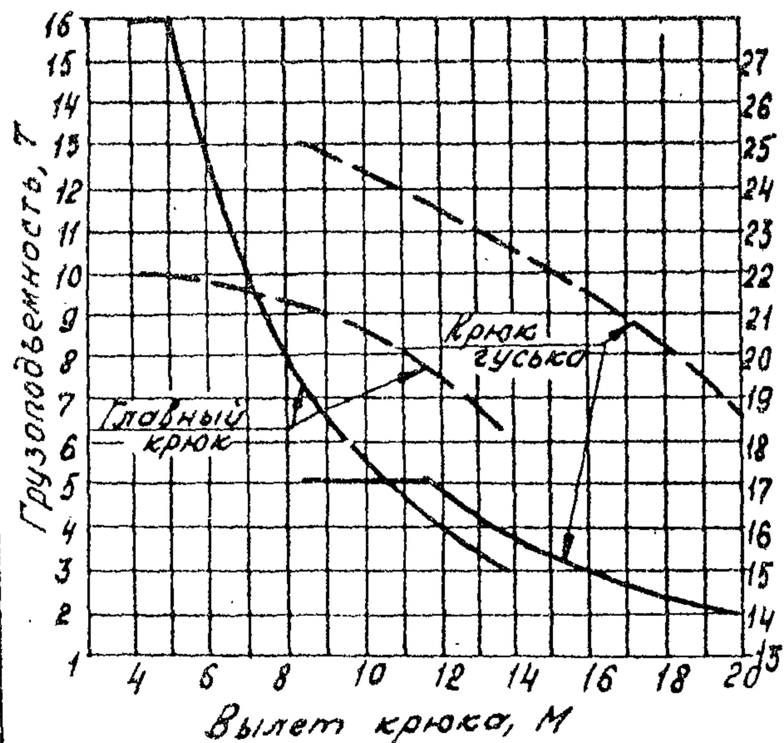
Стрела 22,5 м
