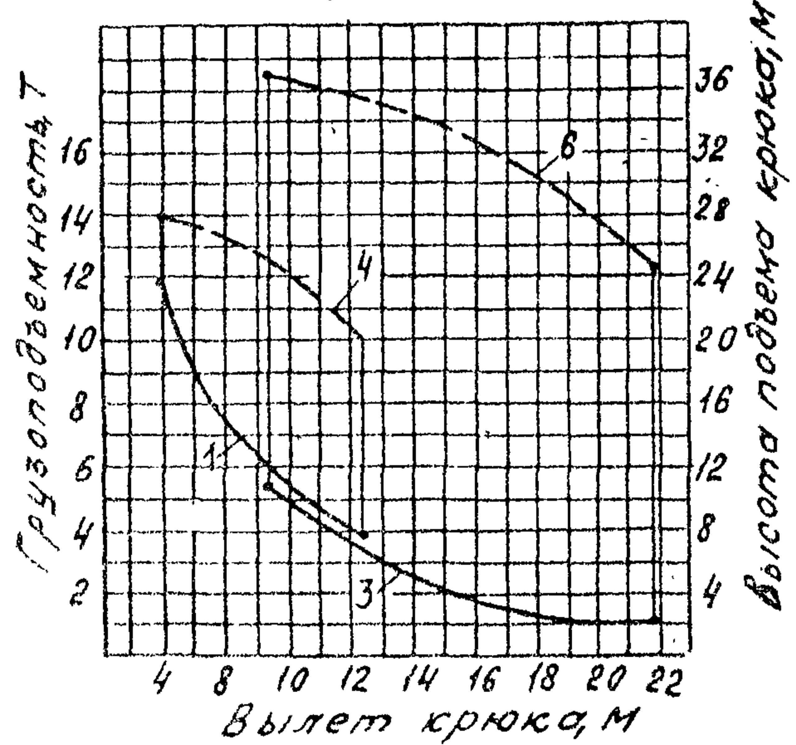
Башня 20м, гусек 10 и 20м
