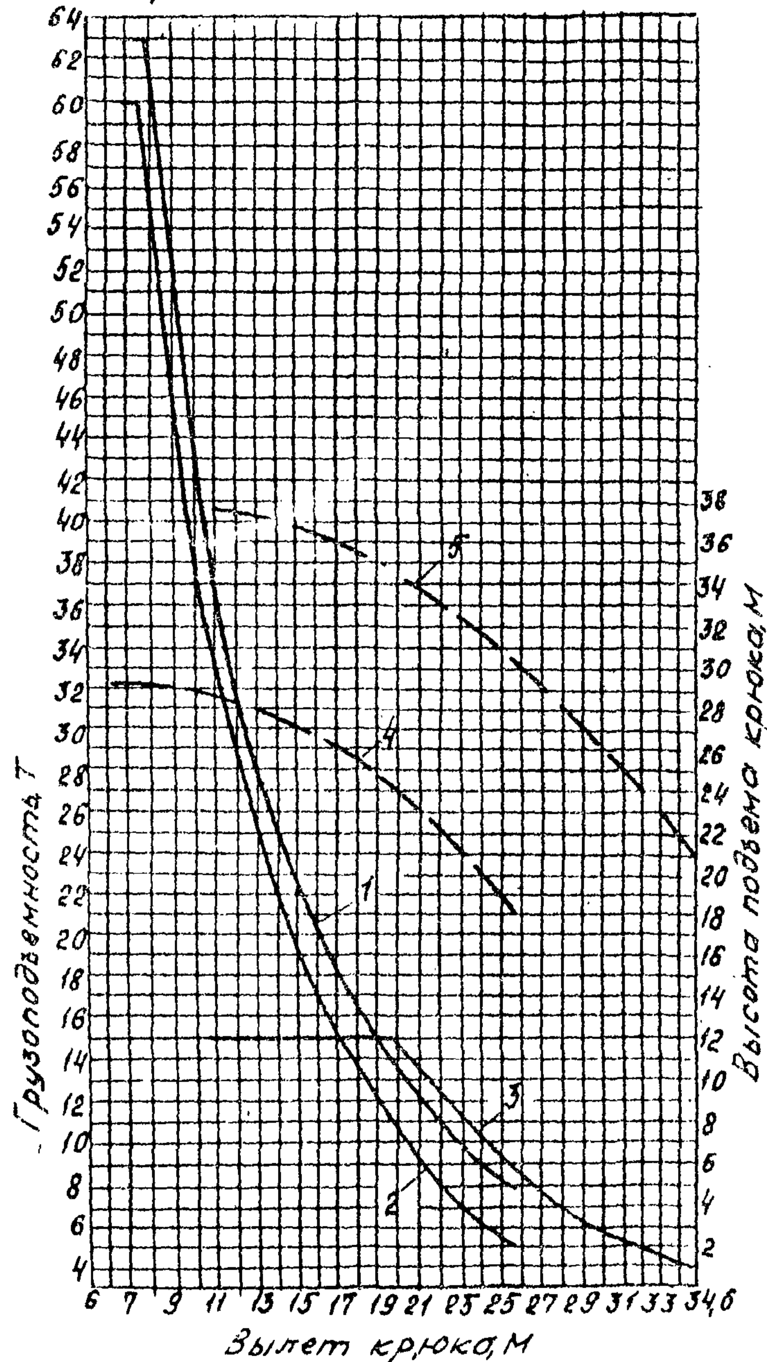
Стрела 30м с гуськом 10м
