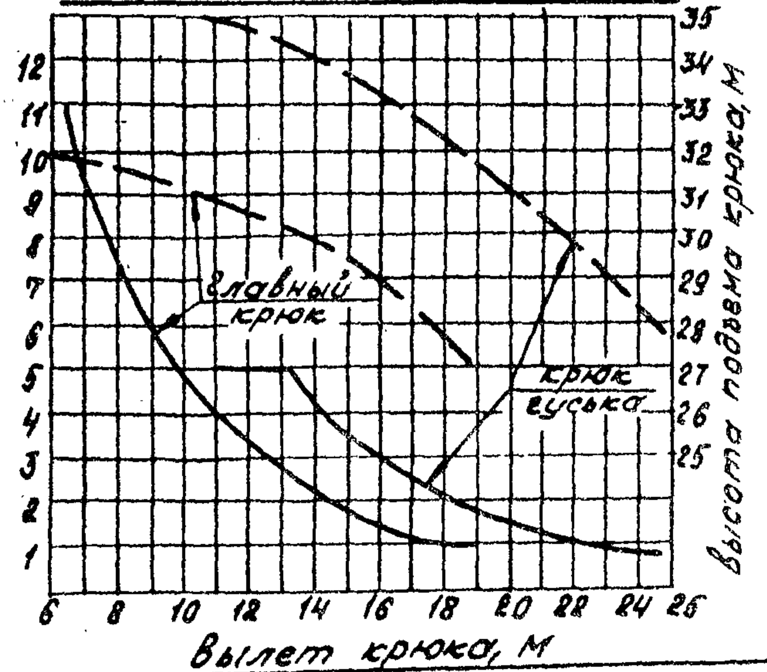
Стрела 32,5 м с гуськом 5 м
