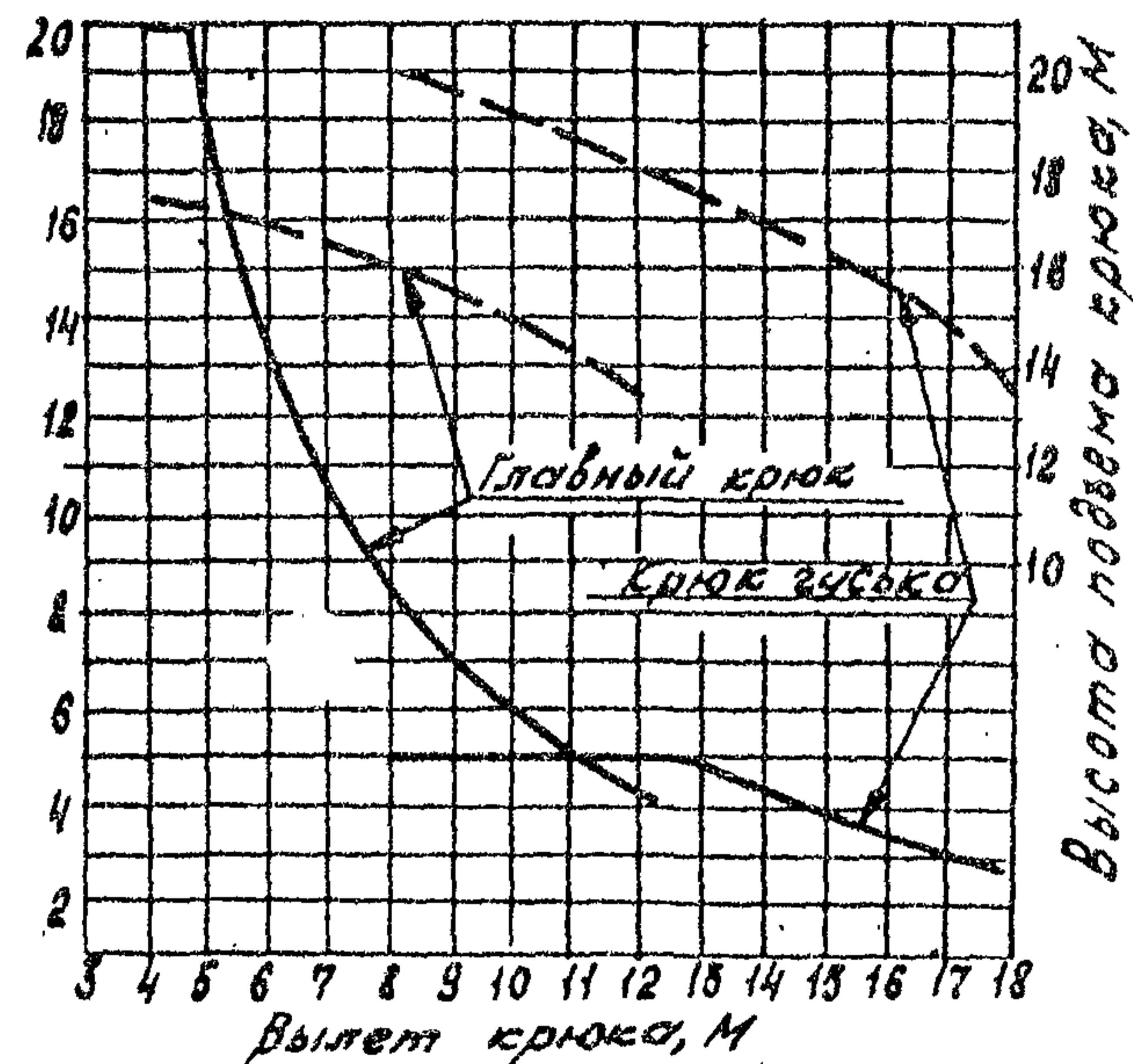
Стрела 17,5 м
