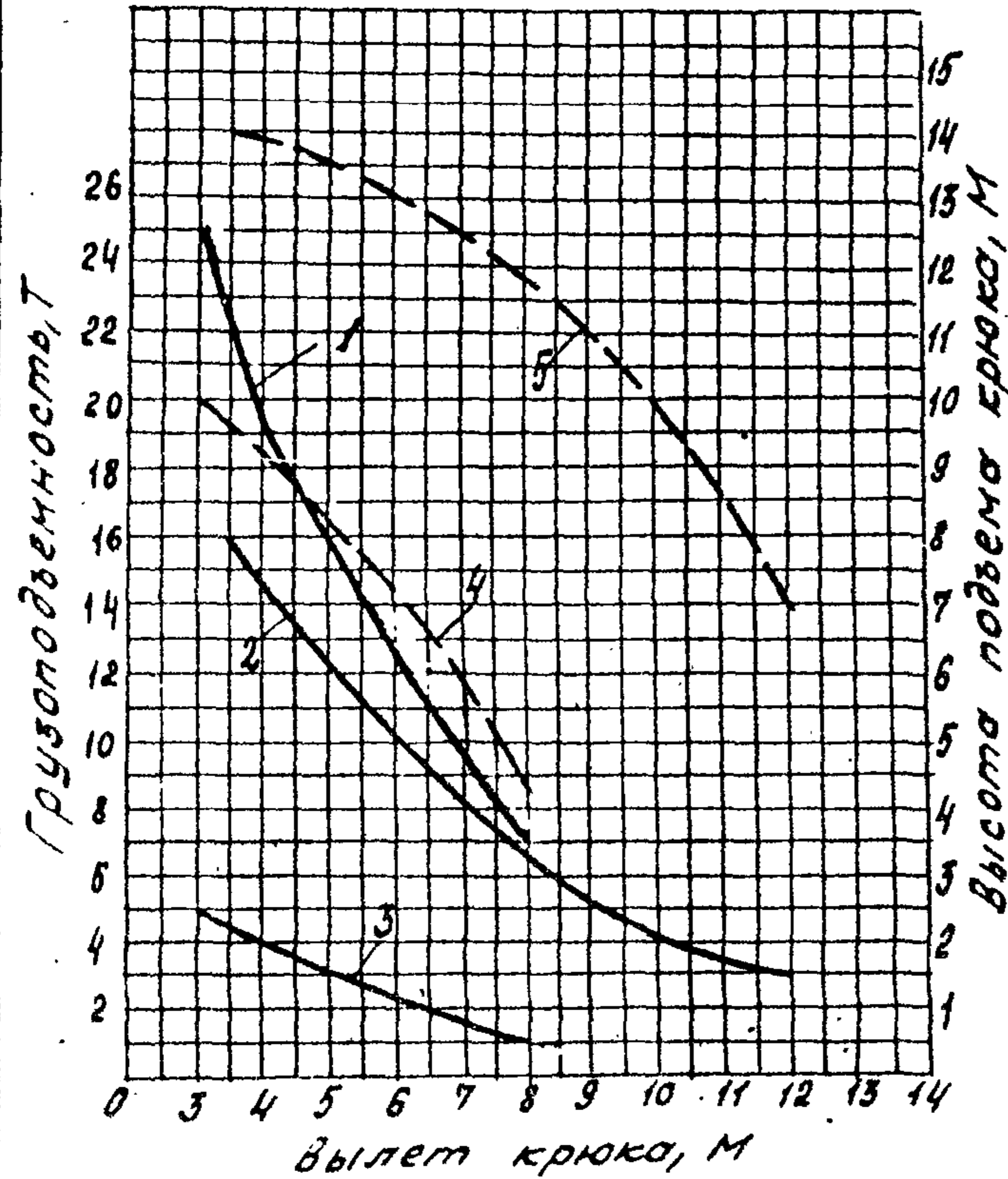
Стрела 10м и 15м
