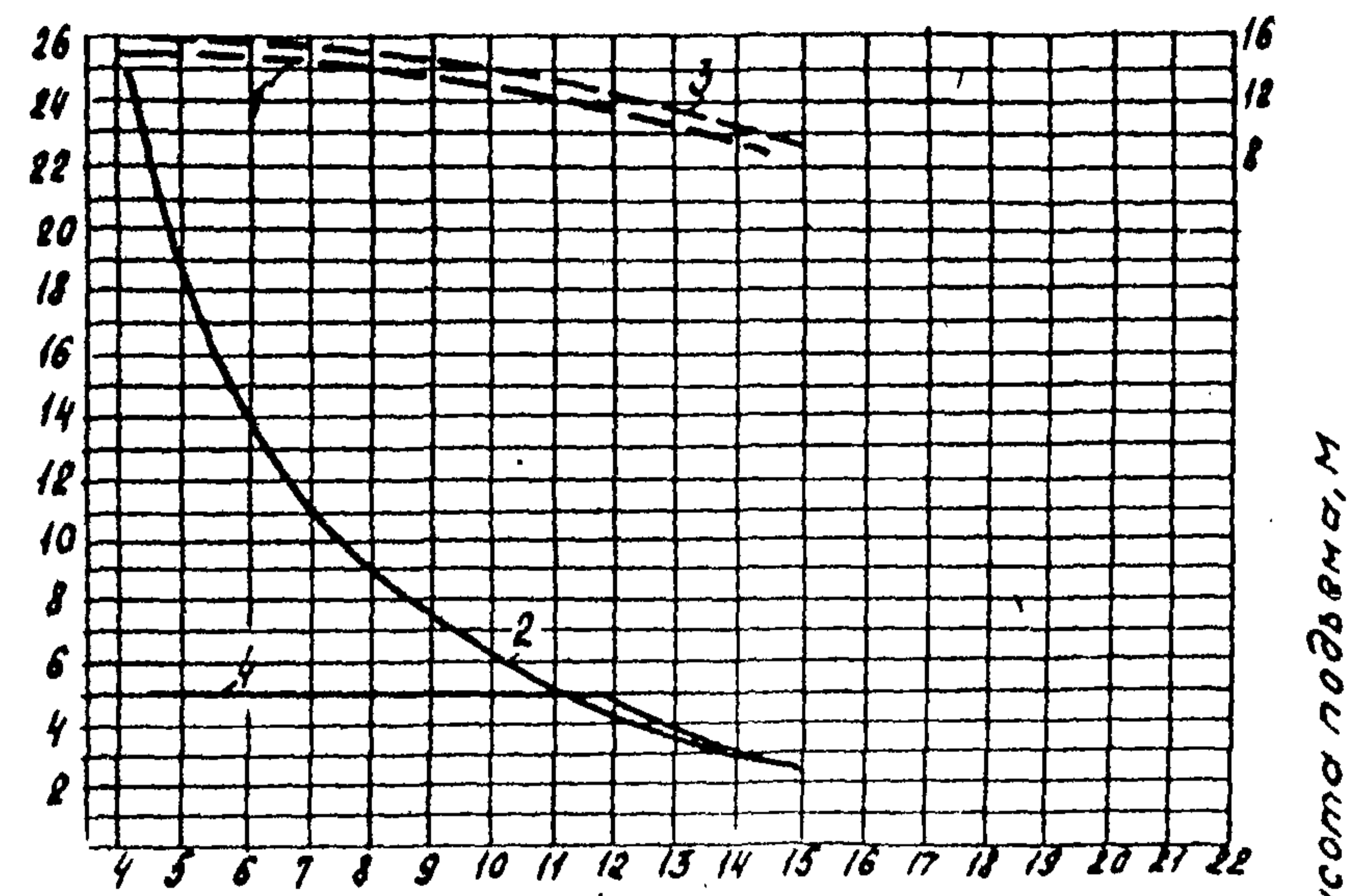
Стрела 20,3 м
