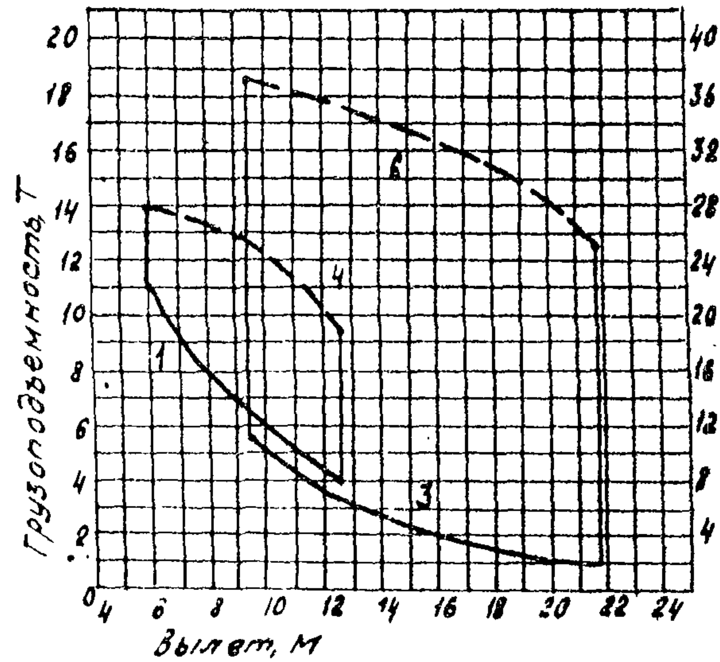
Башня 20м, гуськи 10м и 20м
