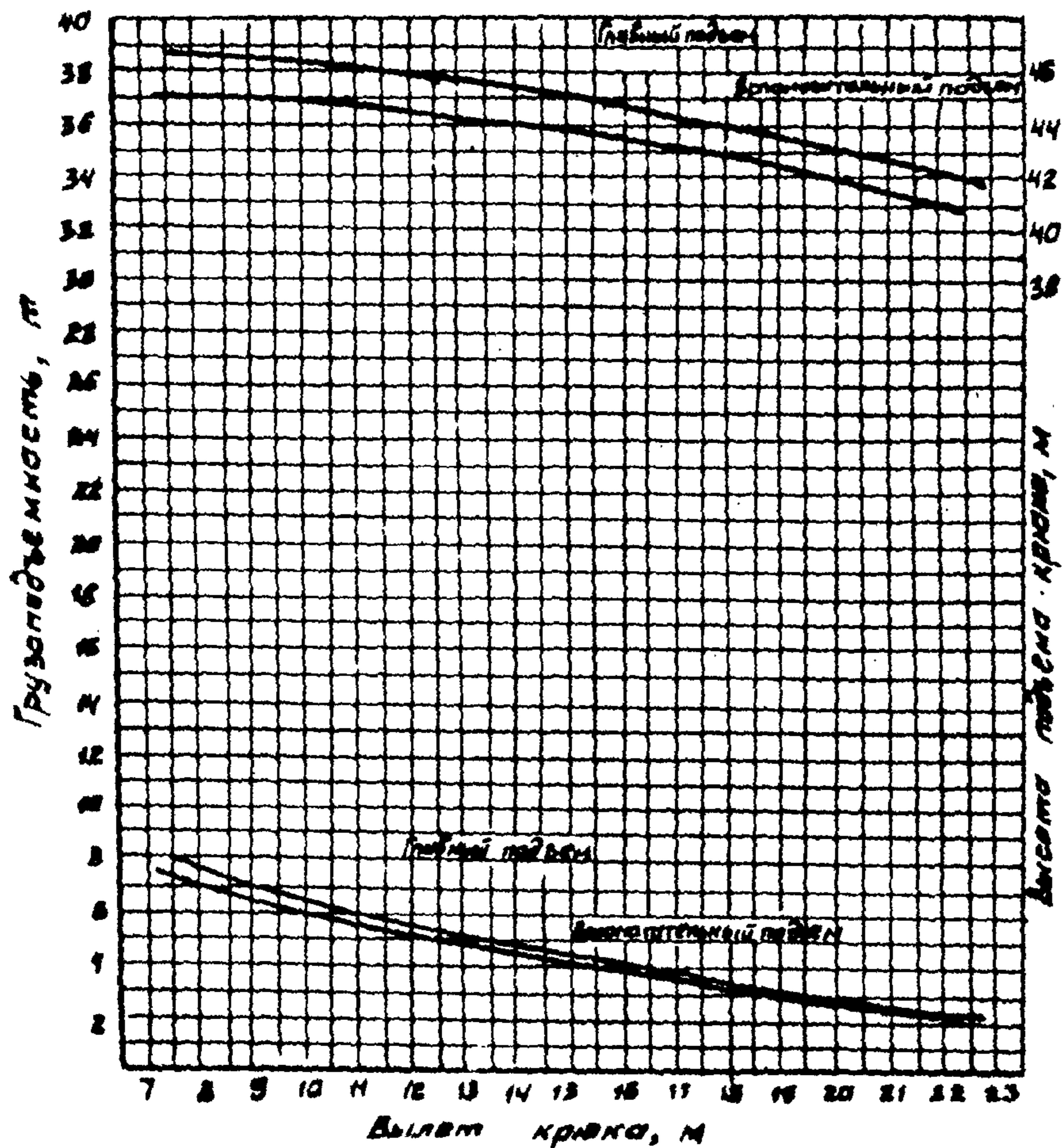
Стрела 46 м без гуська
