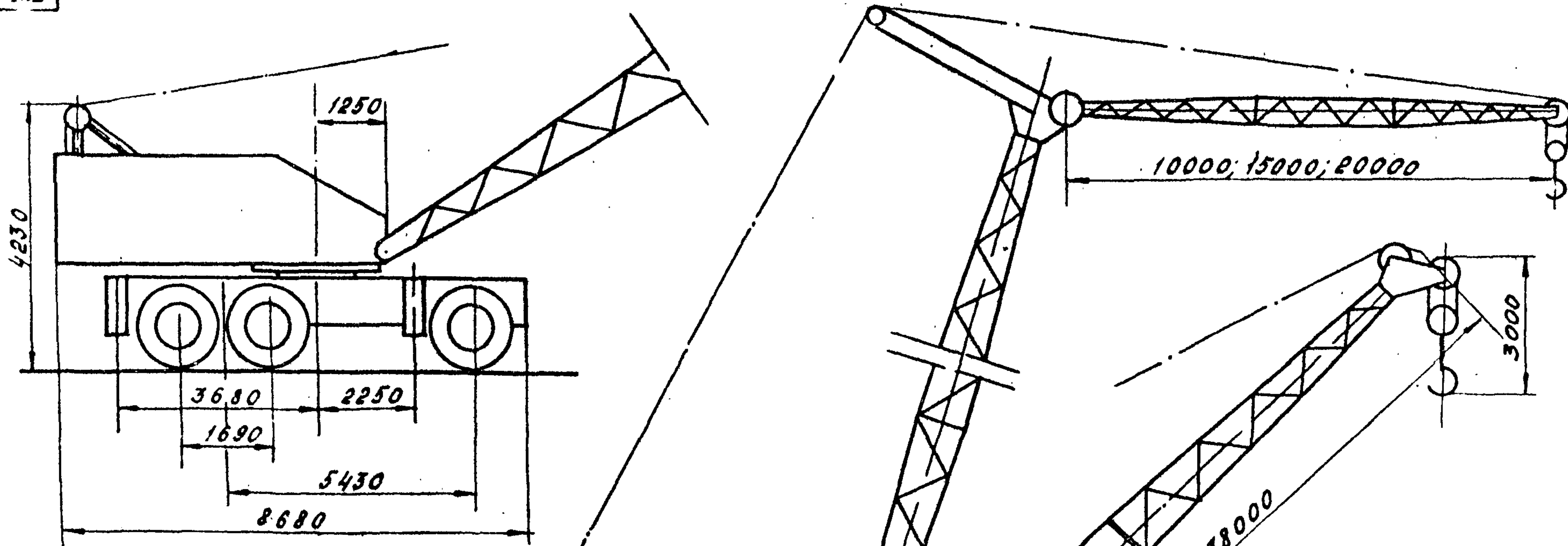
Грузовая характеристика крана
