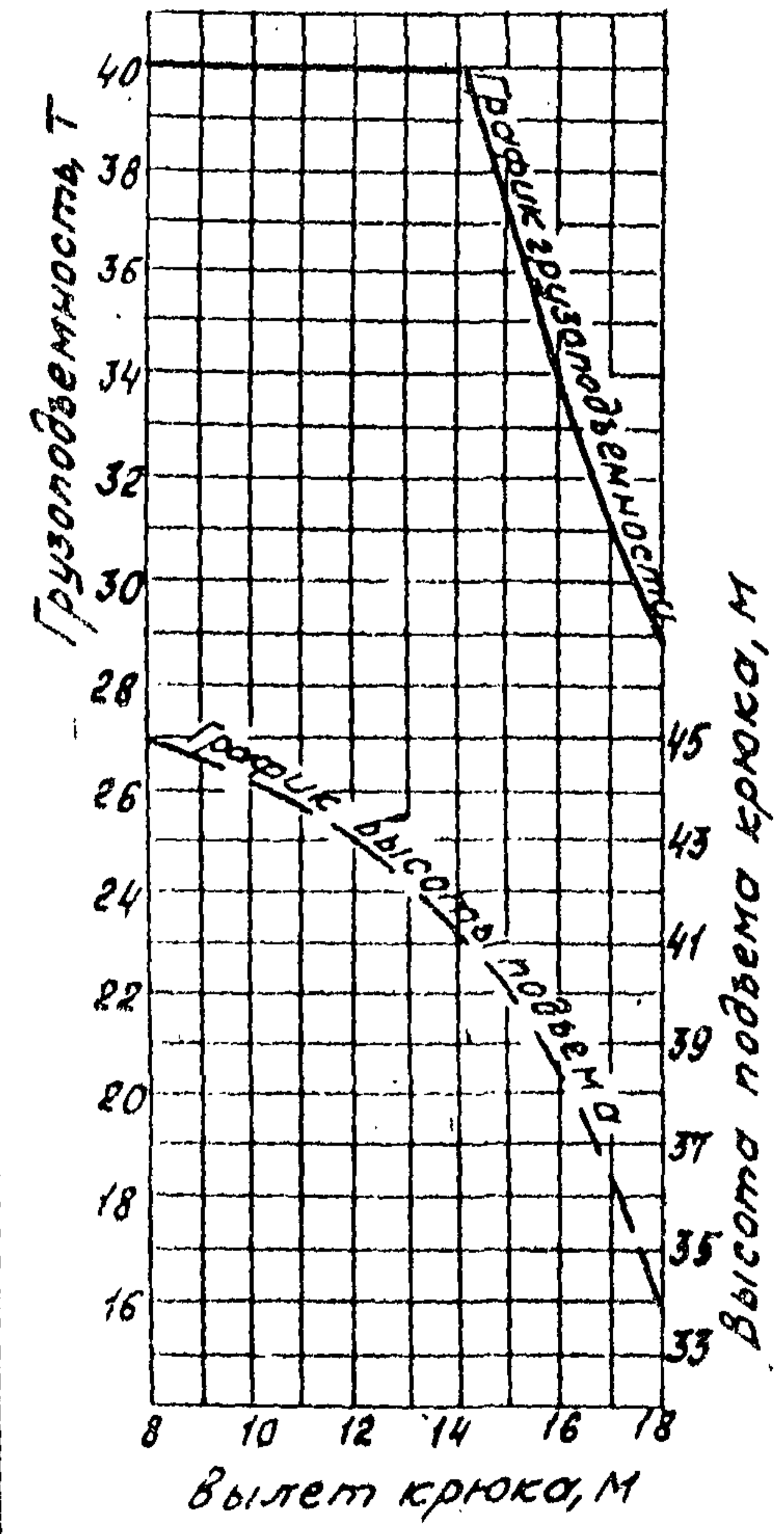
Стрела 31м с гуськом 16м
