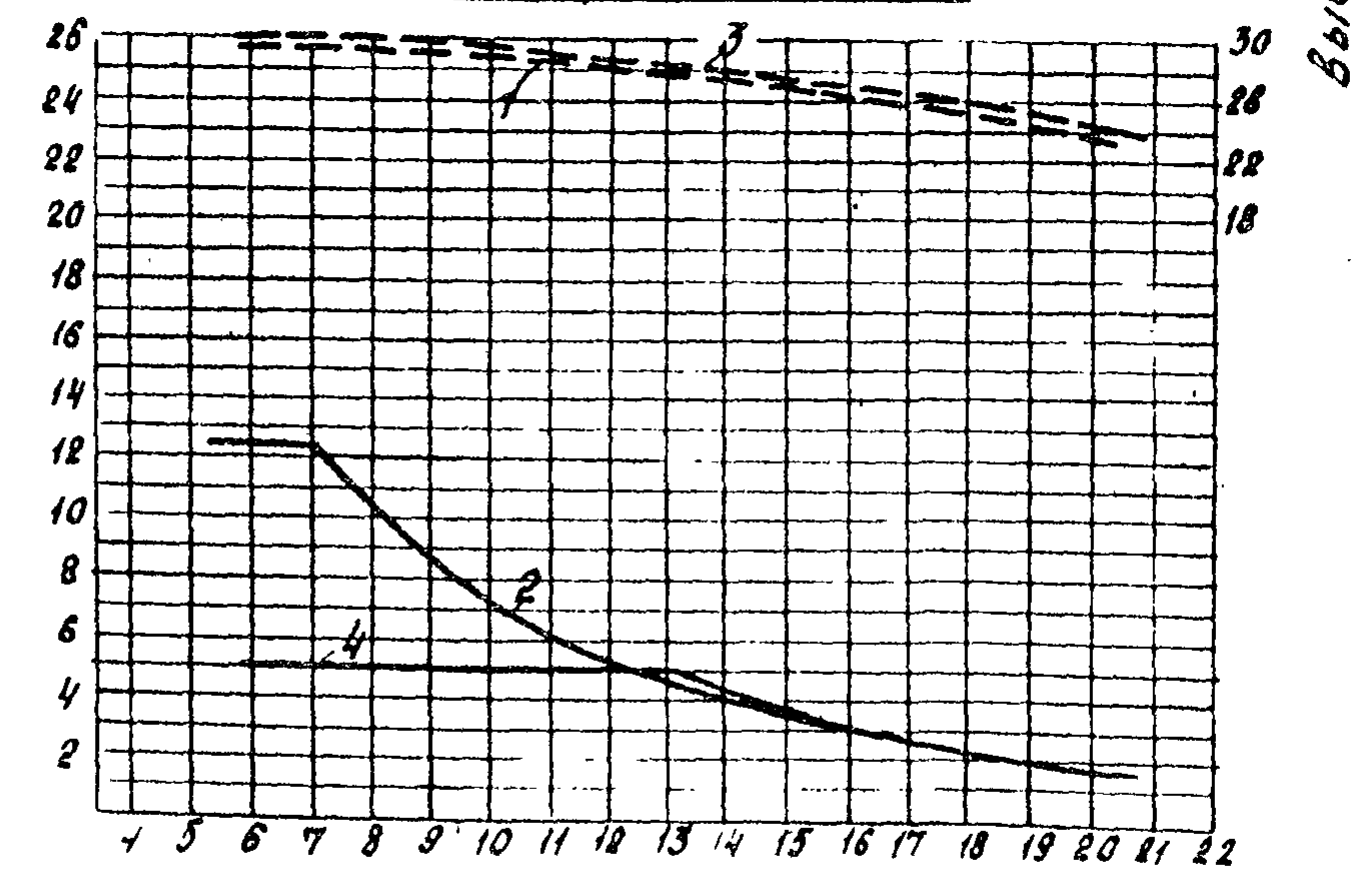
Стрела 30,3м
