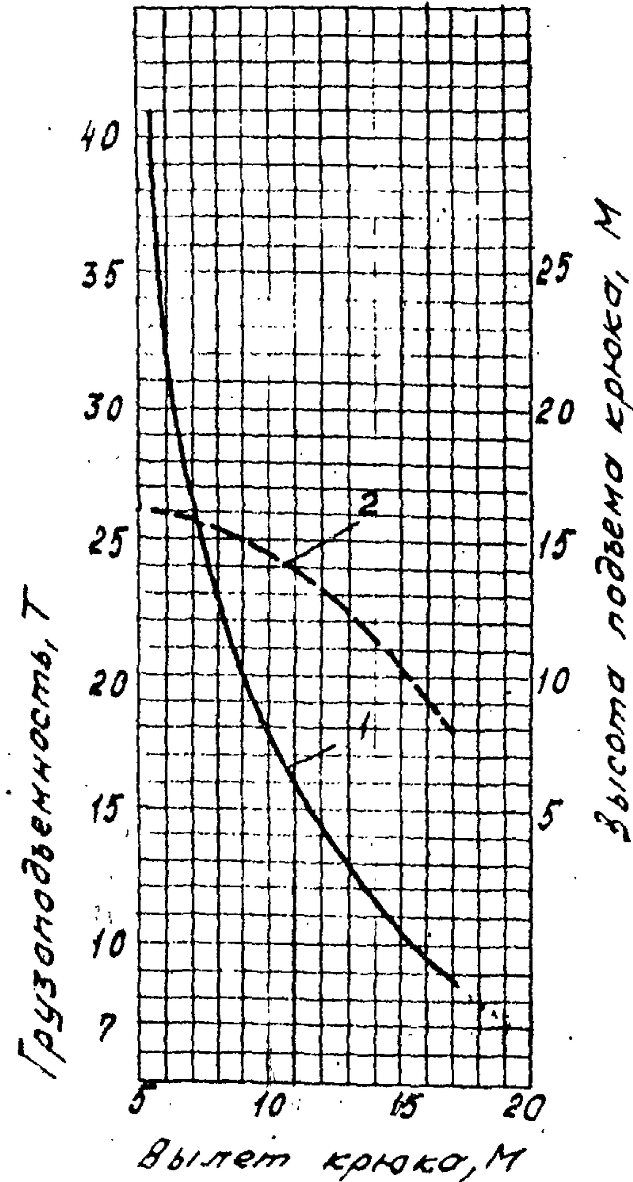
Стрела l=20\text{ м}
