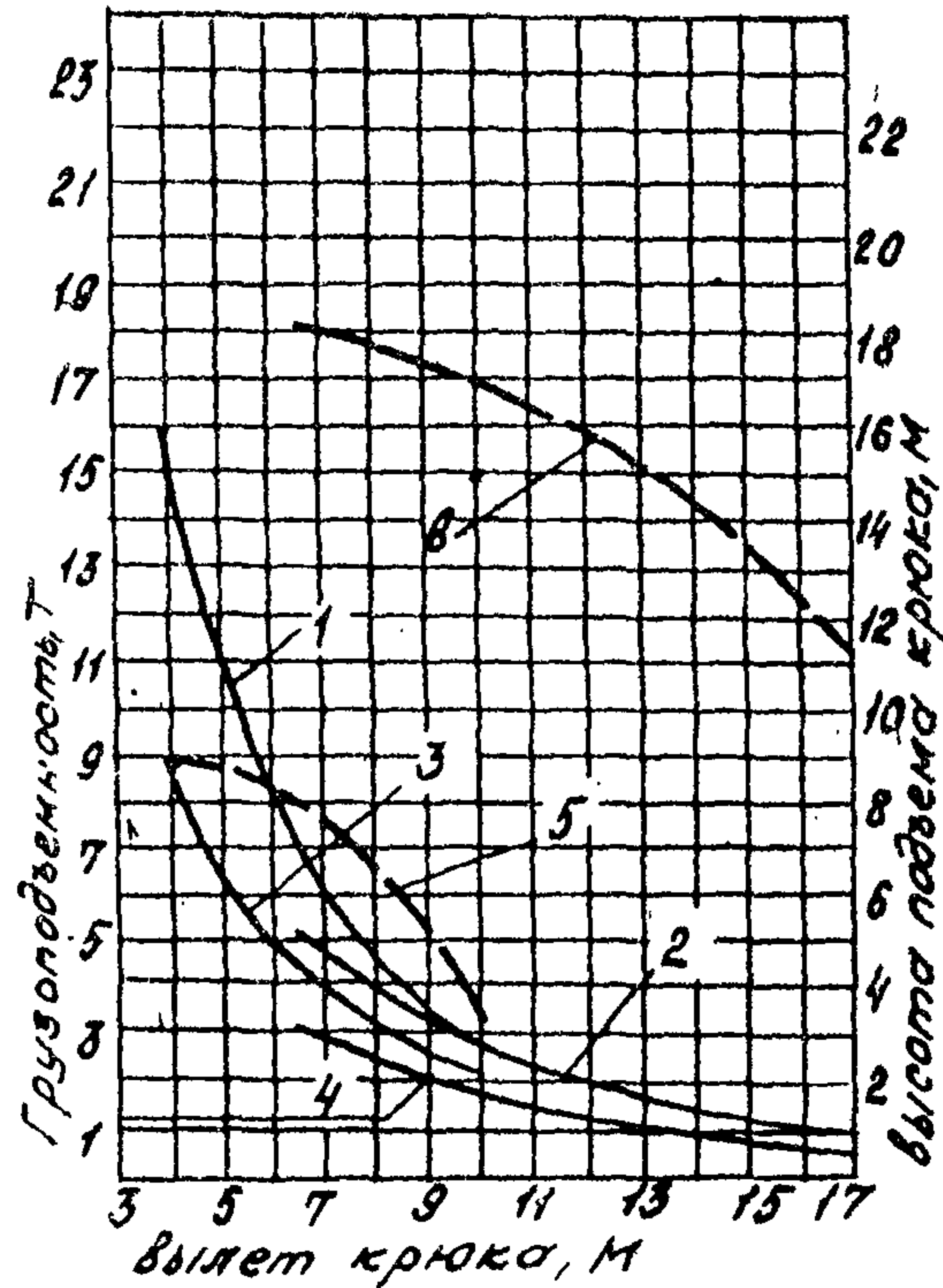
Графики грузоподъемности
