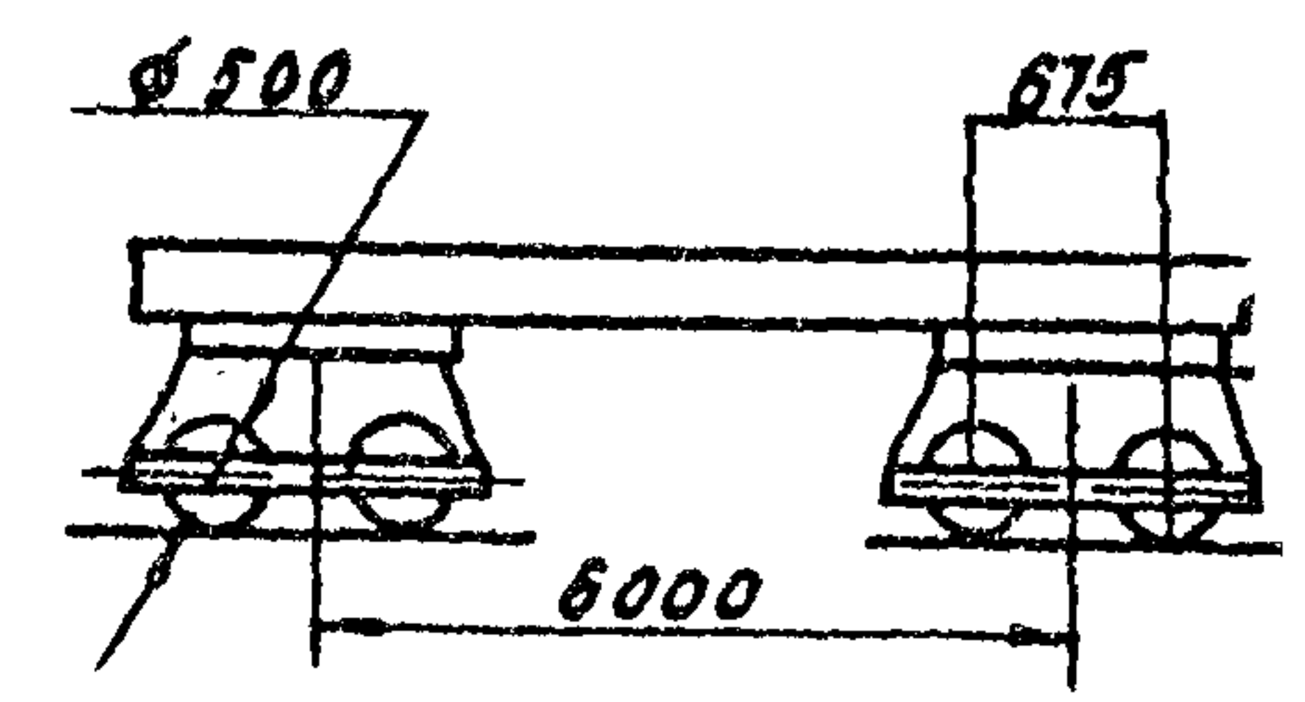
Тележки ведущая ведомая
