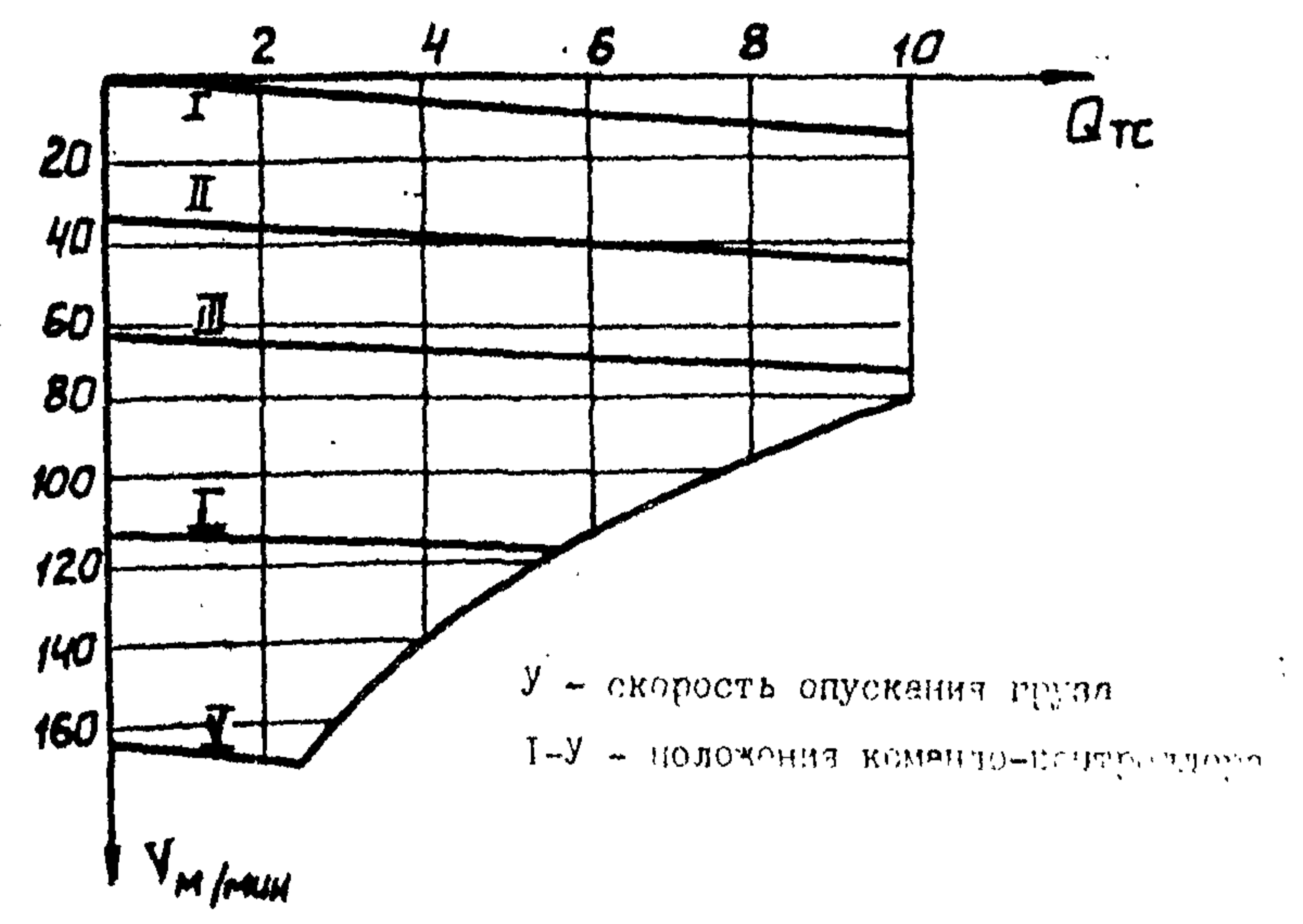
График скорости опускания груза
