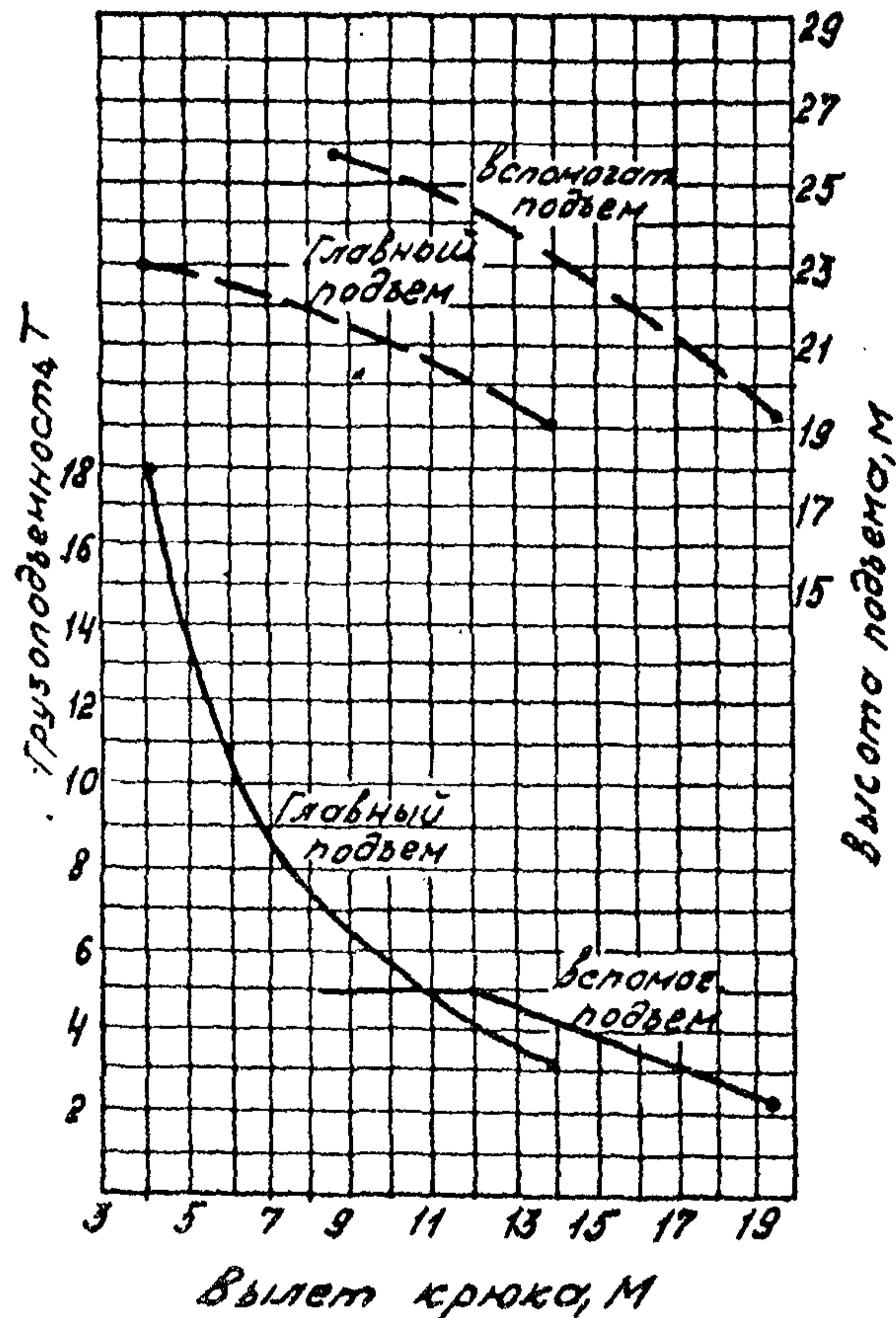
Стрела 23,5 с жестким гуськом 5 м
