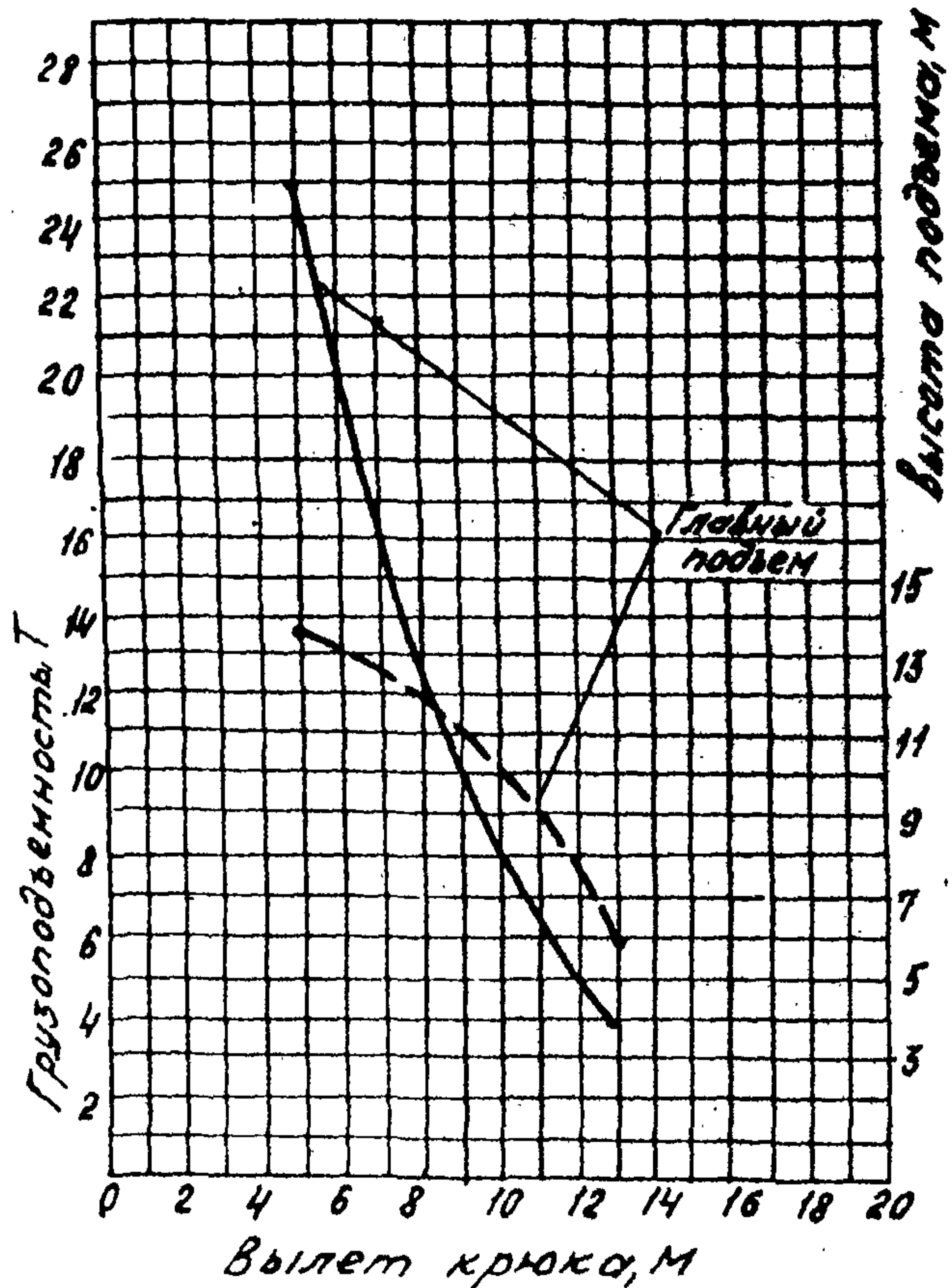
Стрела 13,5 м
