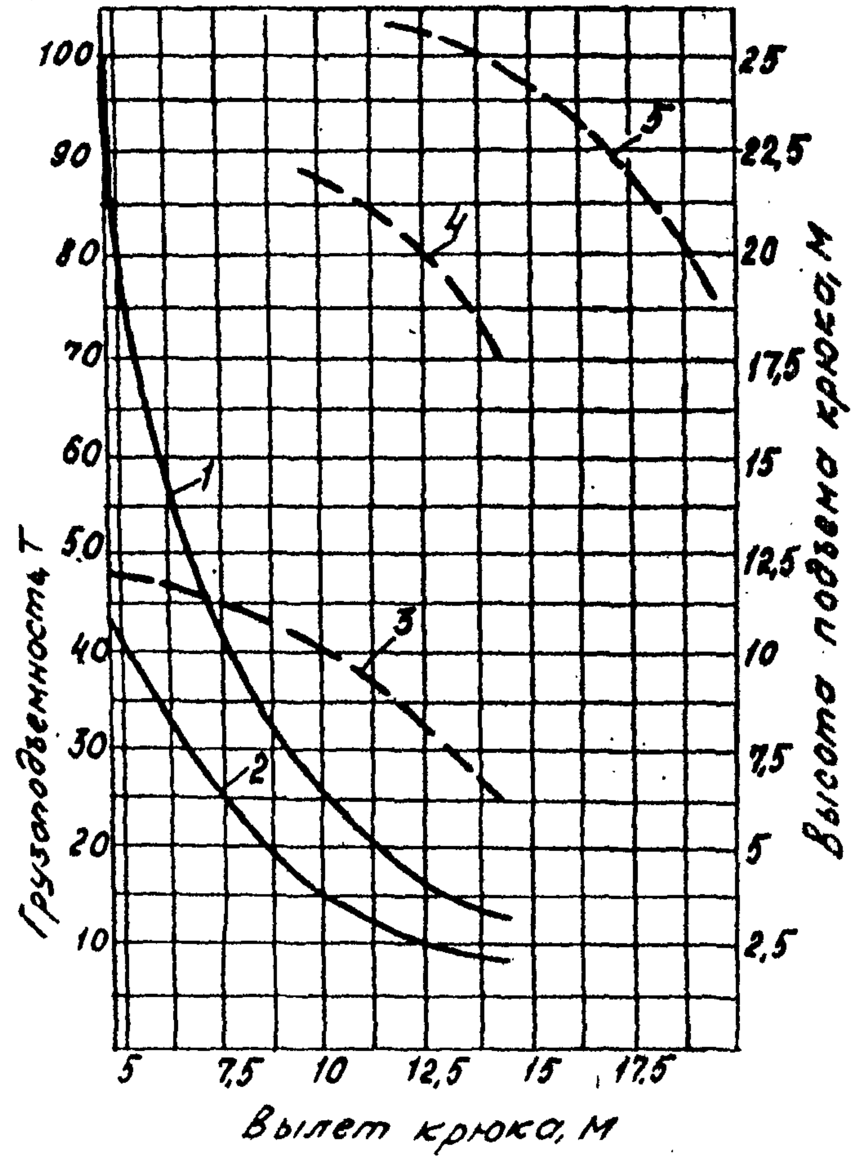
Стрела l=15\text{ м}
