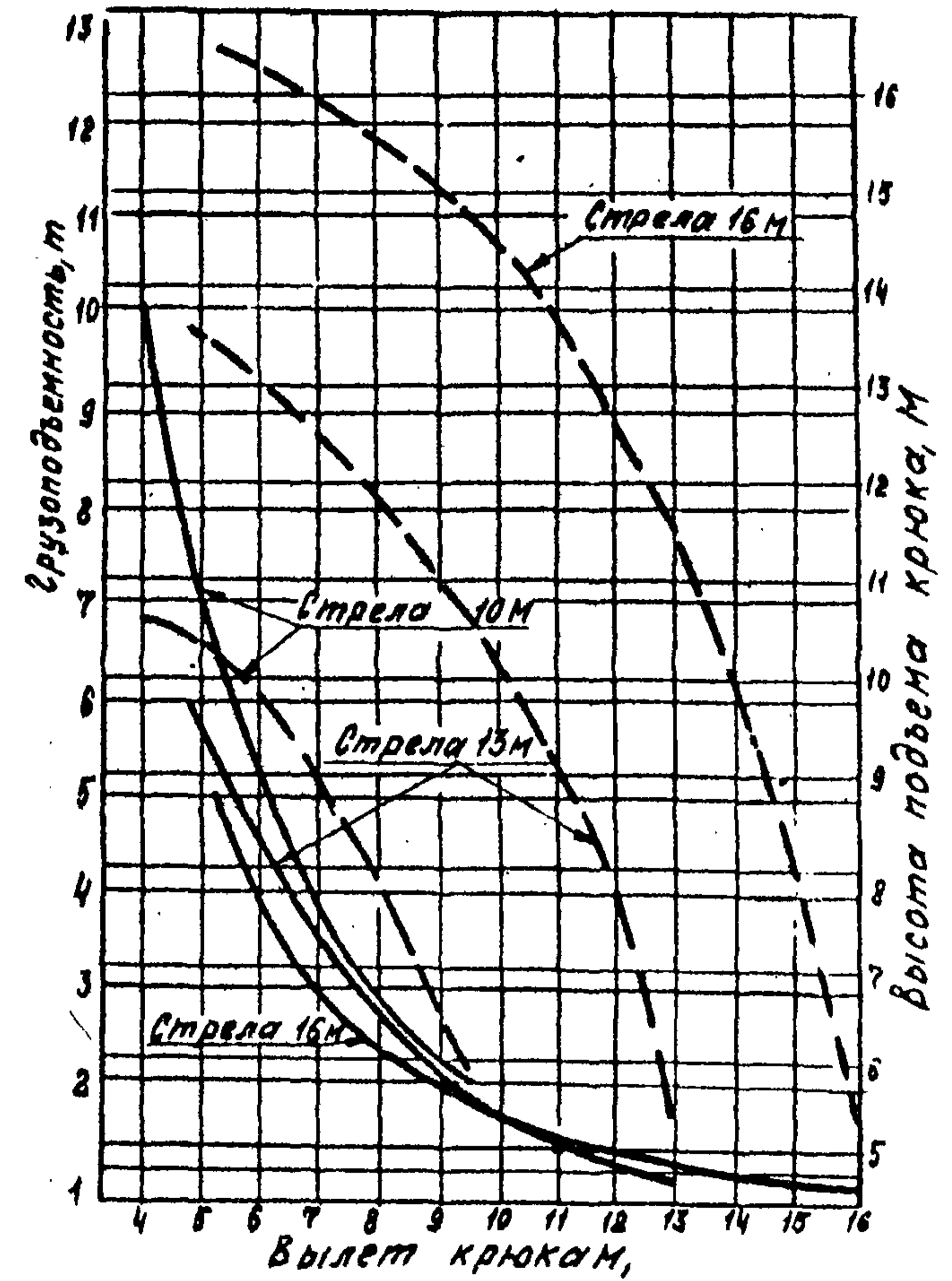
Грузовая характеристика крана
