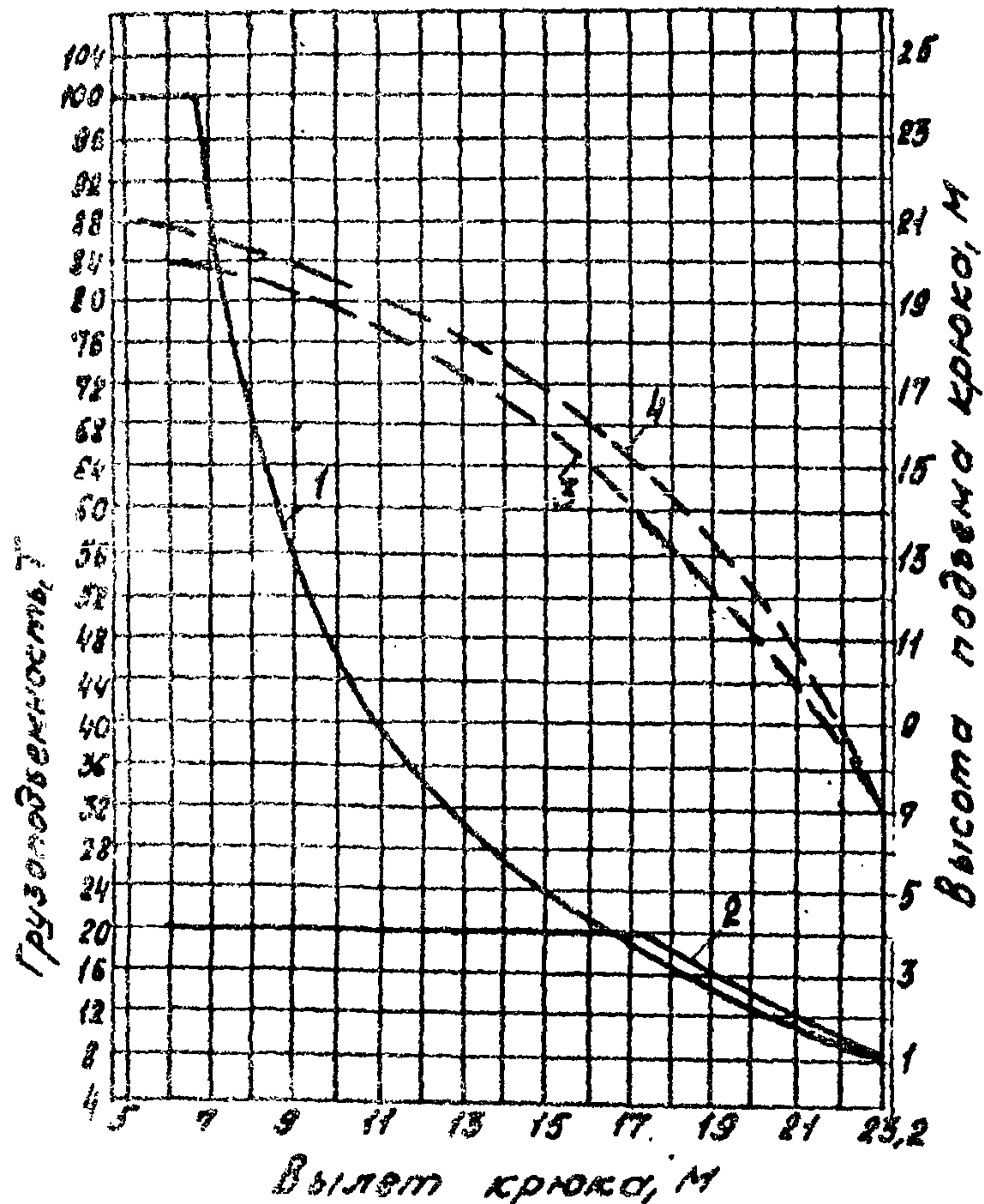
Стрела 21м
