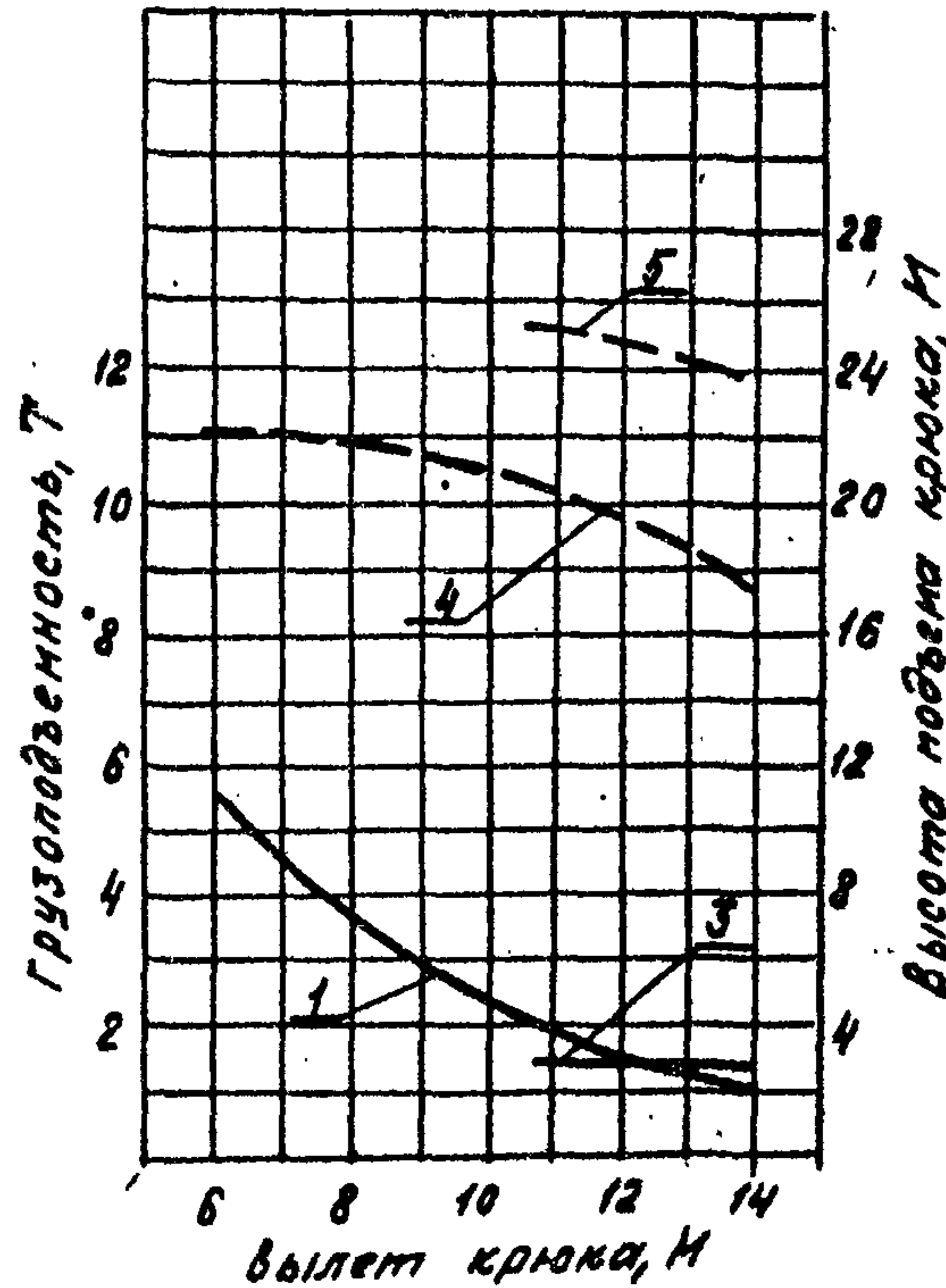
Стрела 22 м
