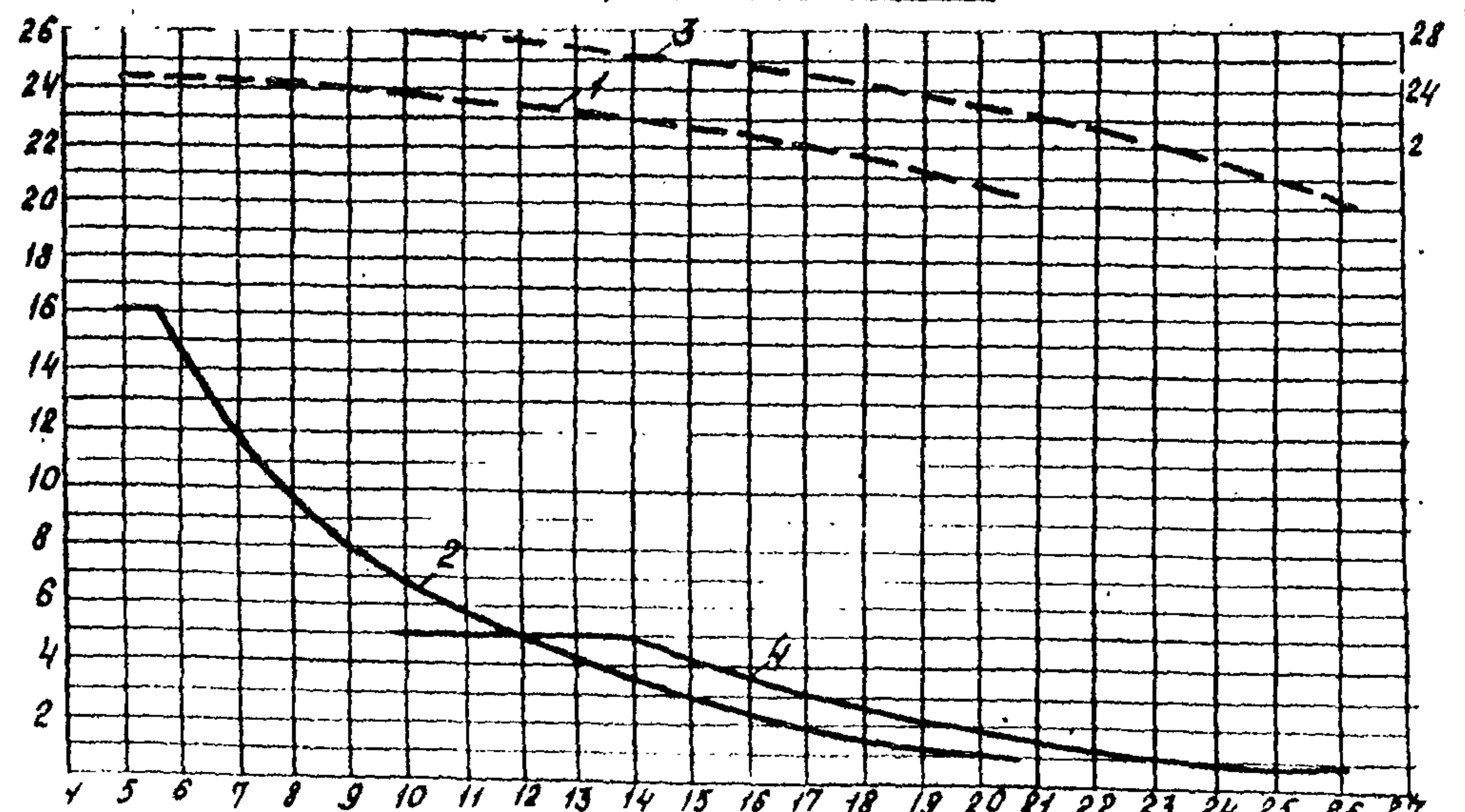
Стрела 25,3 м
