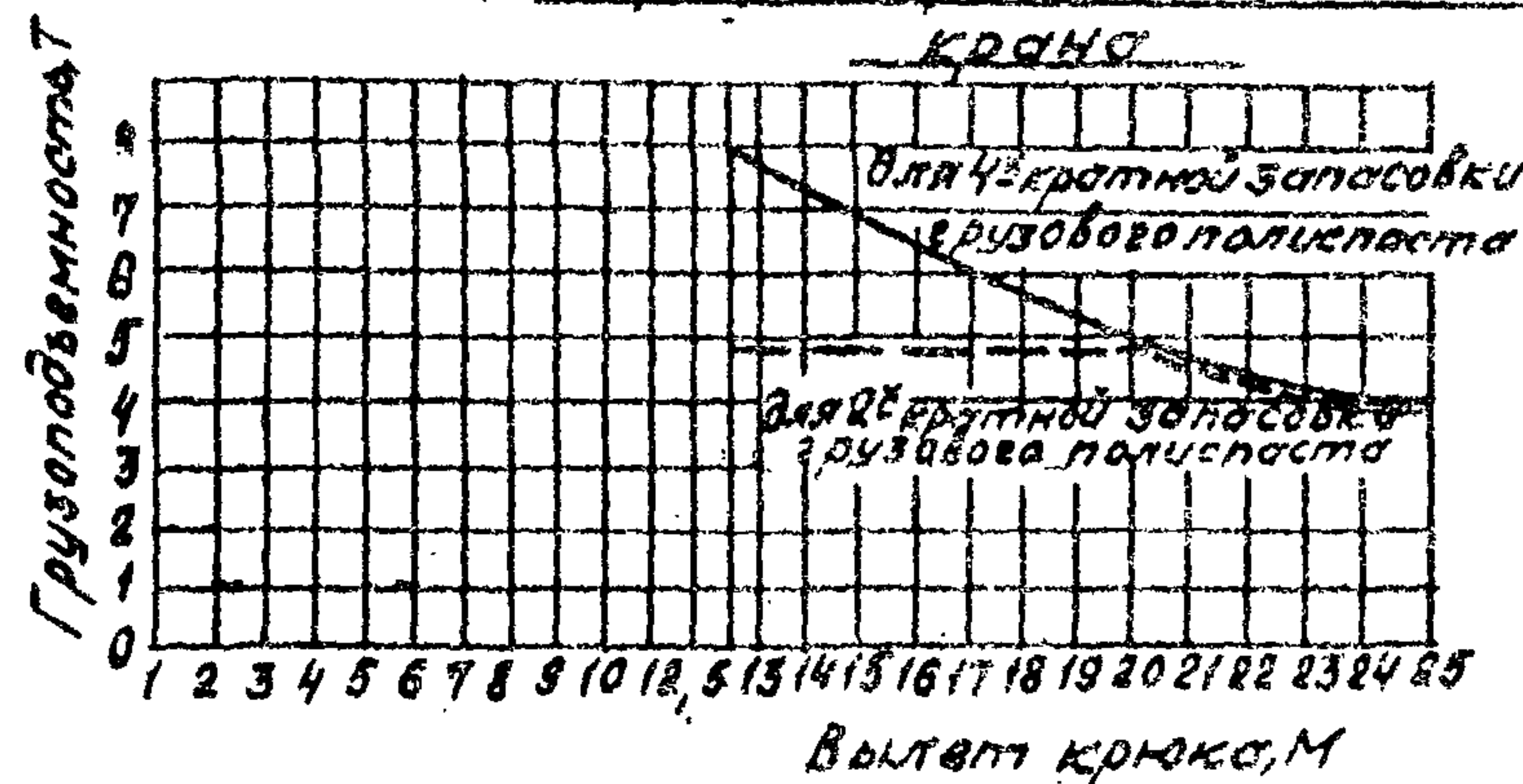
График высоты подъема крюка
