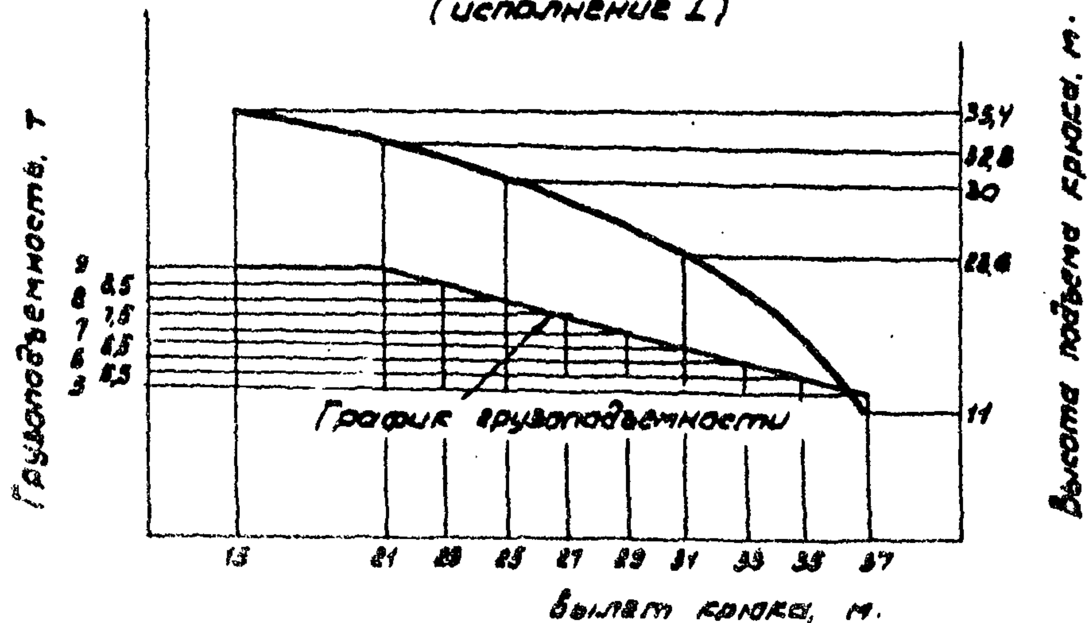
Стрела 36 м с опорной вставкой (исполнение I)
