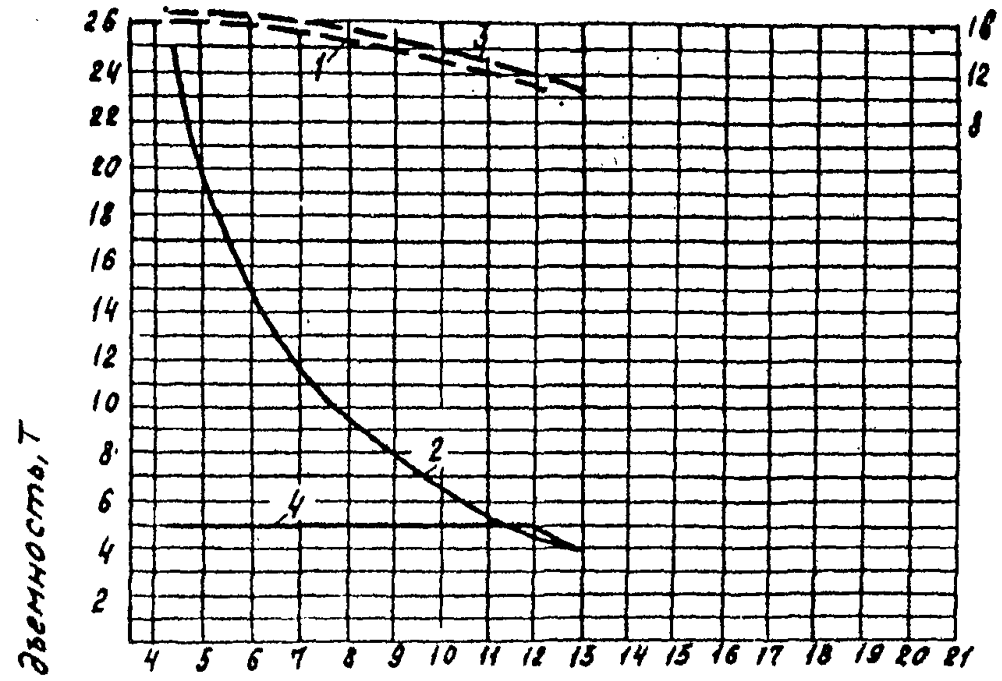
Стрела 17,5 м
