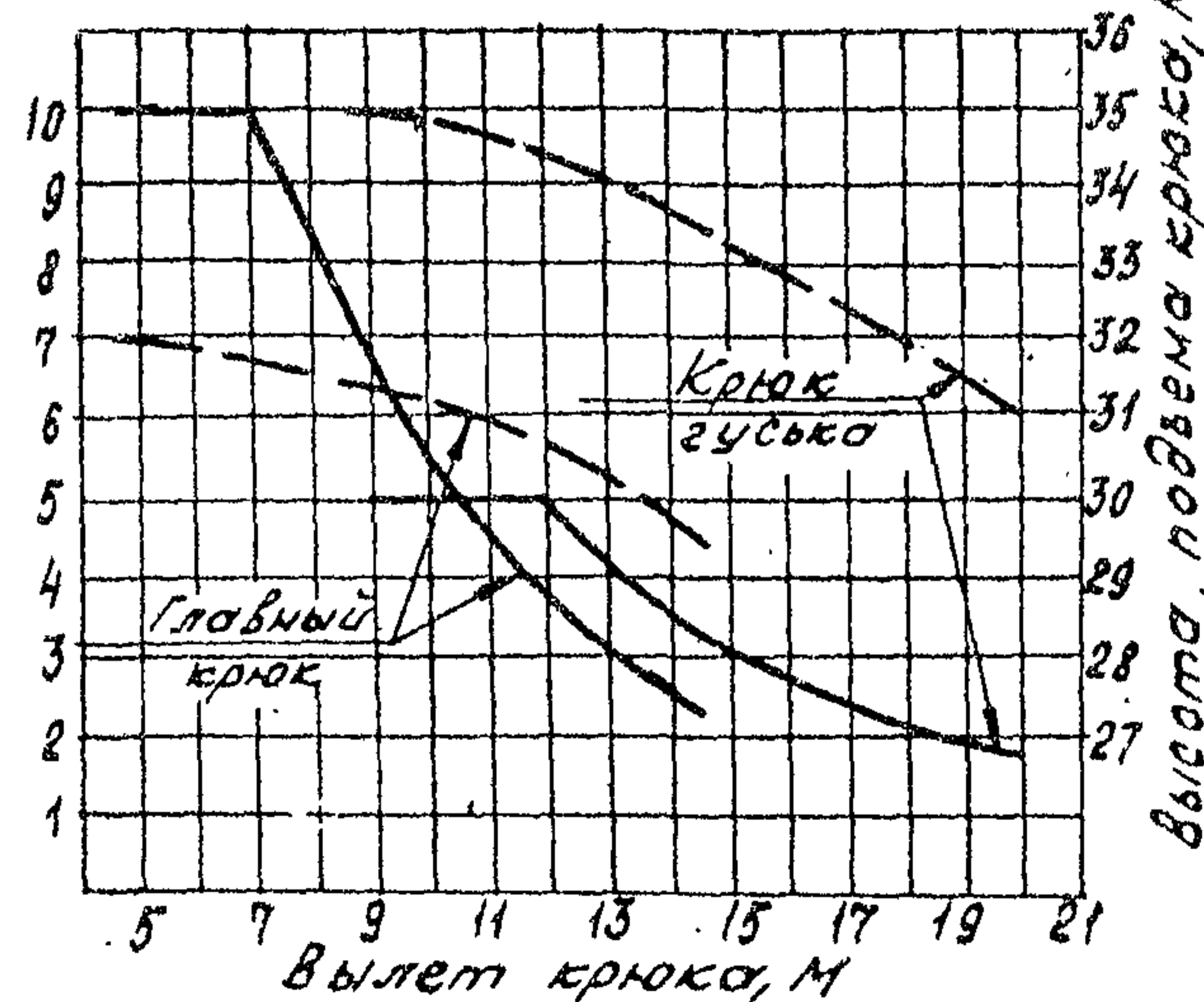
Стрела 32,5 м
