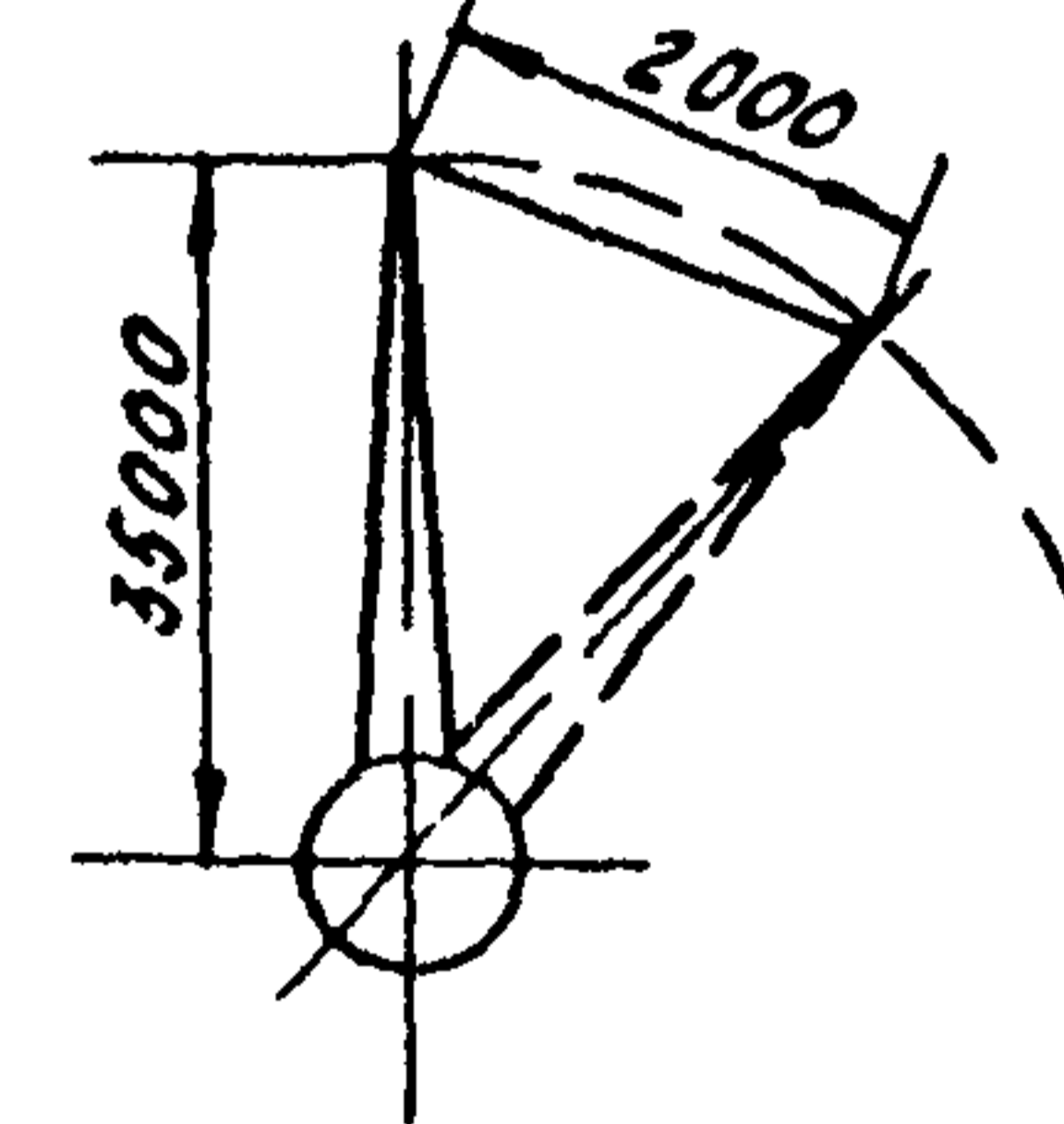
Тормозной путь стрелы с предельным грузом
