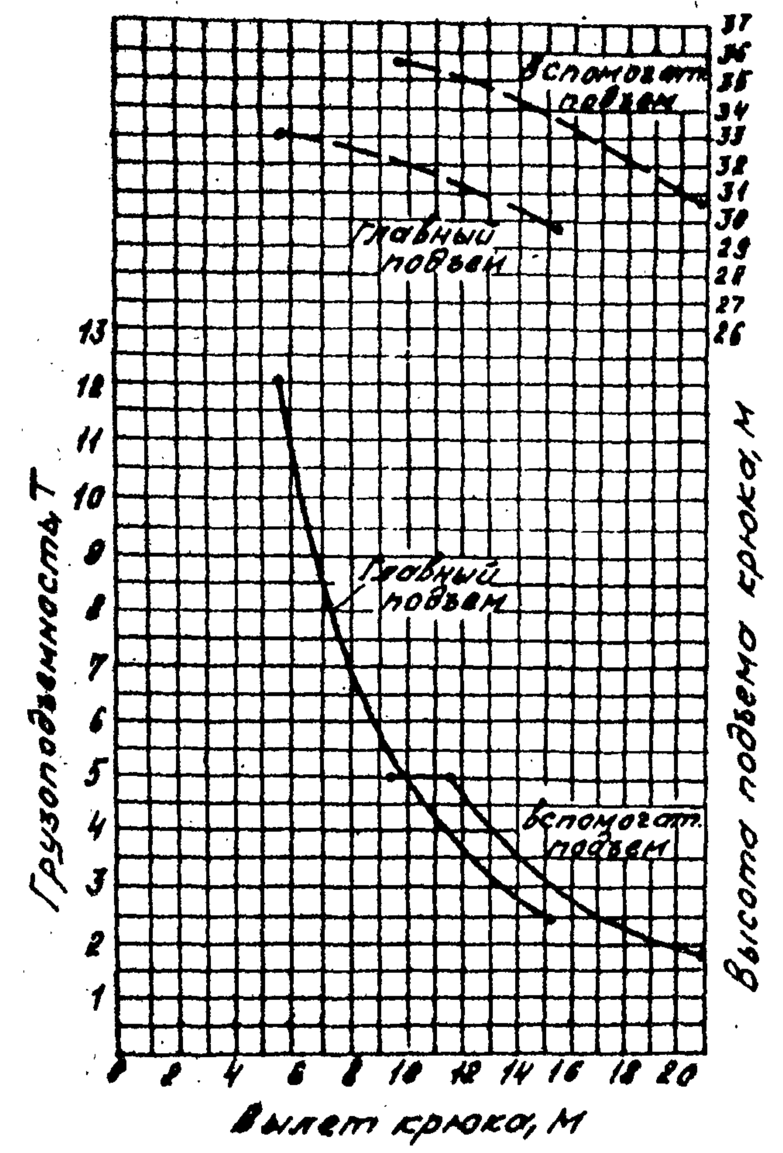
Стрела 33,5 м с жестким гуськом 5 м
