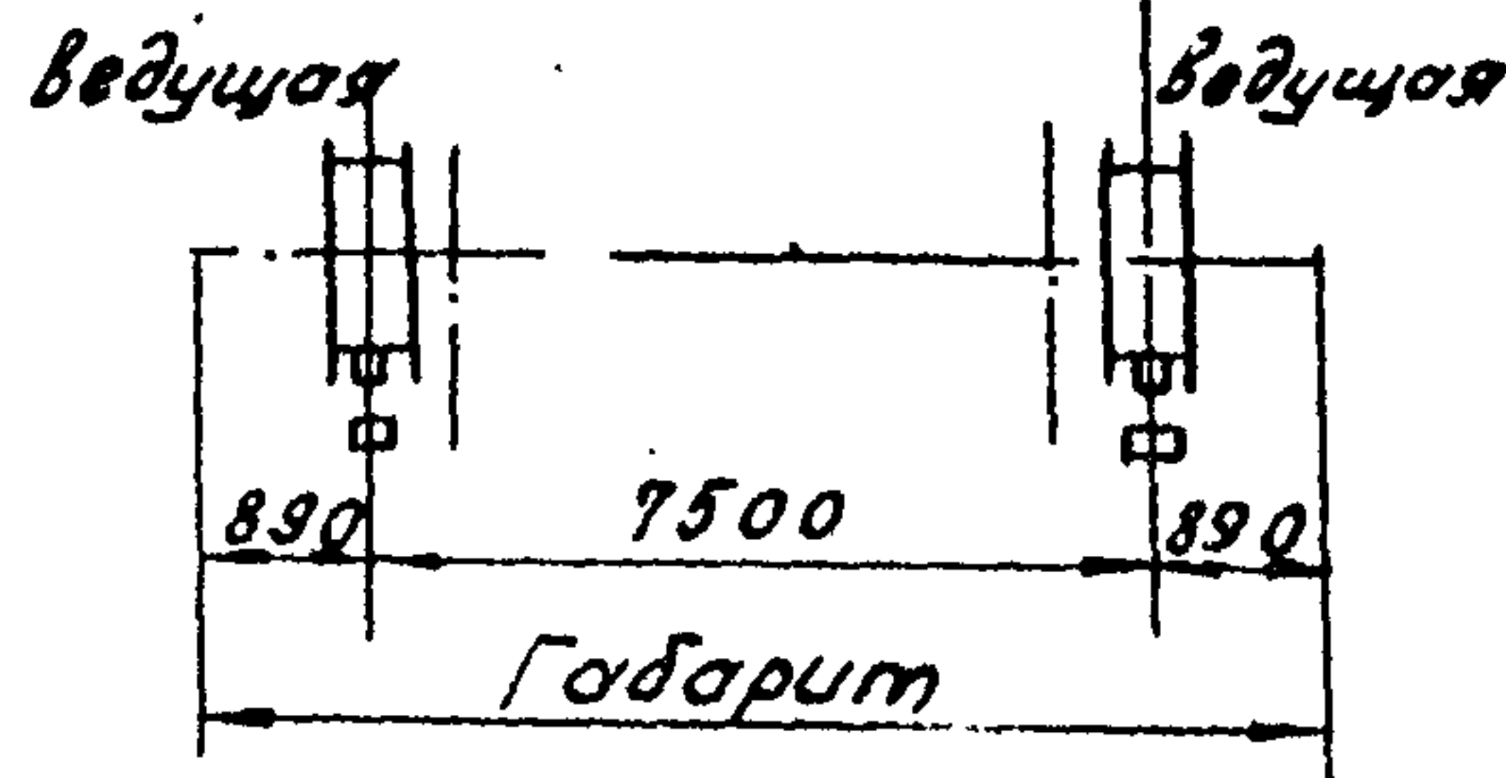
Тележки
