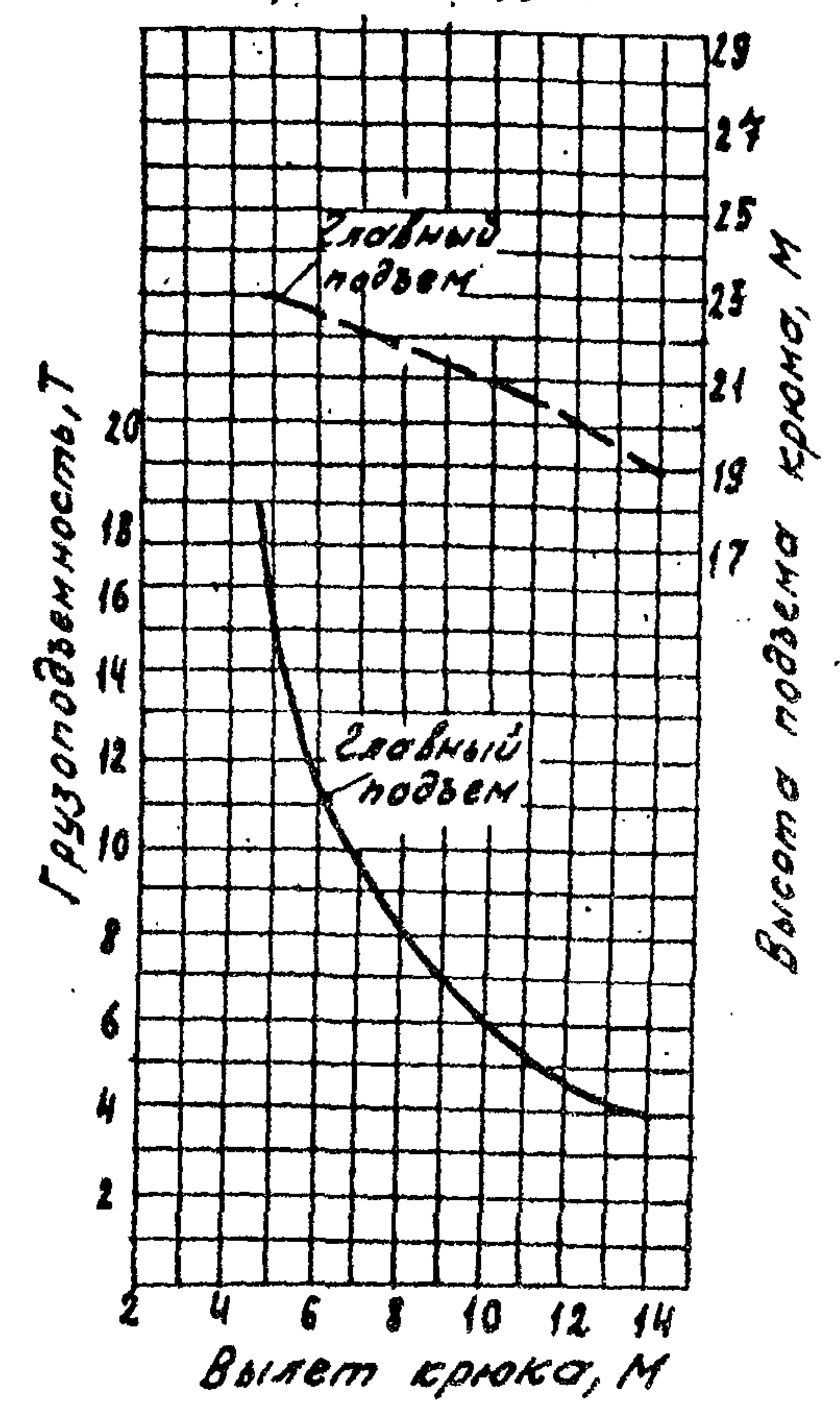
Стрела 23,5 м
