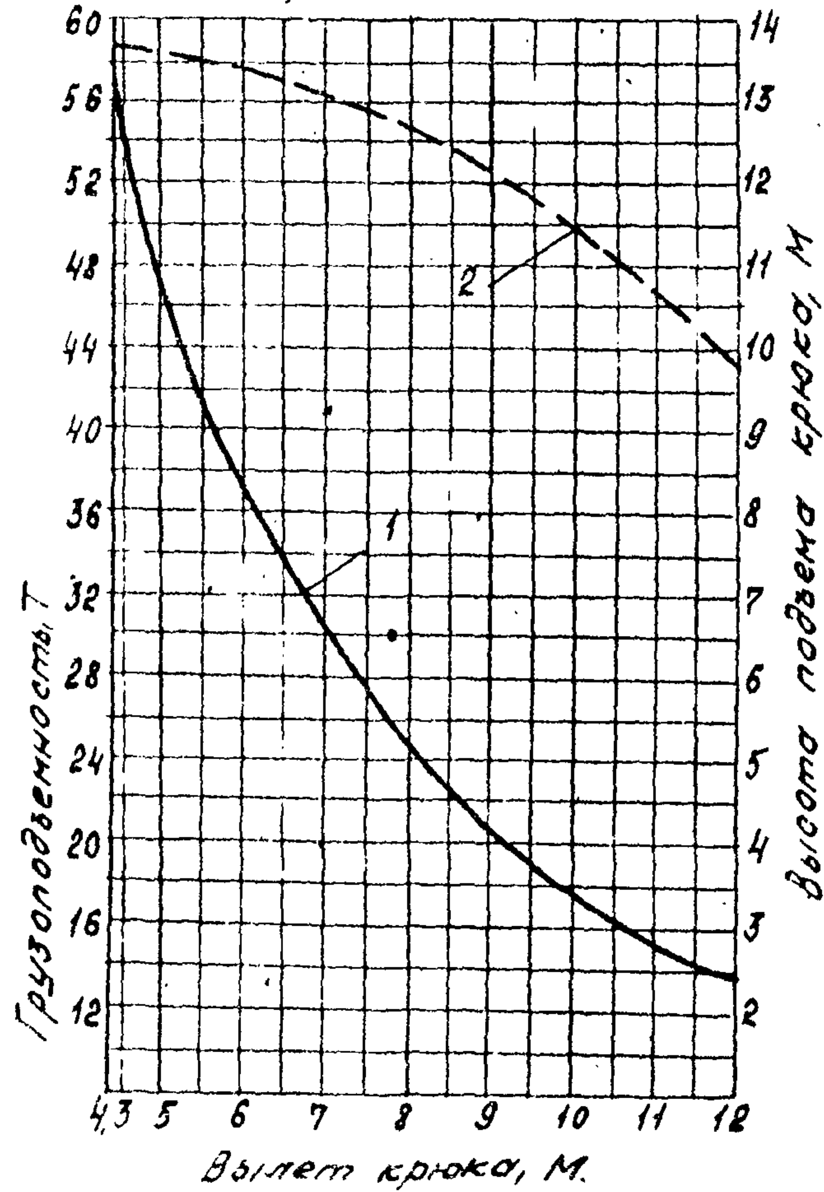
Стрела l=15\text{ м}
