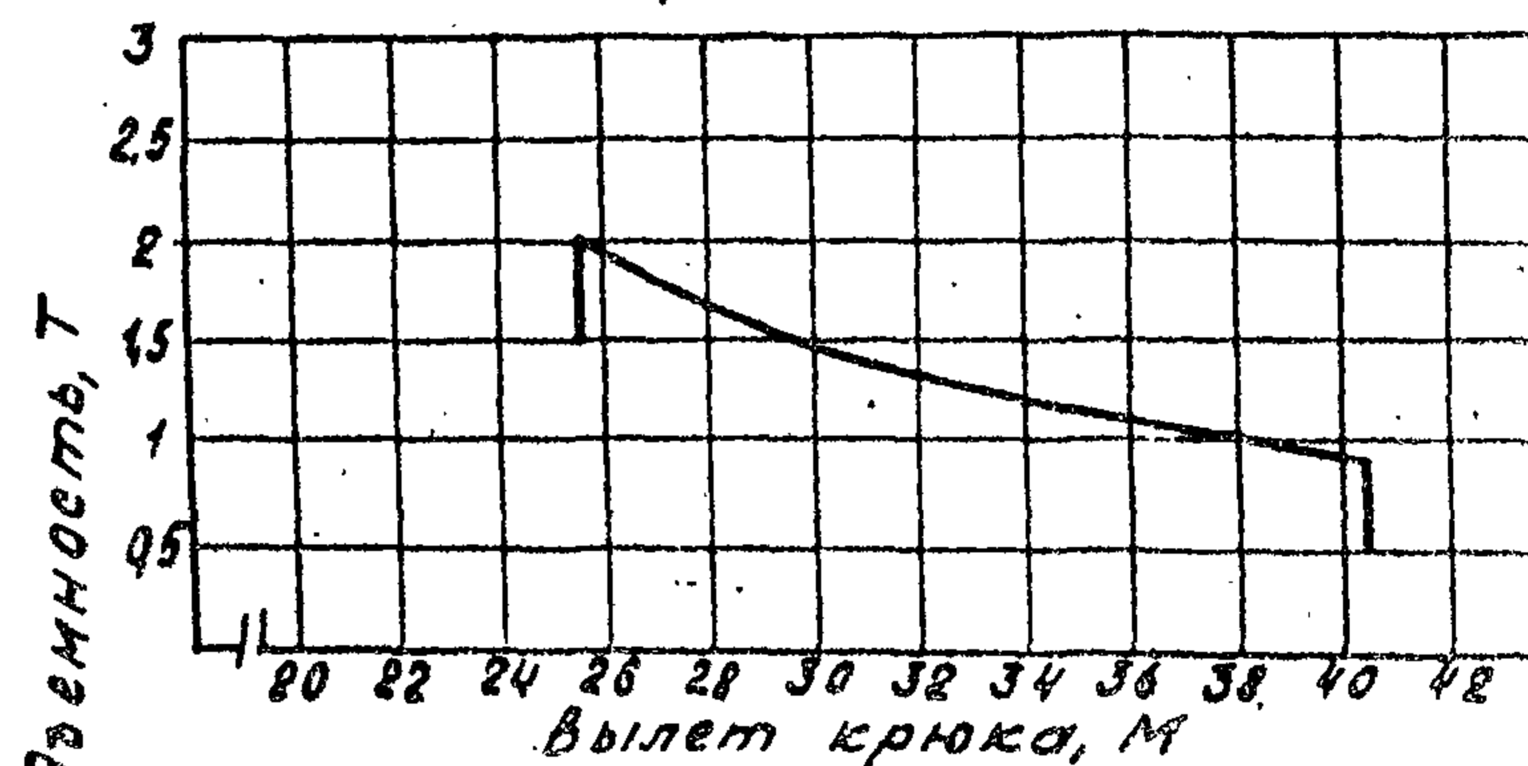
Стрела 80,8 м
