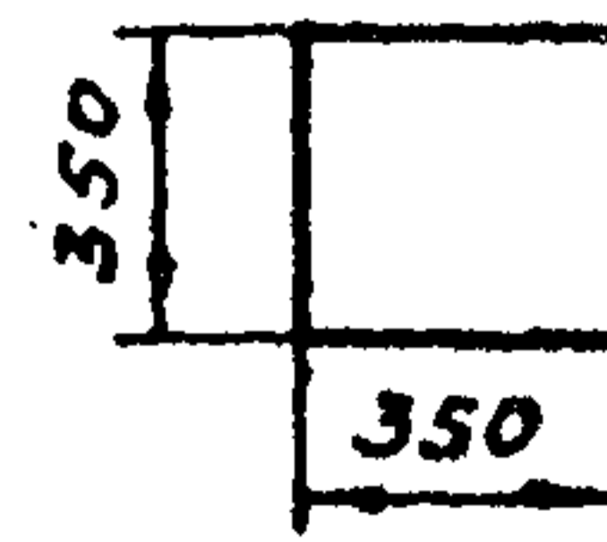
Размеры выносной опоры в плане
