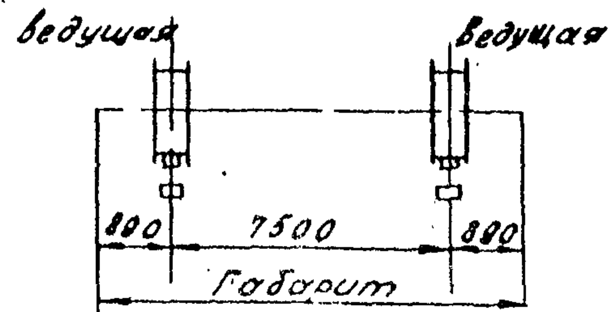
Тележки
