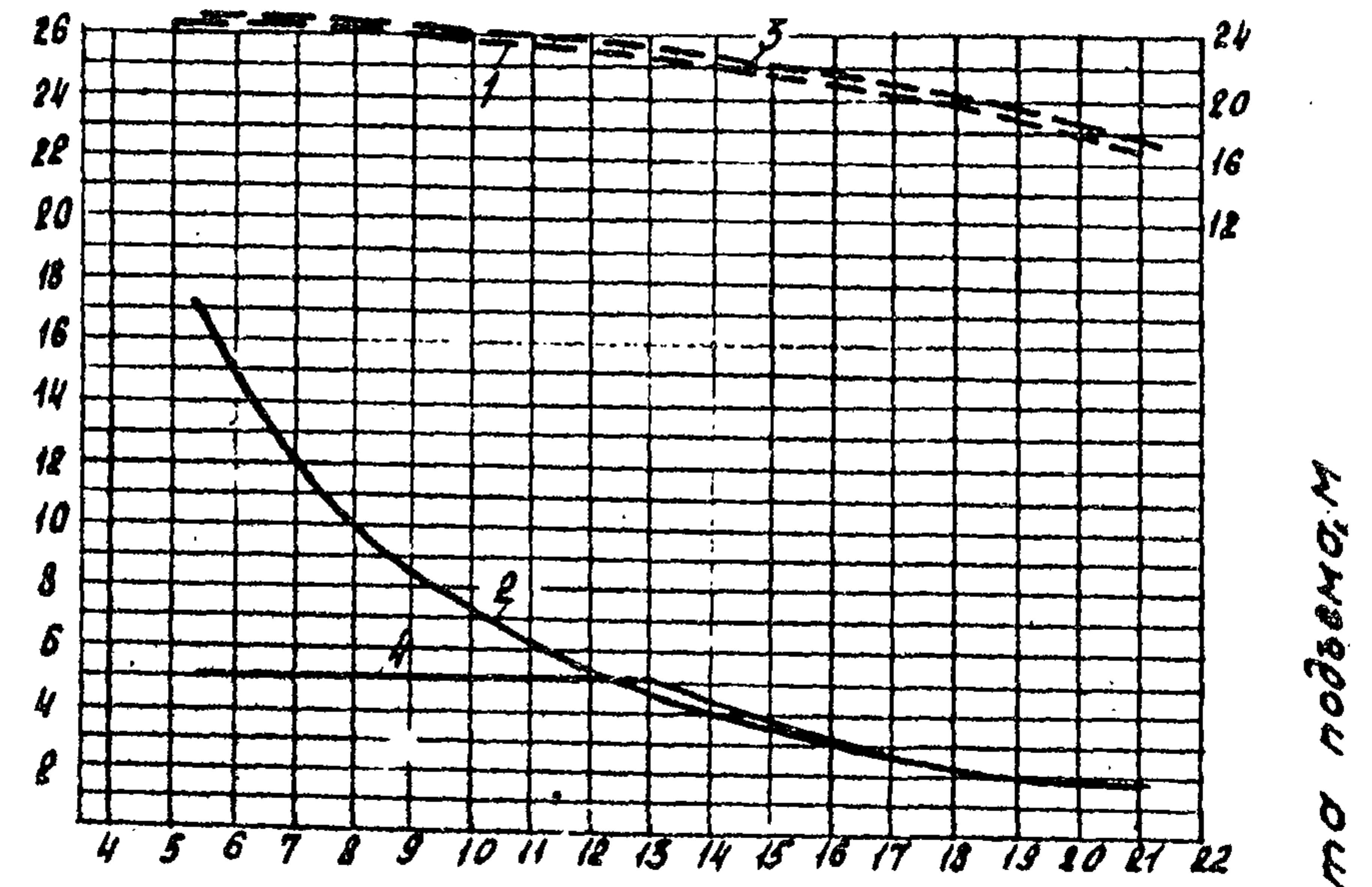
Стрела 30,3м
