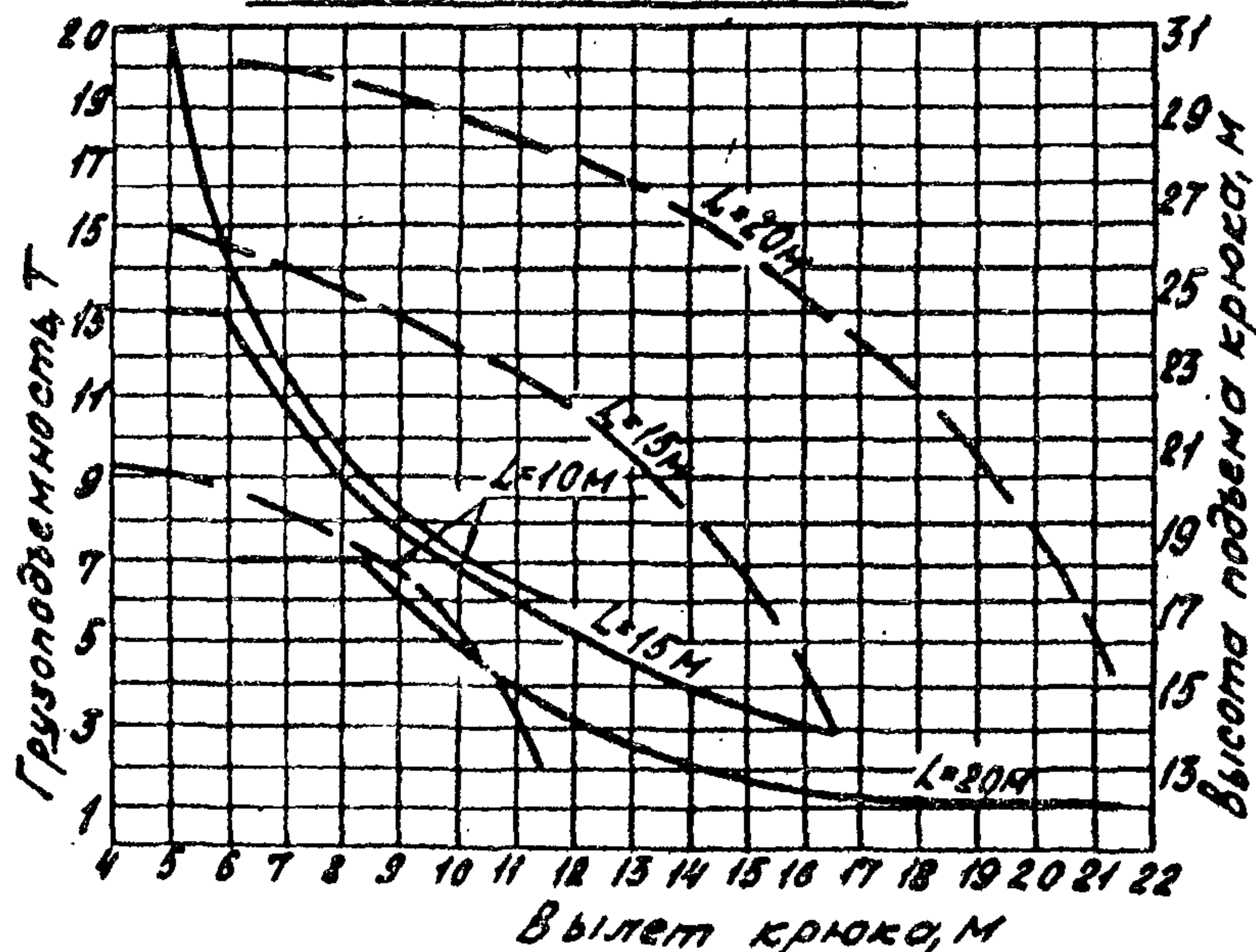
Башня 17,5 метров
