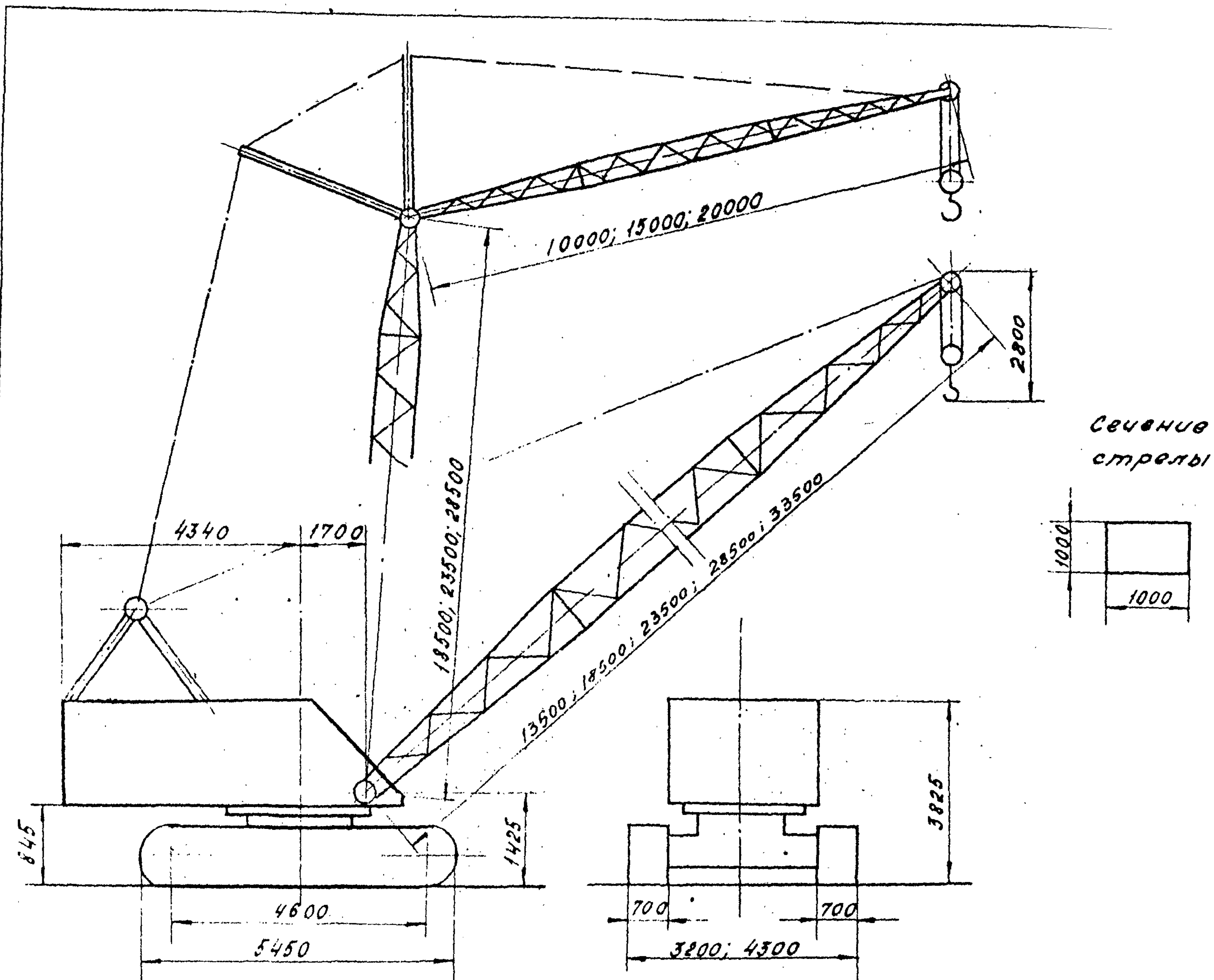
МКГ - 25 Бр
