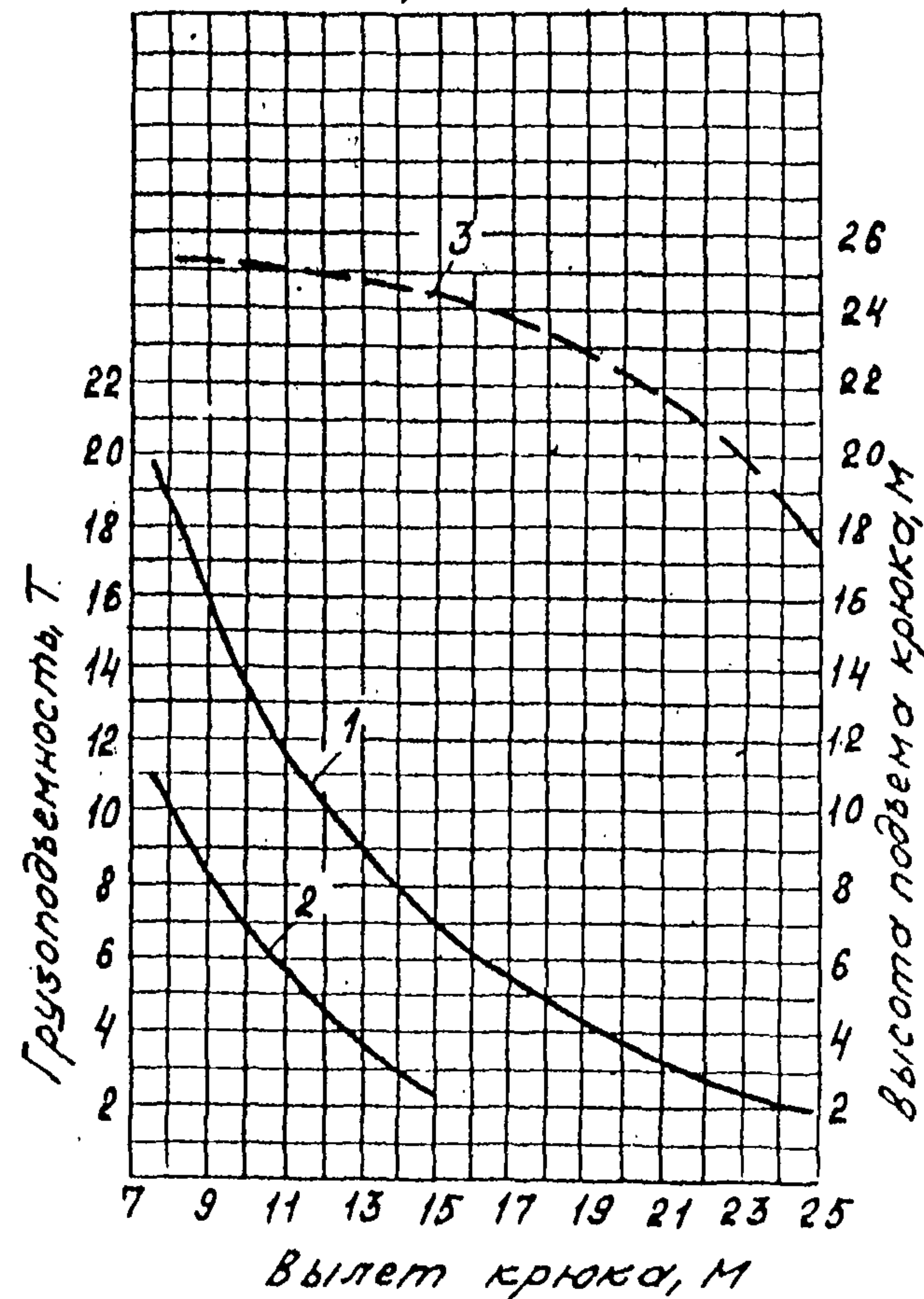
Стрела 31 м
