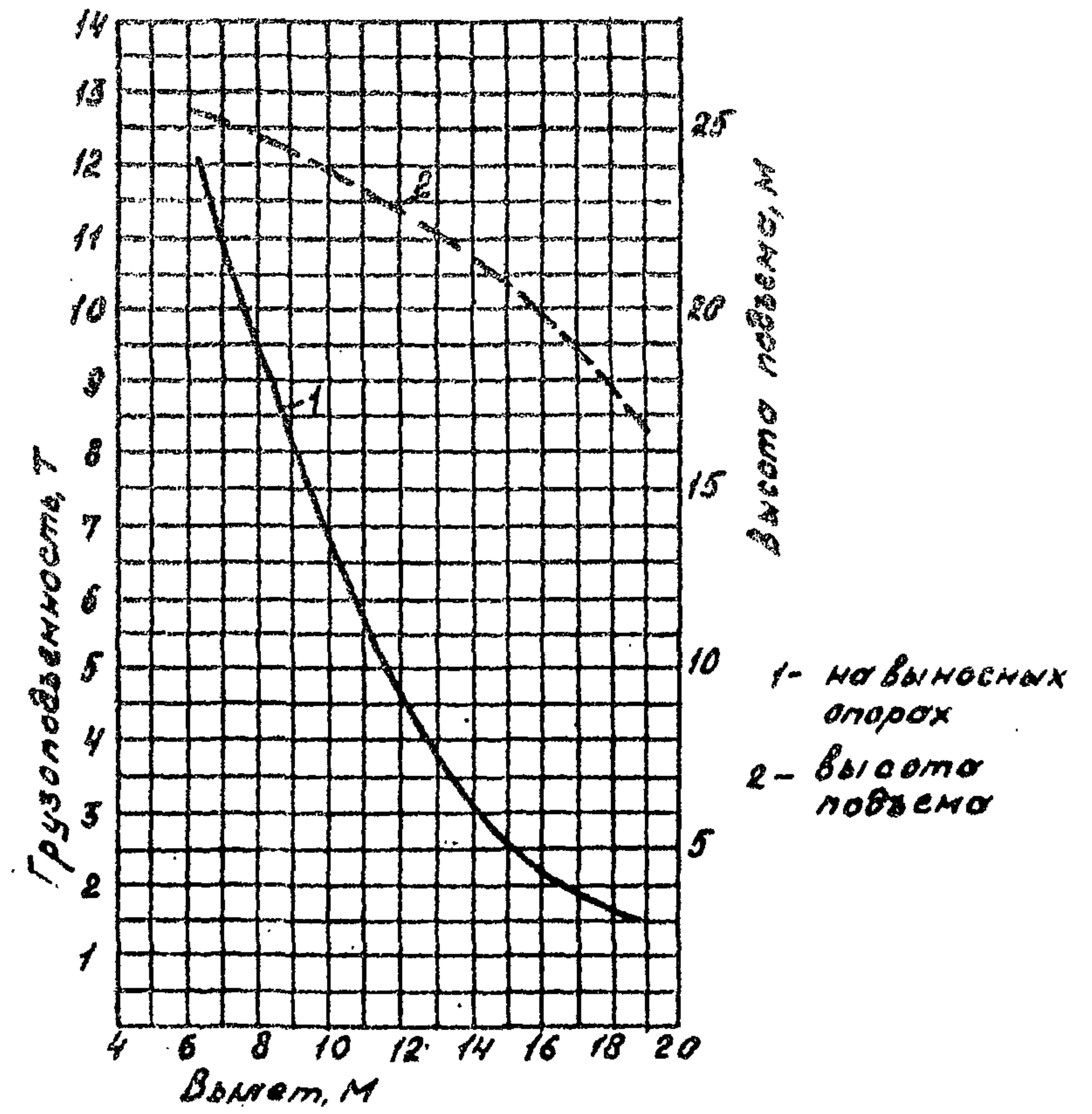
Графики грузоподъемности "высоты подъема" в зависимости от вылетов для стрелы 27,5м
