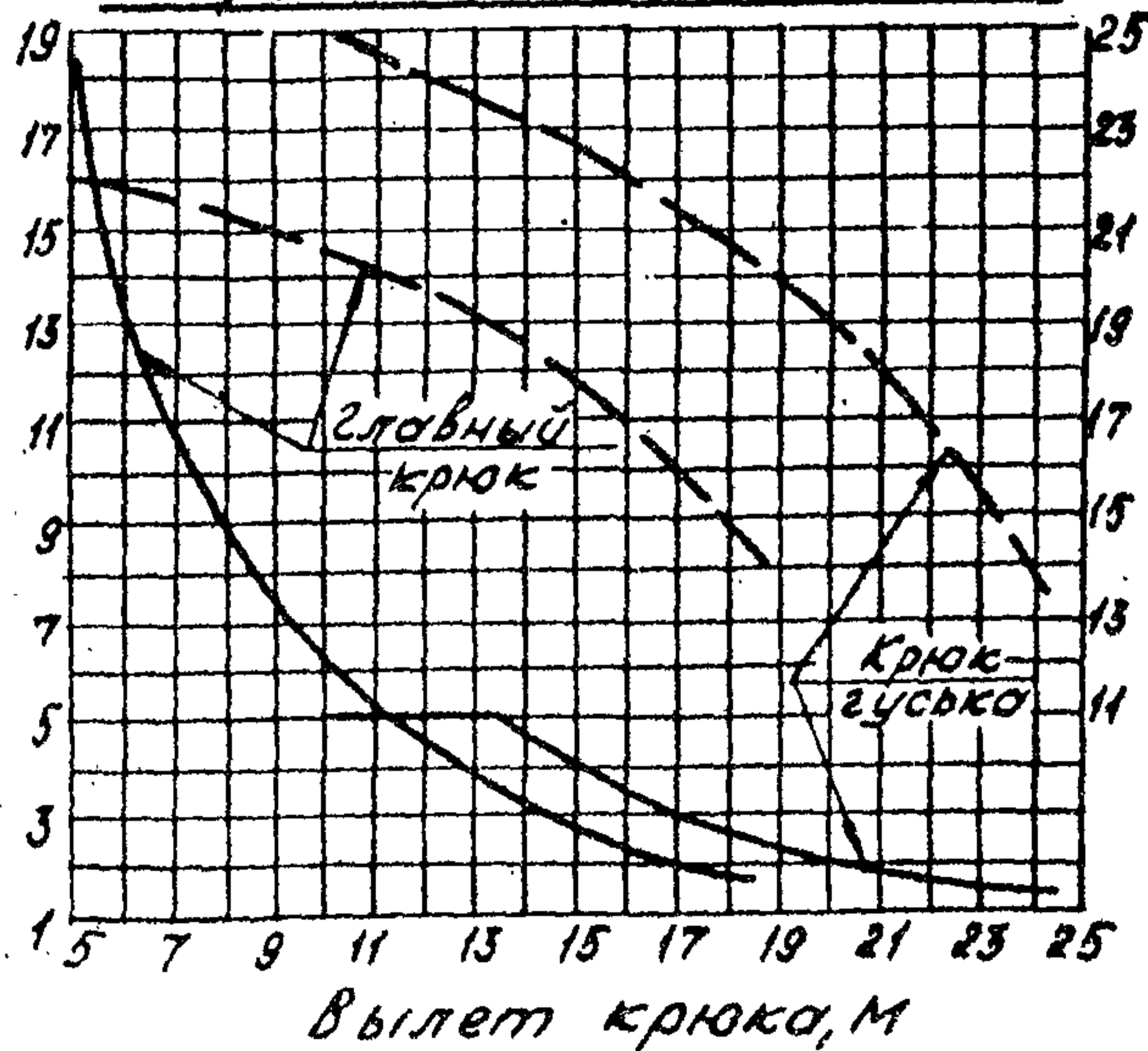
Стрела 22,5 м с гуськом 5 м
