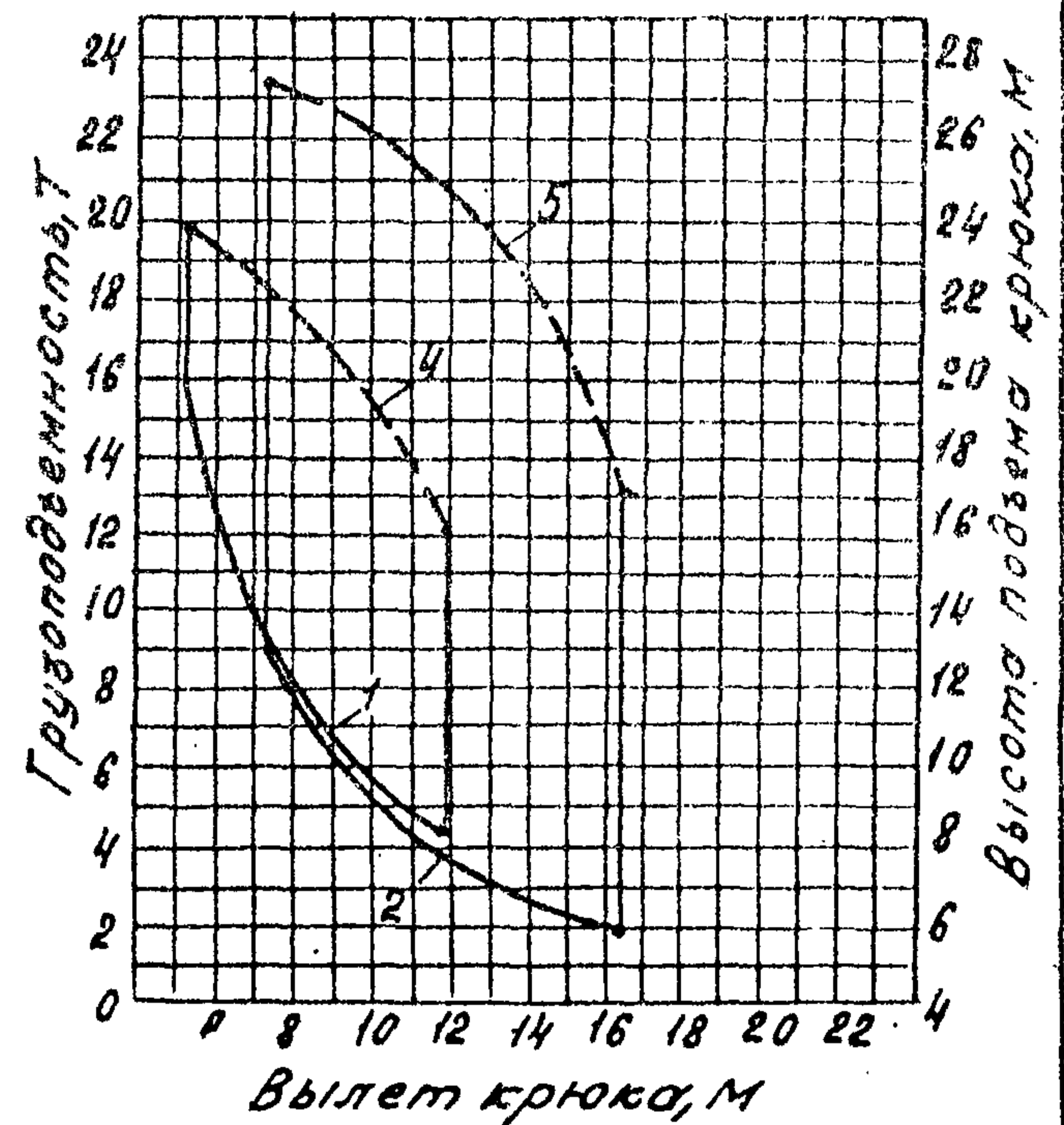
Башня 15м, гуськи 10 и 15м
