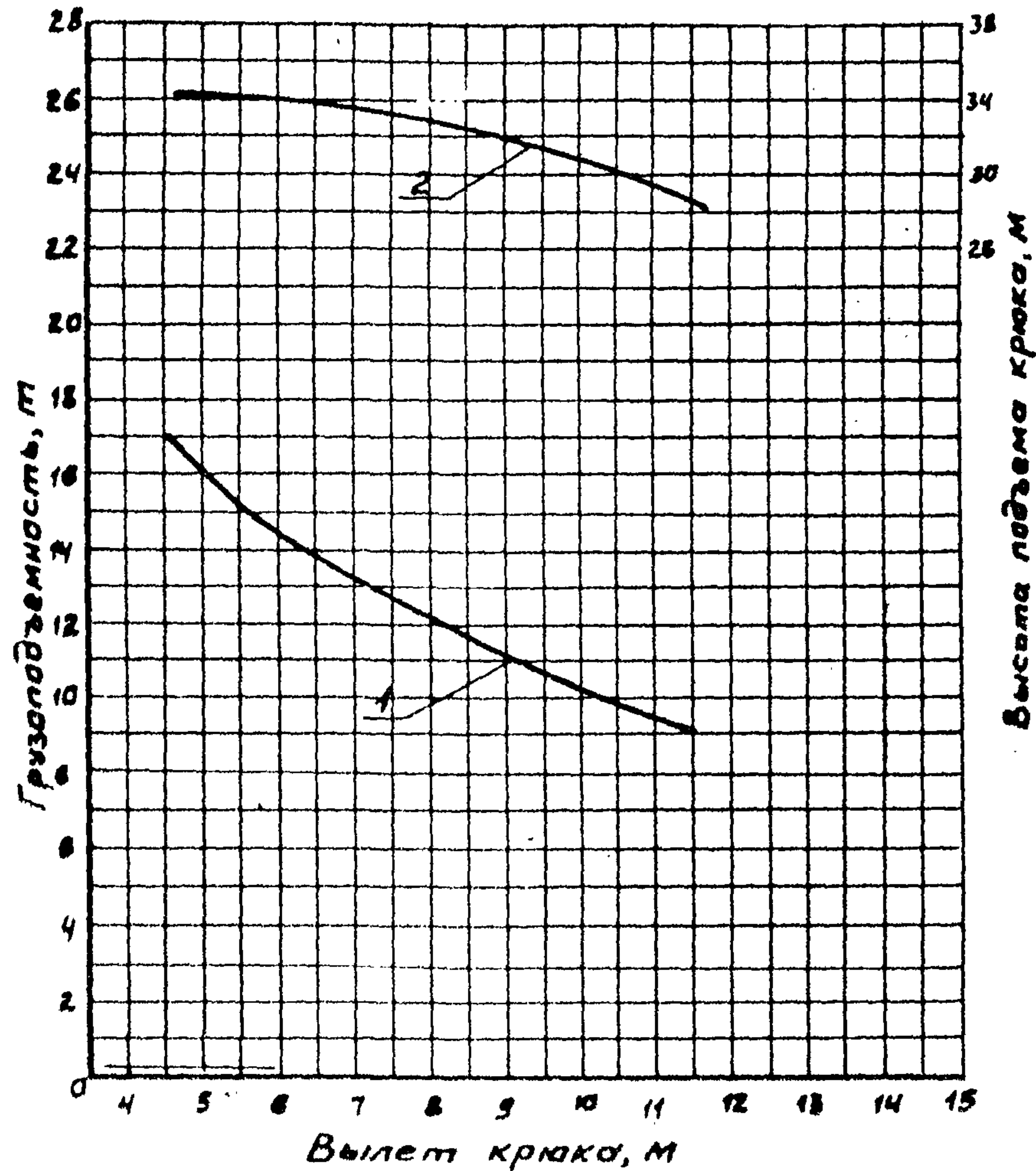
Башня 26 м
