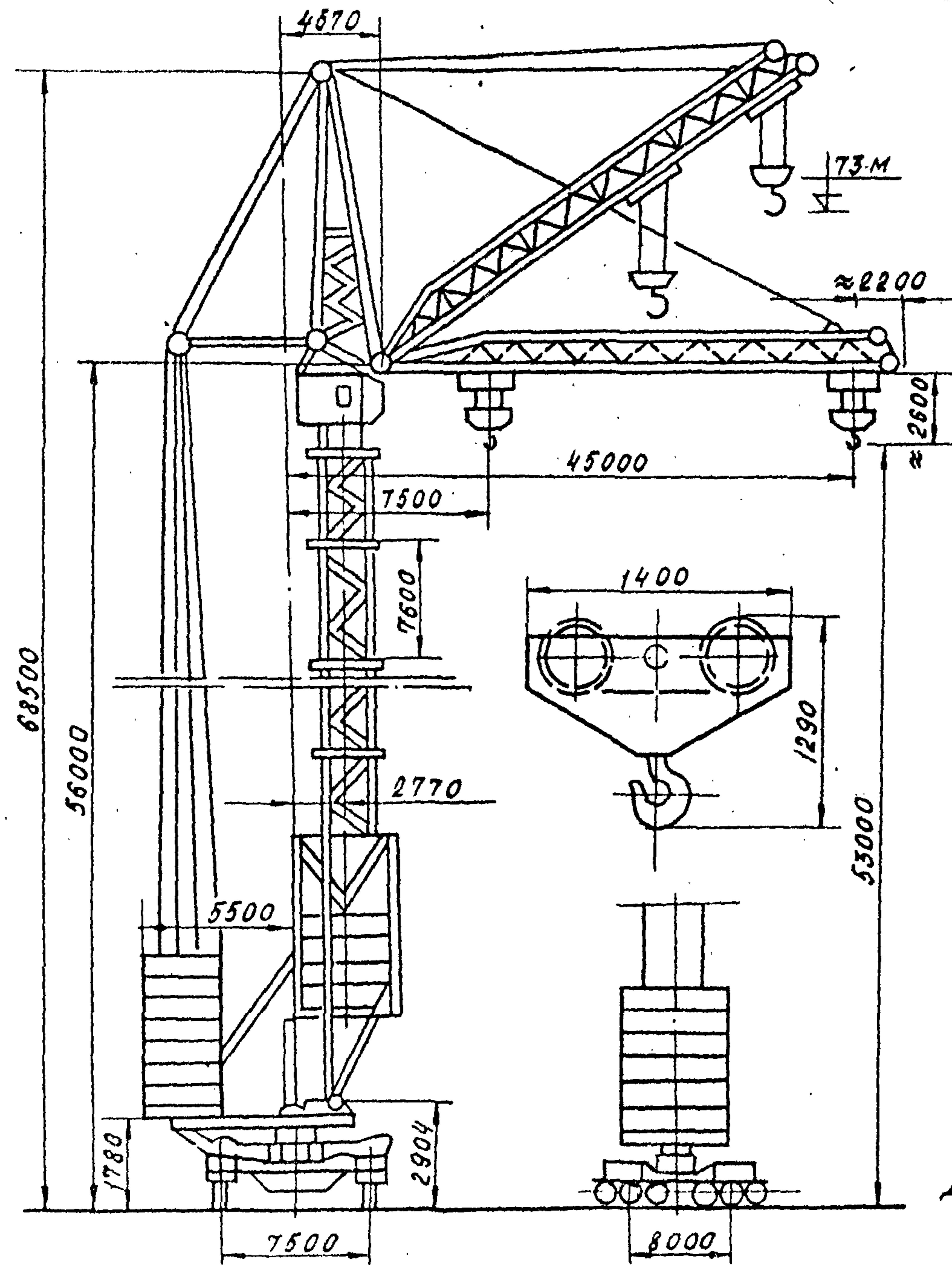
Наружные габариты башни
