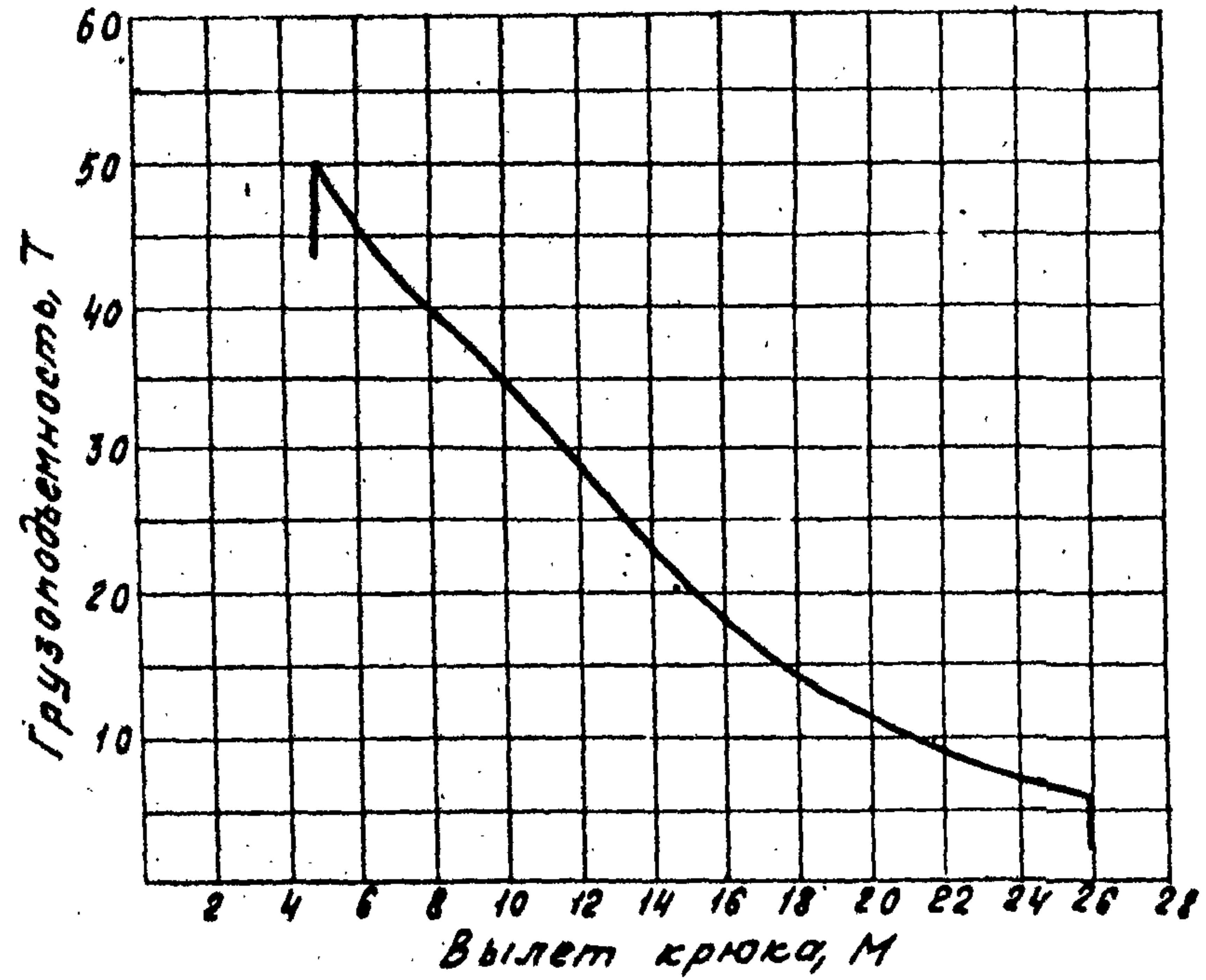
Стрела 27м
