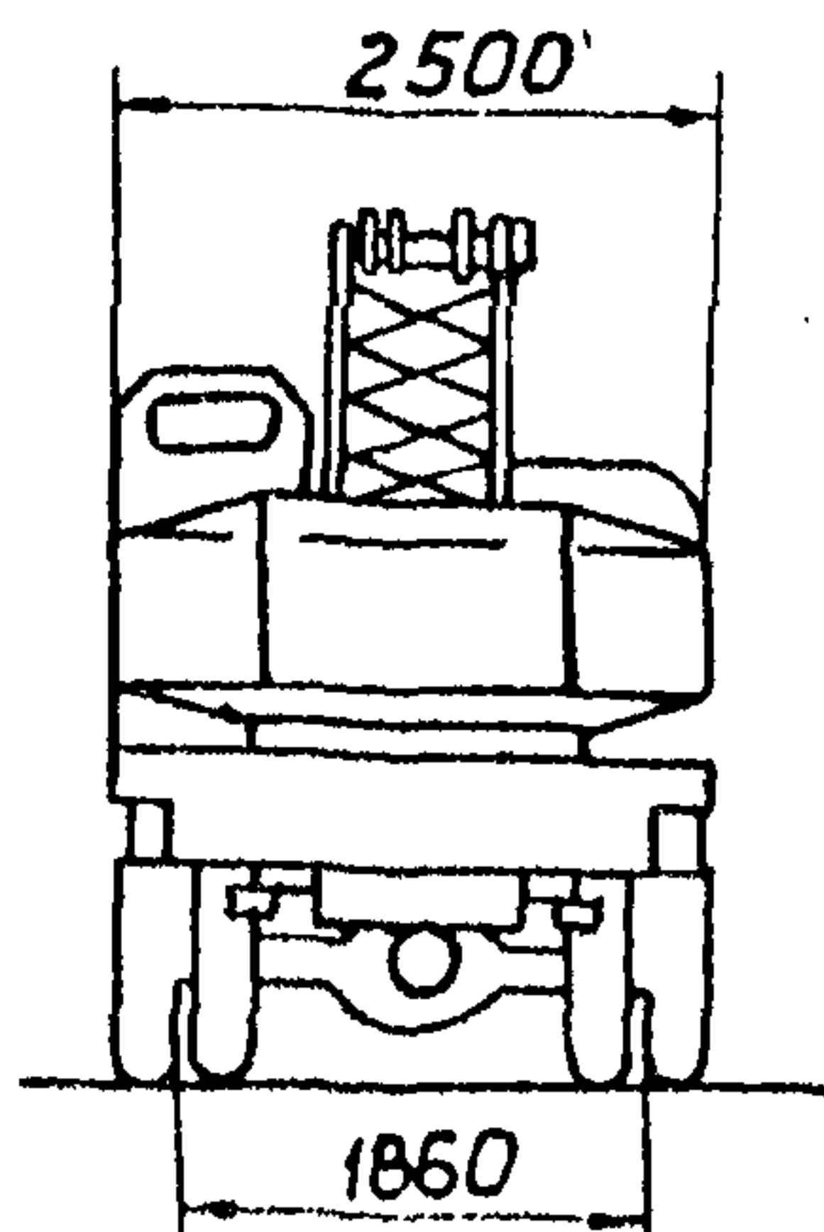
Вид А
