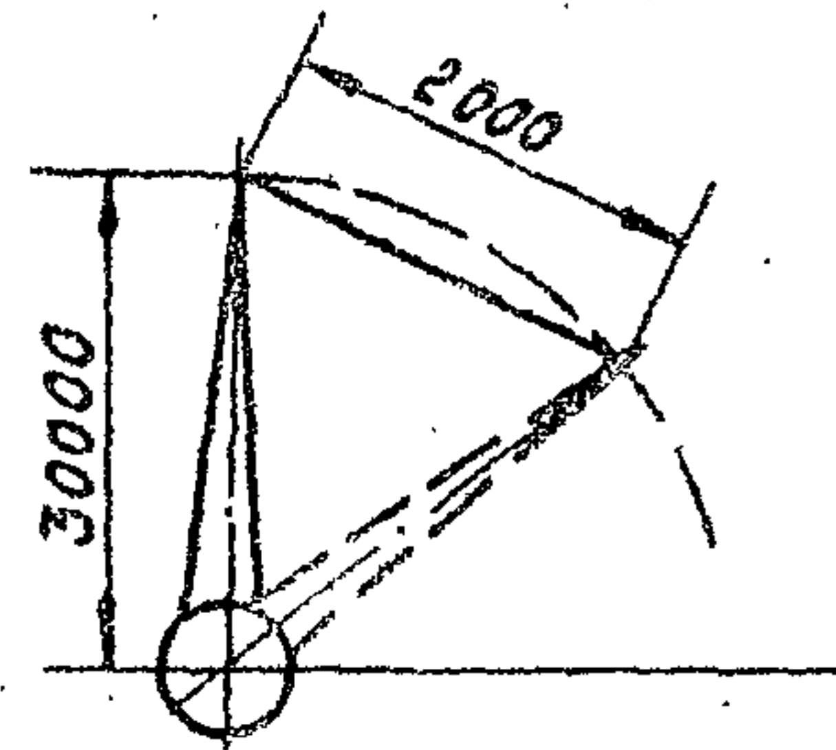
Тормозной путь стрелы с предельным грузом
