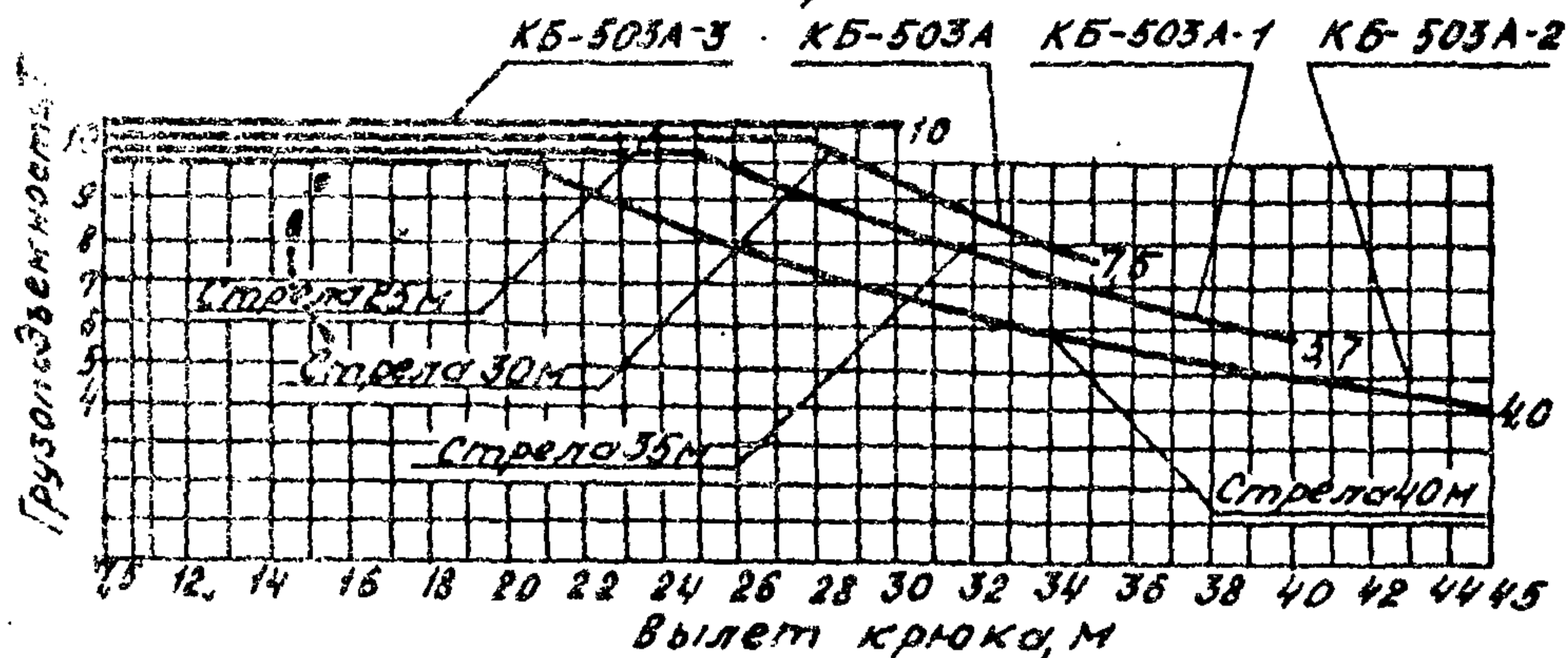
График грузоподъемности при горизонтальном положении стрелы
