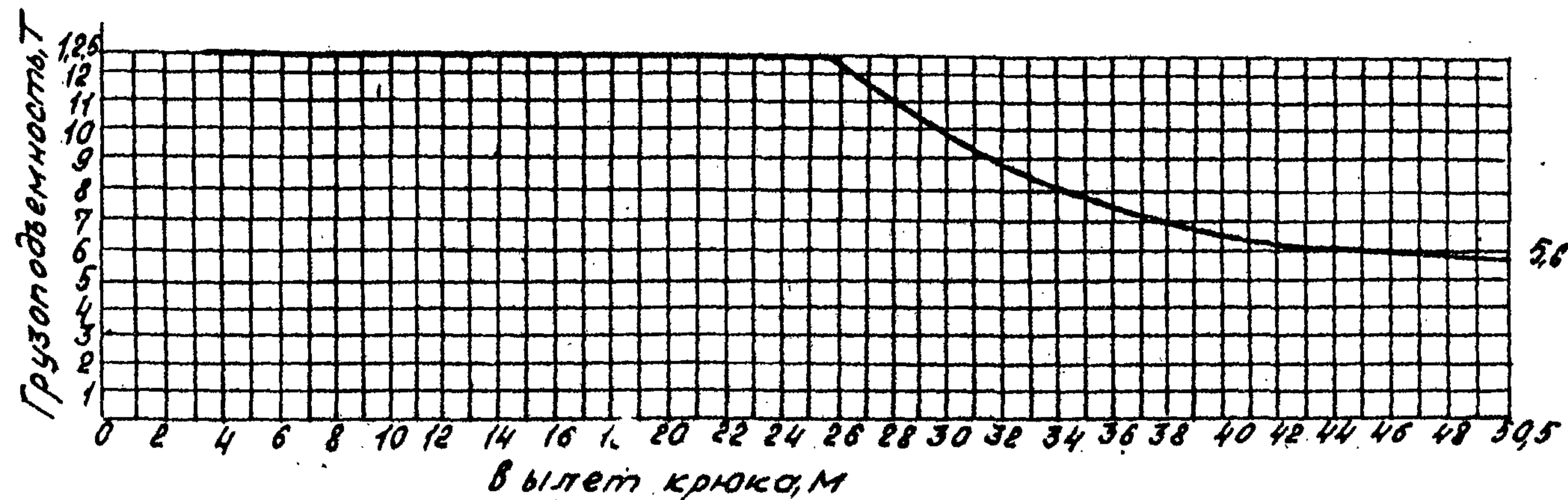
График грузоподъемности крана КБ-676-0; КБ-676,2
