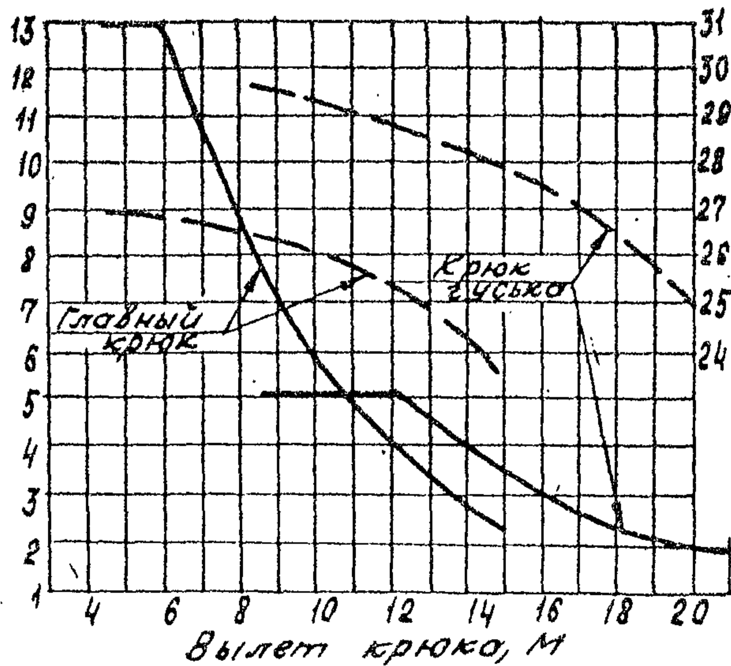
Стрела, 27,5 м
