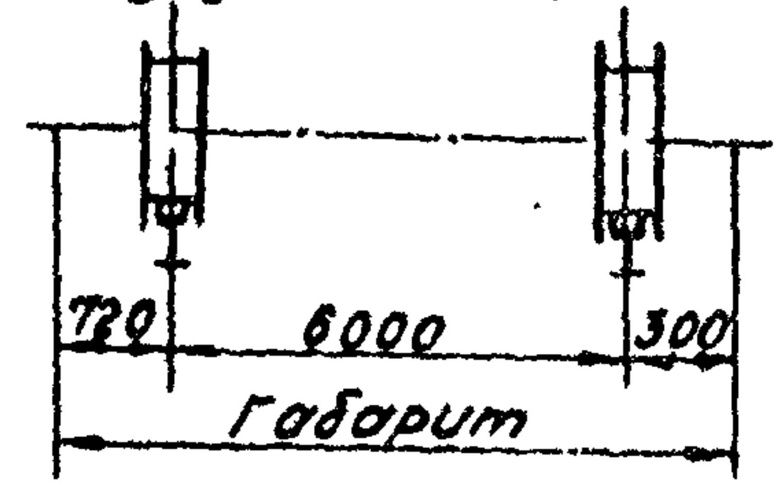
Тележки ведущая ведомая
