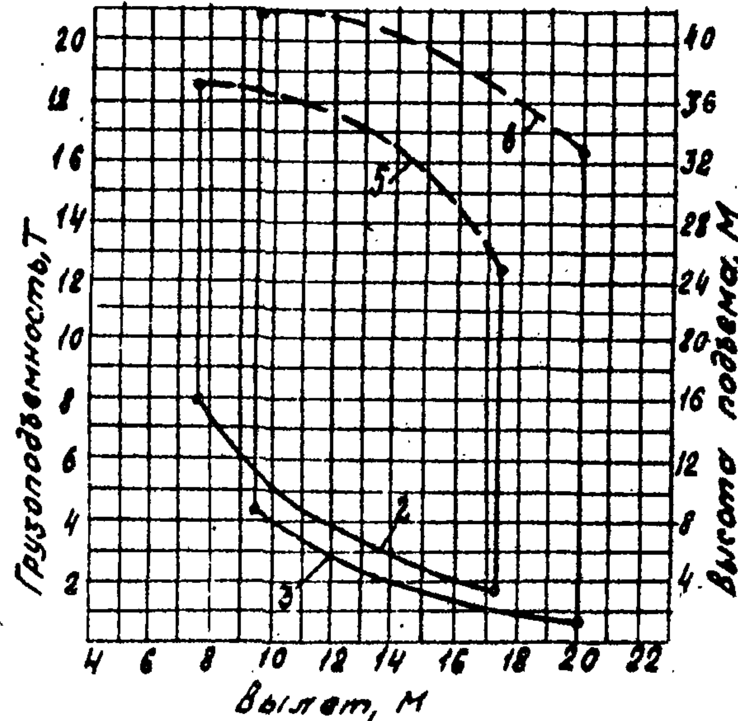
Башня 25 м гуськи 15 м и 20 м
