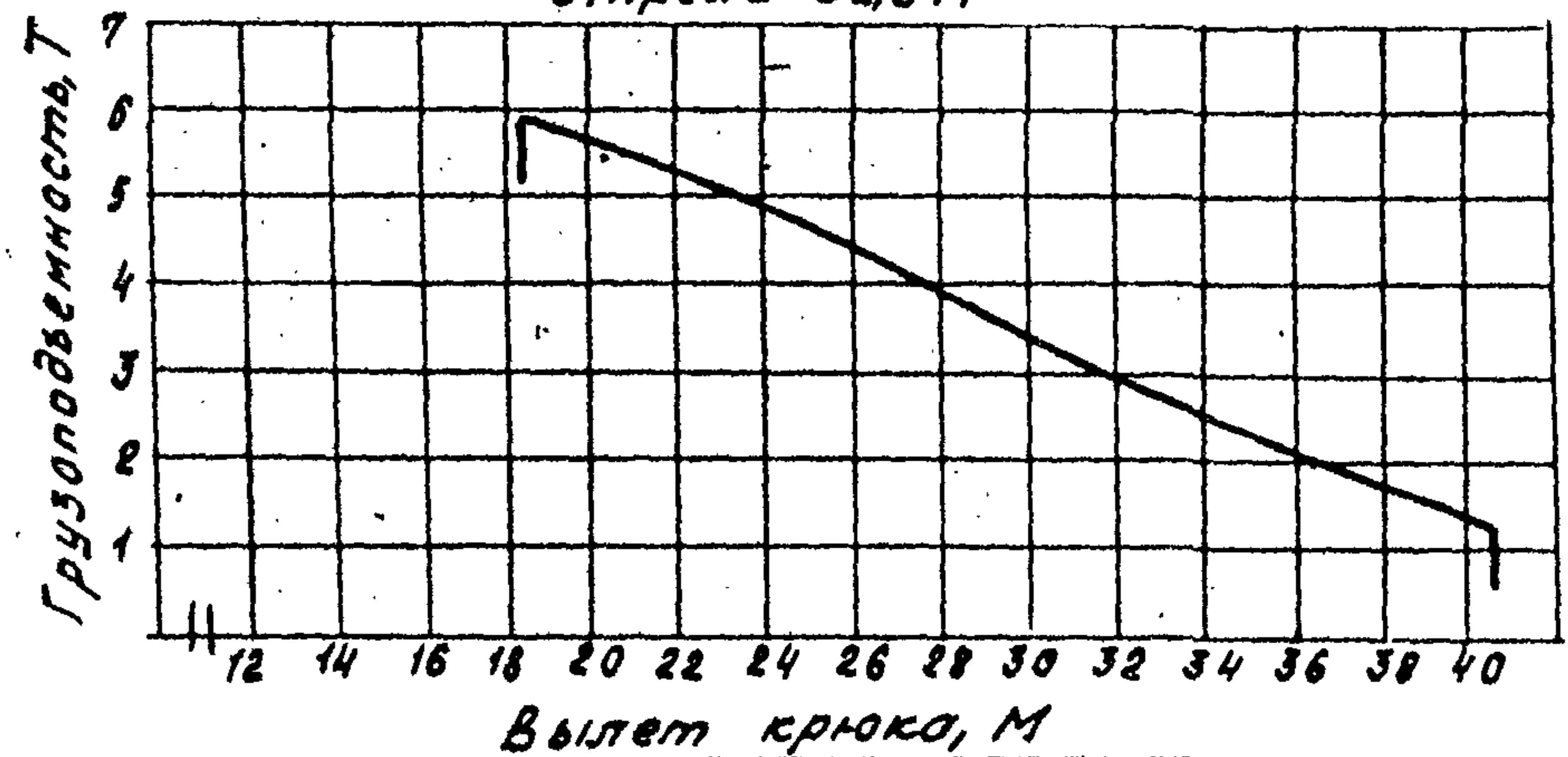
Стрела 62,8м
