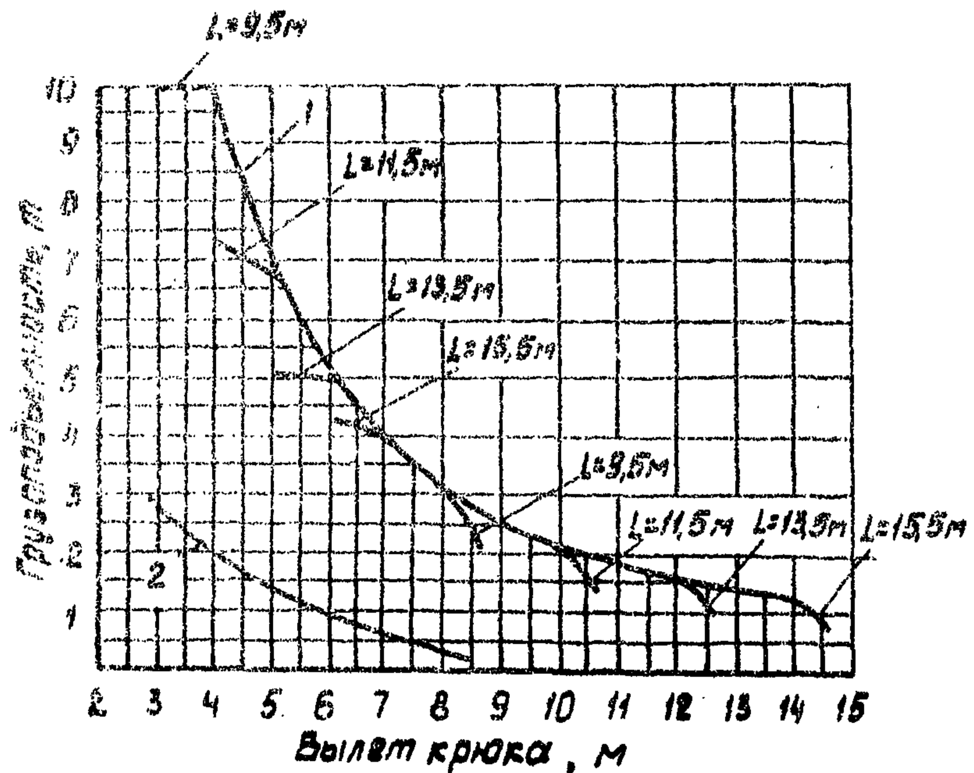
Графики грузоподъемности
