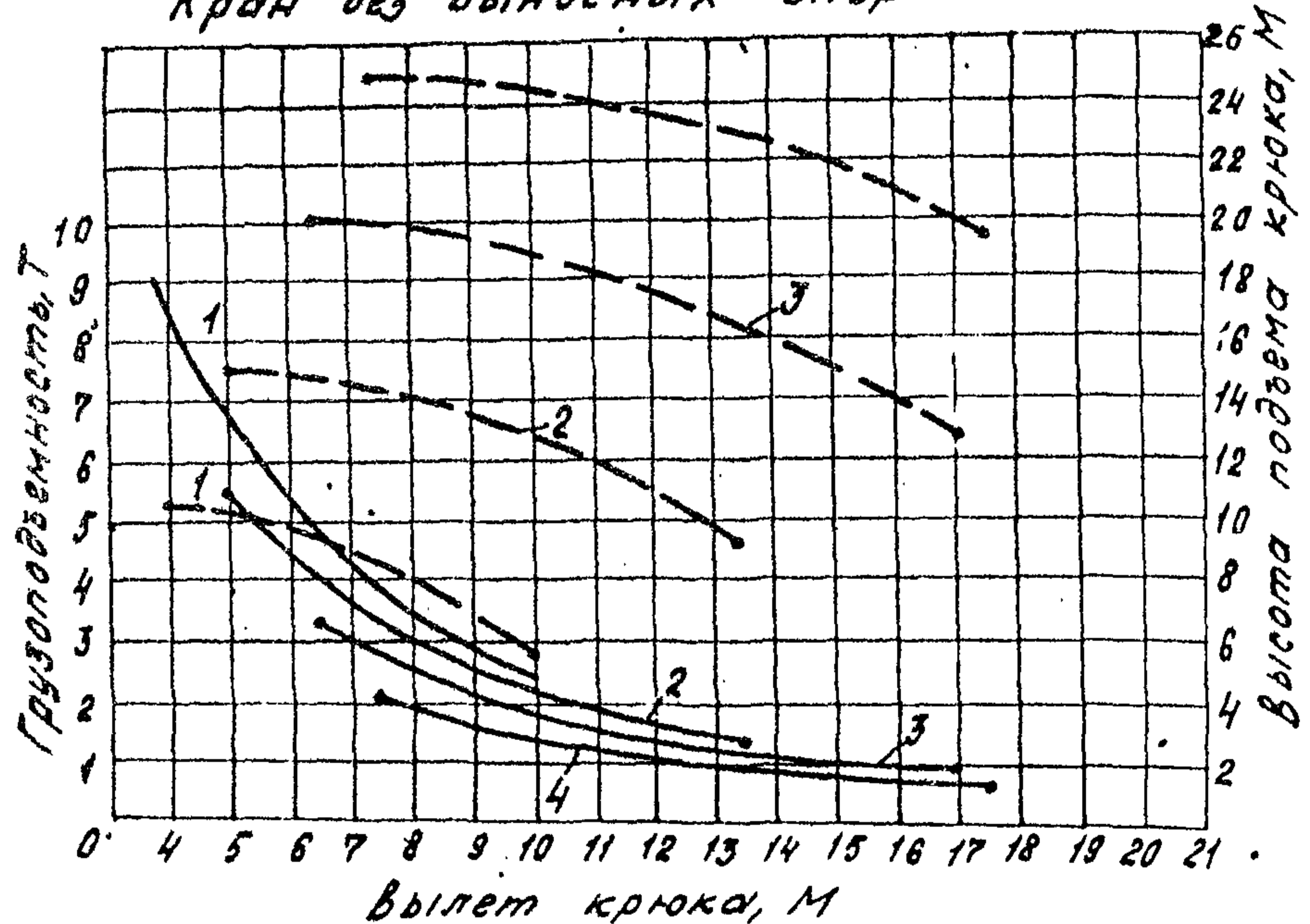
Башенно-стреловое оборудование
