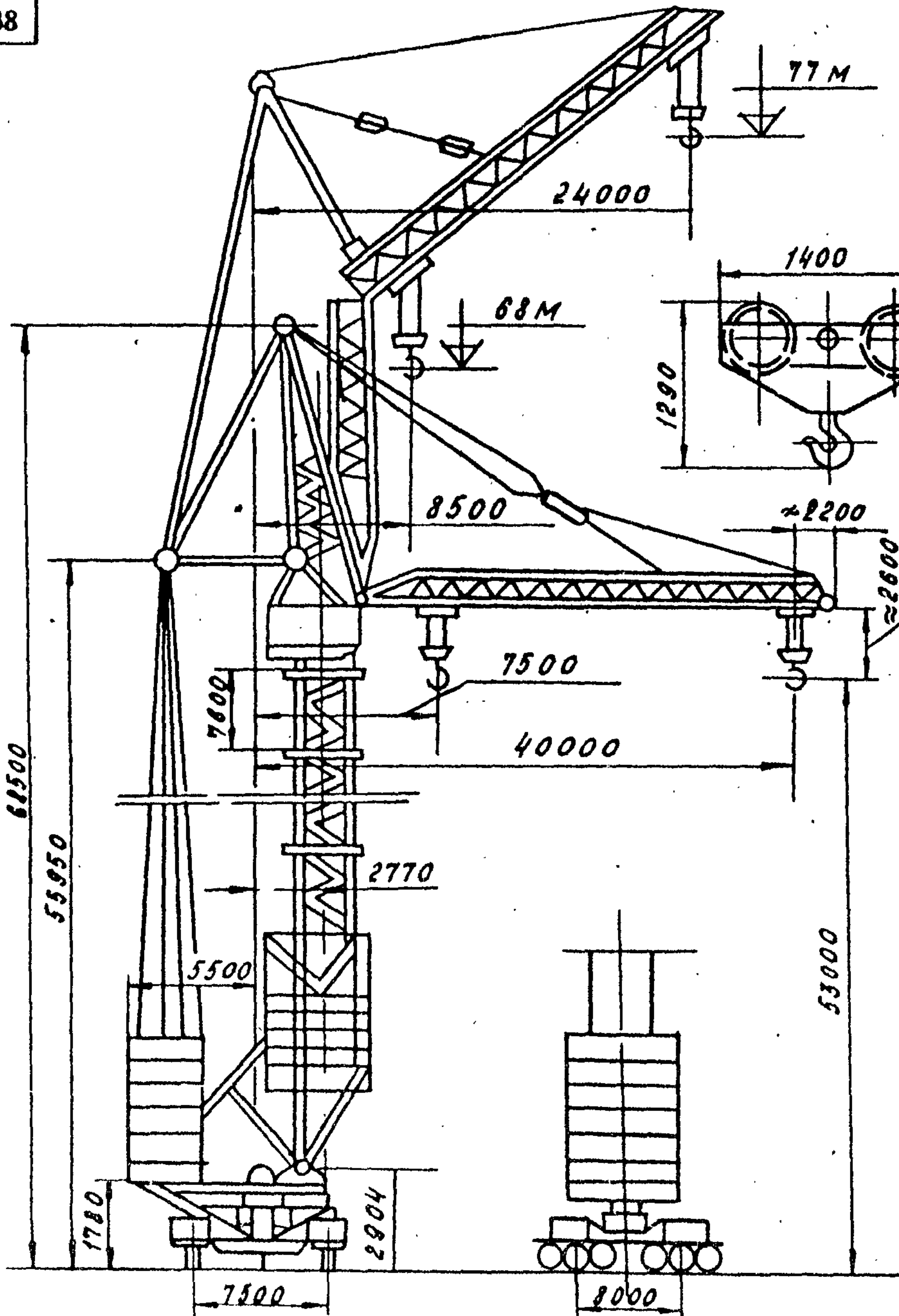
Наружные габариты стрелы
