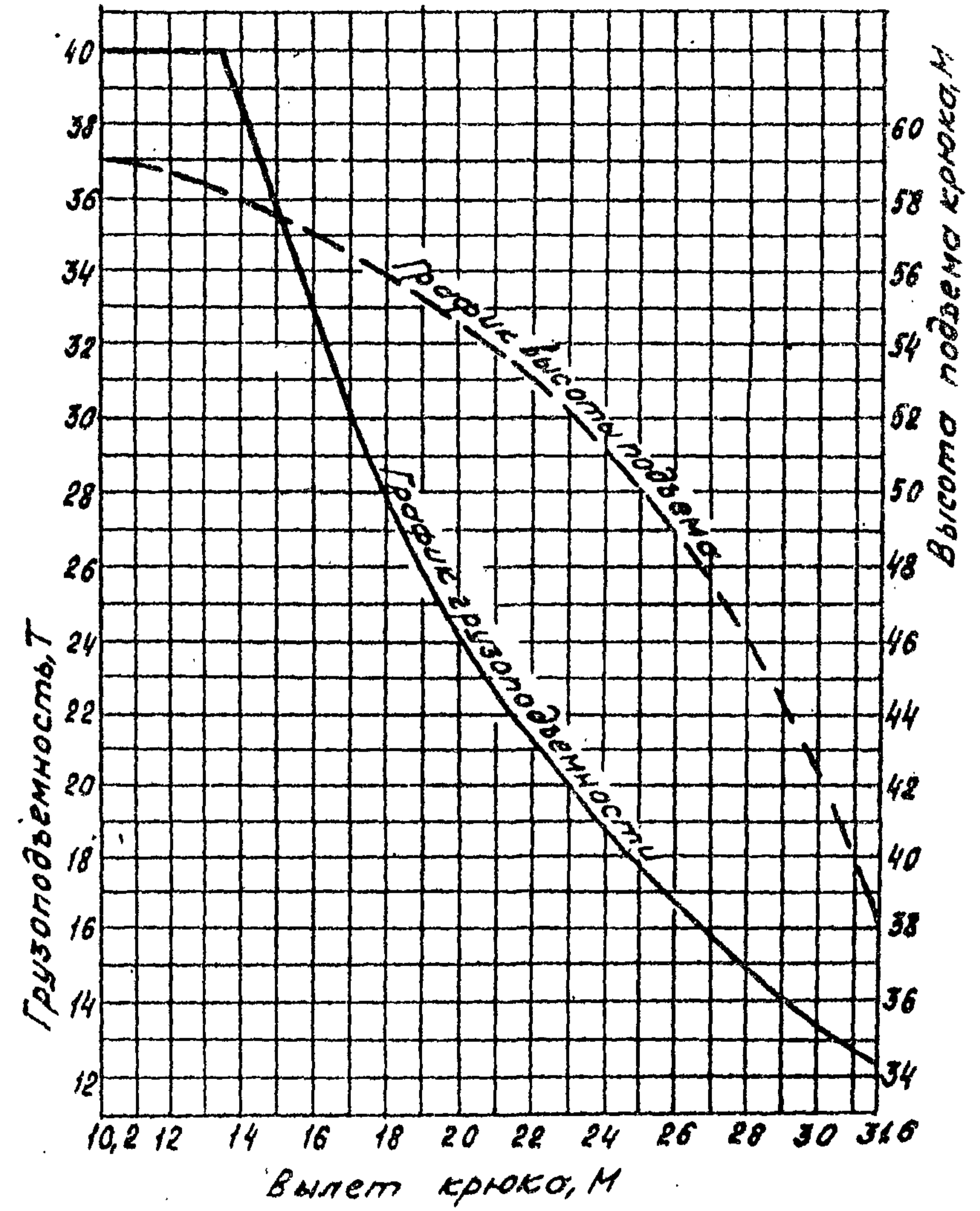
Стрела 31м с гуськом 30м
