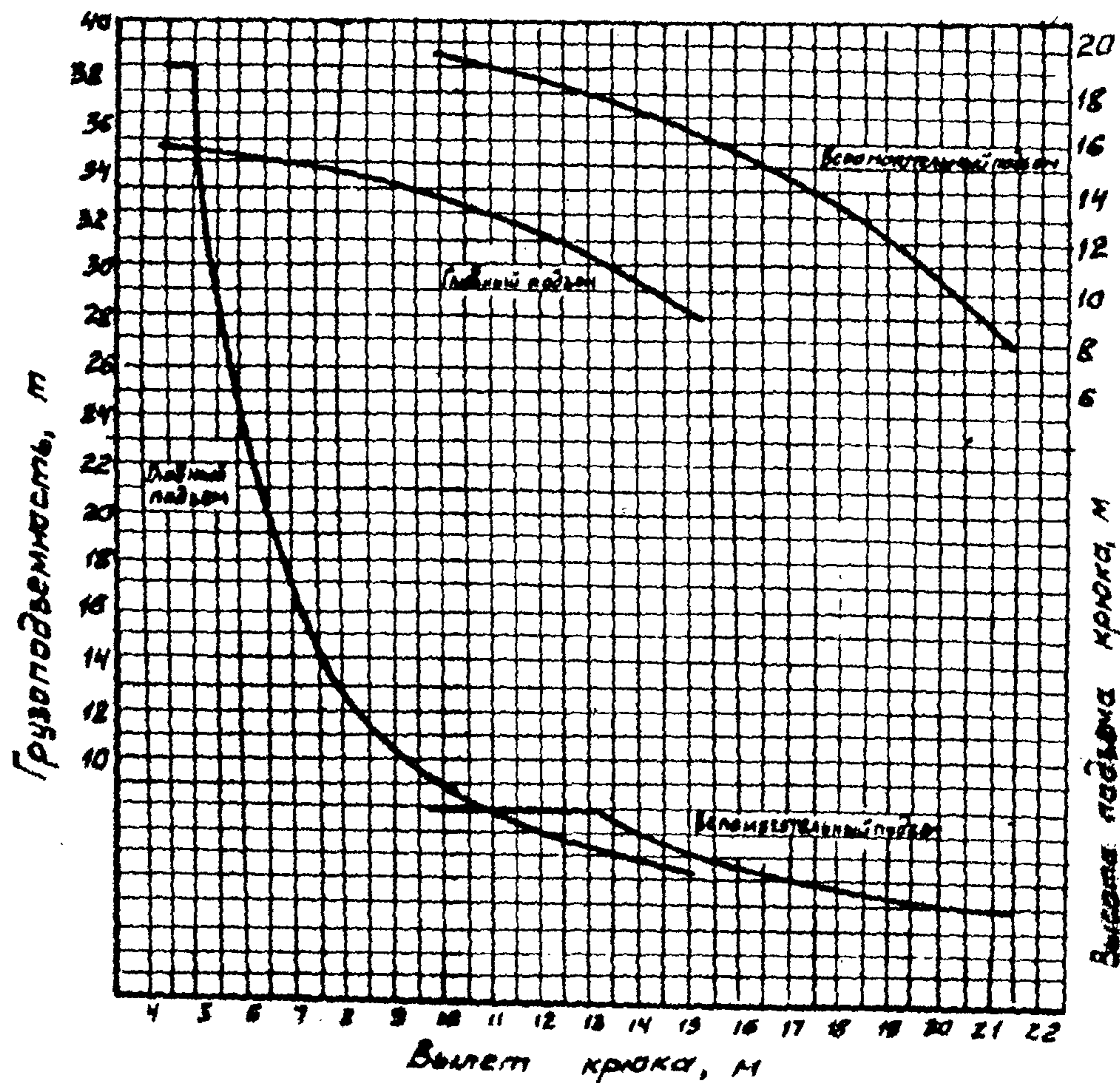
Стрела 16 м с гуськом 6 м
