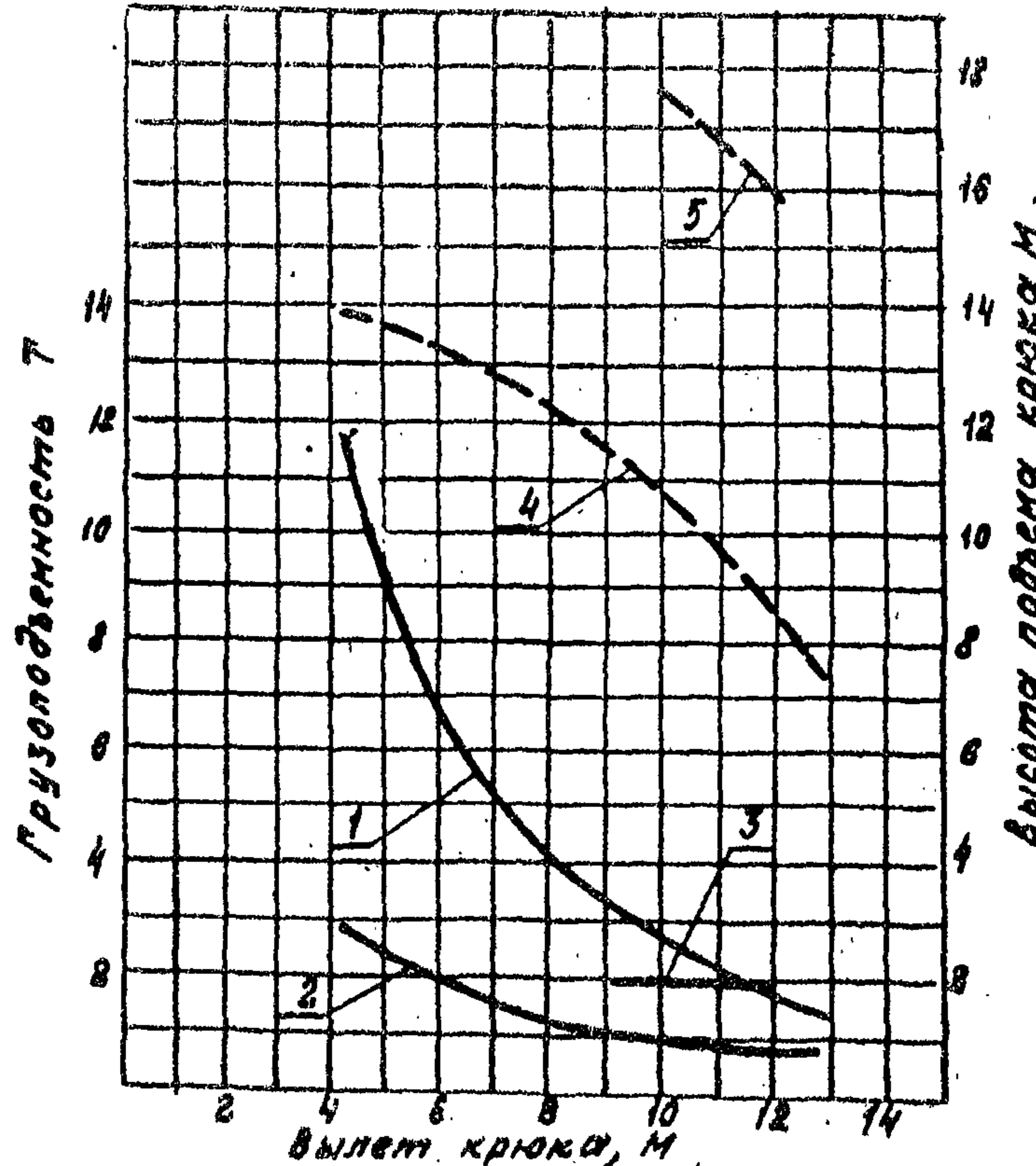
Стрела 14 м
