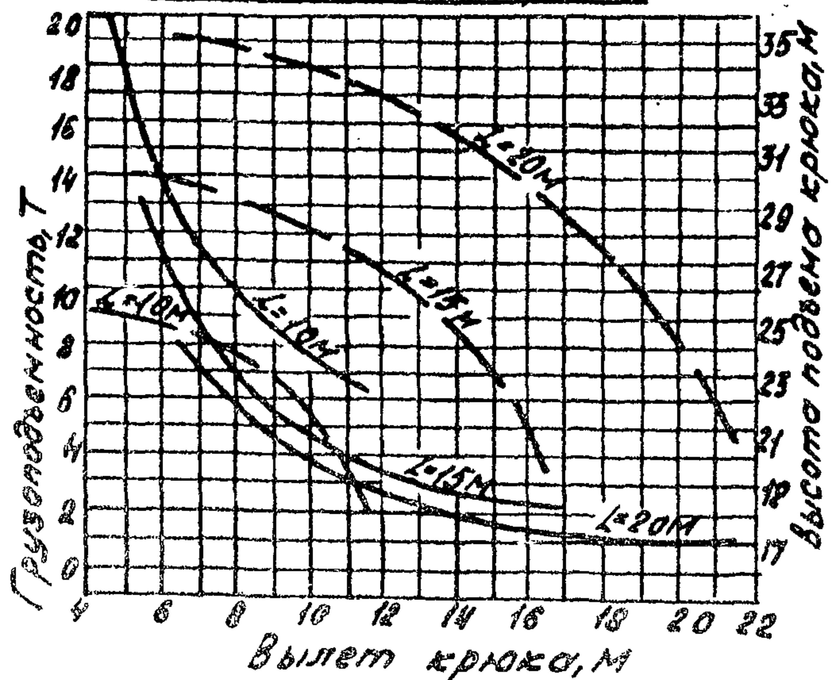
Башня 17,5 метров
