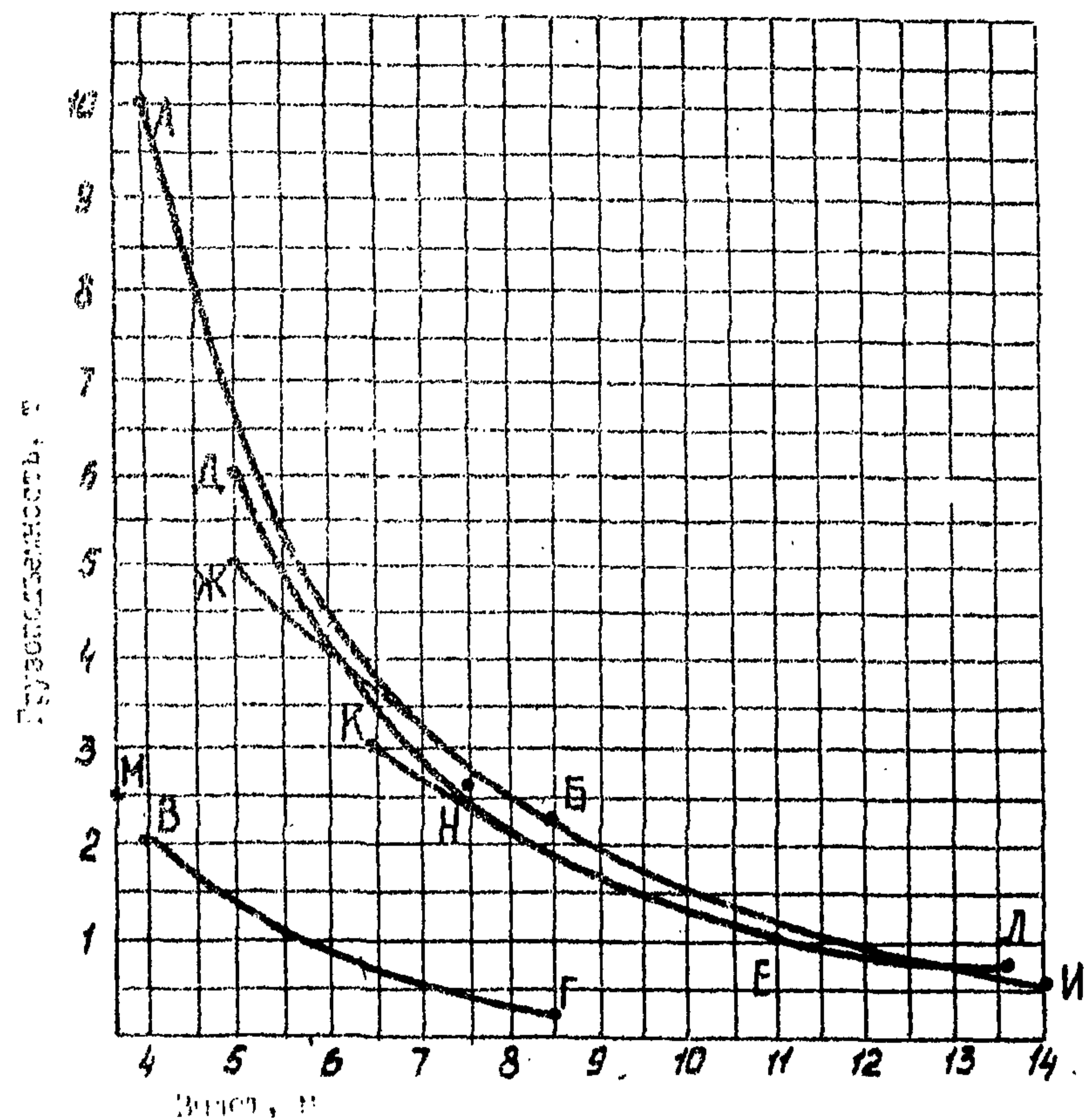
График грузоподъемности
