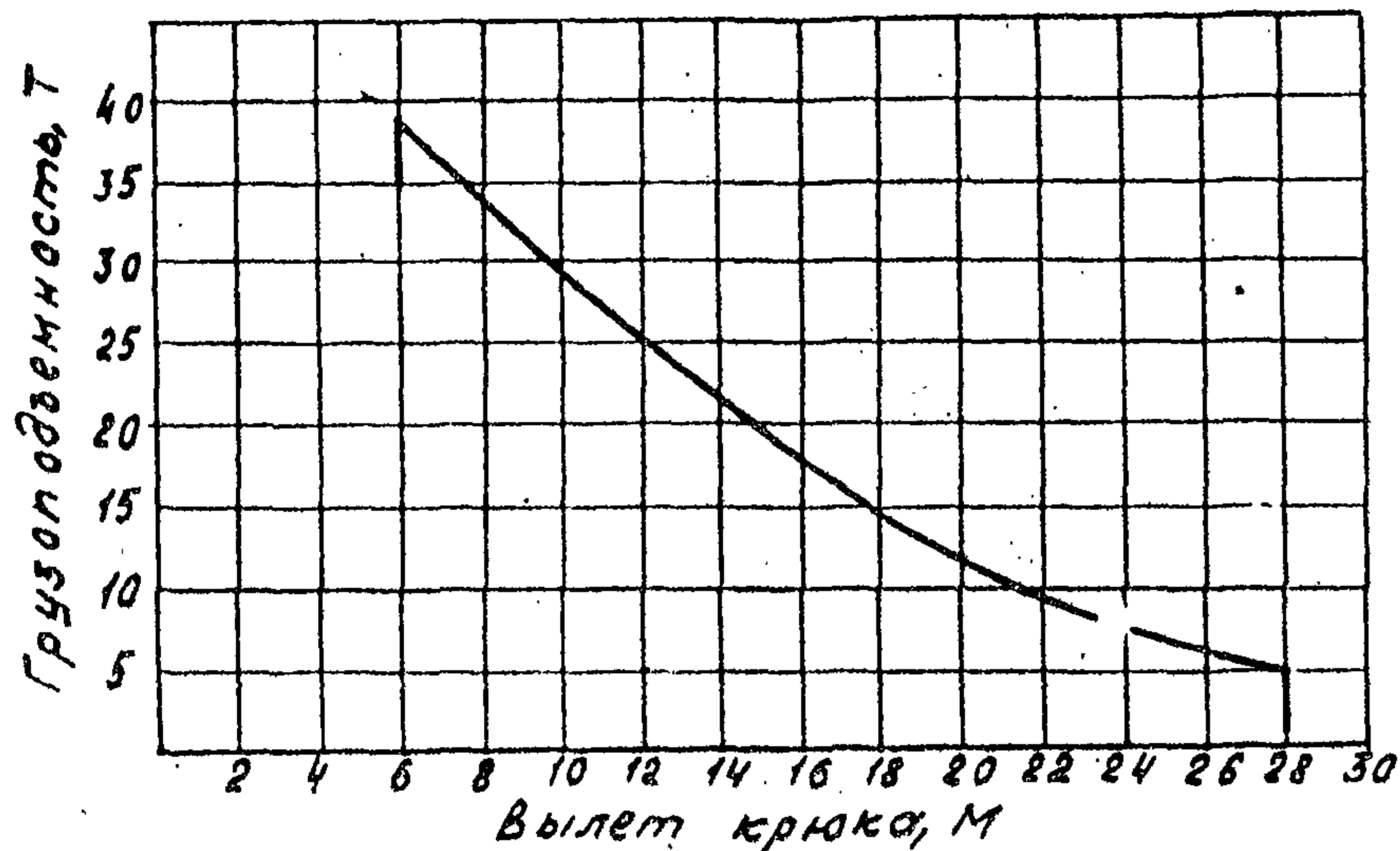
Стрела 30 м
