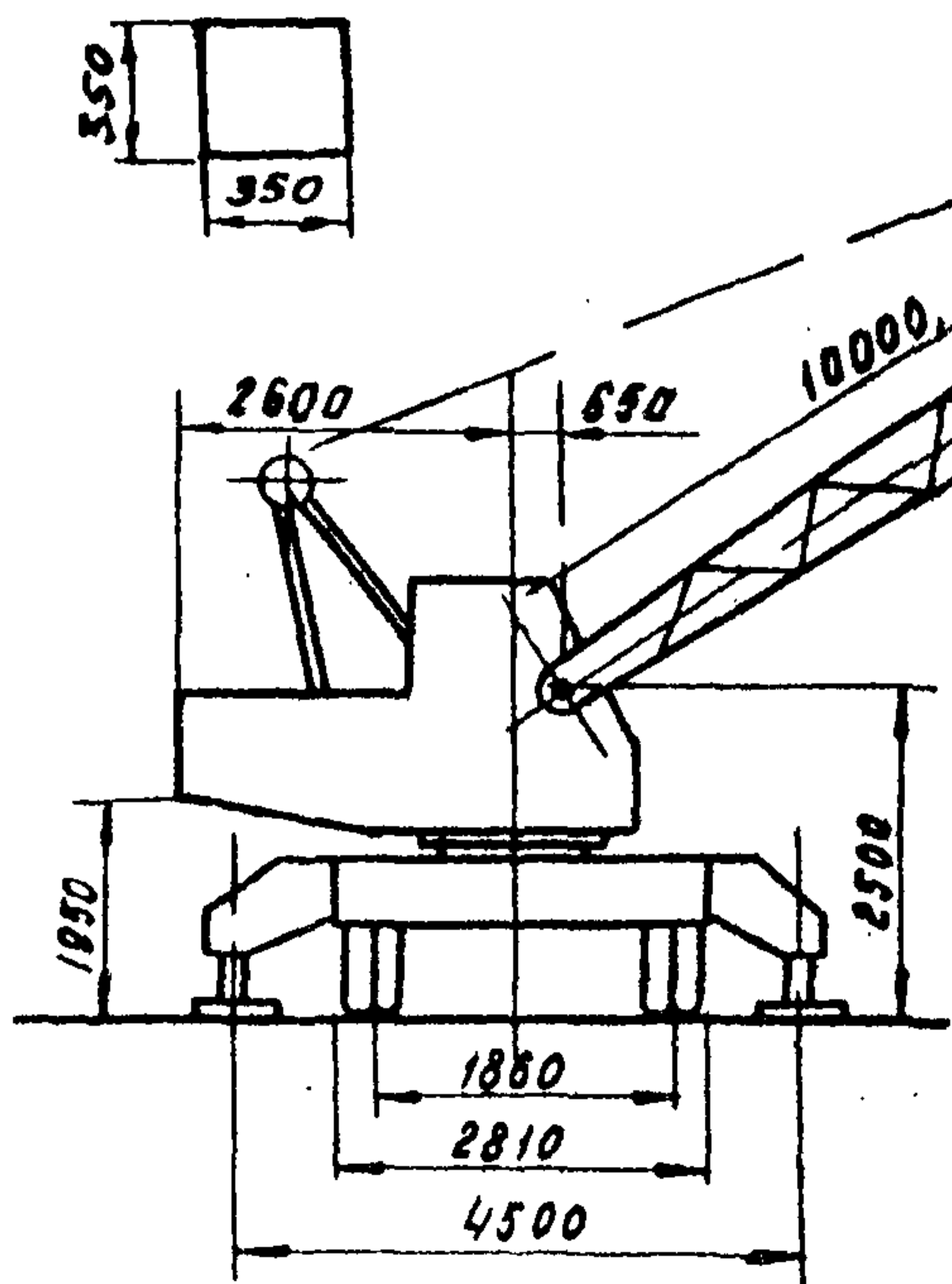
Размеры выносной опоры в плане
