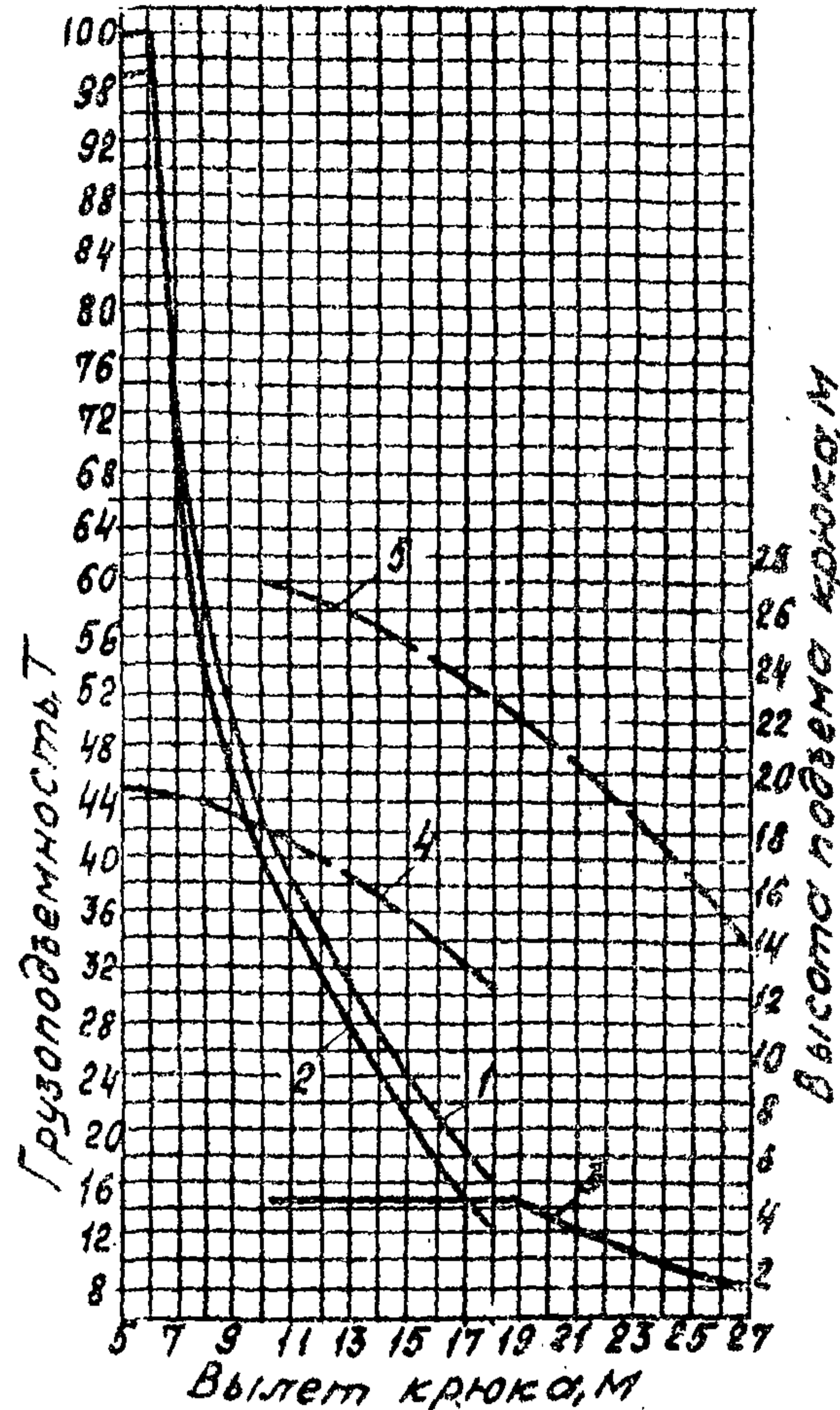
Стрела 20м с гуськом 10м
