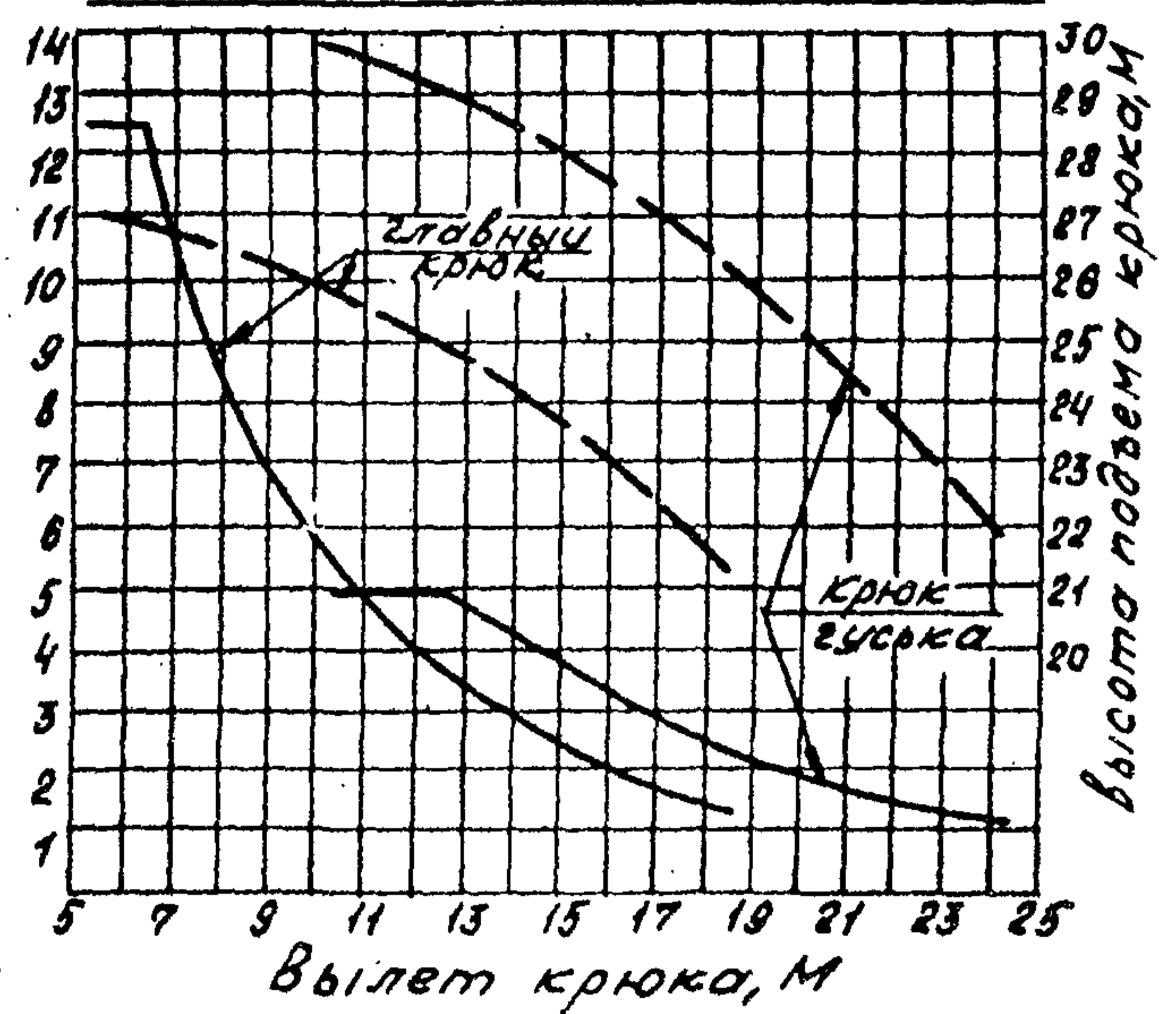
Стрела 27,5 м с гуськом 5 м
