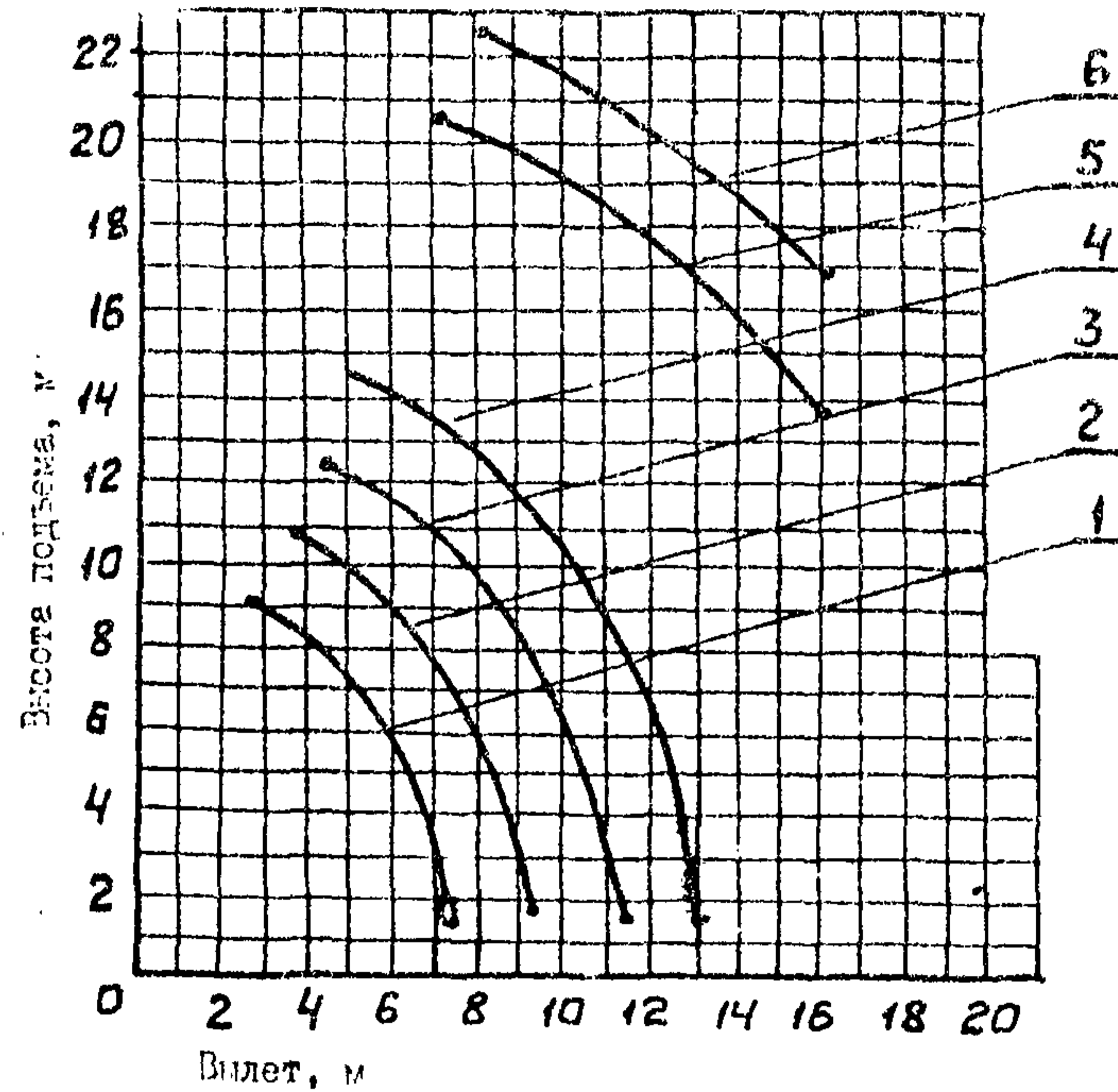
Пределы вылета подъема
