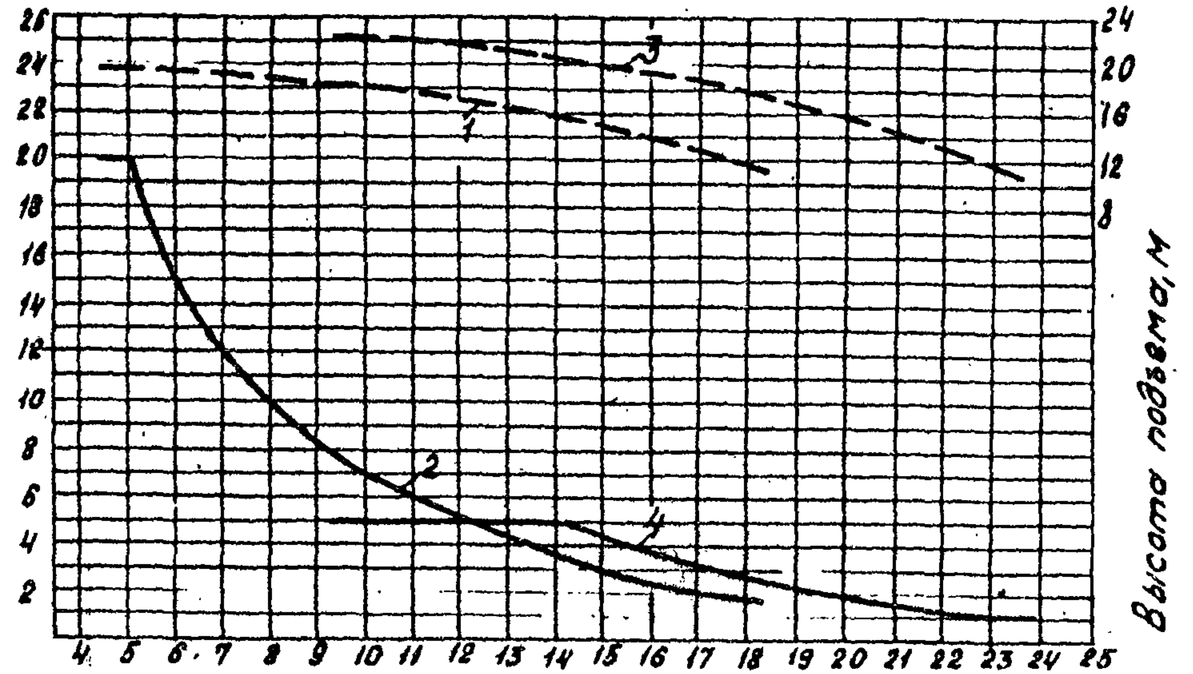
Стрела 25,3 м
