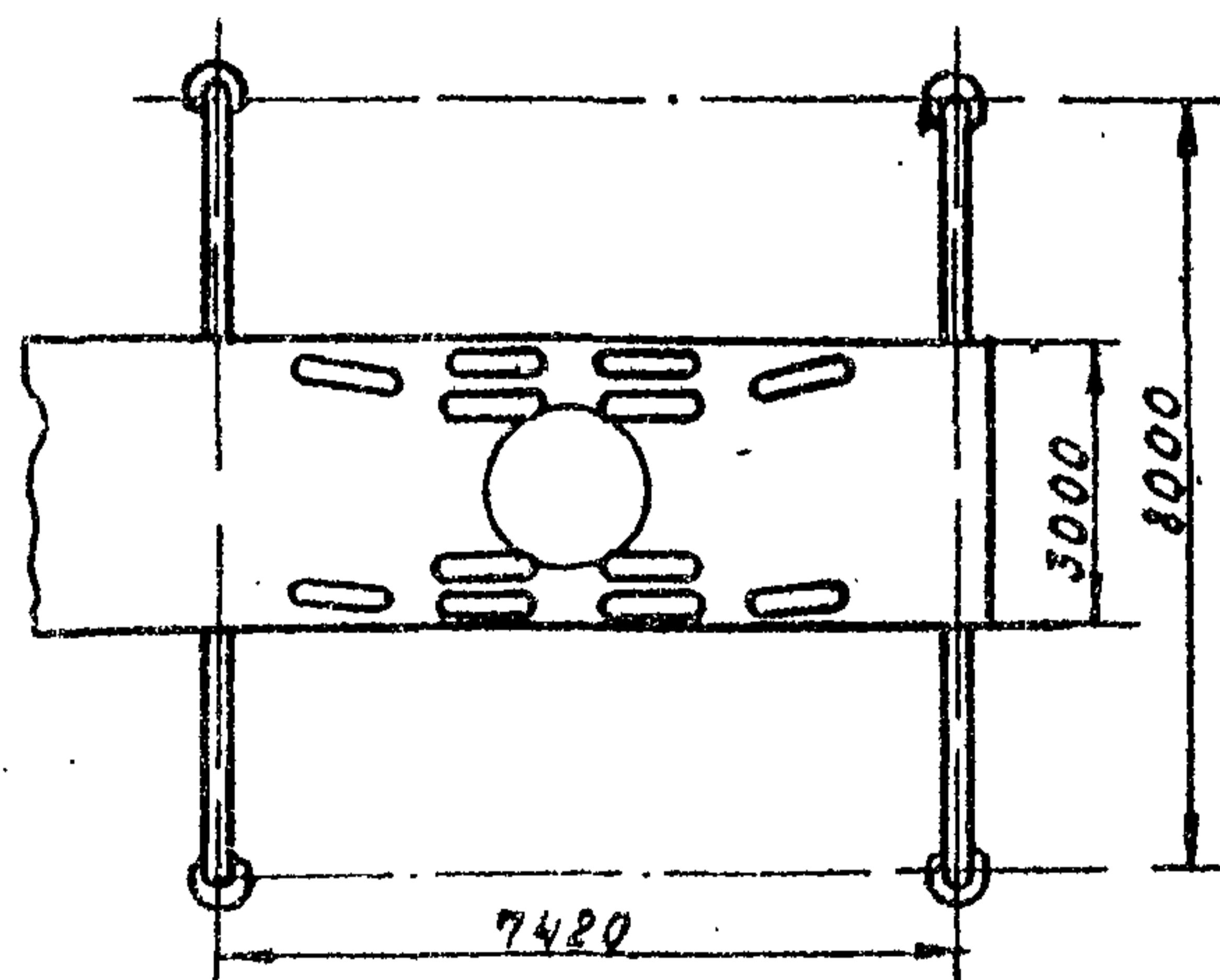
Размеры выносной опоры в плане
