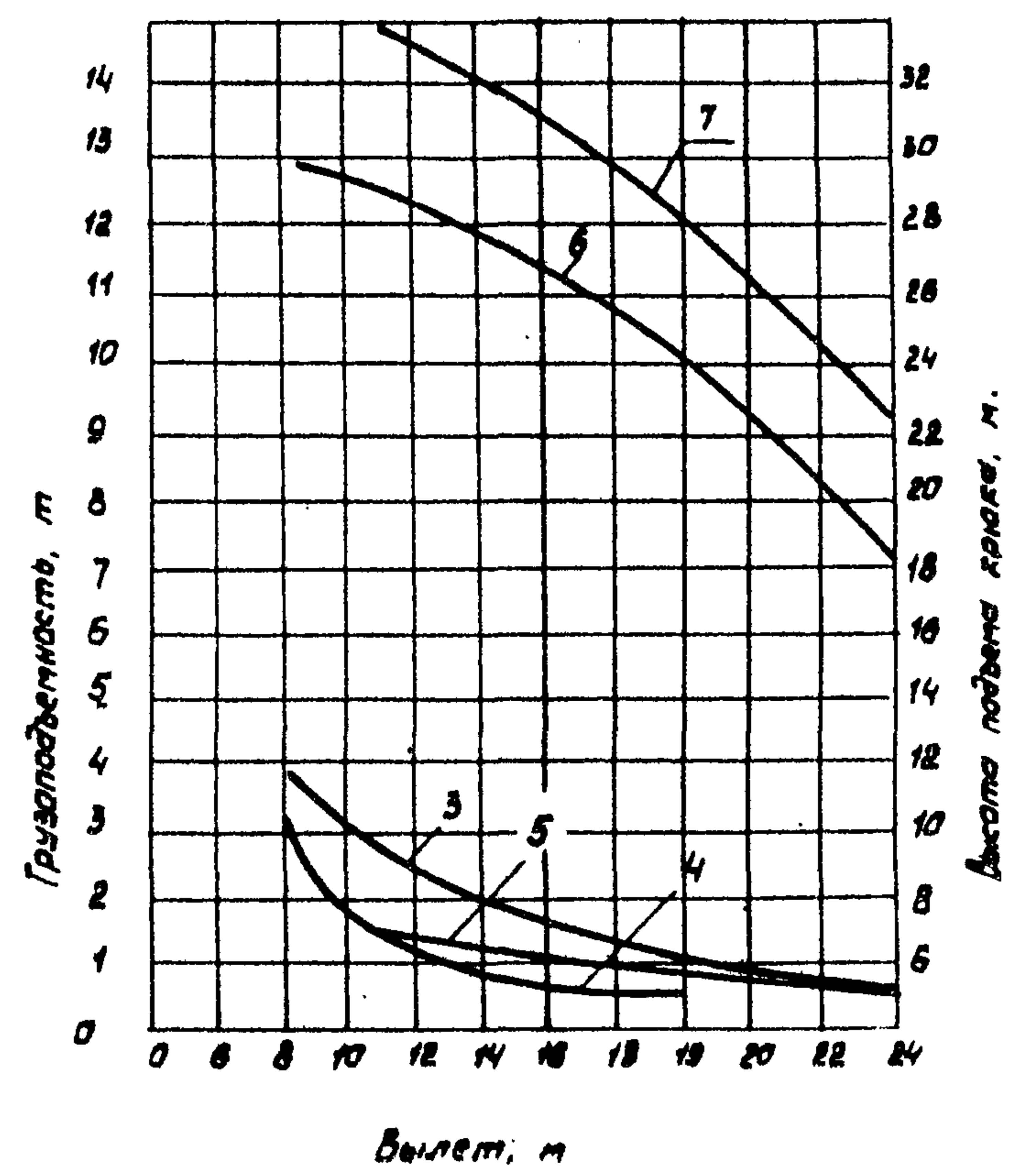
Стрела 30м с гуськом
