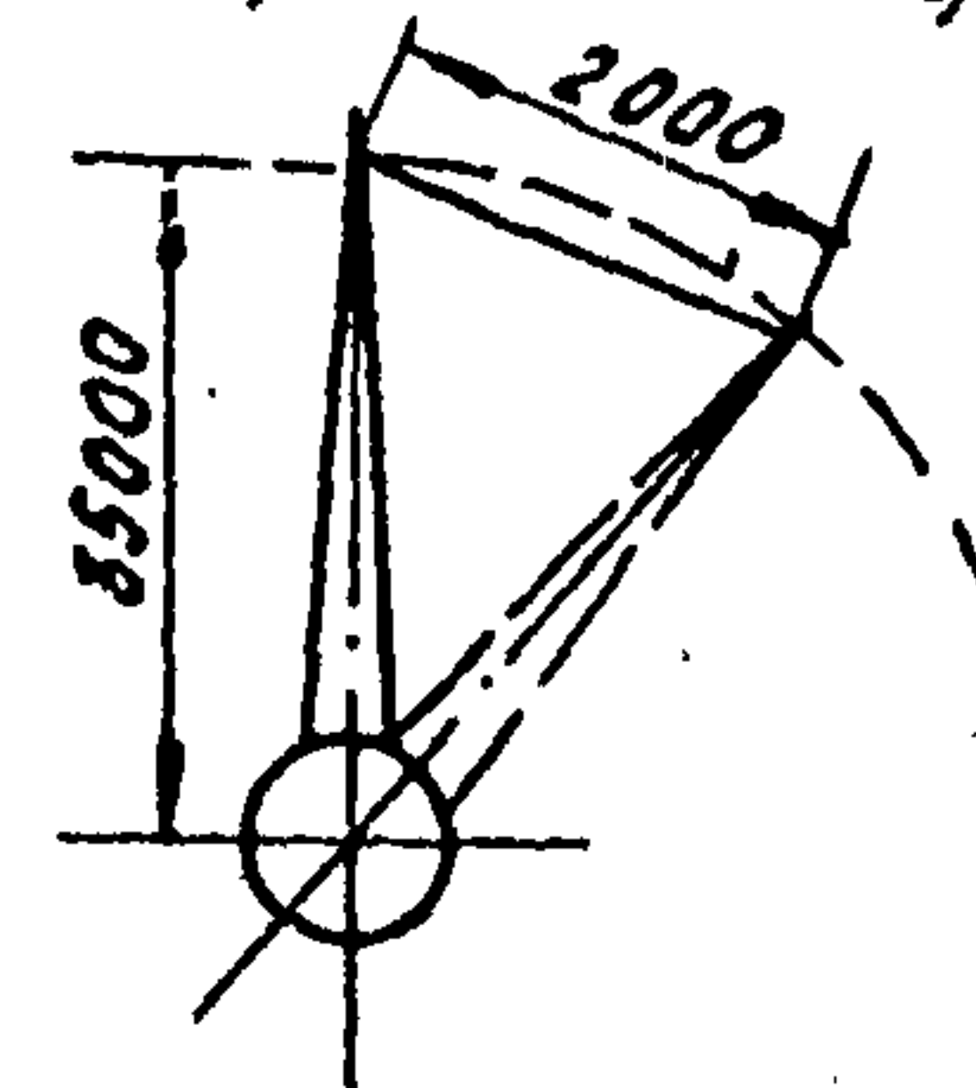
Тормозной путь стрелы с предельным грузом
