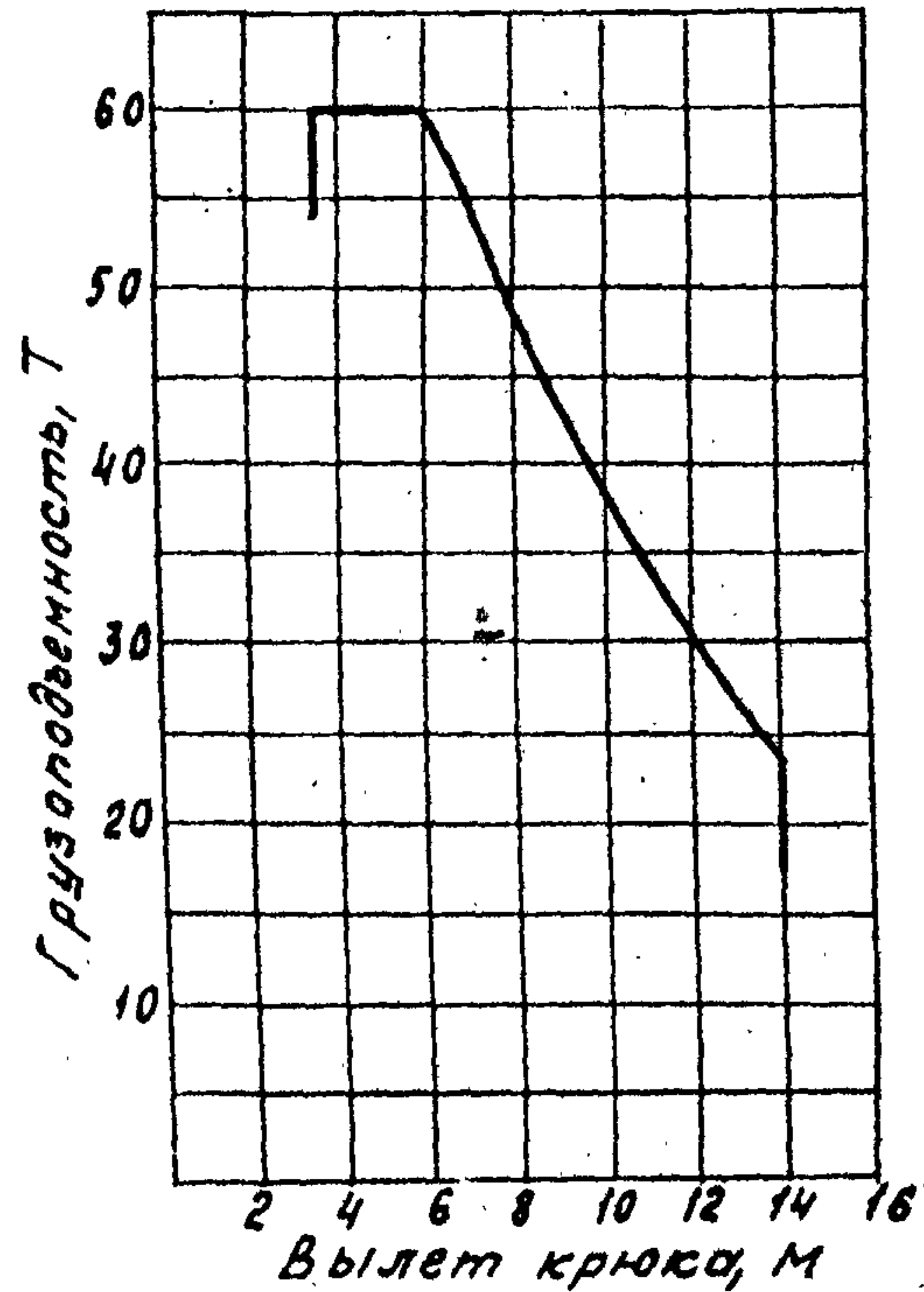
Стрела 54,8м
