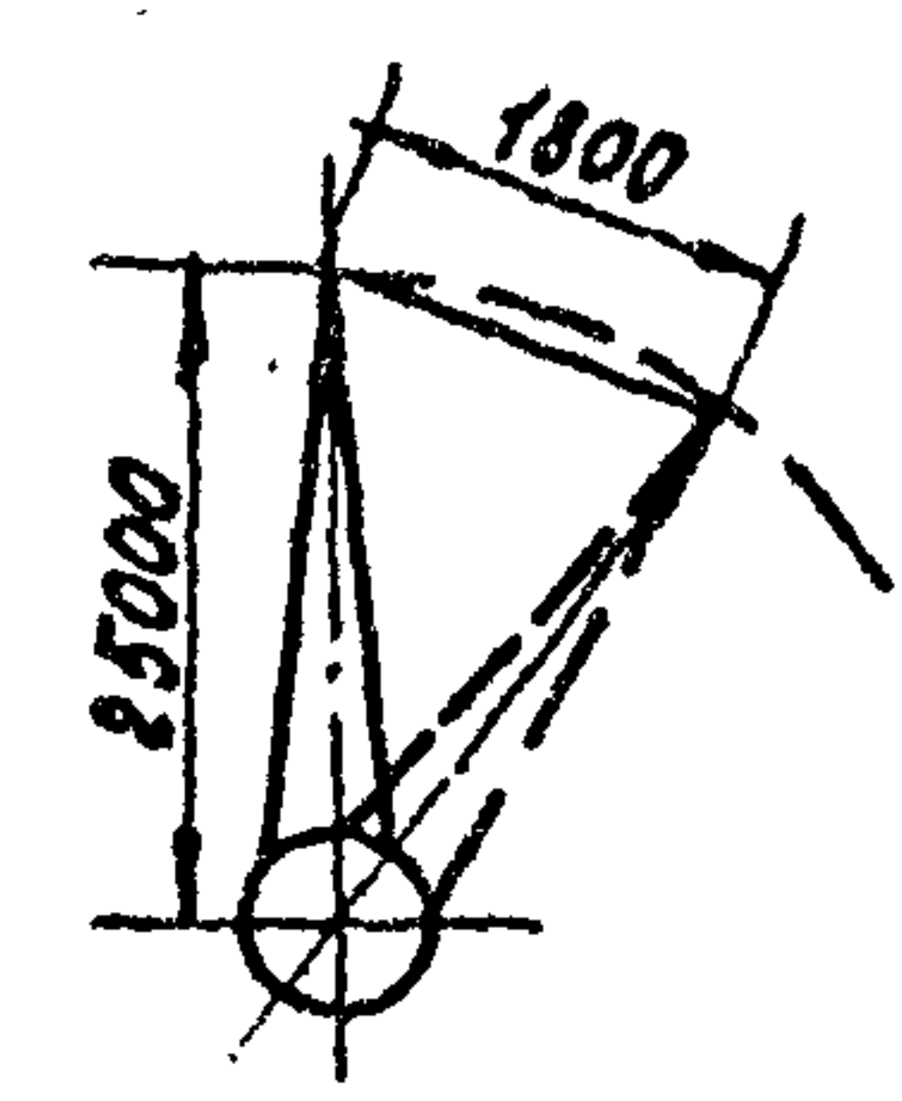
Тормозной путь стрелы с предельным грузом
