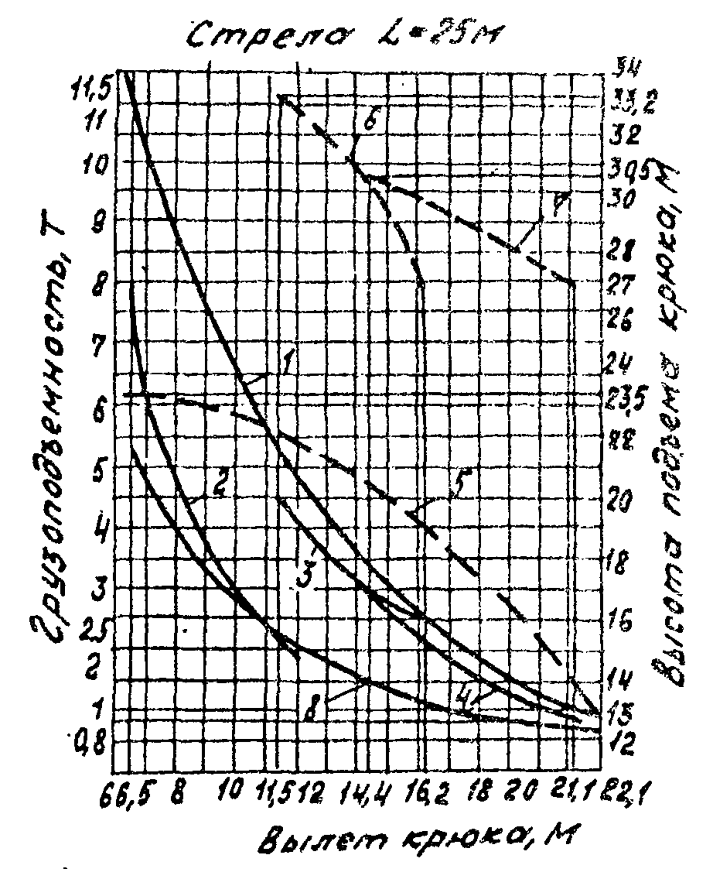
Графики высоты подъема крюка
