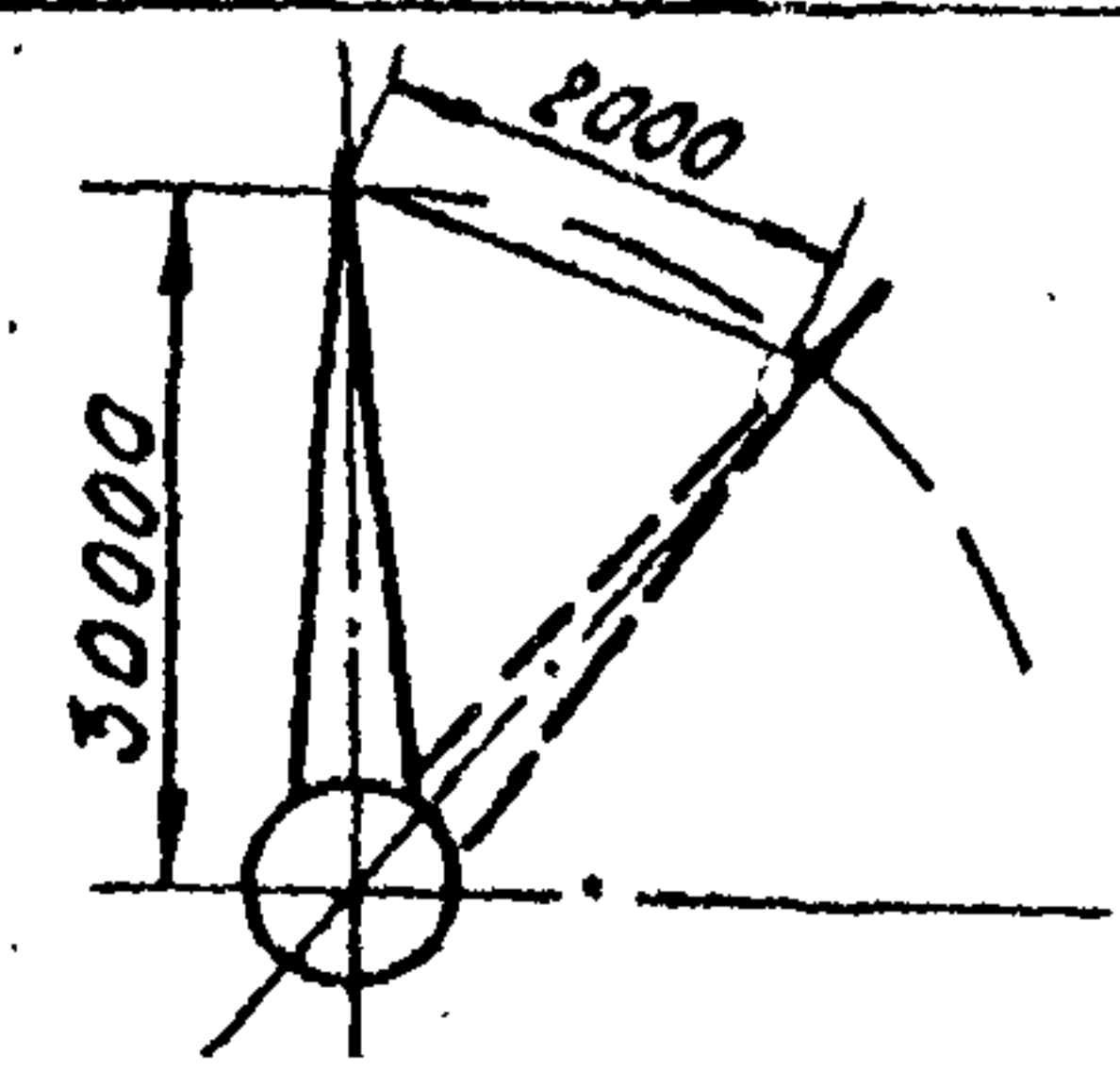
Тормозной путь стрелы с предельным врузом
