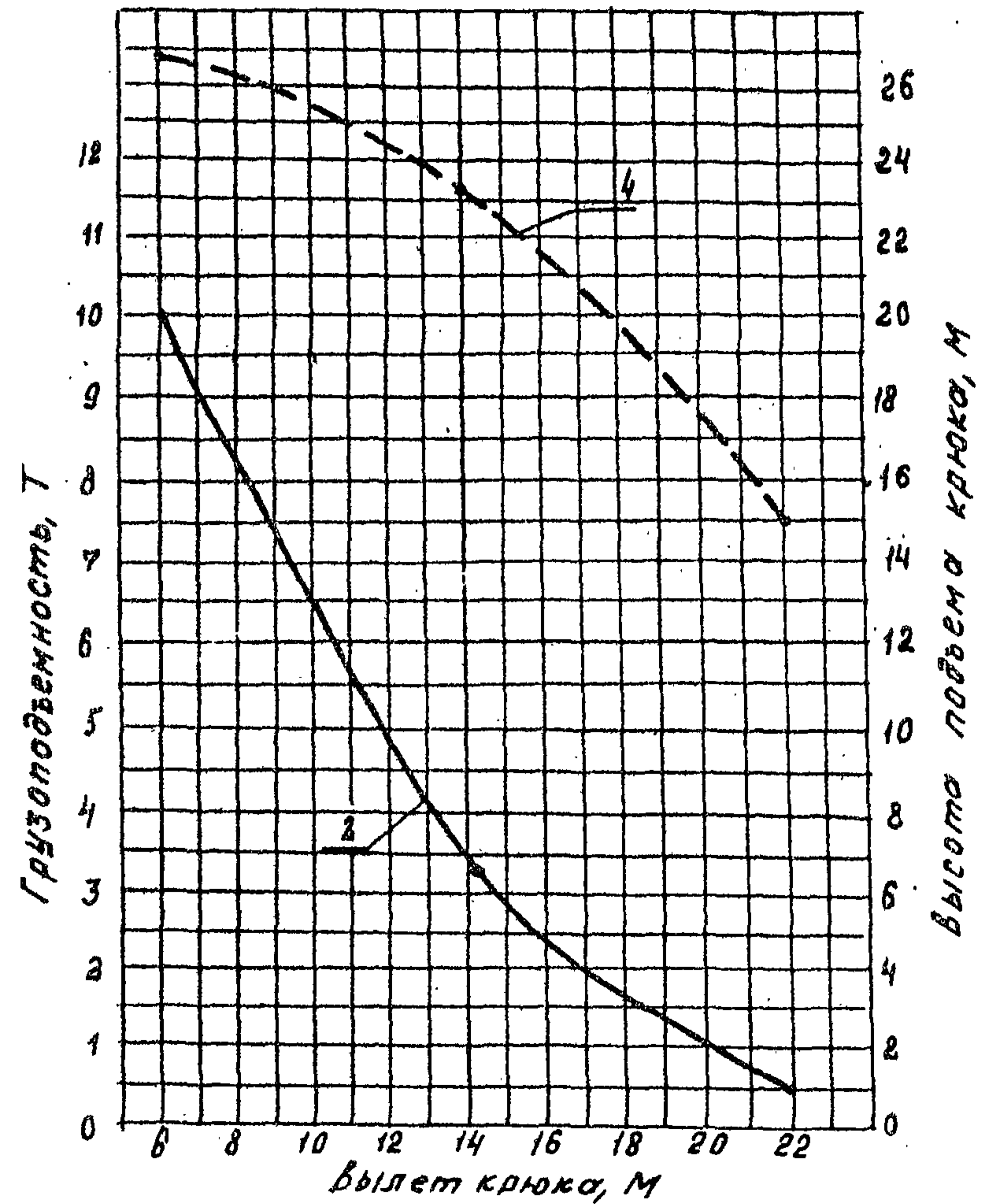
Стрела 27 м
