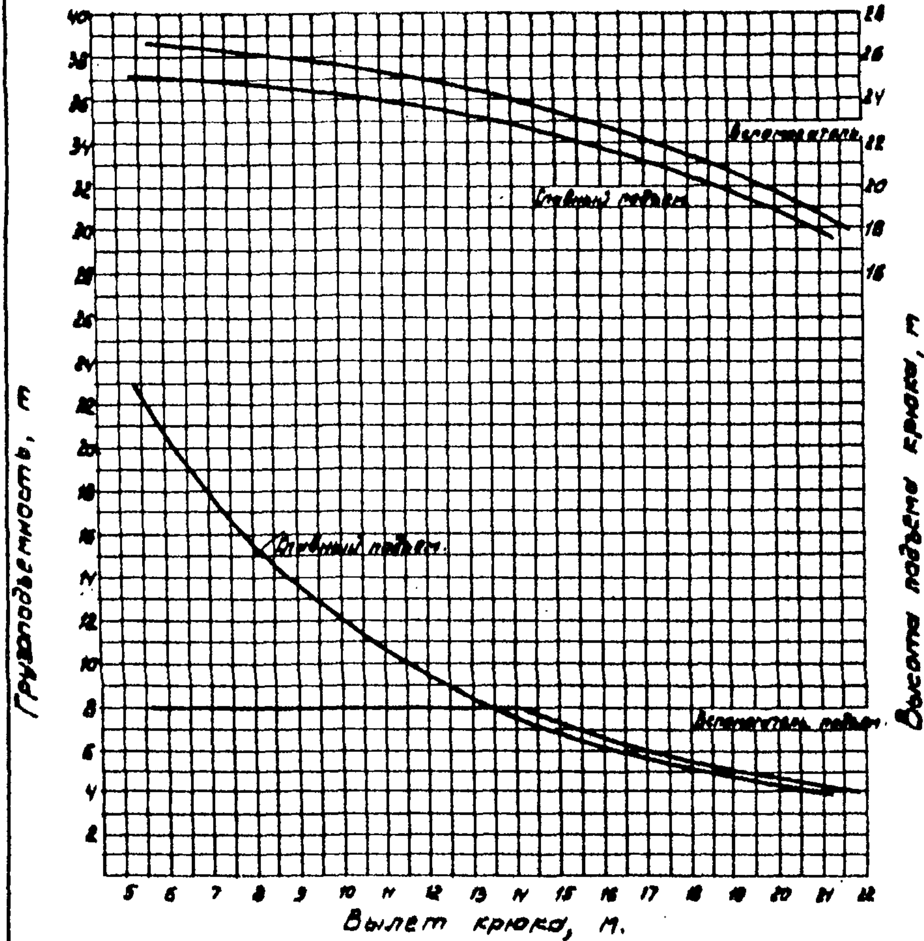
Стрела 26 м. без вышка
