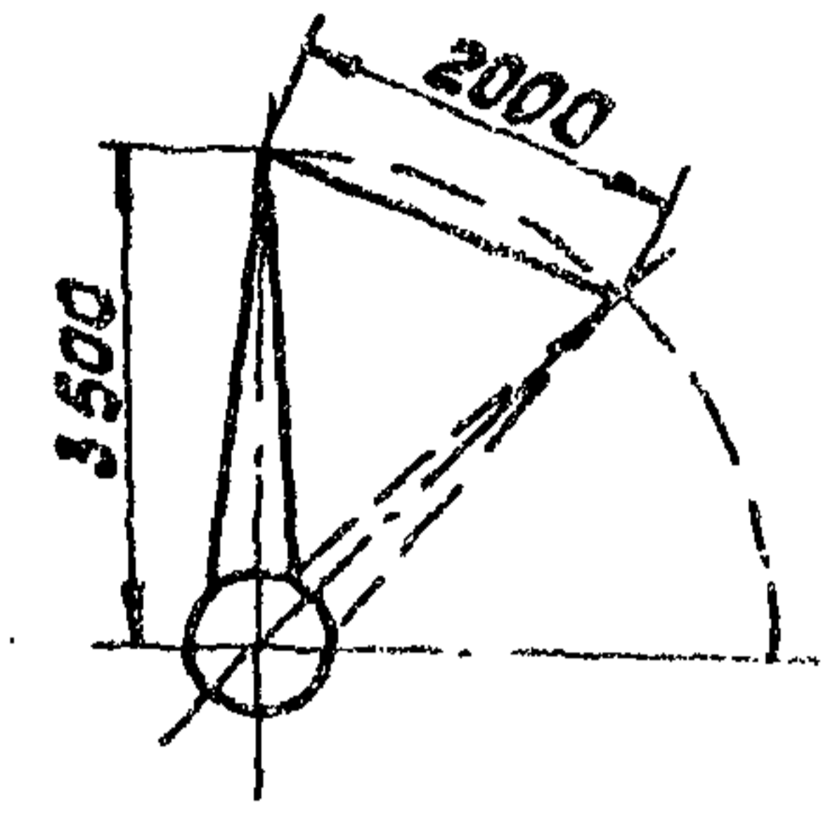
Тормозной путь стрелы с предельным грузом
