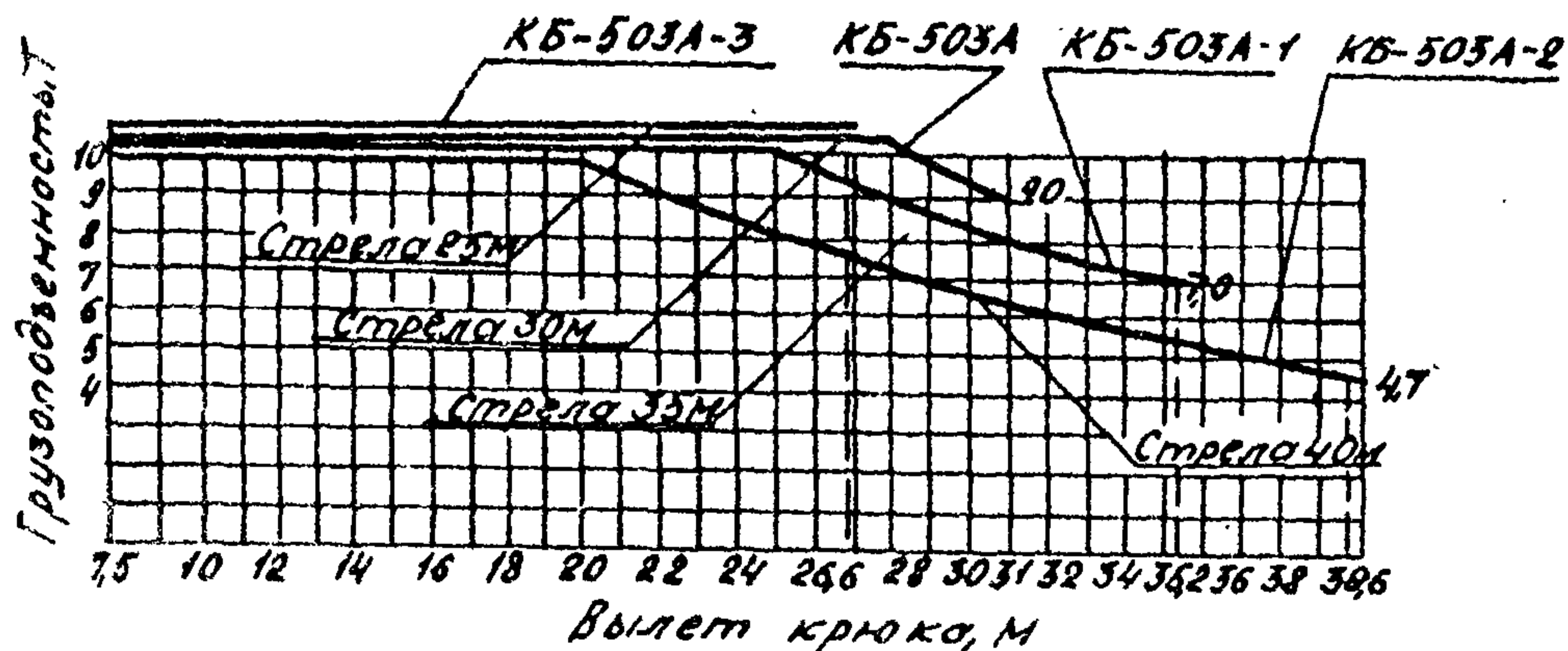
График грузоподъемности при наклонной стреле (30°)
