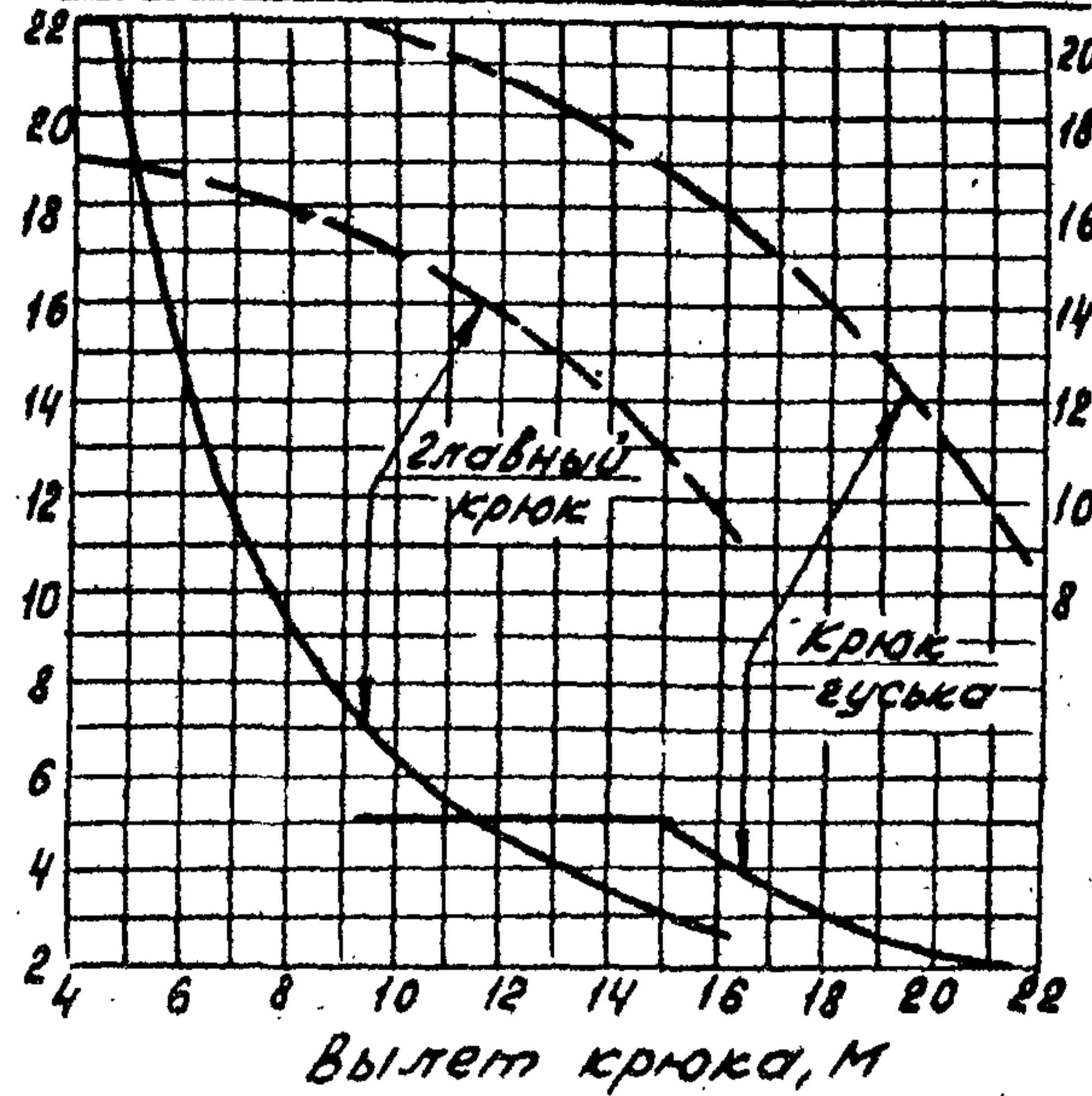
Стрела 17,5 м с гуськом 5 м
