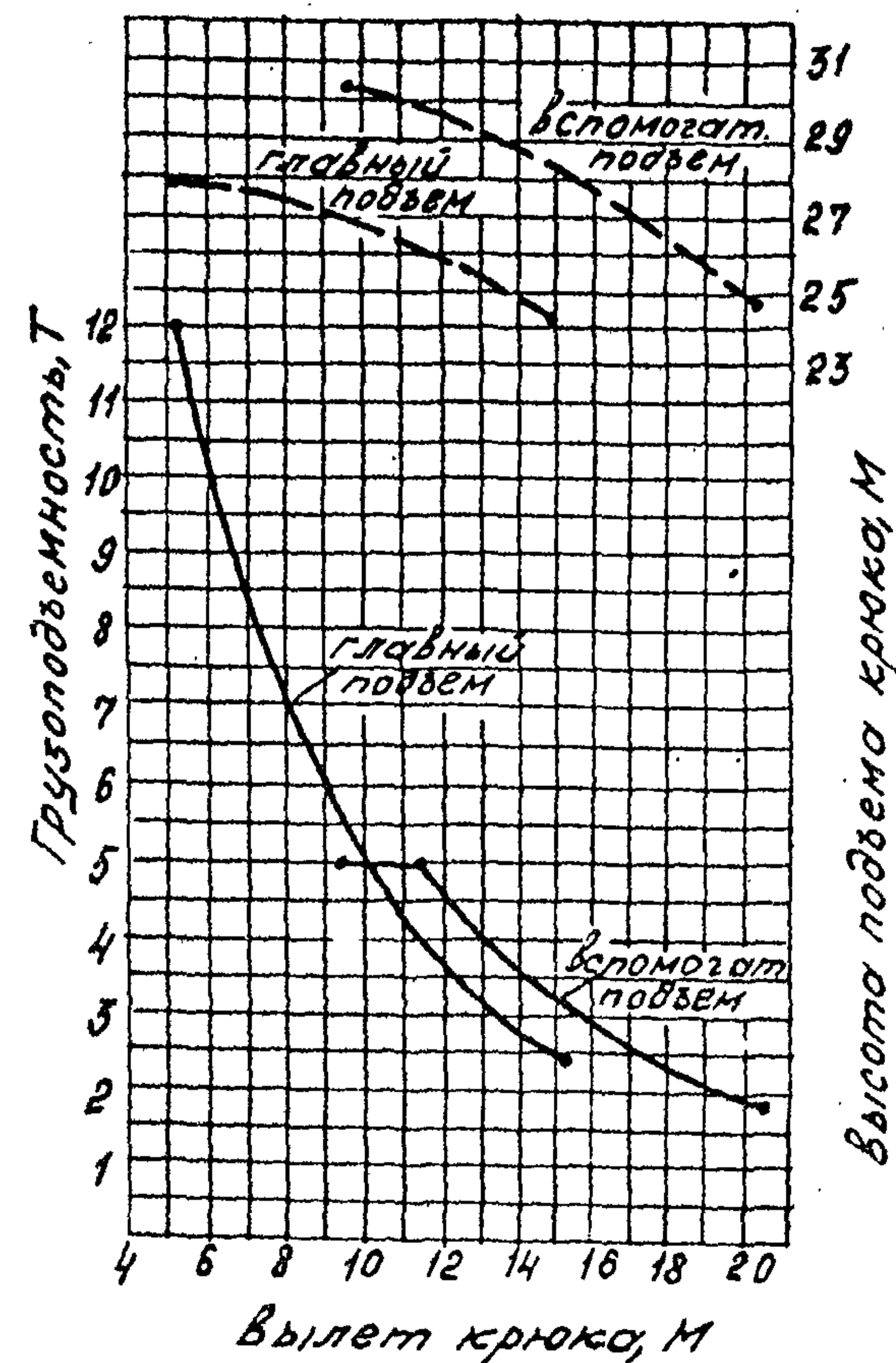
Стрела 28,5 м с жестким гуськом 5 м
