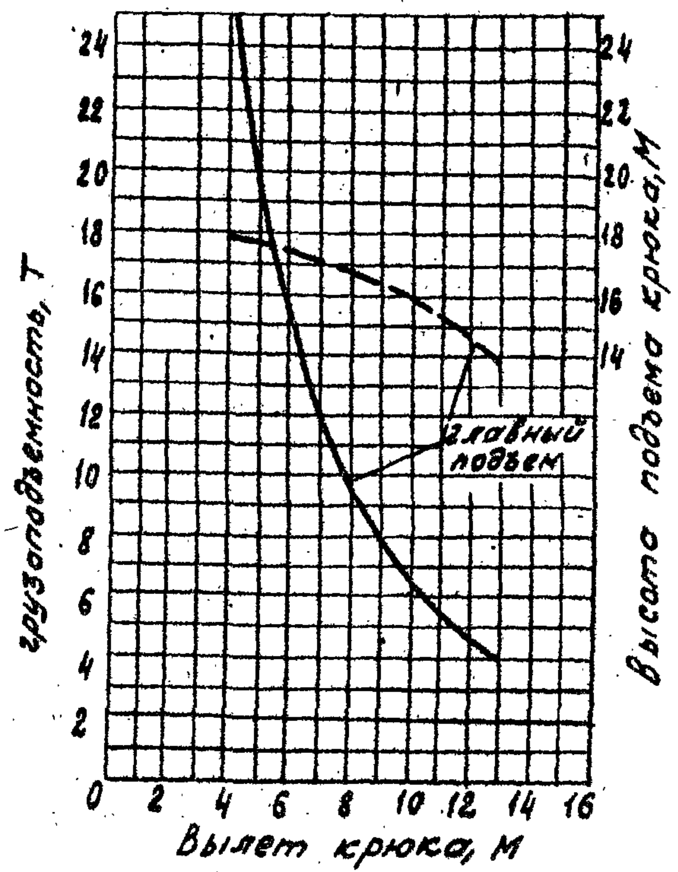
Стрела 18,5 м
