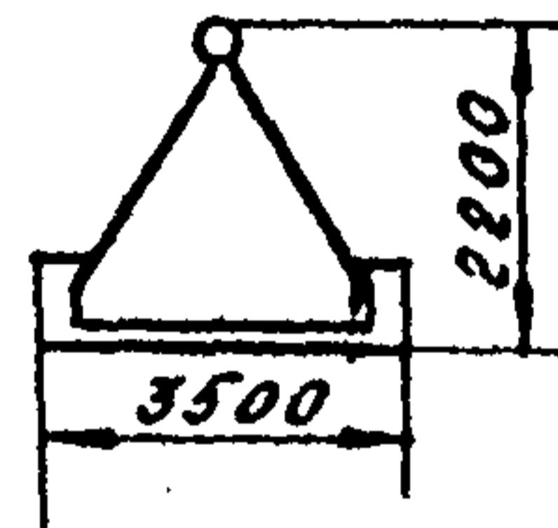
Наружный габарит стрелы с грузовой тележкой
