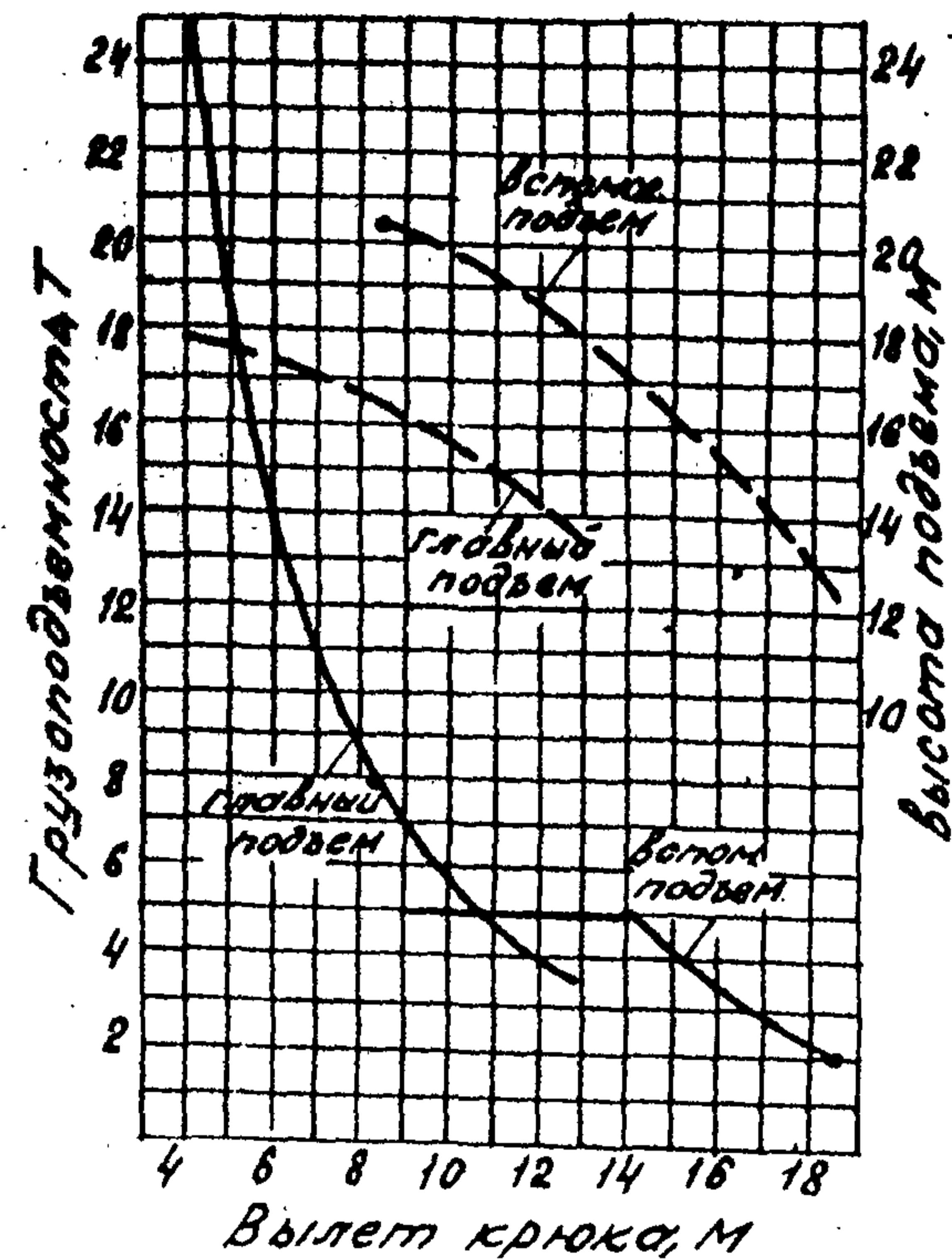
Стрела 18,5 м с жестким гуськом 5 м
