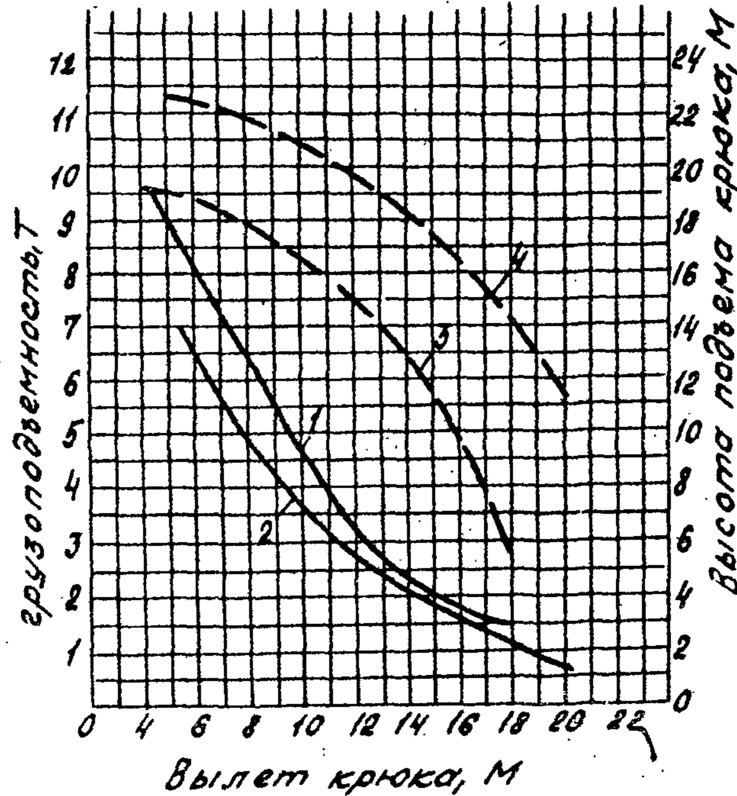
Стрела 20м и 24м
