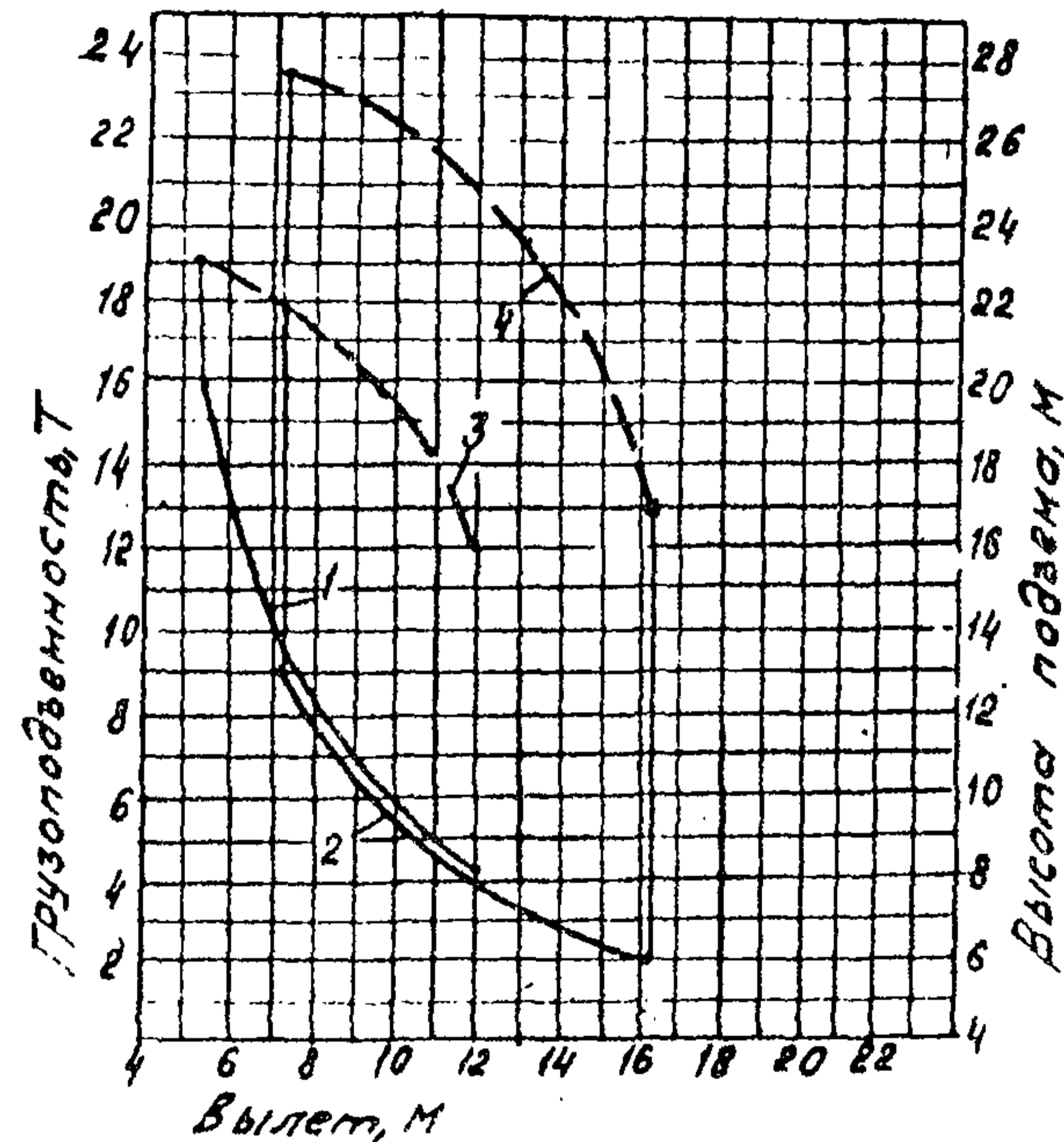
Башня 15 м гуськи 10 м и 15 м
