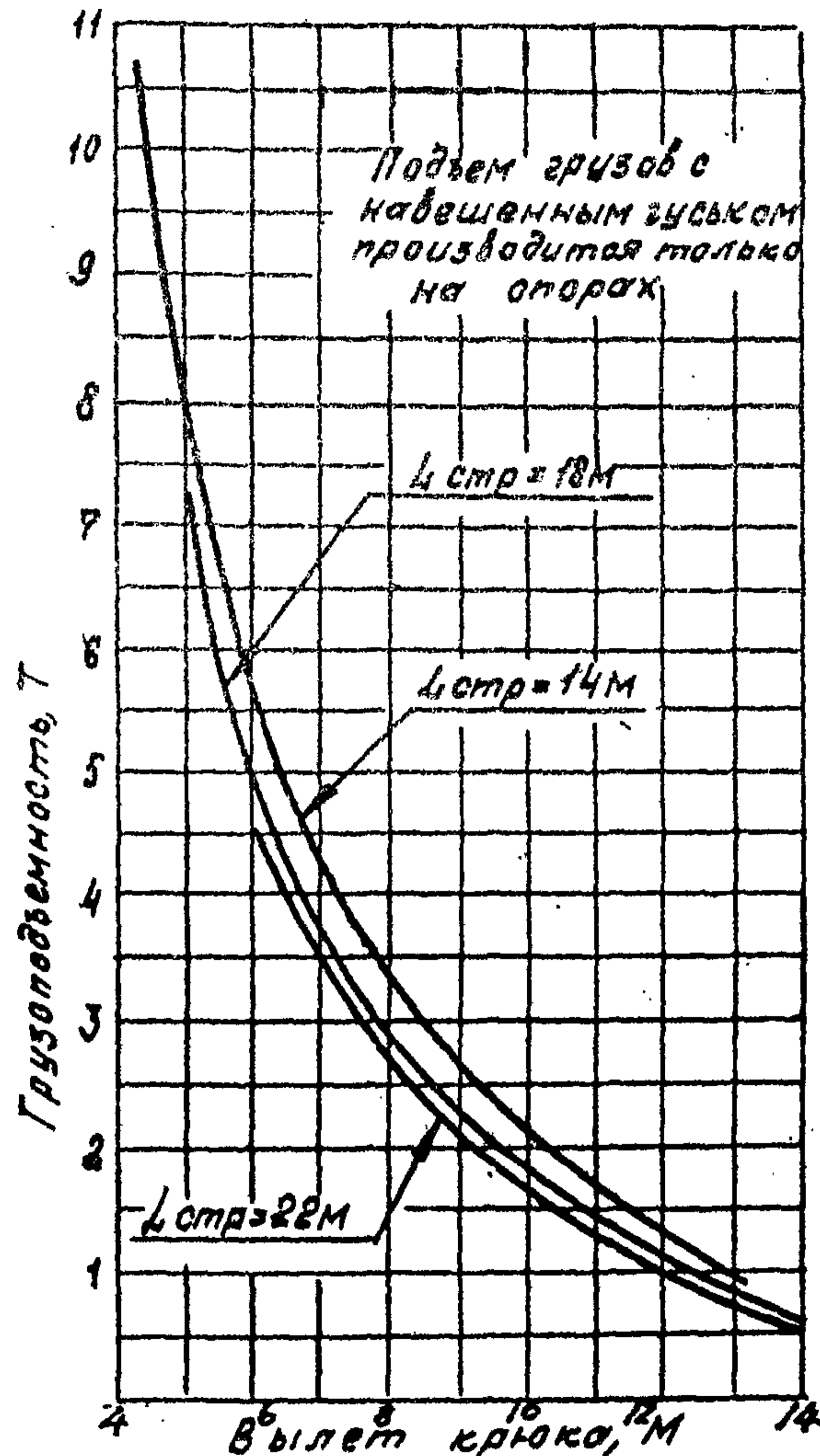
Графики грузоподъемности с навешенным гуськом (основной подъем)
