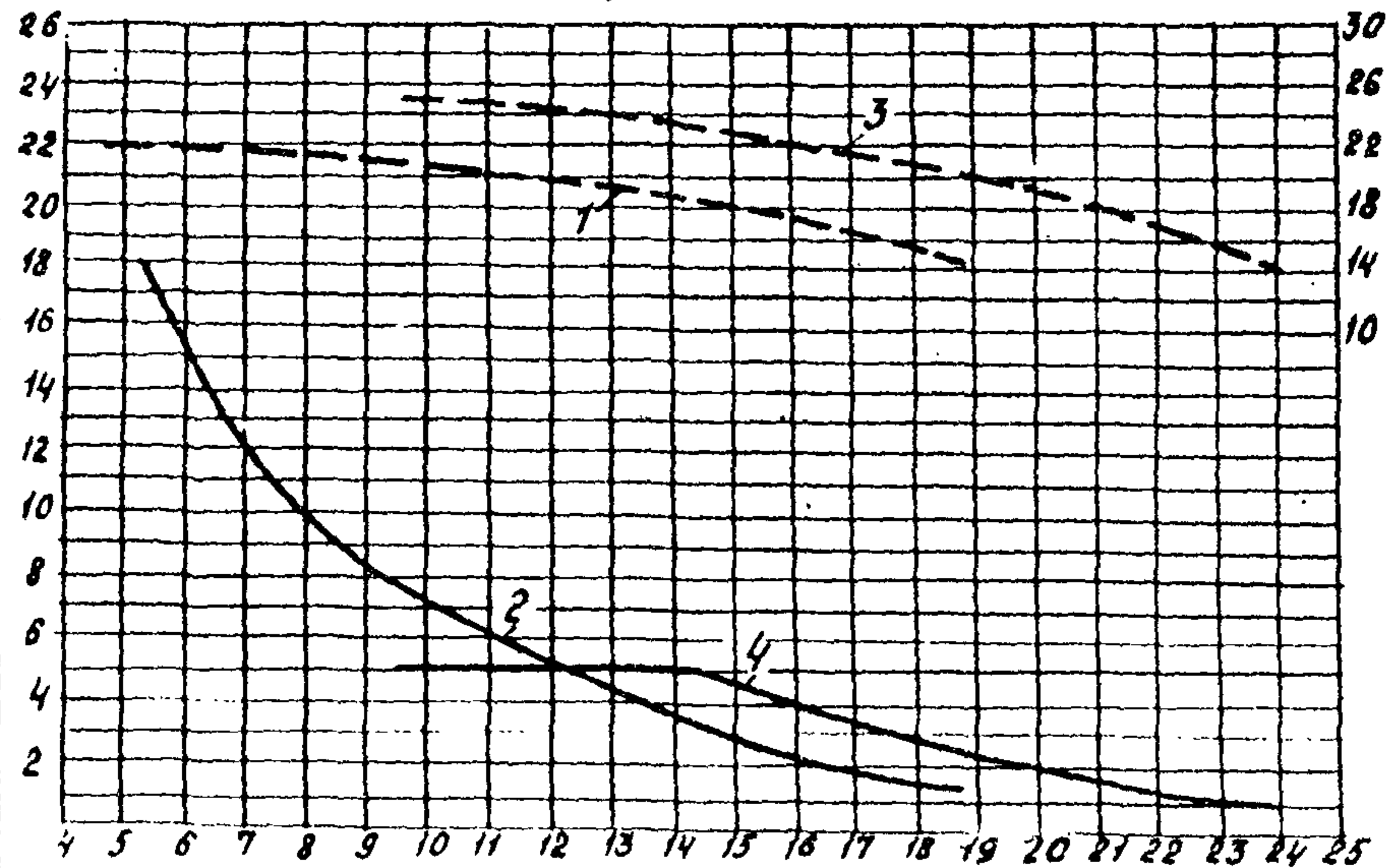
Стрела 22,5 м
