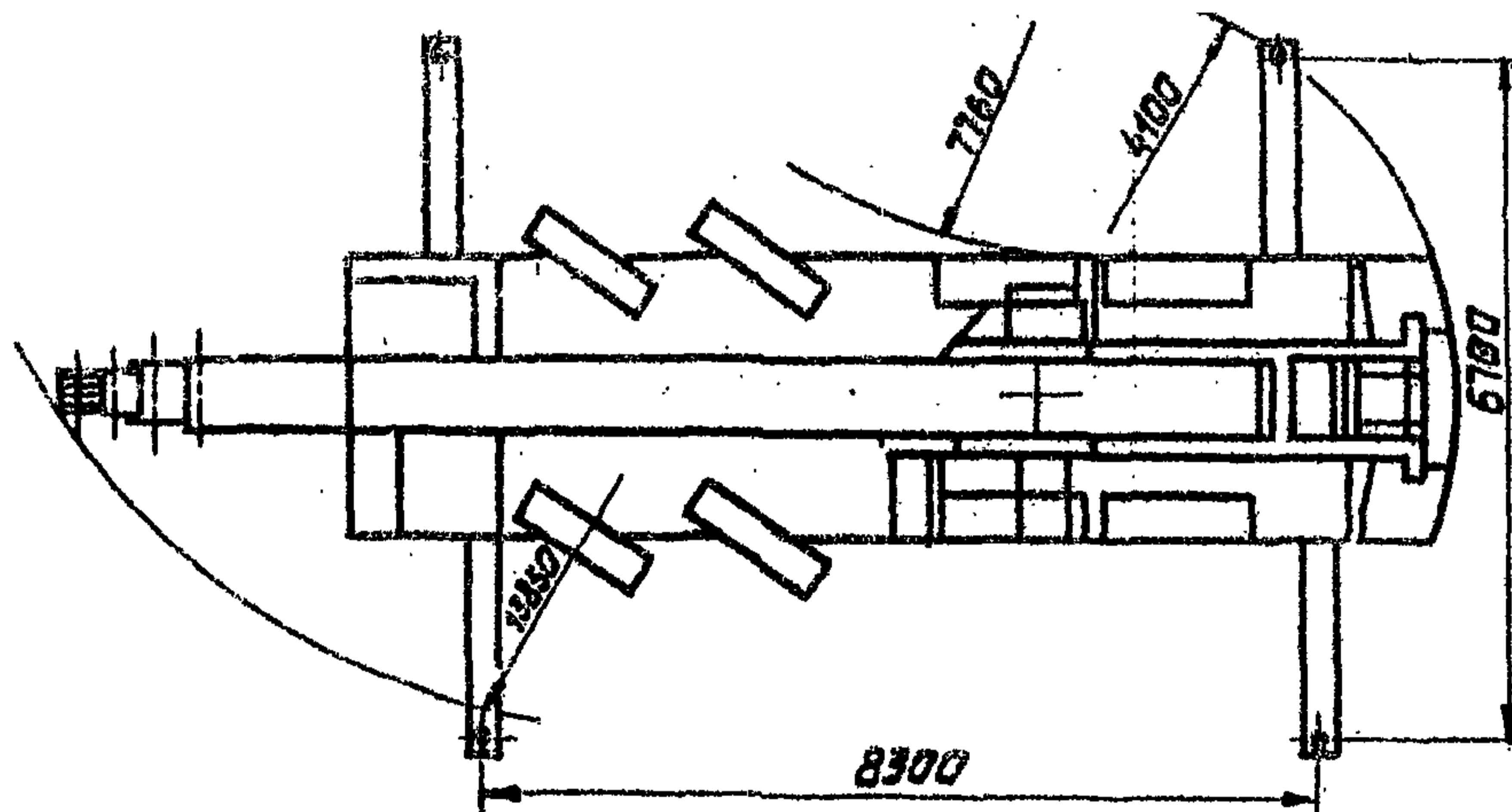
Размер выносных опор в плане
