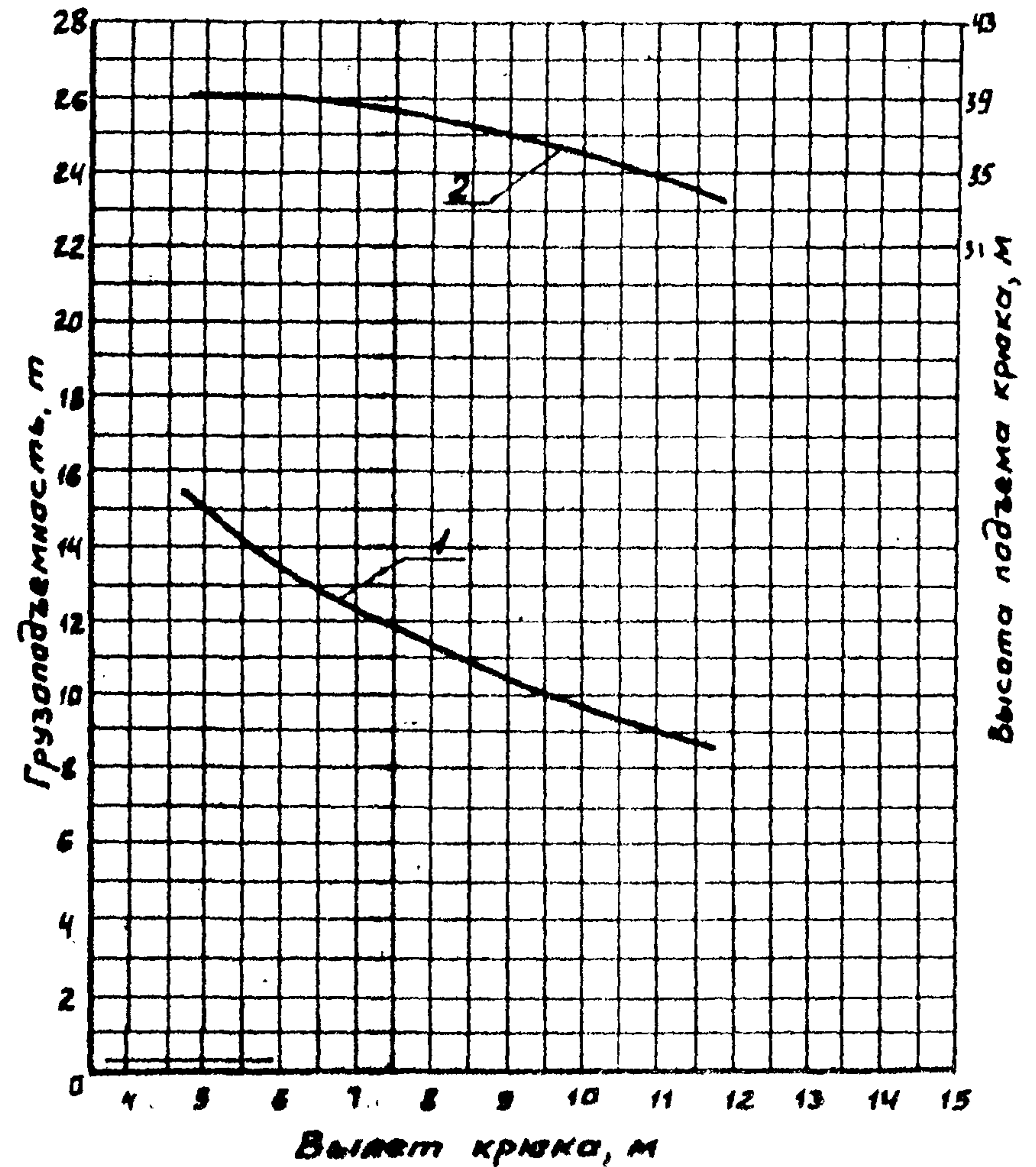
Башня 31 м
