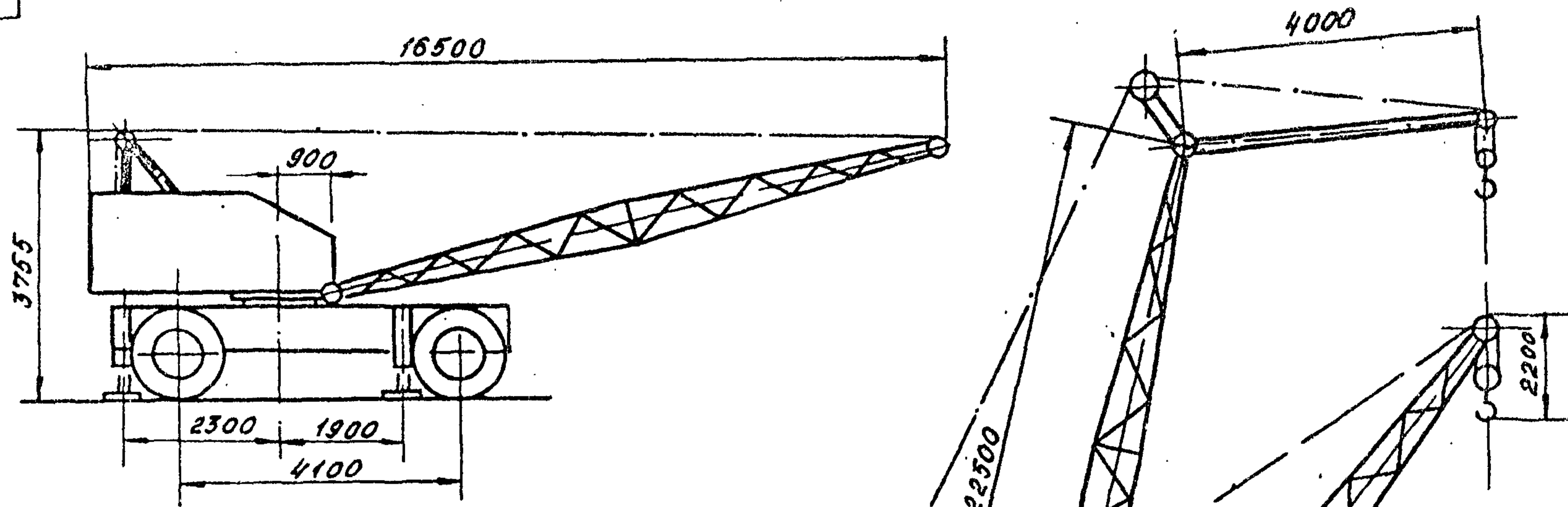
Грузовая характеристика крана
