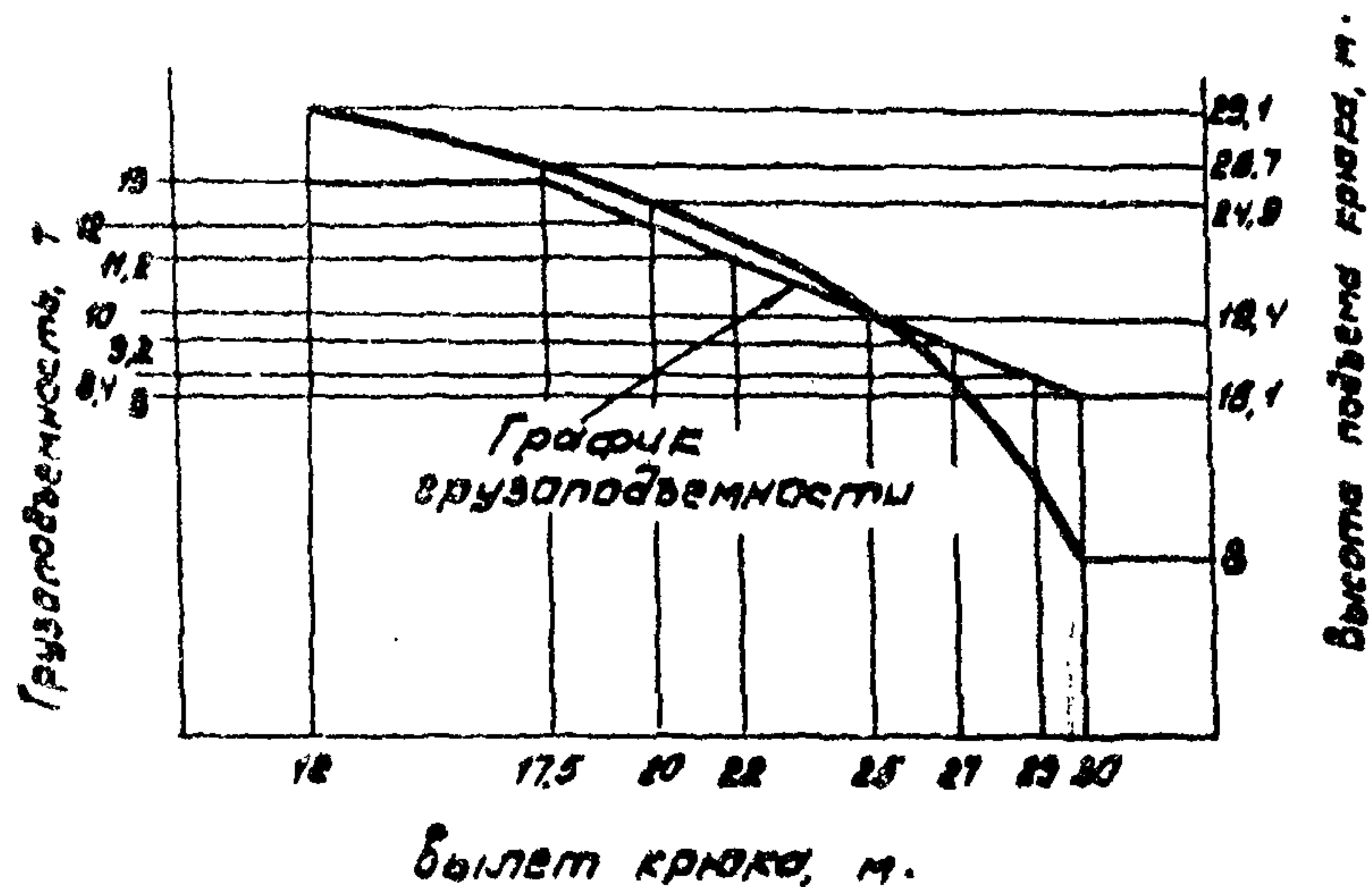
стрела 28,9 м с опорной вставкой (исполнение II)
