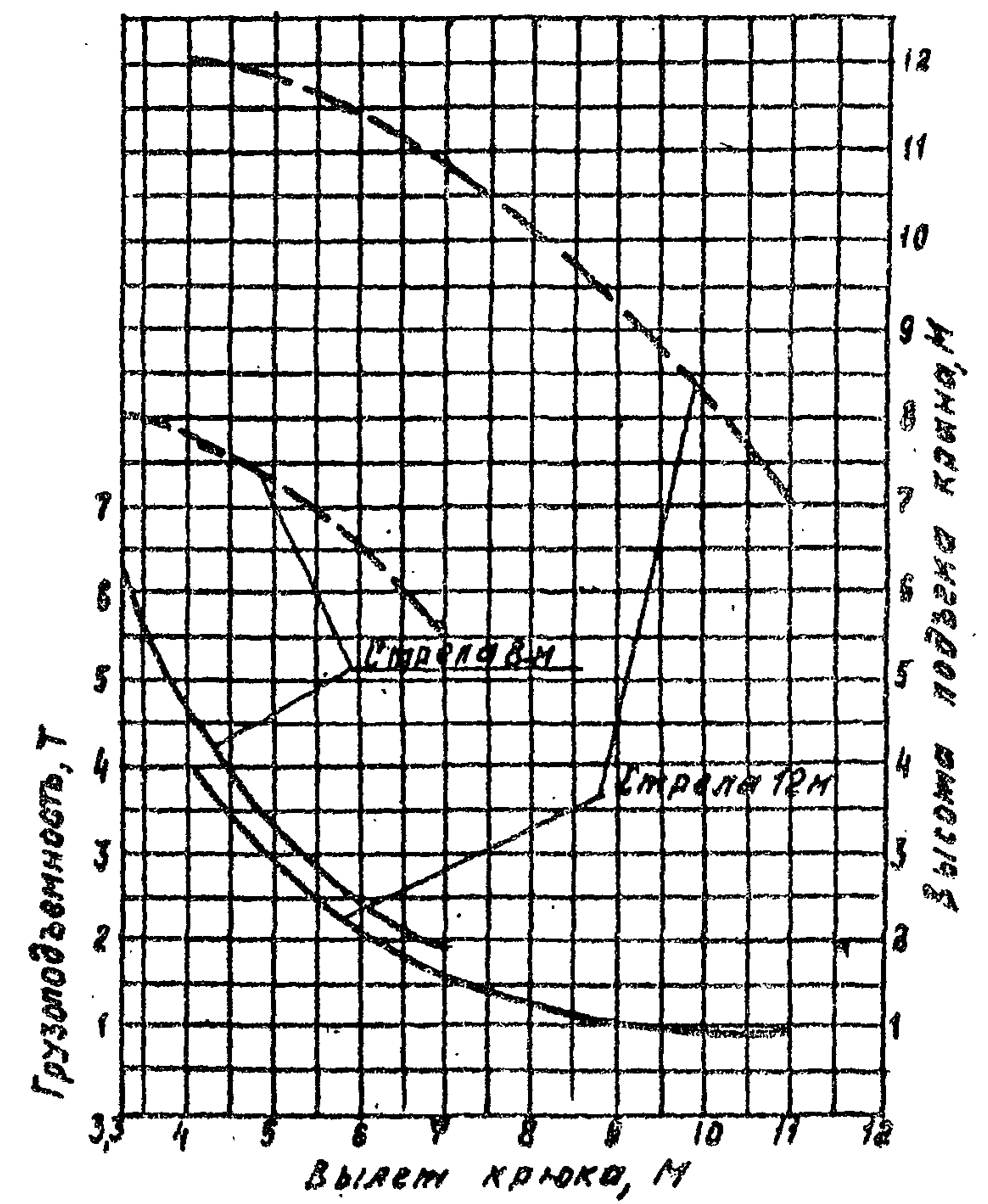
Грузовая характеристика крана
