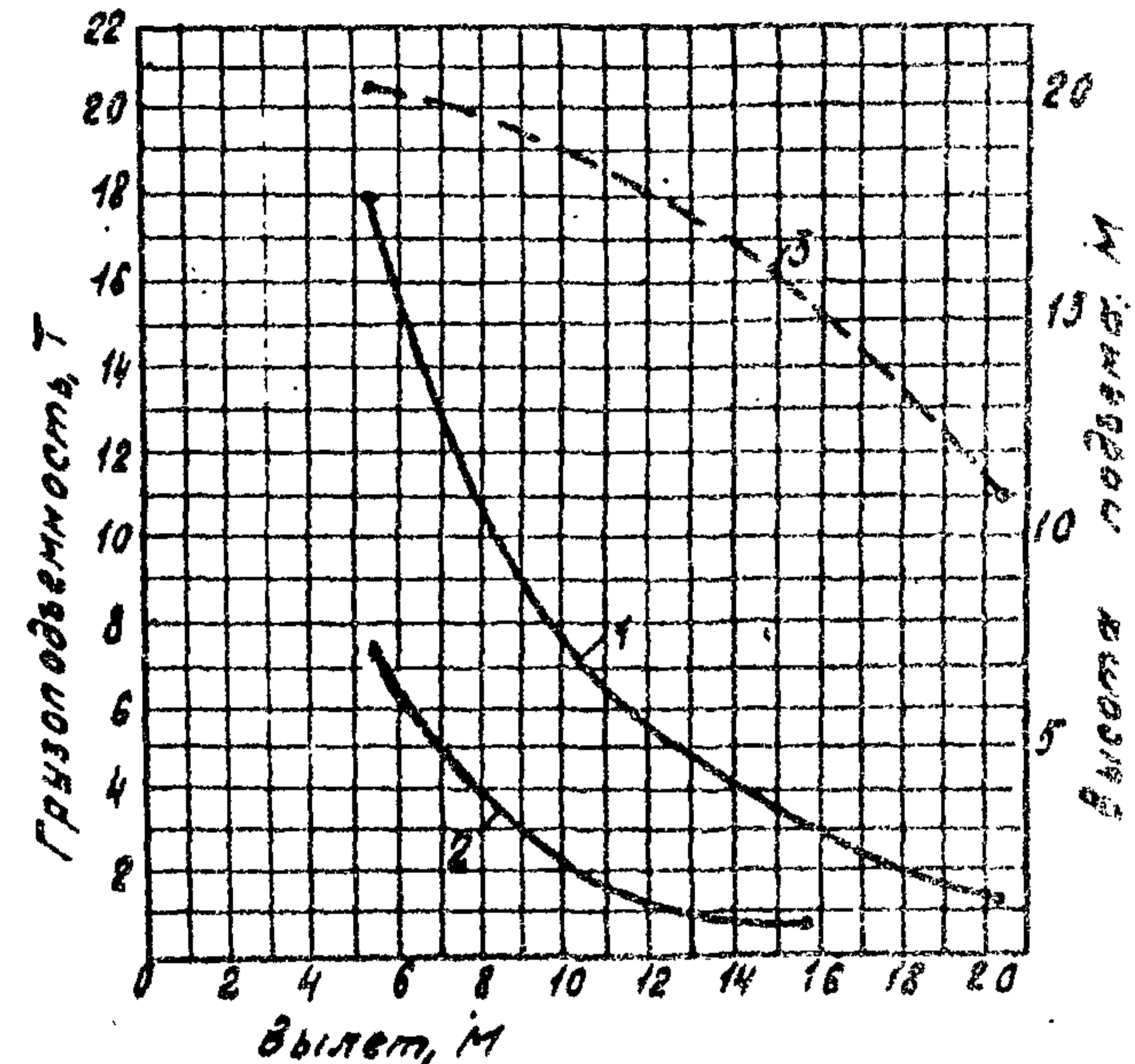
Стрела 22,5 м
