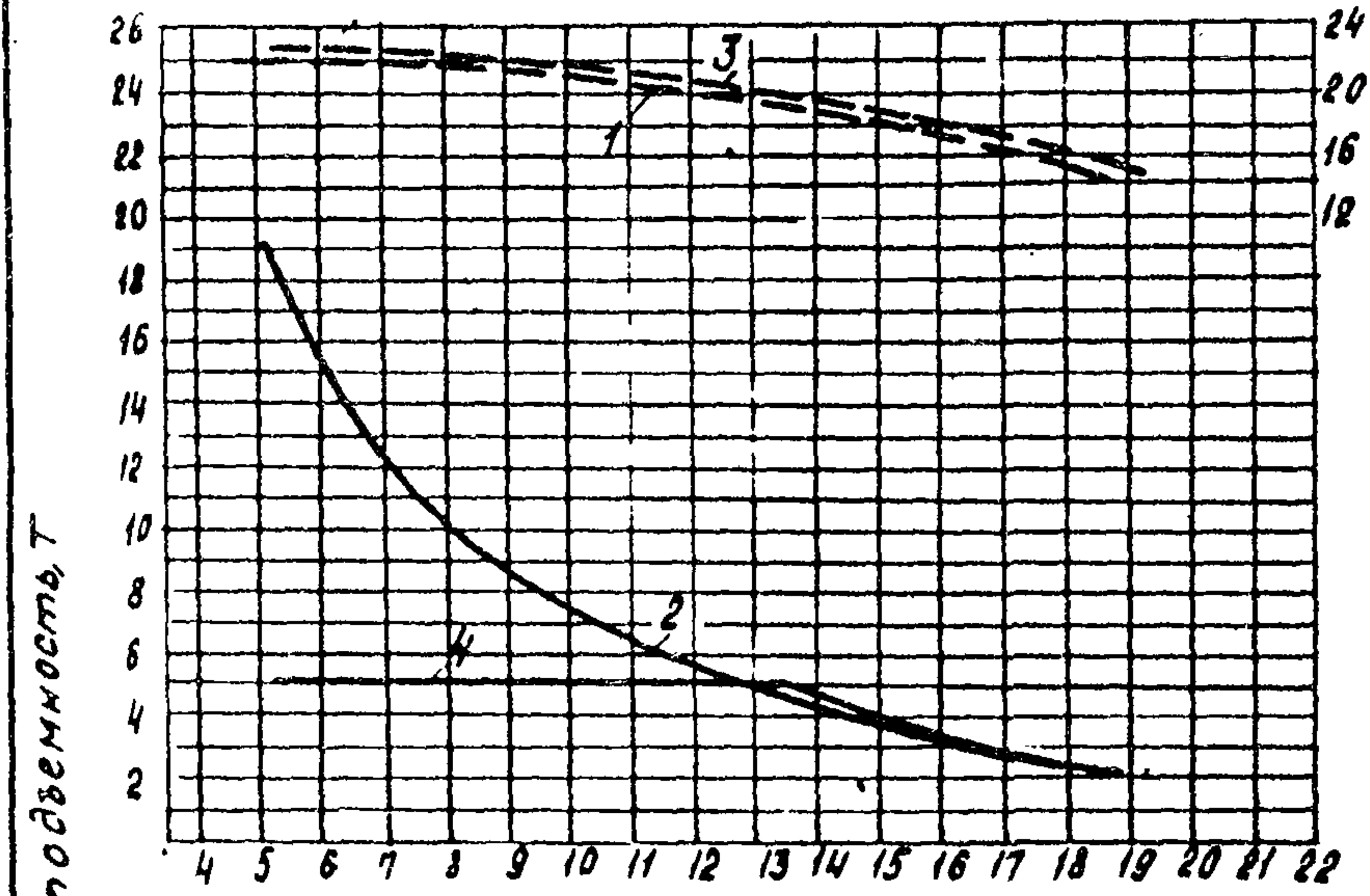
Стрела 27,5м
