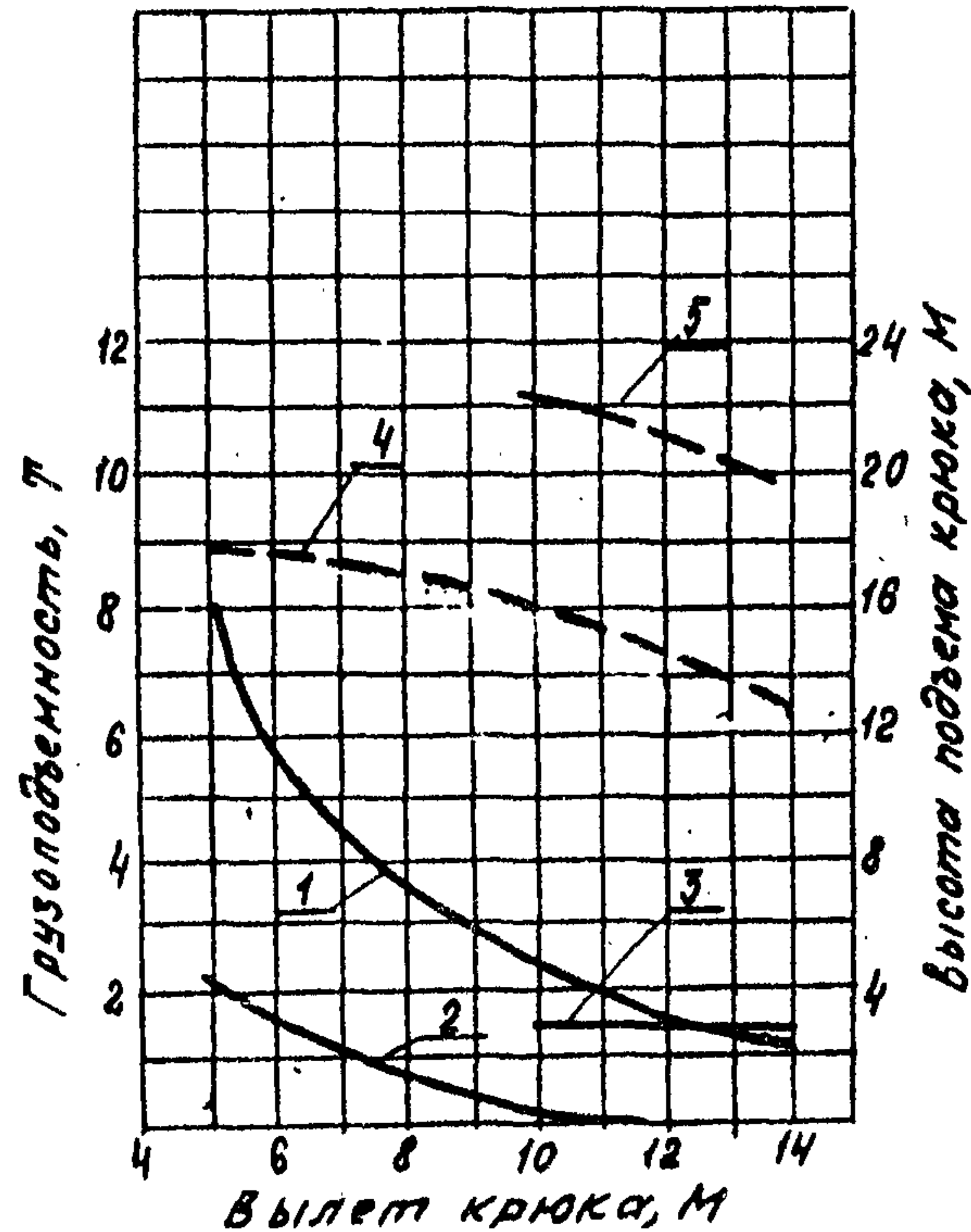
Стрела 18 м
