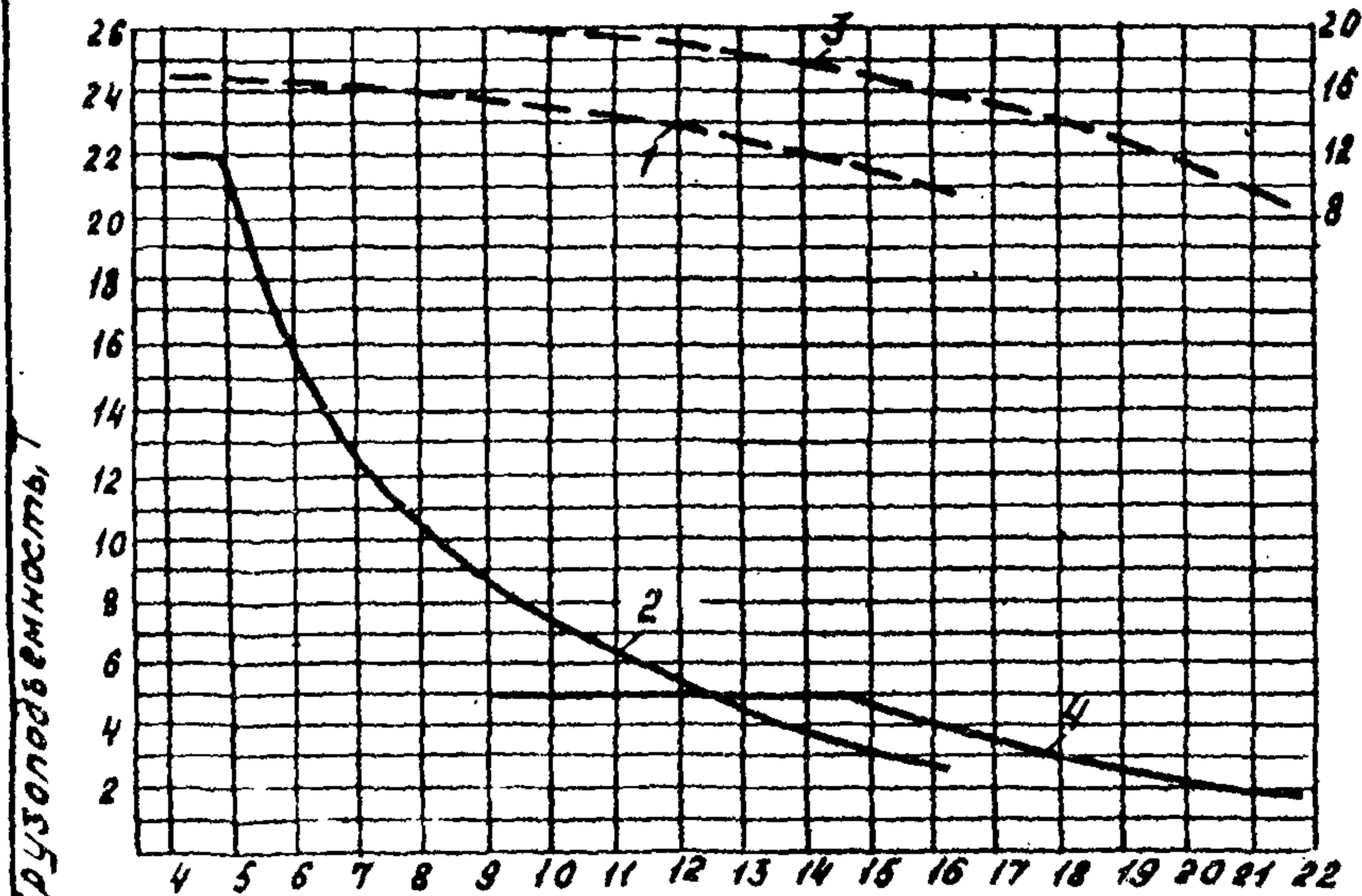
Стрела 22,5 м
