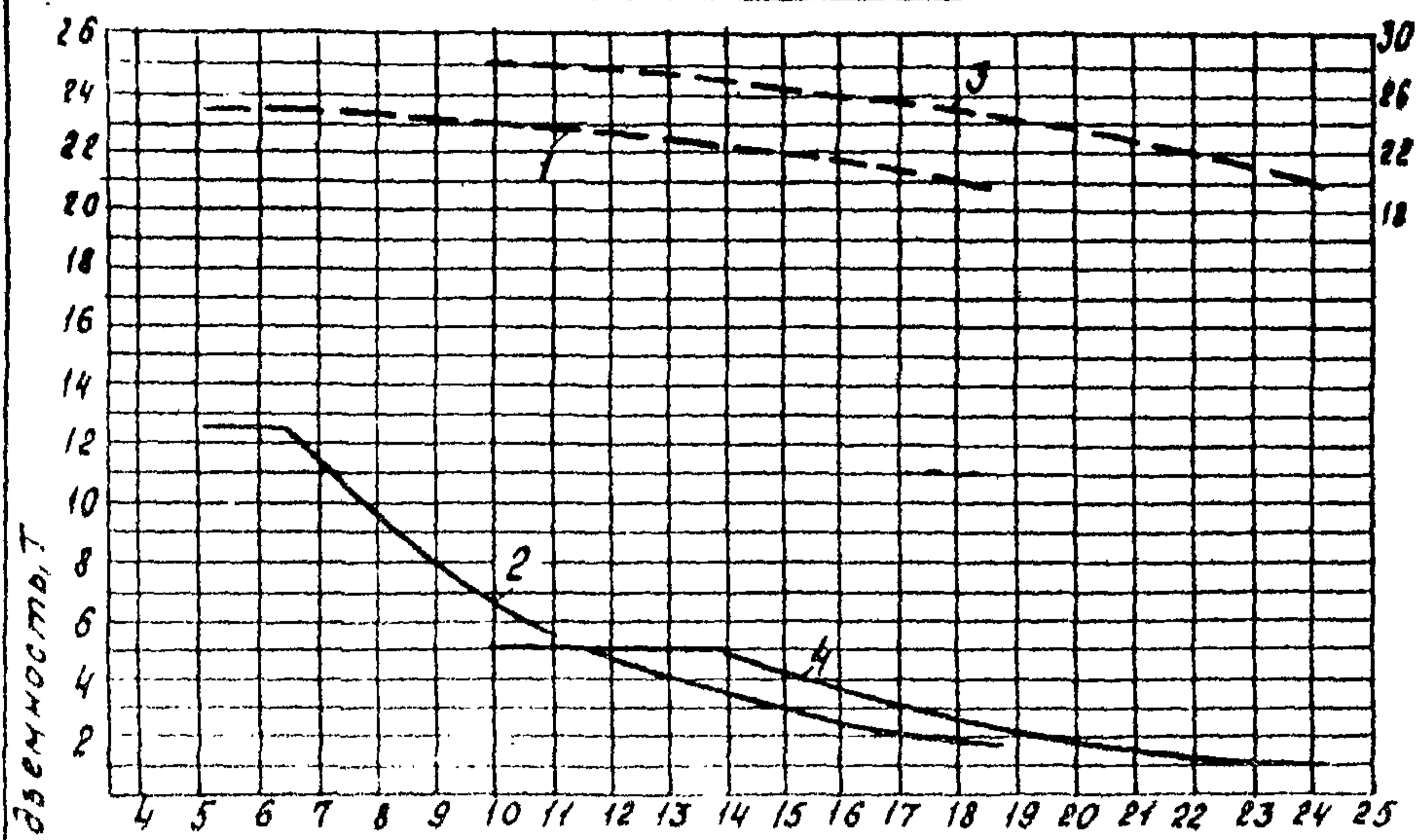
Стрела 32,5м
