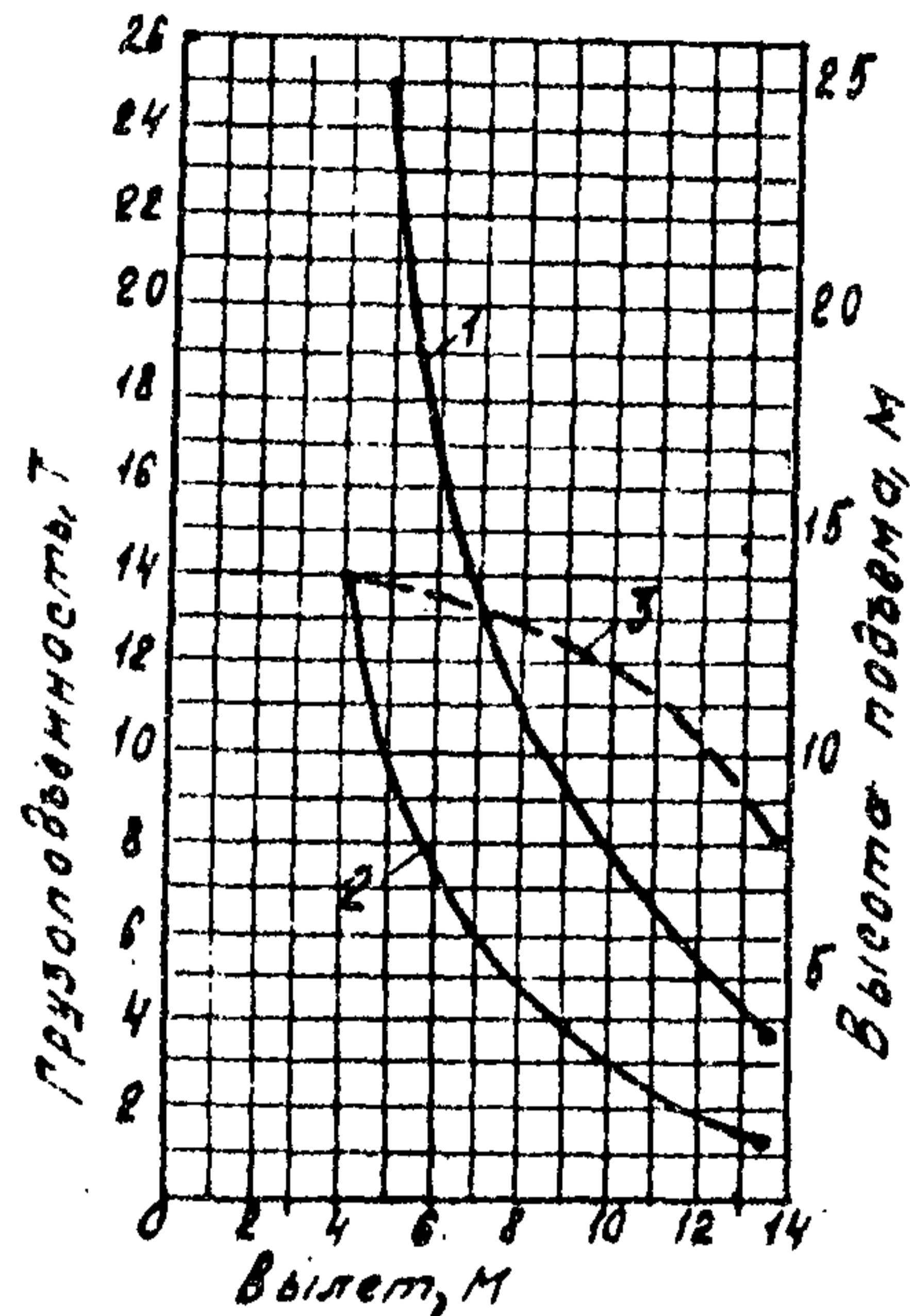
Стрела 15 м
