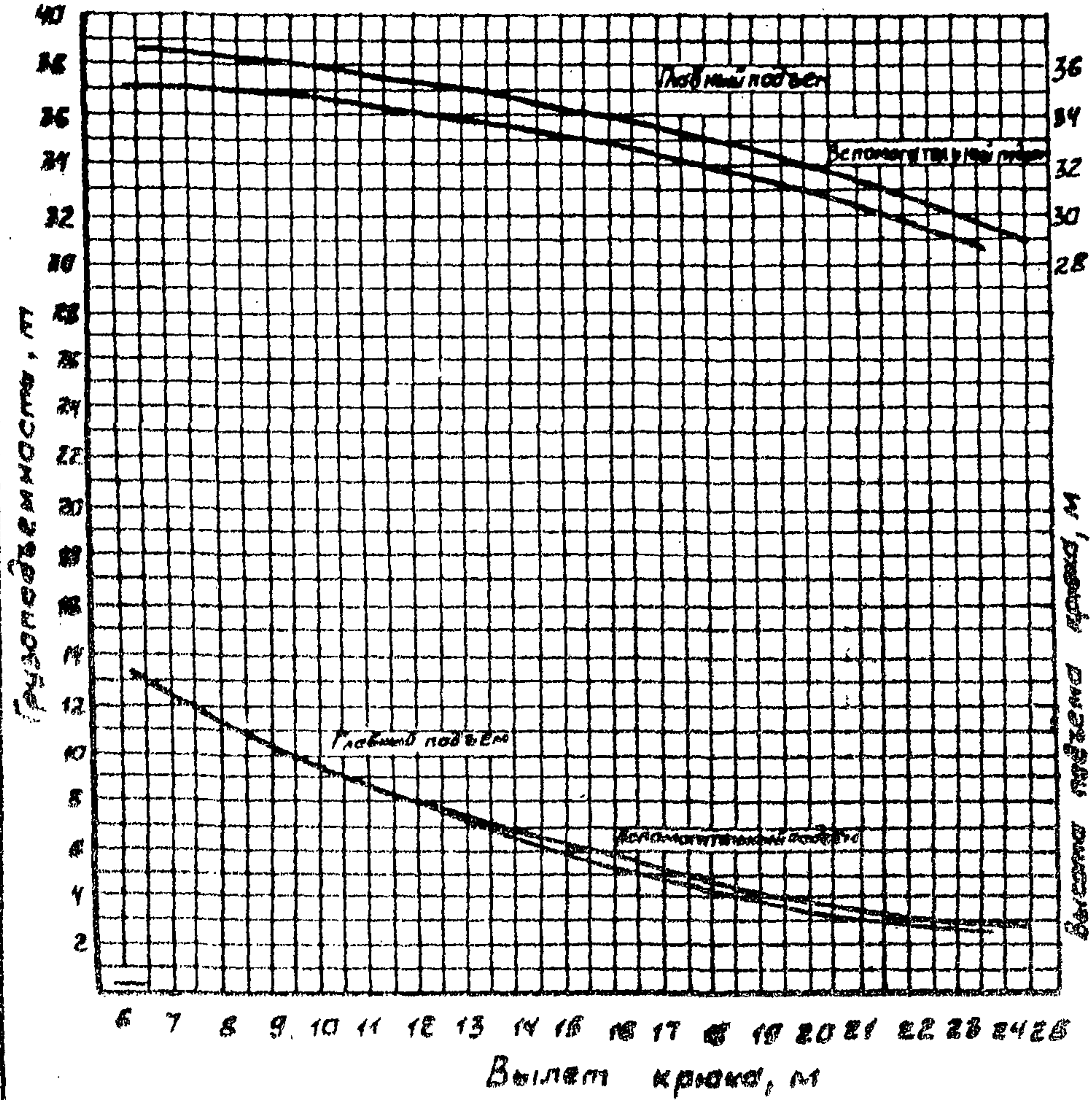
Стрела 36 м без гуська
