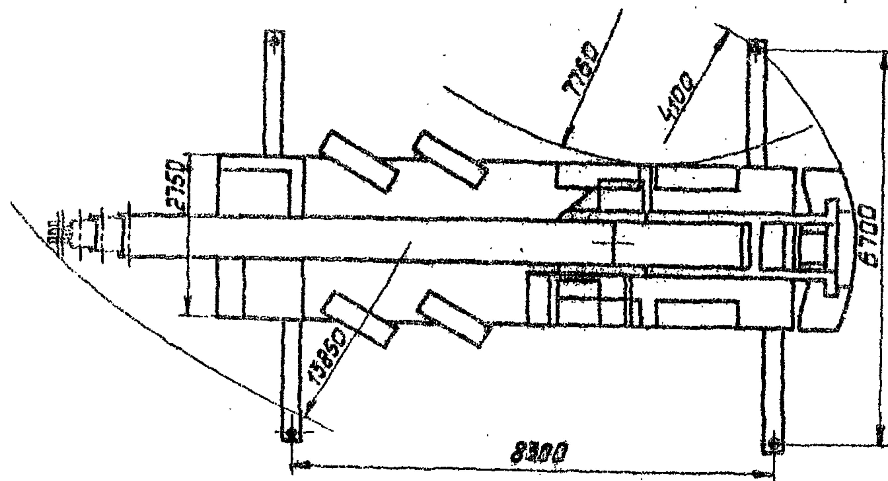
Размер внешних опор в плане
