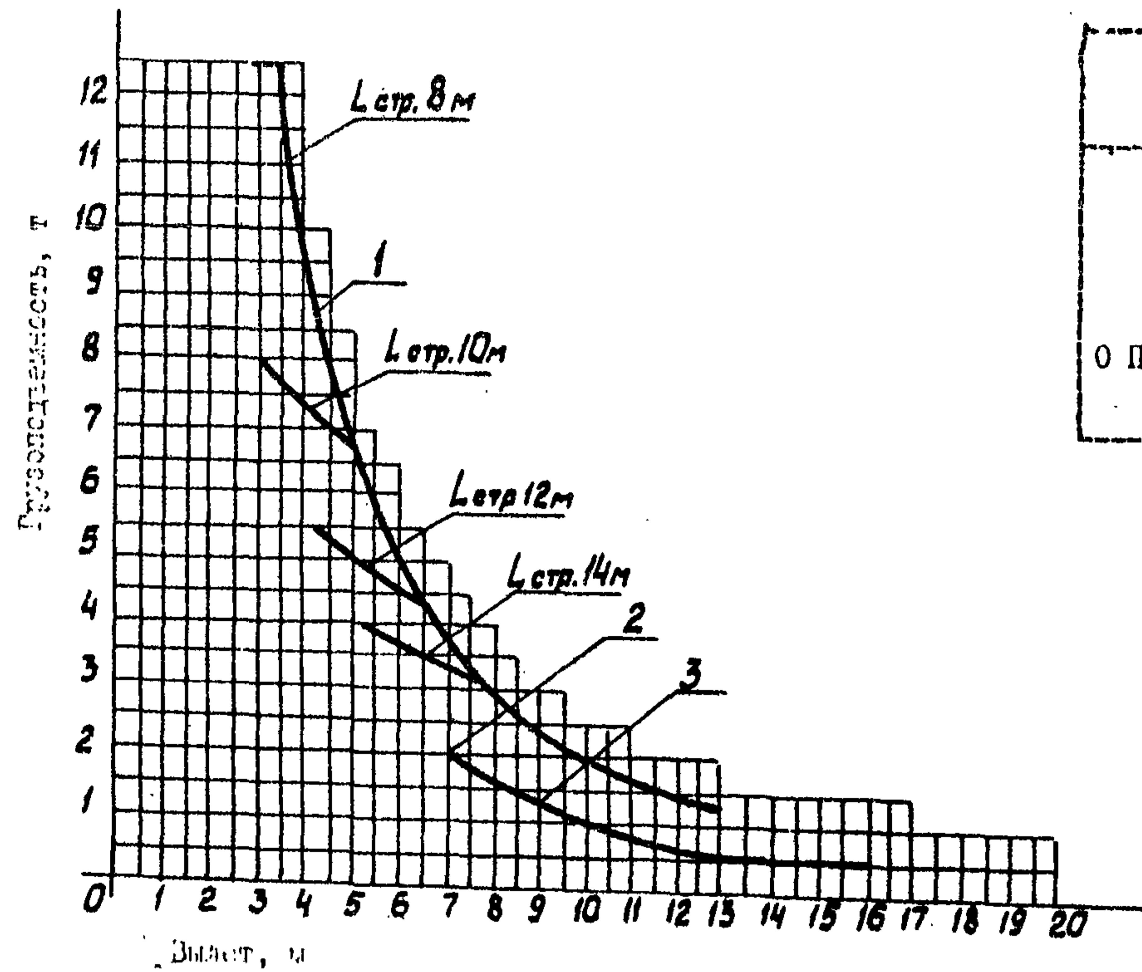
График грузоподъемности
