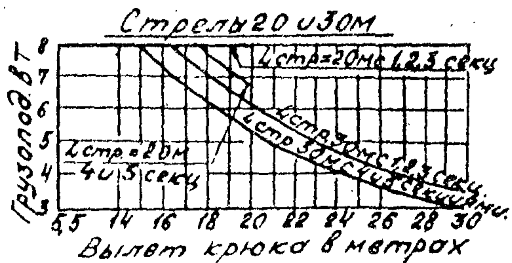
Кривые грузоподъемности для стрел с движущейся кареткой.
