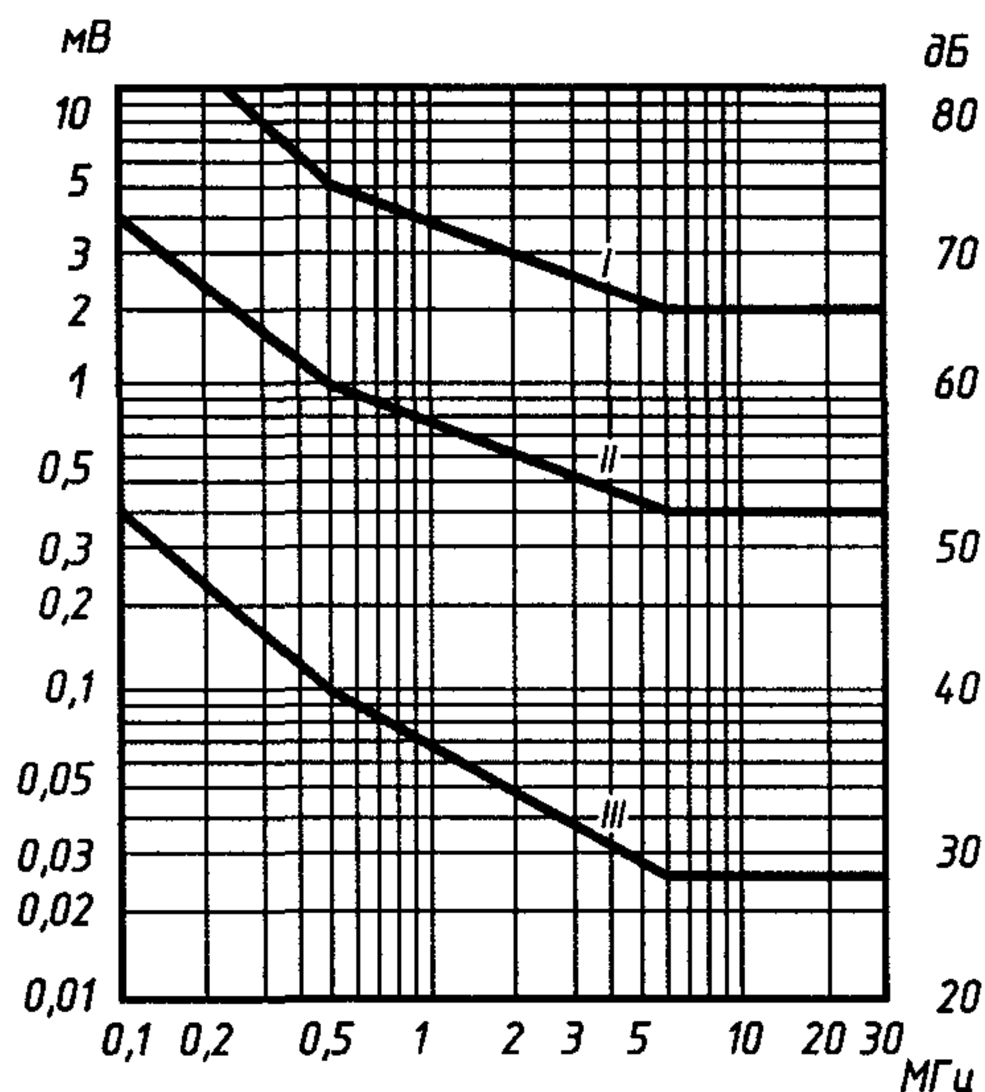
Рис. 2.7.1 Напряжения помех, допустимые для устройств, расположенных:
