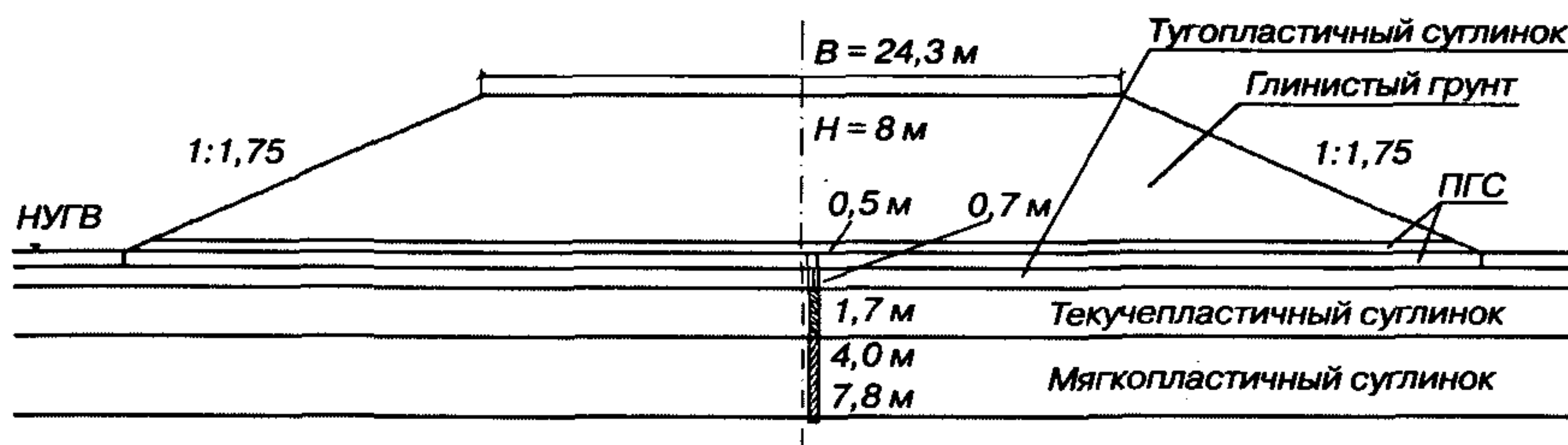
Рис. 3.2.10. Схема насыпи на ПК 9+50
