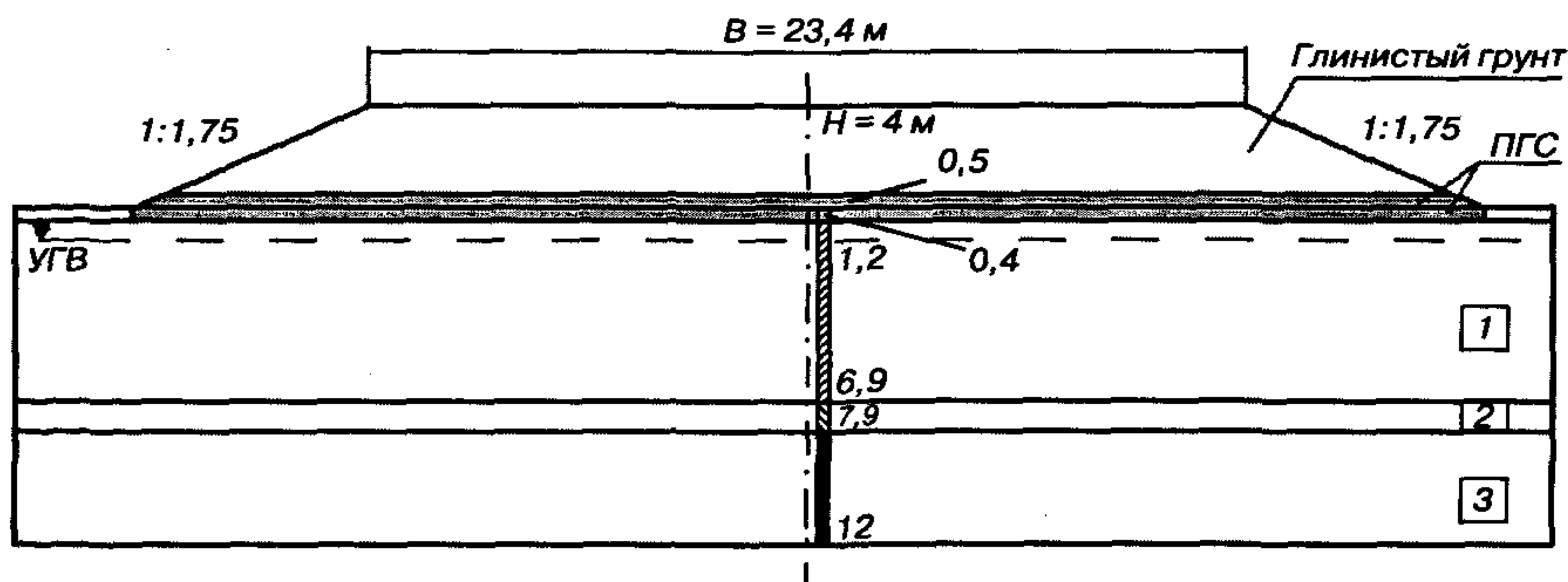
Рис. 3.2.5 Насыпь высотой 4 м на слабом основании
