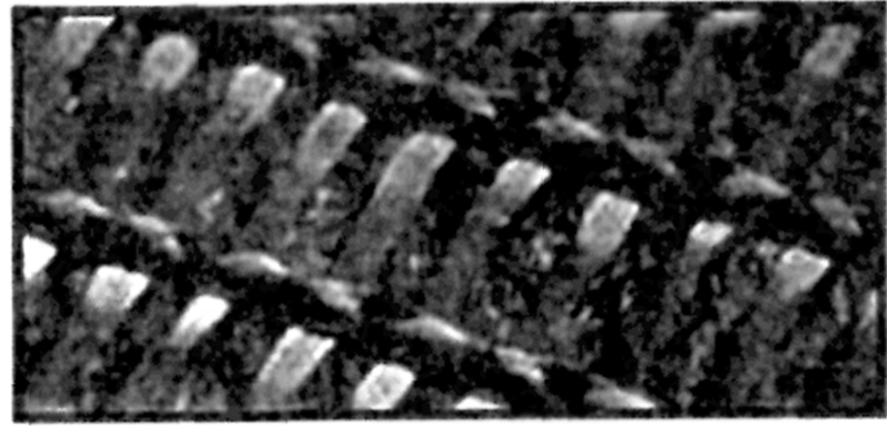
Рис. 6.2. Армирующий материал с высоким пределом прочности Полифелт Rock PES
