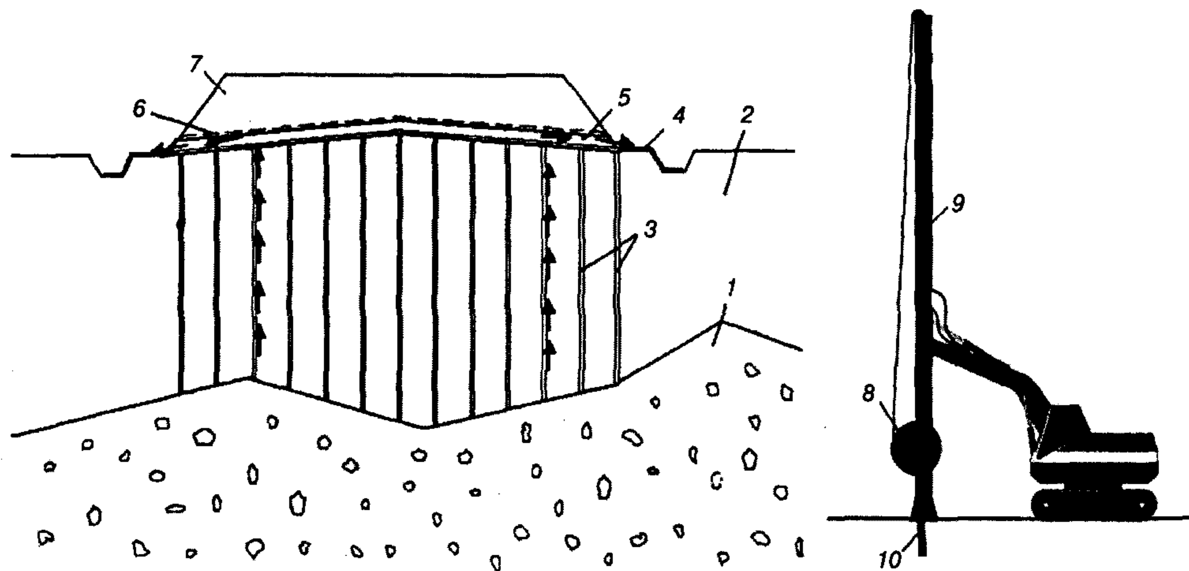
Рис. 13.1. Устройство вертикальных дренажных проколов на строительстве КАД в г. Санкт-Петербург:
