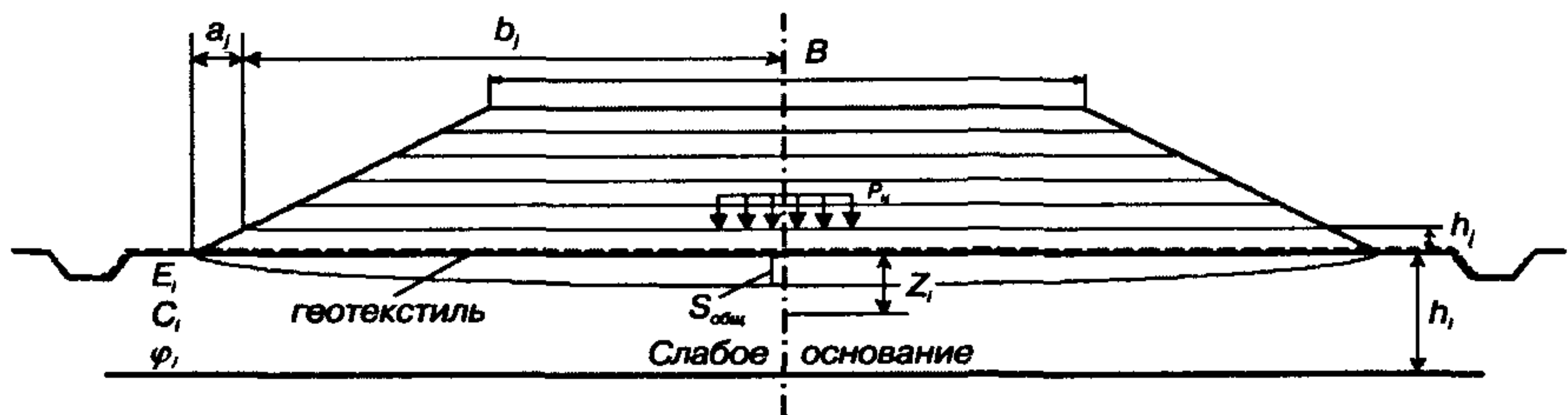
Рис. 6.6. Схема укладки геотекстиля в основании
