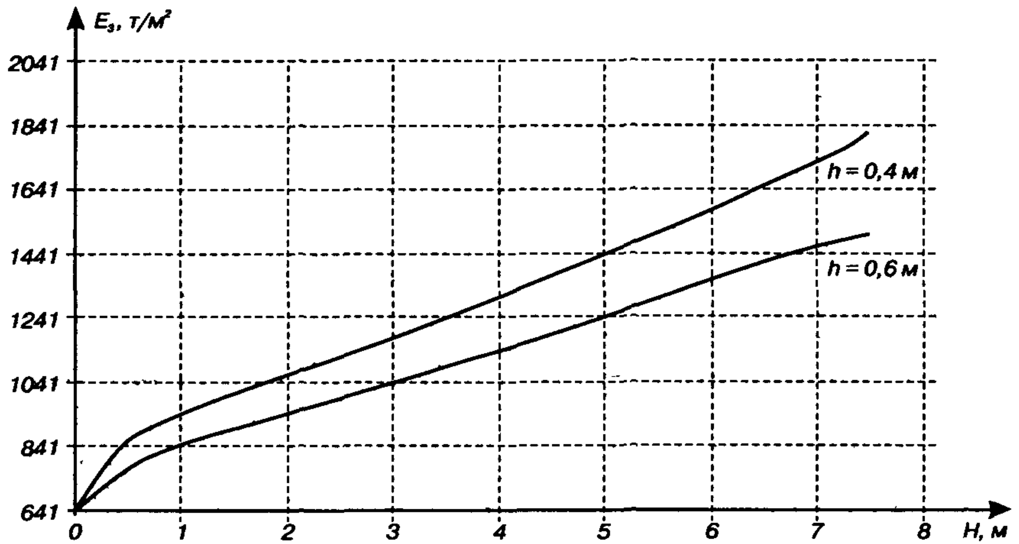
Рис. 3.2.15. Зависимость модуля деформации 3-го слоя основания от режима отсыпки насыпи H = 7,5 м
