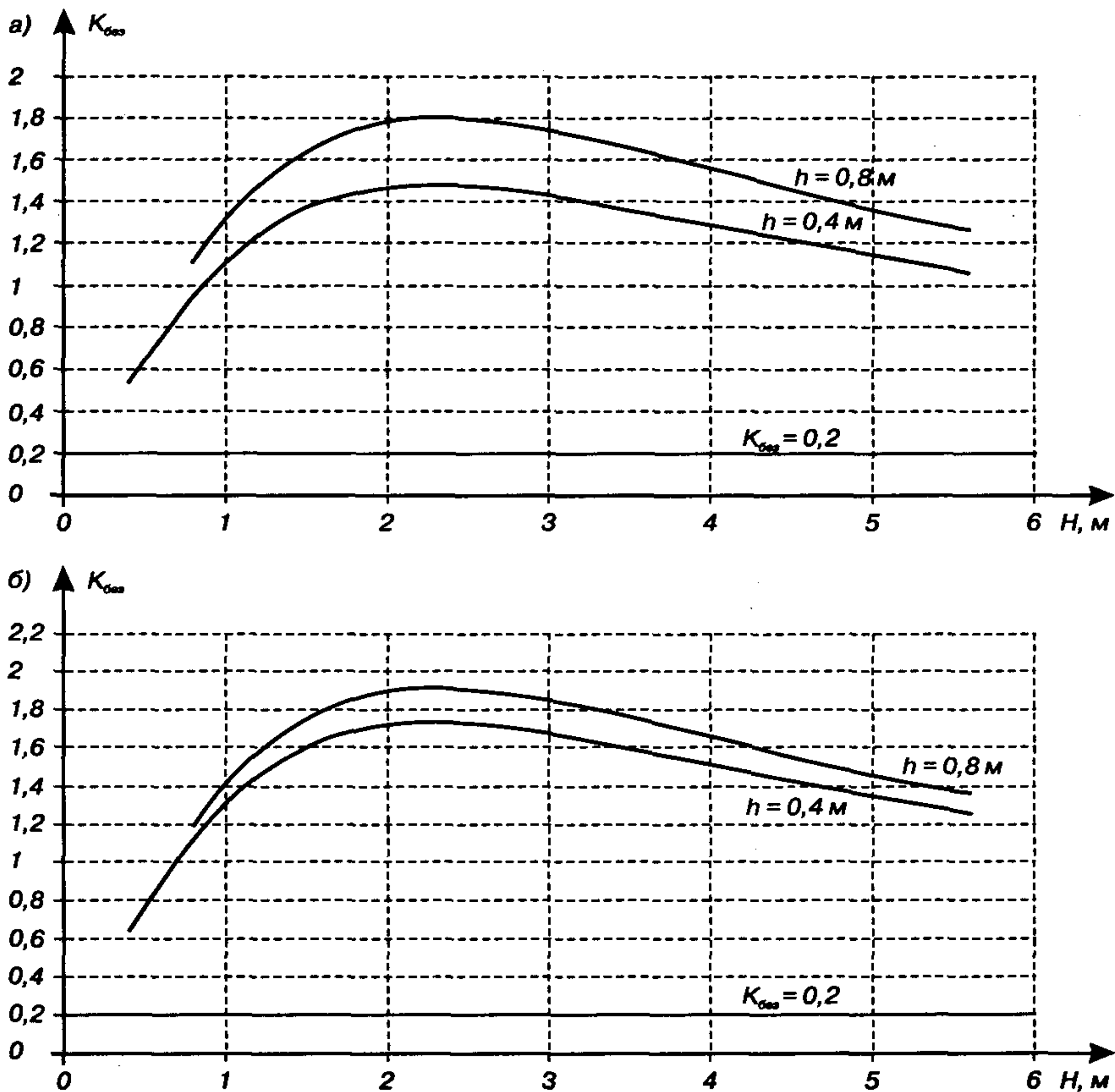
Рис. 4.2.1. Изменение K_{\text{без}} в процессе послойной отсыпки насыпи высотой 5,6 м: а - слоя суглинка мягкопластичного, б - слоя супеси текучепластичной
