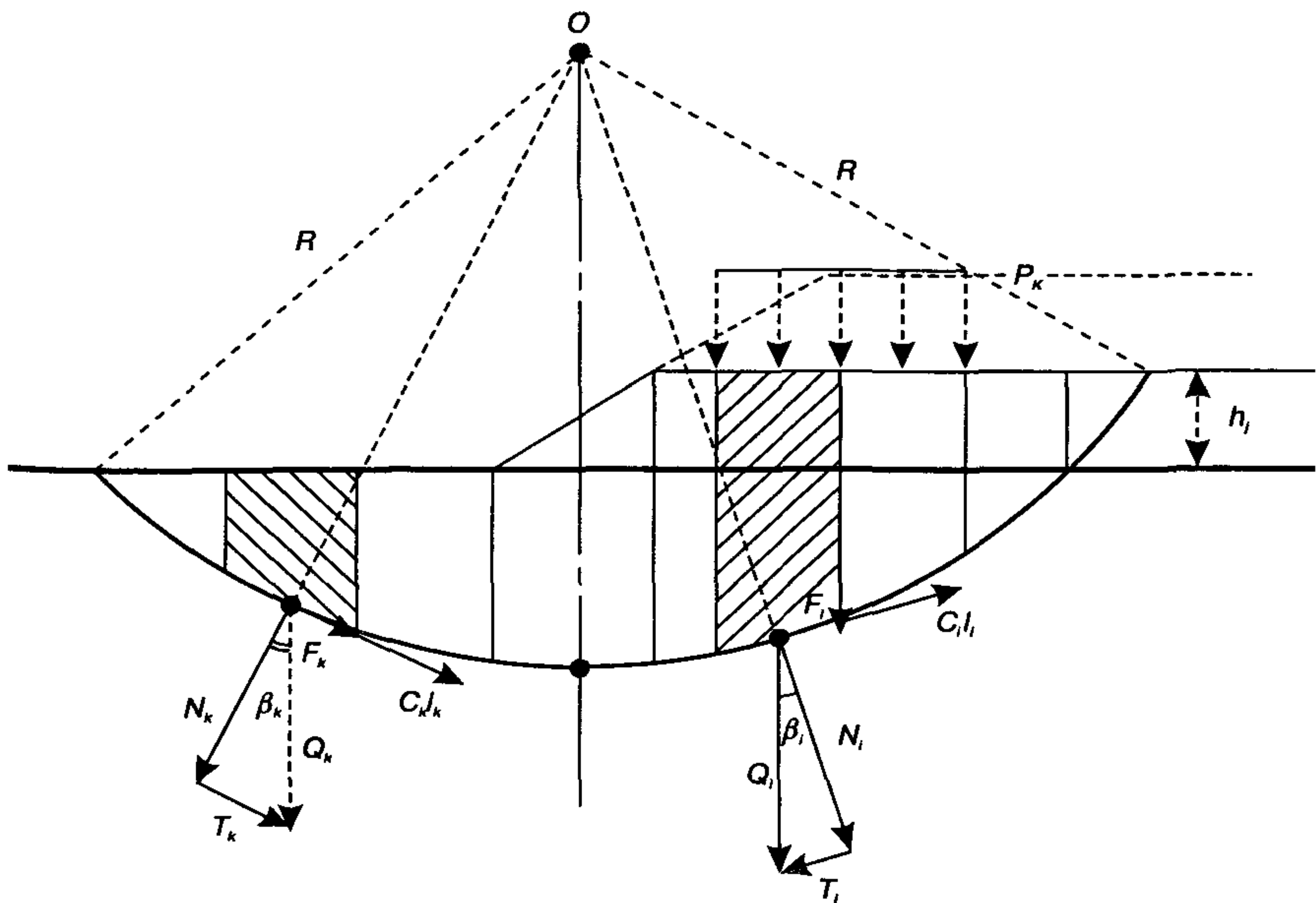
Рис. 5.1. Схема разбивки на блоки поперечного сечения насыпи и основания
