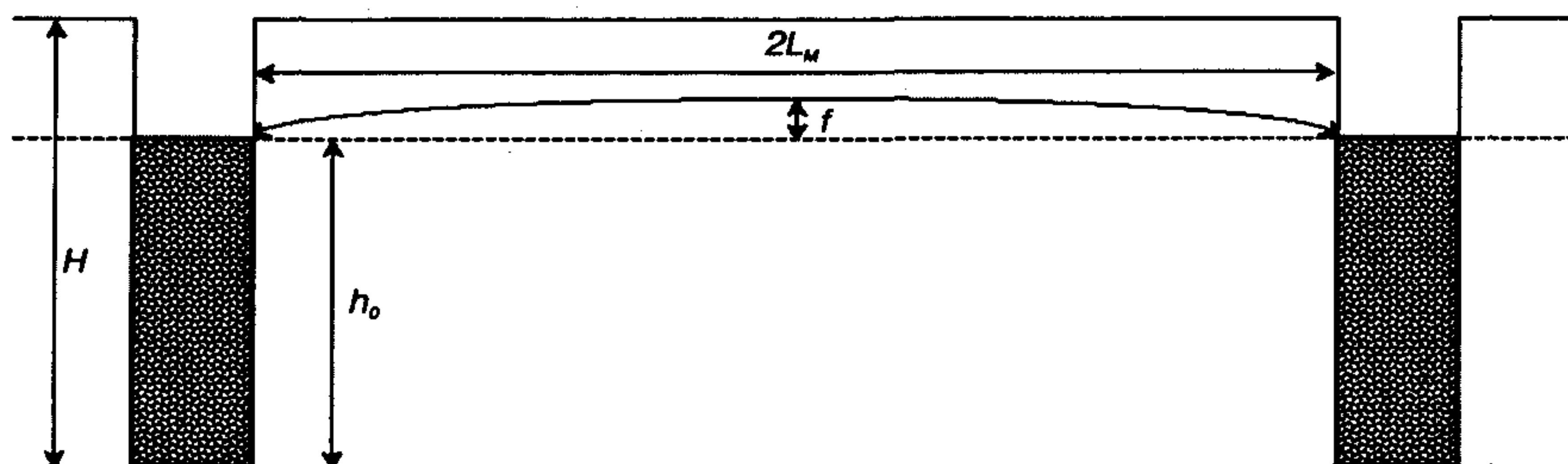
Рис. 8.1. Расчётная схема осушения дренажа
