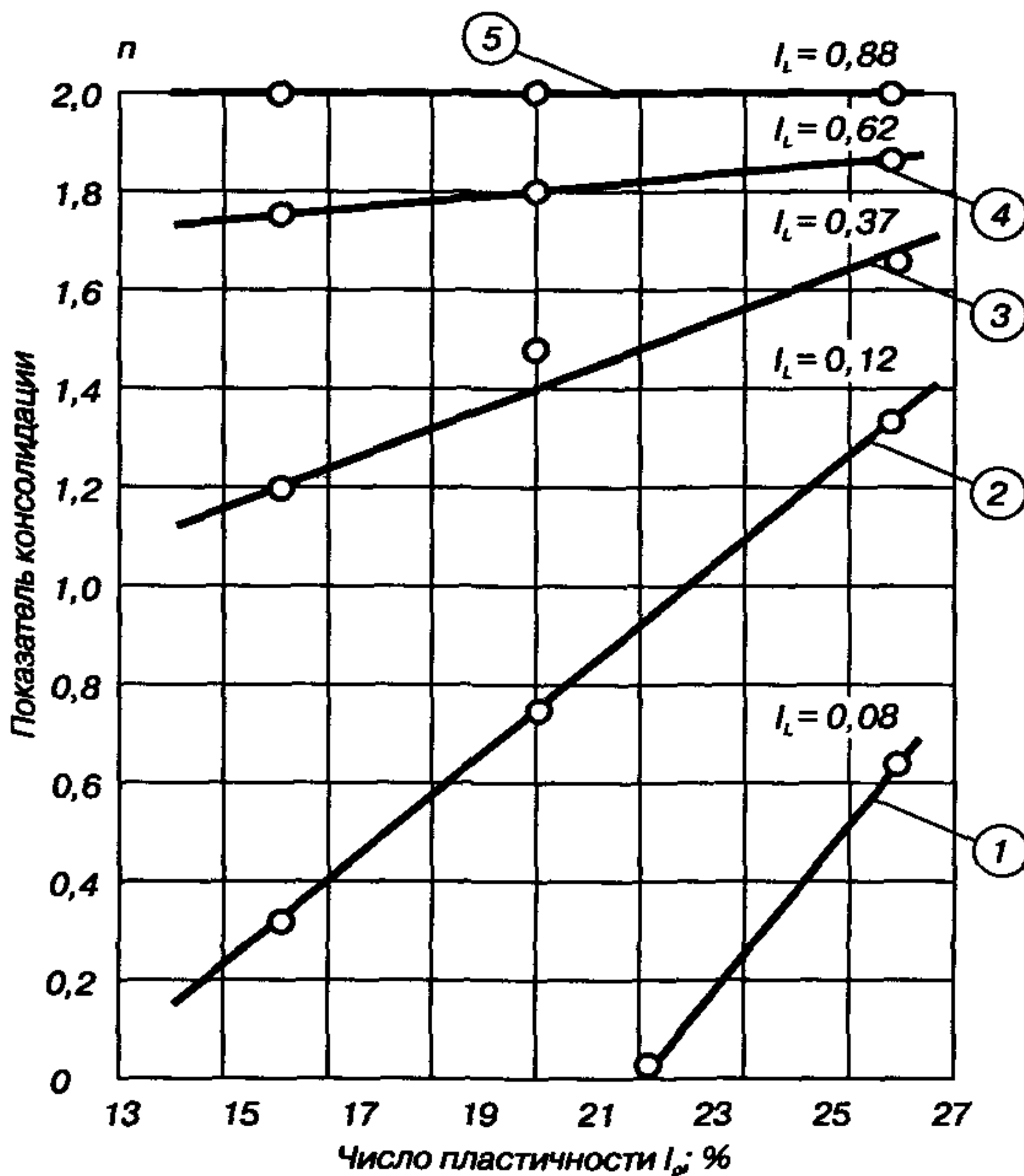
Рис. 7.1.1. Зависимость показателя консолидации n от числа пластичности грунта J_p и его консистенции J_L :
