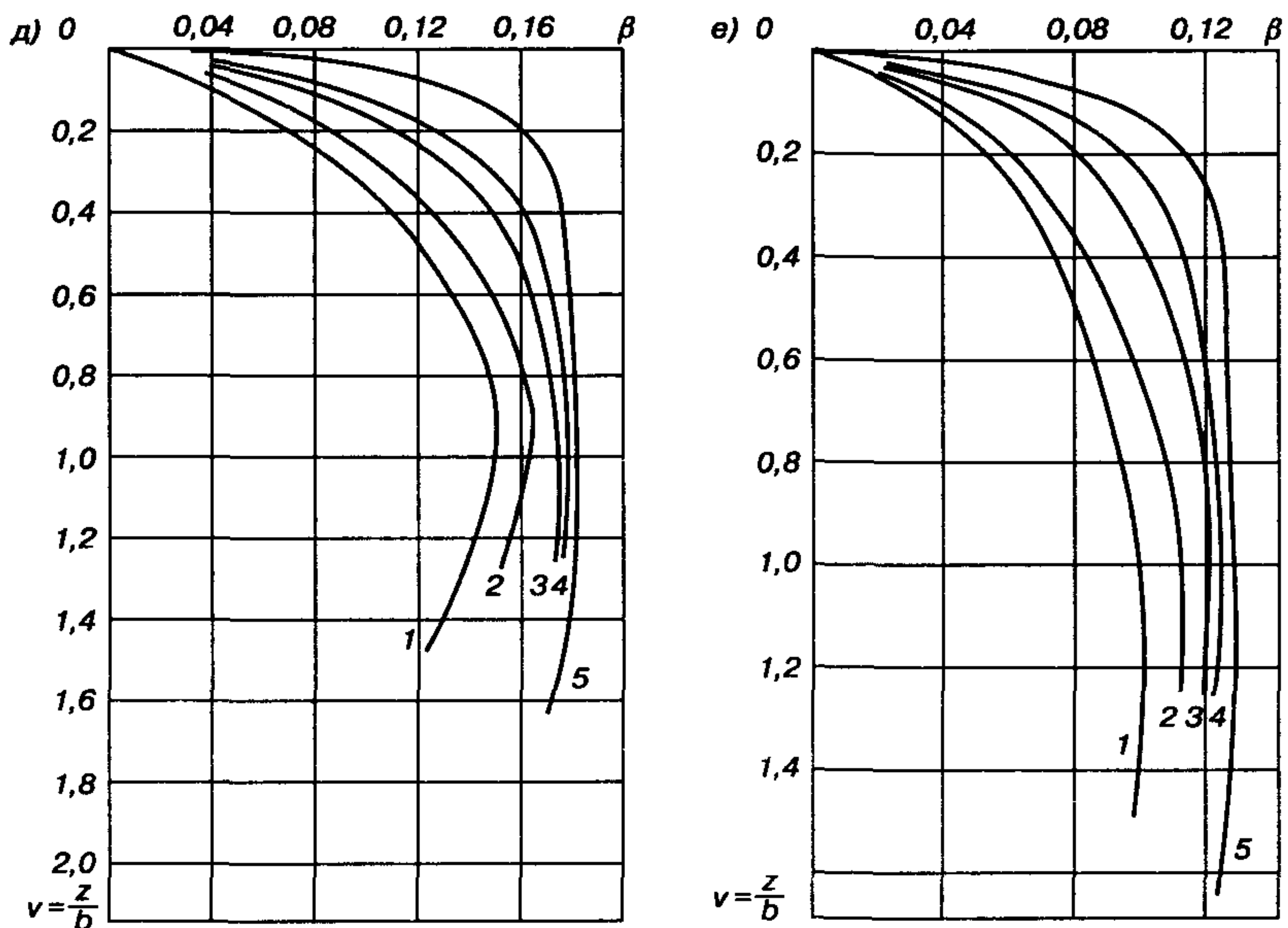
Рис. 4.1.1. Графики для определения коэффициента \beta при угле внутреннего трения: а - \varphi = 0^\circ , б - \varphi = 5^\circ , в - \varphi = 10^\circ , г - \varphi = 15^\circ , д - \varphi = 20^\circ , е - \varphi = 30^\circ ; при отношении 2a/B равном: 1 - 10,0; 2 - 3,0; 3 - 1,0; 4 - 0,6; 5 - 0,2.
