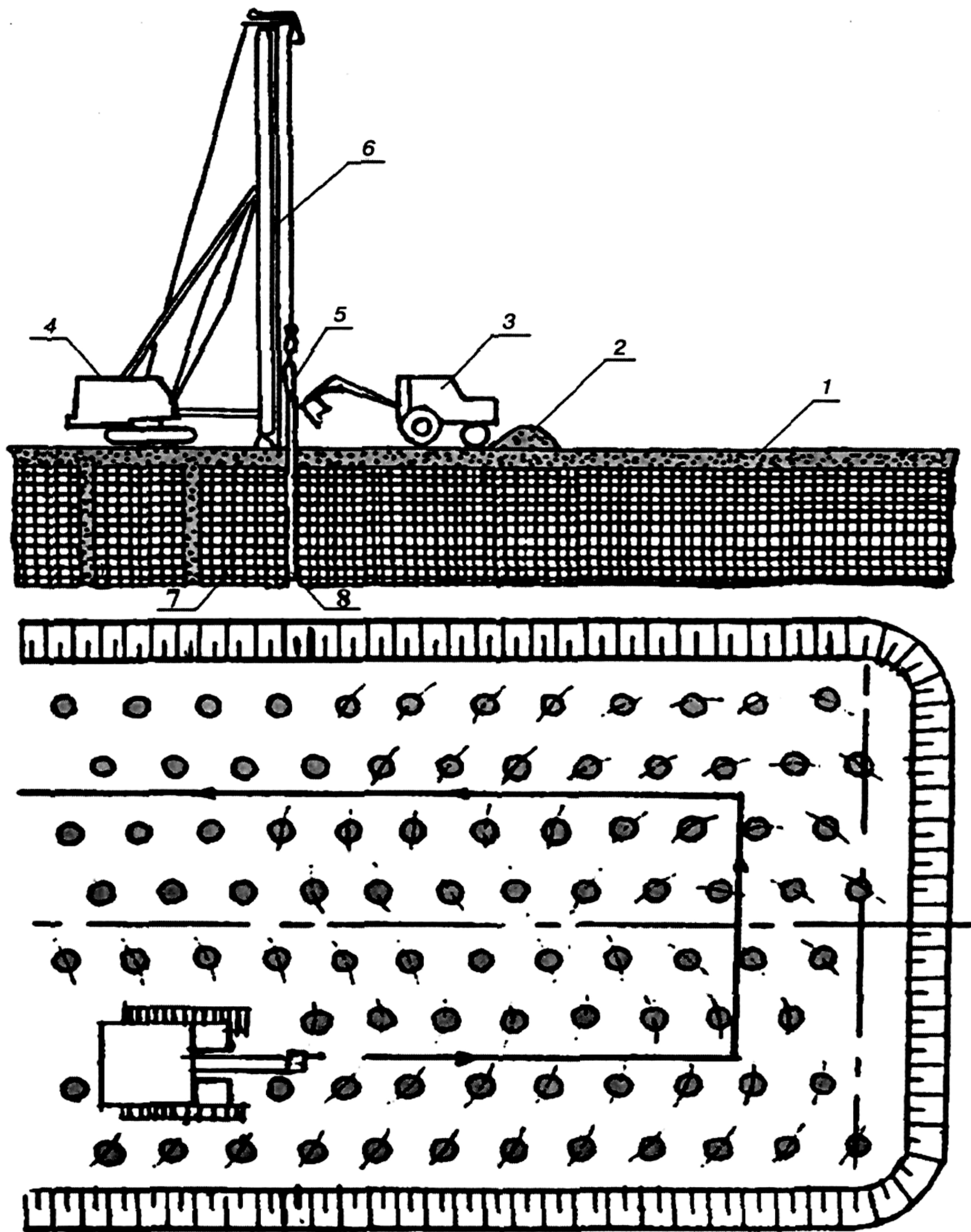
Рис. 11.2.3. Технологическая схема устройства вертикальных песчаных дрен: 1 - защитный слой; 2 - песок для дрен; 3 - погрузчик; 4 - базовая машина; 5 - вибропогружатель; 6 - копровая мачта; 7 - торф; 8 - обсадная труба
