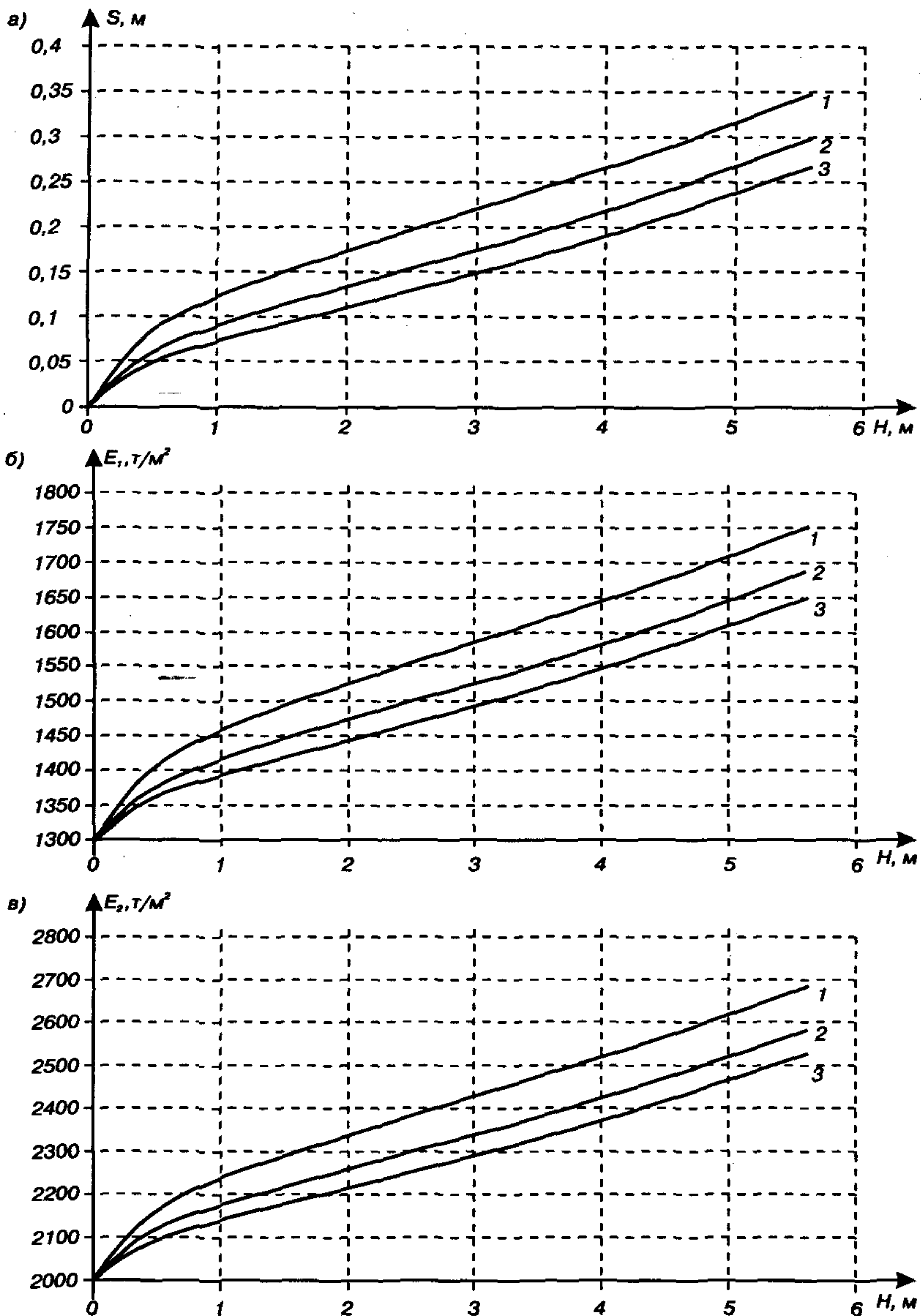
Рис. 3.2.4 Зависимость деформационных характеристик грунтов основания от общей нагрузки катков:
