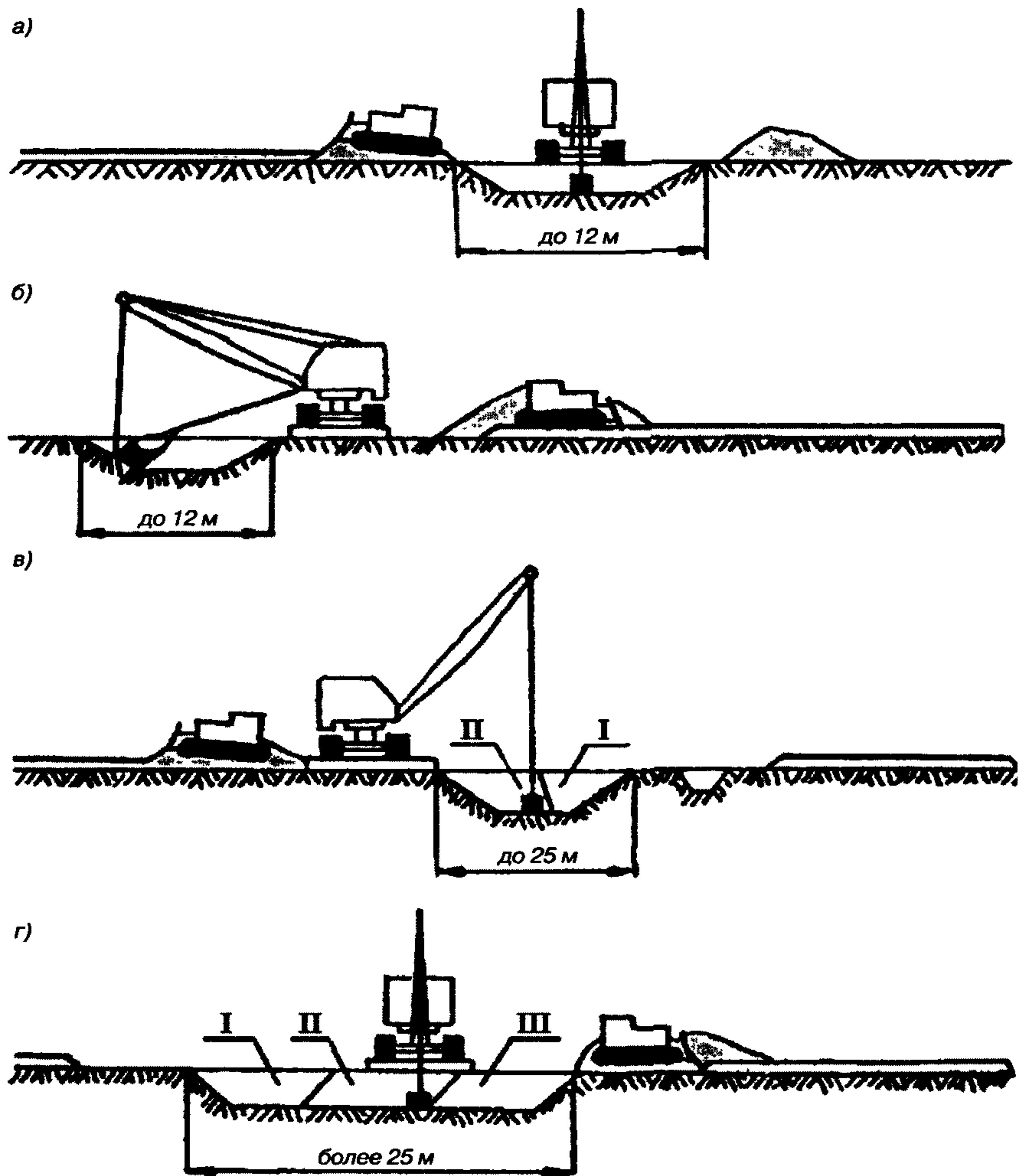
Рис. 11.2.1. Схемы разработки траншеи:
