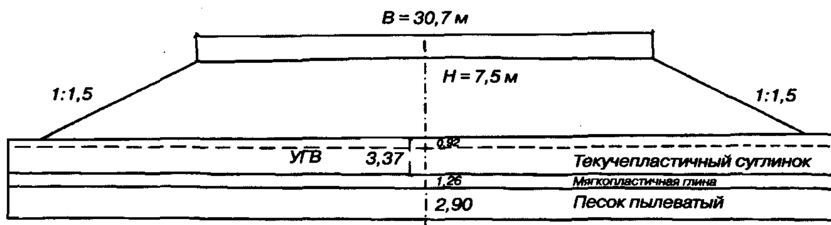
Рис. 3.2.9. Насыпь высотой 7,5 м на ПК 5+17,77
