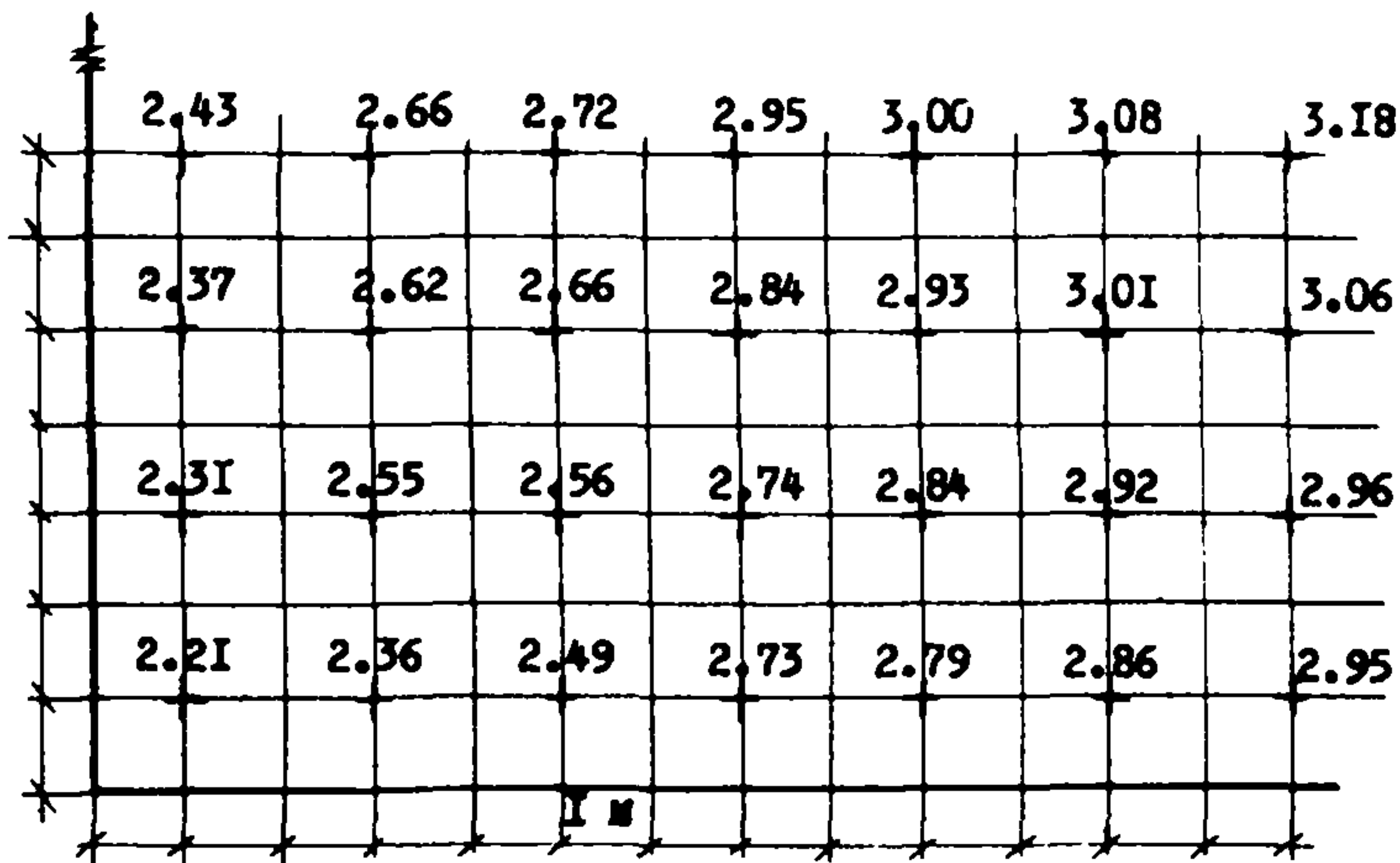
Рис. 1. Нагрузка на плиту, т (I т =100 кН)
