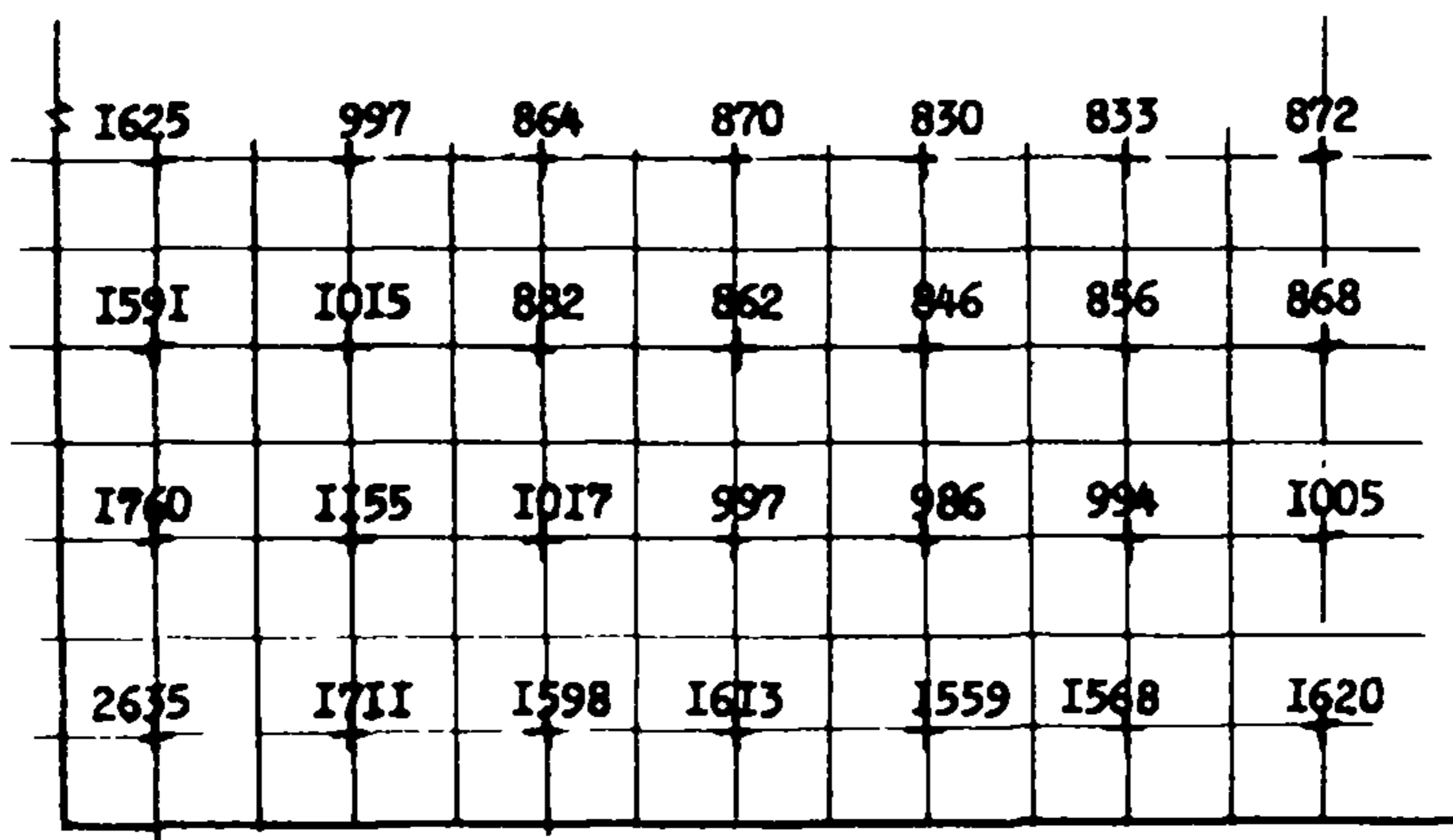
Рис. 3. Распределение давлений на свайное поле, т/м 2 ( 1 т/м 2 ≈ 0,01 МПа )
