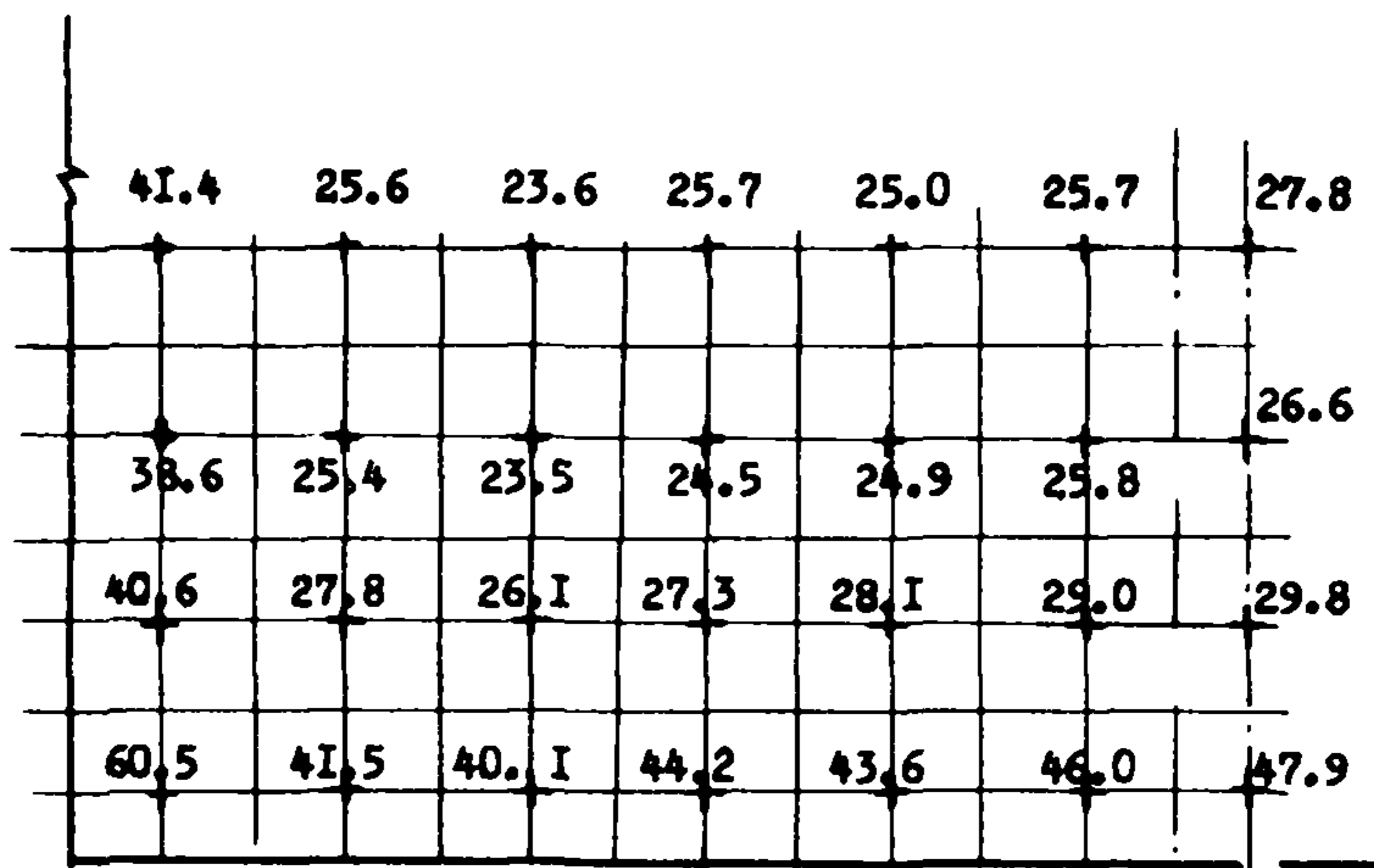
Рис. 3. Распределение давлений на свайное поле, т/м 2 ( 1 т/м 2 ≈ 0,01 МПа )
