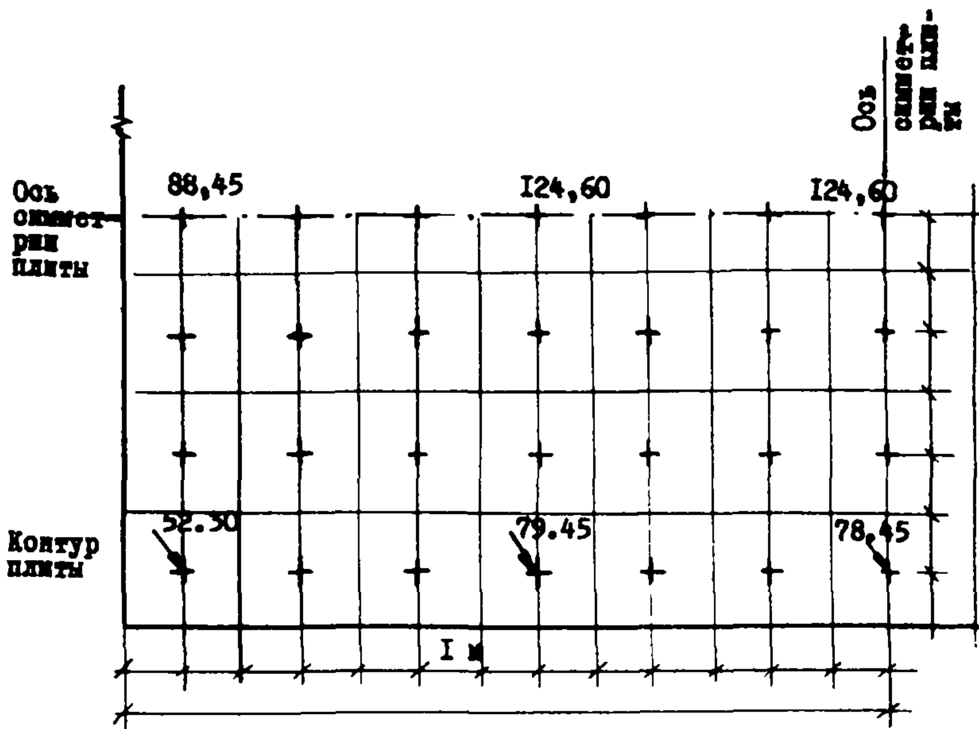
Рис. 1. Нагрузка на плиту, т (I т =100 кН)
