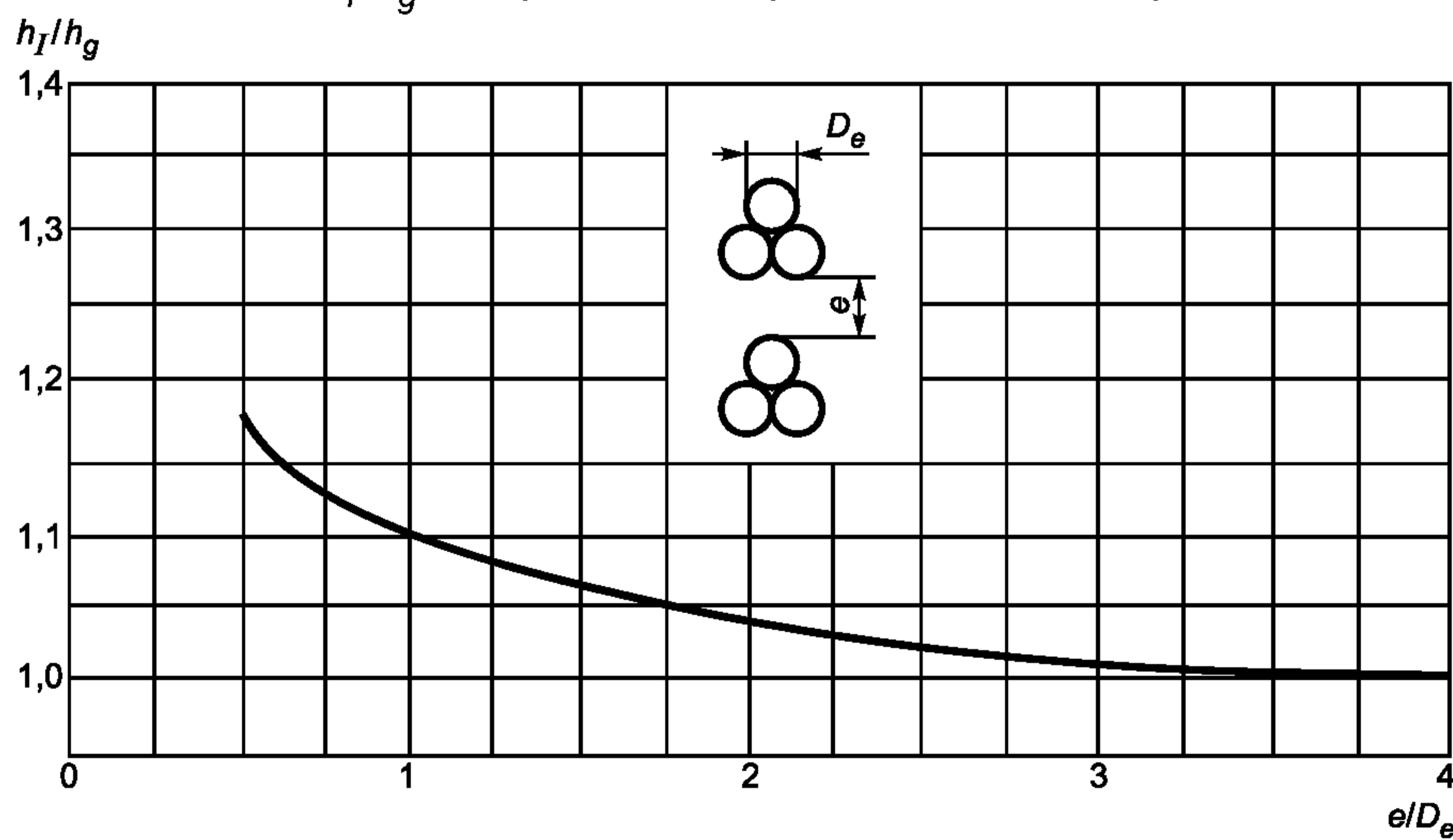
Рисунок 5 — Значения h_I/h_g для двух групп из трех кабелей, расположенных треугольником, в вертикальной плоскости
