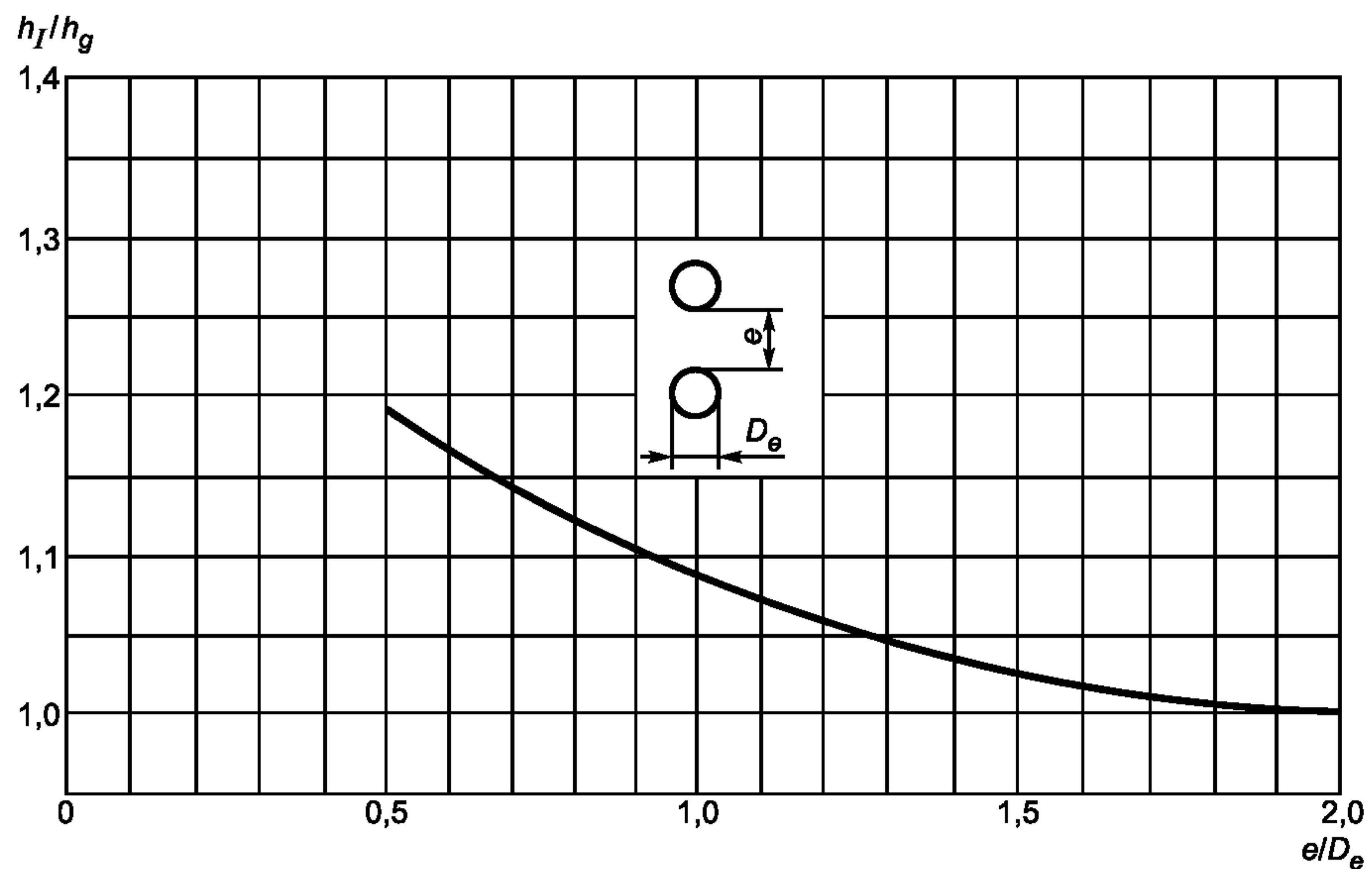
Рисунок 3 — Значения h_I/h_g для двух кабелей, расположенных в вертикальной плоскости
