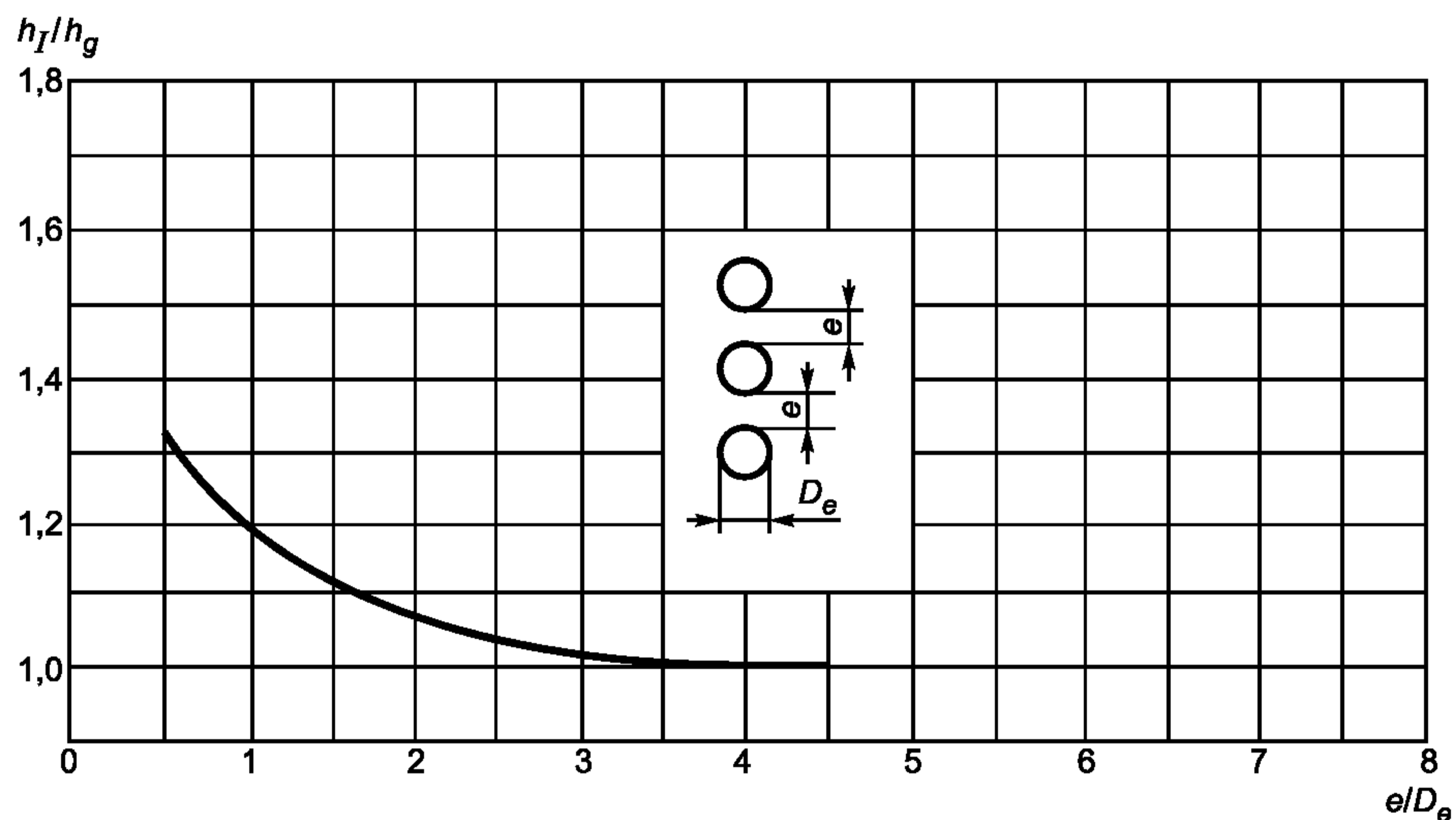
Рисунок 4 — Значения h_I/h_g для трех кабелей, расположенных в вертикальной плоскости
