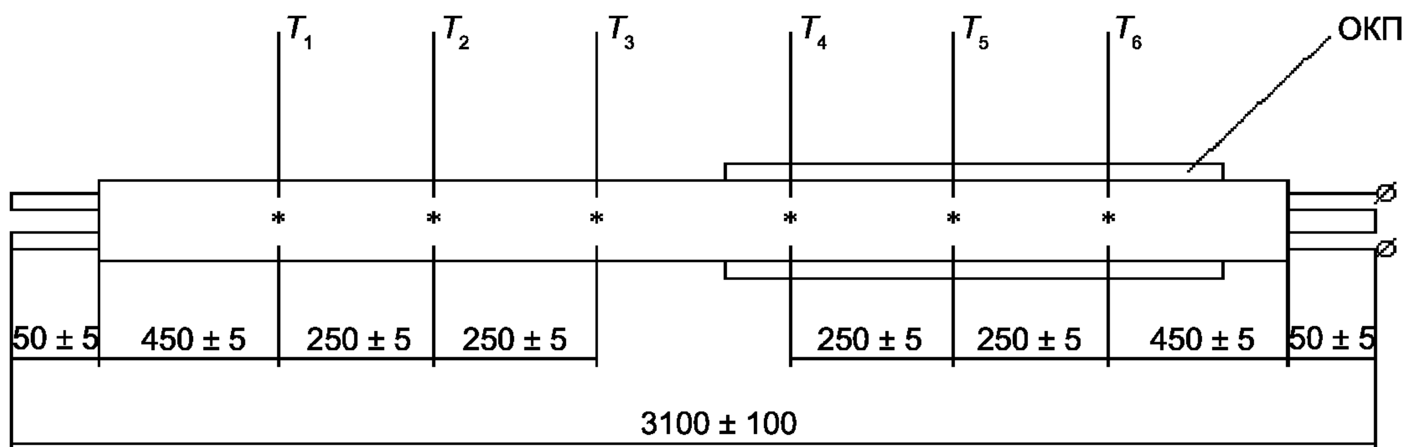
Рис. 1 — Размещение термоэлектрических преобразователей
