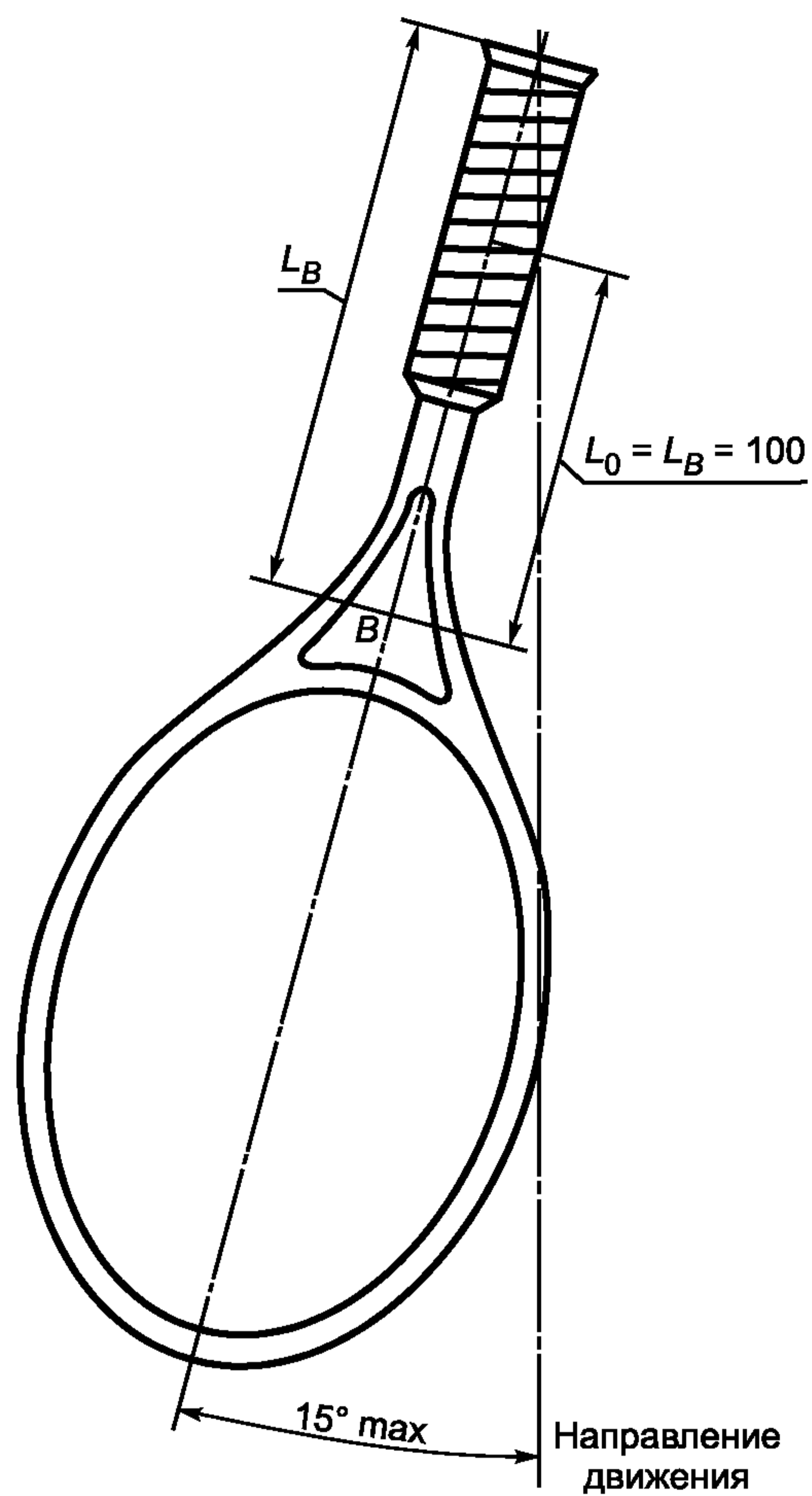
Рисунок А.1 — Момент инерции относительно оси Y
