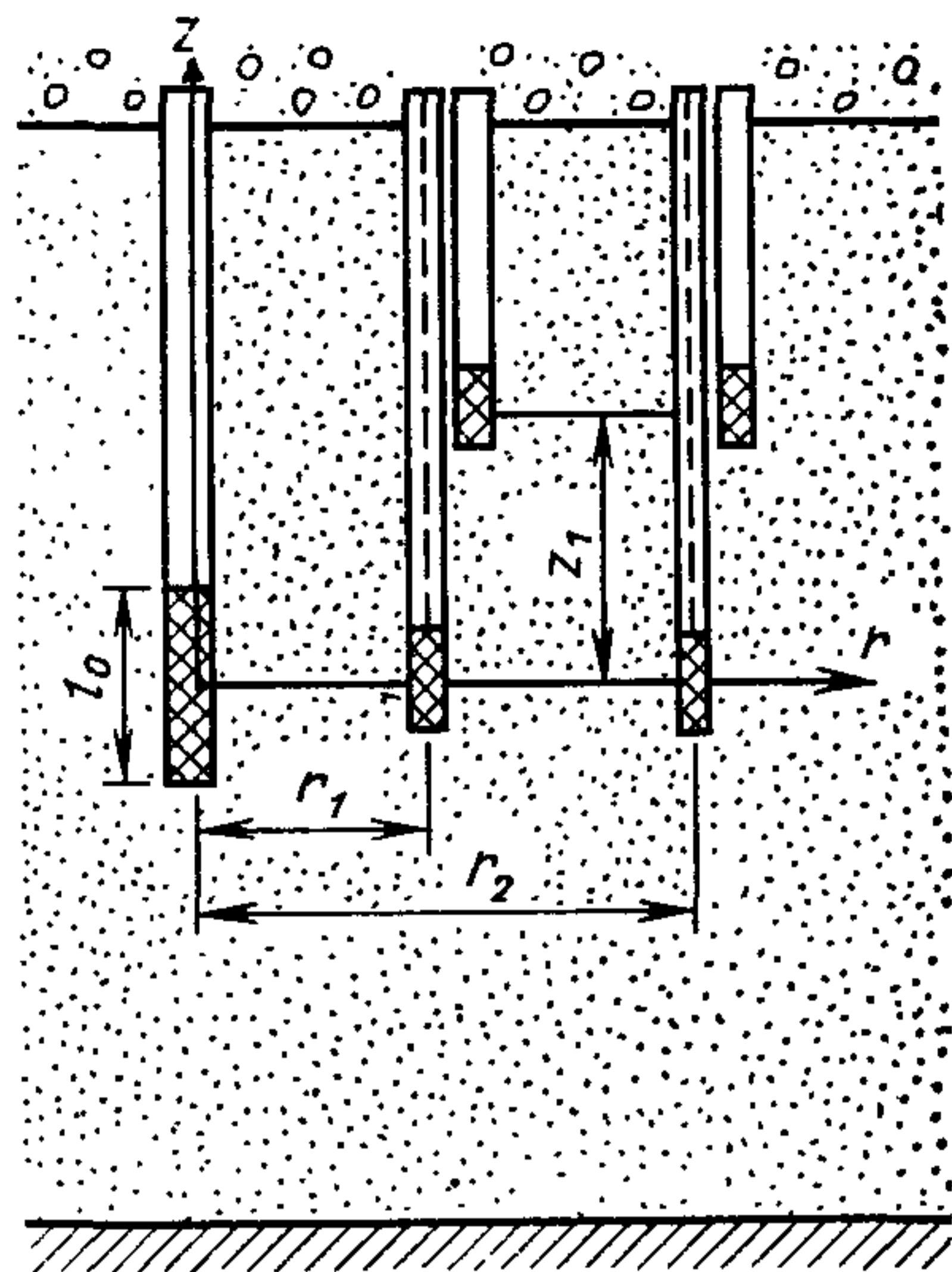
Рис. 32. Схема установки фильтров в однородно-анизотропной толще
