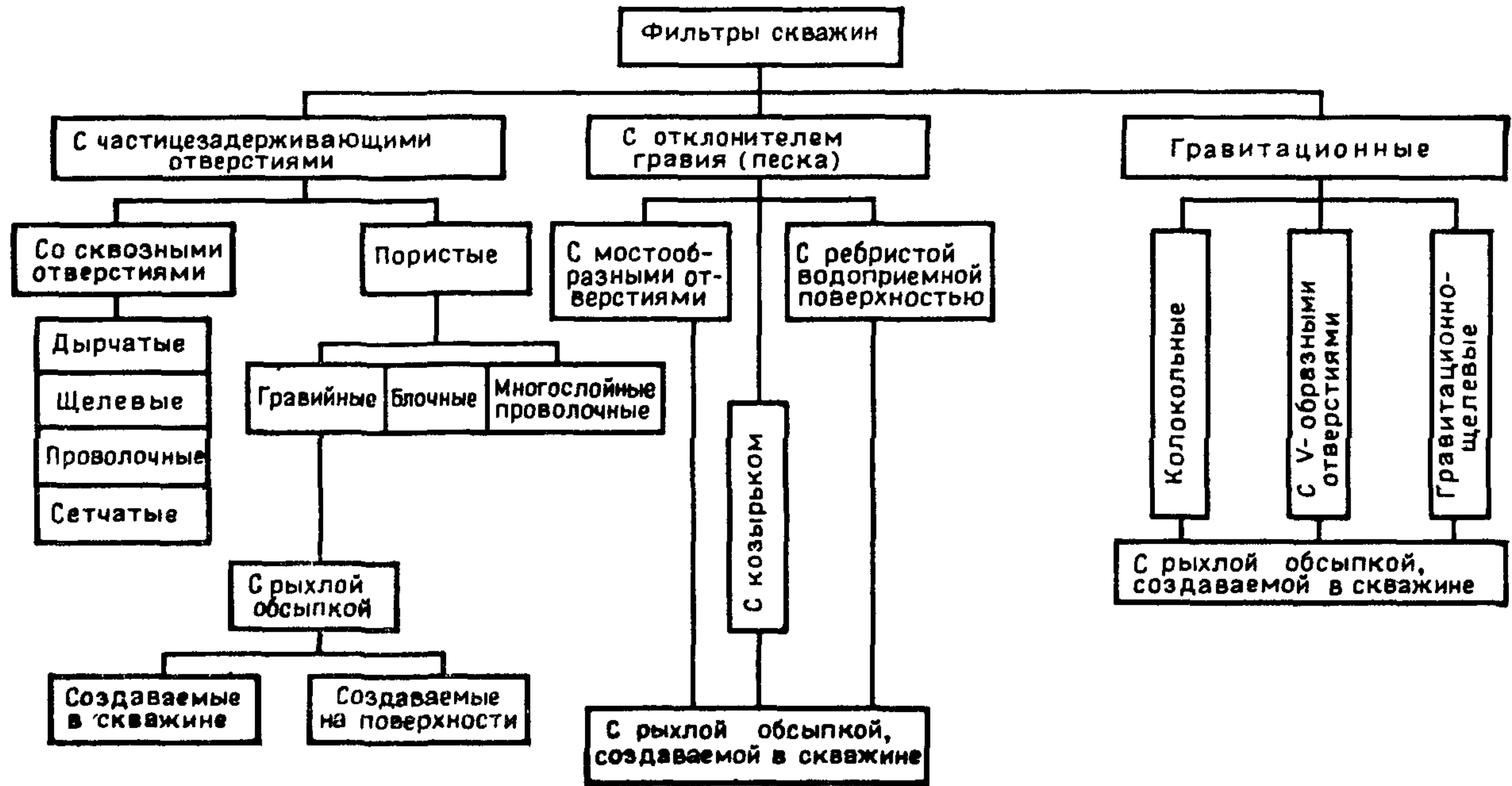
Рис. 16. Классификация фильтров
