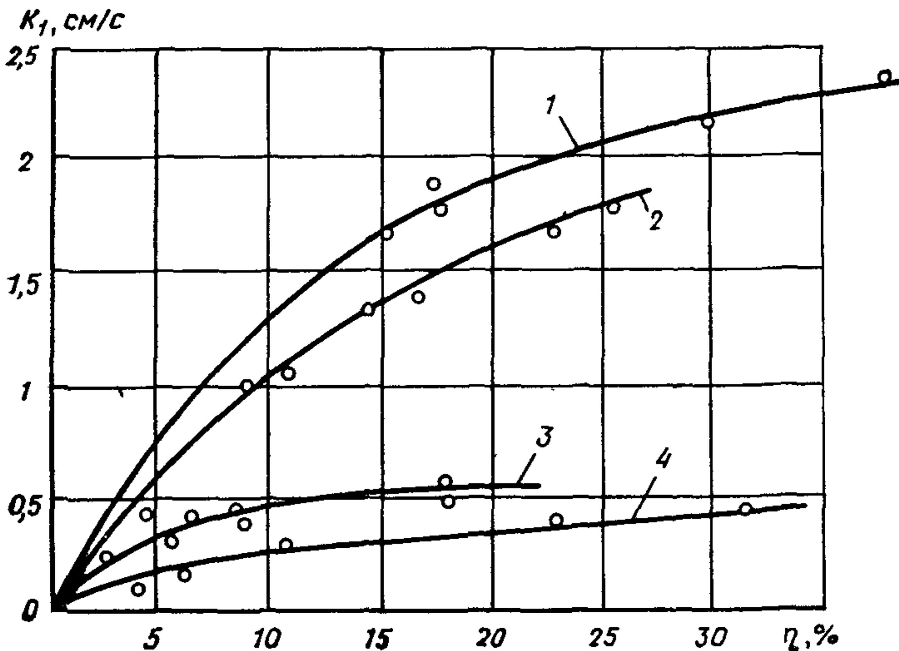
Рис. 17. Зависимость коэффициента водопроницаемости фильтров от скважности для
