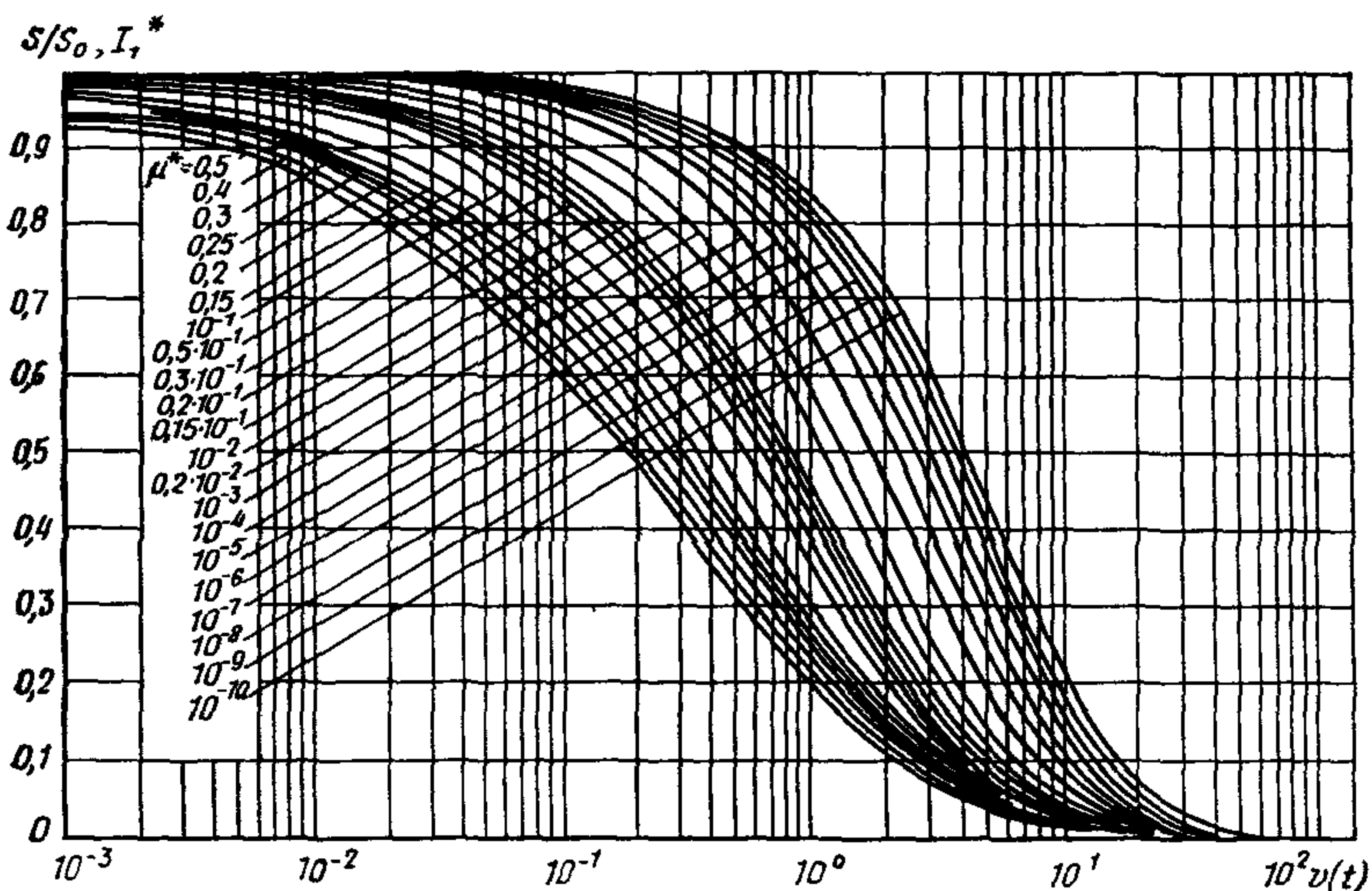
Рис. 34. График I^* ( \mu^* , v )
