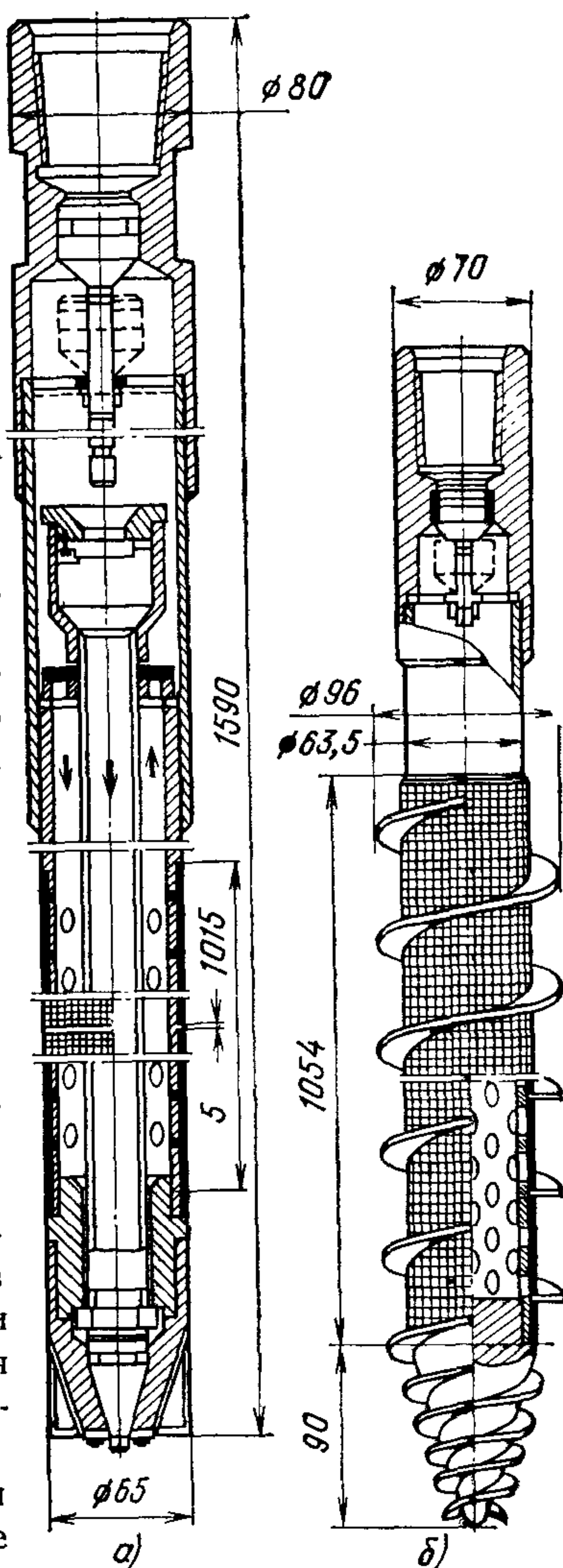
Рис. 18. Фильтры-опробователи а — промывочный; б — шнековый
