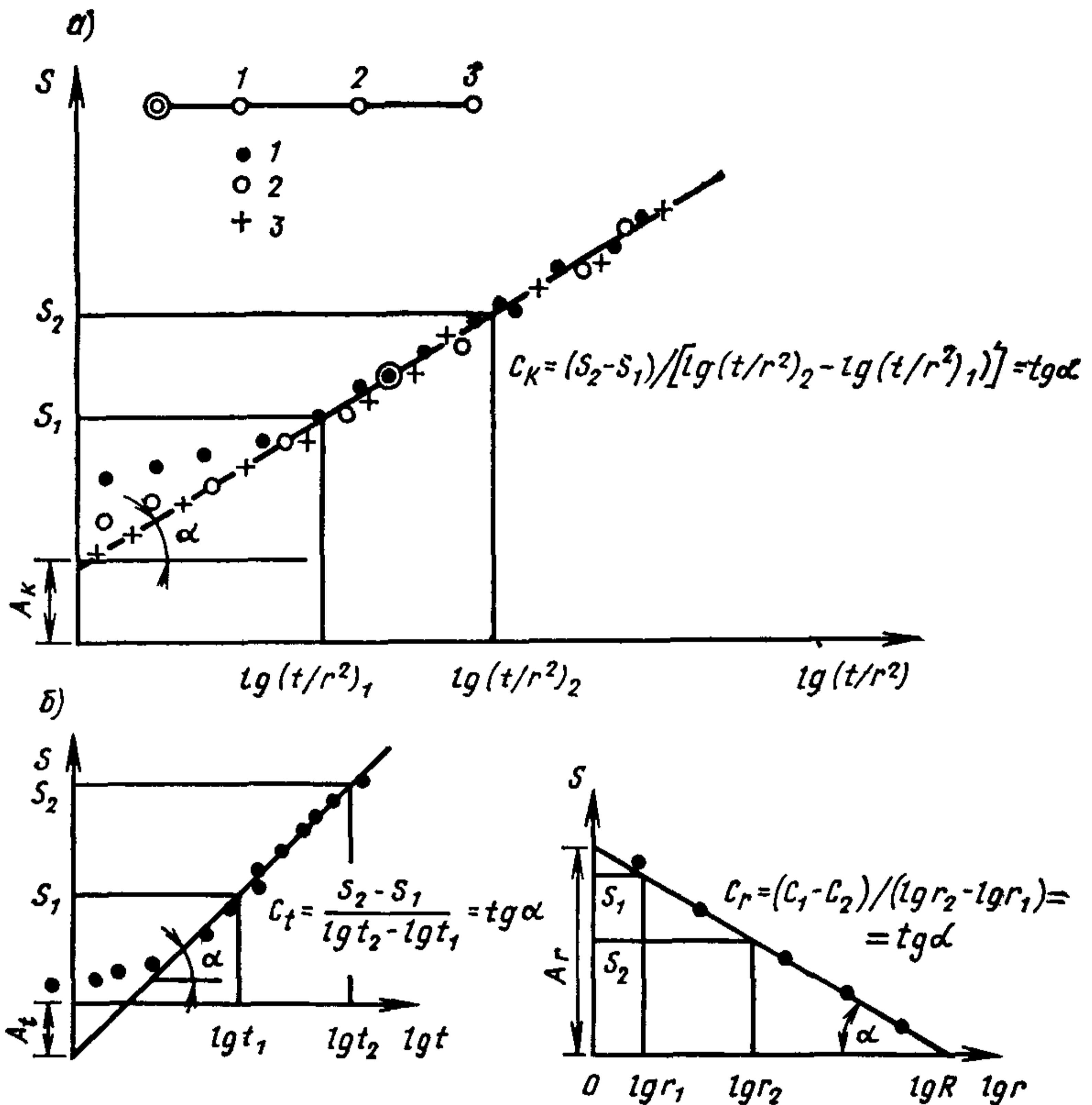
Рис. 22. Графики прослеживания понижения уровня а — комбинированного S=f(t/r^2) ; б — временного S=f(\lg t) ; в — площадного S=f(\lg r)
