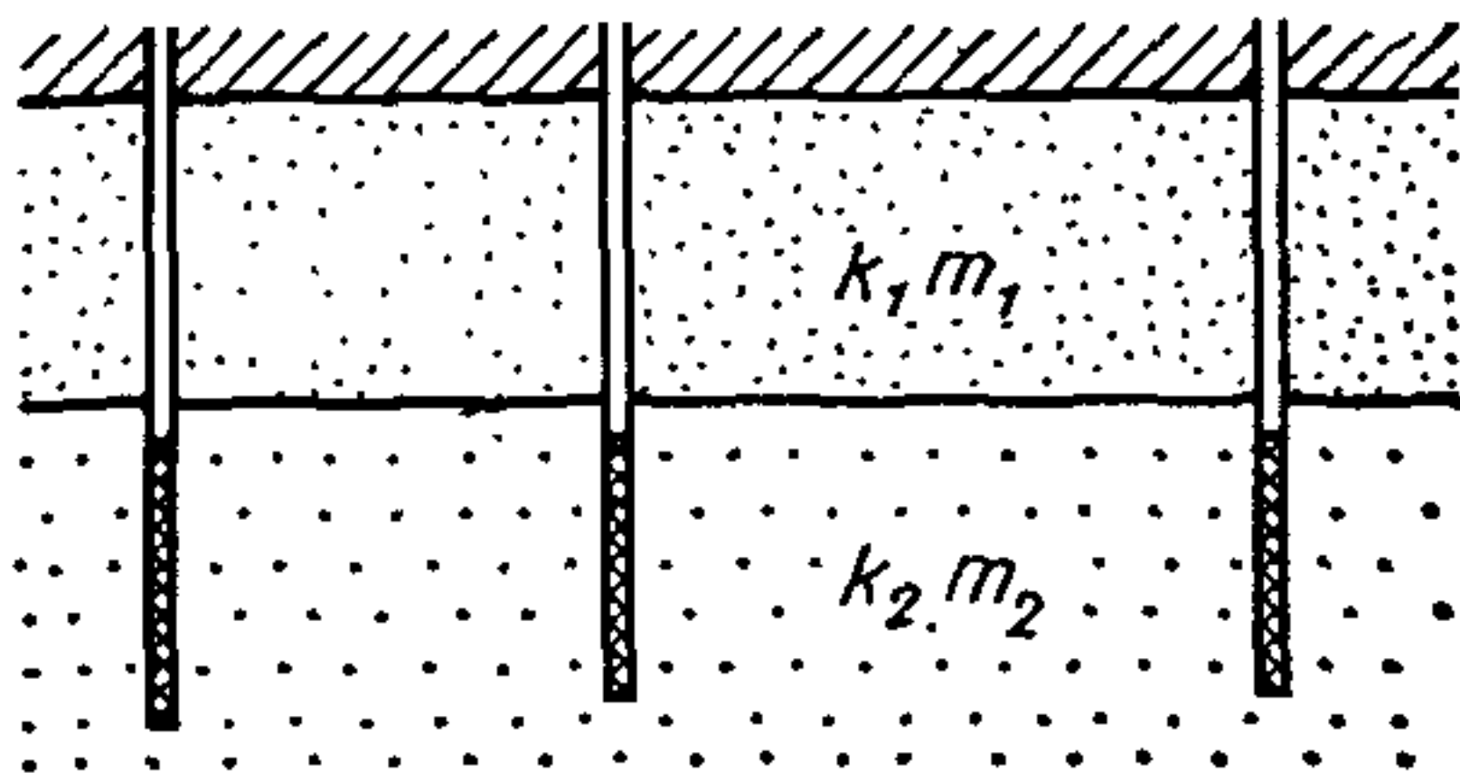
Рис. 8. Схема двухслойной толщи (пласт ограничен водупором или свободной поверхностью)
