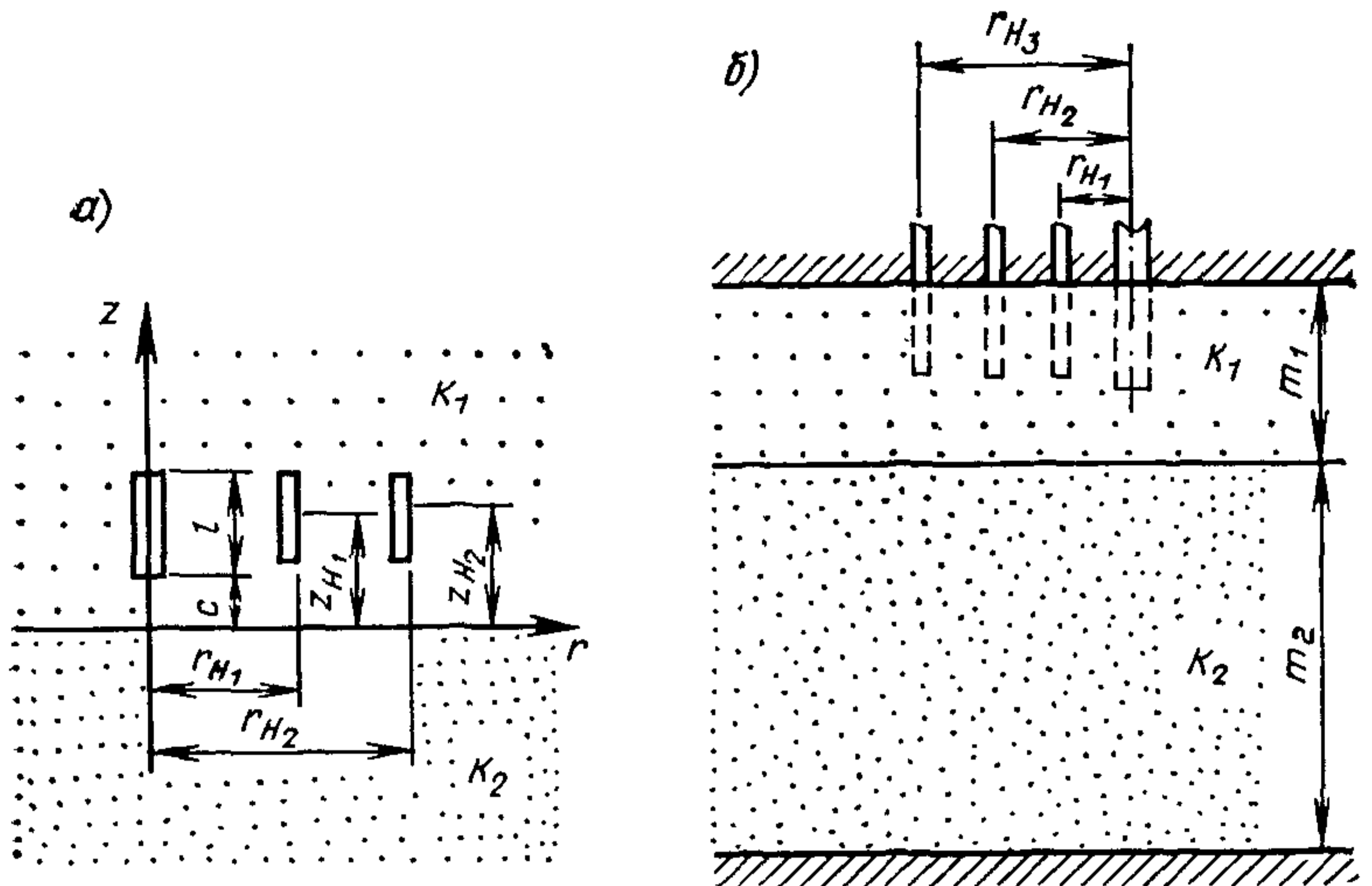
Рис. 25. Схема (разрез) опытного куста скважин в двухслойной толще пород
