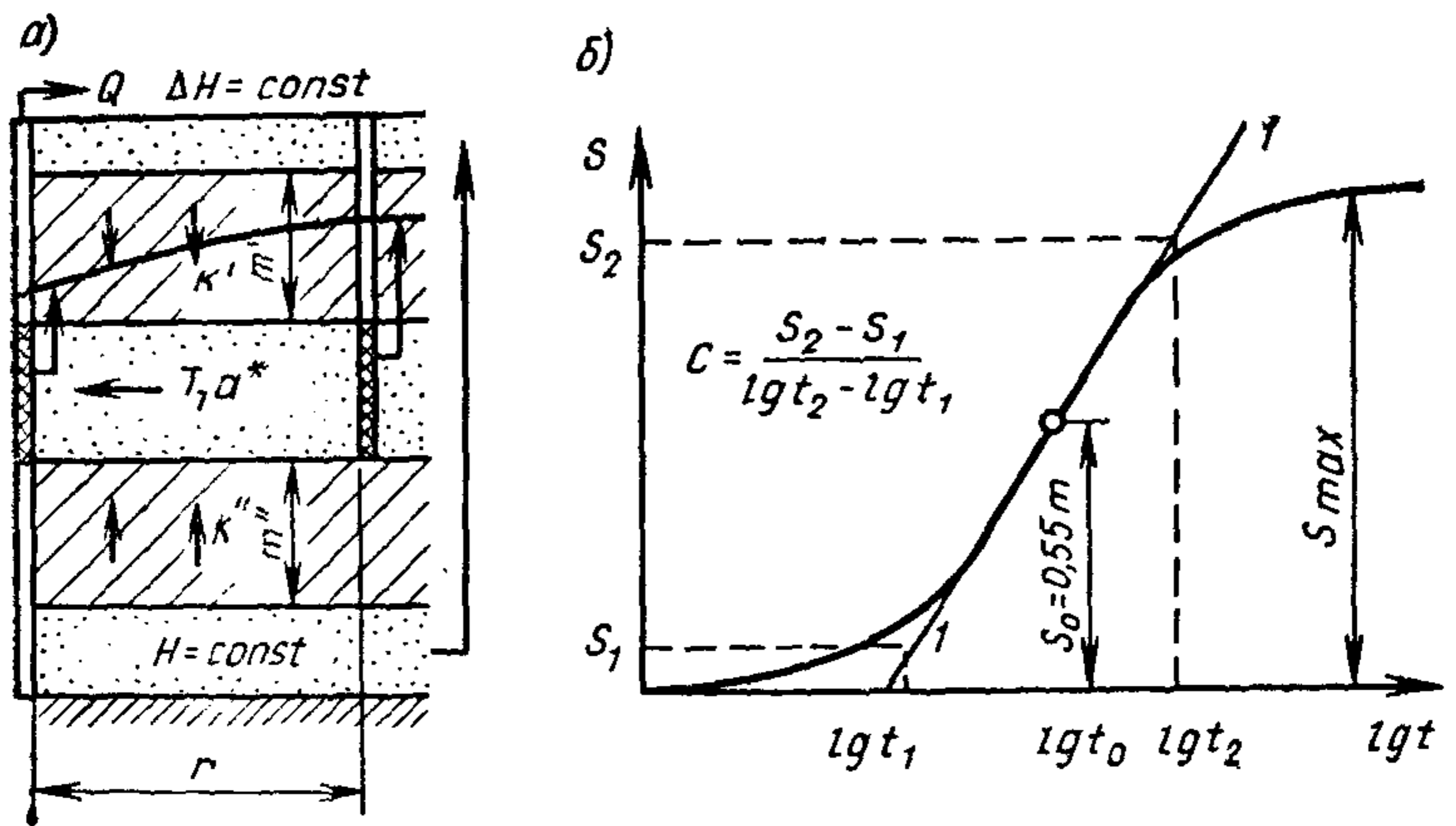
Рис. 26. Откачка при перетекании из водоносных горизонтов с постоянным напором
