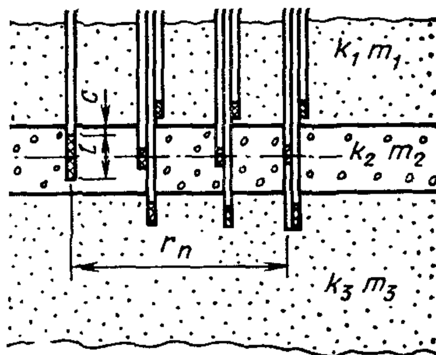
Рис. 10. Схема трехслойной толщи (крайние слои ограниченные)
