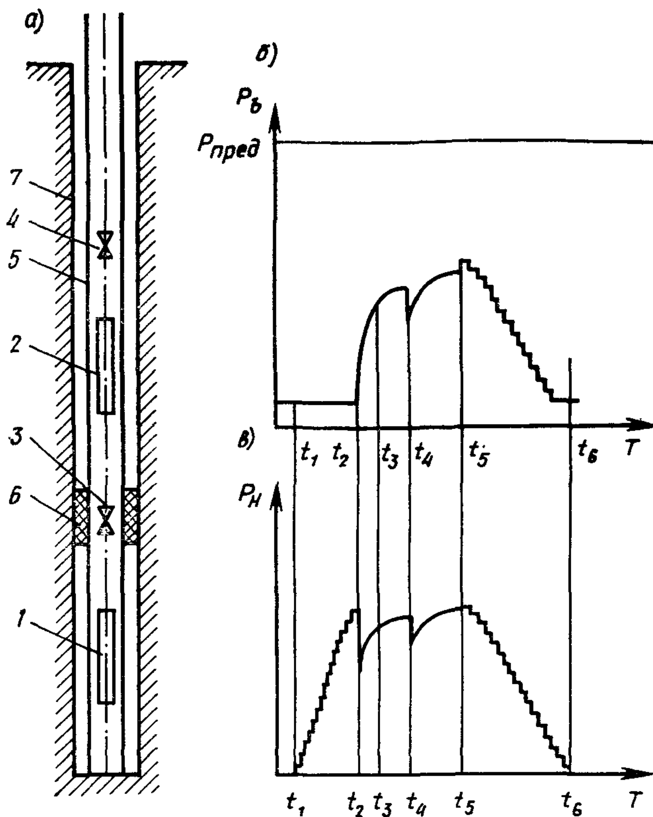
Рис. 1. Схема установки испытательного инструмента (а) и диаграммы верхнего (б) и нижнего (в) манометров
