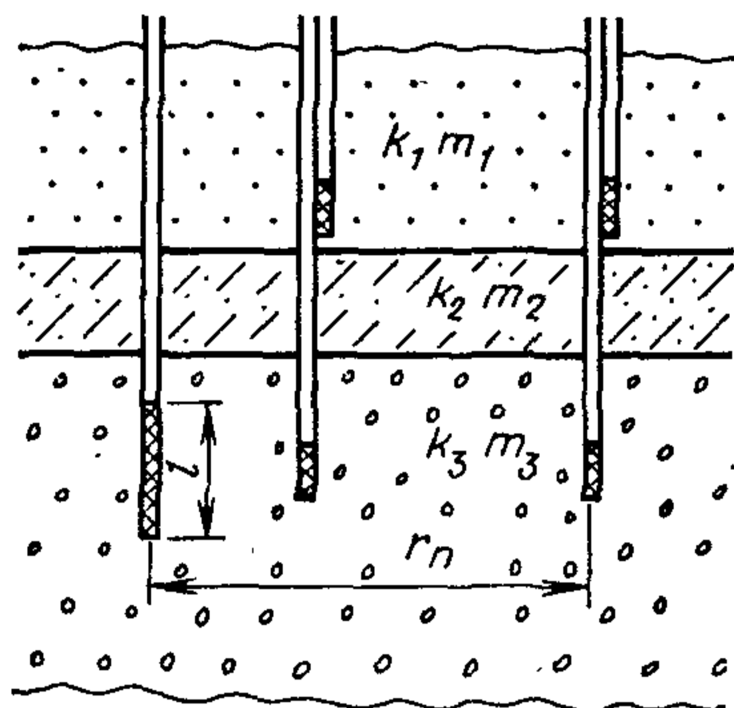
Рис. 9. Схема трехслойной толщи (крайние слои полуограниченные)
