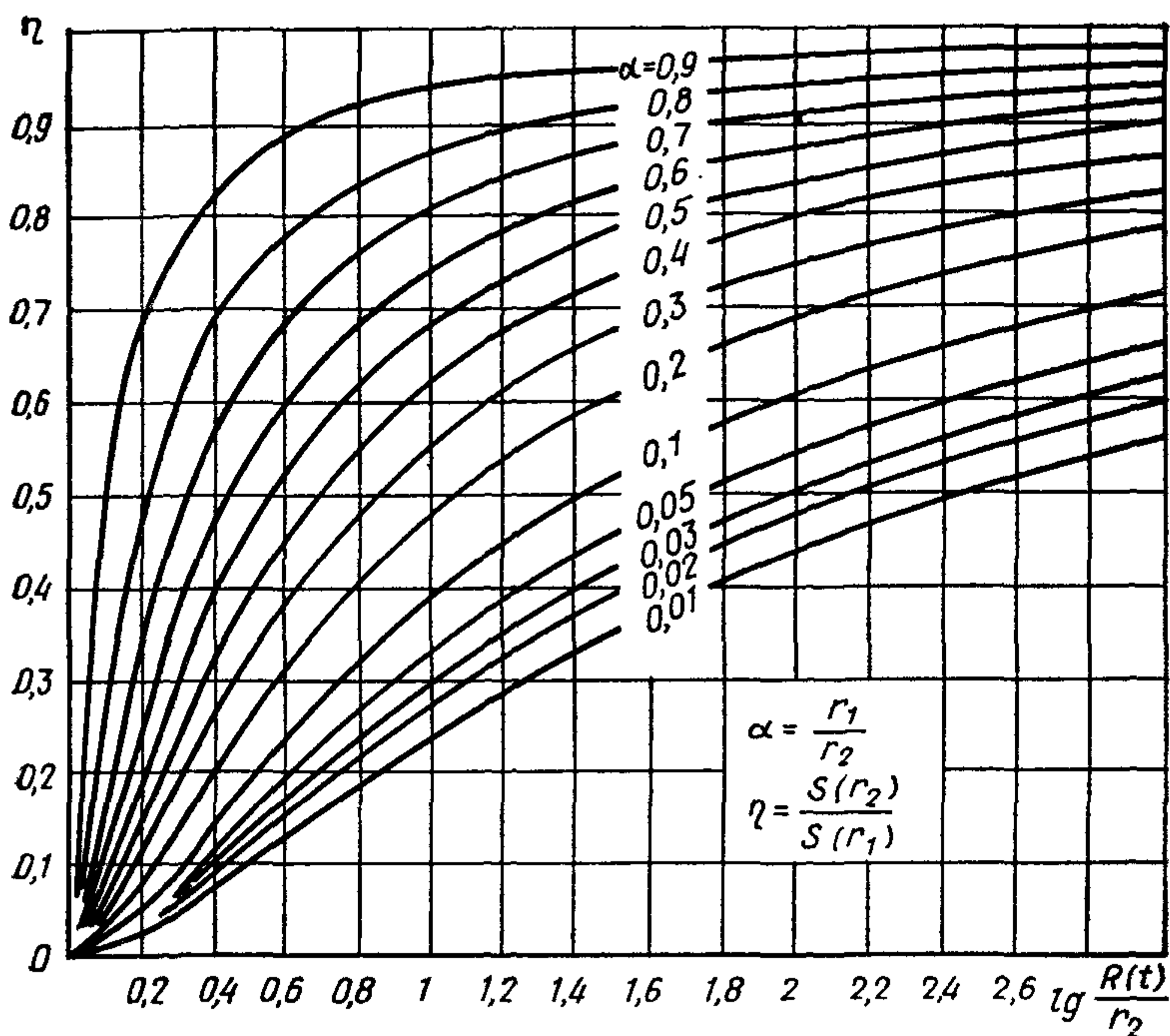
Рис. 28. Вспомогательный график для определения R(t)
