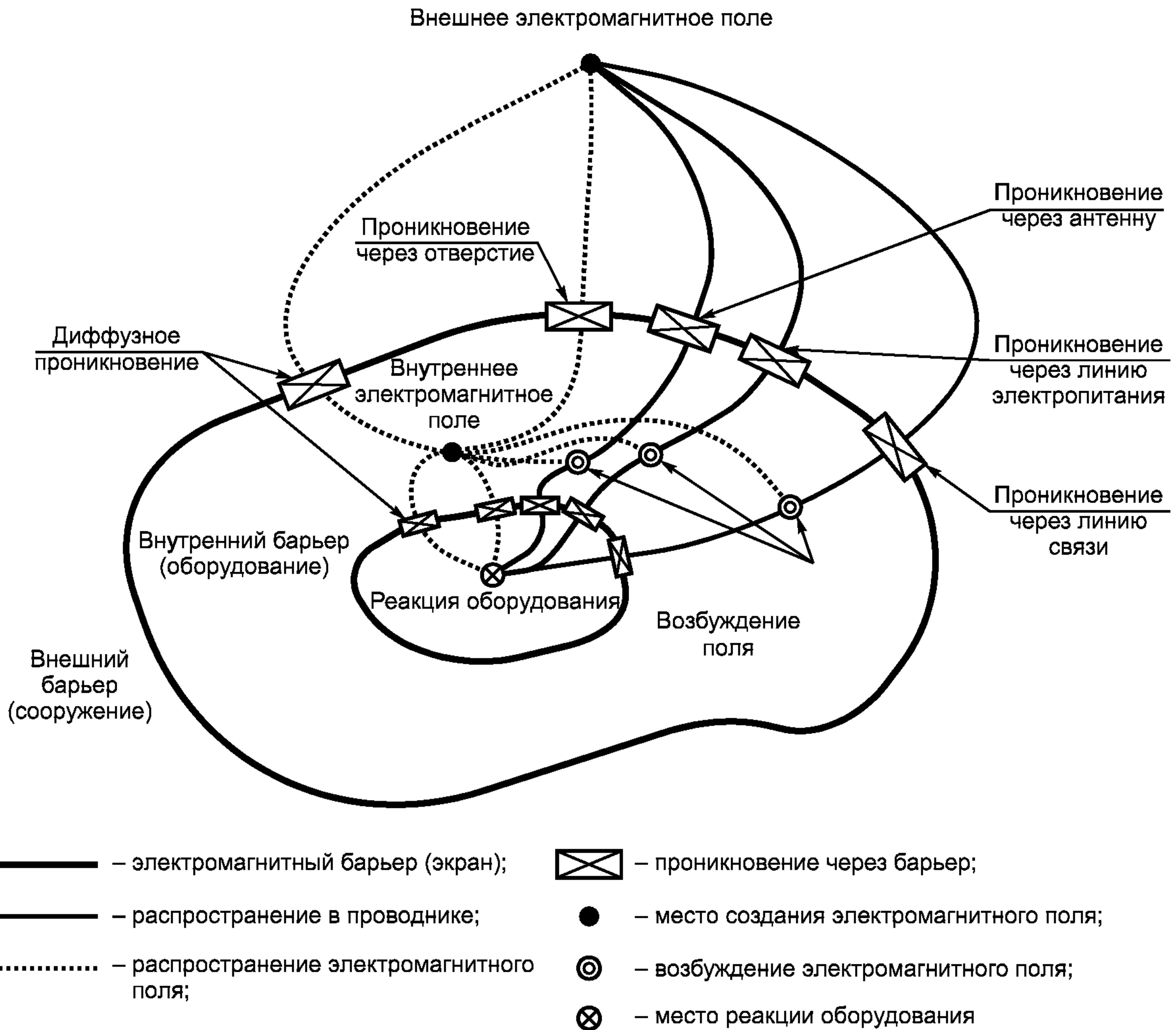
Рисунок 6 — Топологическая схема простой системы, представленной на рисунке 5
