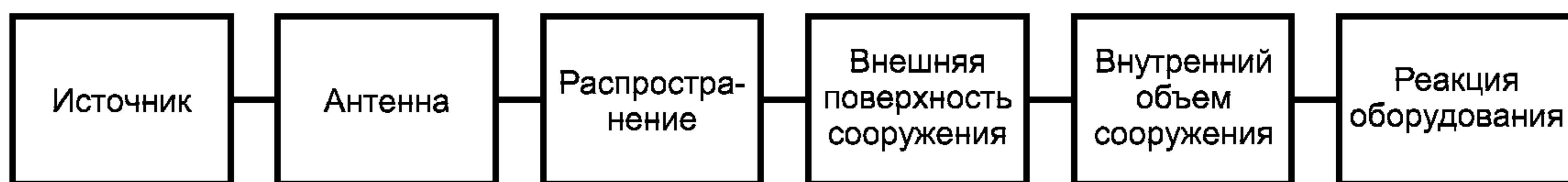
Рисунок 7 — Обобщенная диаграмма последовательности взаимодействия для системы, представленной на рисунке 5
