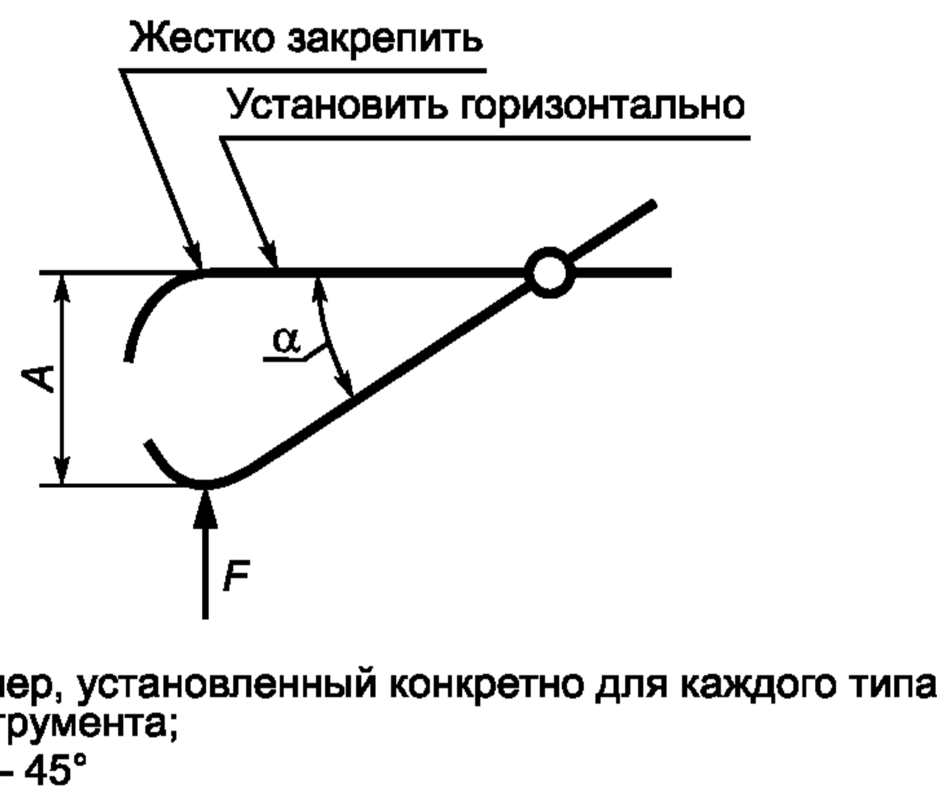
Рисунок 1 — Положение инструмента перед измерением и направление действия усилия свободного хода
