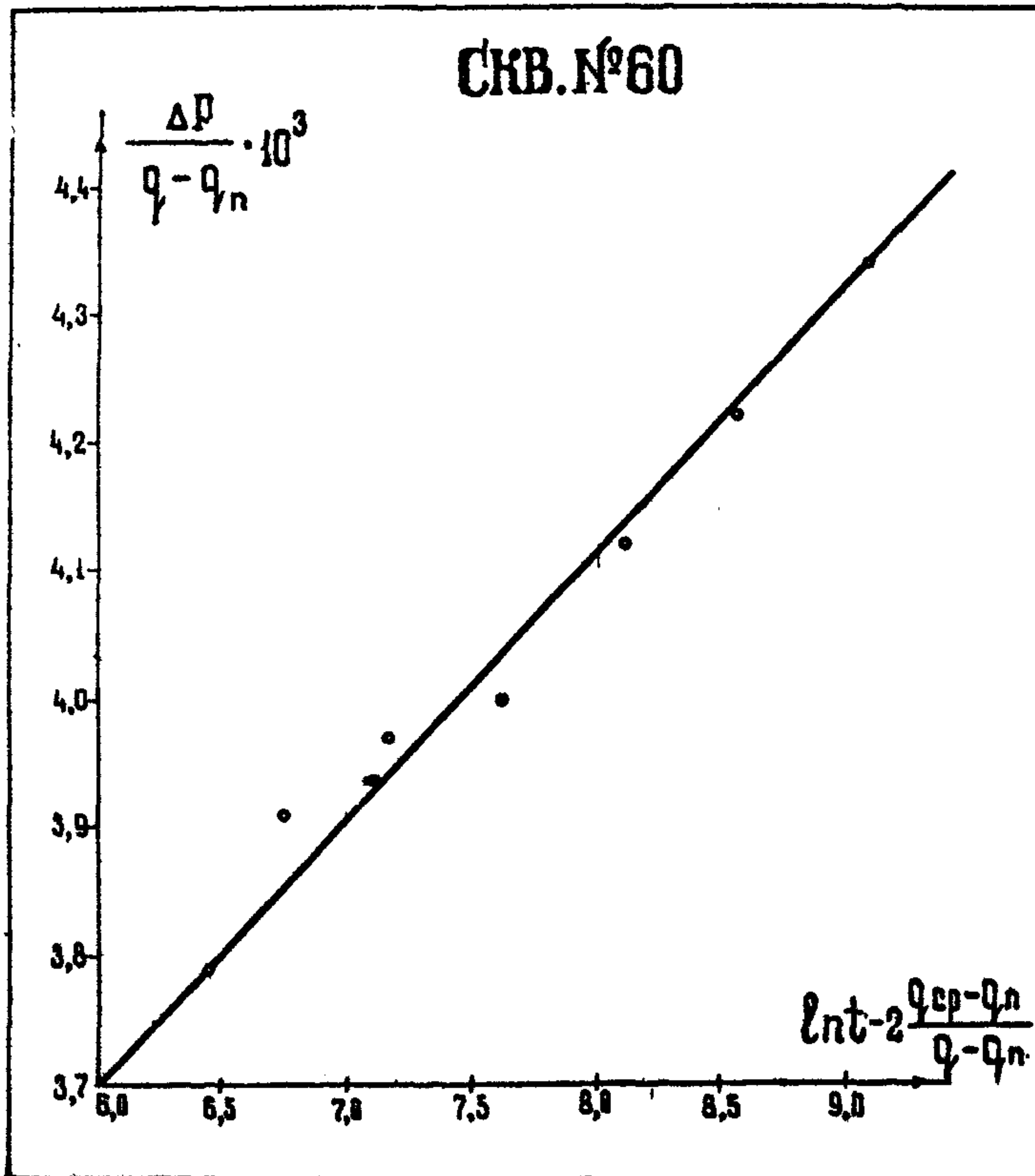
Рис. 11 К примеру обработки кривой восстановления давления с учетом притока методом В.Н.Щелкачева- А.С.Кундина.
