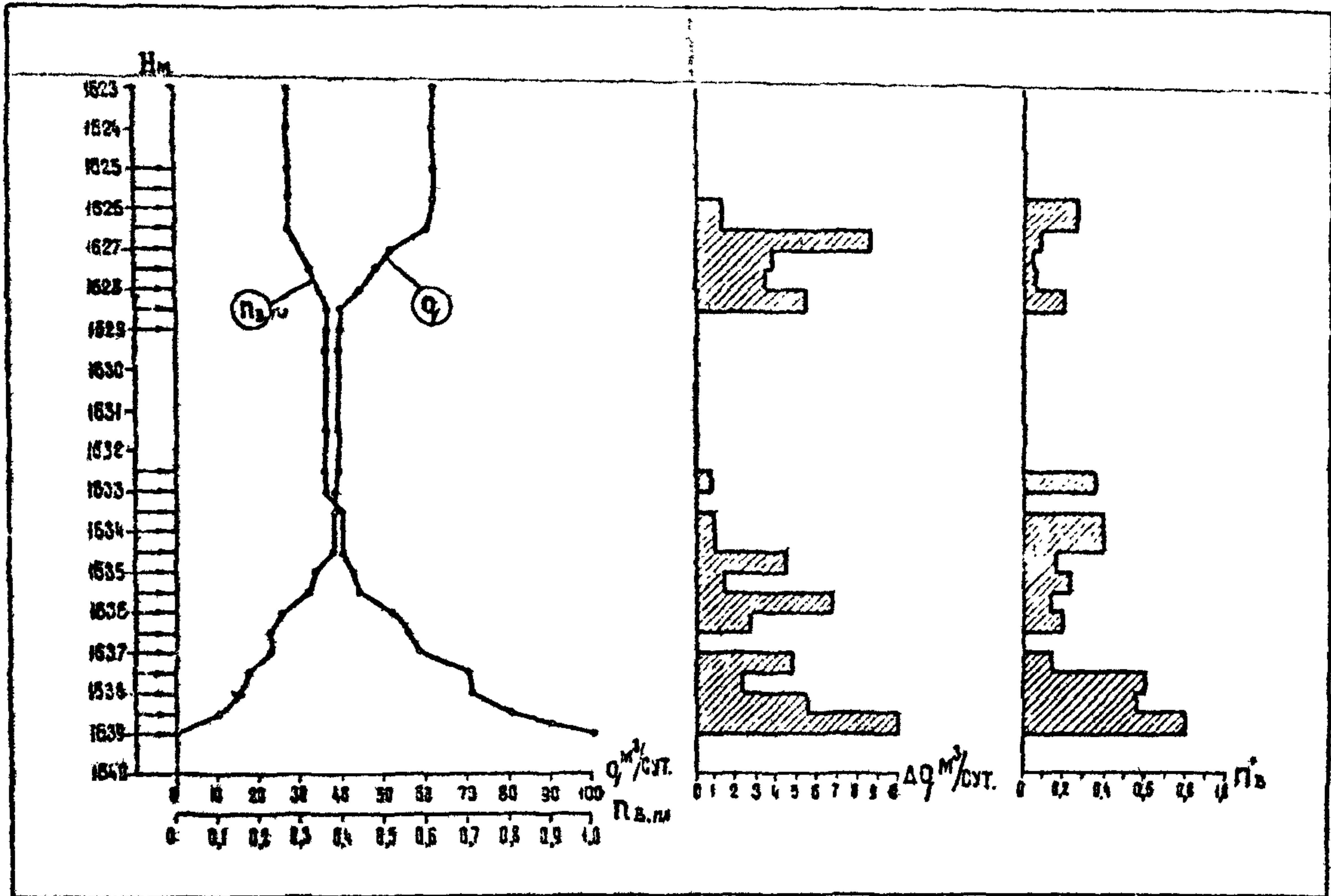
Рис. 1 Характерные интегральные и дифференциальные профили притока по дебиту и обводненности.
