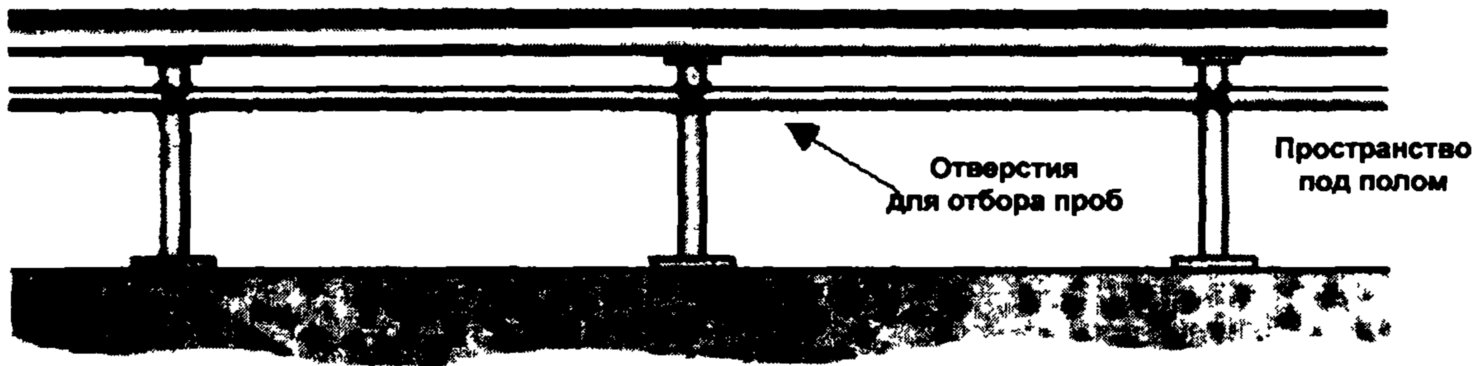
Рис. 9. Отбор проб из пространства под полом
