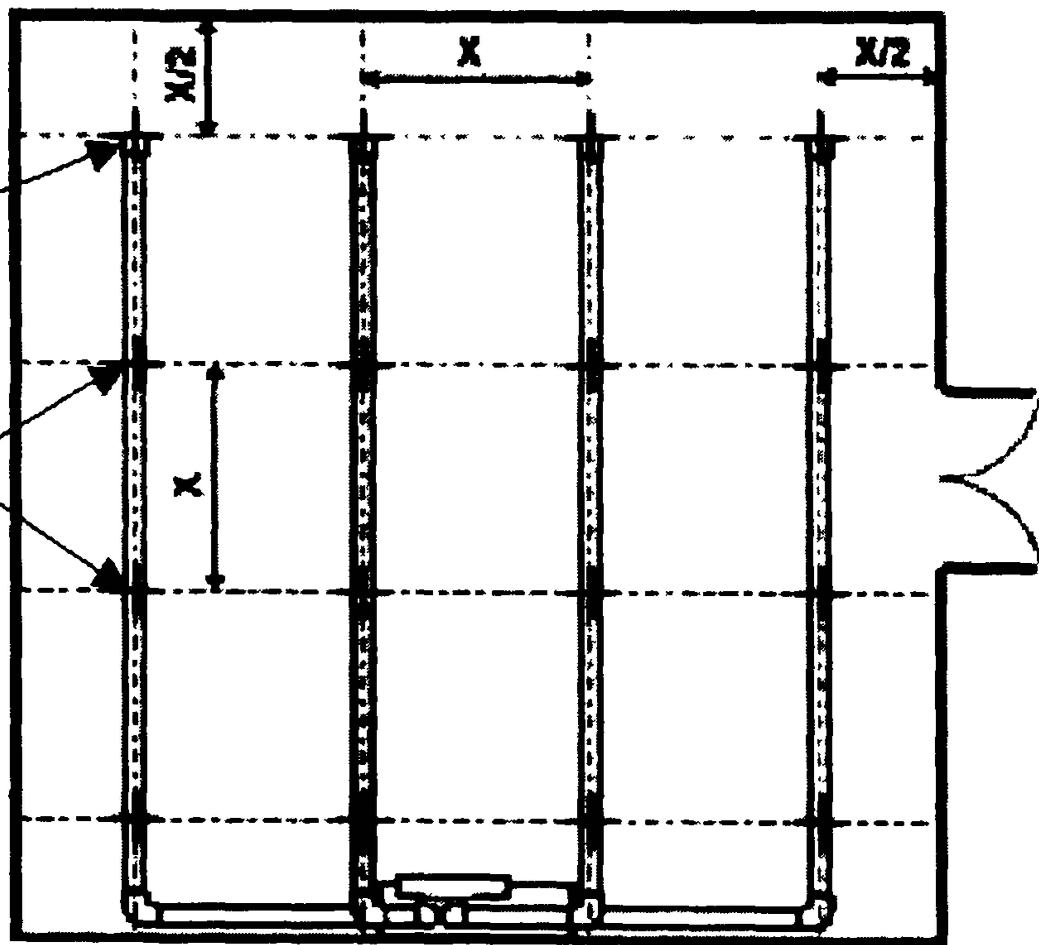
Рис. 2. Сеточная схема расположения точек забора проб воздуха
