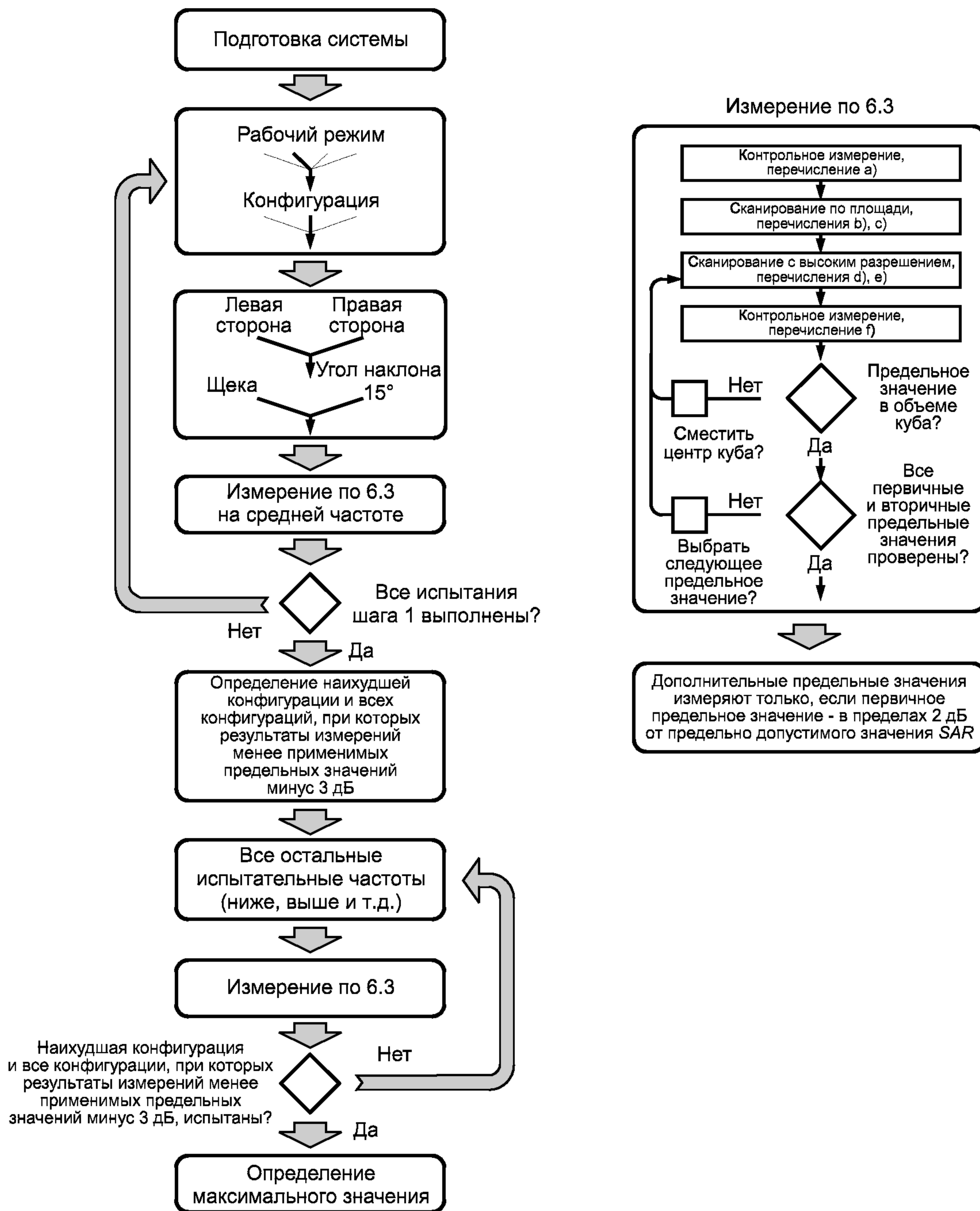
Рисунок 8 — Блок-схема процесса испытаний
