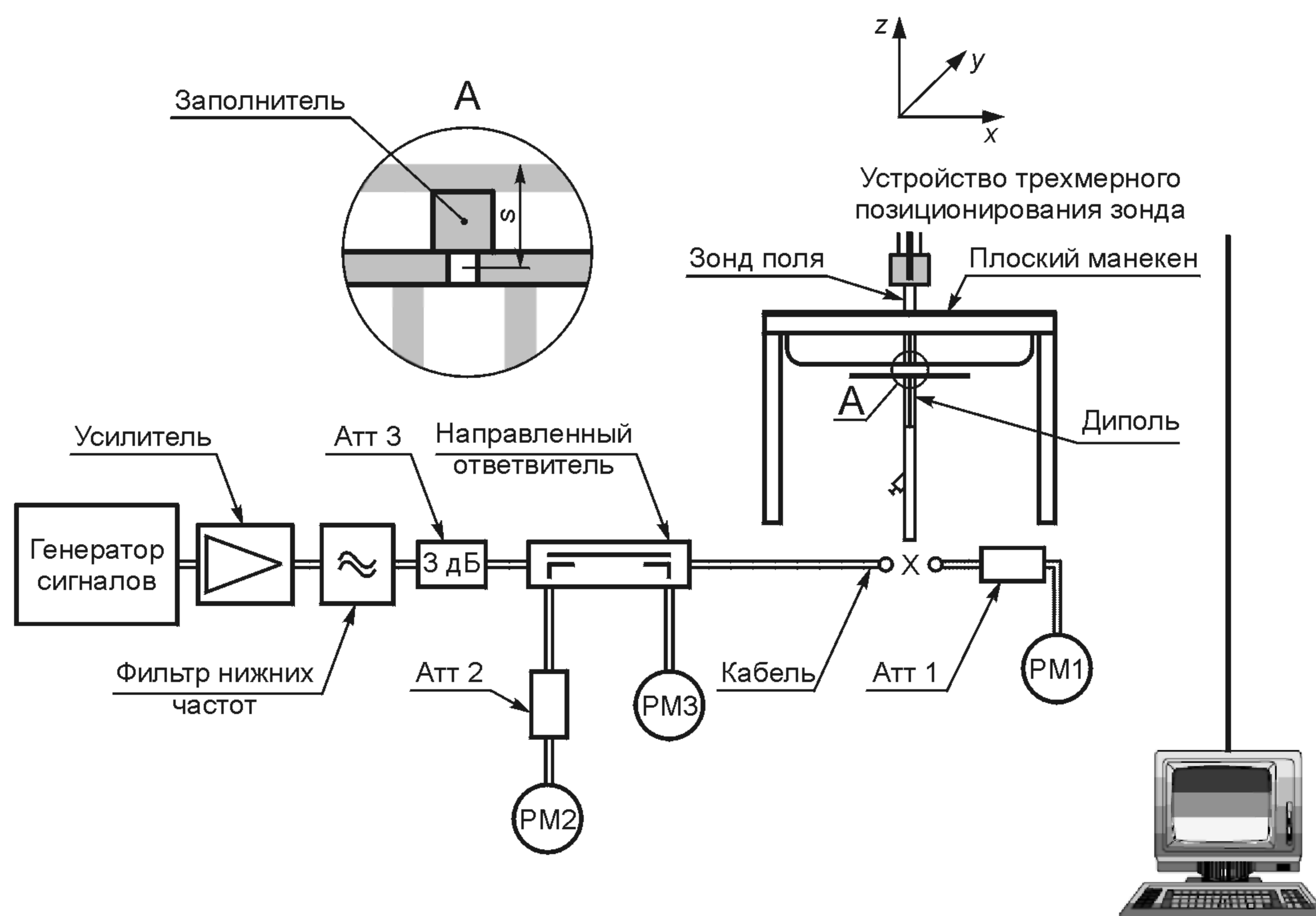
Рисунок D.1 — Установка для проверки системы
