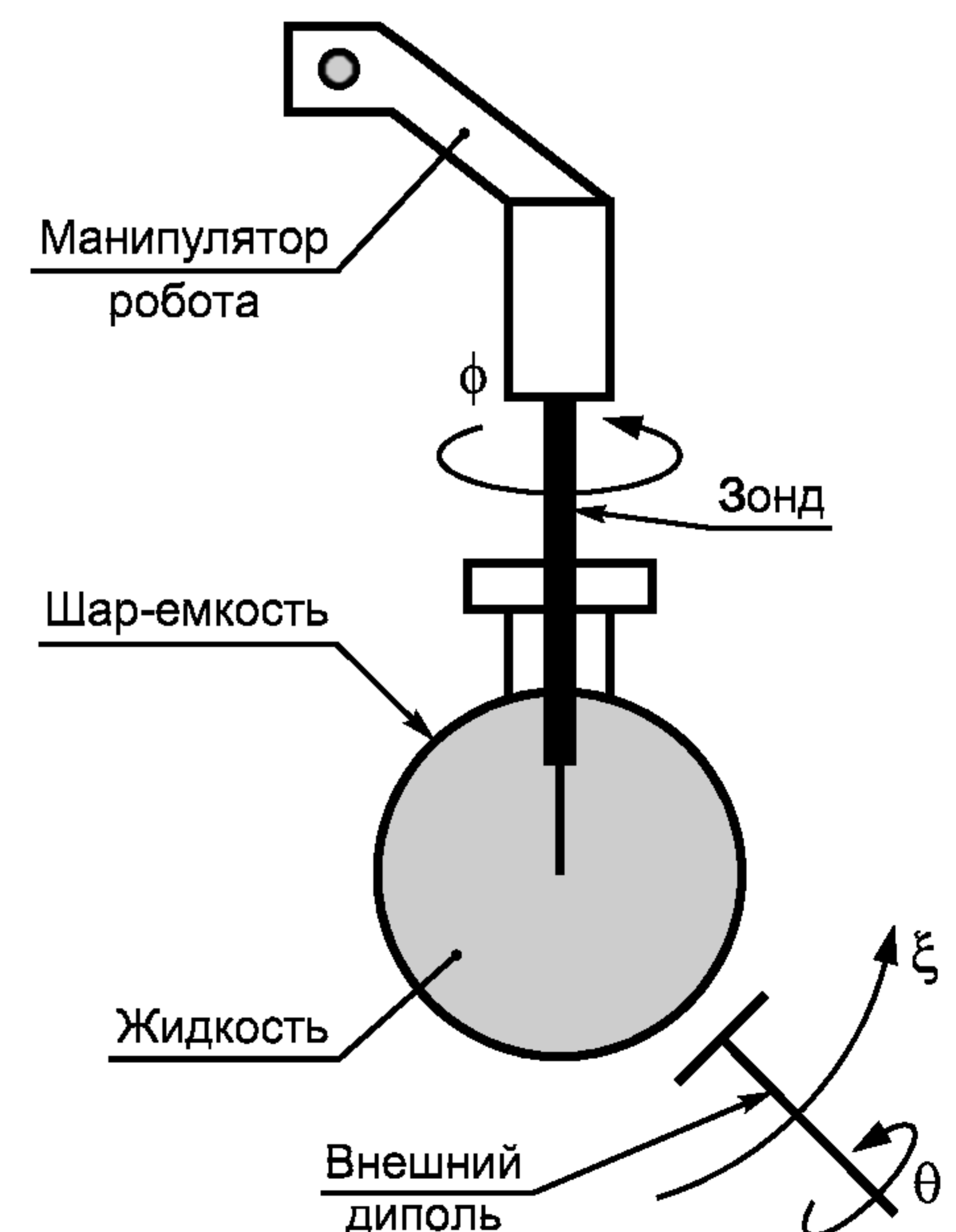
Рисунок В.5 — Экспериментальная установка для оценки полусферической изотропии [11]
