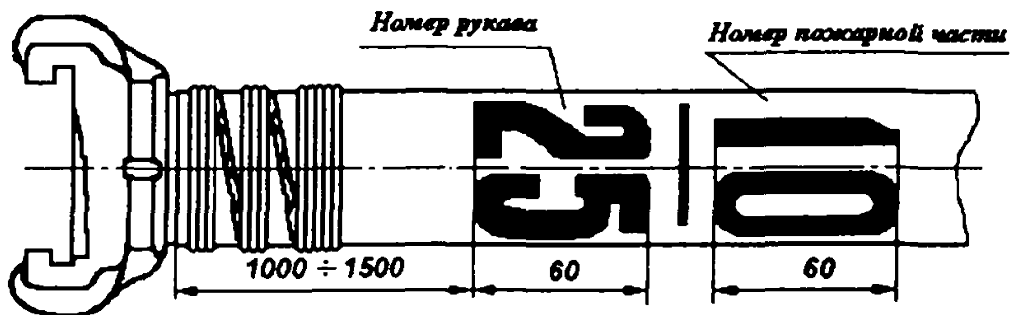
Рис. 3. Дополнительная маркировка рукава в пожарной части
