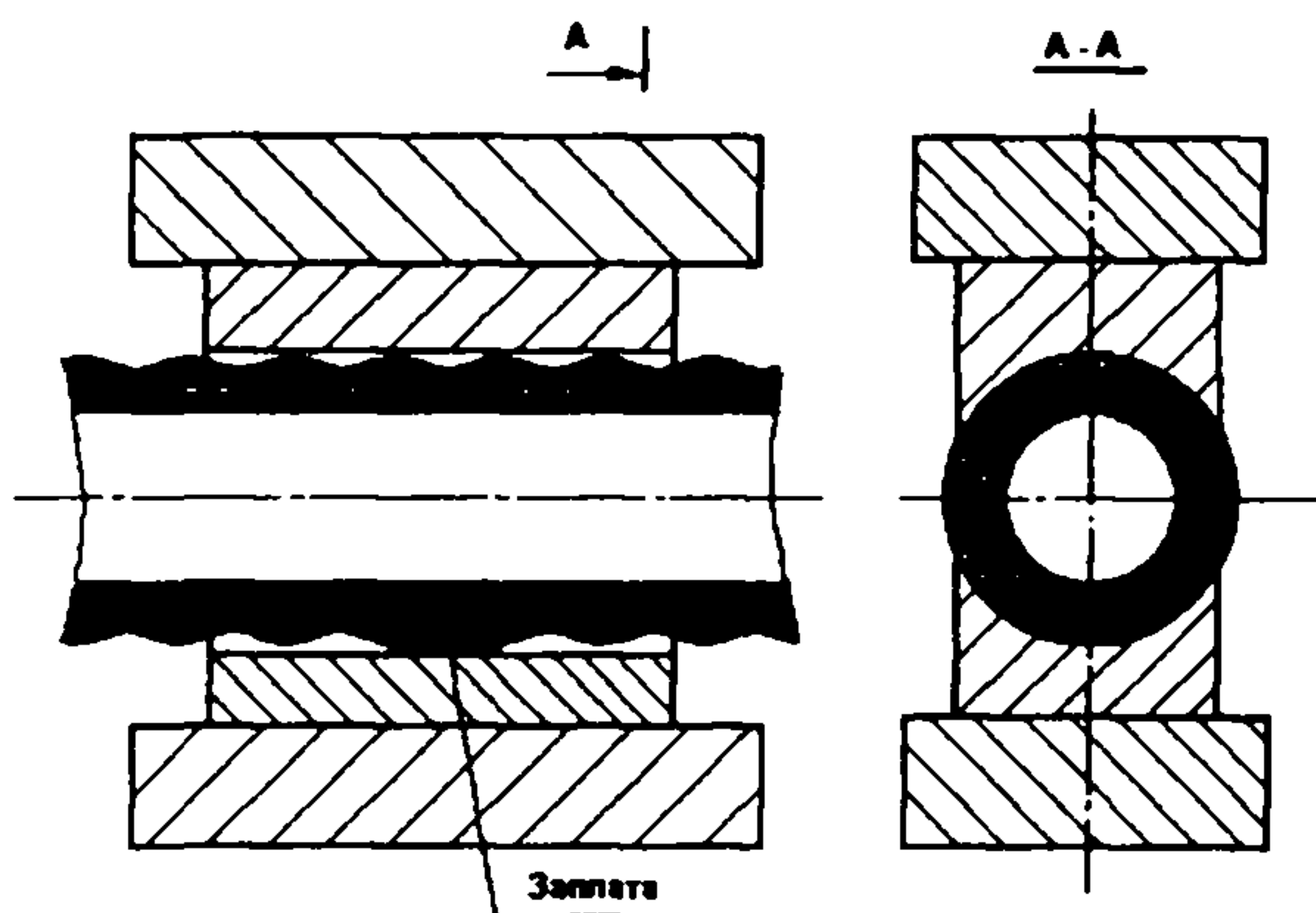
Рис. 6. Приспособление для ремонта посредством вулканизации
