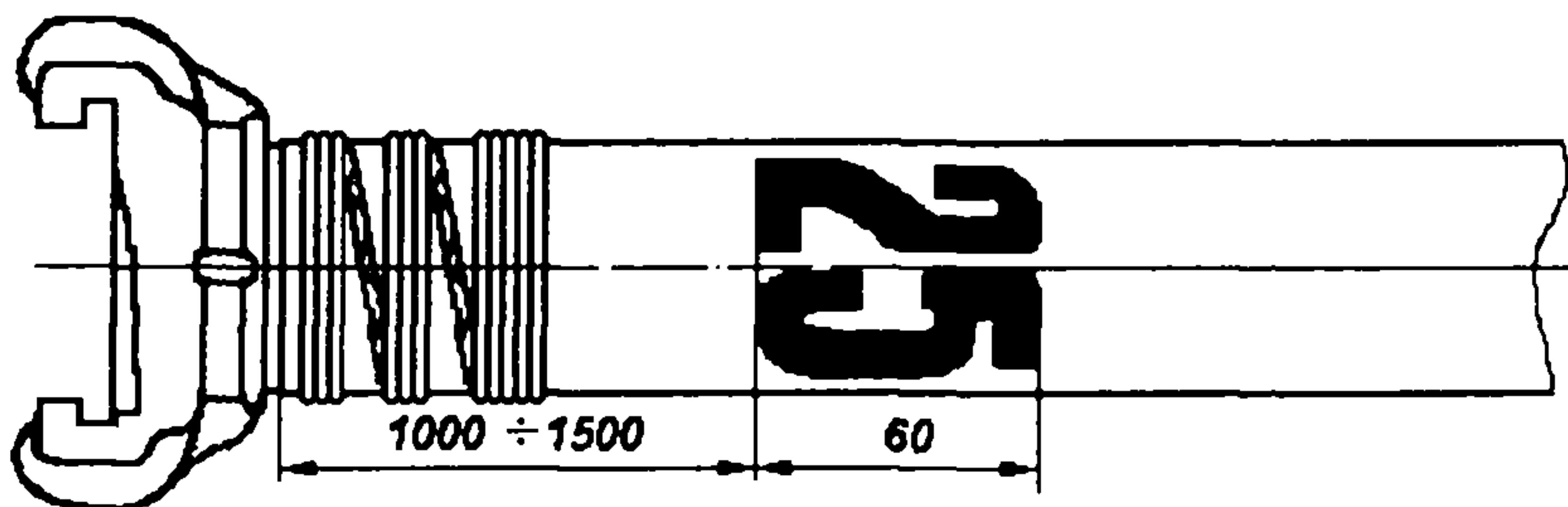
Рис. 4. Дополнительная маркировка рукава на рукавной базе
