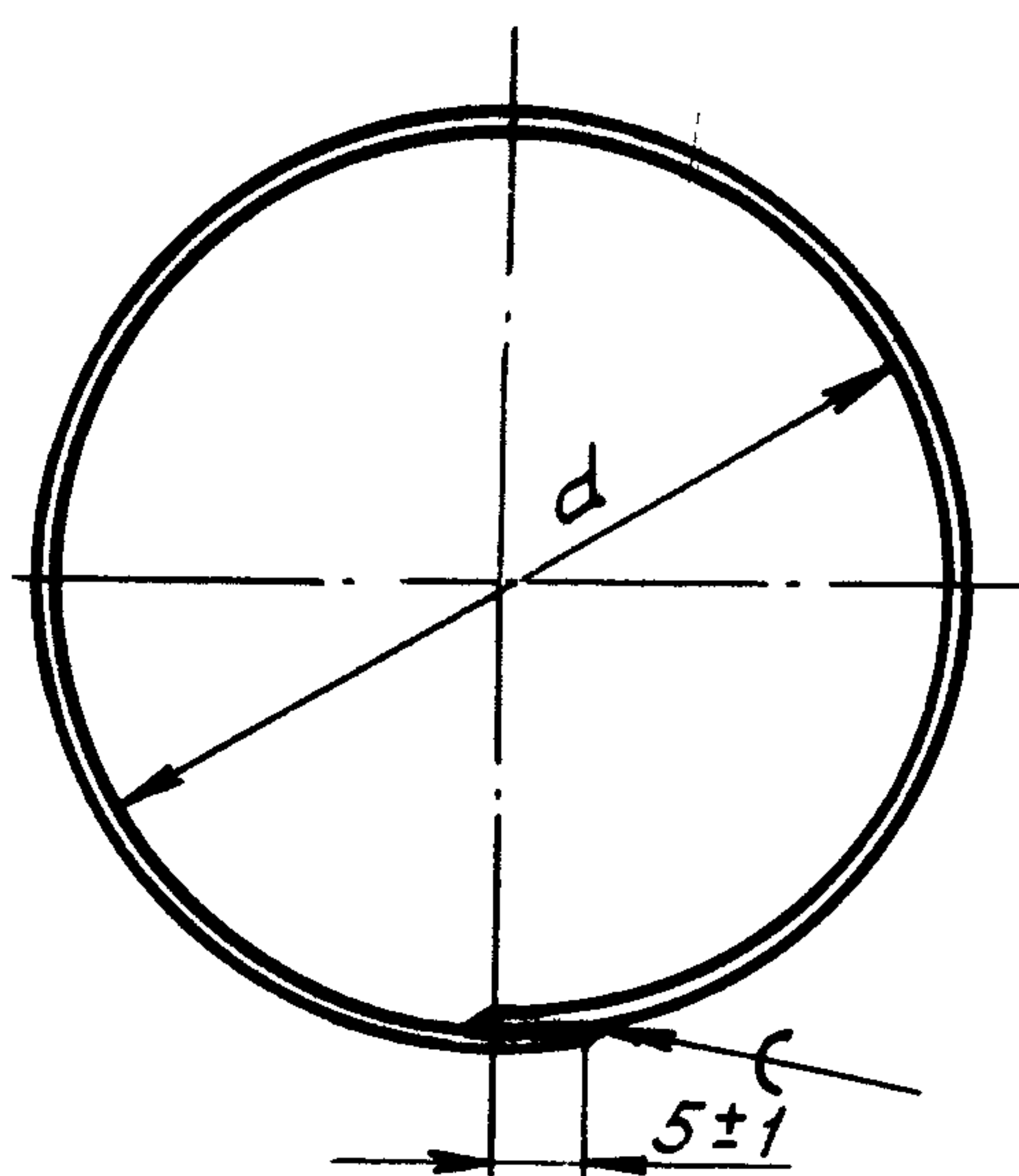
Размеры, мм
