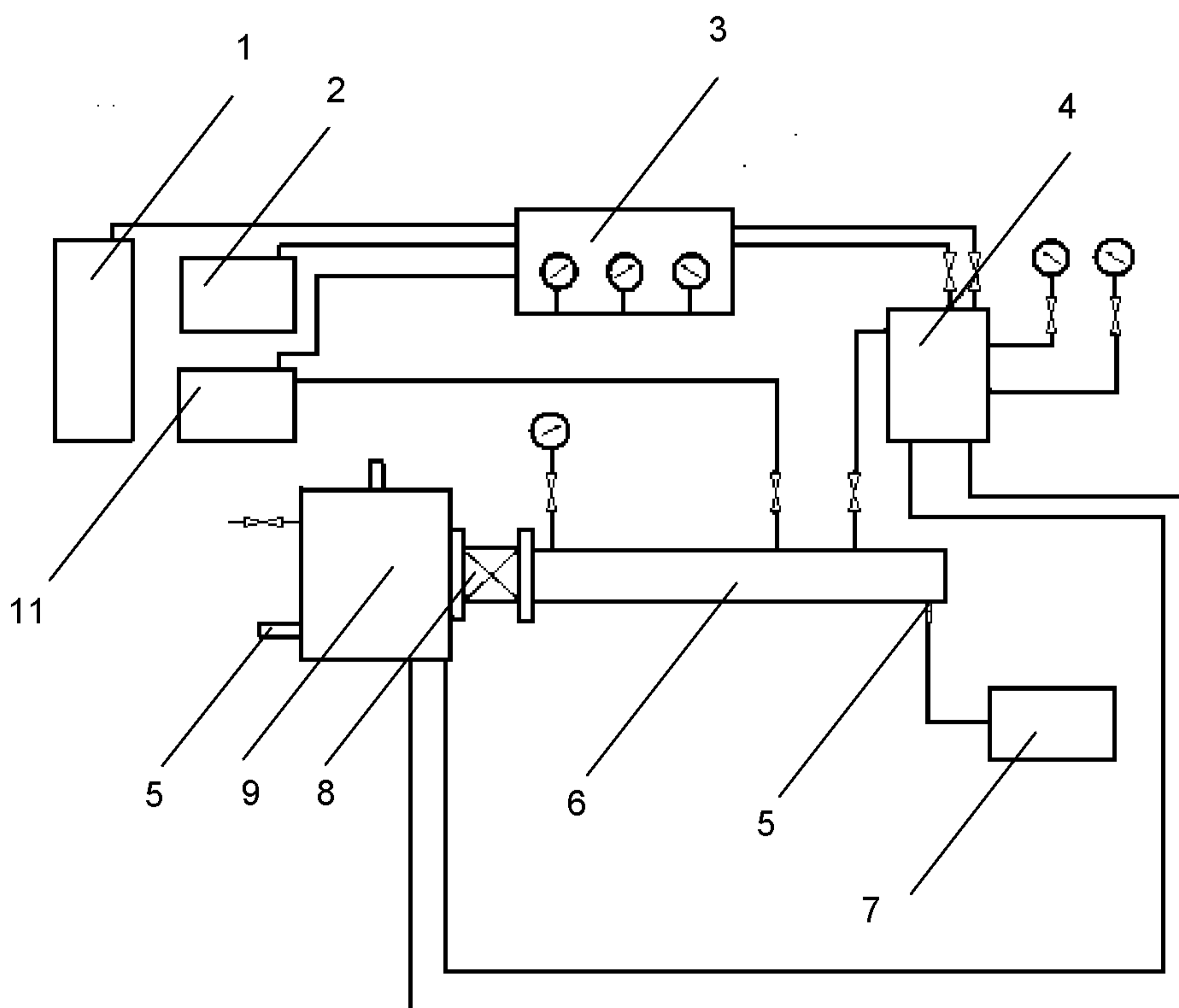
1 — баллон с горючим газом; 2 — компрессор; 3 — газовый пульт; 4 — смеситель; 5 — свечи зажигания; 6 — реакционная труба; 7 — блок зажигания; 8 — пламегасящий элемент огнепреградителя; 9 — контрольная емкость; 10 — датчик давления; 11 — вакуумный насос
