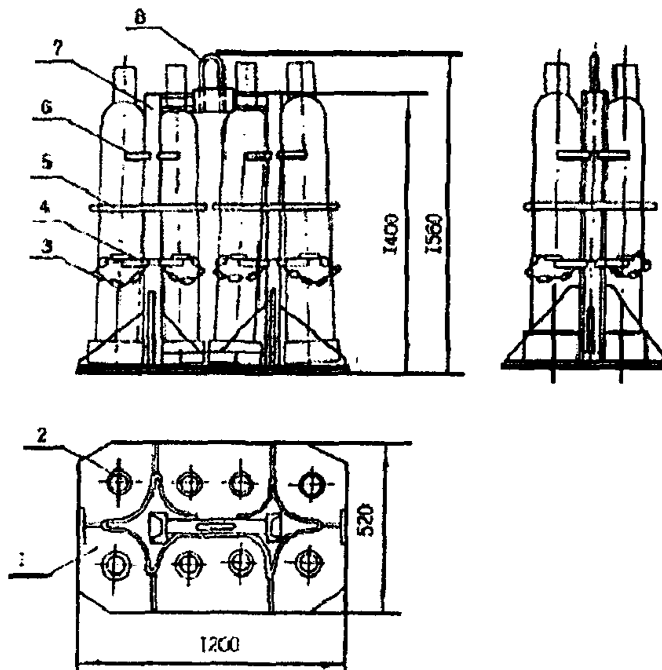
Рис.3. Контейнер на 8 баллонов вместимостью 40 литров
