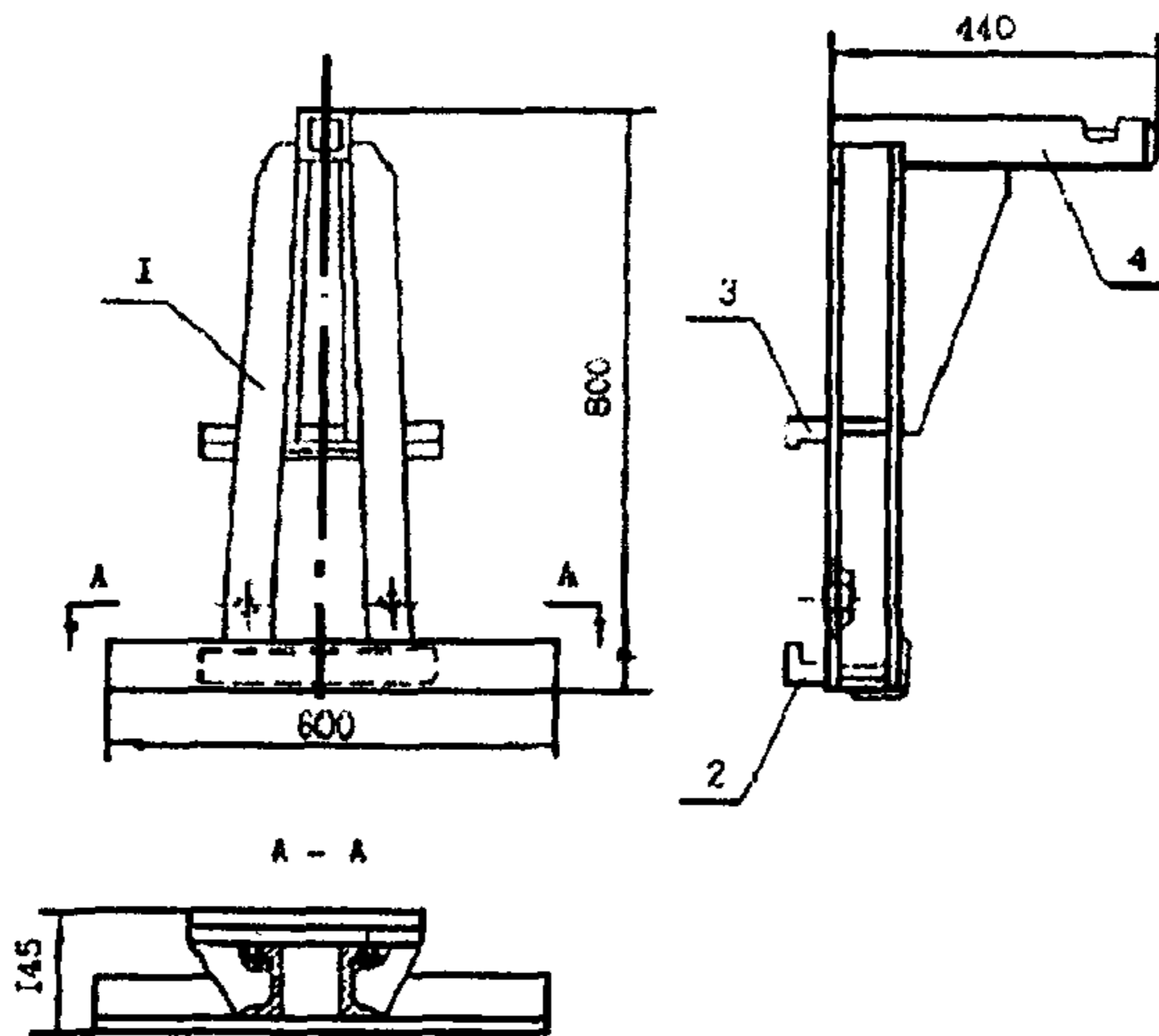
Рис. 6. Стержневой захват на электропогрузчик для транспортировки контейнеров
