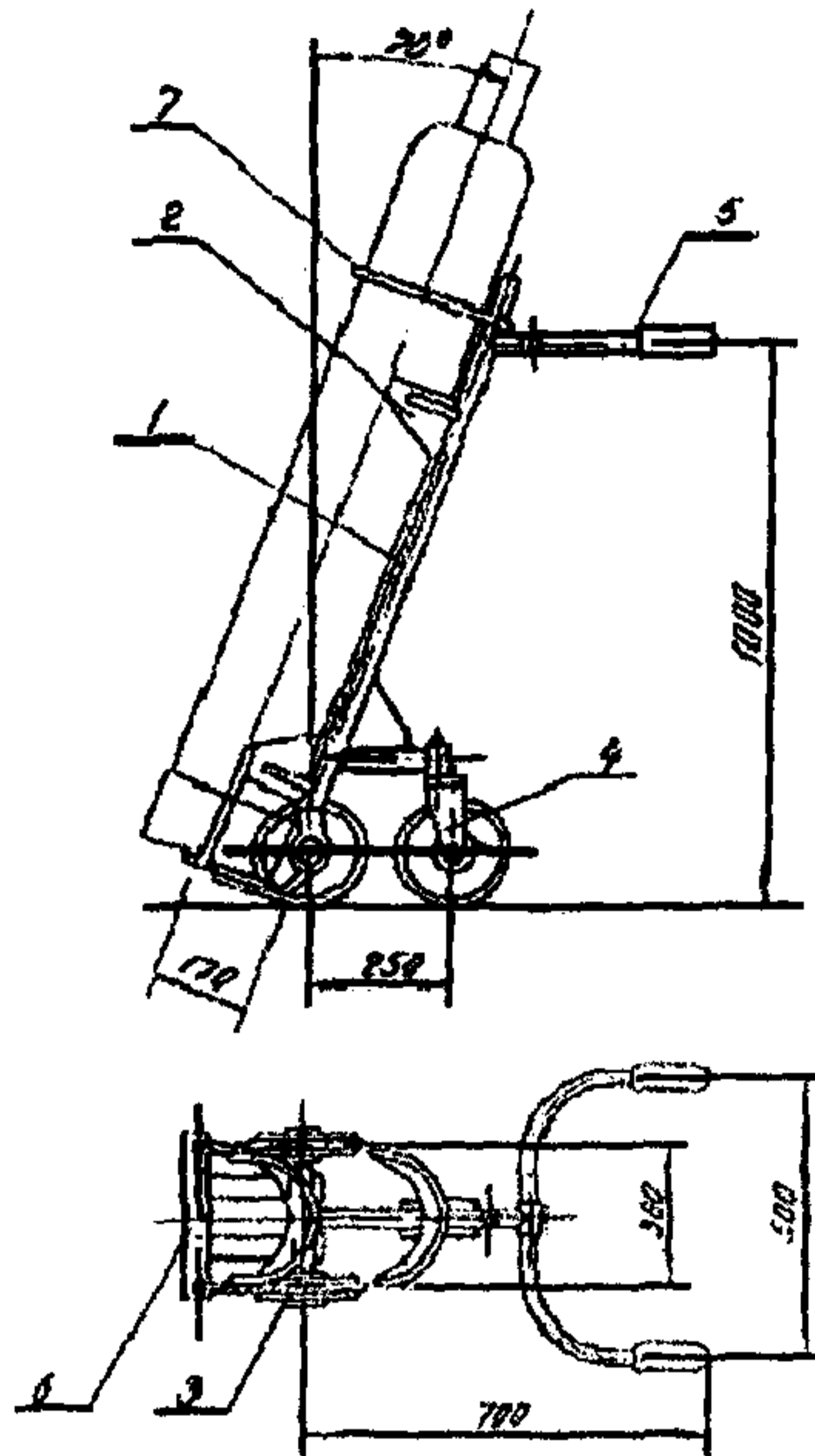
Рис.8. Тележка
