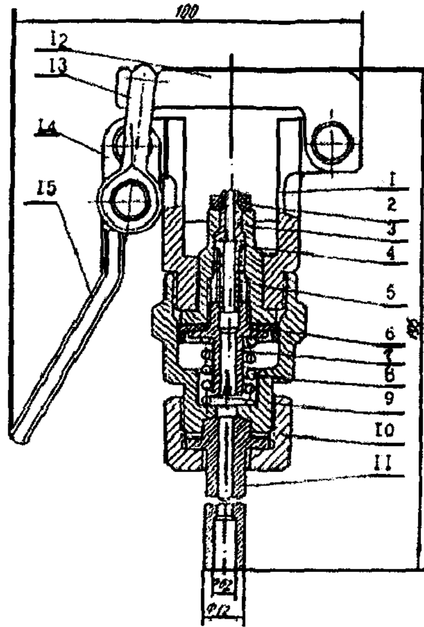
Рис.7. Зажим
