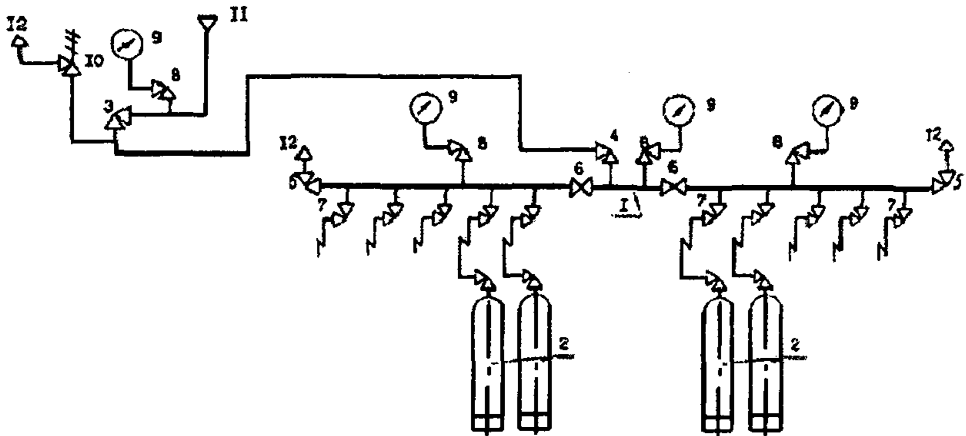
Рис.2. Типовая схема наполнения одиночных кислородных баллонов
