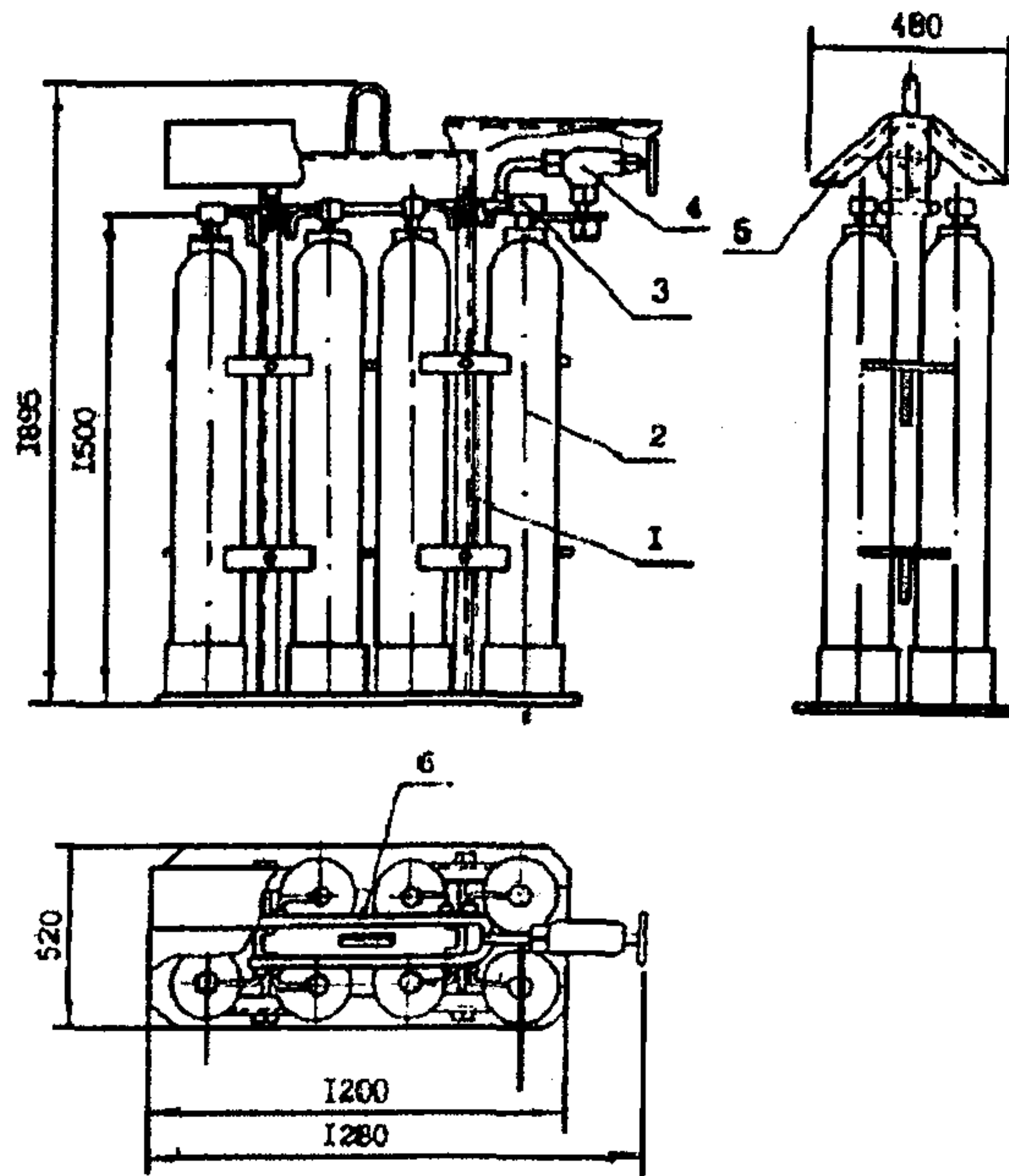
Рис.4. Блок баллонов
