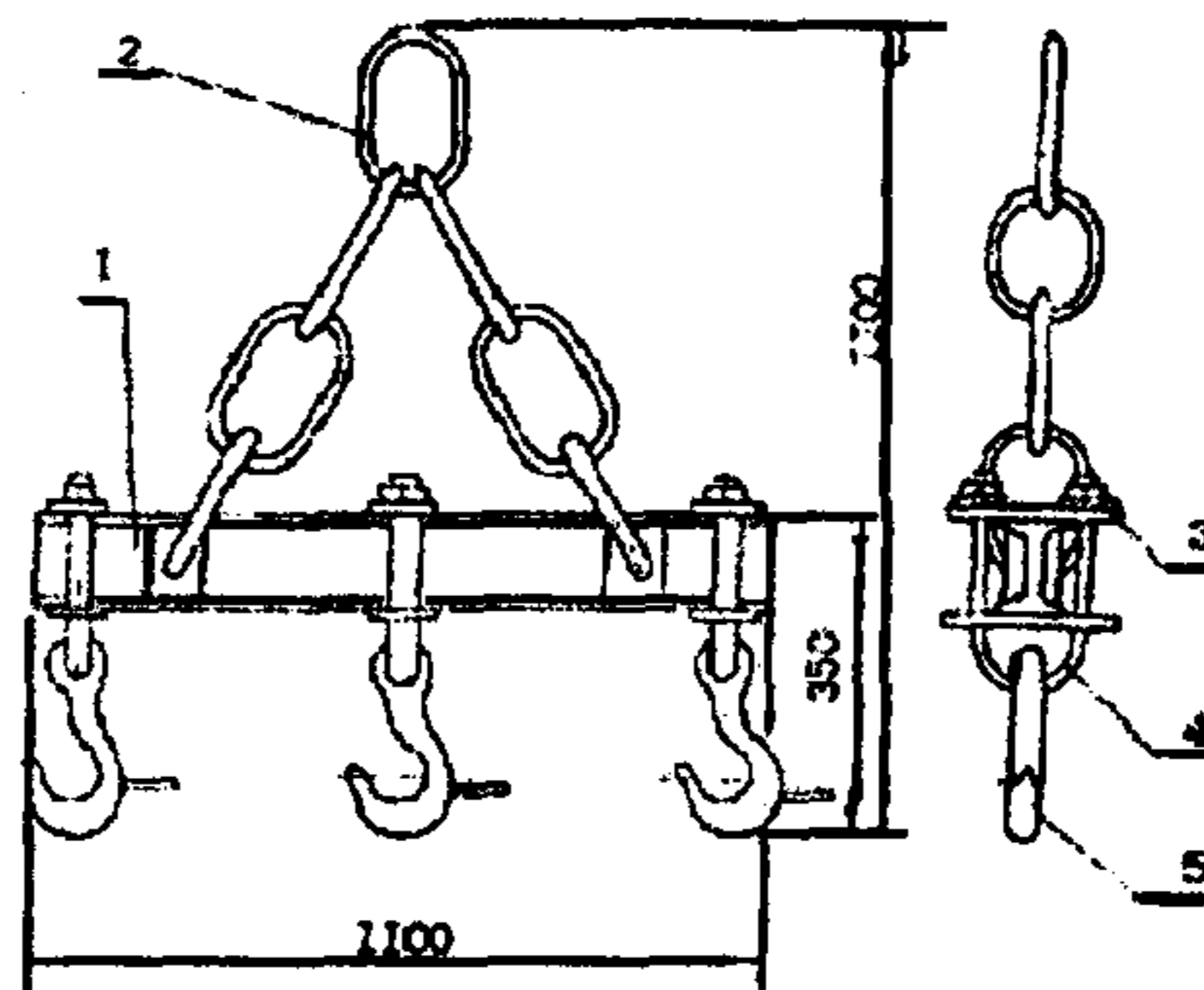
Рис.5. Траверса для подъема контейнеров
