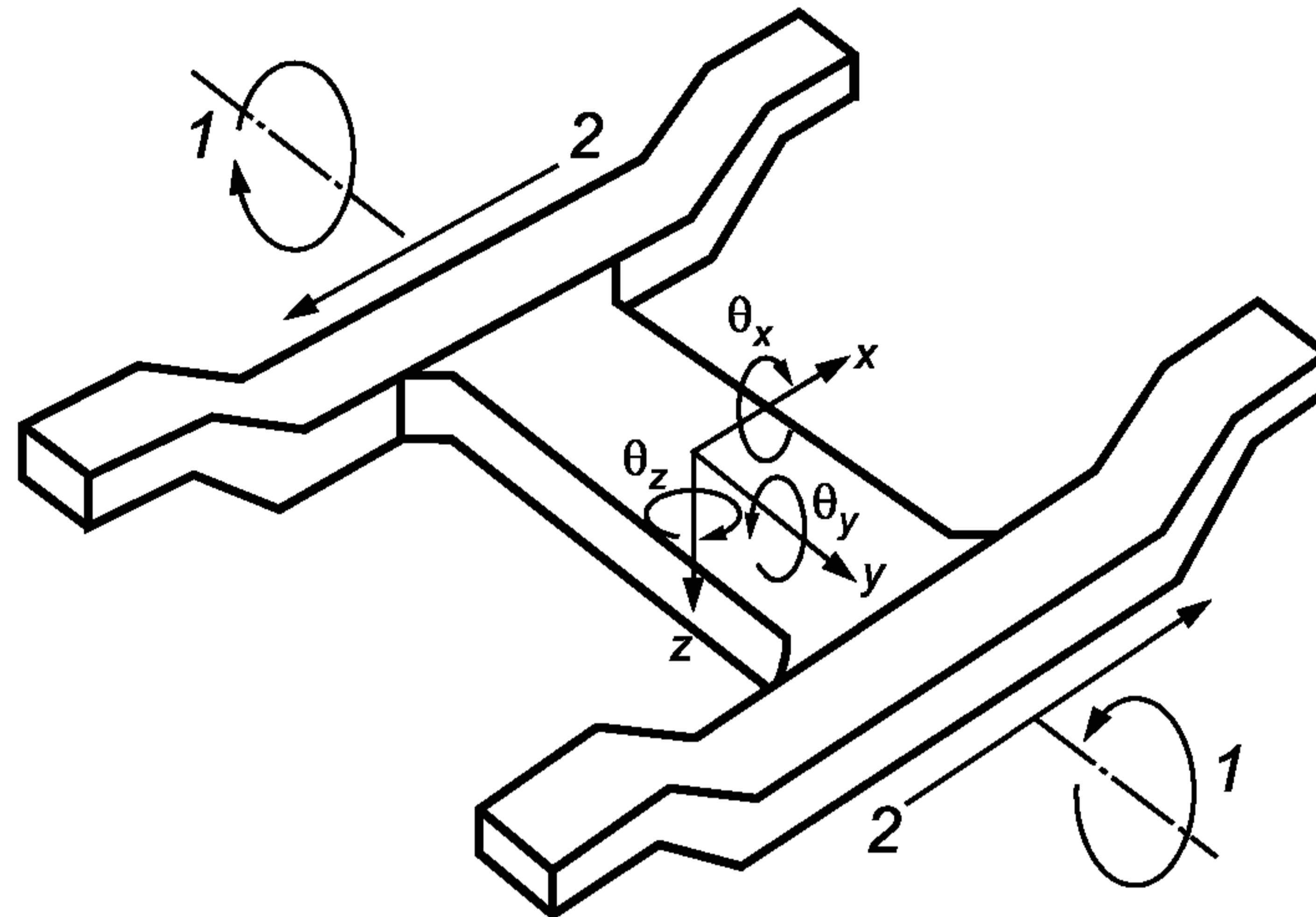
1 — скручивание; 2 — забегание боковин (виляние)
