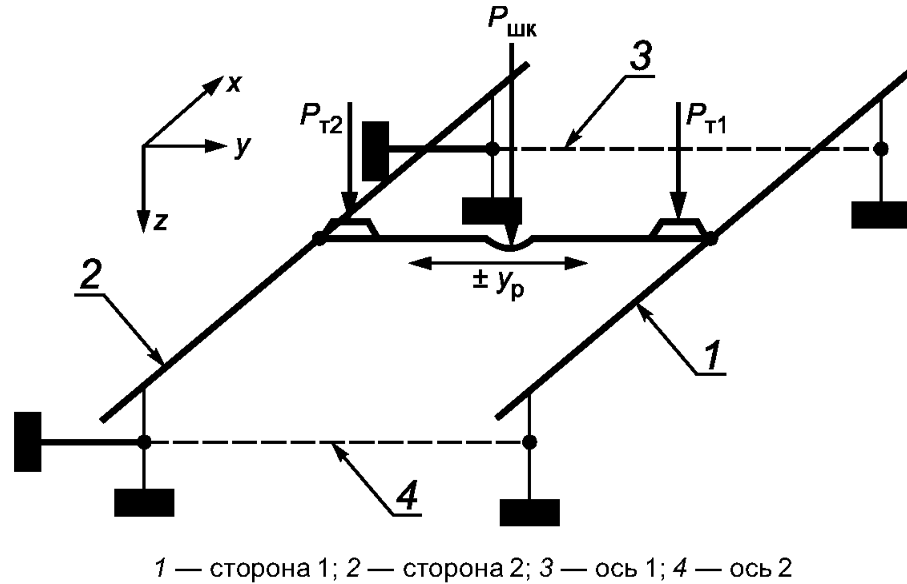
Рисунок Е.2 — Принцип нагружения тележки со шкворнем
