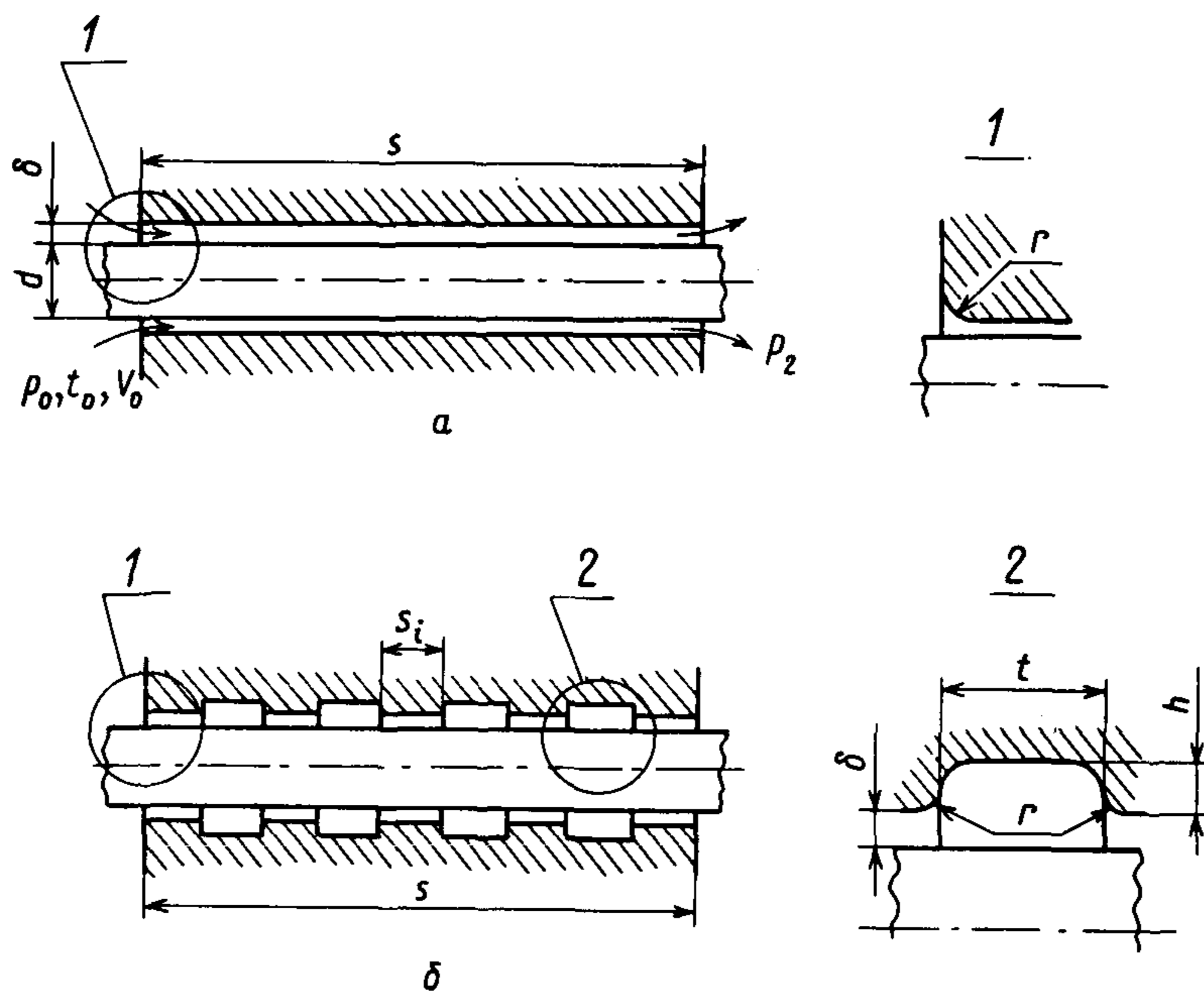
а — гладкая щель; б — щель с канавками
