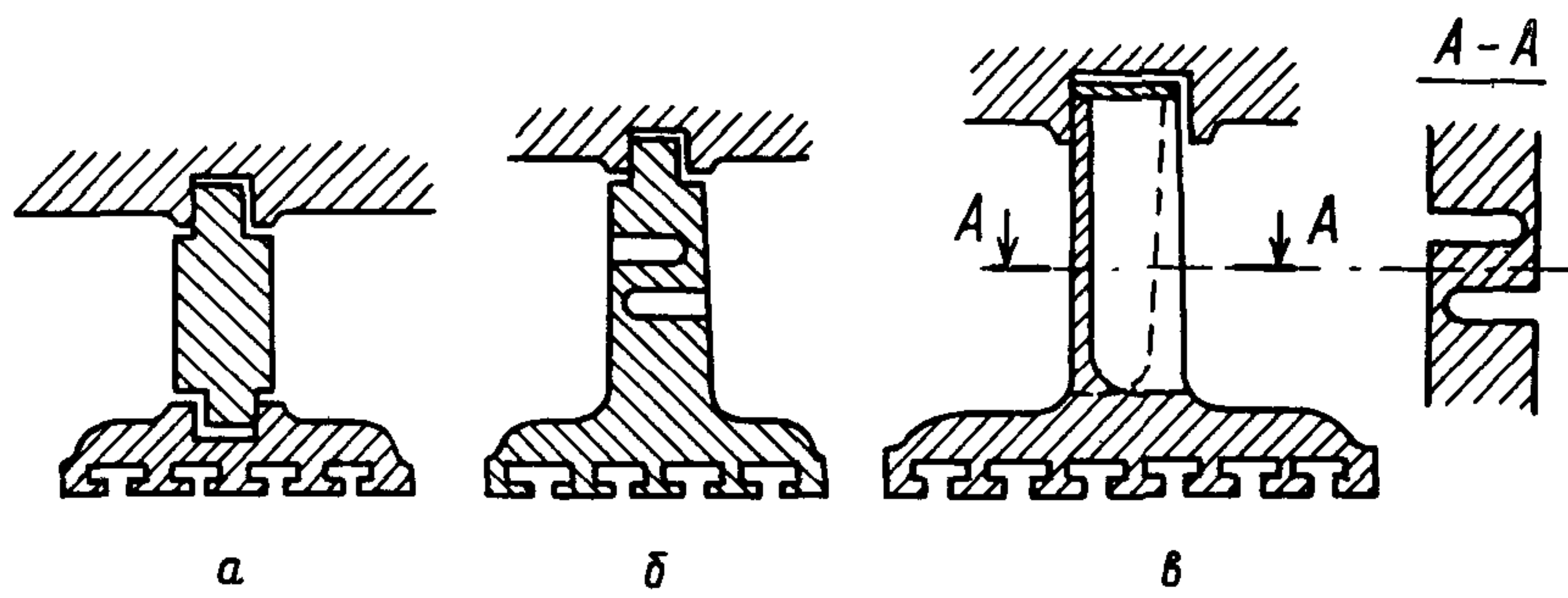
a — составная конструкция; b, v — варианты термокомпенсационных выемок
