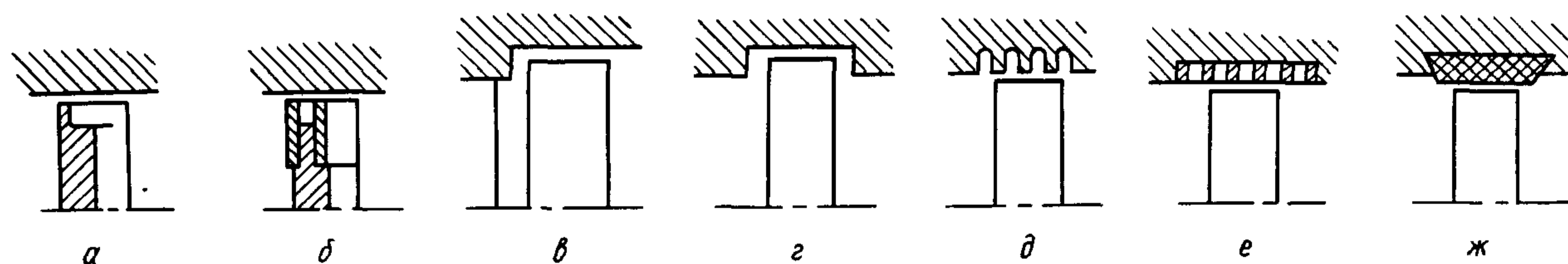
Уплотнения необандаженных лопаточных аппаратов
