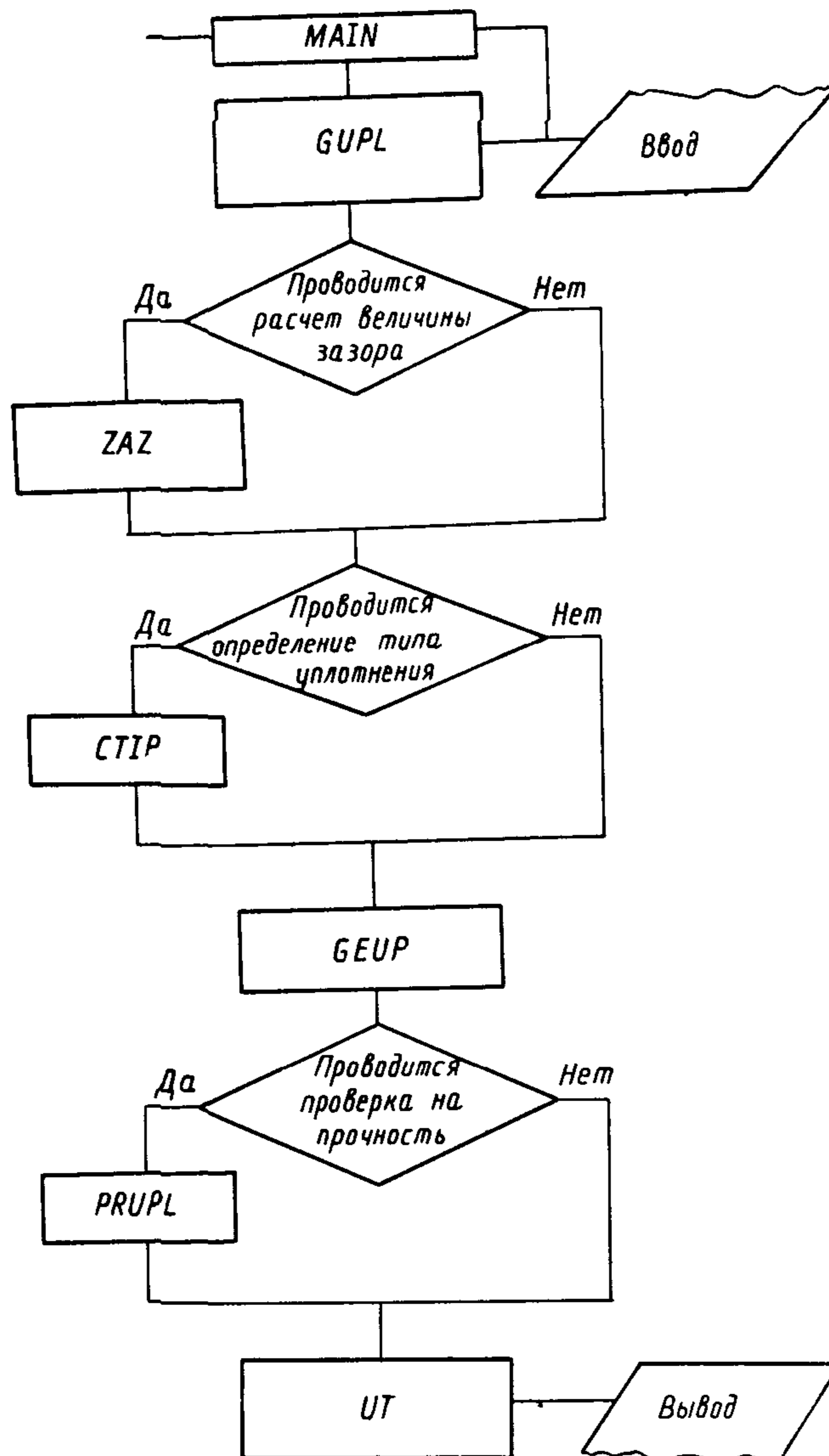
Блок-схема программы проектирования и расчета лабиринтов
