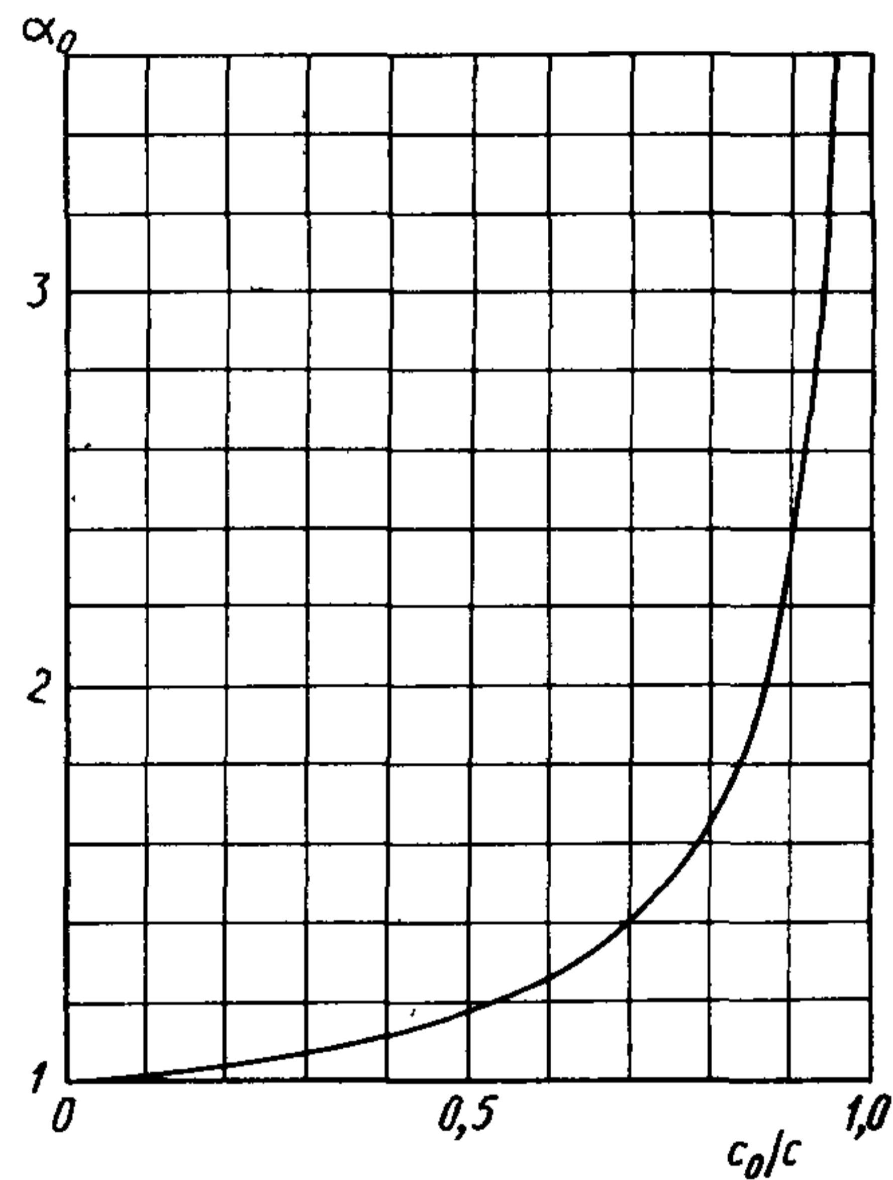
Коэффициент расхода при скругленных кромках ( r > 0,6\delta )
