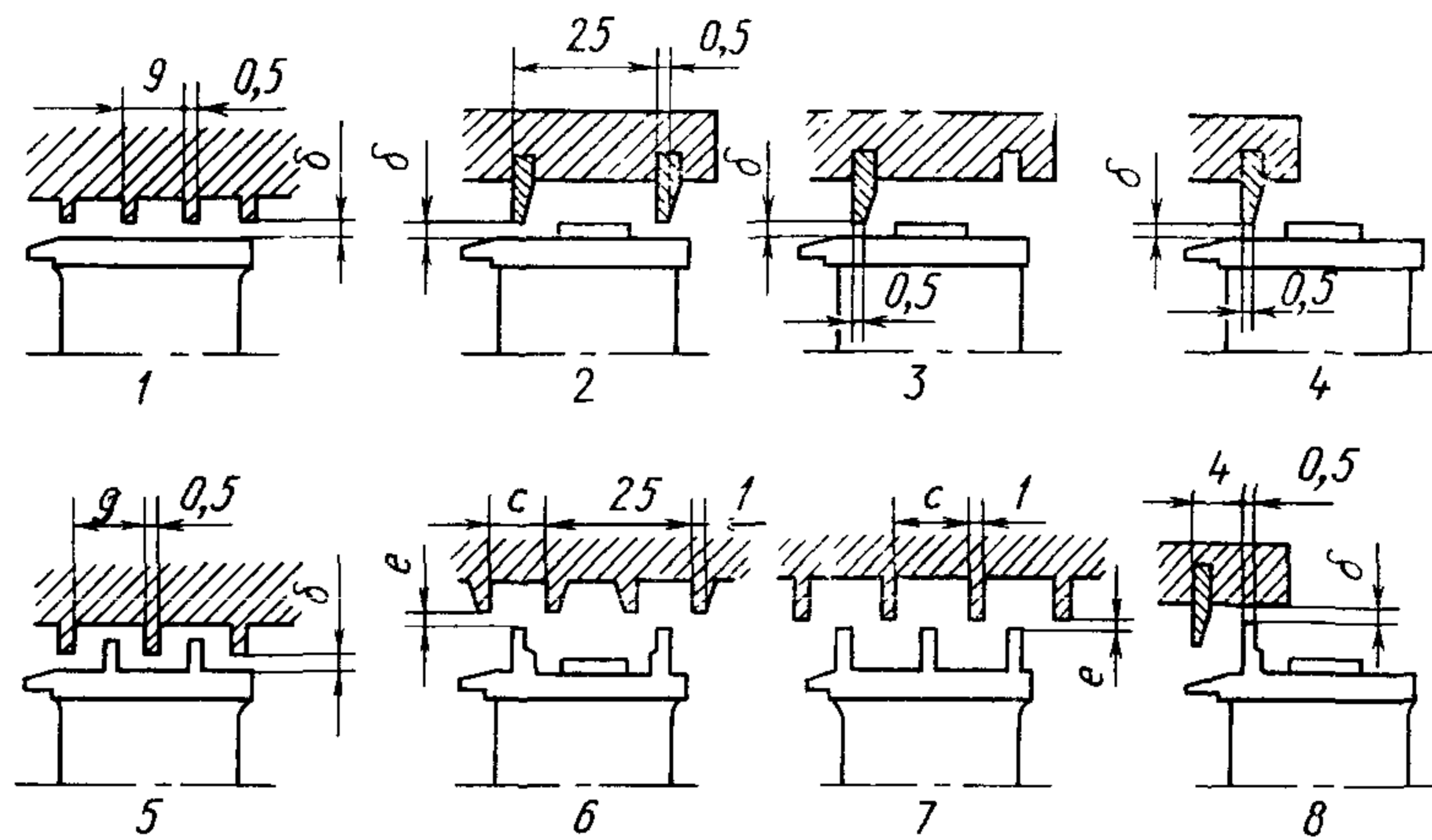
Расходные характеристики некоторых модификаций надбандажных уплотнений
