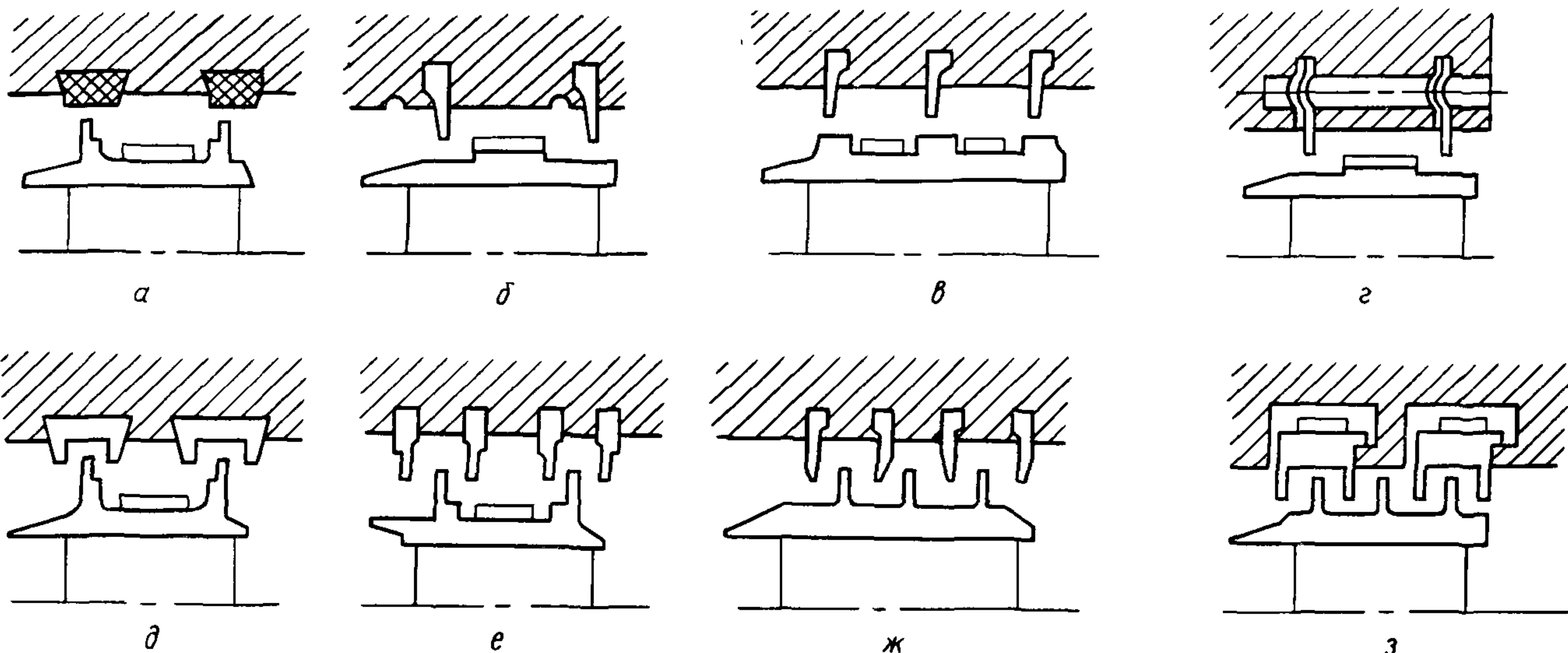
Варианты конструктивного исполнения надбандажных уплотнений
