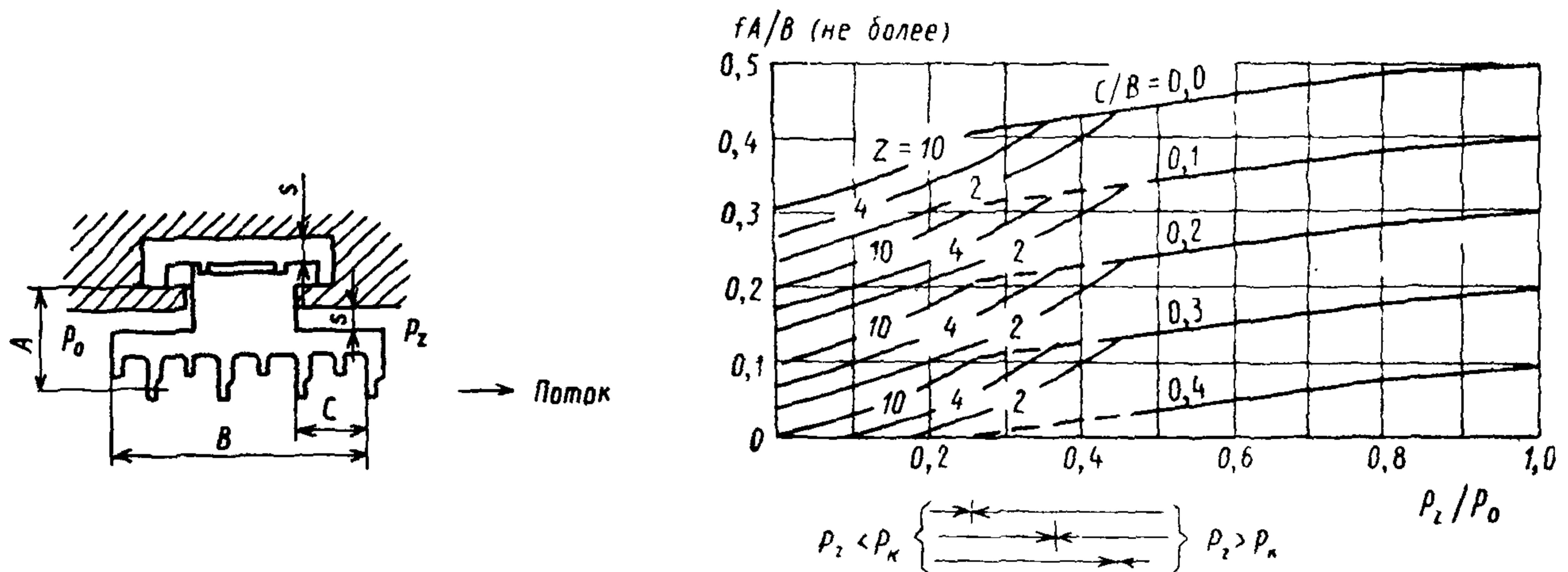
Предельные соотношения размеров сегментных уплотнительных колец
