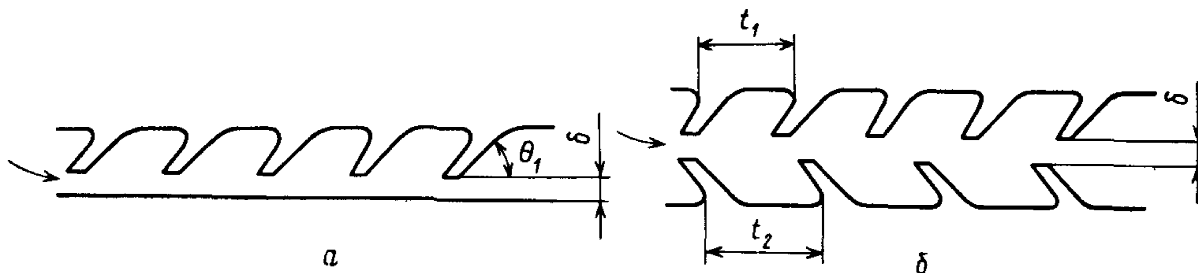
а — одностороннее расположение гребней; б — двустороннее расположение гребней с различными шагами t (нониусное)
