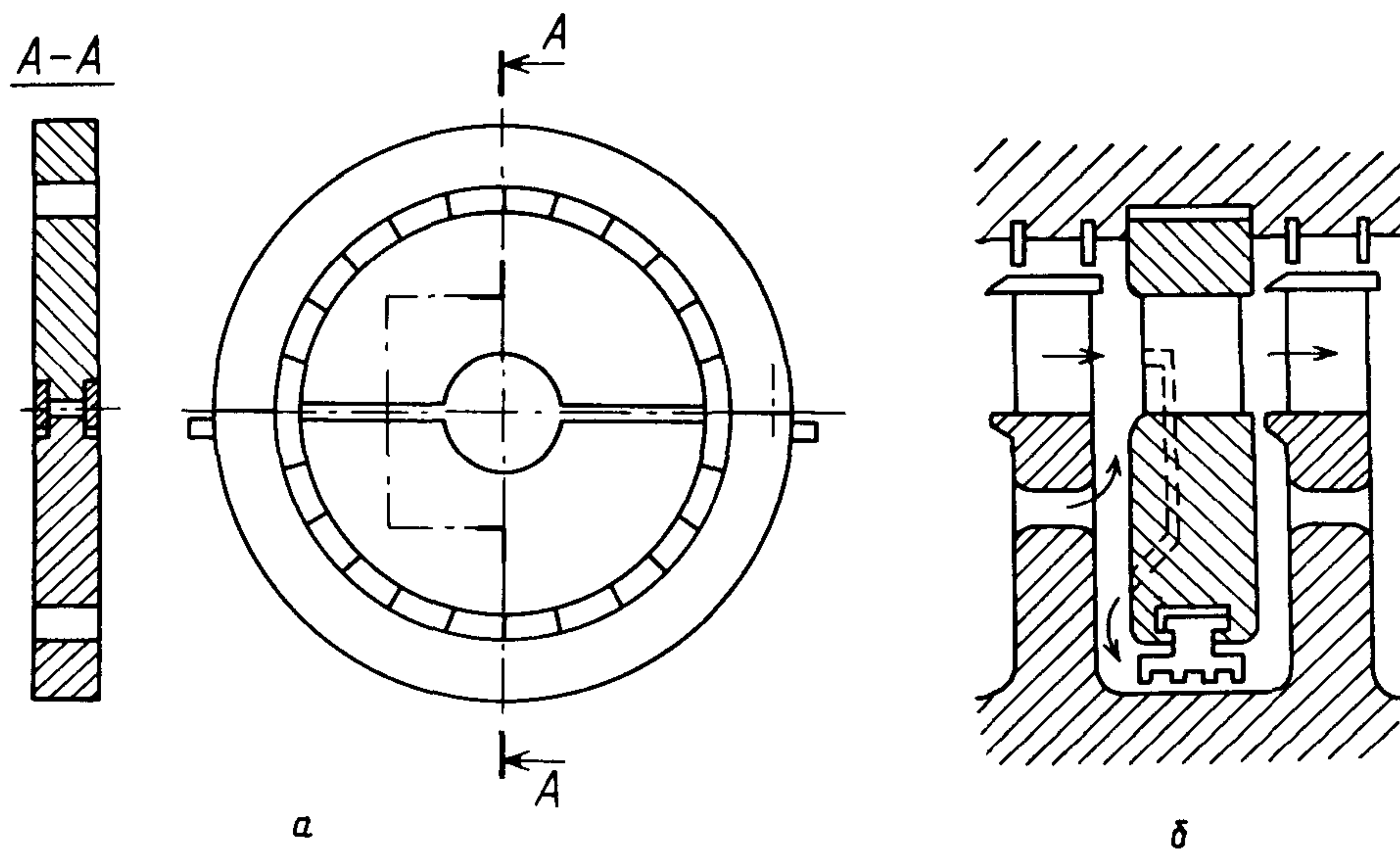
a — независимая подвеска верхних половин; b — перепуск пара для выравнивания температур
