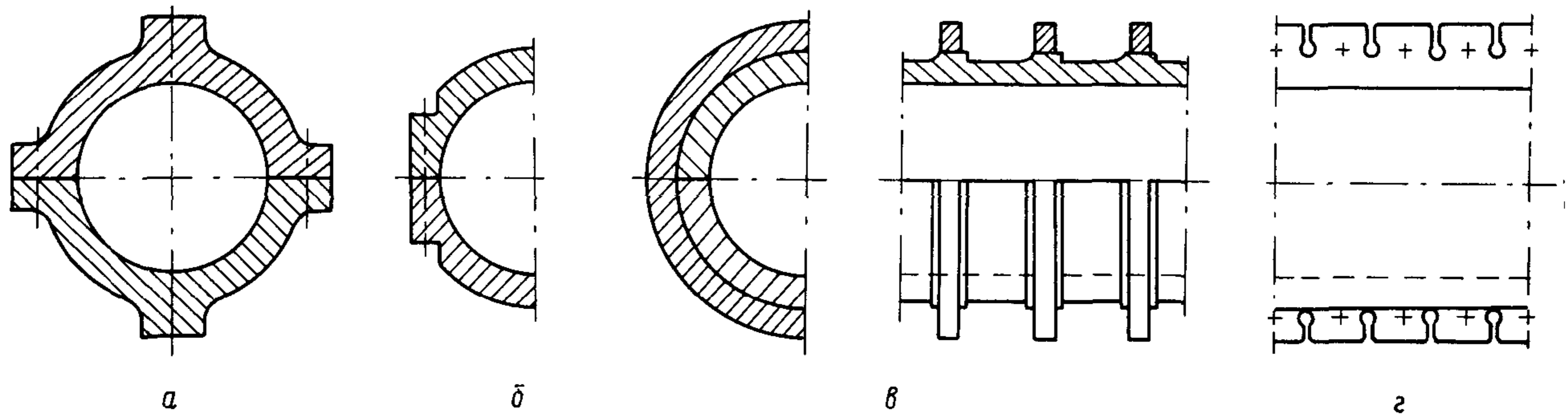
а — ложные фланцы; б — узкие фланцы; в — стяжные кольца; г — разрезной фланец
