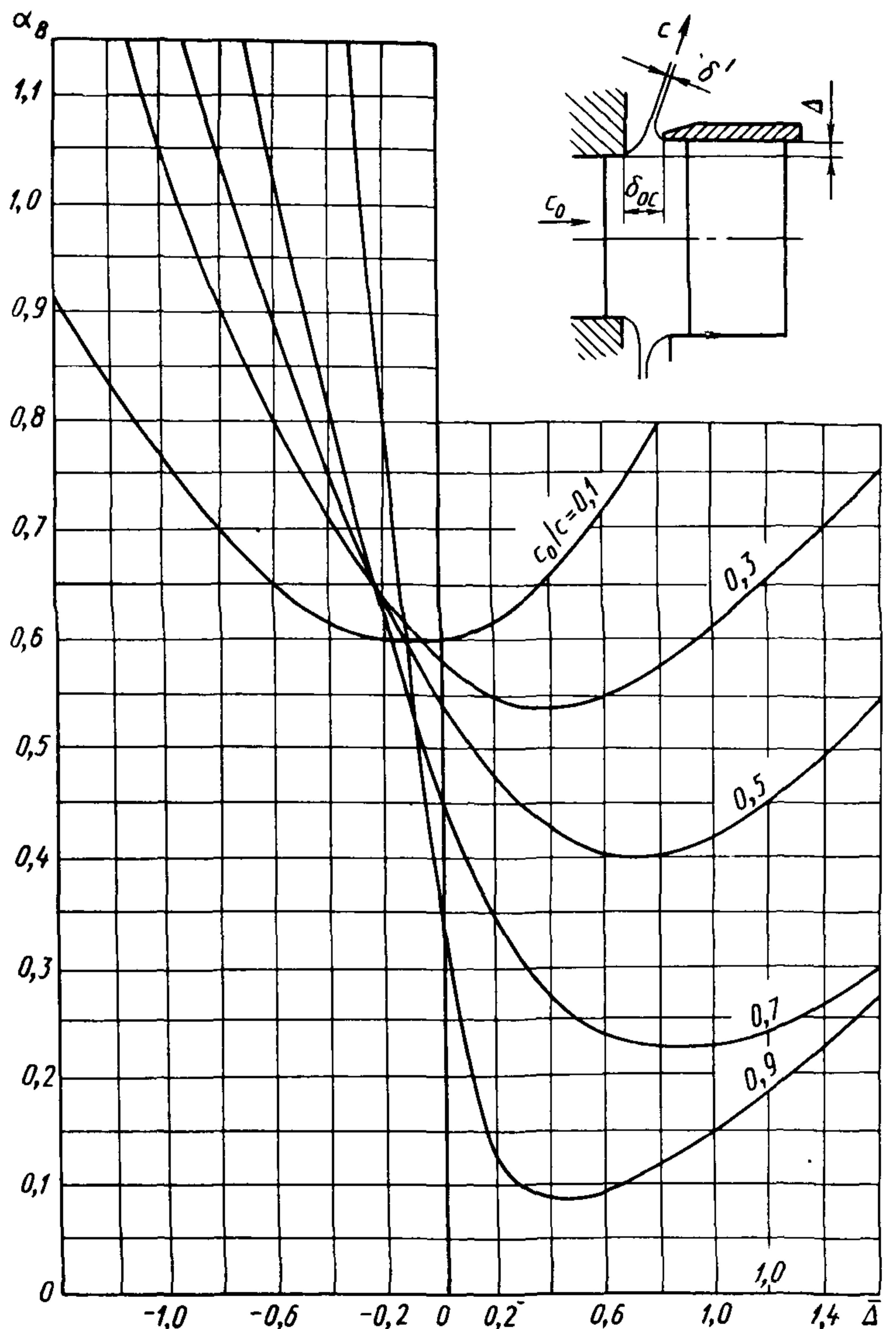
Коэффициент расхода через межвенцовый зазор
