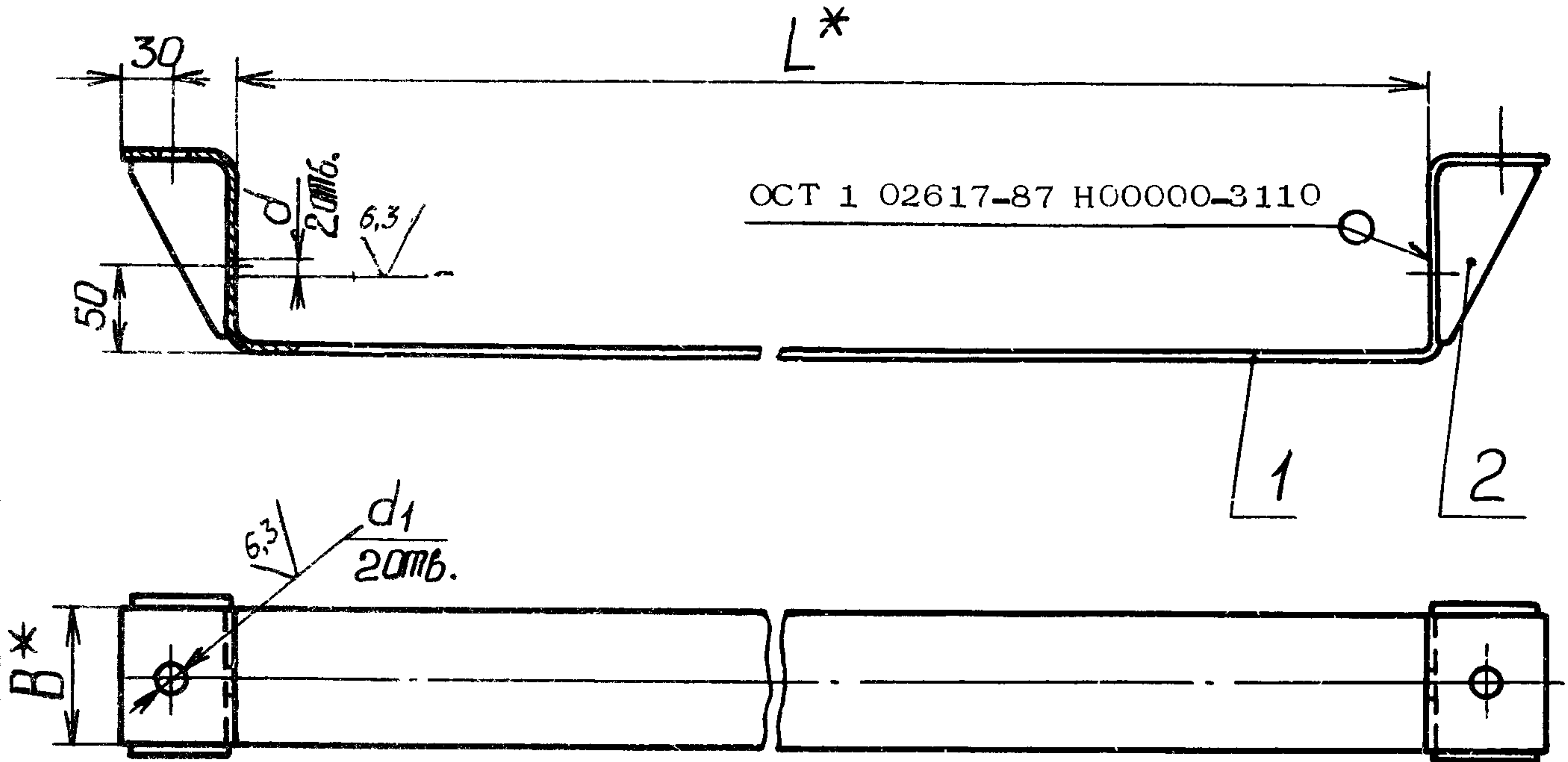
Размеры, мм
