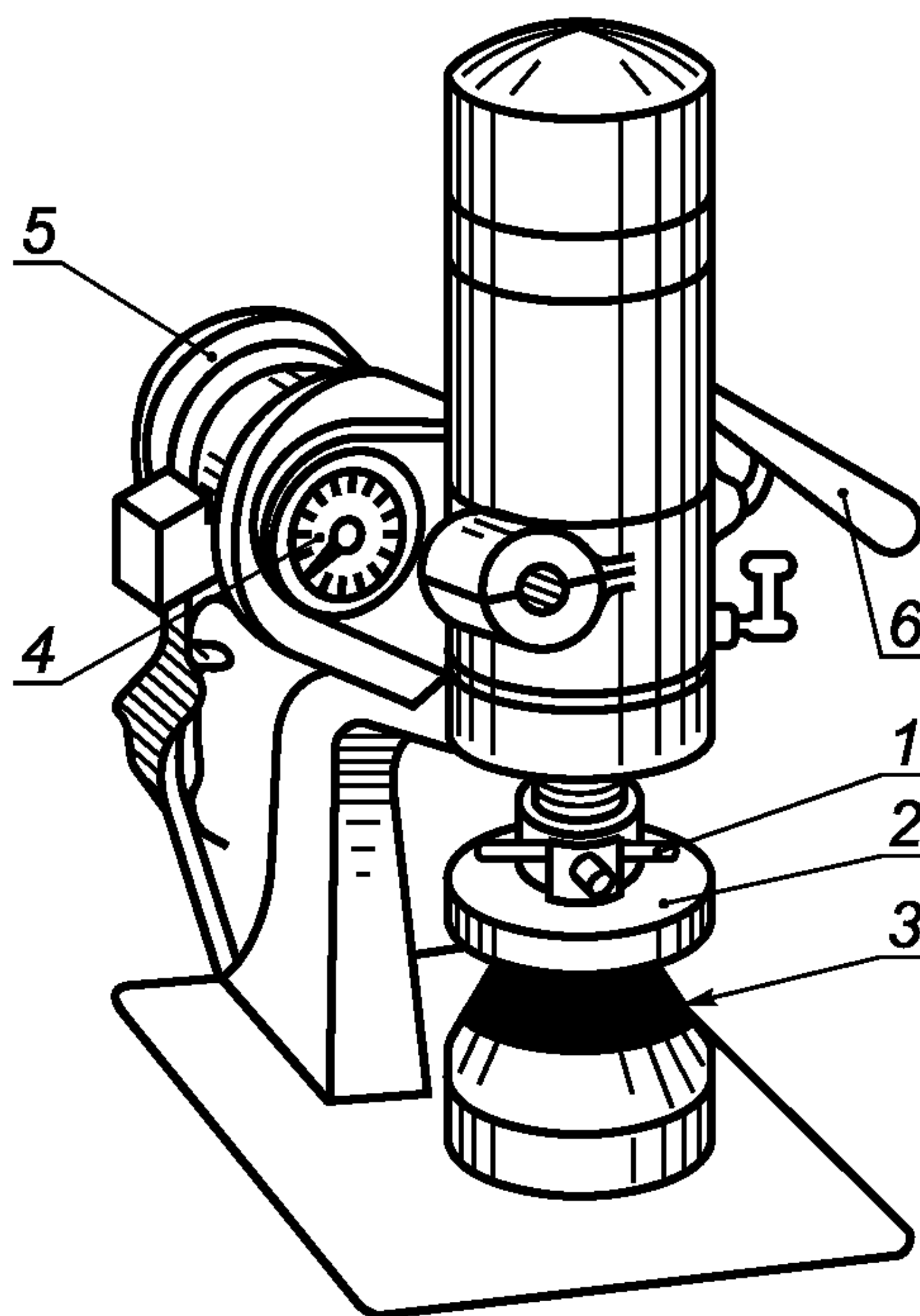
1 — гайка; 2 — патрон; 3 — подушка; 4 — счетчик; 5 — мотор; 6 — рукоятка
