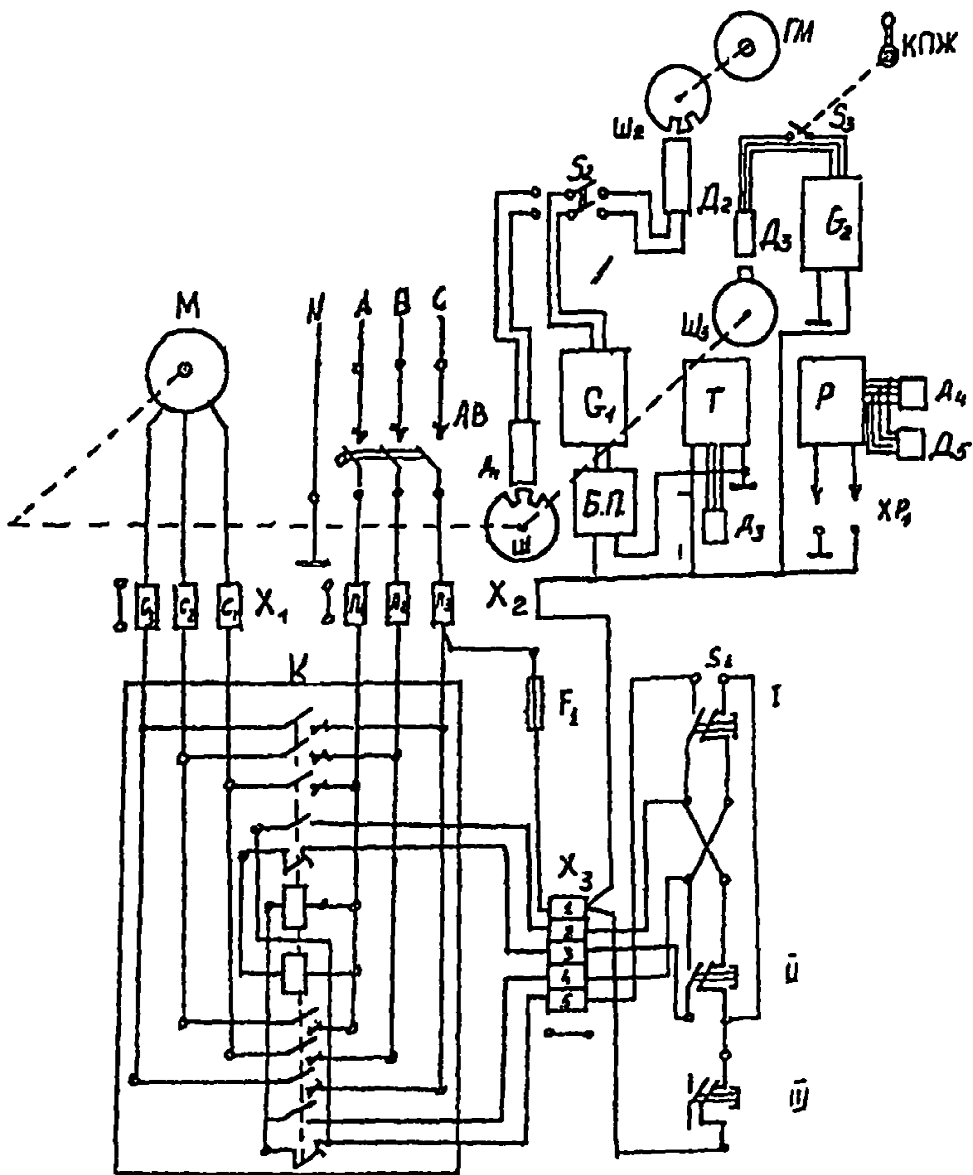
Рис. 18. Схема электрическая принципиальная:
