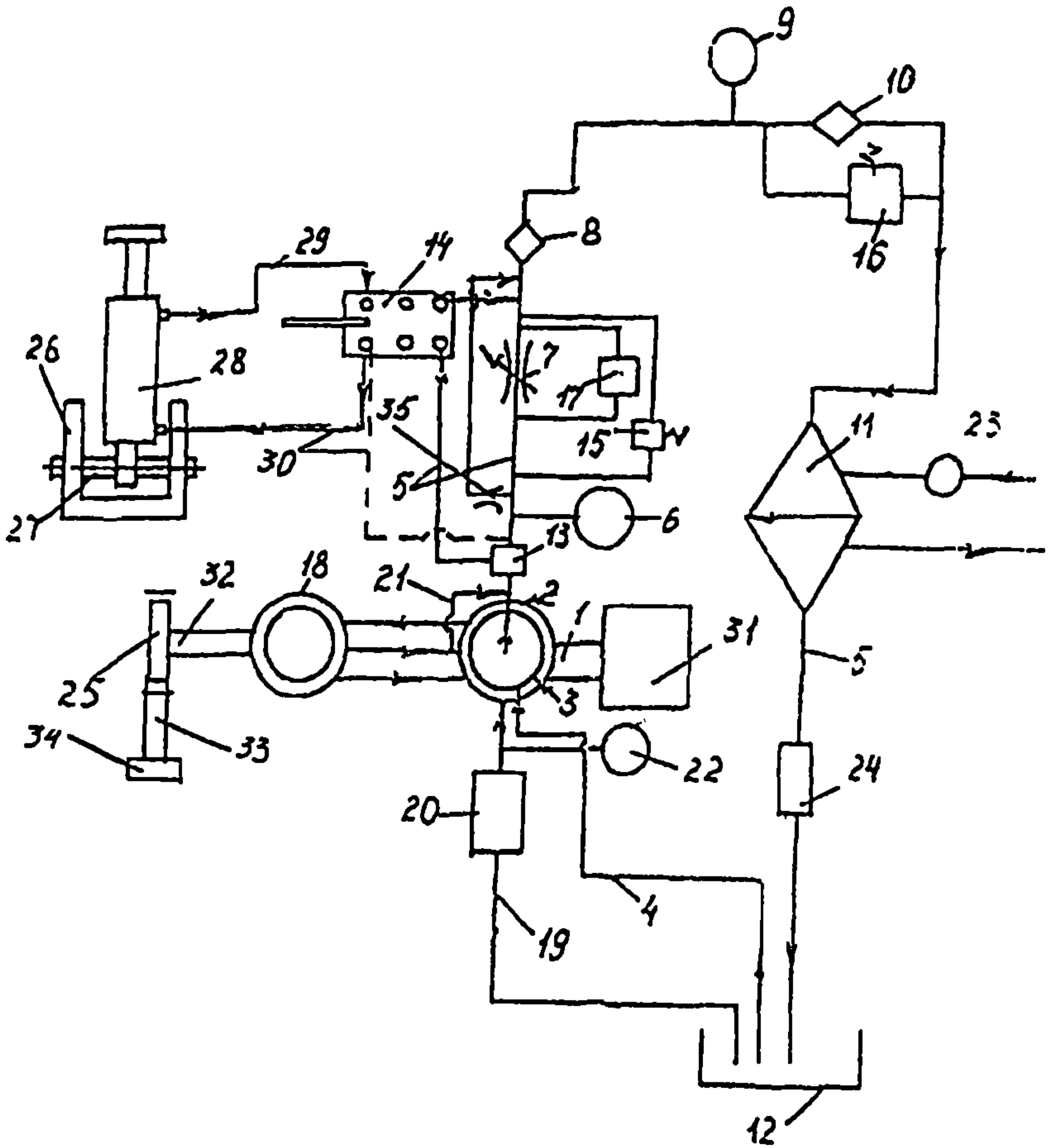
Рис. 17. Схема стенда для испытания гидрообъемных приводов:
