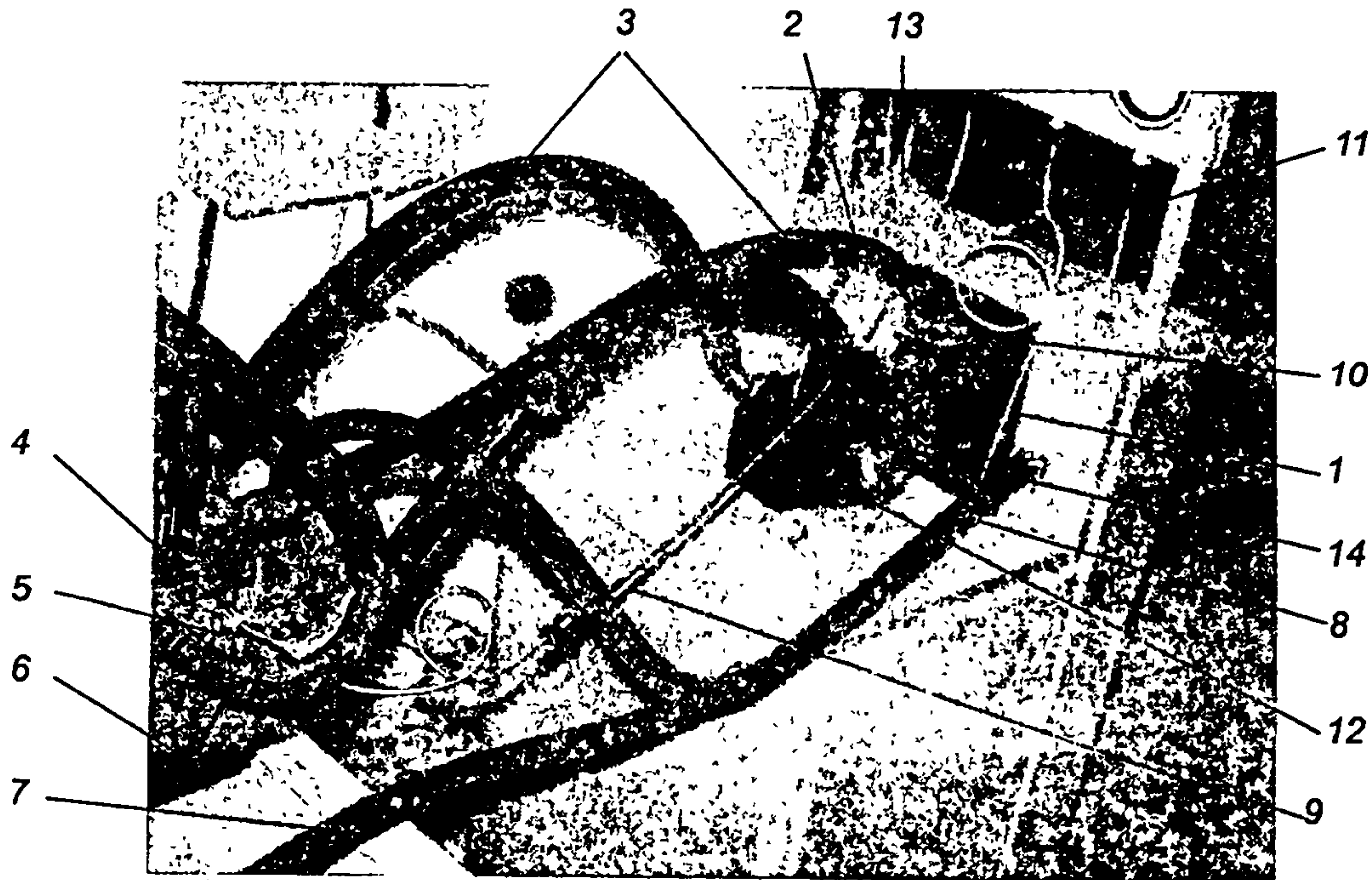
Рис. 11. Монтаж гидролинии ГСТ:
