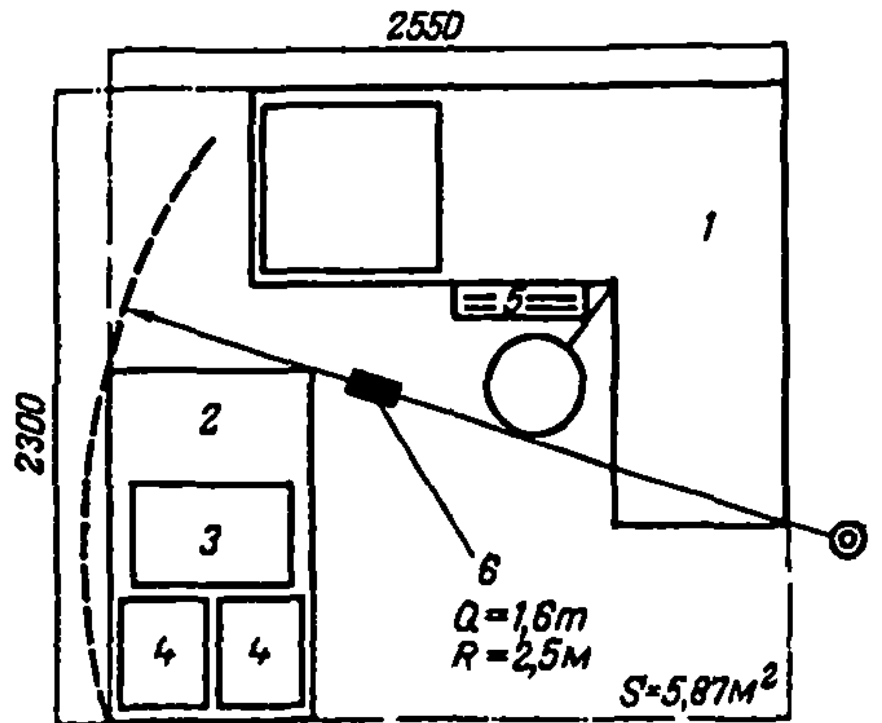
Рис. 2.5. Планировка рабочего места дефектовщика:
