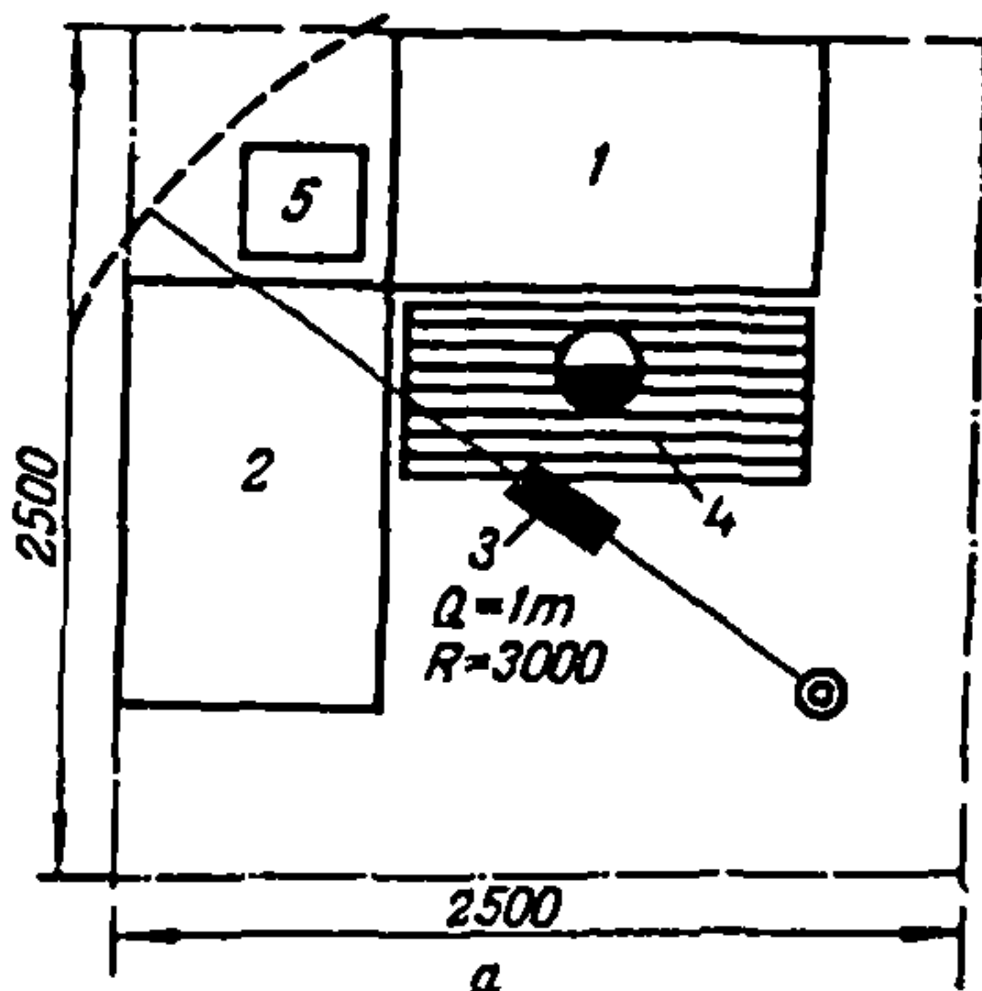
Рис. 2.6. Рабочее место слесаря-ремонтника по ремонту и сборке узлов станка:
