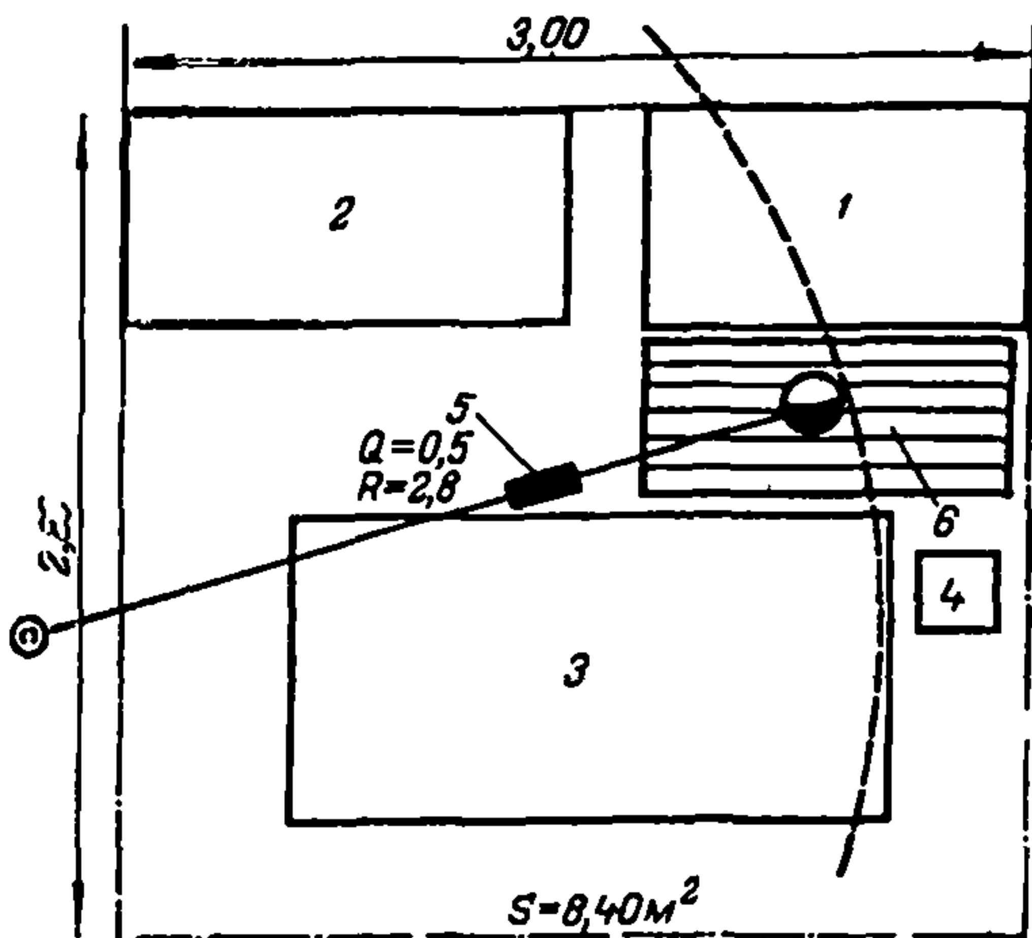
Рис. 2.4. Планировка рабочего места слесаря-ремонтника по разборке узлов станка:
