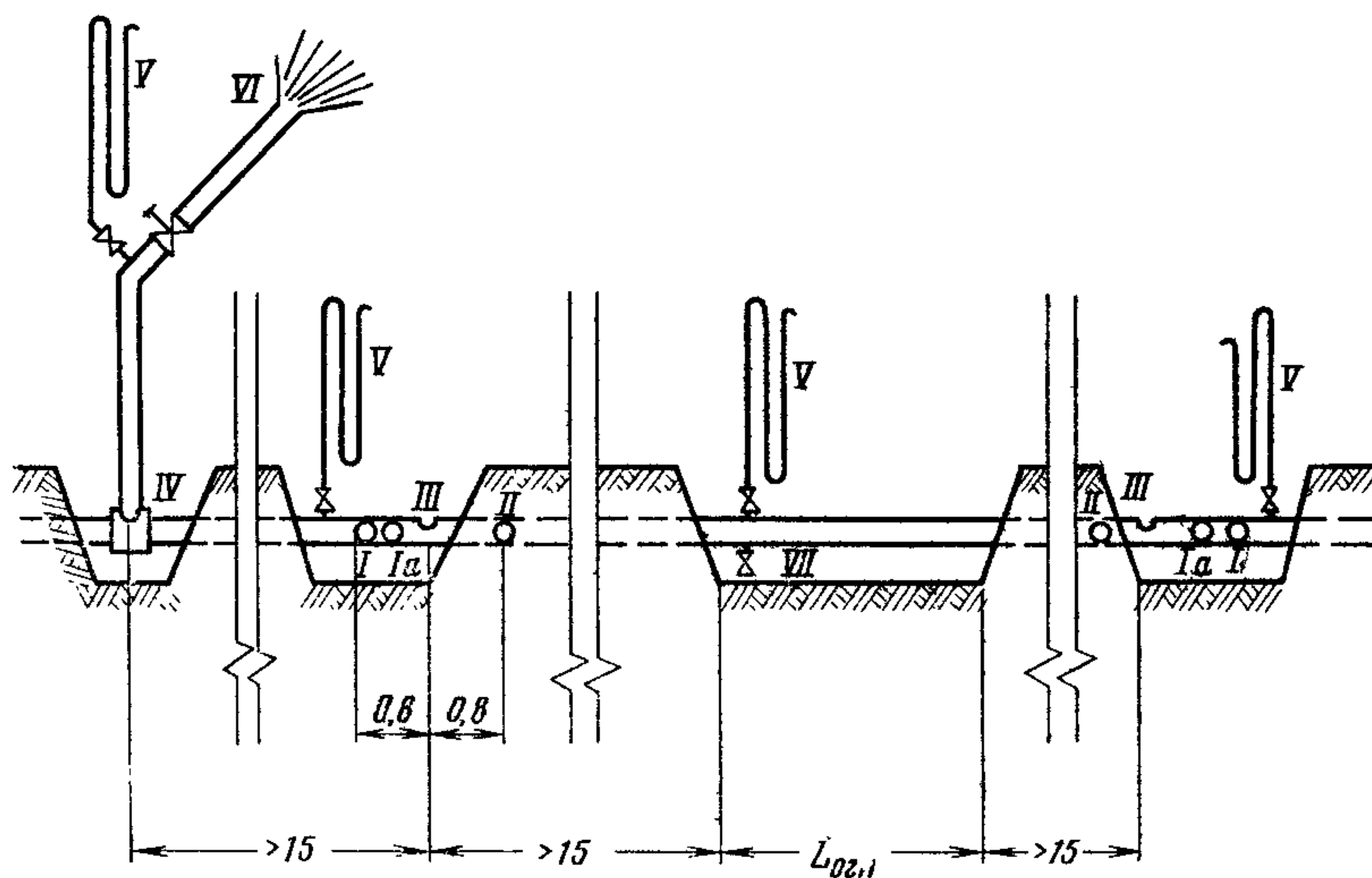
Схема установки запорных шаров:
