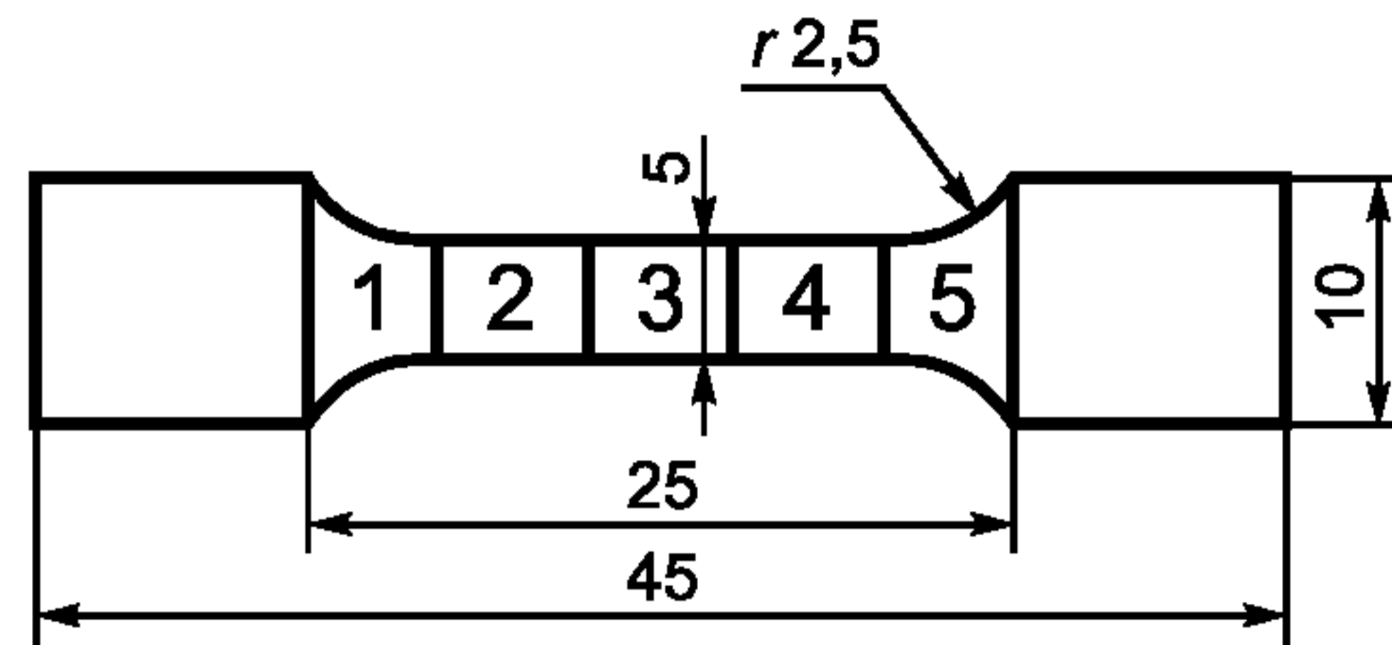
Рисунок 6 — Разметка рабочей части ремешка
