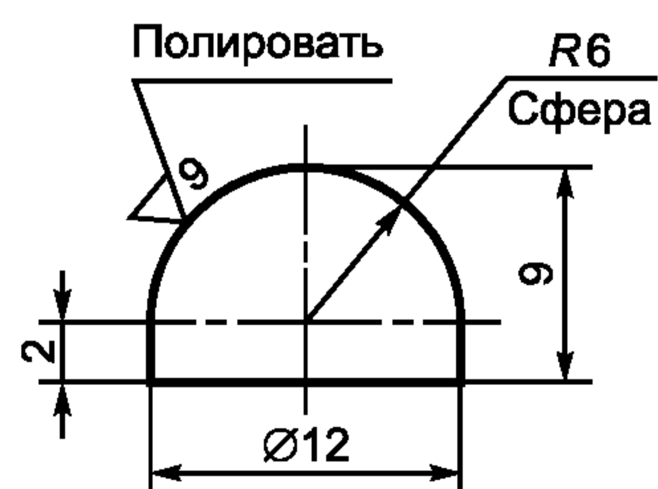
Рисунок 3 — Сферическая площадка для толщиномера
