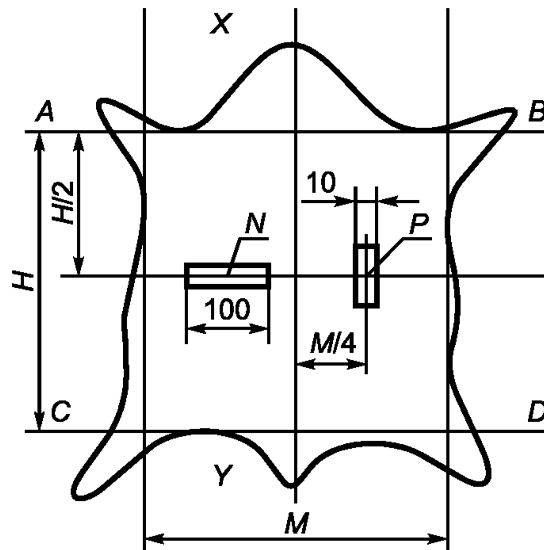
Рисунок 9 — Разметка шкур овчины
