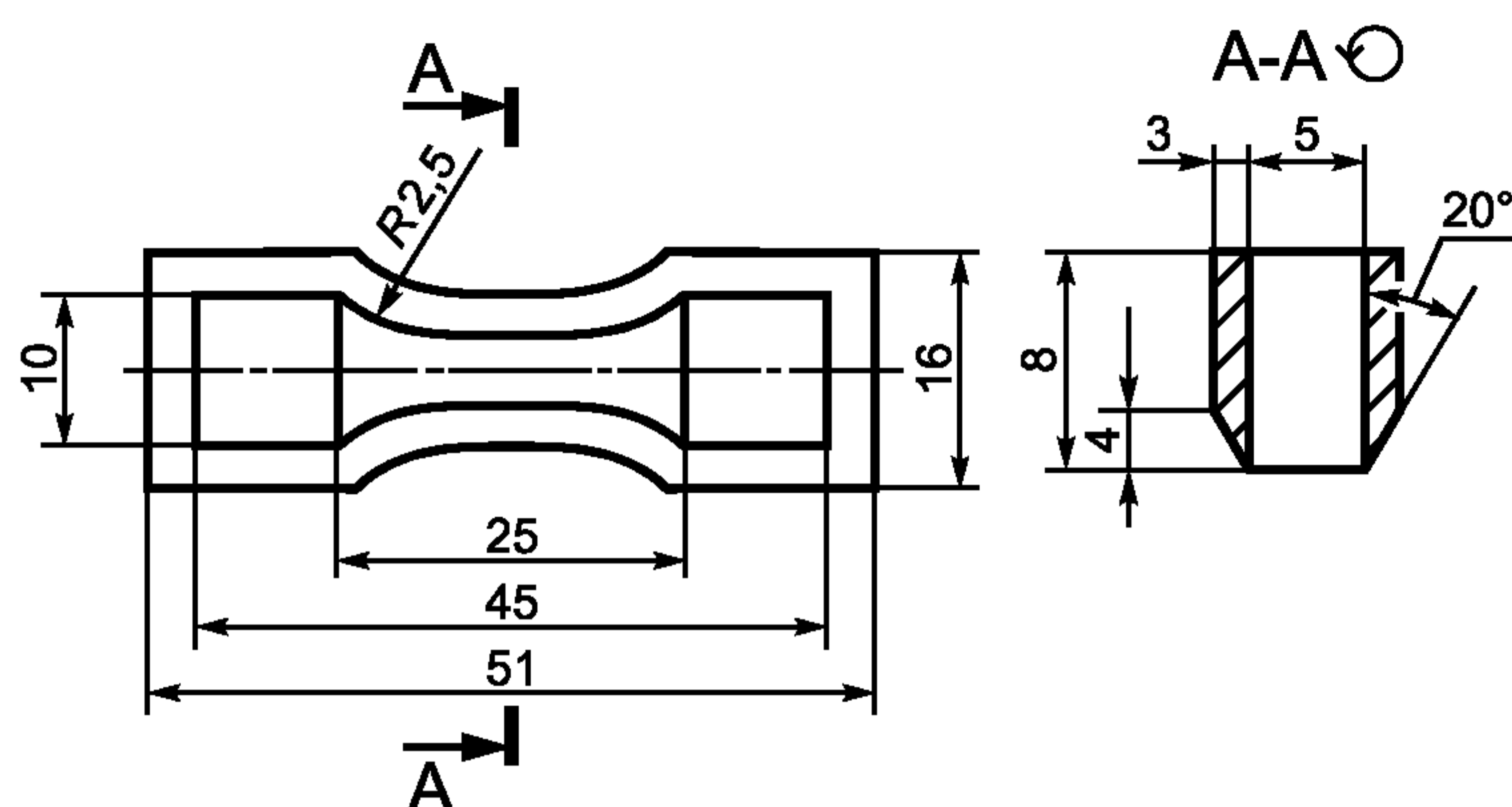
Рисунок 4 — Резак для вырубания ремешков
