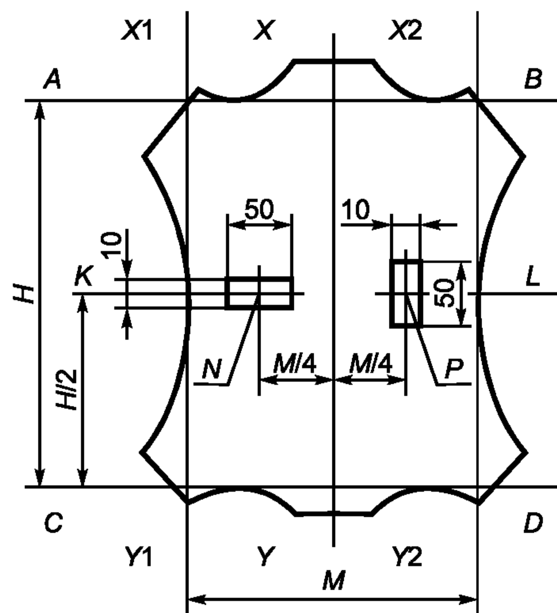
Рисунок 8 — Разметка шкурок шириной более 16 см
