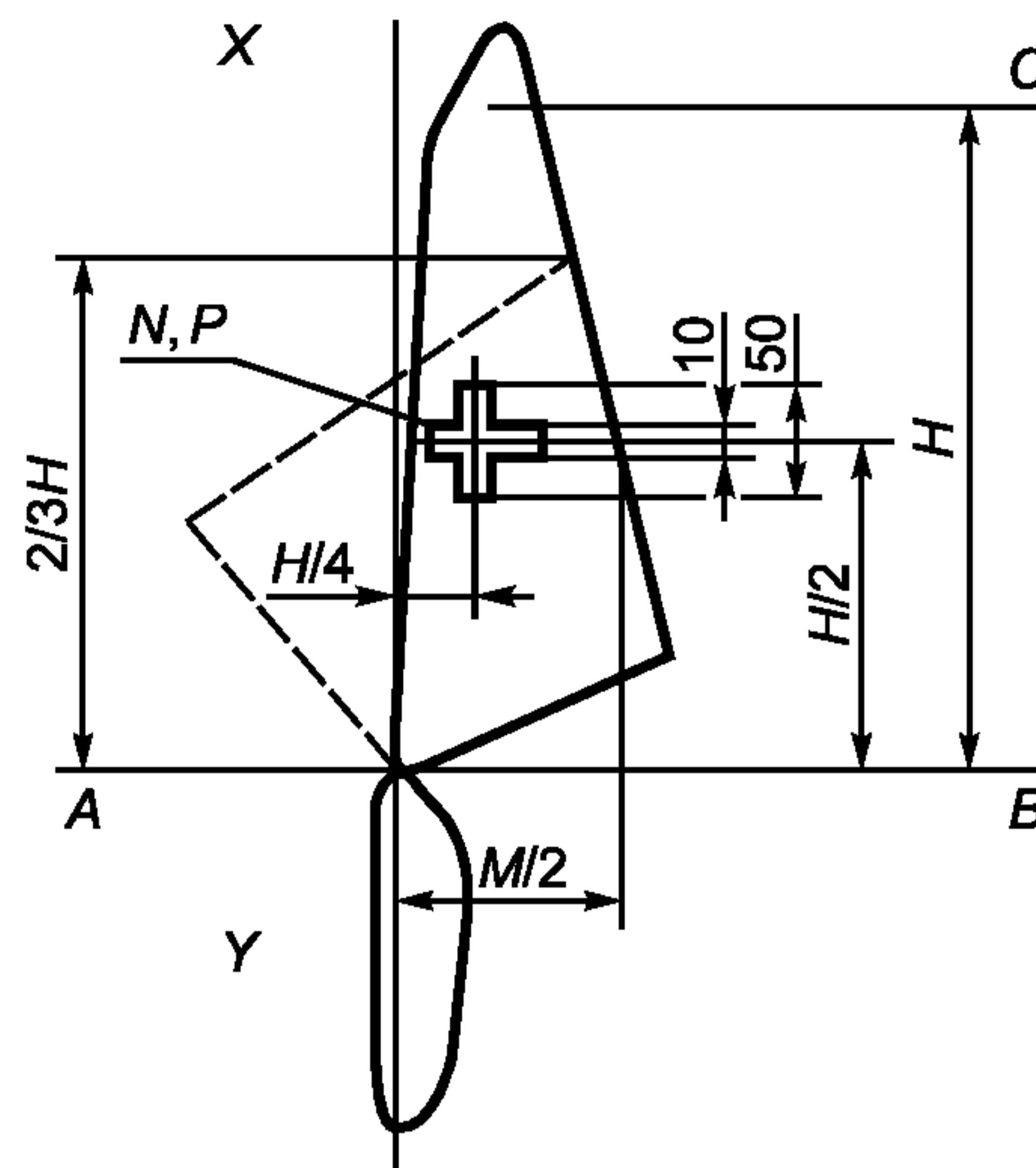
Рисунок 11 — Разметка шкурок, выделанных трубкой
