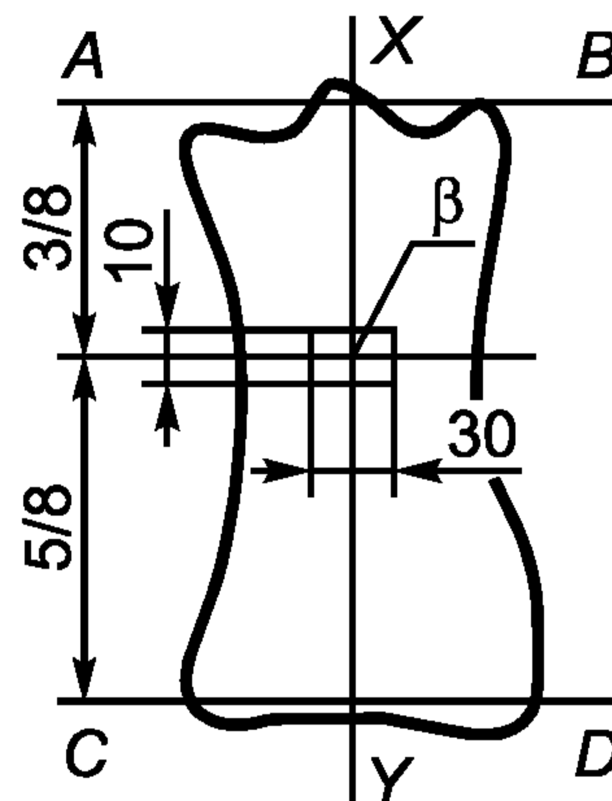
Рисунок 7 — Разметка шкурок шириной до 16 см
