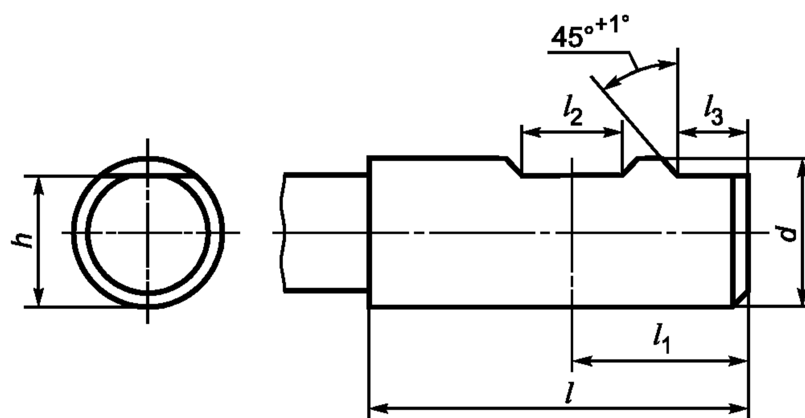
Рисунок 2 — Хвостовики исполнений 2 и 3
