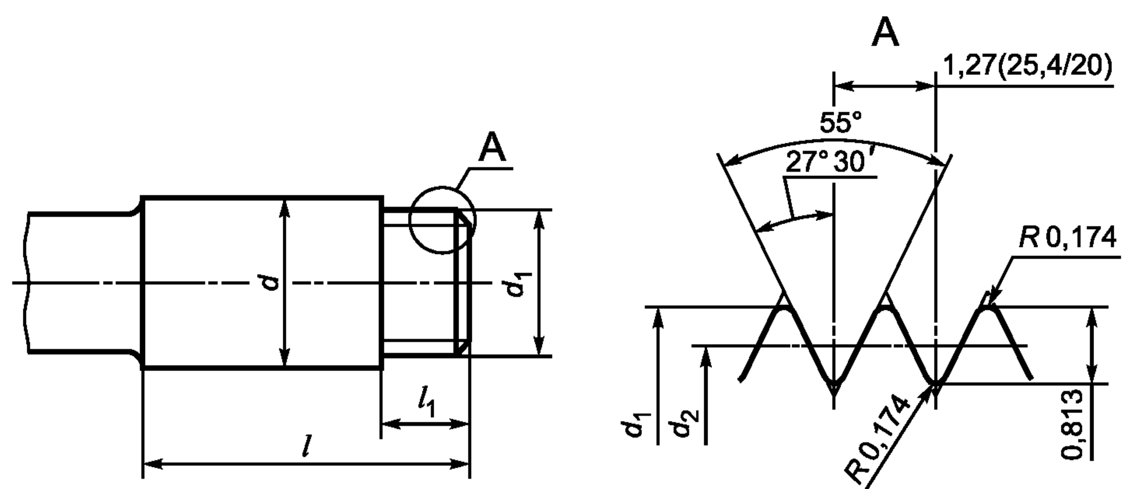
Рисунок 4 — Хвостовик исполнения 5
