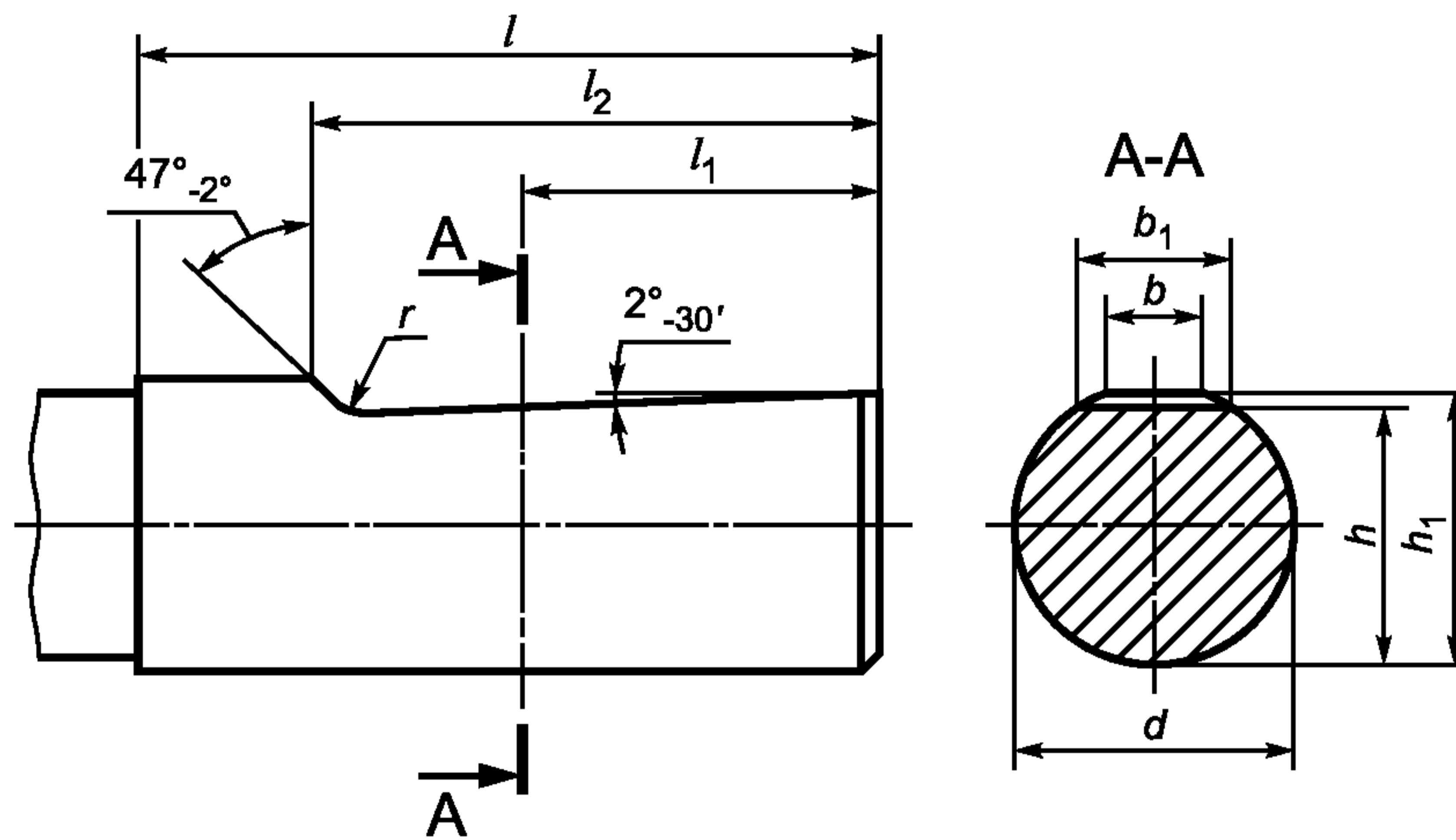
Рисунок 3 — Хвостовик исполнения 4
