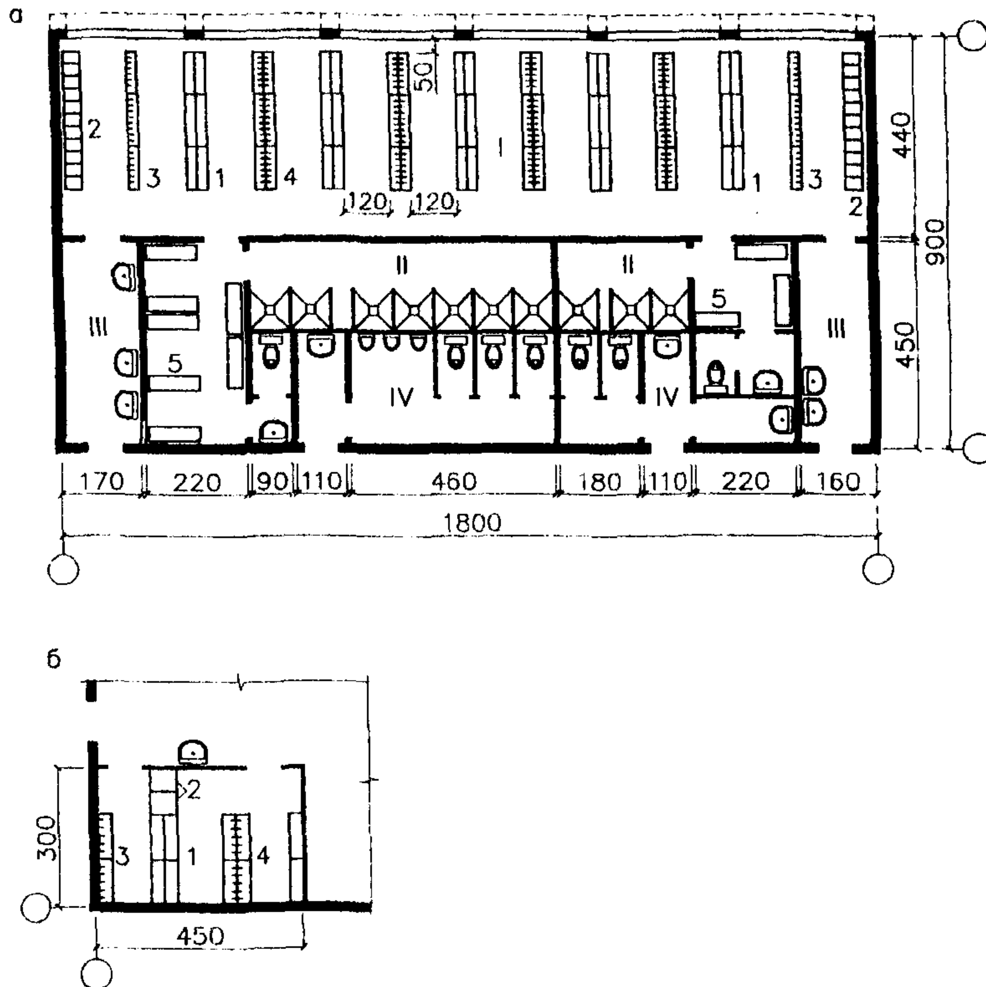
Рис.41. Примеры планировки санитарно-бытовых помещений. а - централизованный блок санитарно-бытовых помещений на 150 мест;
