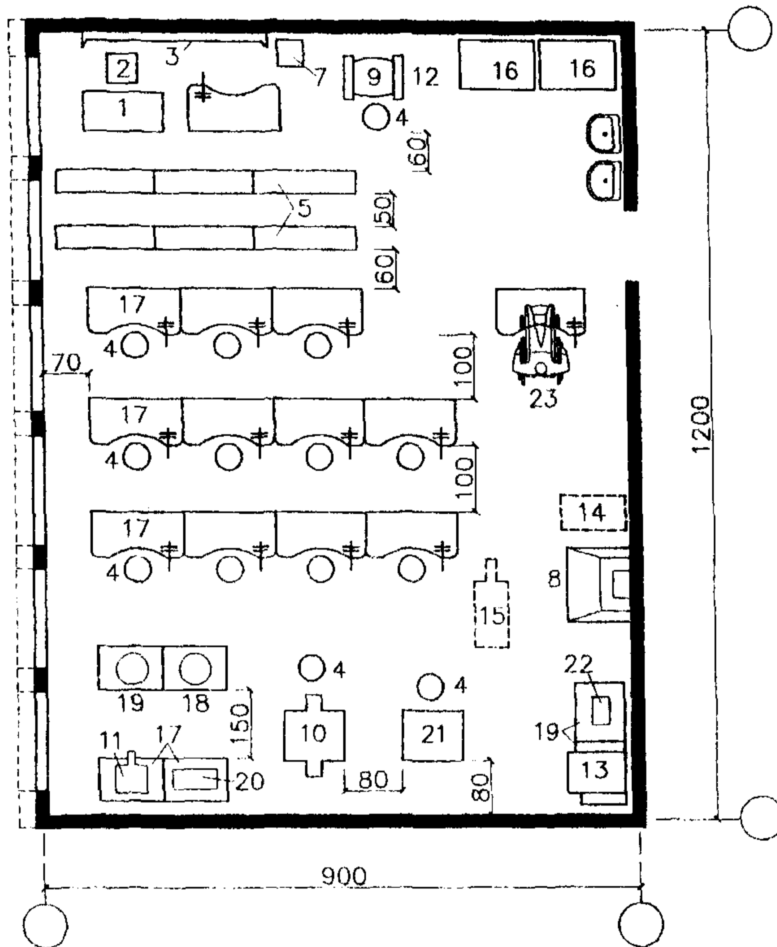
Рис.29. Пример планировки учебно-производственной радиомонтажной мастерской на 12 мест.
