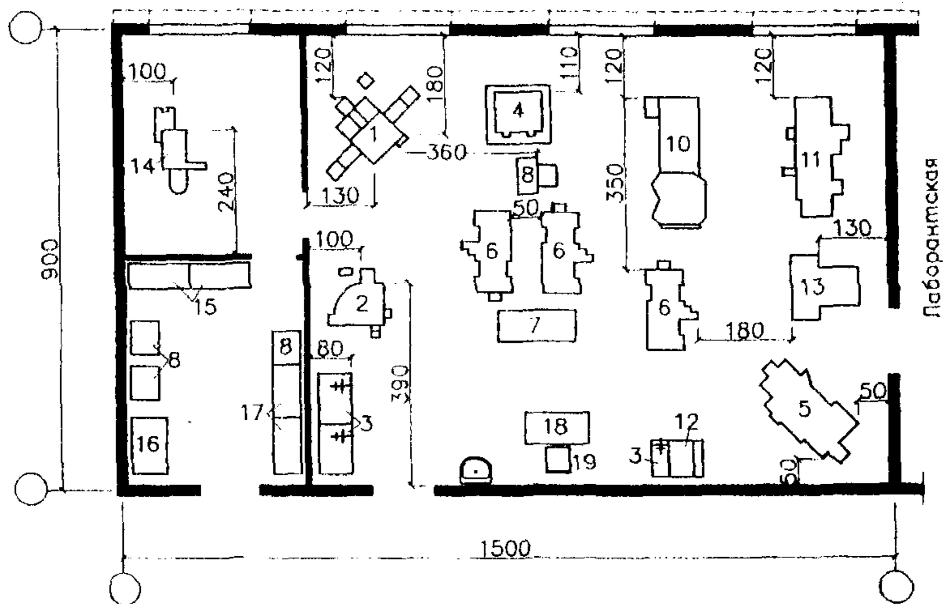
Рис.20. Пример планировки лаборатории технологии машиностроения на 12 мест.
