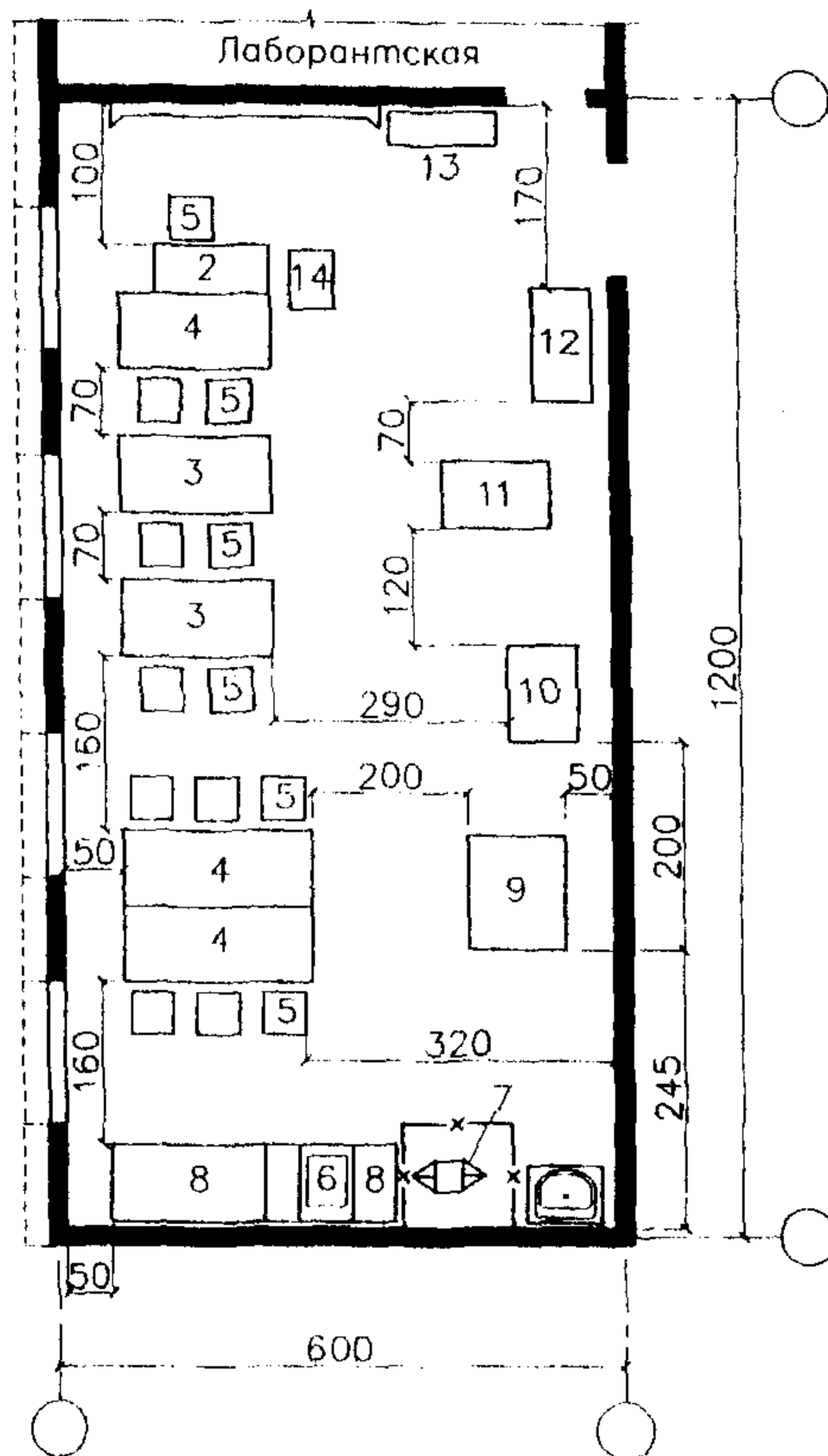
Рис.10. Пример планировки лаборатории материаловедения на 13 мест.
