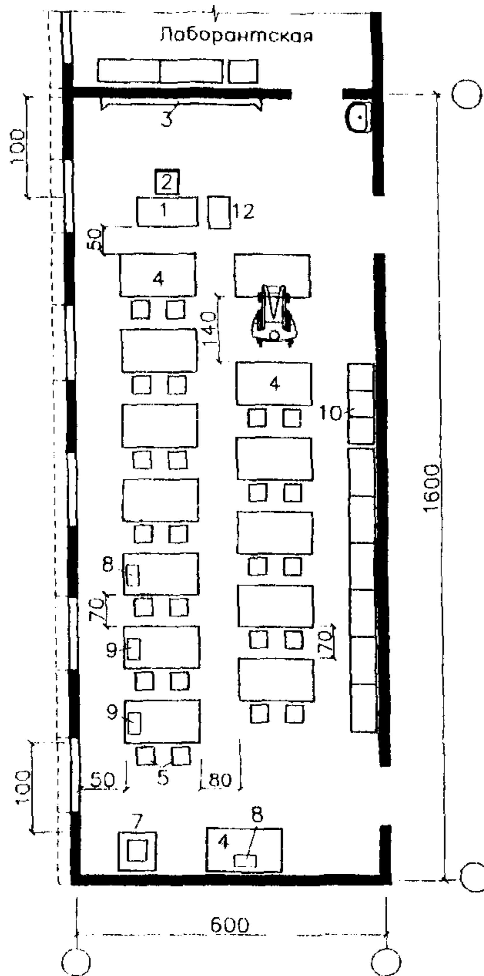
Рис.12. Пример планировки лаборатории метрологии, стандартизации и сертификации на 25 мест.
