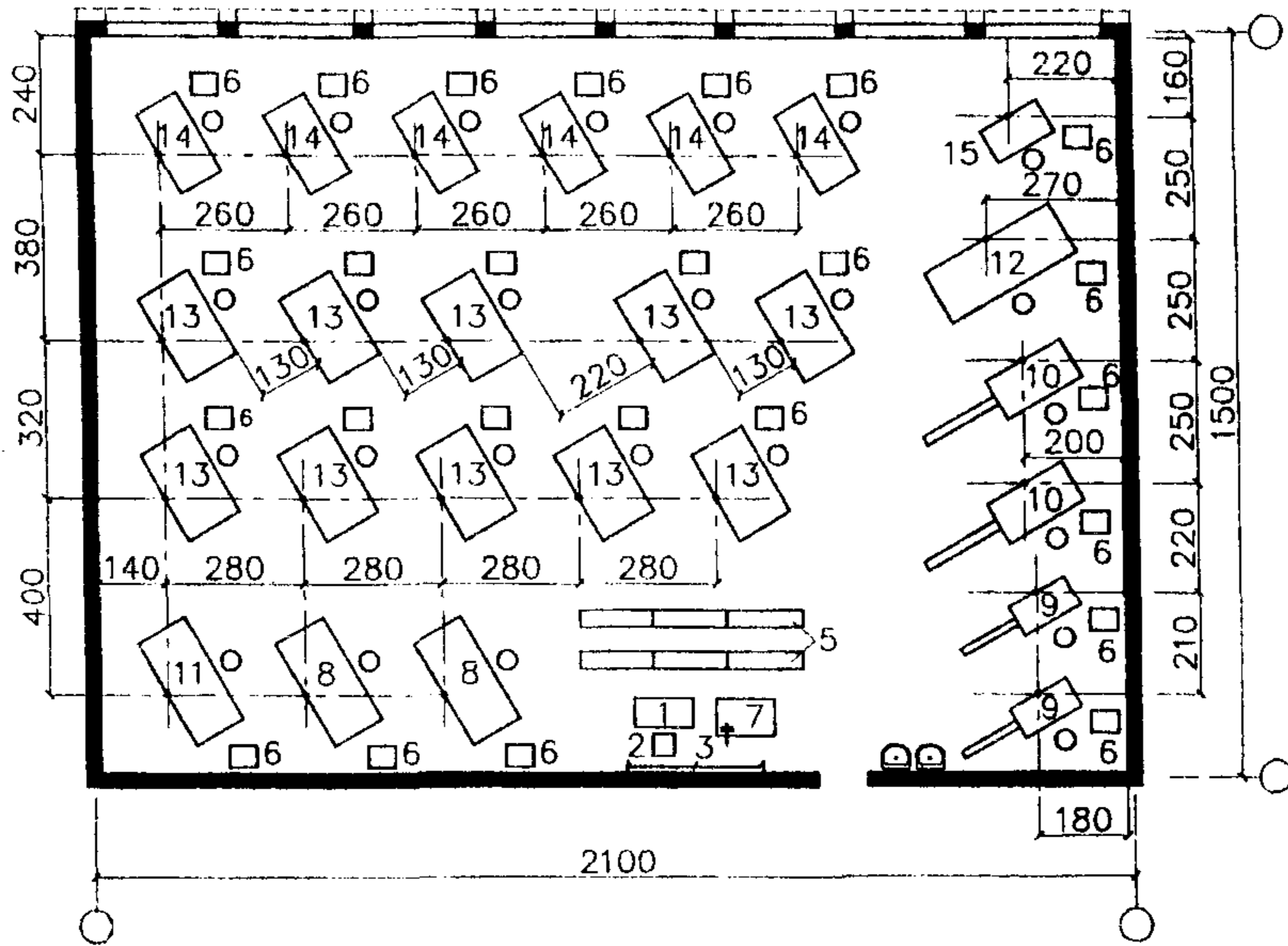
Рис.25. Пример планировки учебно-производственной токарной мастерской на 25 мест.
