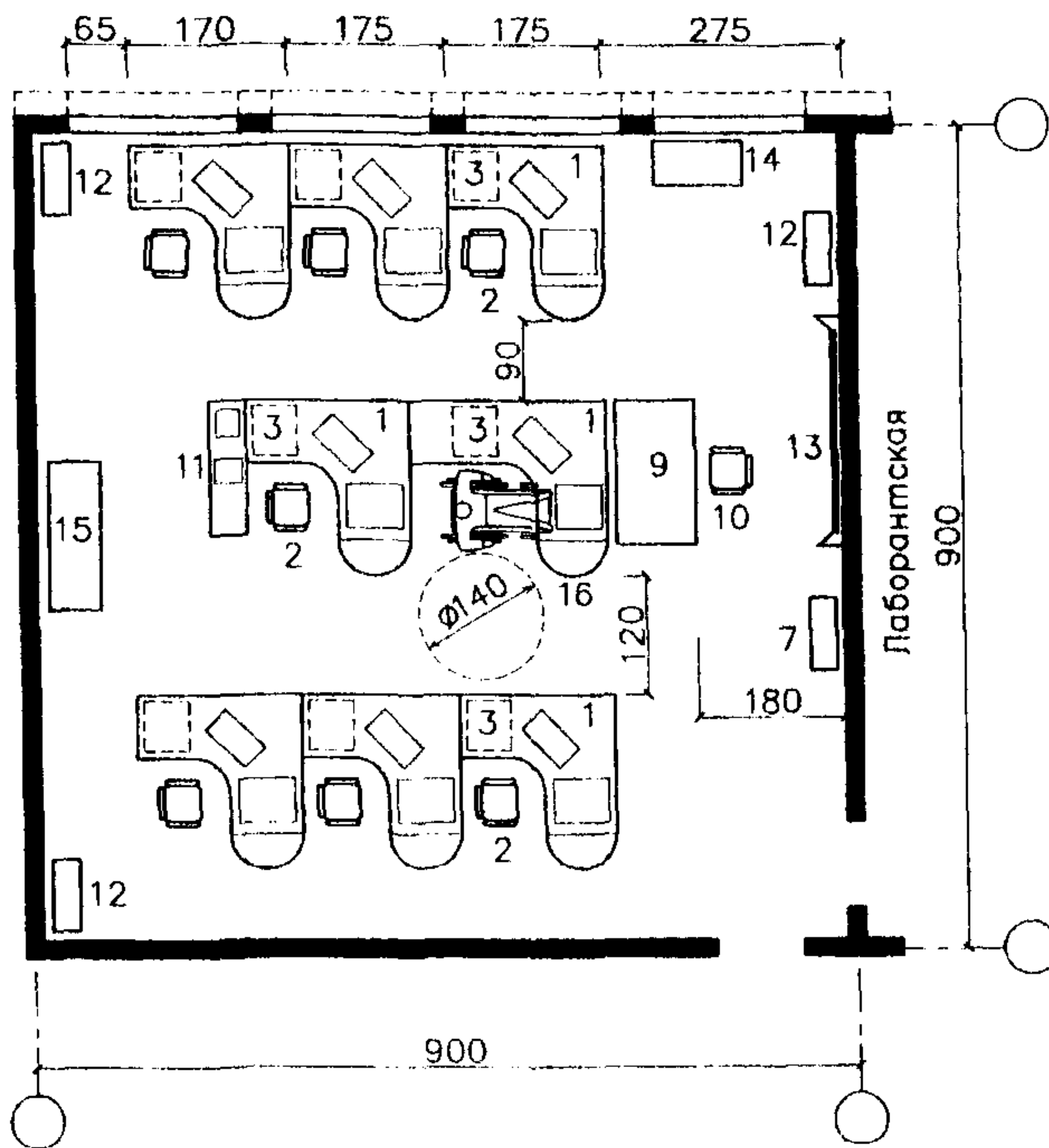
Рис.9. Пример планировки лаборатории информационных технологий на 8 мест.
