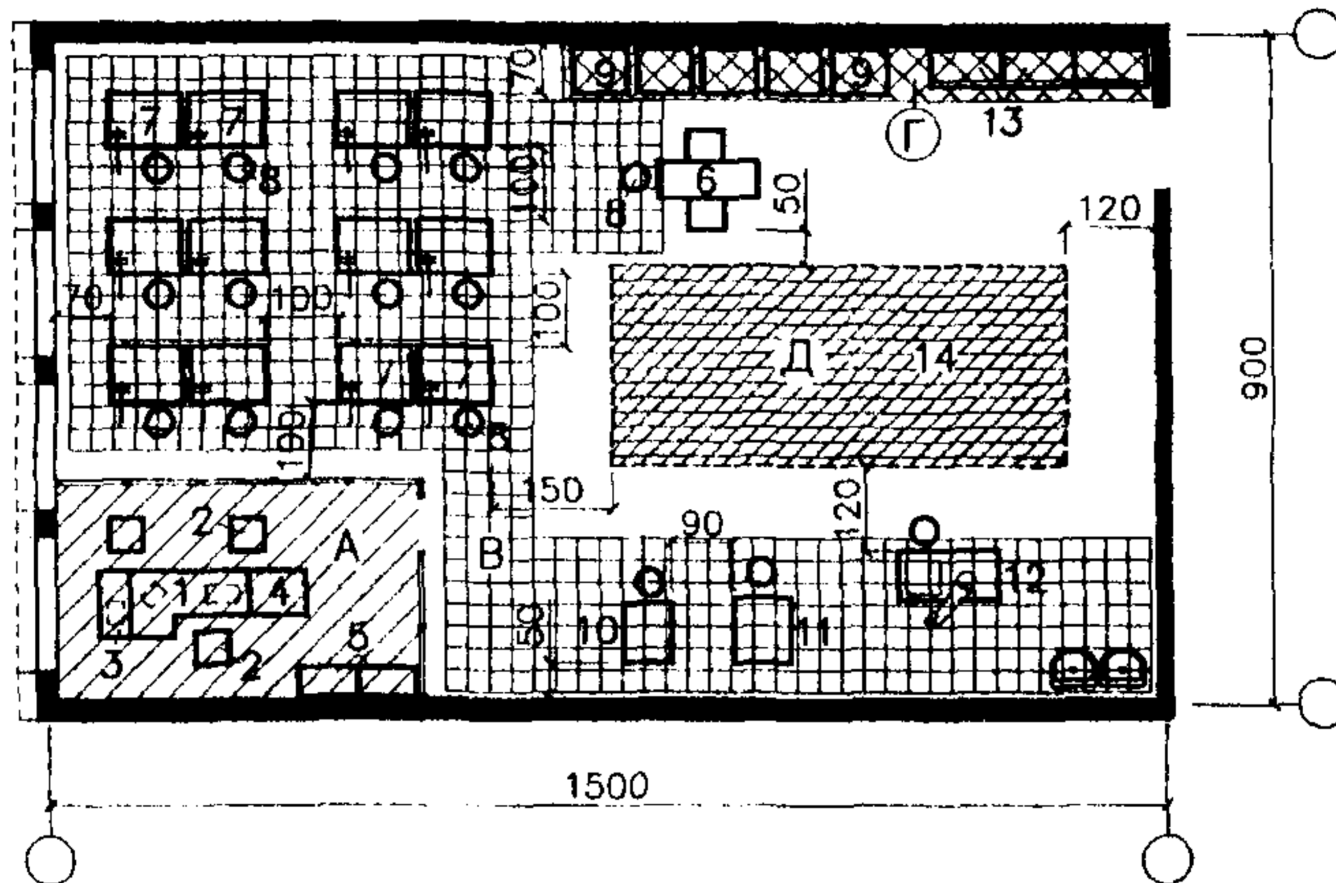
Рис.7. Зонирование учебно-производственных мастерских на примере слесарной (слесарно-сборочной) мастерской с размещением зоны преподавателя (мастера) за прозрачной звукозащитной перегородкой.
