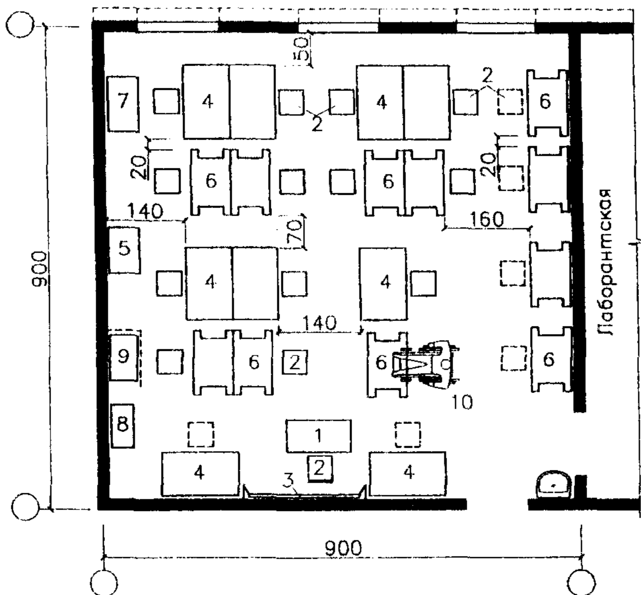
Рис.13. Пример планировки лаборатории промышленного электрооборудования на 12 мест.
