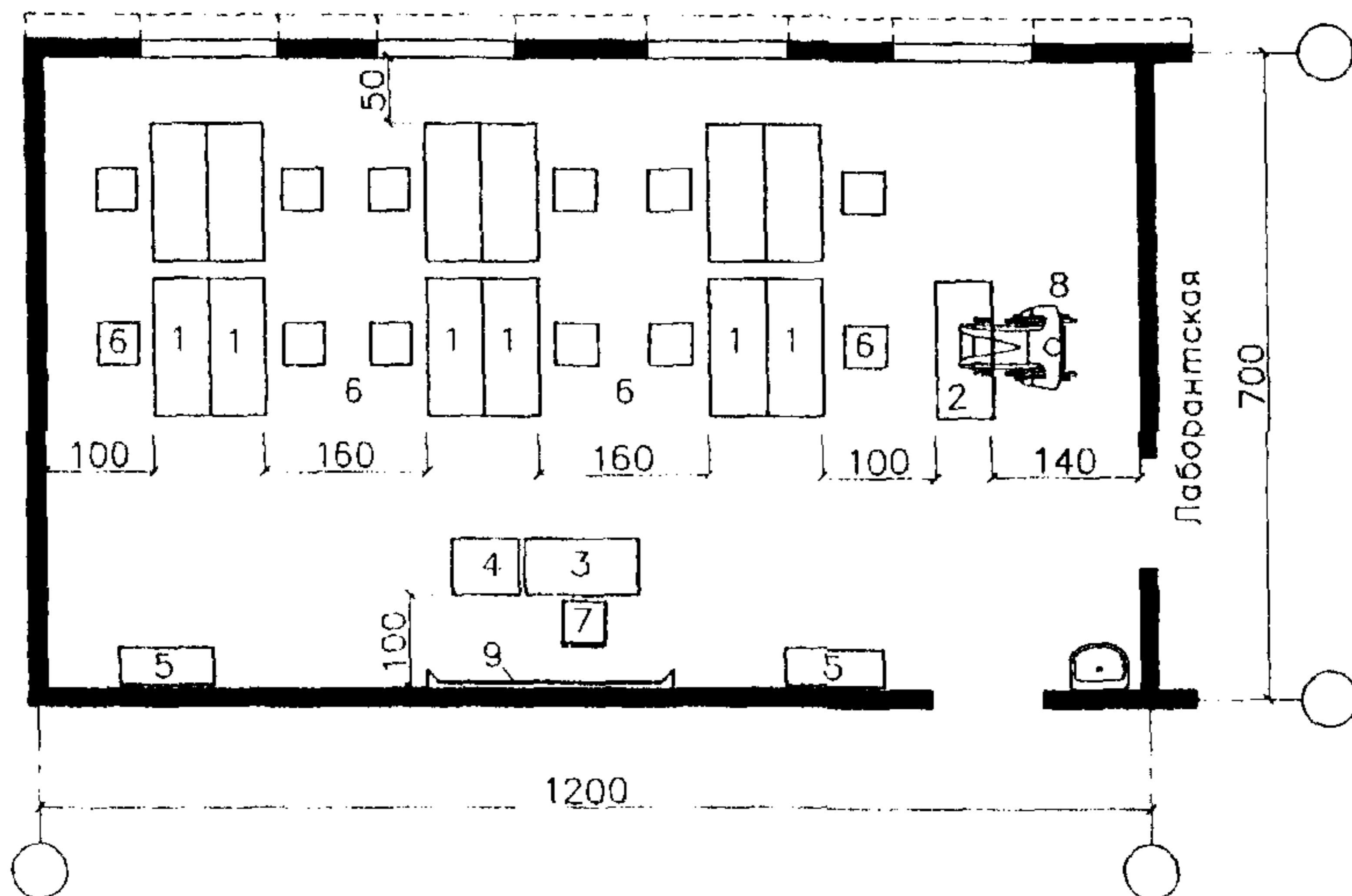
Рис. 14. Пример планировки лаборатории технической механики на 12 мест.
