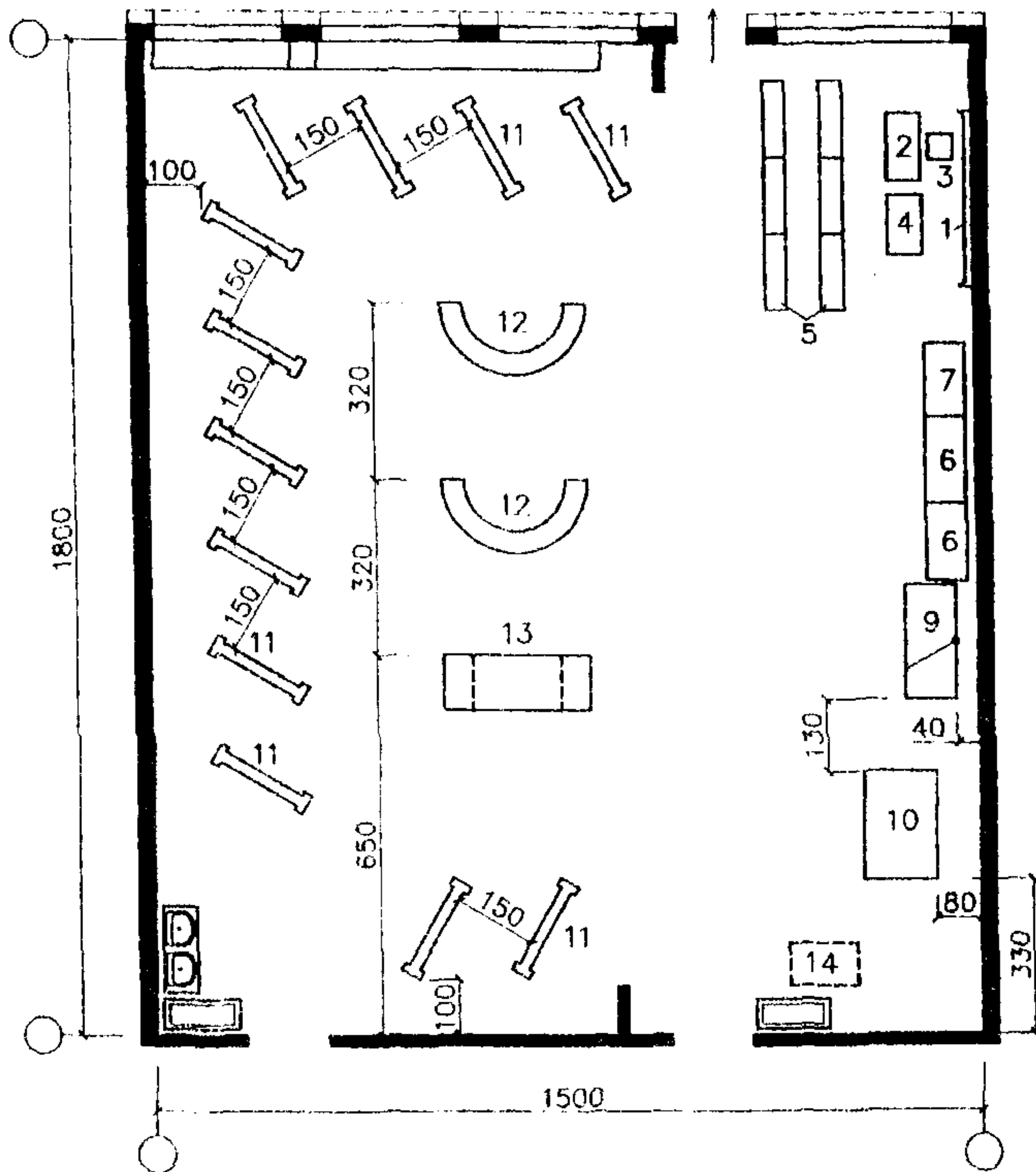
Рис.39. Пример планировки учебно-производственной мастерской плиточников на 12 мест.
