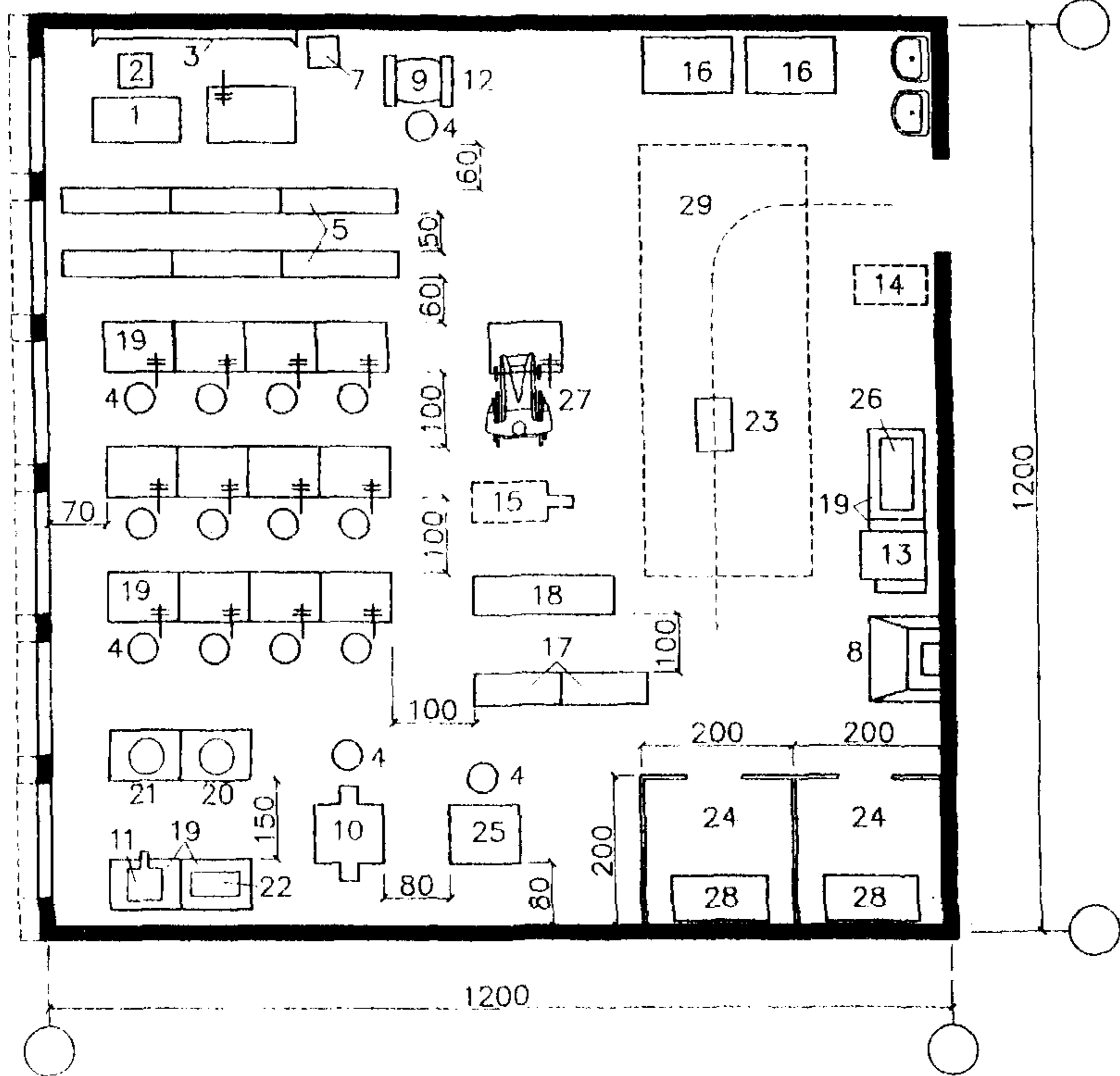
Рис.24. Пример планировки учебно-производственной электромонтажной мастерской на 12 мест.
