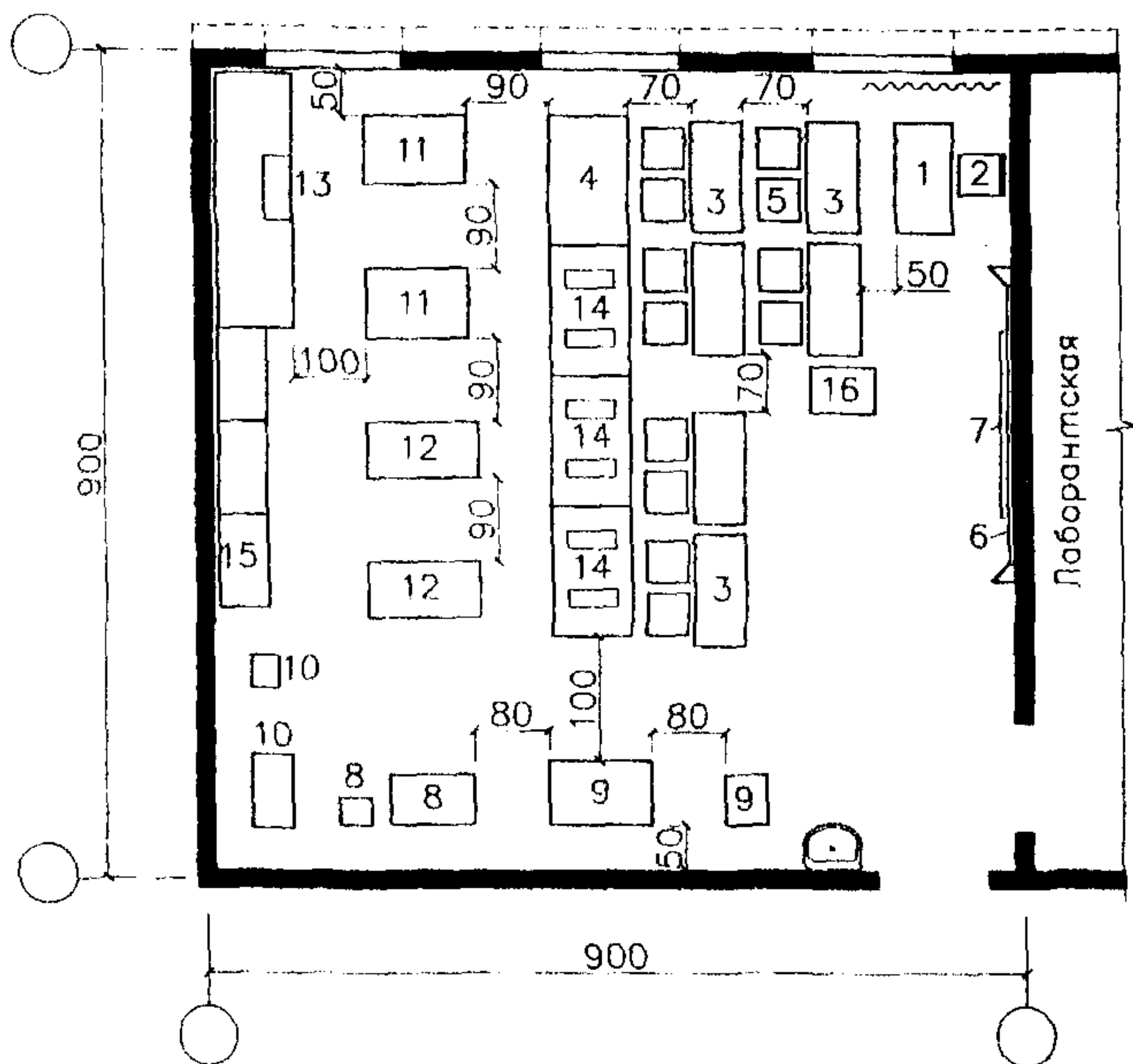
Рис.18. Пример планировки лаборатории сопротивления материалов на 12 мест.
