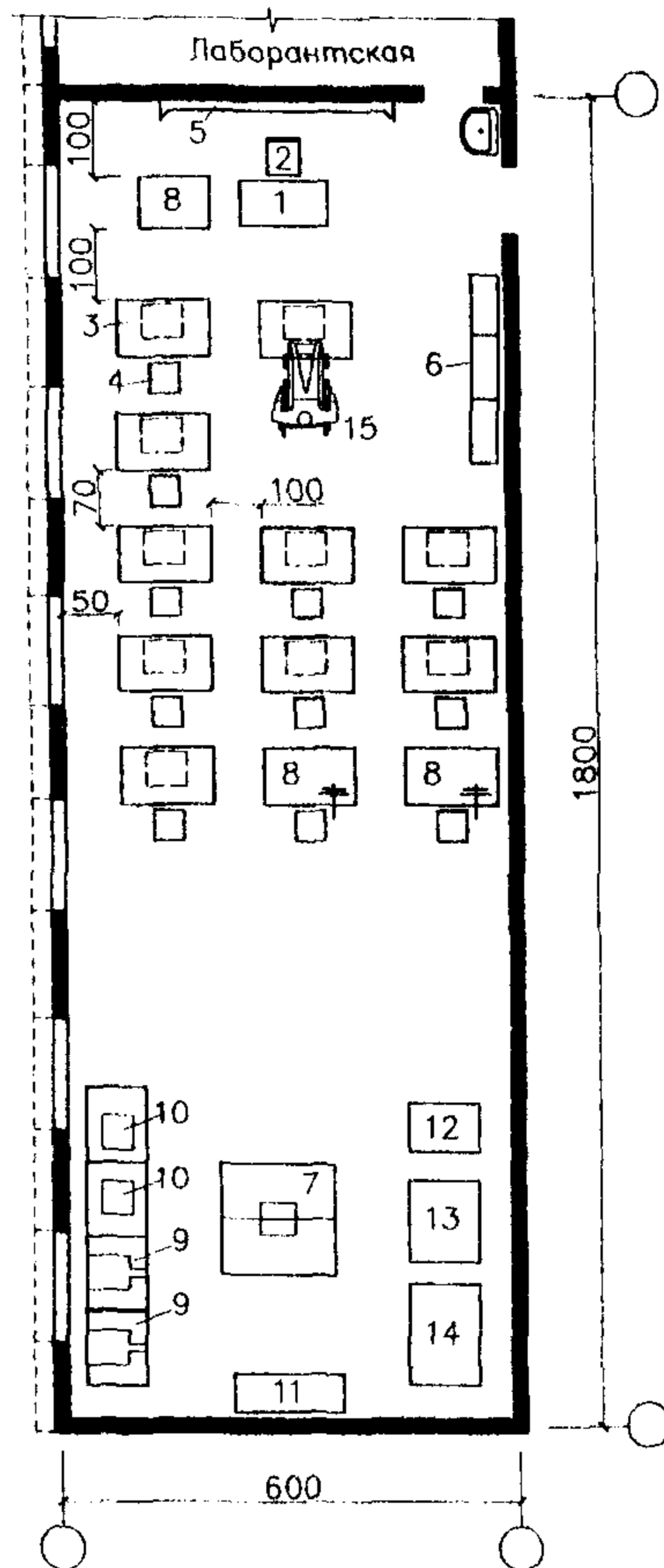
Рис. 15. Пример планировки лаборатории основ автоматизации производства и контрольно-измерительных приборов на 12 мест.
