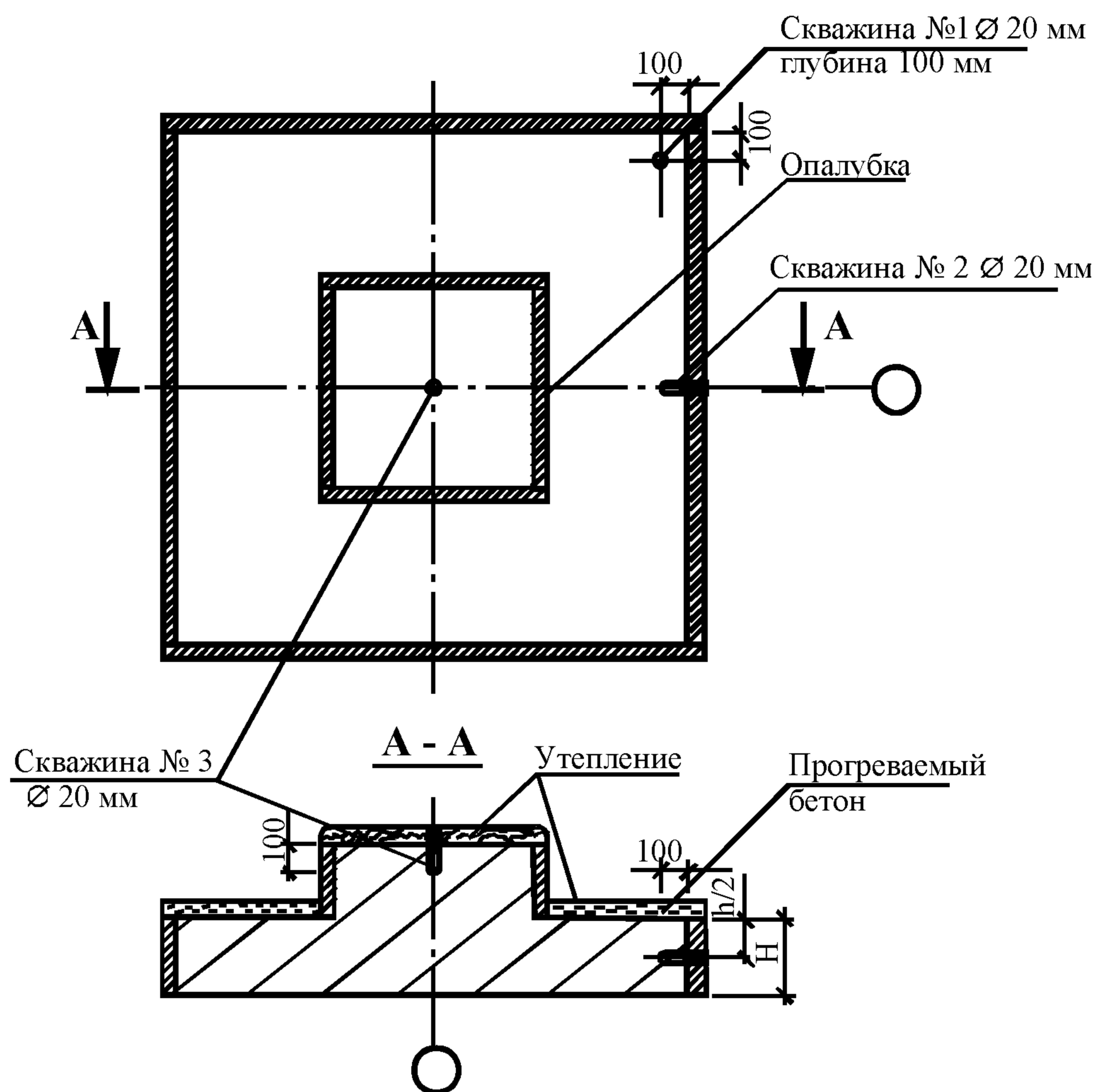
Рисунок 4 – Схема расстановки температурных скважин
