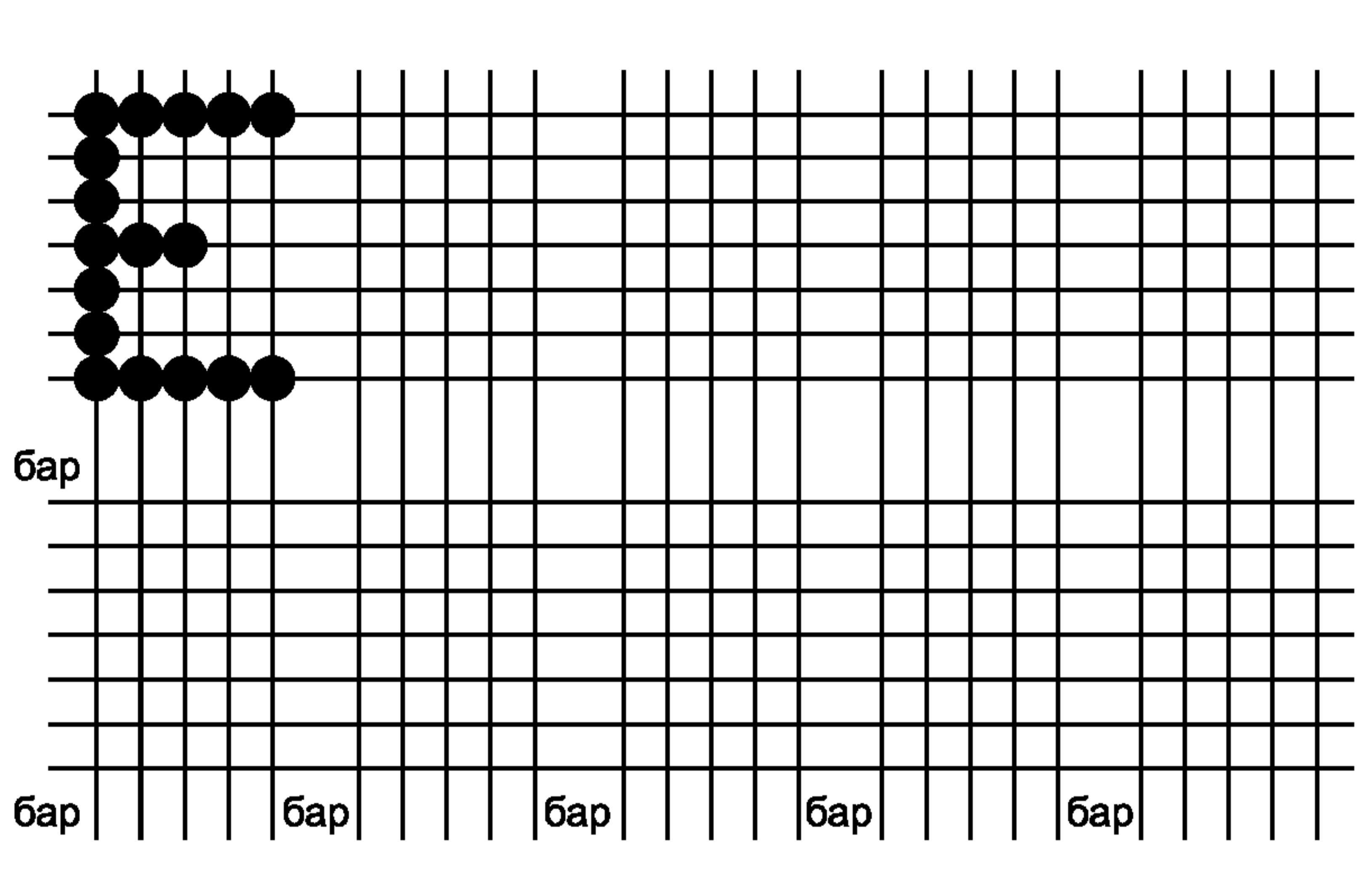
Рисунок 2 — Дисплей с промежутками между символами
