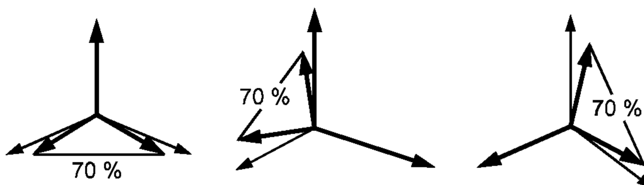
в) Испытания «фаза — фаза» — допустимый метод 2
