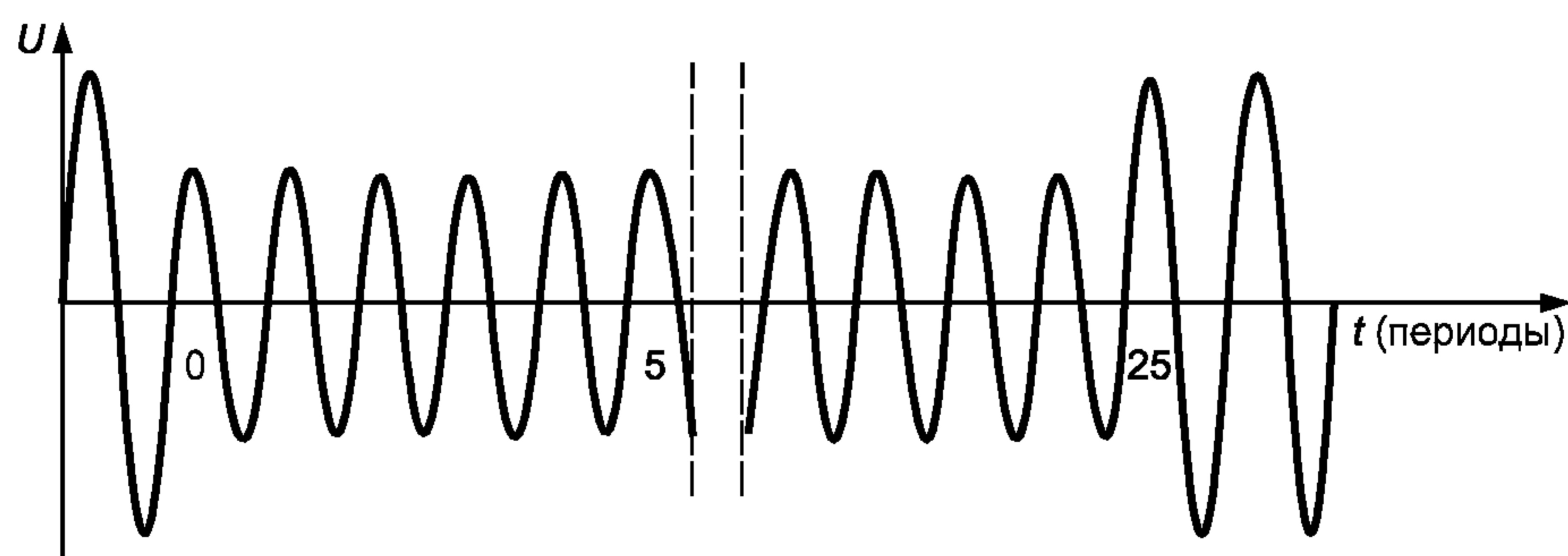
П р и м е ч а н и е — Напряжение понижается до 70 % U_T в течение 25 периодов при переходе через нуль
