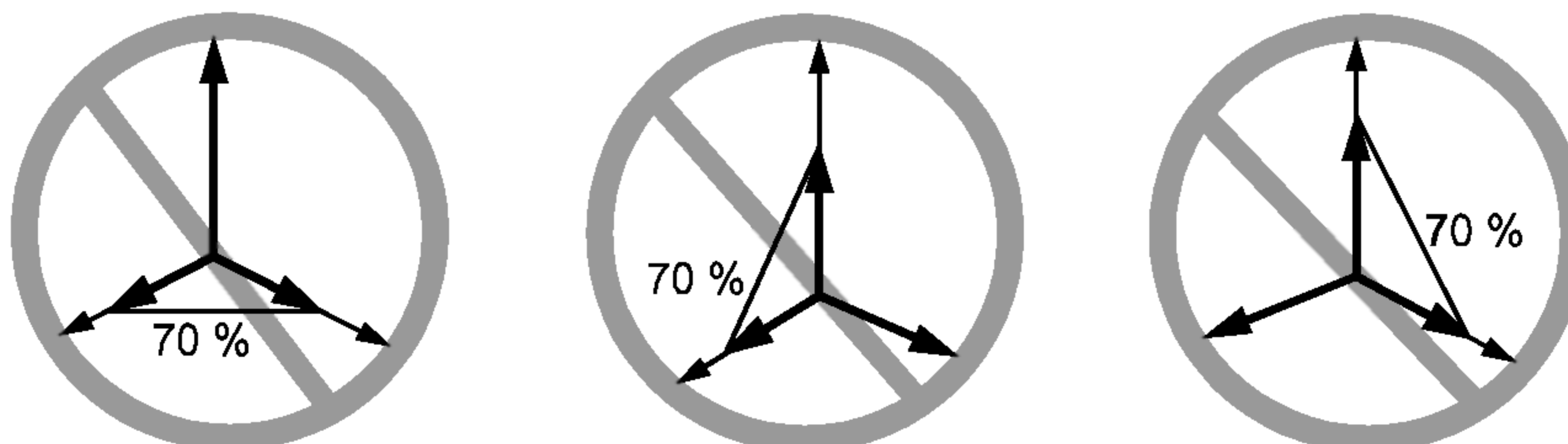
г) Испытания «фаза — фаза» без фазового сдвига (неприемлемый метод)
