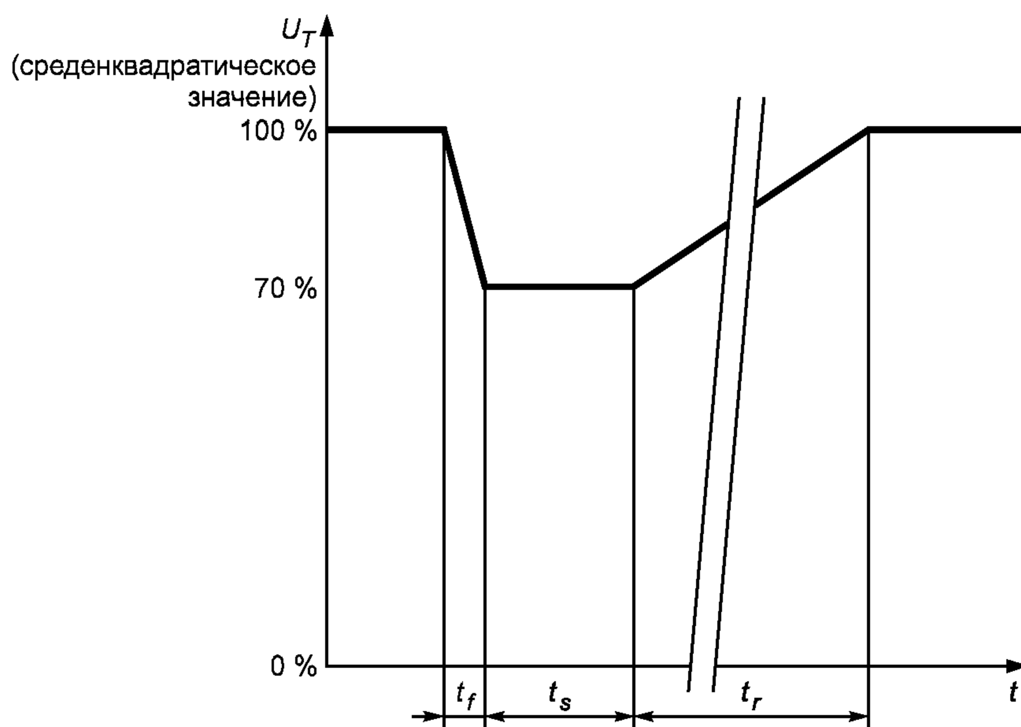
Рисунок 1 — Провал напряжения 70 % U_T
