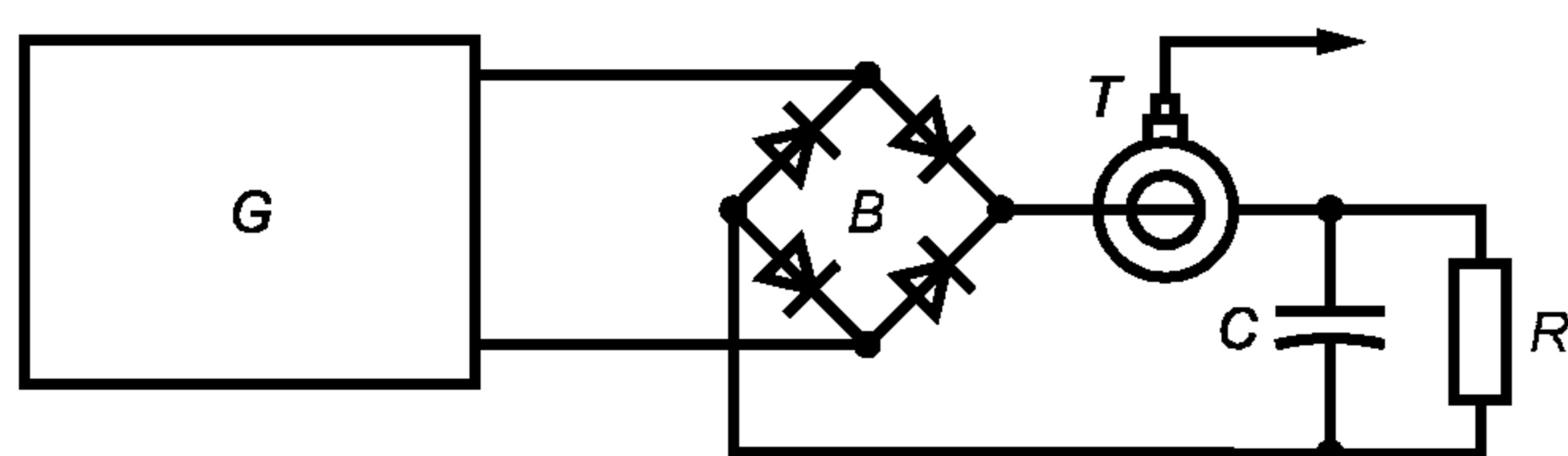
Рисунок А.1— Схема измерения пикового значения нагрузочного тока ИГ
