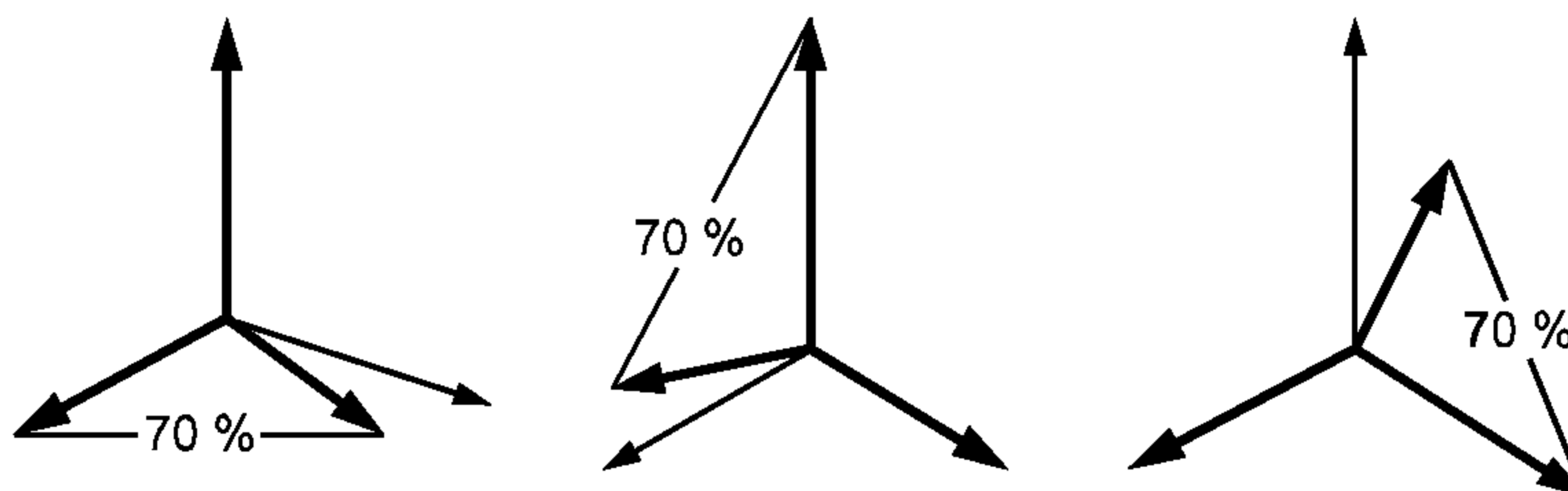
а) Испытание «фаза — нейтраль»
