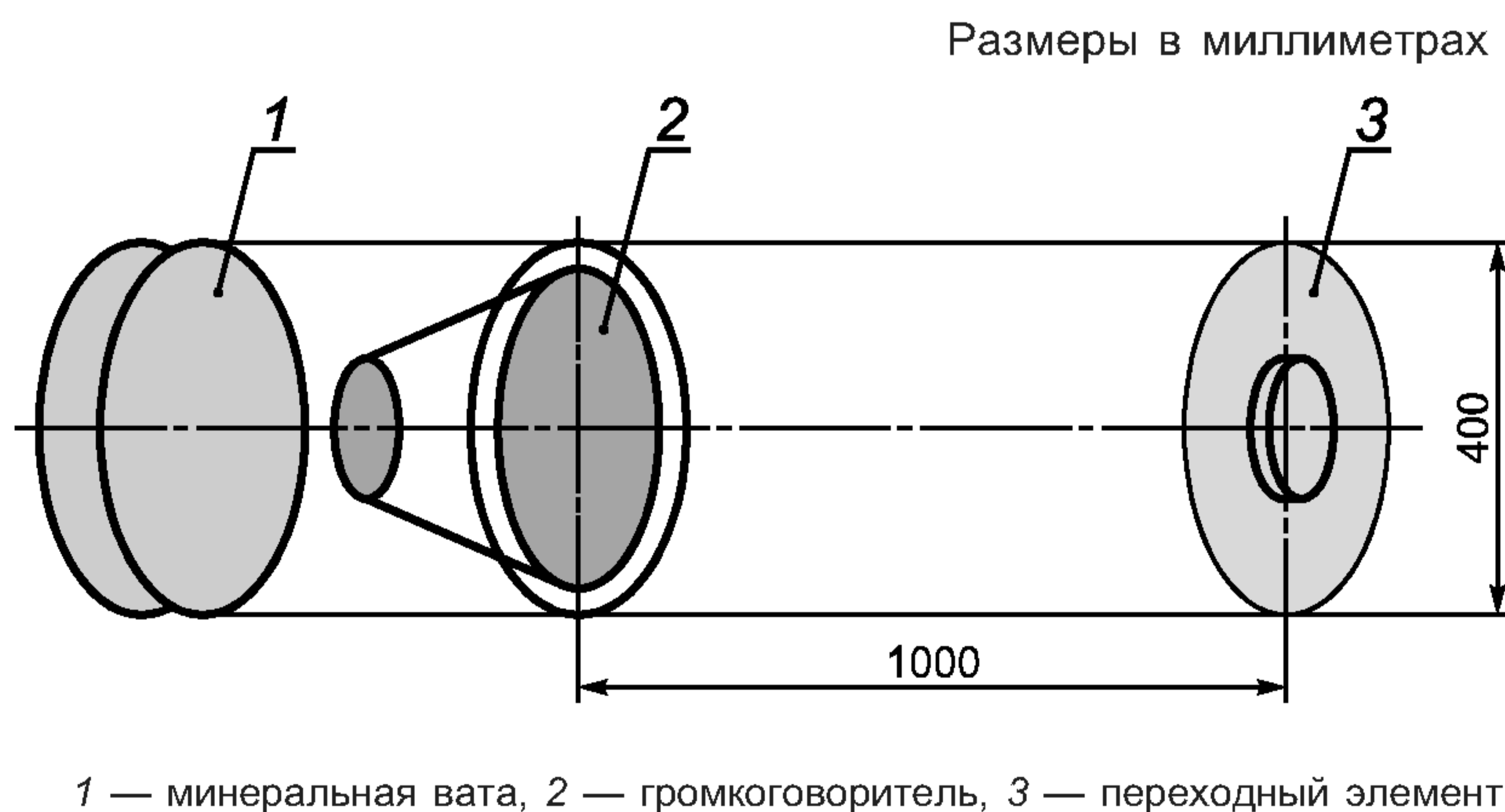
Рисунок 2 — Источник звука
