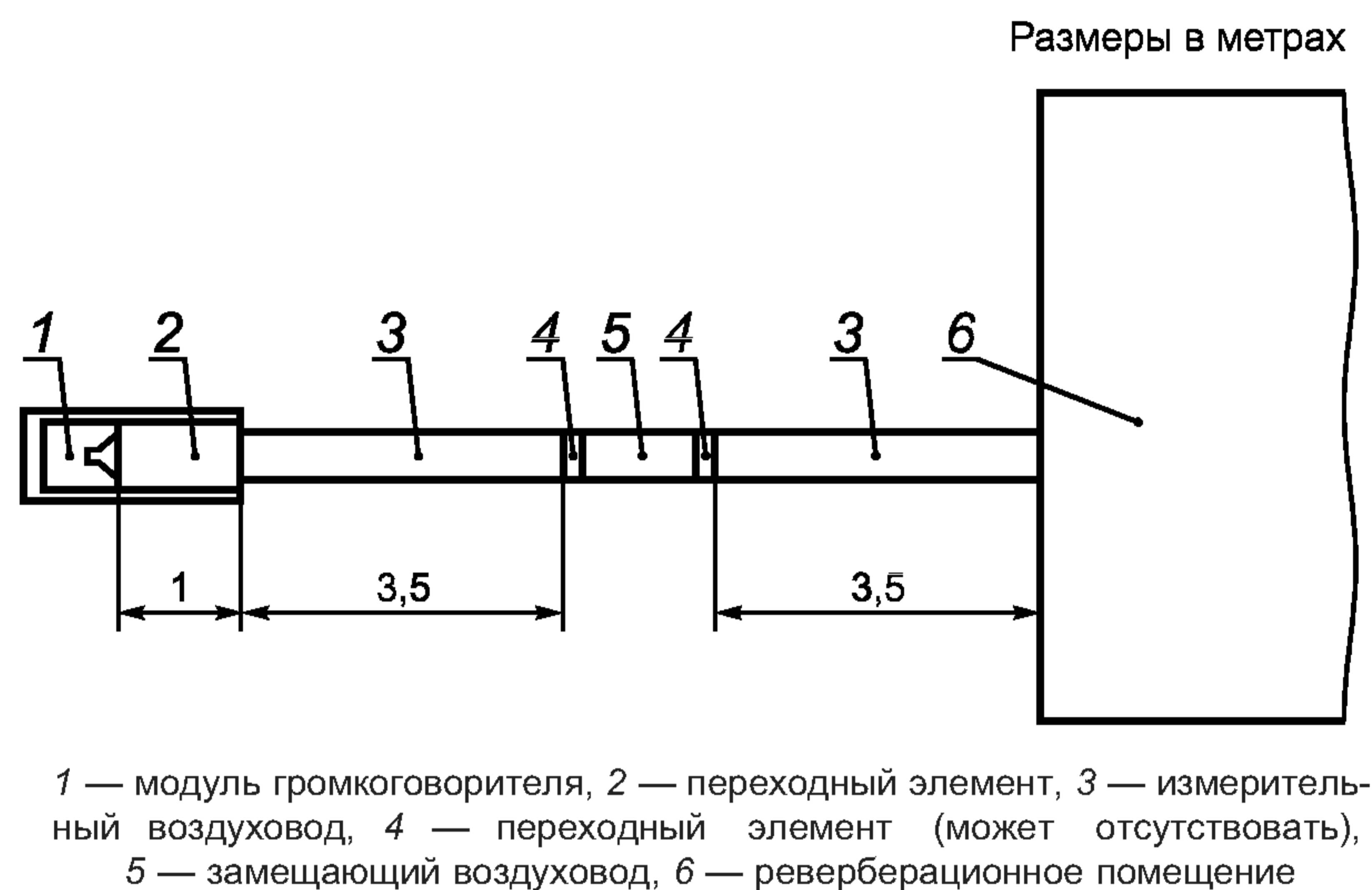
Рисунок 1 — Испытательная установка
