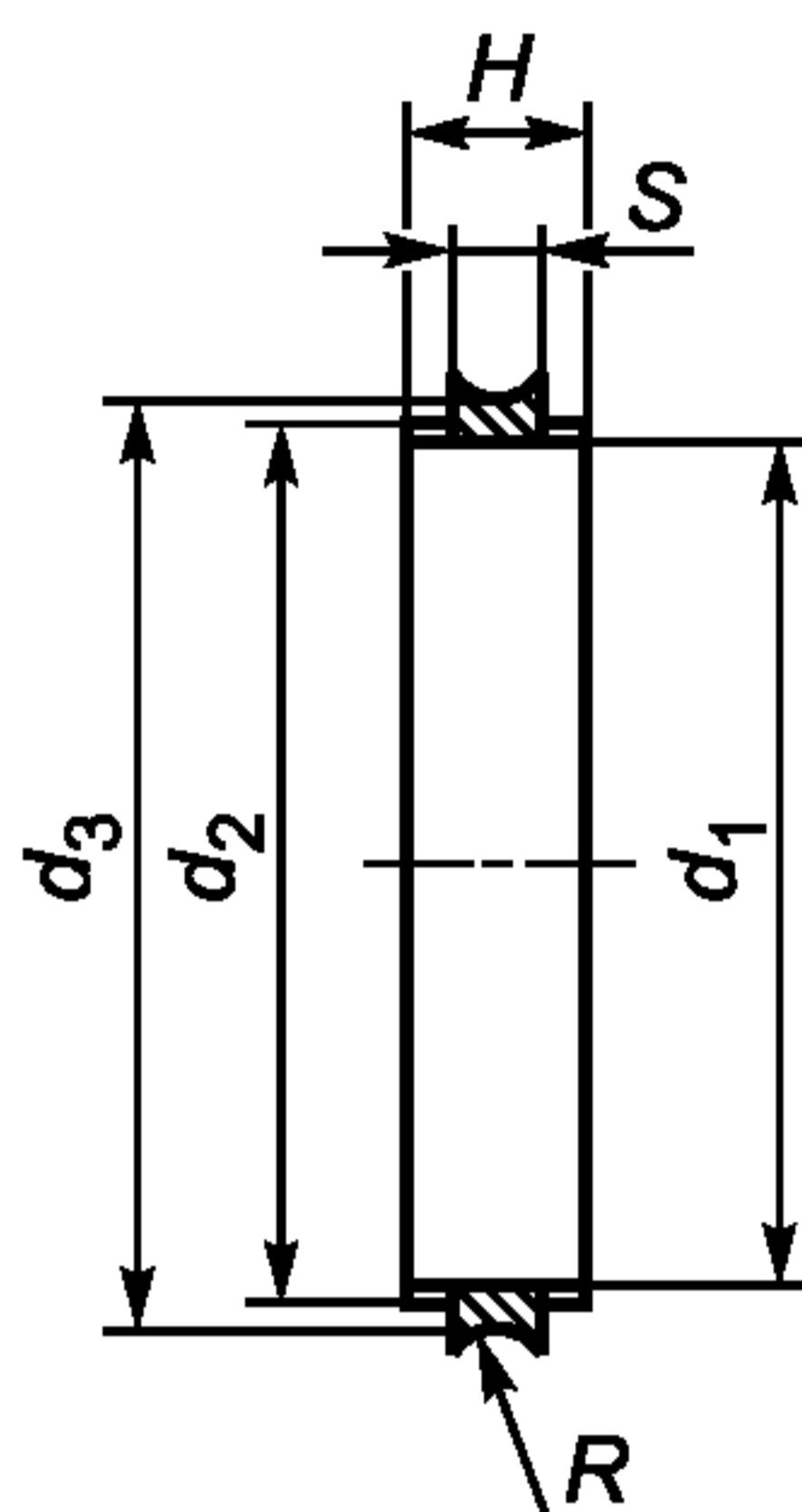
Рисунок В.1 — Центрирующее кольцо
