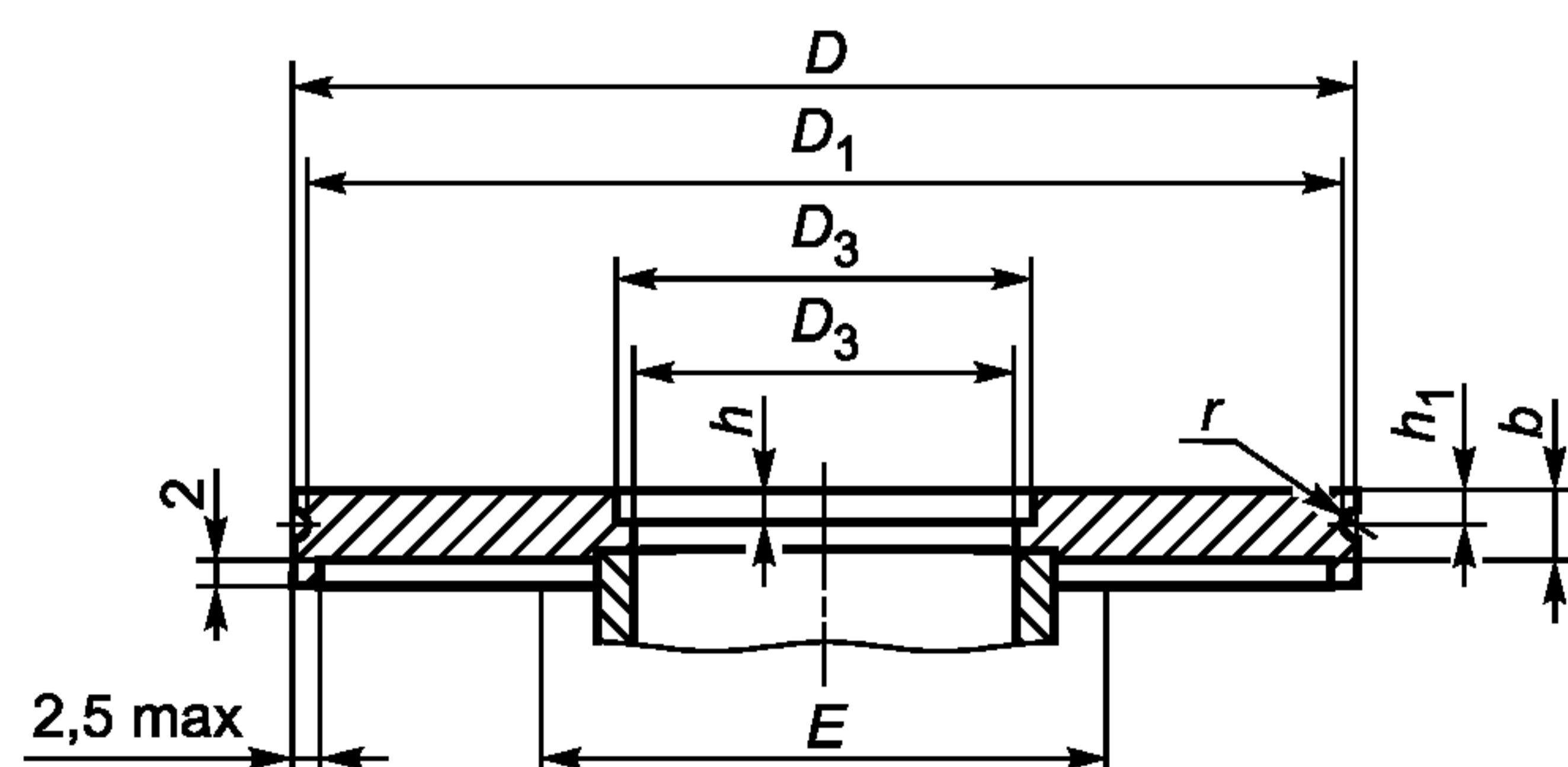
Рисунок 2 — Опорный фланец
