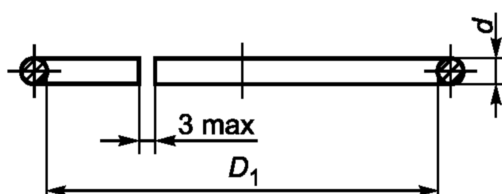
Рисунок 4 — Установочное кольцо
