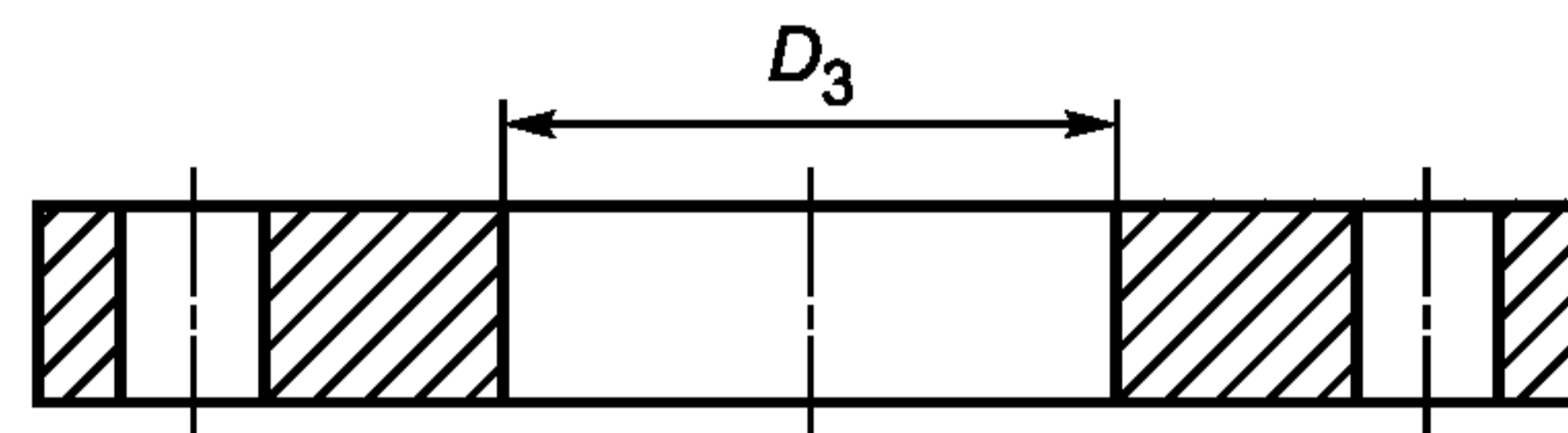
Рисунок Б.1 — Расточка фланца
