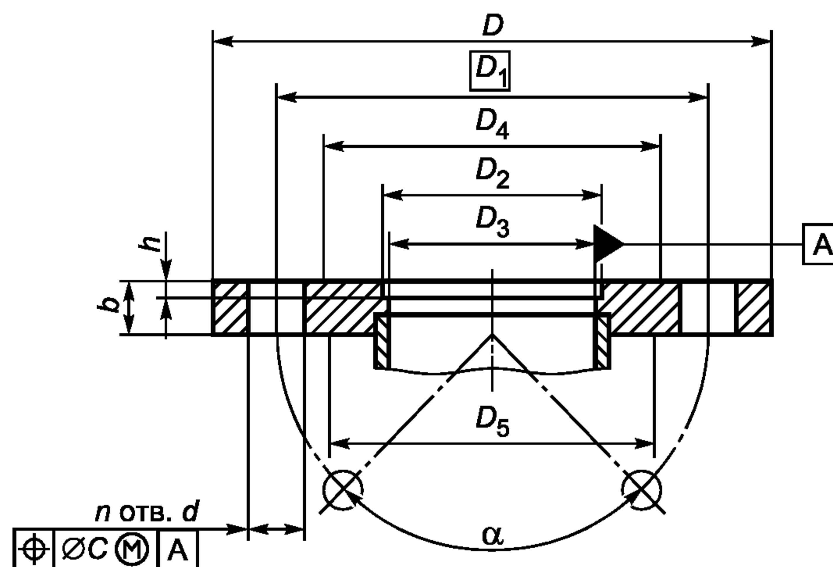
Рисунок 1 — Неподвижный фланец
