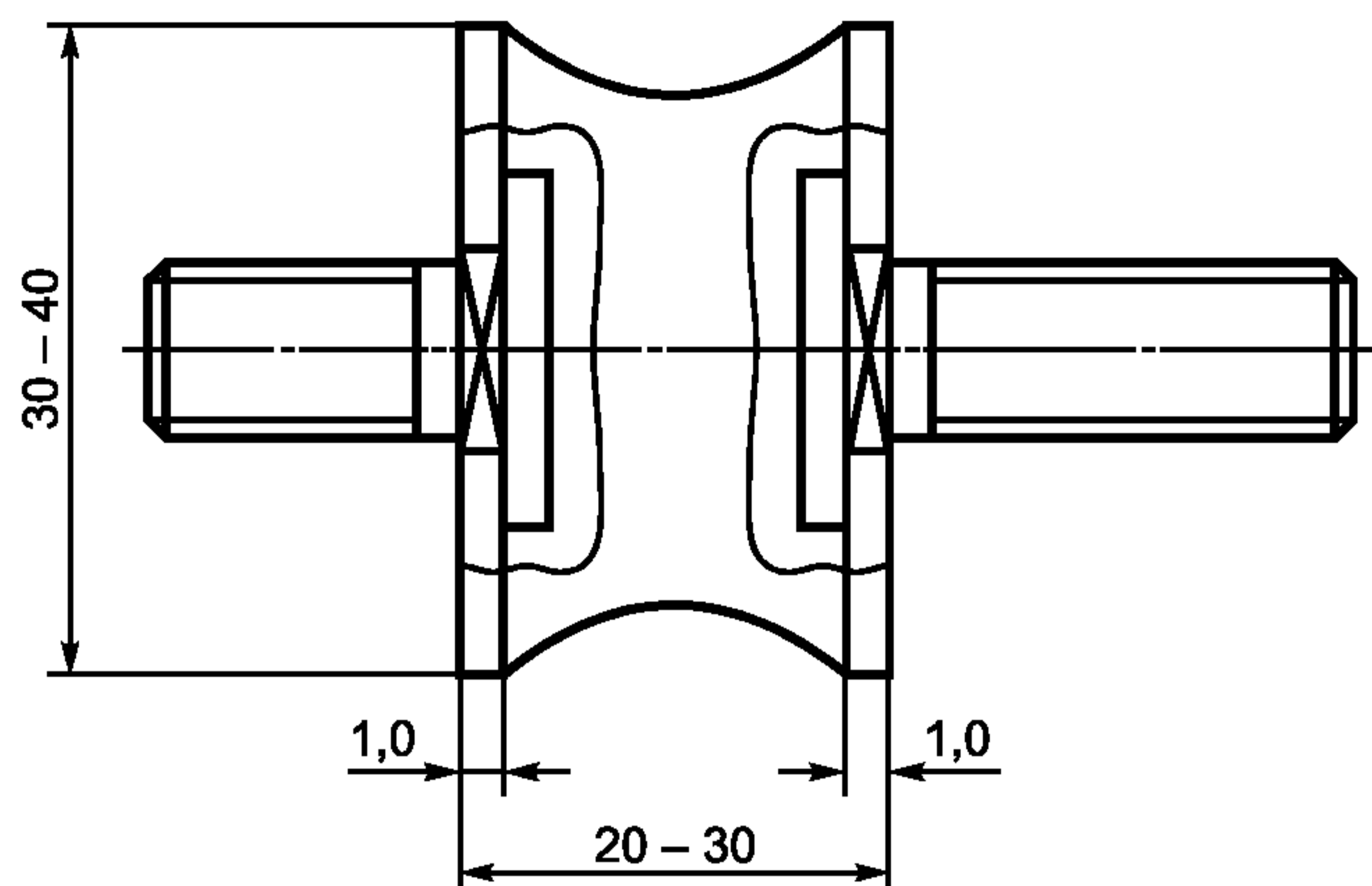
Рисунок 4 — Типовая резиновая втулка для крепления испытательной лестницы
