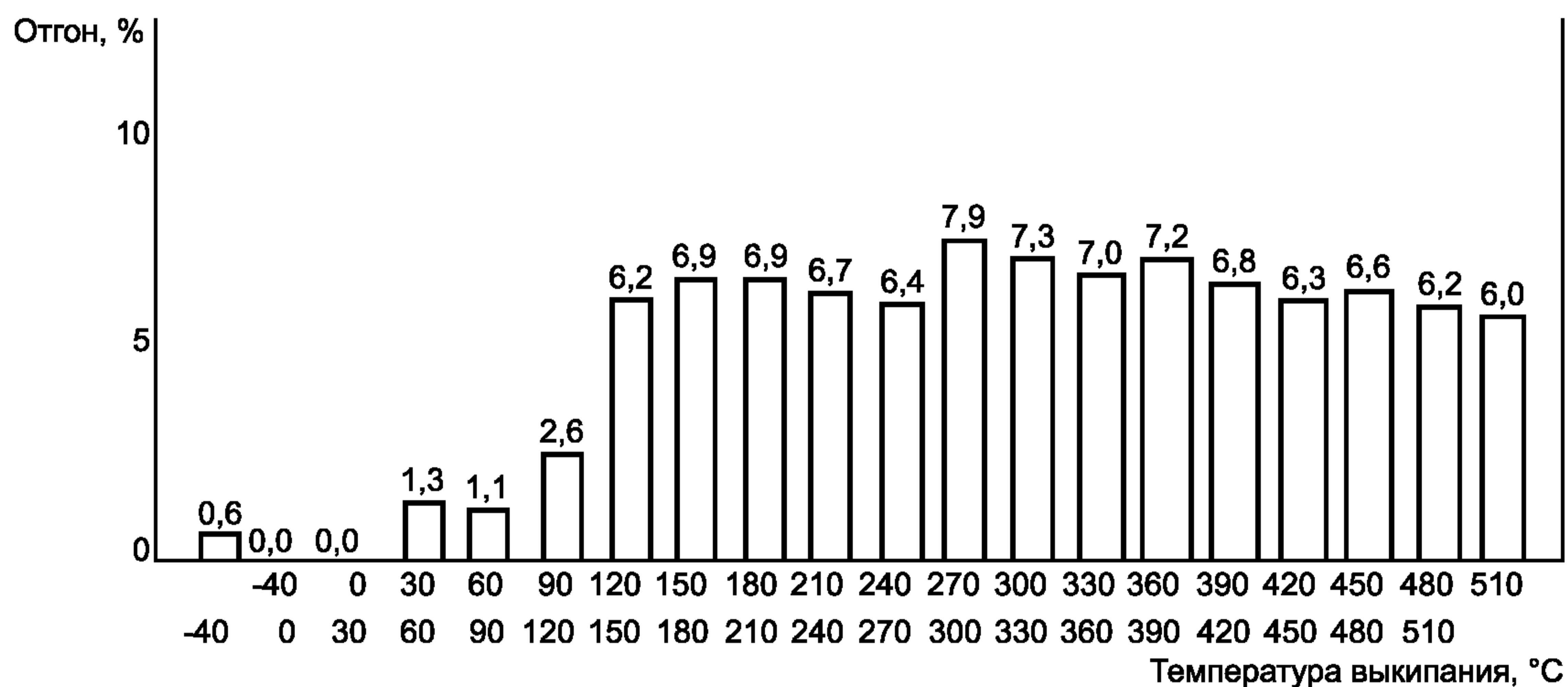
Рисунок А.2 — Диаграмма кривой распределения фракций по температурам выкипания саратовской нефти
