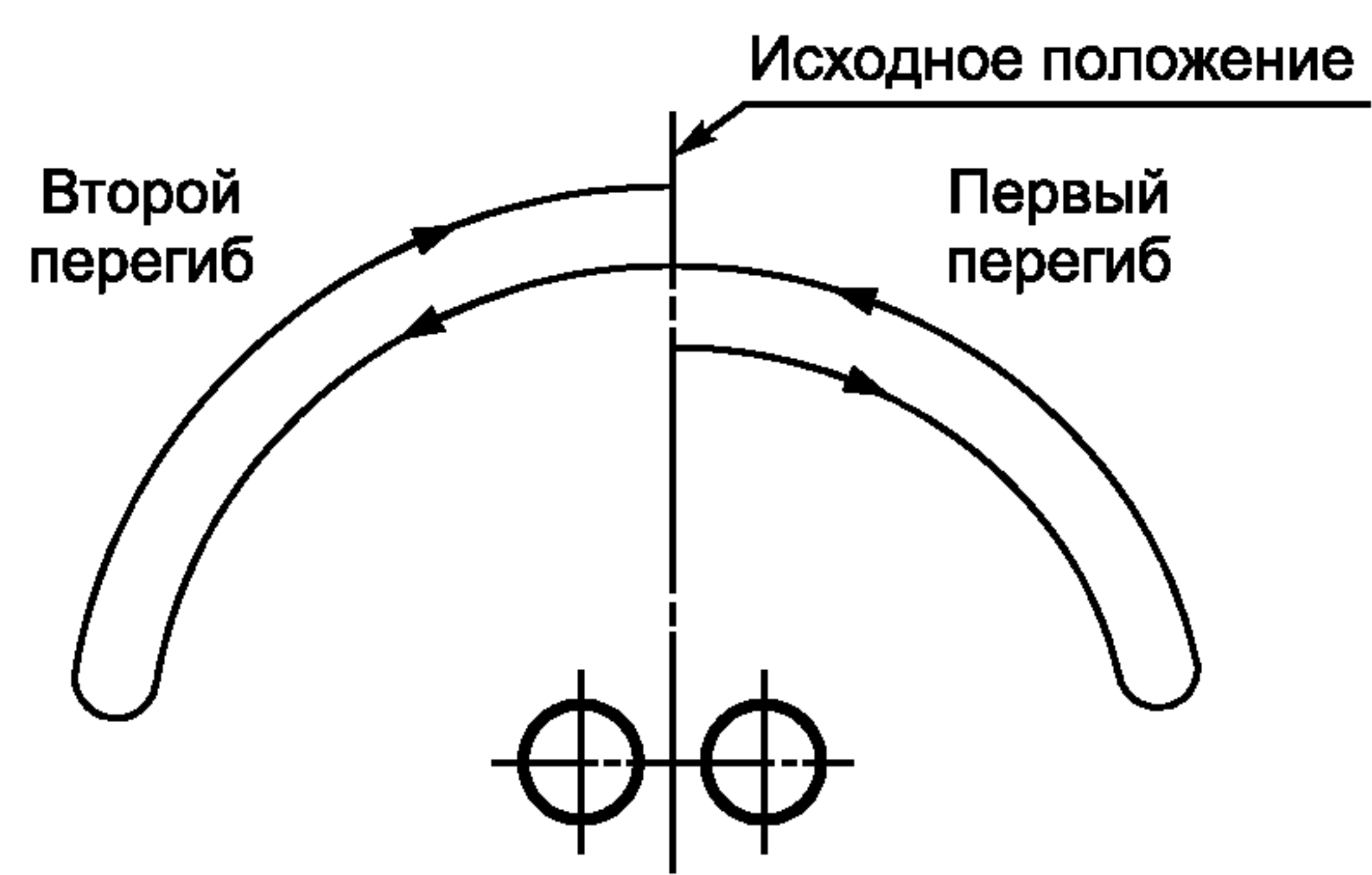
Рисунок 1 — Схема испытания на перегиб
