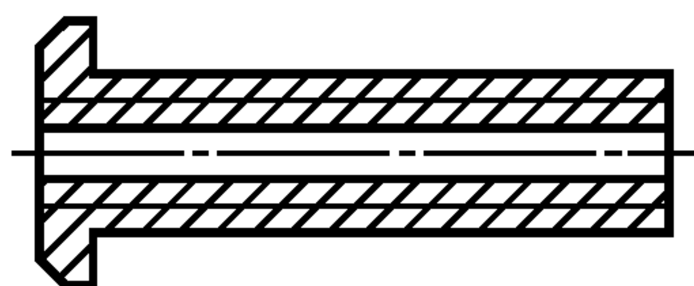
Рисунок Б.1 — Корпус шипа без износостойкого элемента
