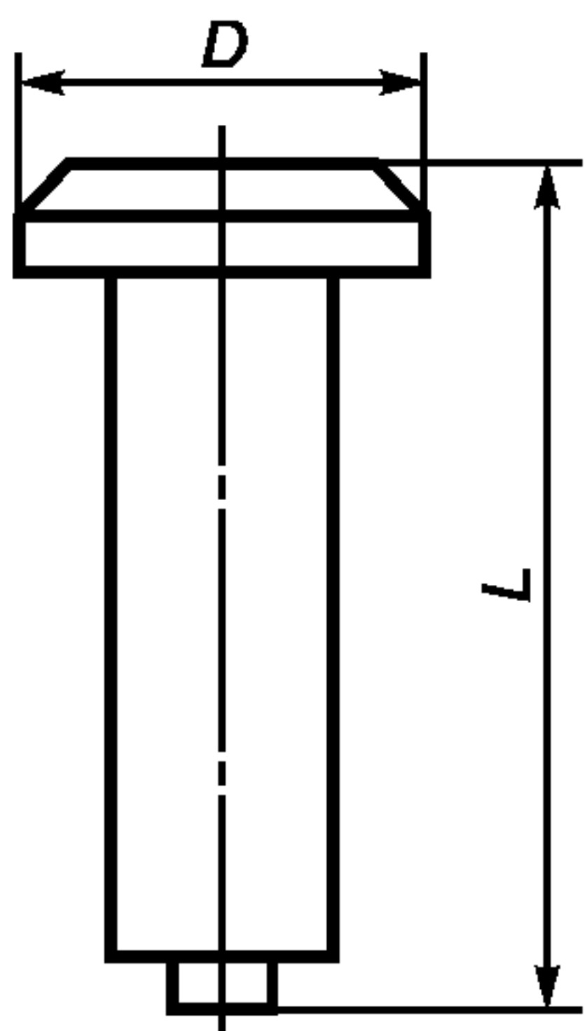
D — диаметр наибольшего фланца; L — длина шипа
