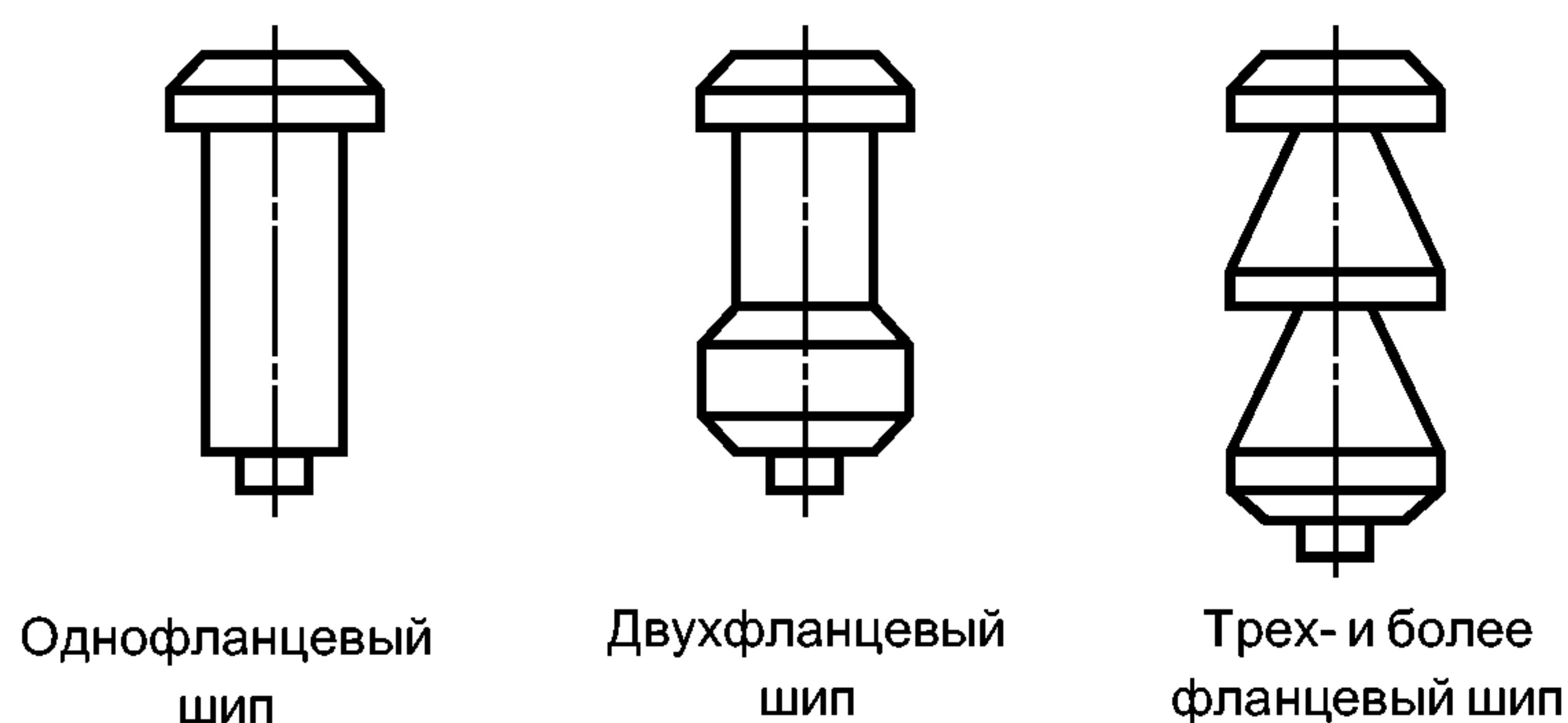
Рисунок 1 — Виды шипов по количеству фланцев
