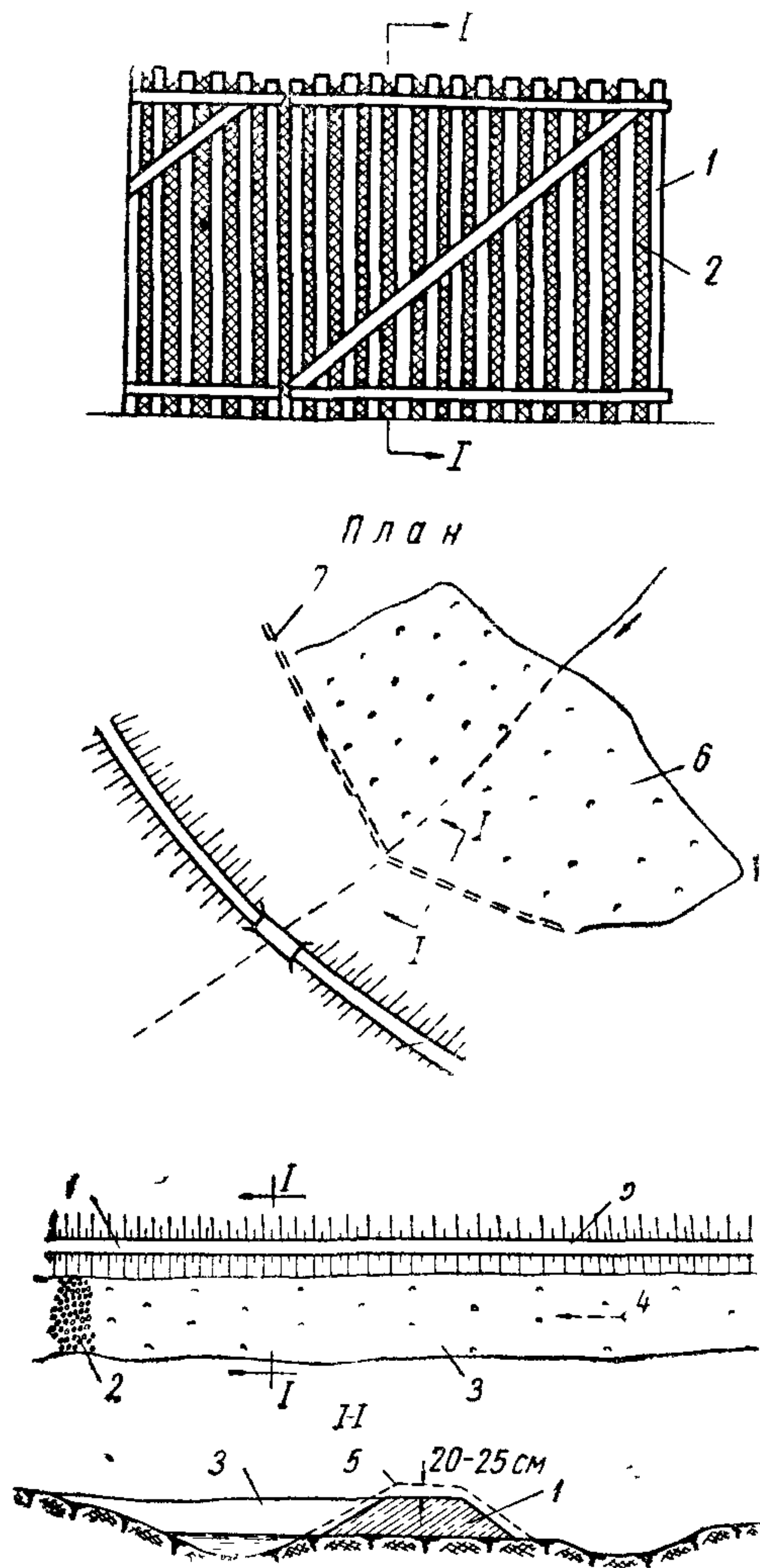
Рис. 9 Схема повышения высоты насыпи для защиты от естественно развивающихся речных наледей:
