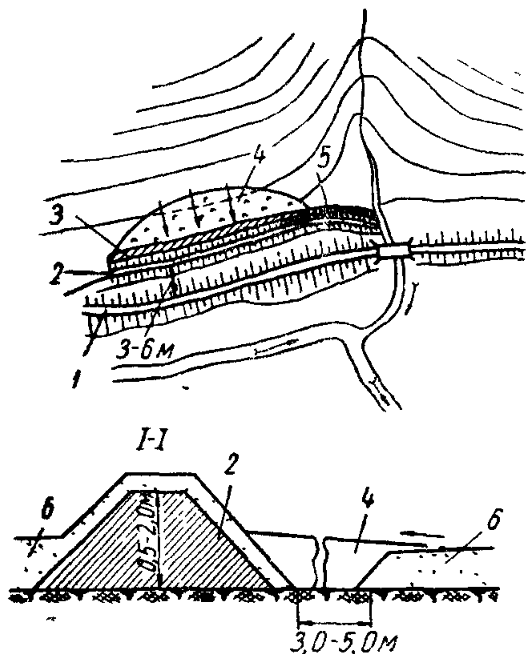
Рис. 7. Схема устройства задерживающих валов:
