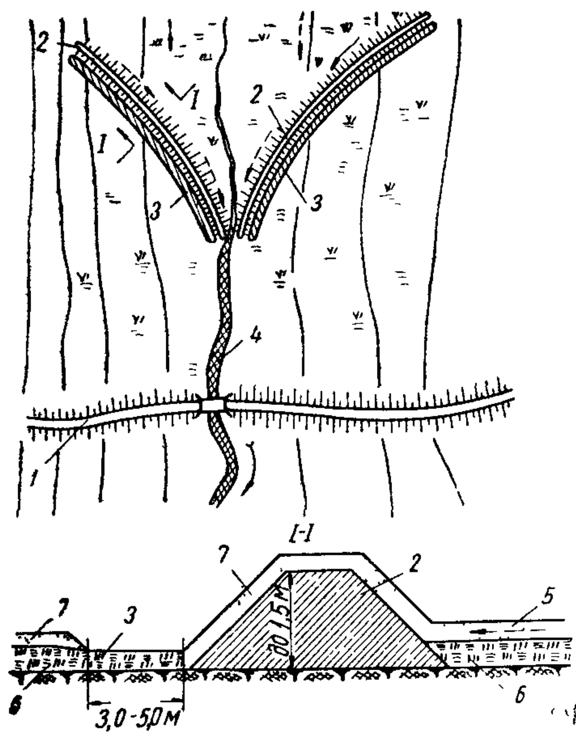
Рис. 4. Схема устройства направляющих валов:
