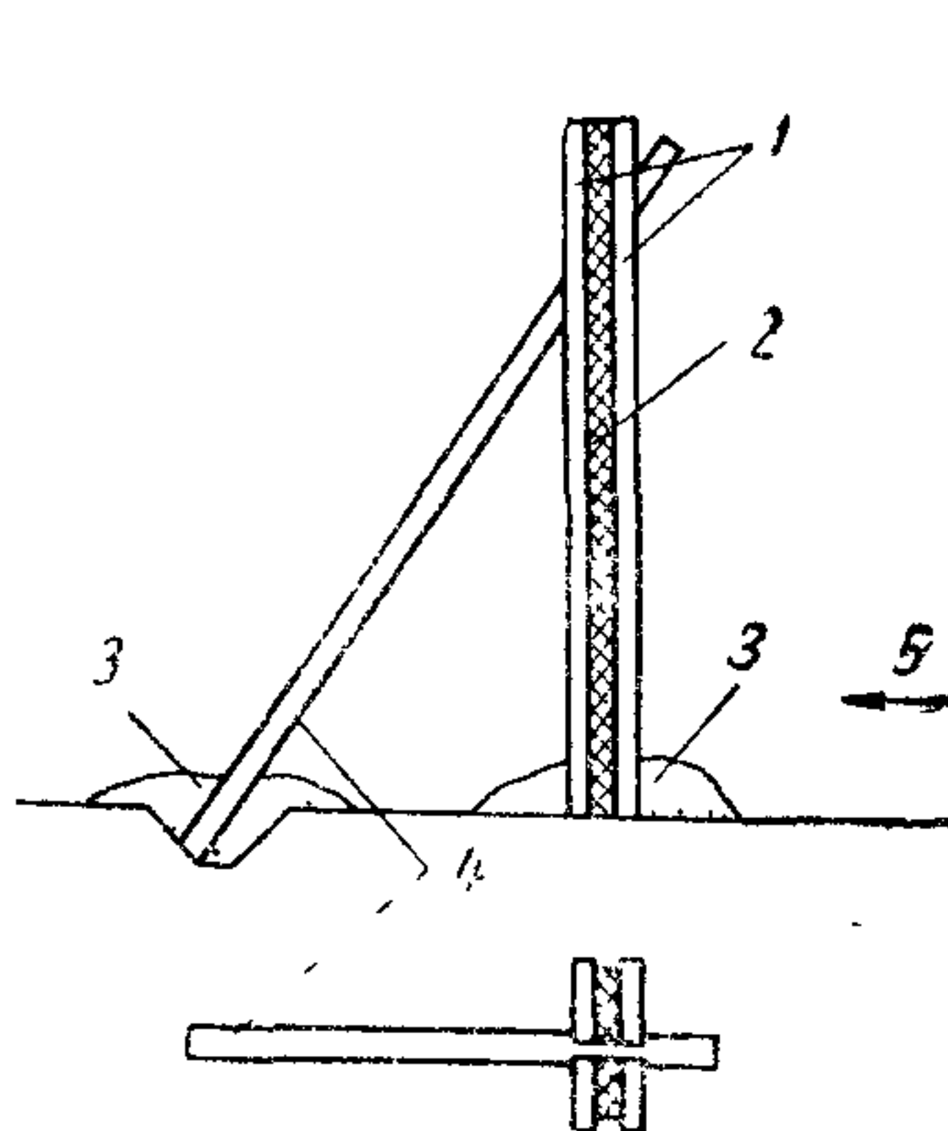
Рис. 8. Схема использования снегозадерживающих планочных щитов для задержания натечных наледей.
