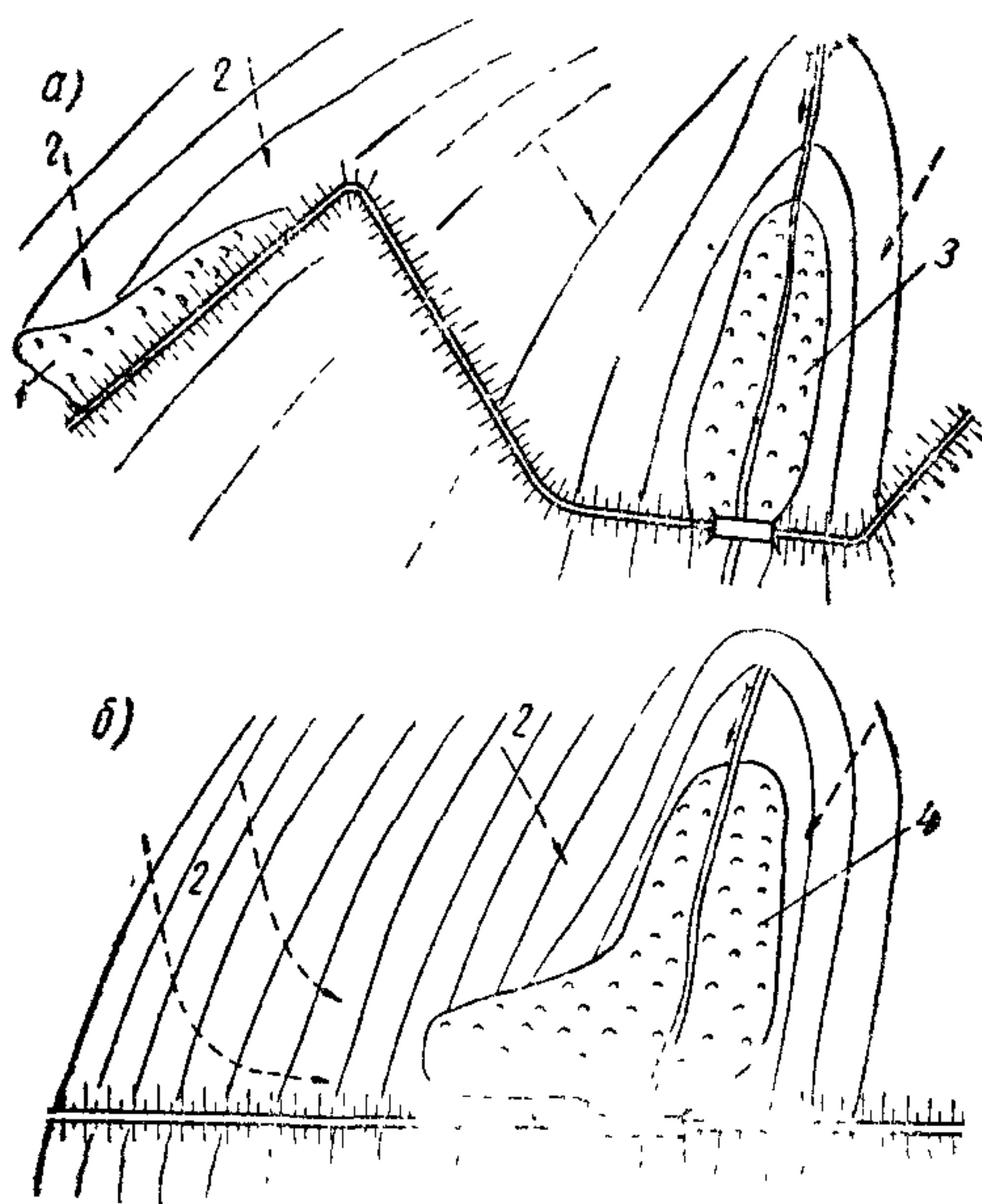
Рис. 3. Варианты пересечения трассой долины в наледных районах: а — по ломаной (с развитием трассы на склонах); б — по прямой;
