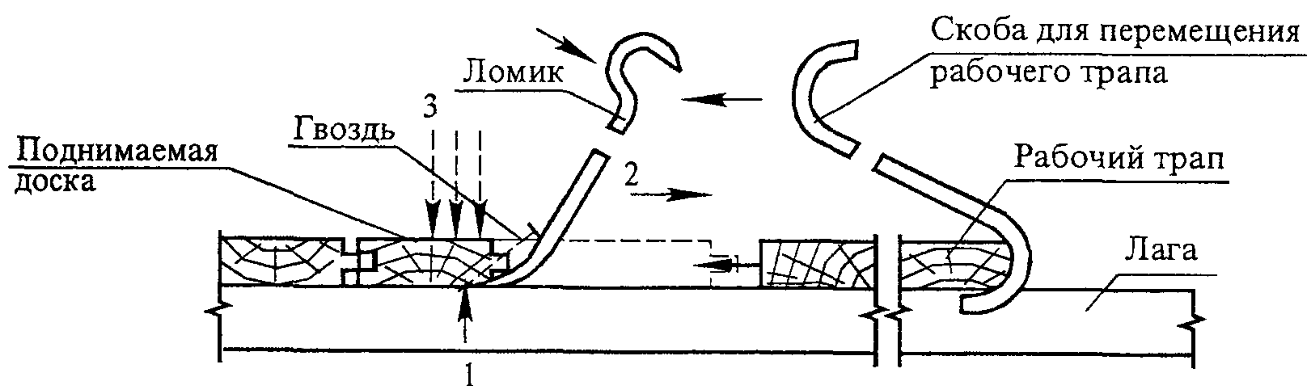
Деталь разборки
