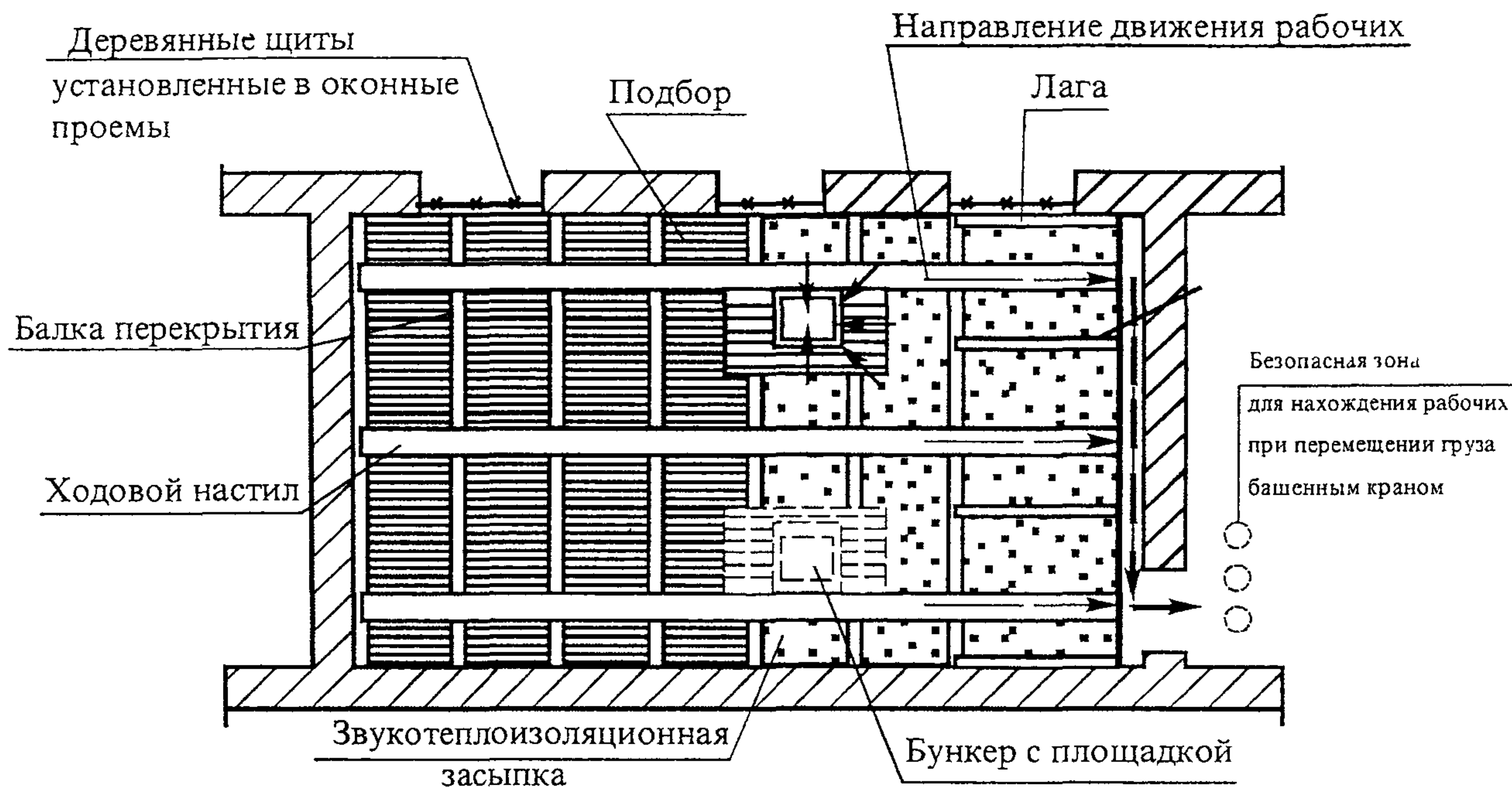
Рисунок 5 – Схема удаления звукоизоляции (засыпки) перекрытия
