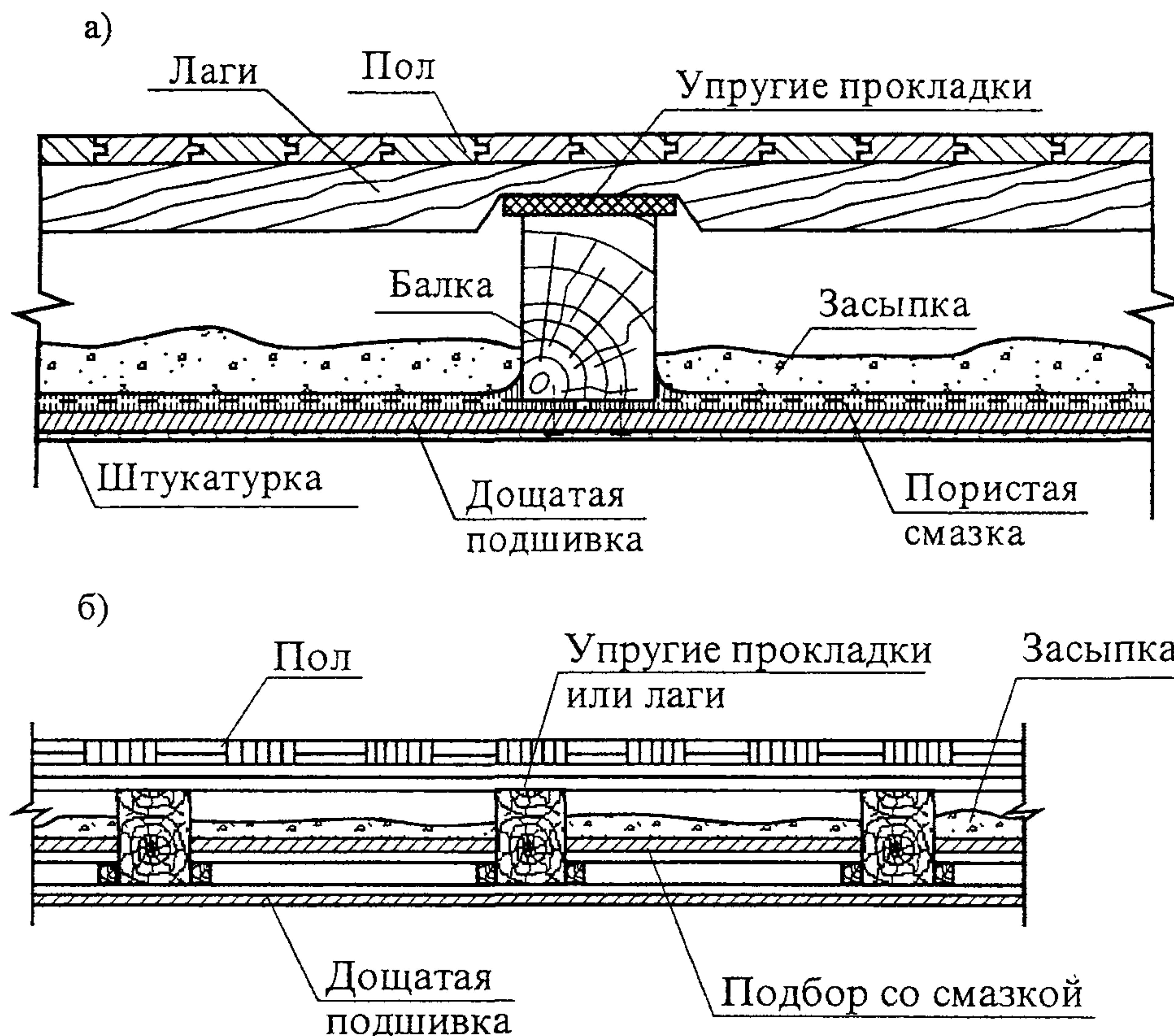
Рисунок 1 – Перекрытие по деревянным балкам с чистым полом из шпунтованных досок (а) и паркетным полом (б)
