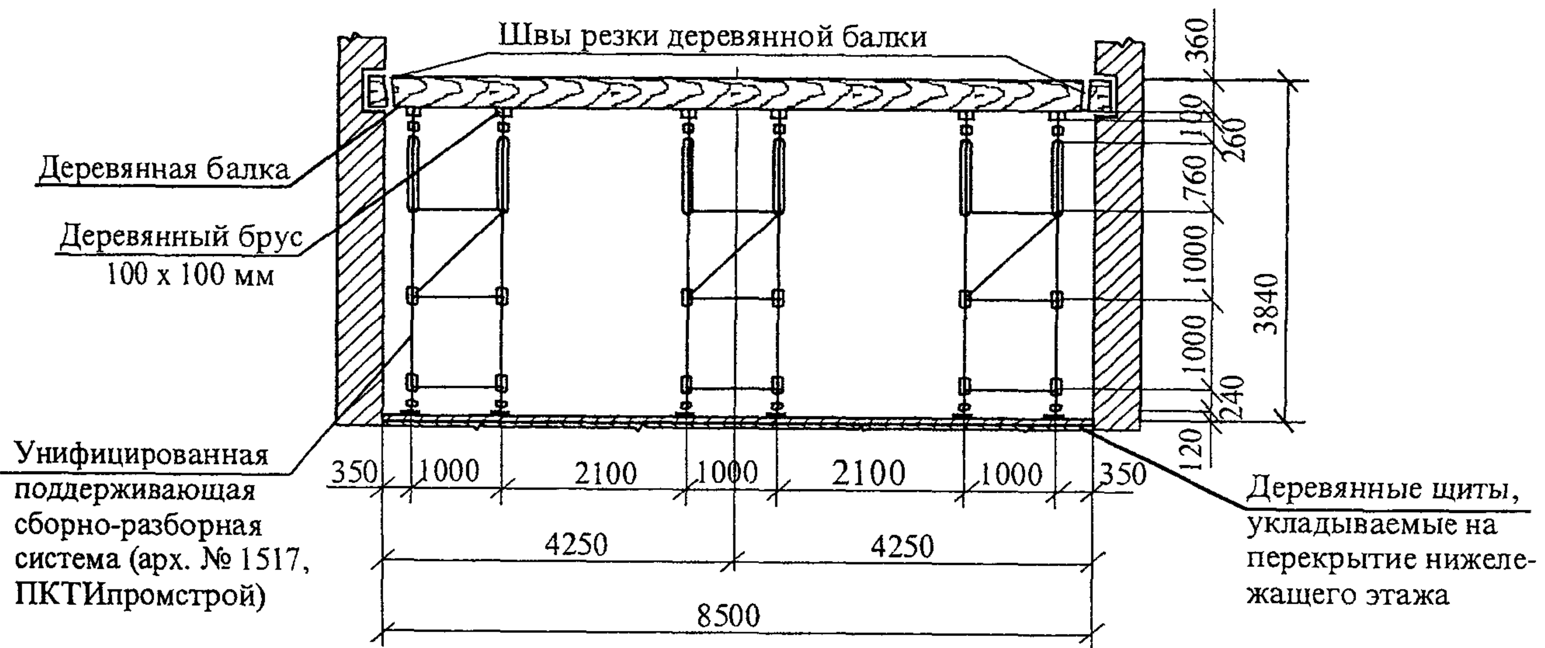
Рисунок 8 – Схема разборки междуэтажного перекрытия по деревянным балкам
