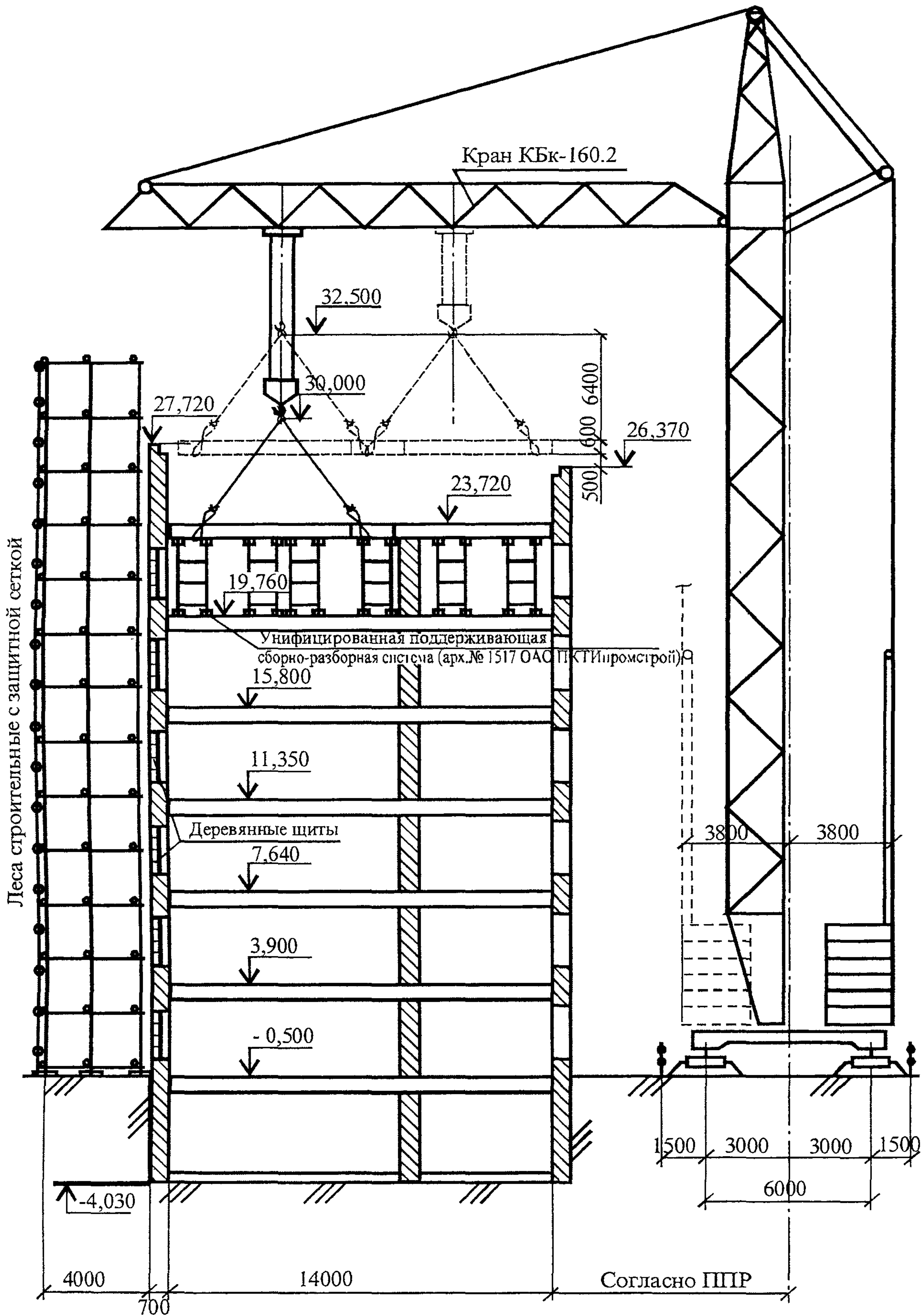
Рисунок 7 – Схема привязки крана на период разборки перекрытий
