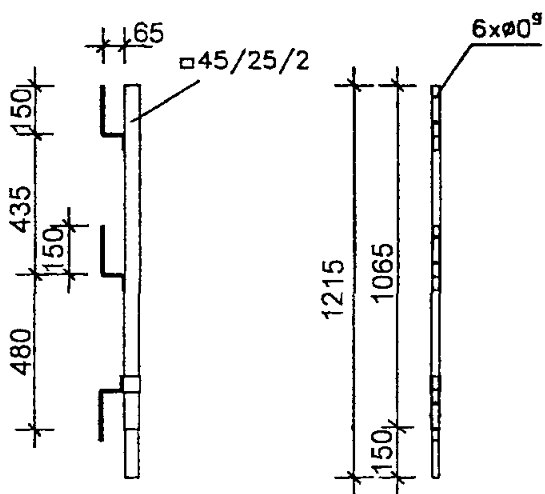
Рисунок 15 – Конструкция консоли для мостков 125
