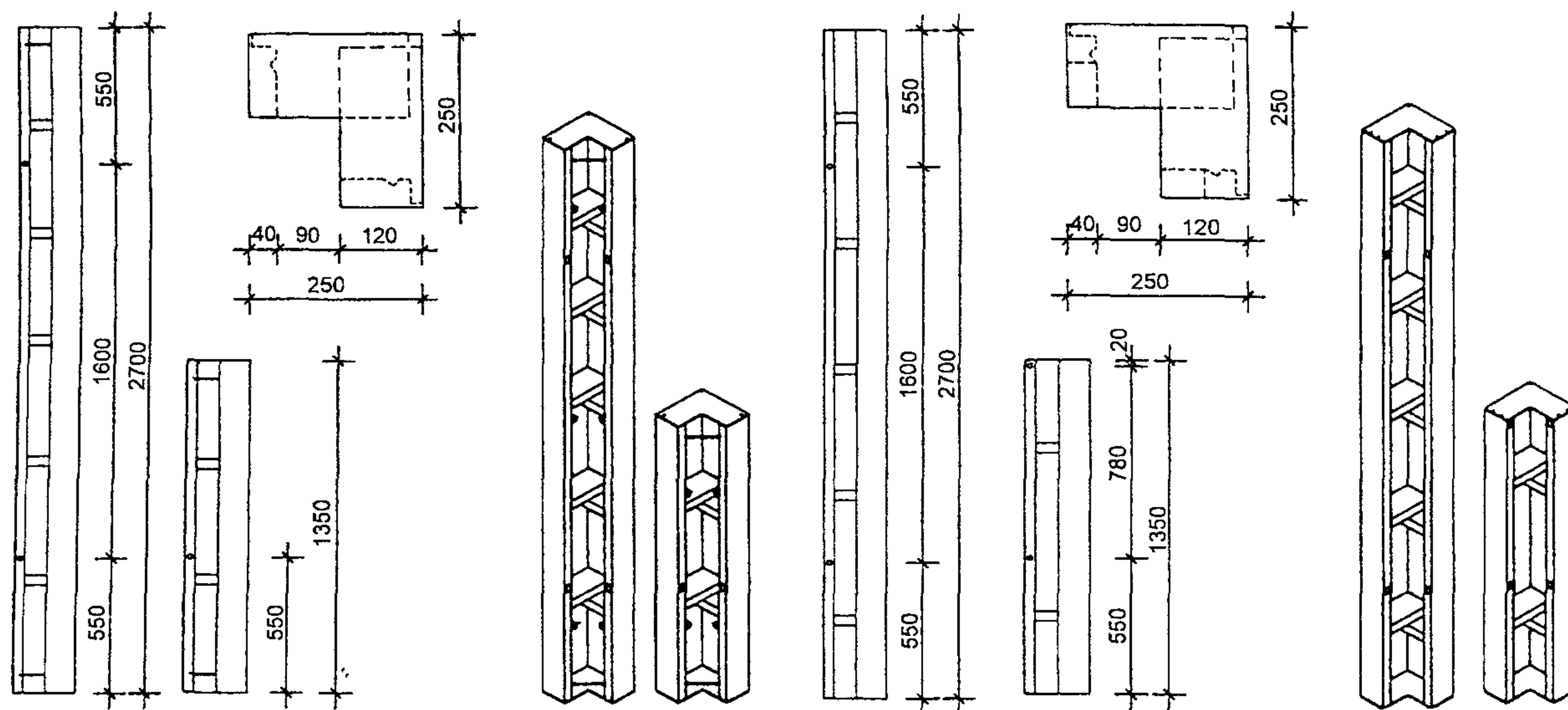
а) Внутренний уголок ST
