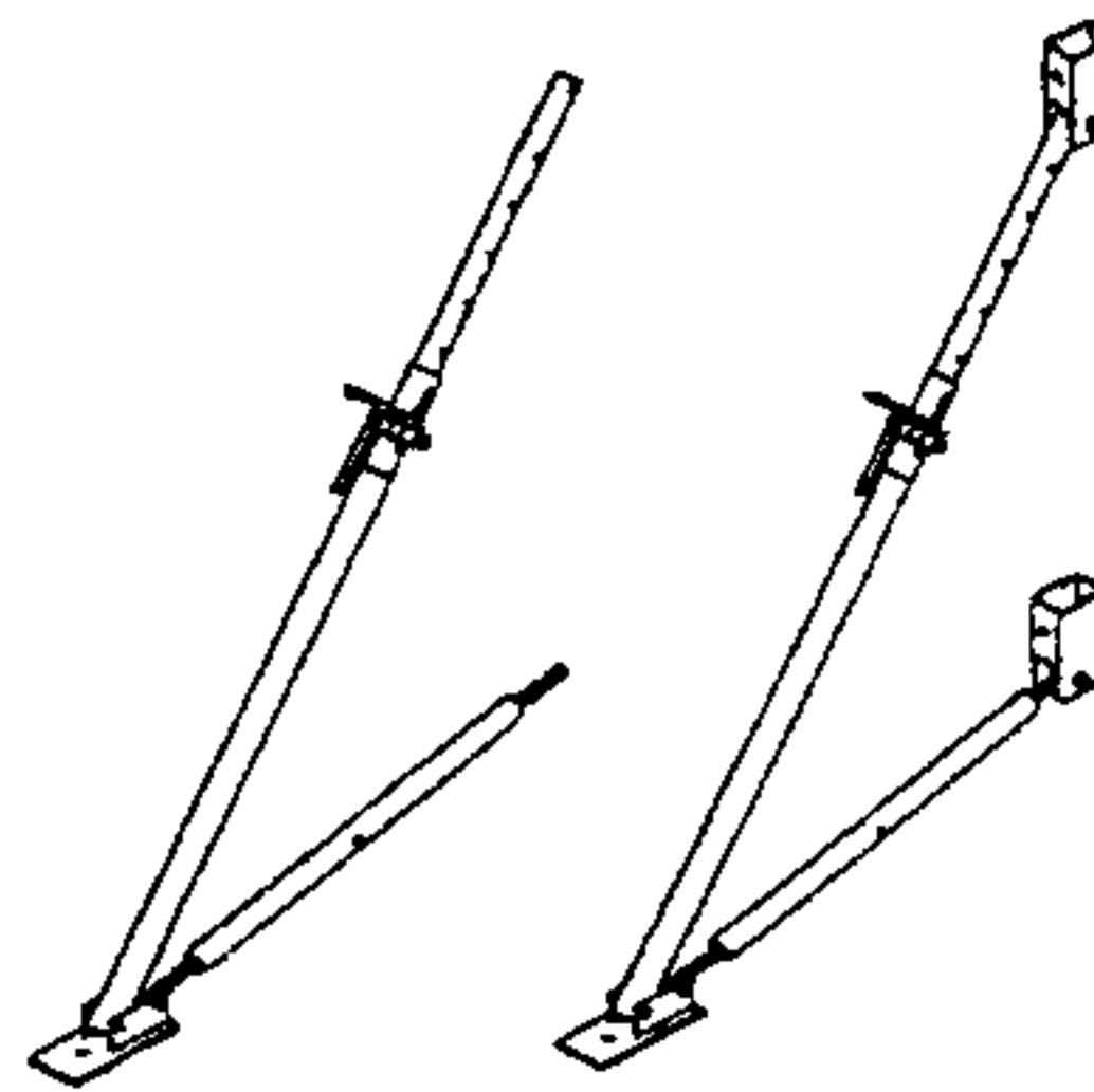
Рисунок 17 – Консольная подпорка
