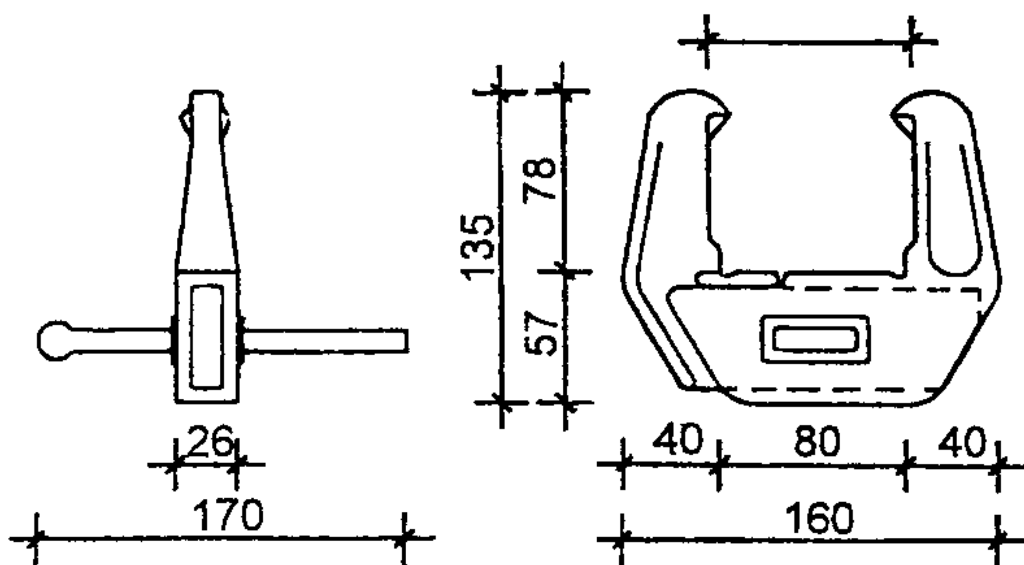
Рисунок 7 – Схема соединения элементов опалубки замком
