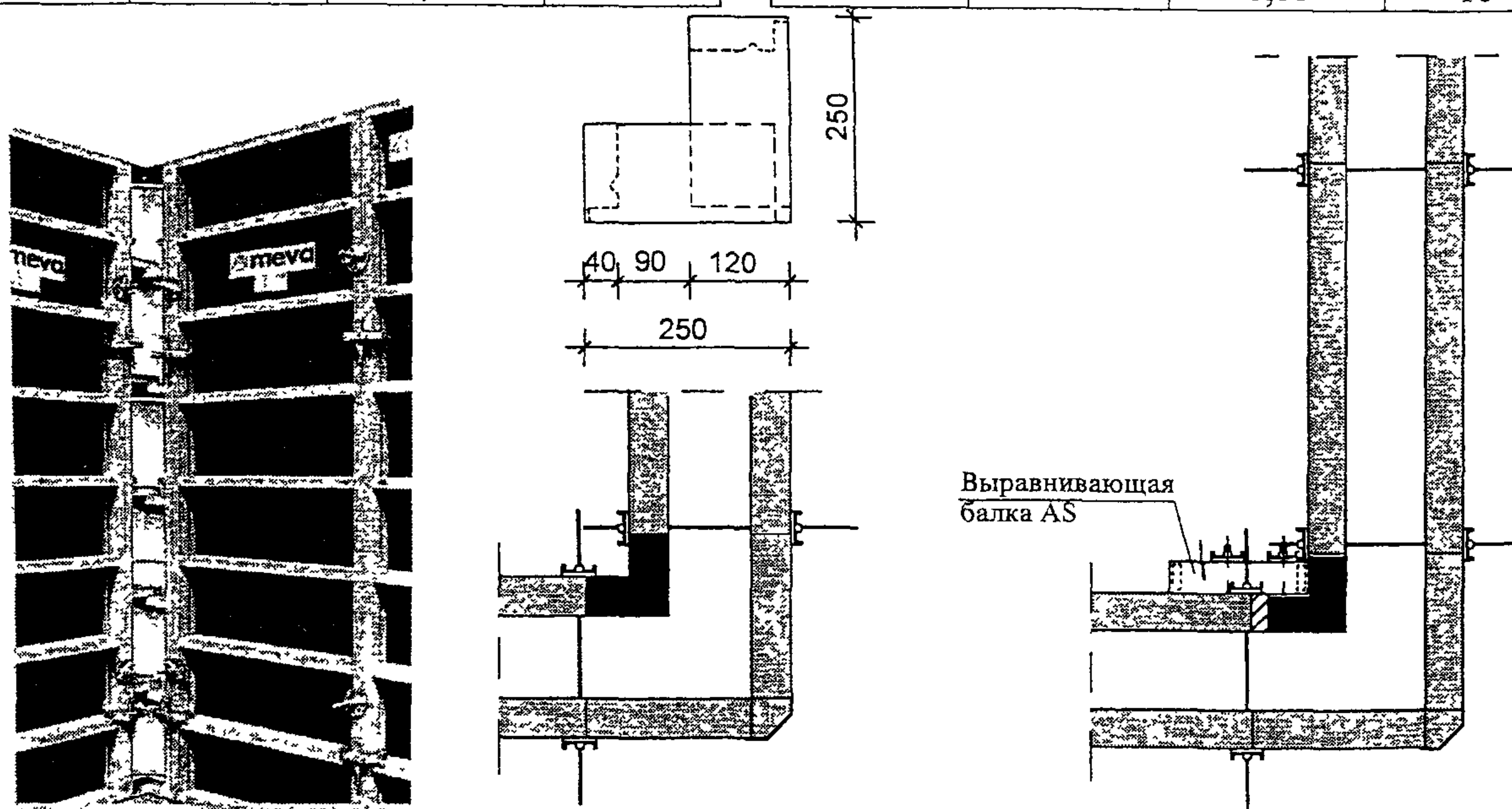
Рисунок 9 – Оснастка внутреннего угла 90° систем «Star Tec» и «Alu Star»
