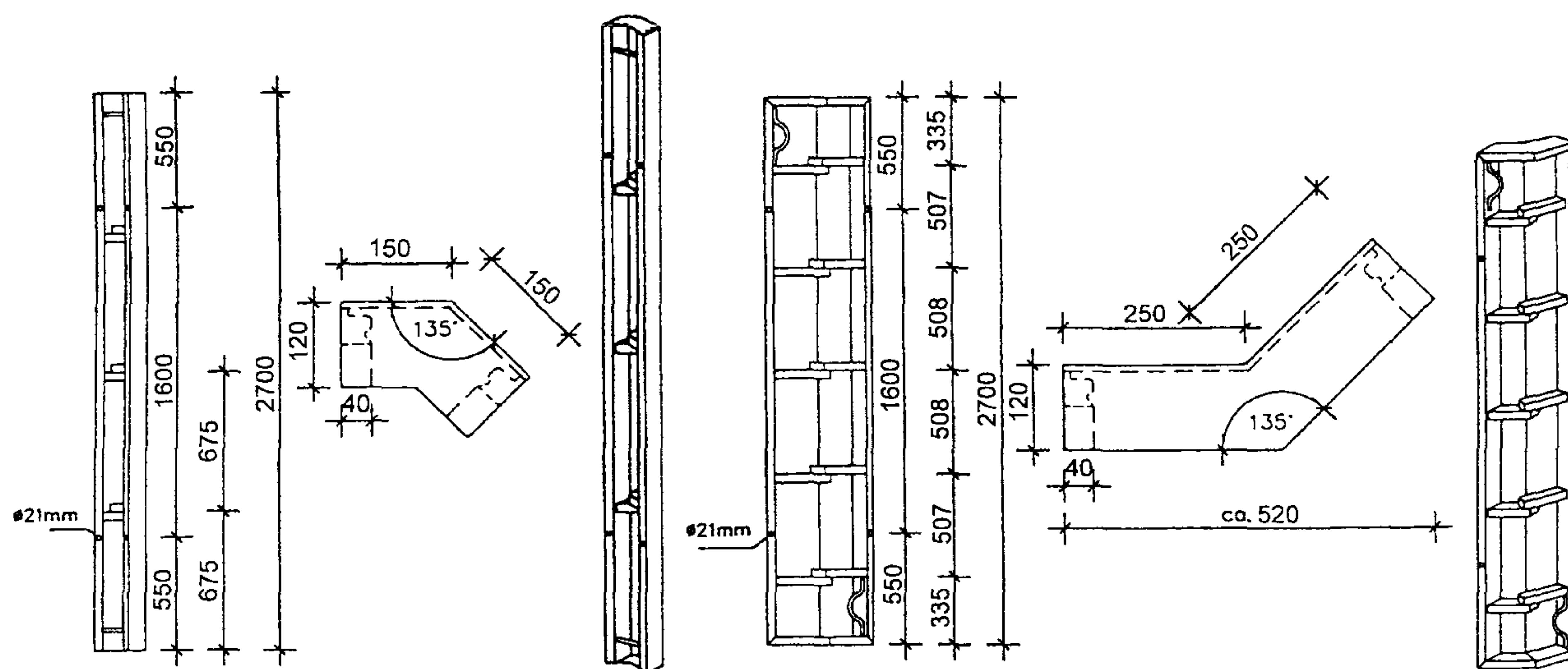
а) Внутренний уголок AS 135°
