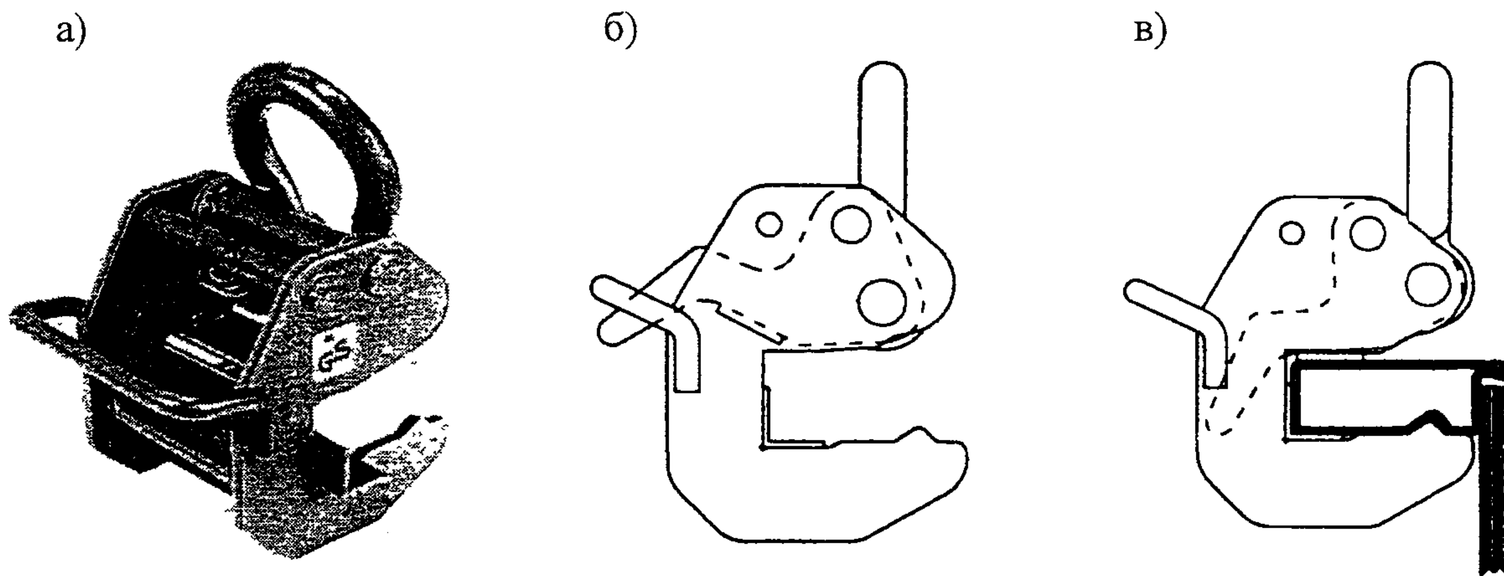
Рисунок 5 – Захватное устройство (крюк крана) для опалубки «Мева»
