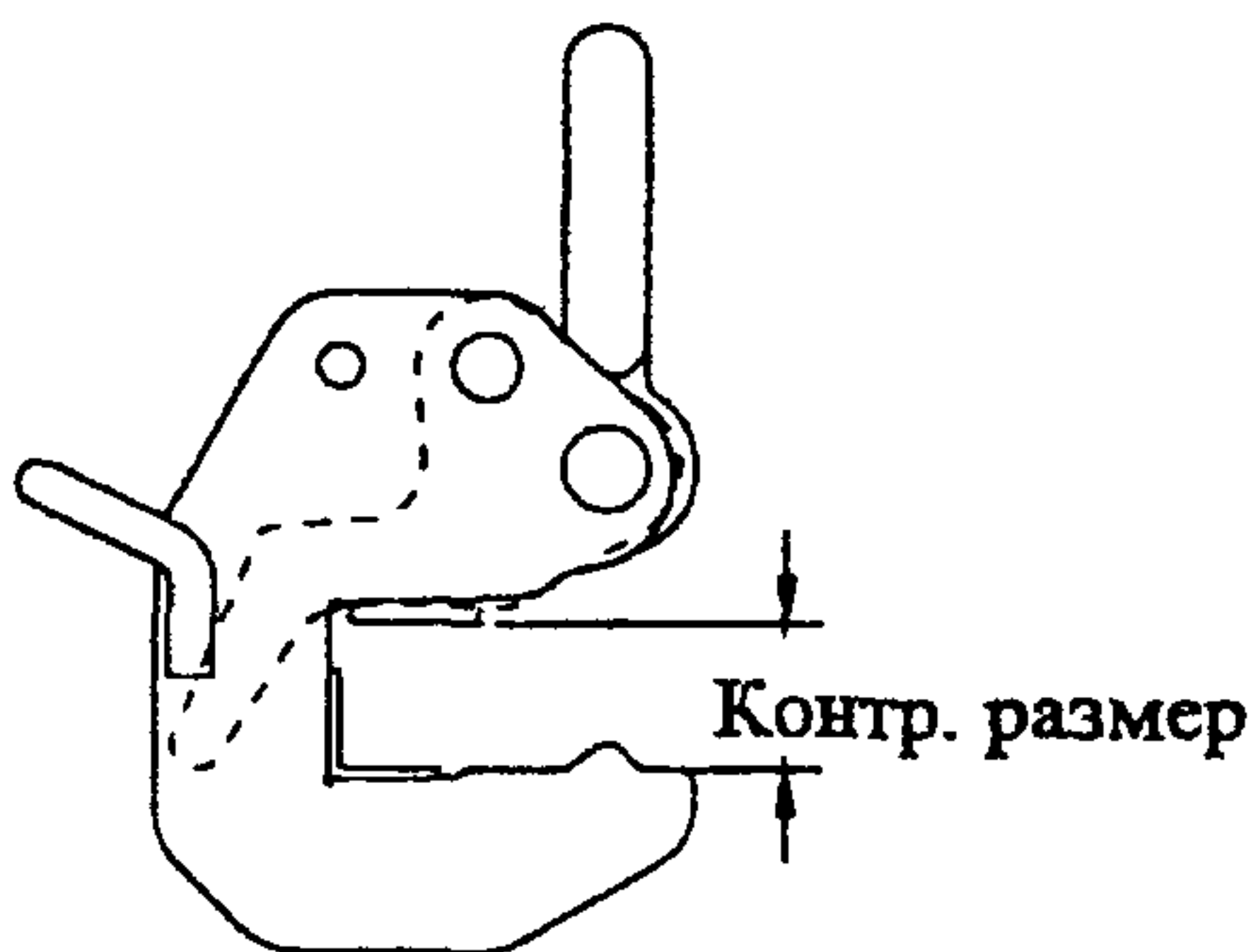
Рисунок 18 – Критерий для выбраковки захватного устройства (крюка крана)
