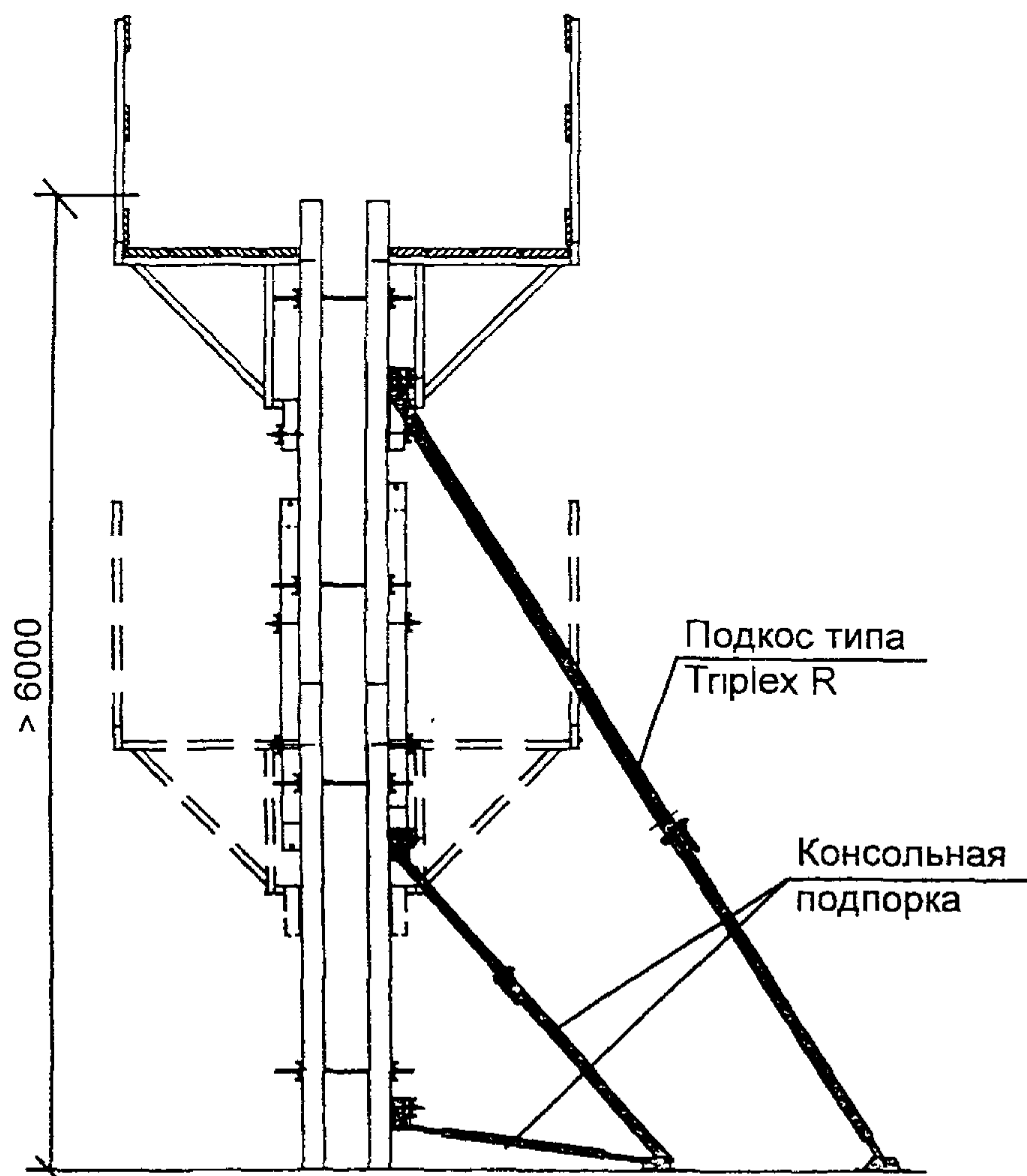
Рисунок 11 – Раскрепление щитов опалубки
