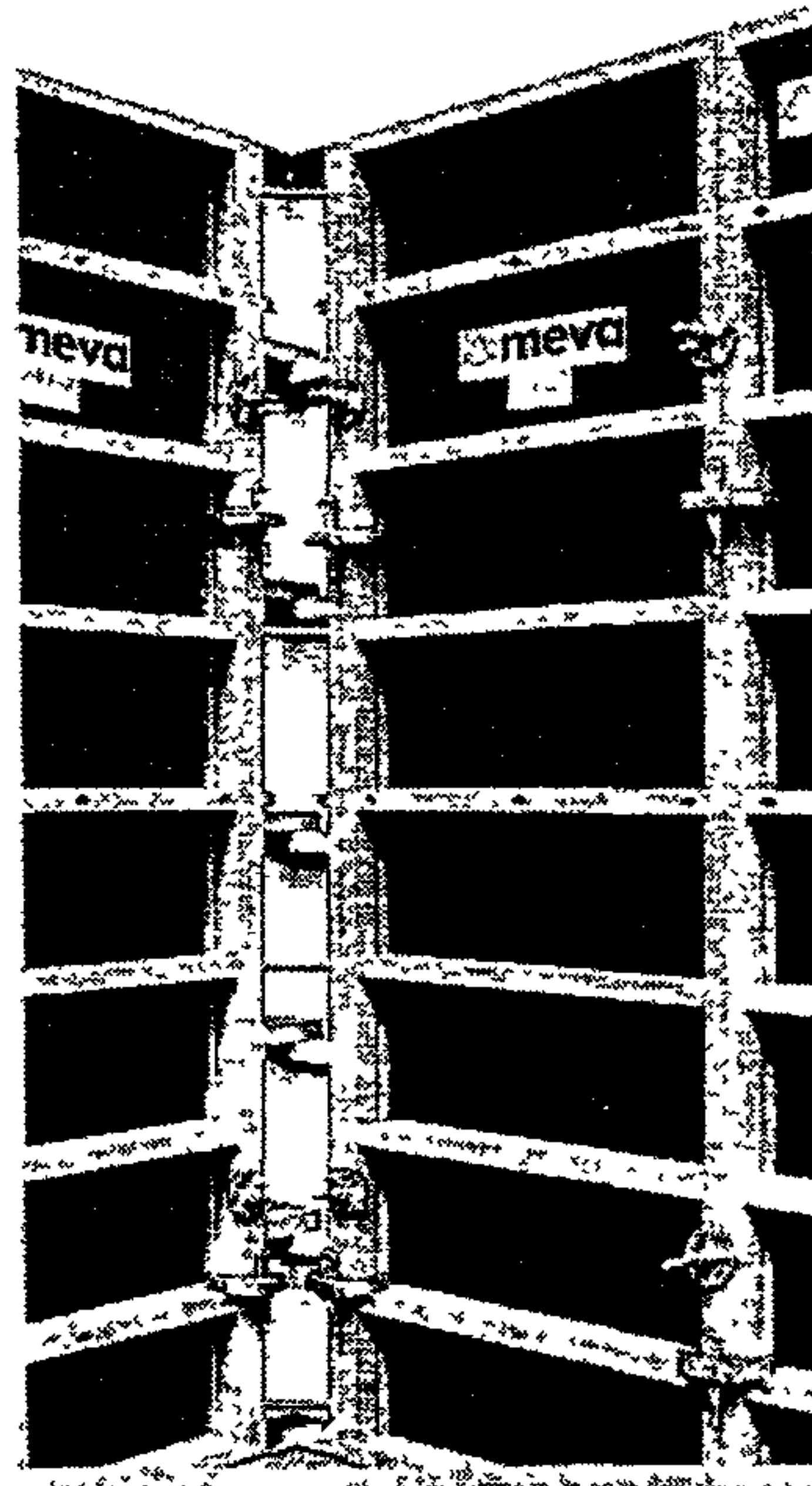
Рисунок 2 – Опалубка системы «Стар Тек»
