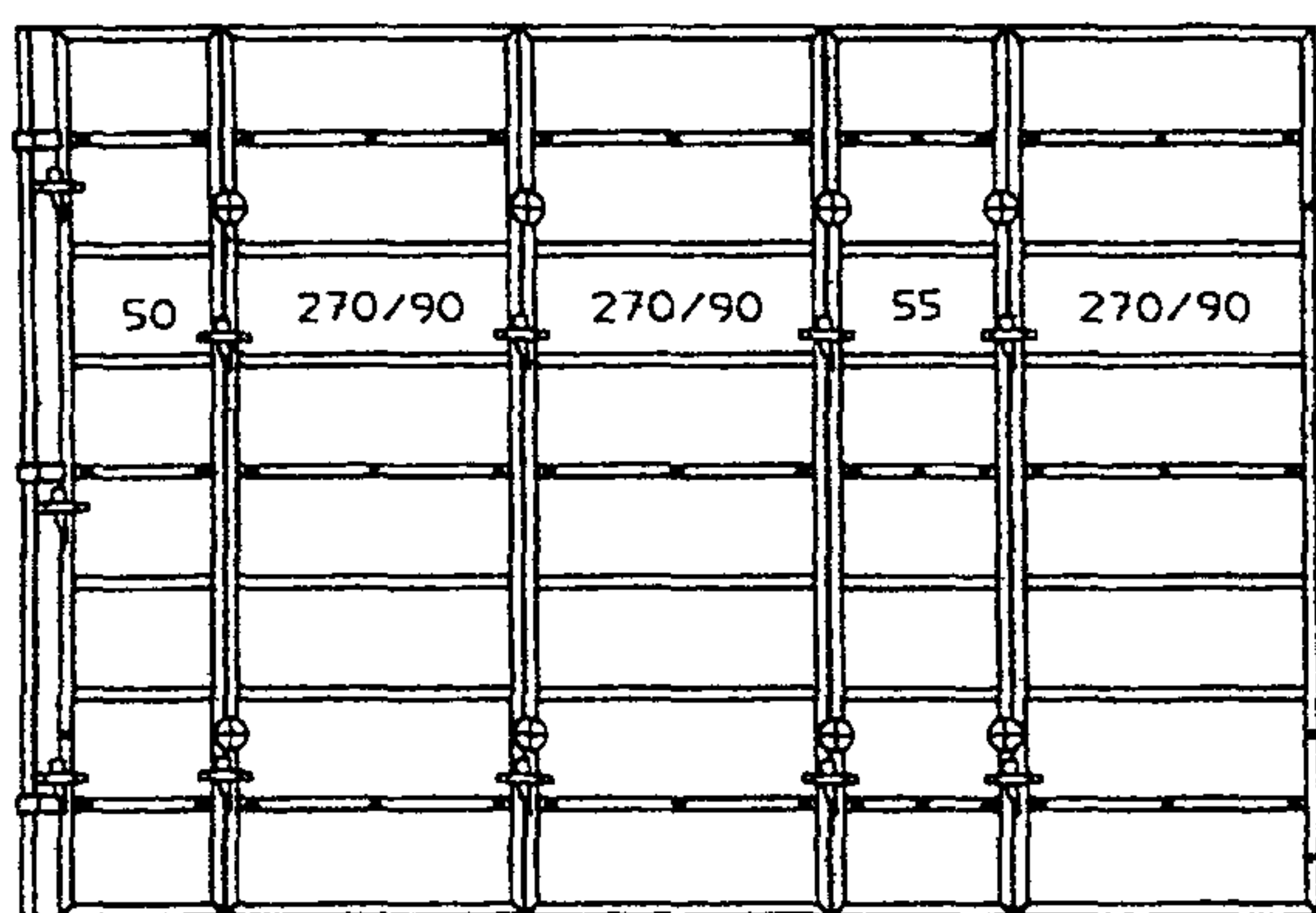
Рисунок 12 – Соединение элементов опалубки
