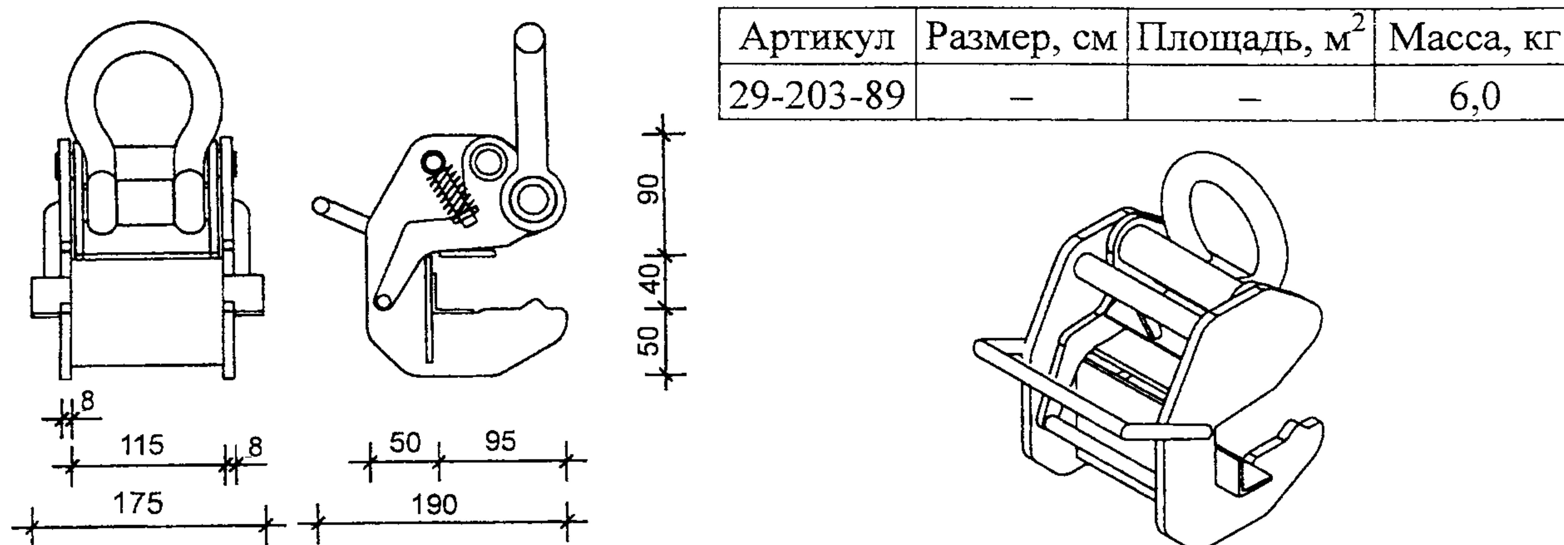
Рисунок 4 – Конструкция захватного устройства (крюка крана AS)
