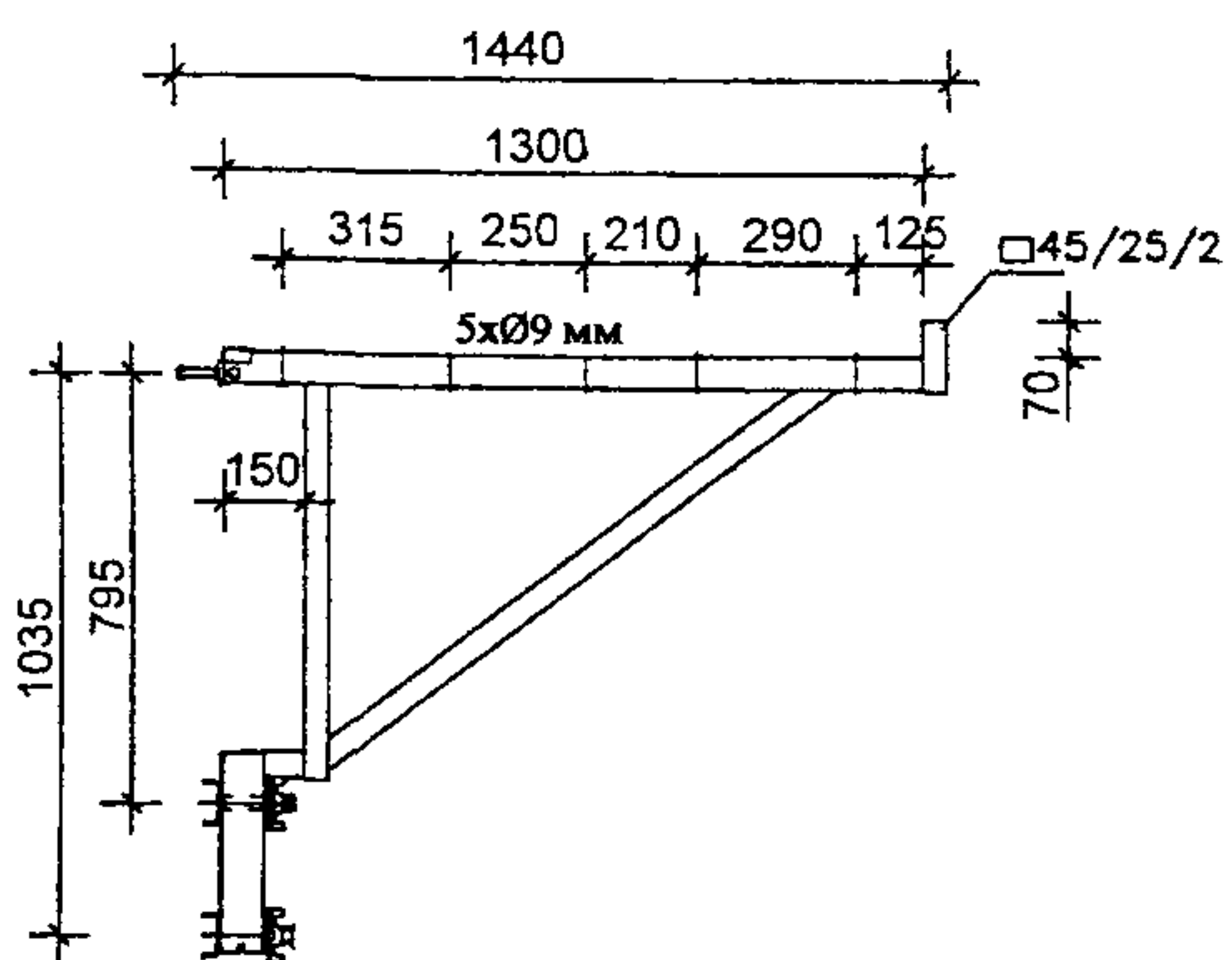
Рисунок 15 – Конструкция консоли для мостков 125
