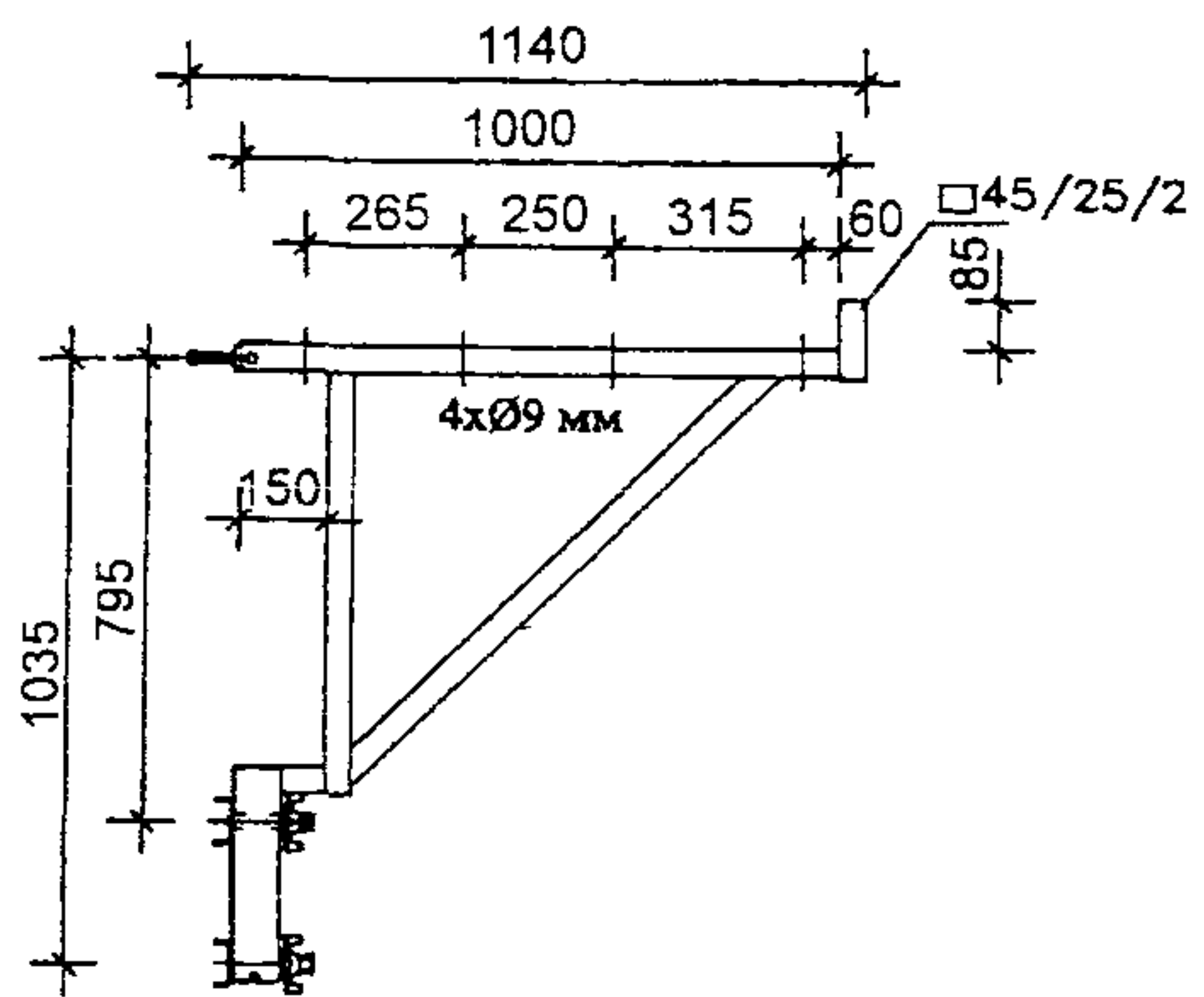
Рисунок 14 – Конструкция консоли для мостков 90
