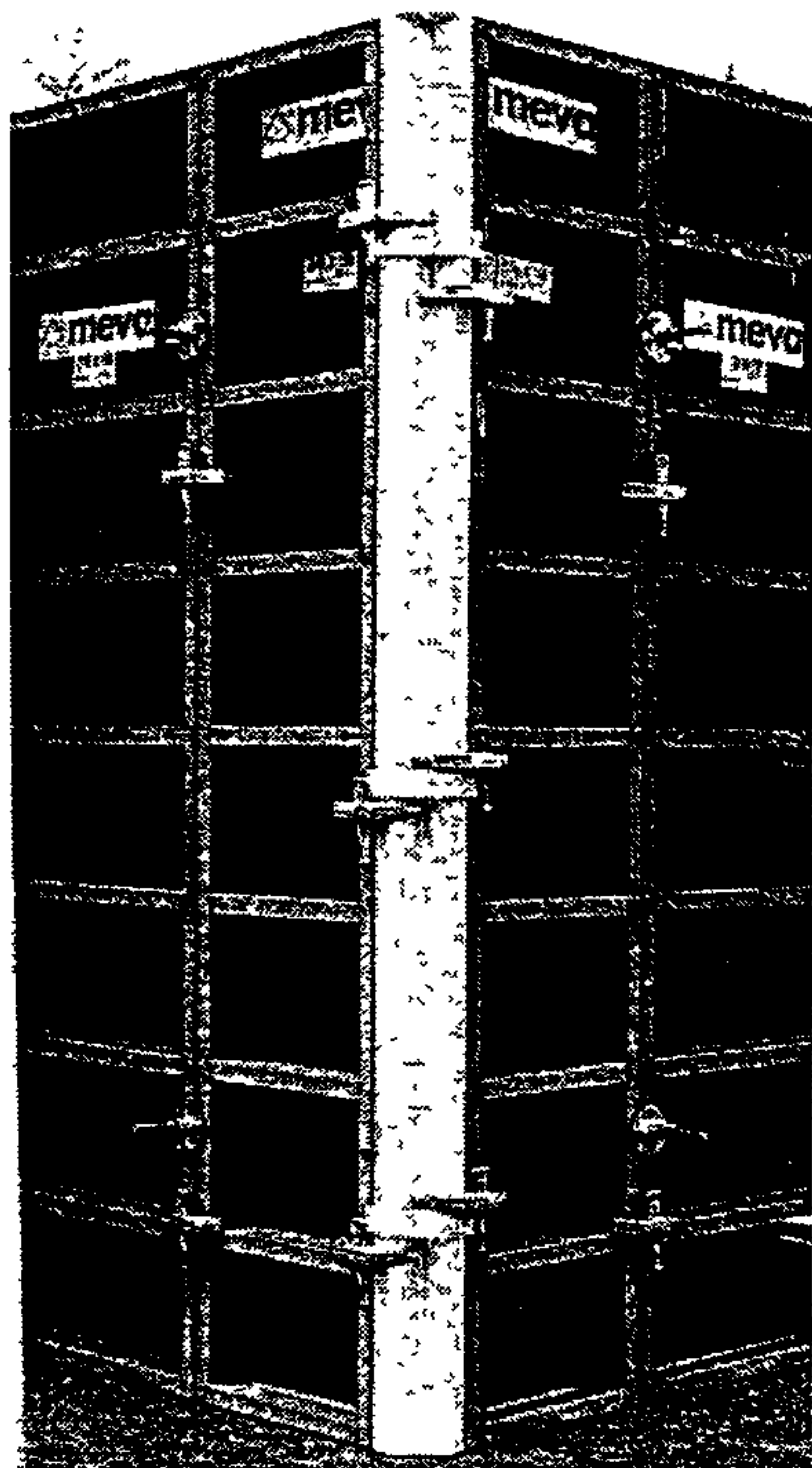
Рисунок 1 – Опалубка системы «Alu Star»
